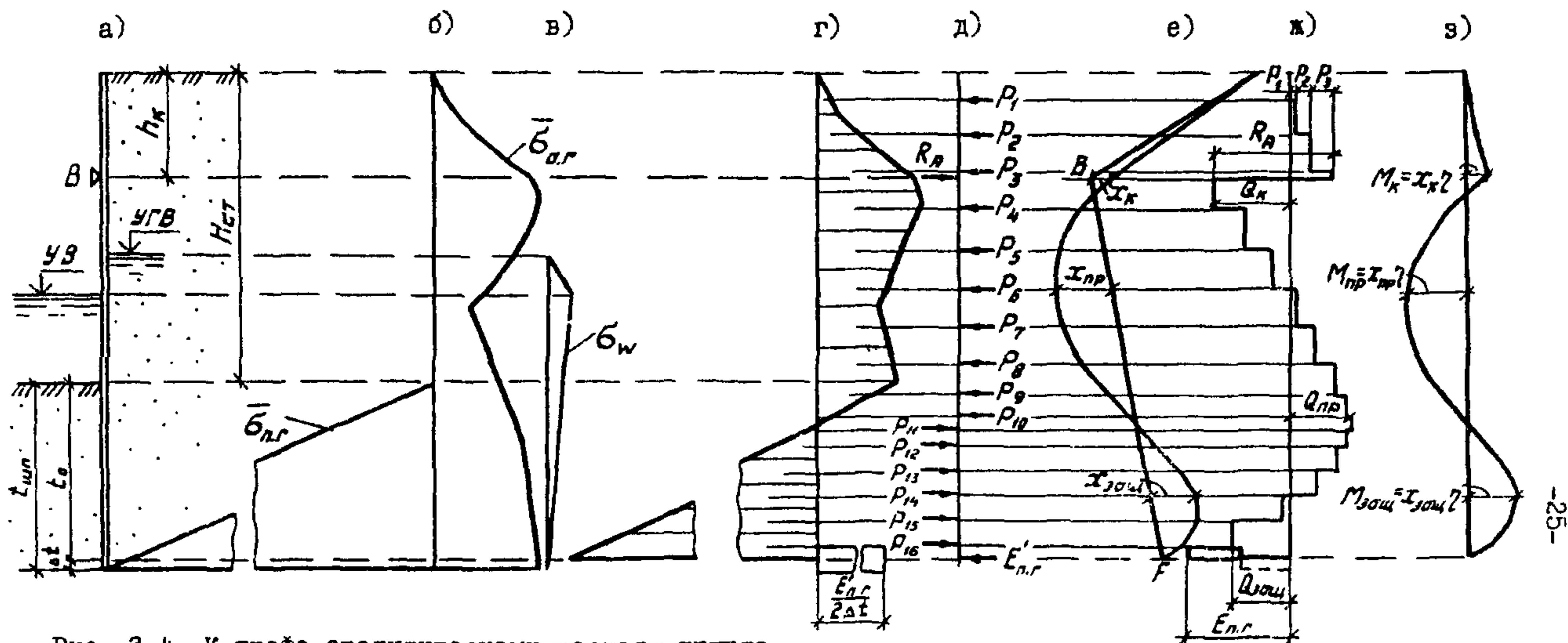
Рис. 3.4. К графо-аналитическому расчету шпунта
