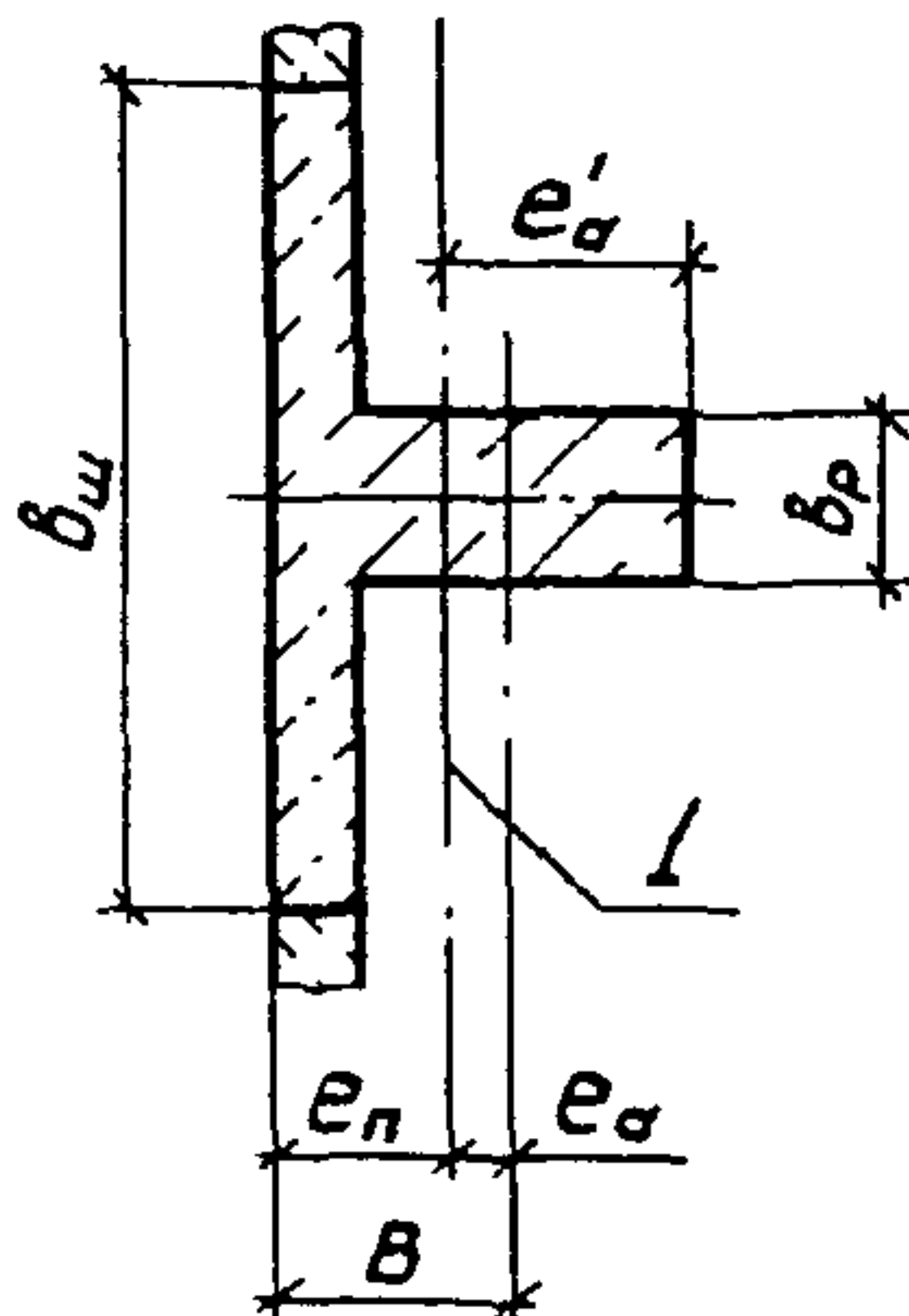
Рис. 2.3. К определению приведенной высоты сечения железобетонных шпунтов
