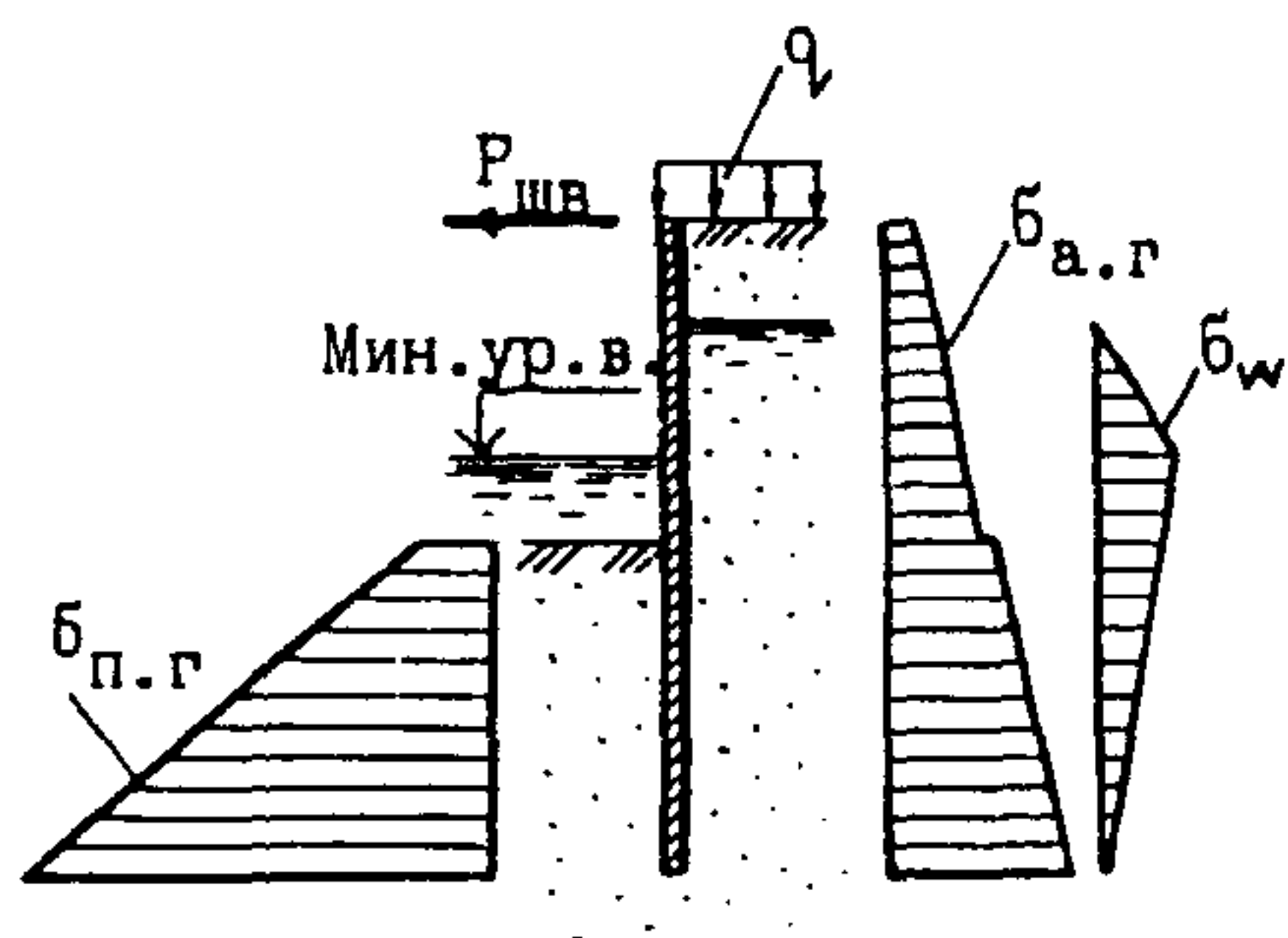
Сочетание 4 (для t_{шп} и M < 0 )
