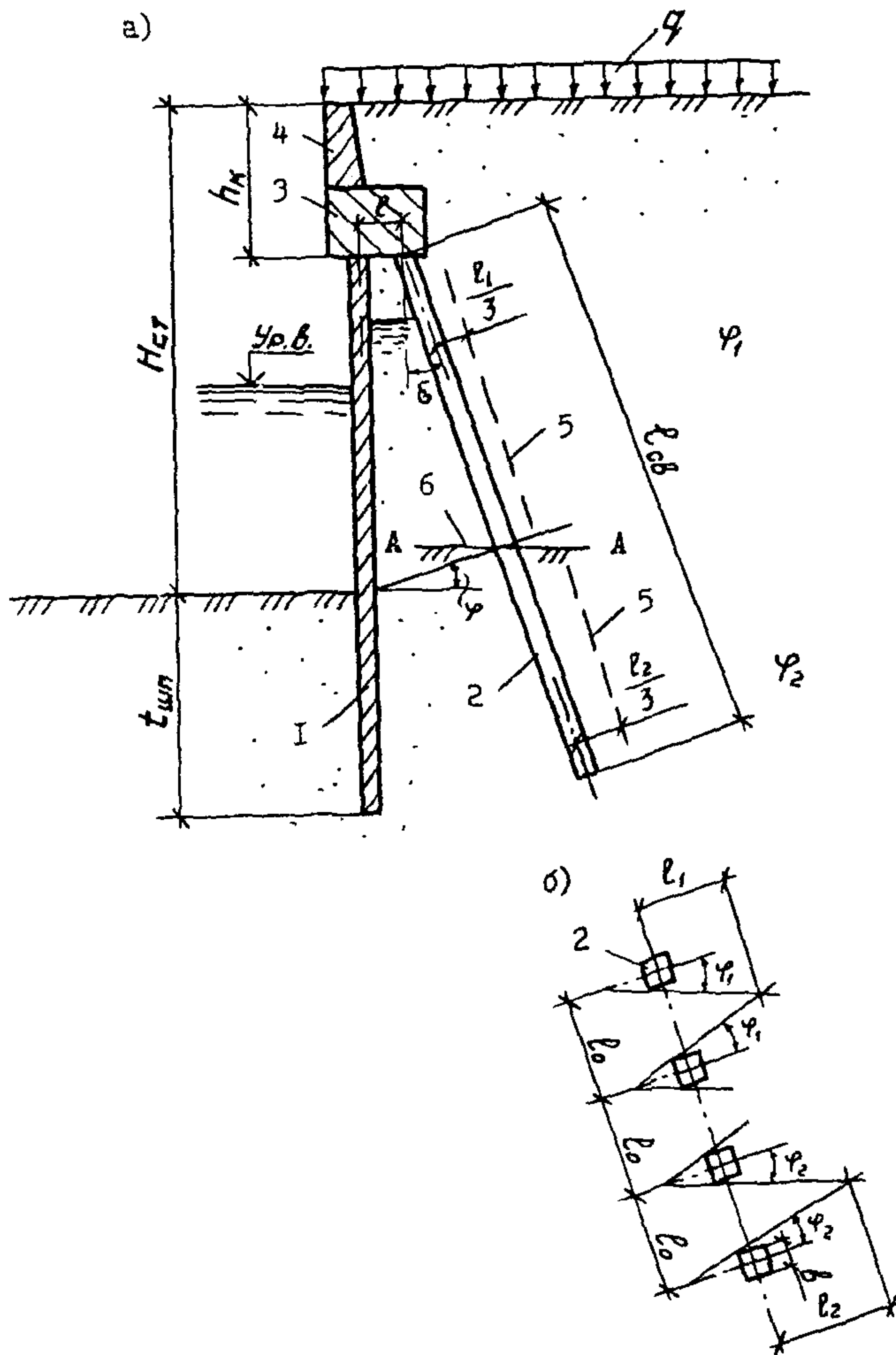
Рис. 5.1. К расчету шпунтовой набережной, заанкеренной наклонными сваями
