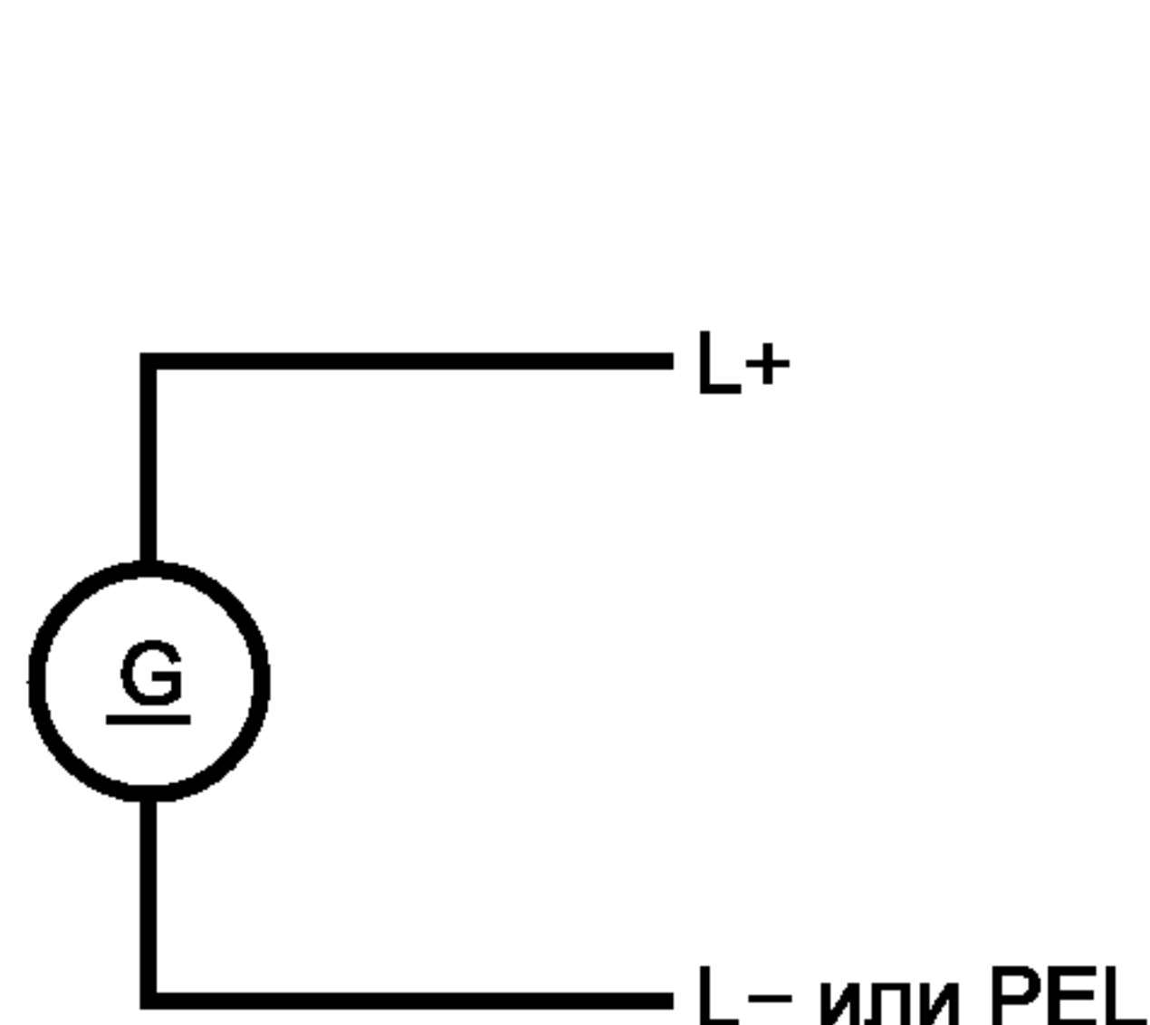
Рисунок 6 — Двухпроводная система
