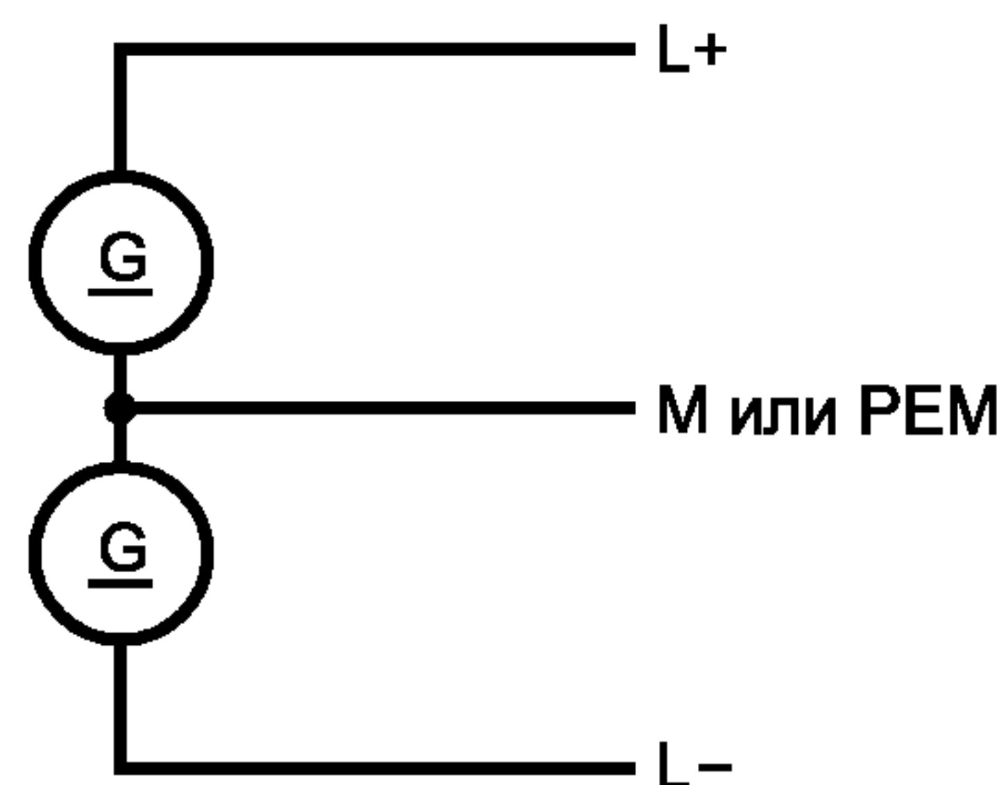
Рисунок 7 — Трехпроводная система
