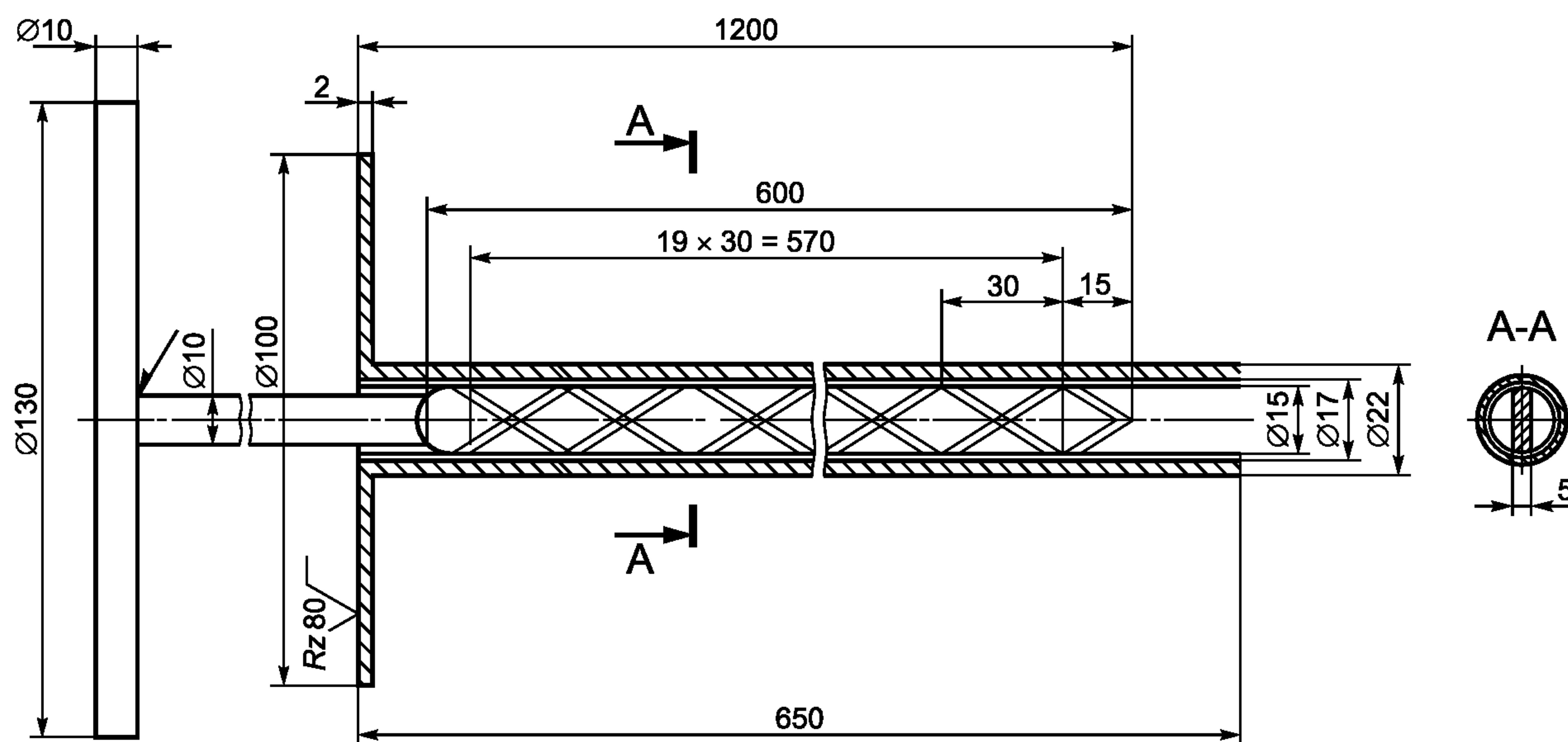
Рисунок 1 — Щуп для отбора проб
