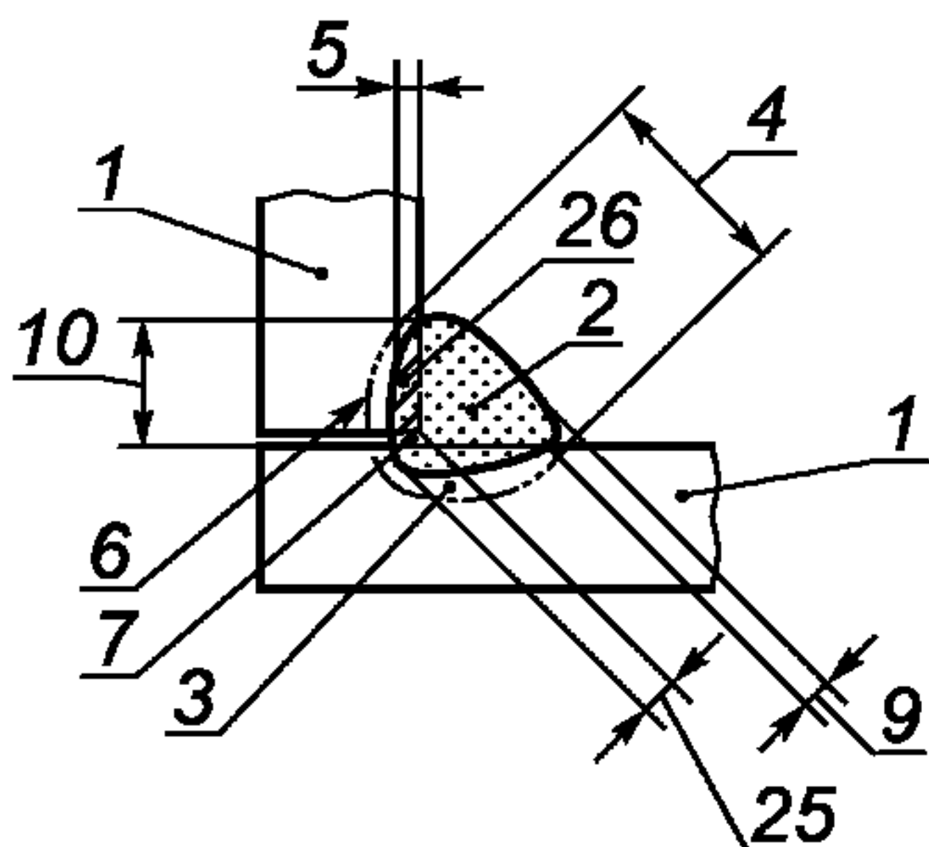
б) угловой шов Fillet weld Soudure d'angle
