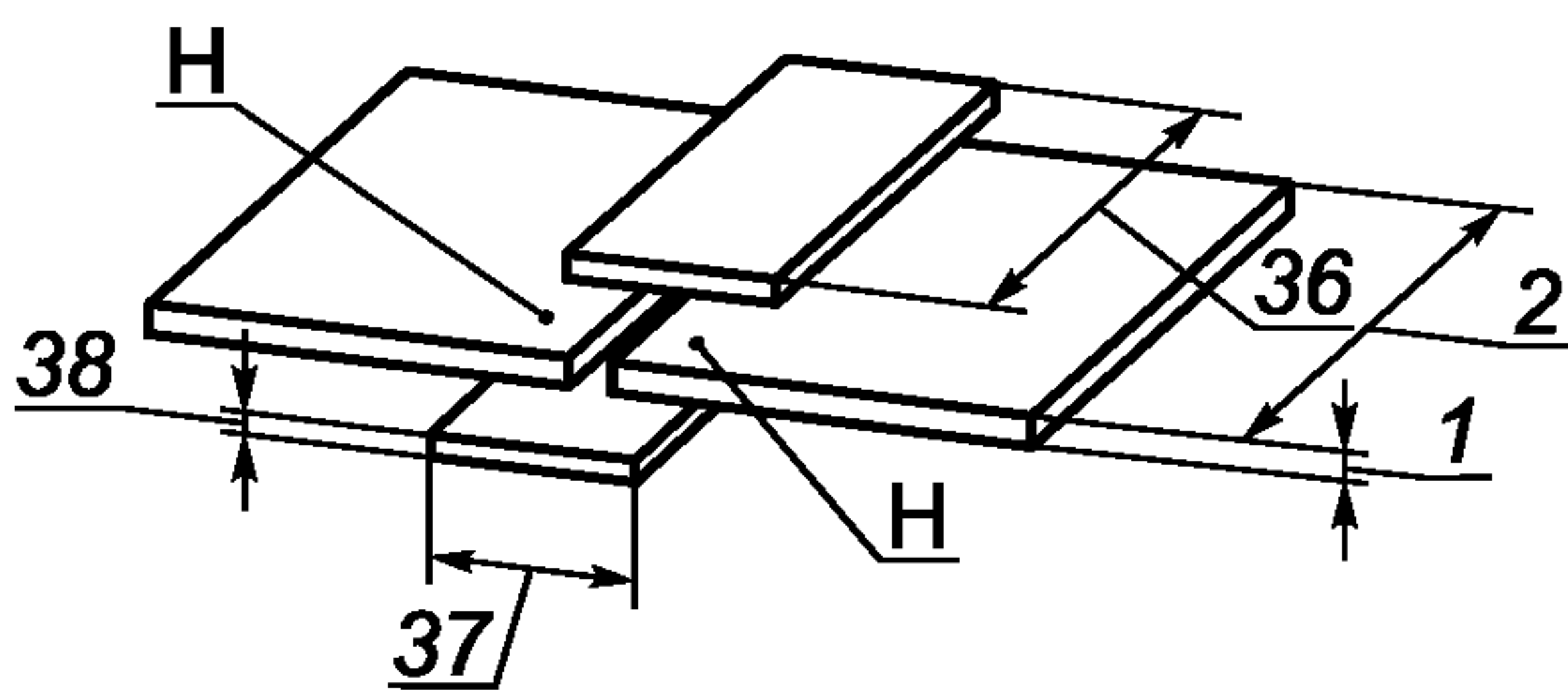
Рисунок 11 — Сборка под шовную контактную стыковую сварку по фольге Figure 11 — Configuration for foil-seam-welds Figure 11 — Configuration pour soudure à la molette avec feuillard d'apport
