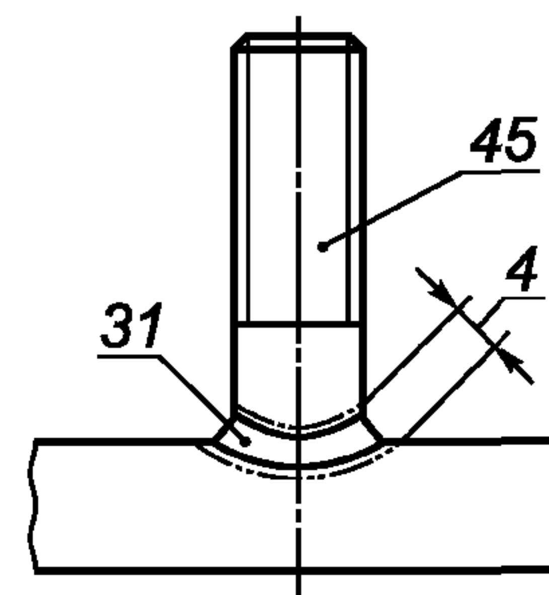
c) шов при приварке шпильки Arc stud weld Soudure de goujon
