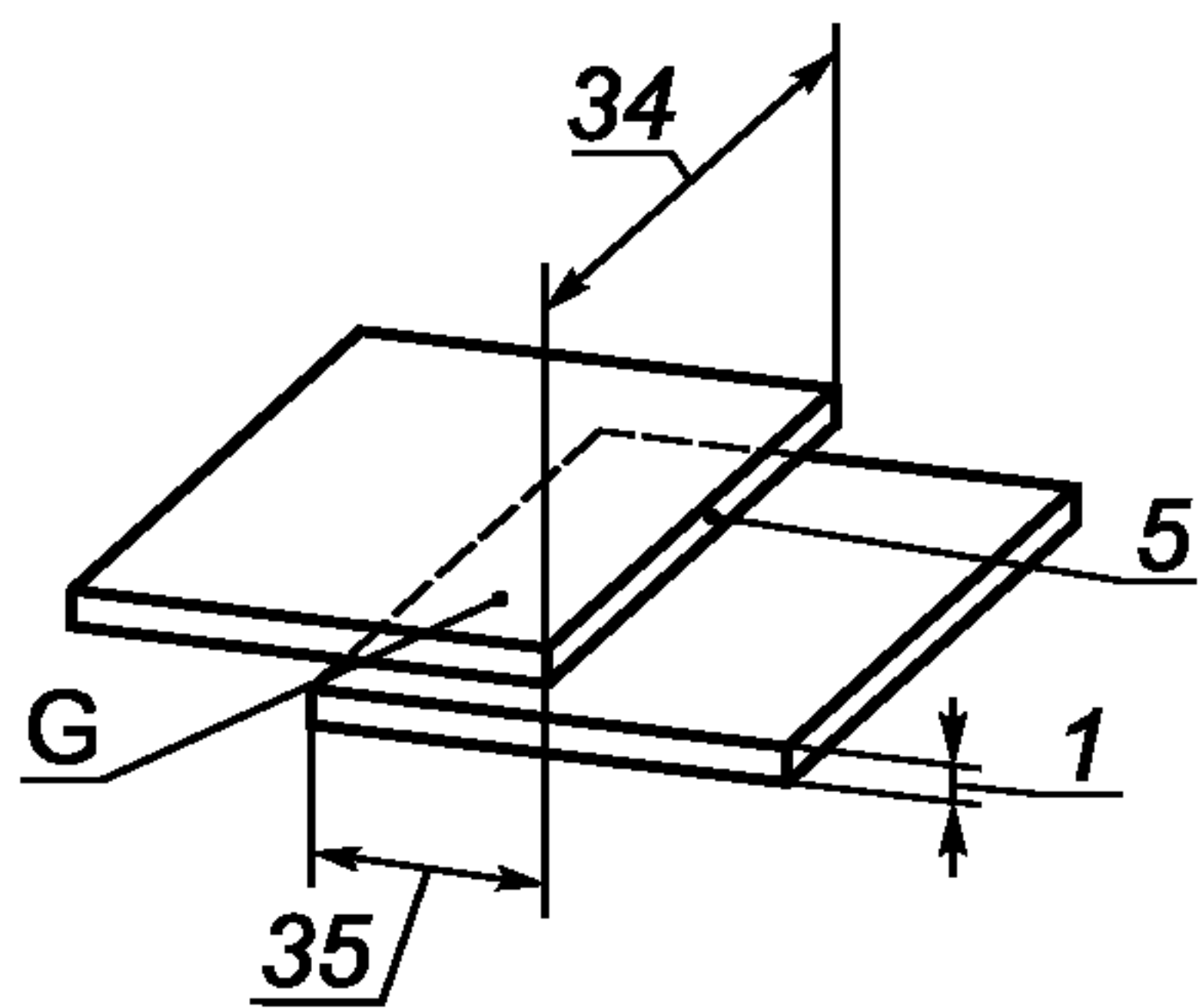
Рисунок 10 — Сборка под контактную точечную и шовную сварки с раздавливанием кромок Figure 10 — Configuration for spot, seam or mash welds Figure 10 — Configuration pour soudure par points, à la molette ou par écrasement
