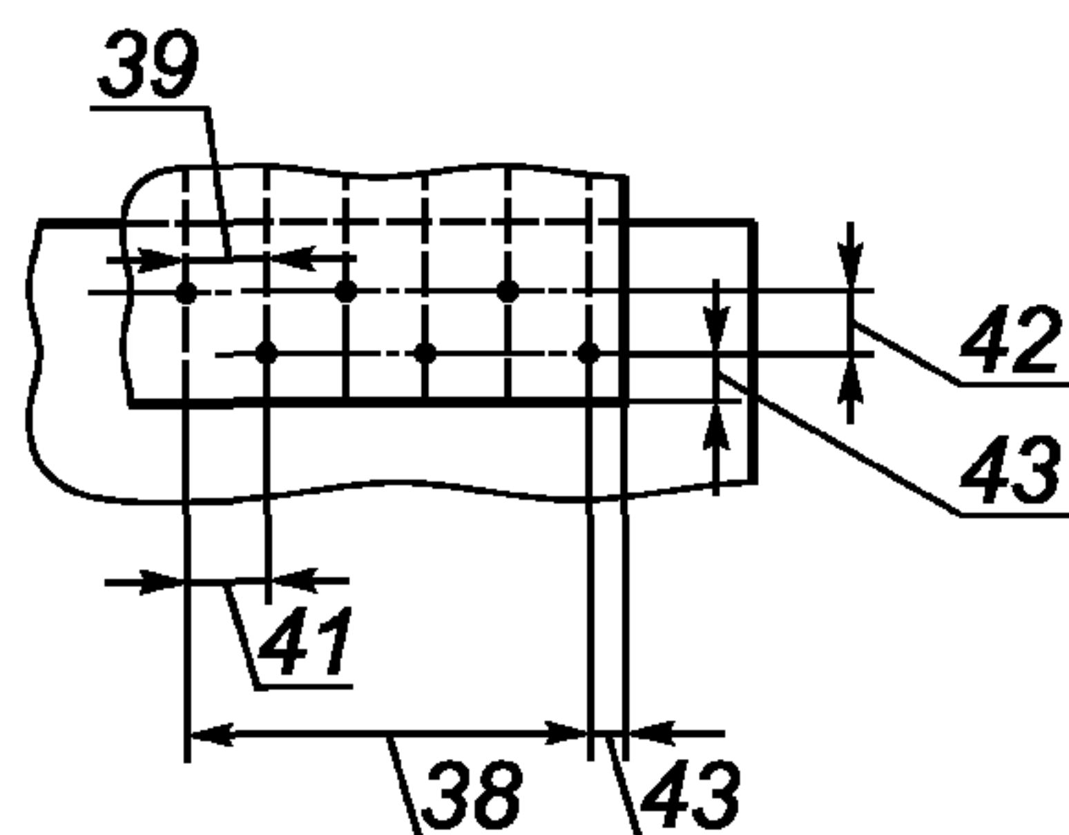
f) двойной ряд сварных точек, расположенных в шахматном порядке Double row of staggered, spaced spot welds Double rangée de soudures par points en quinconce
