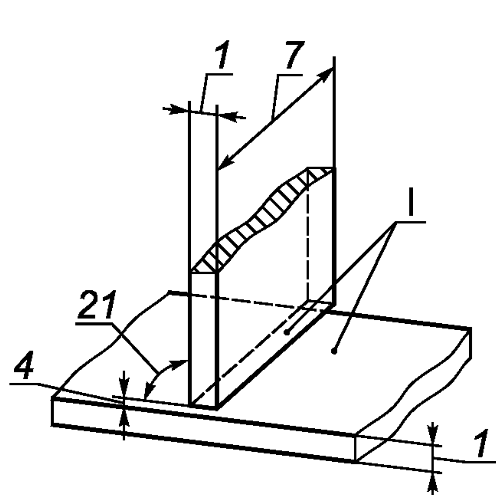
Рисунок 6 — Подготовка под сварку таврового соединения Figure 6 — Preparation for fillet weld (T-joint) Figure 6 — Préparation pour soudures d’angle sur assemblage en T
