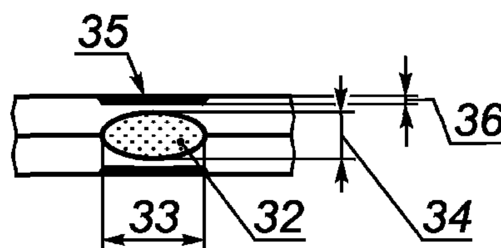
g) шов при точечной контактной сварке Resistance spot weld Soudure par résistance points
