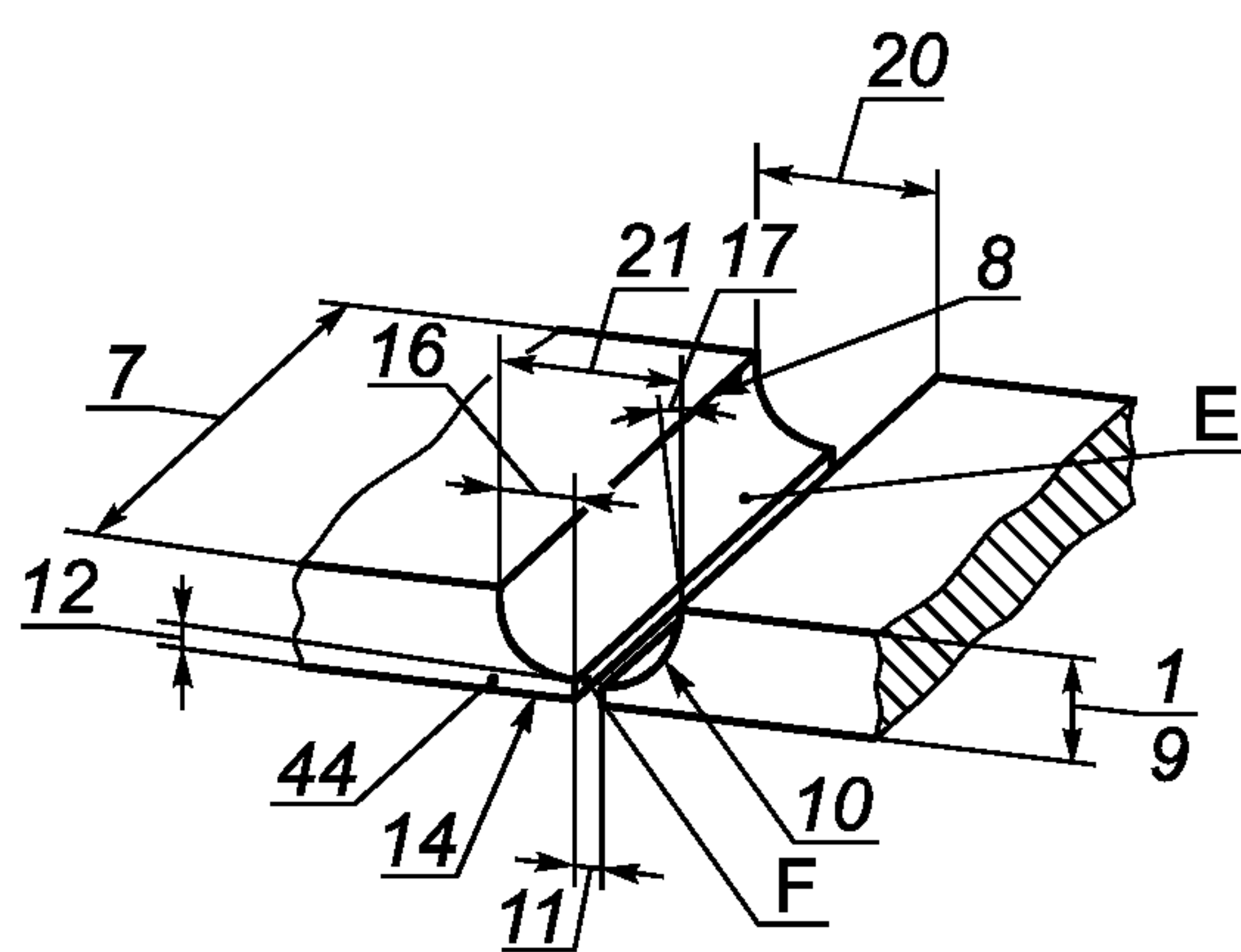
Рисунок 5 — Подготовка под сварку стыкового соединения с U-образным скосом кромок
