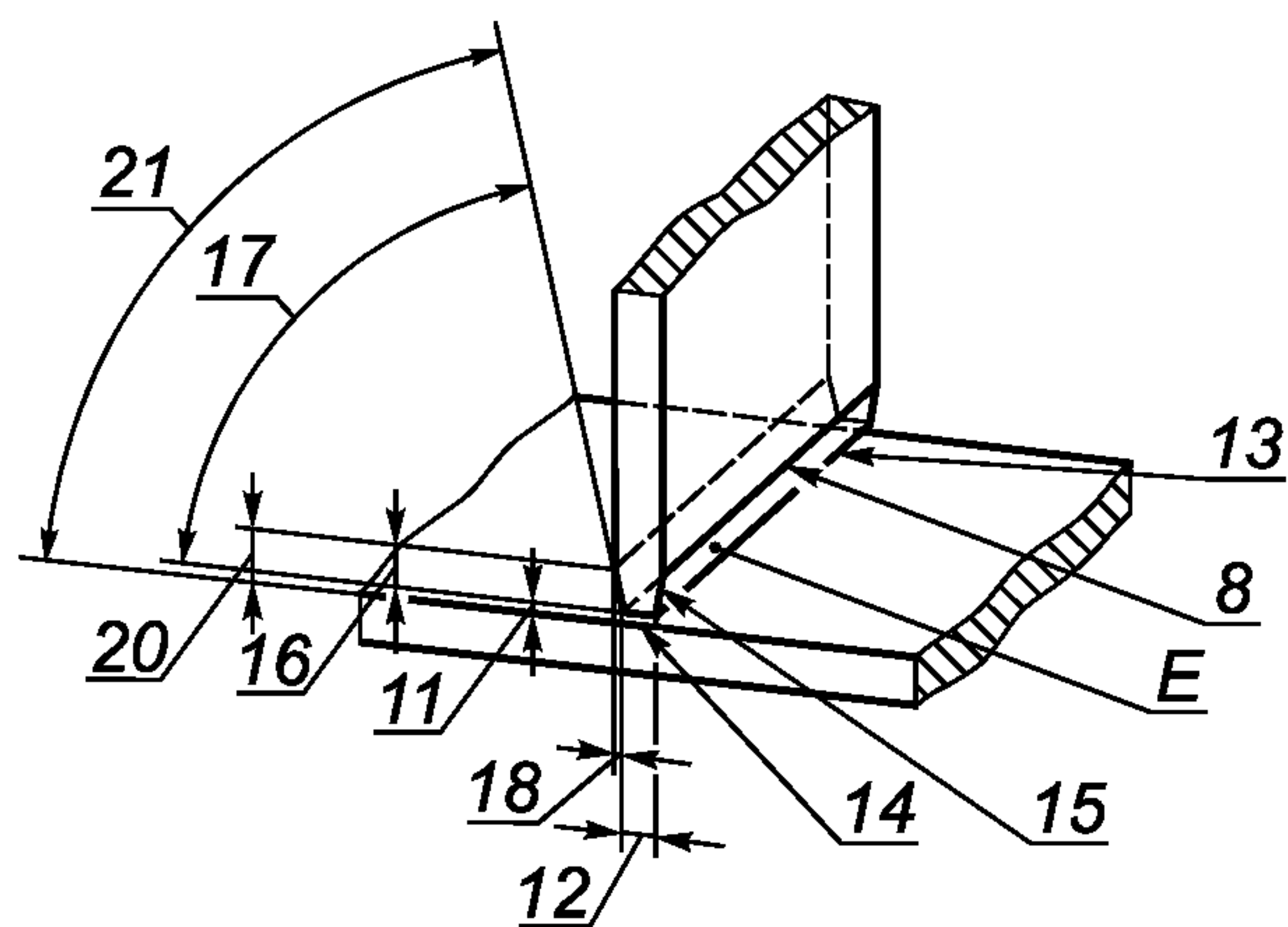
Рисунок 7 — Подготовка под сварку таврового соединения с двусторонним скосом кромки Figure 7 — Preparation for double-bevel T-butt welds Figure 7 — Préparation pour soudures d’angle sur assemblage en T avec double chanfrein
