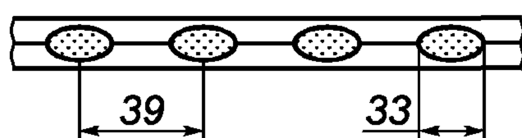
d) шов при точечной контактной сварке Spot welds Soudure par points
