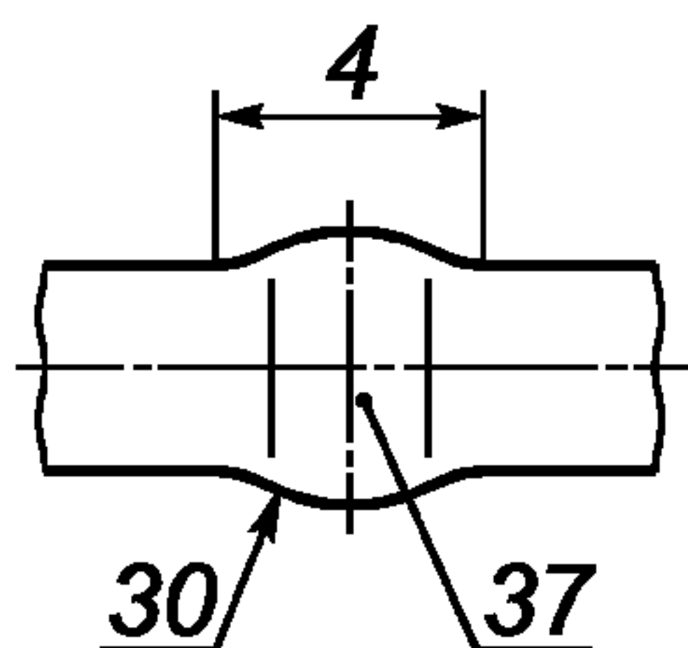
a) шов с гратом при стыковой сварке сопротивлением Butt weld with upset Soudure avec bourrelet de refoulement
