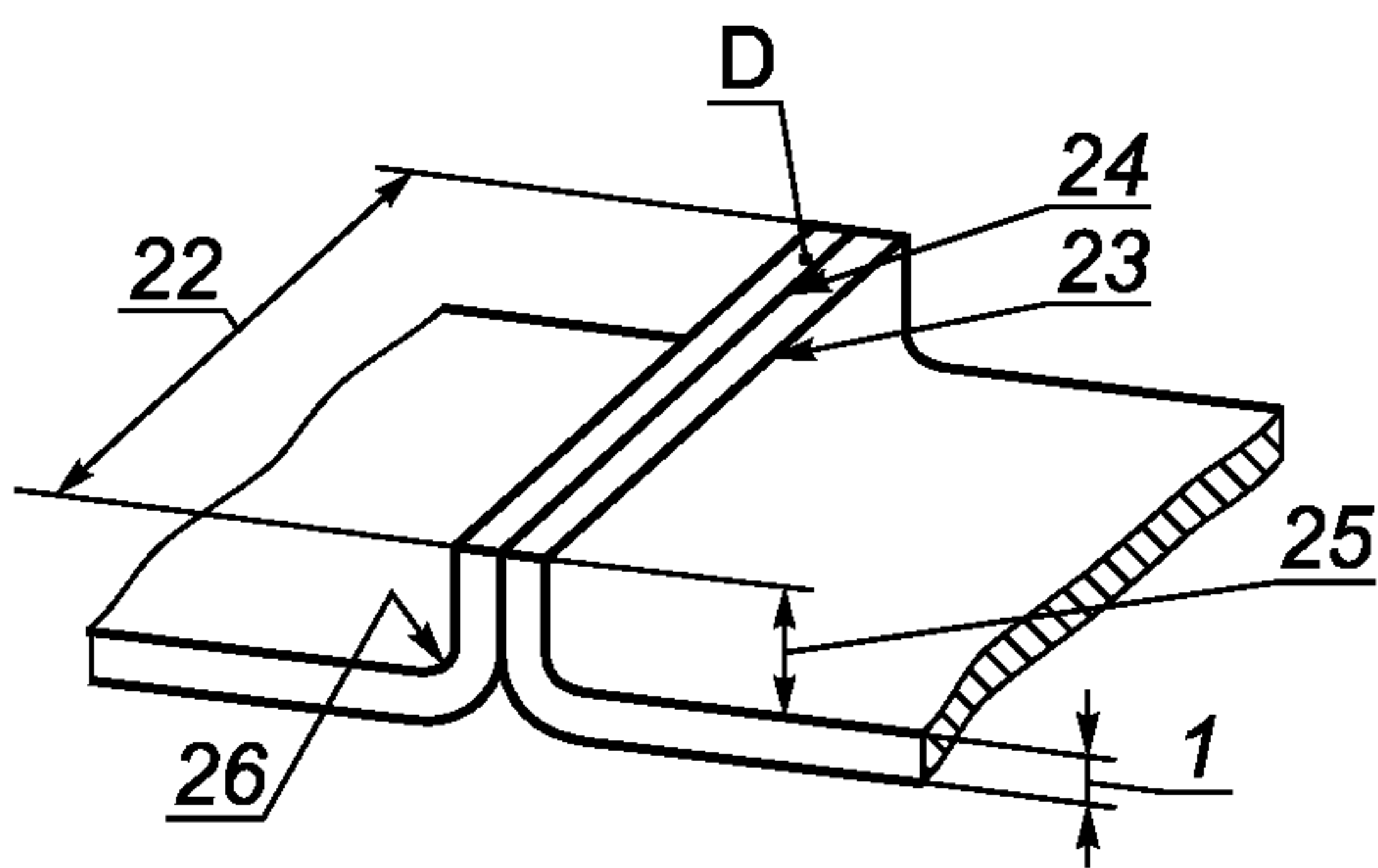
Рисунок 8 — Подготовка под сварку стыкового соединения с отбортовкой кромок Figure 8 — Preparation for butt weld between plates with raised edges Figure 8 — Assemblage à bords relevés
