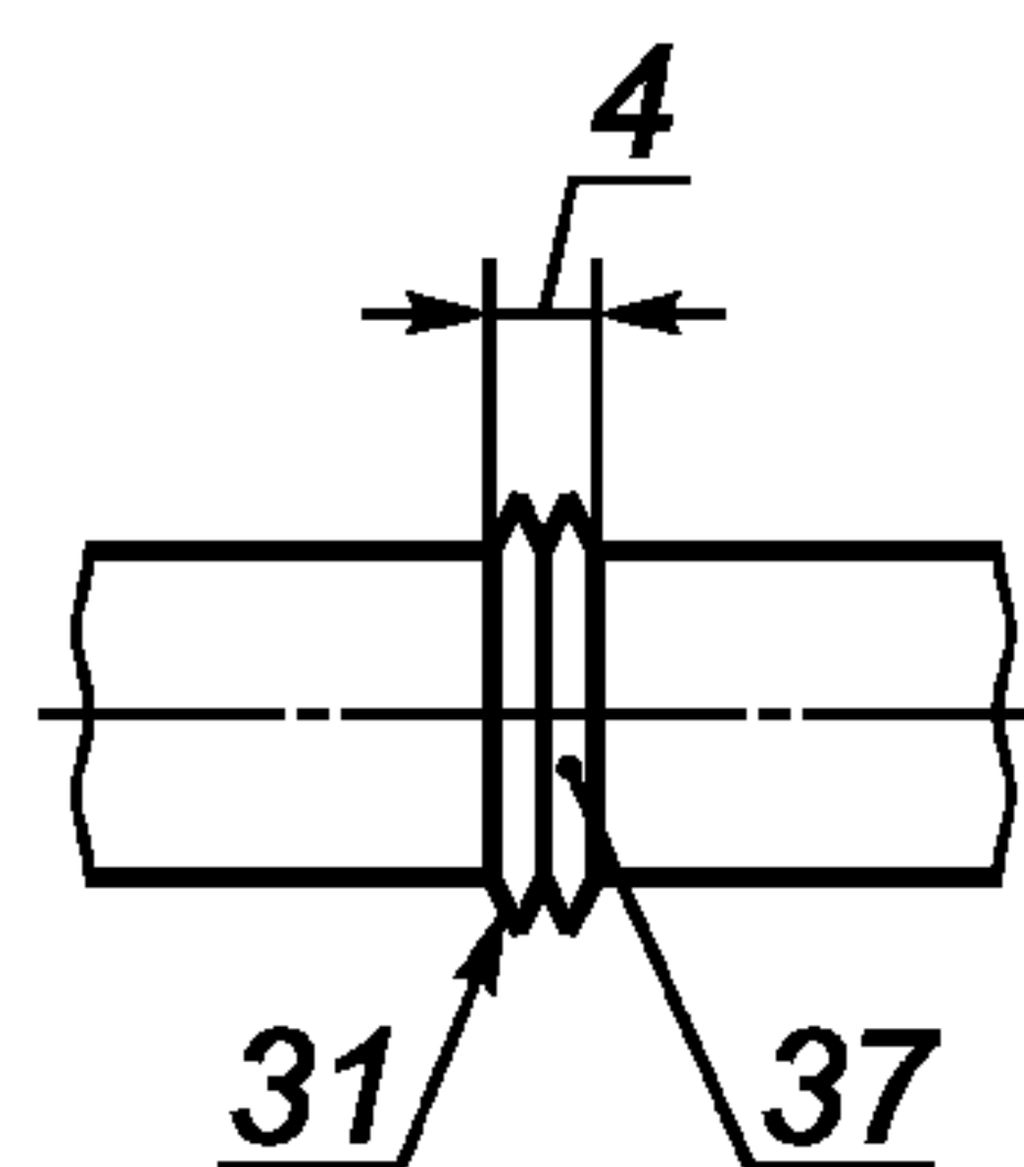
b) шов с гратом при стыковой сварке оплавлением или трением Butt weld with flash (flash or friction) Soudure avec bavure d'étincelage ou de friction
