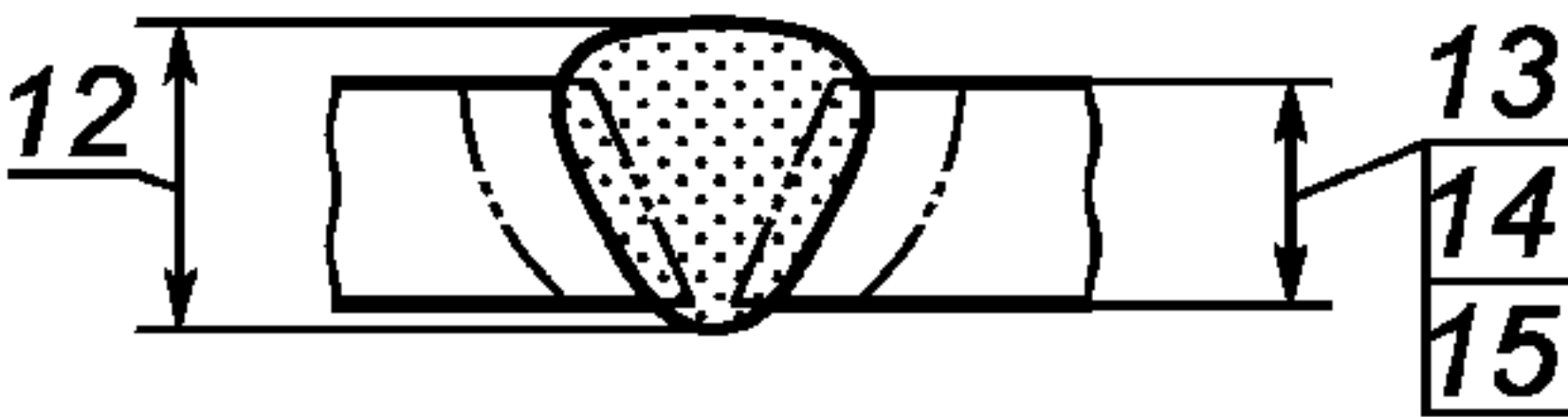
б) стыковой шов с полным проплавлением Full penetration butt weld Soudure à pleine pénétration
