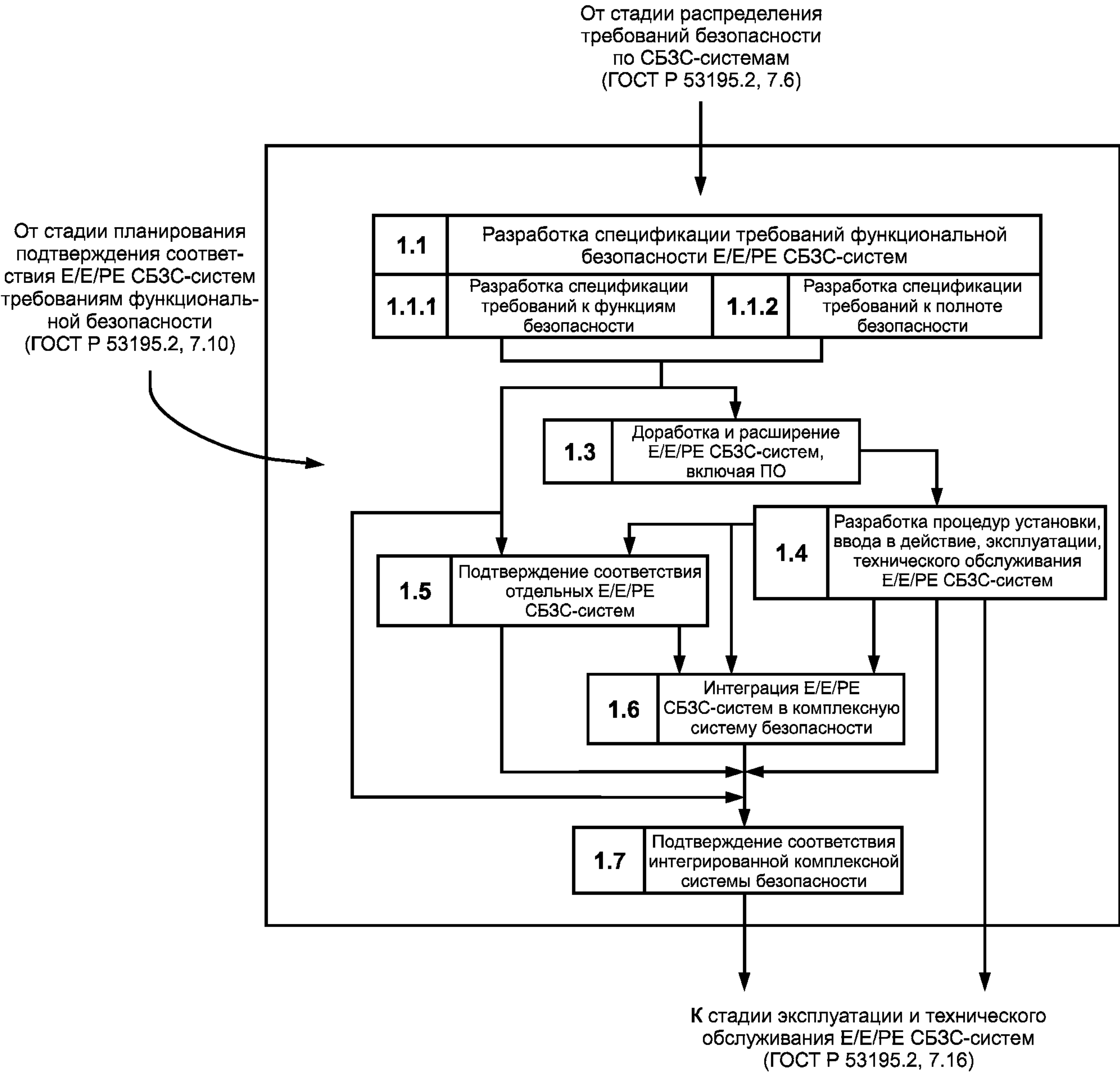
Рисунок 2 — Детализация промежуточных стадий жизненного цикла Е/Е/РЕ СБЗС-систем
