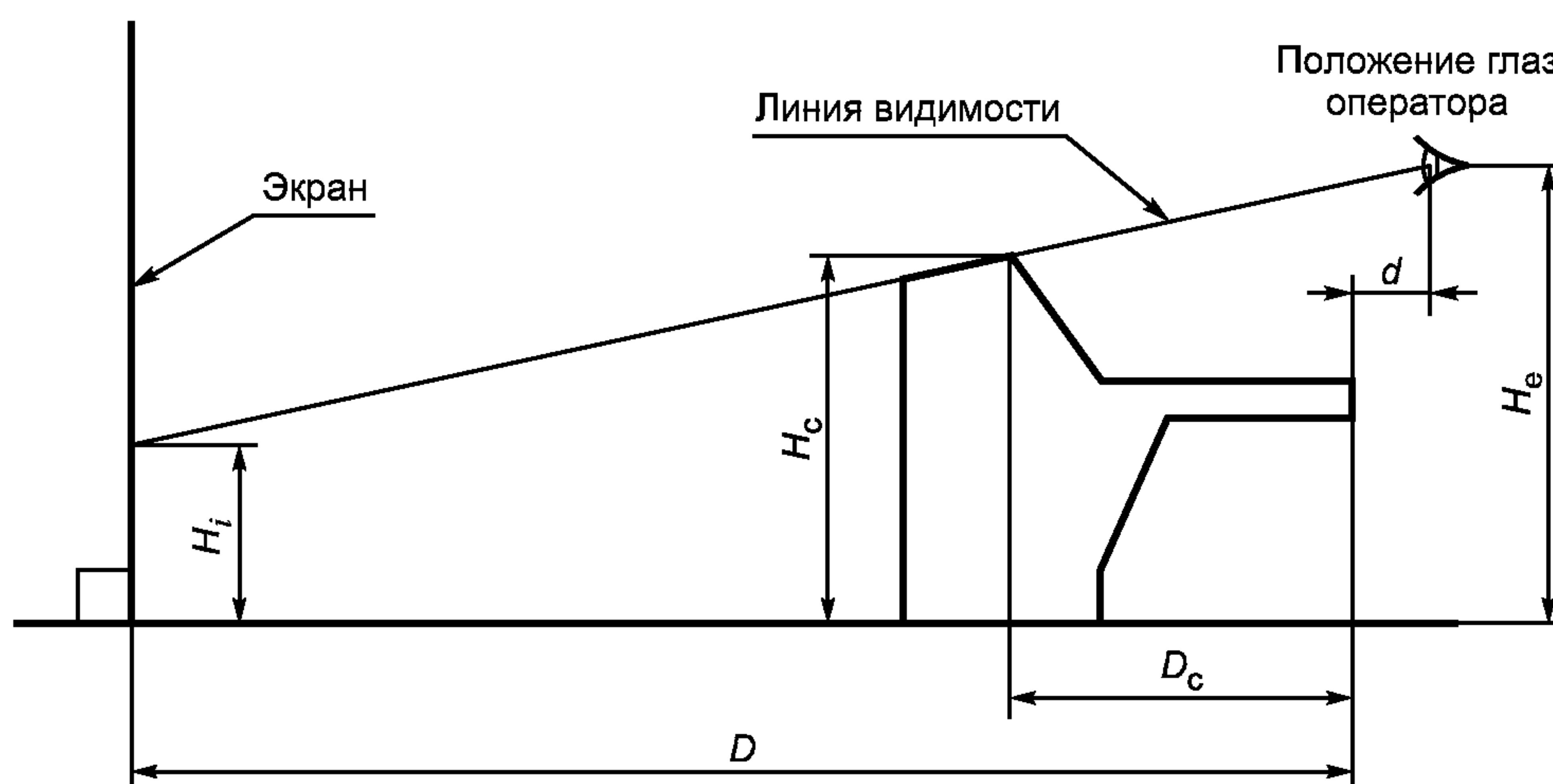
Рисунок Д.4 — Элементы оборудования АРМ
