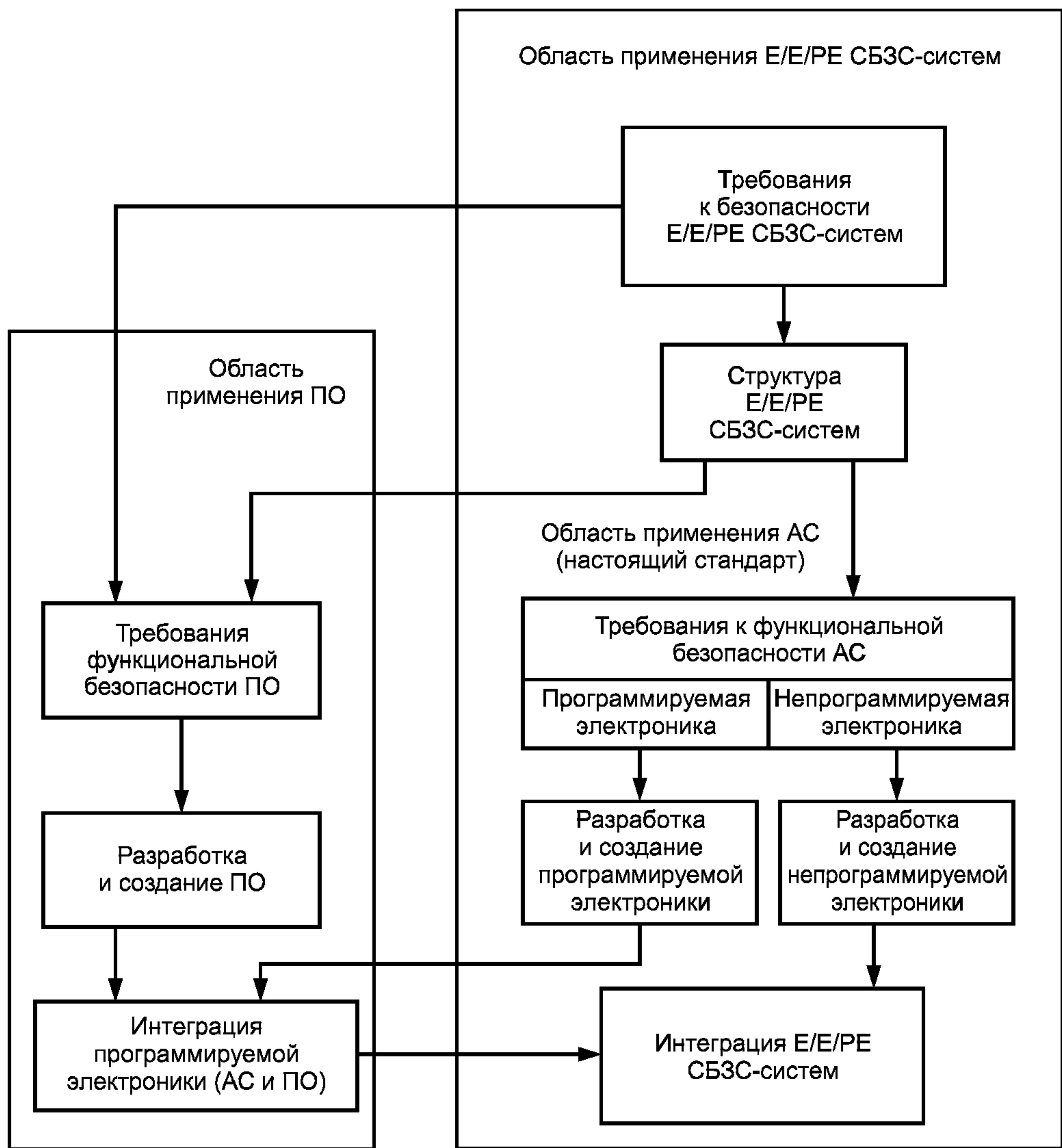
Рисунок 1 — Взаимосвязь областей применения АС и ПО
