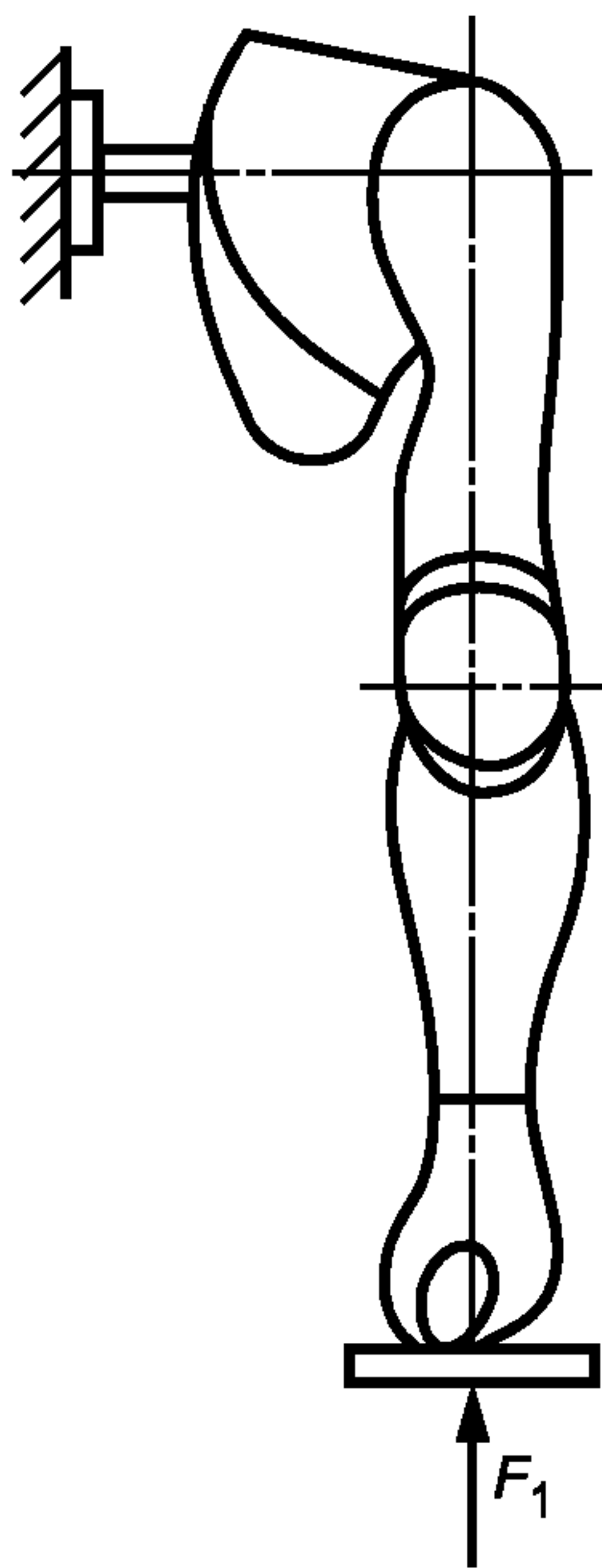
Рисунок 3 — Схема испытания на осевое нагружение концевой устройства
