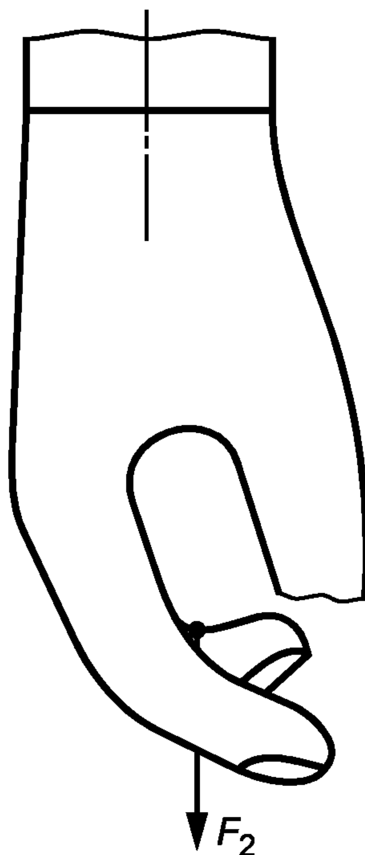
Рисунок 4 — Схема испытания фиксатора пальцев
