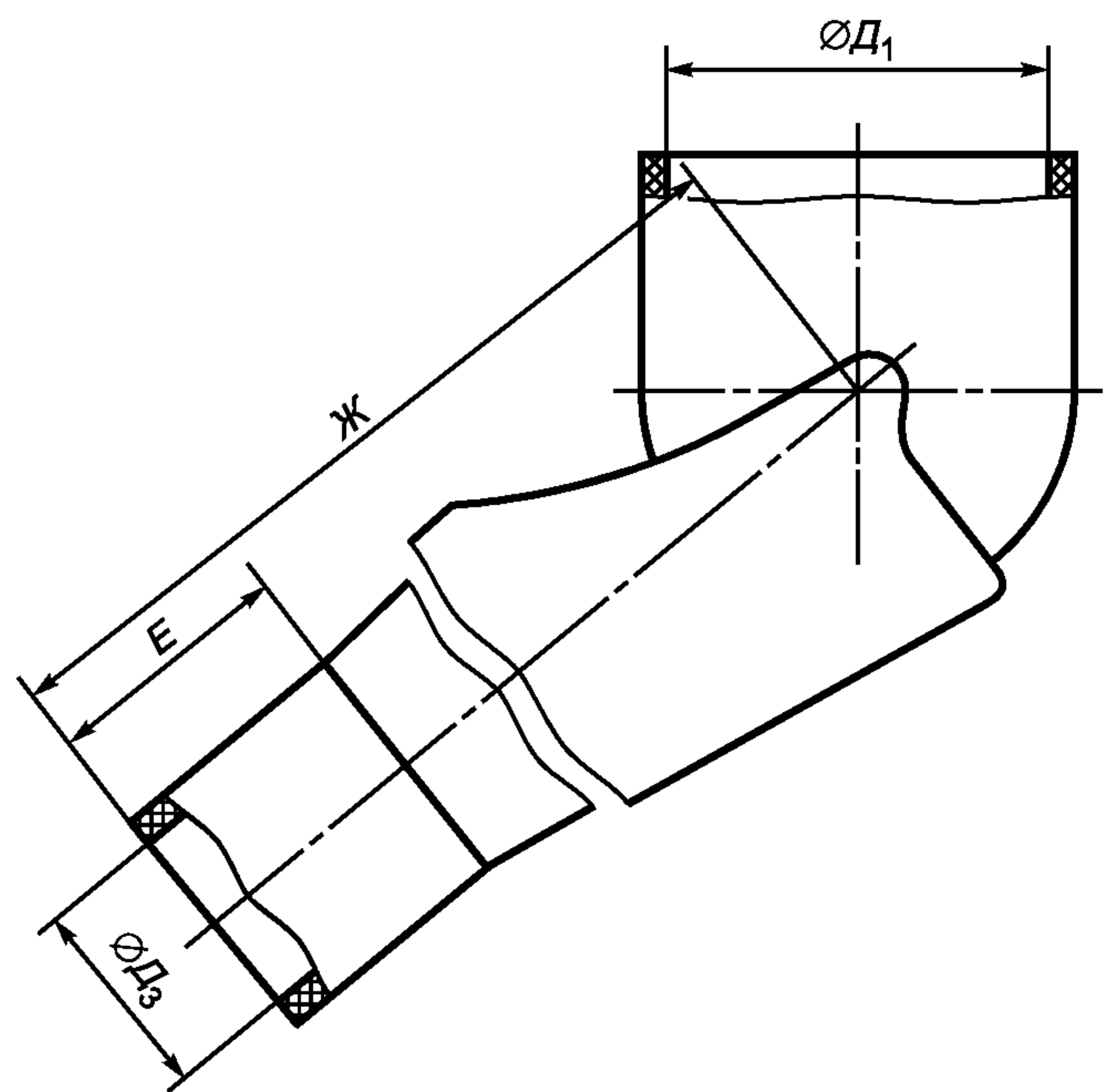
Рисунок 2 — Параметры узлов локоть — предплечье экзоскелетной конструкции
