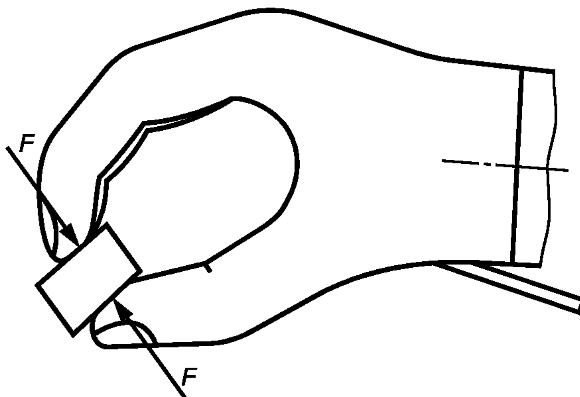
Рисунок 6 — Измерение усилия схвата
