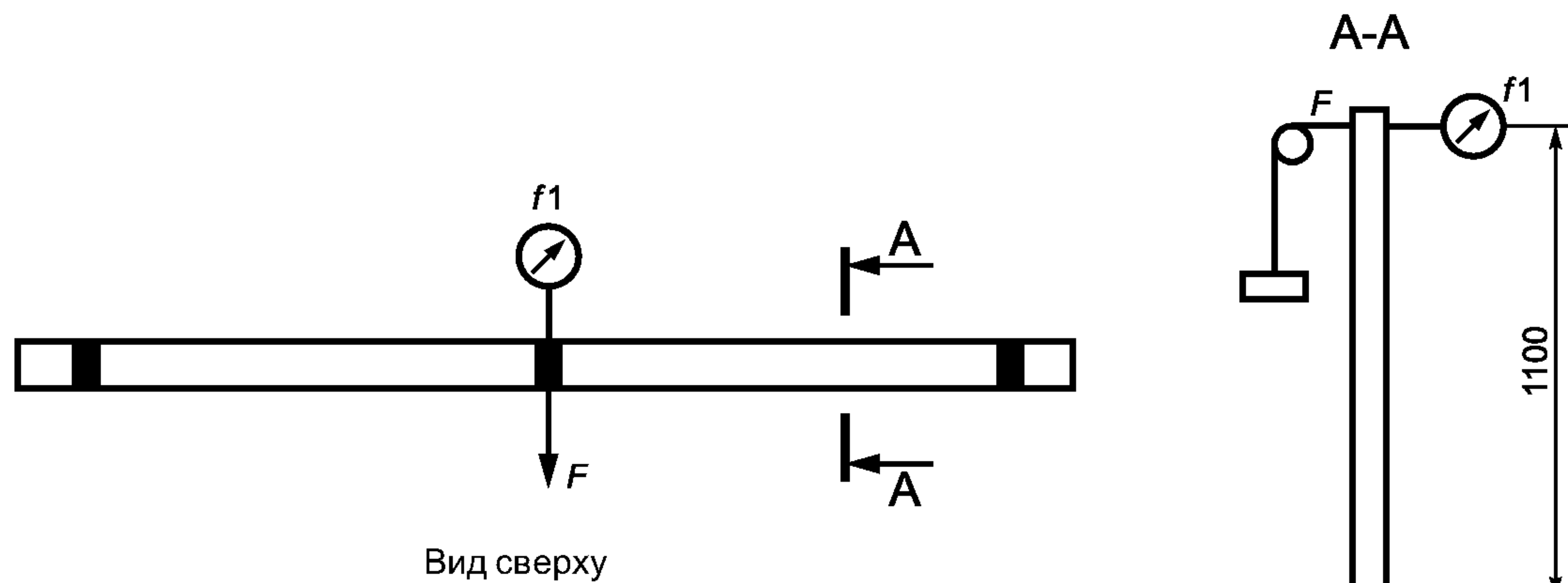
Рисунок 10 — Схема испытания опор
