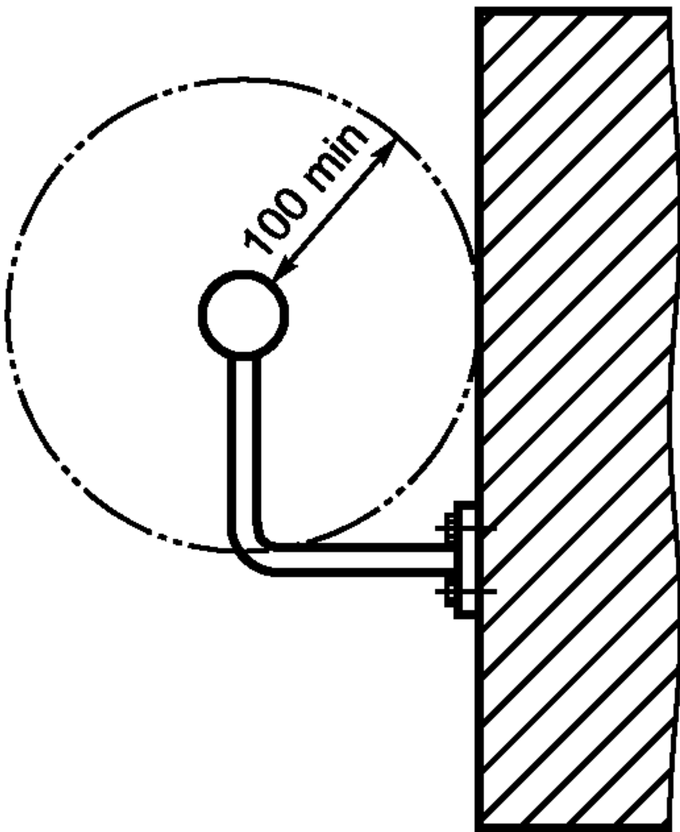
Рисунок 8 — Минимальный зазор между поручнем и любым препятствием
