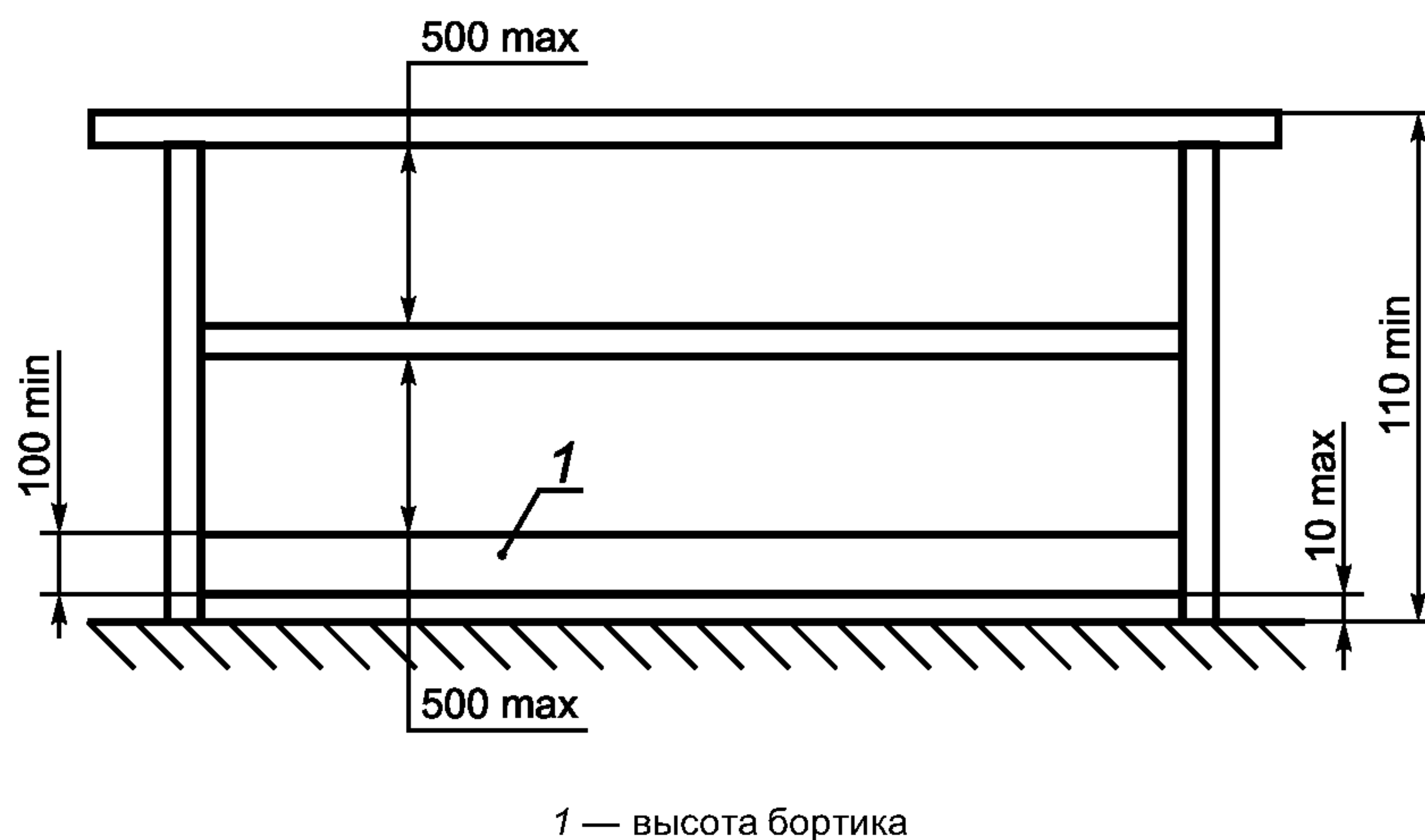
Рисунок 4 — Пример горизонтальных перил
