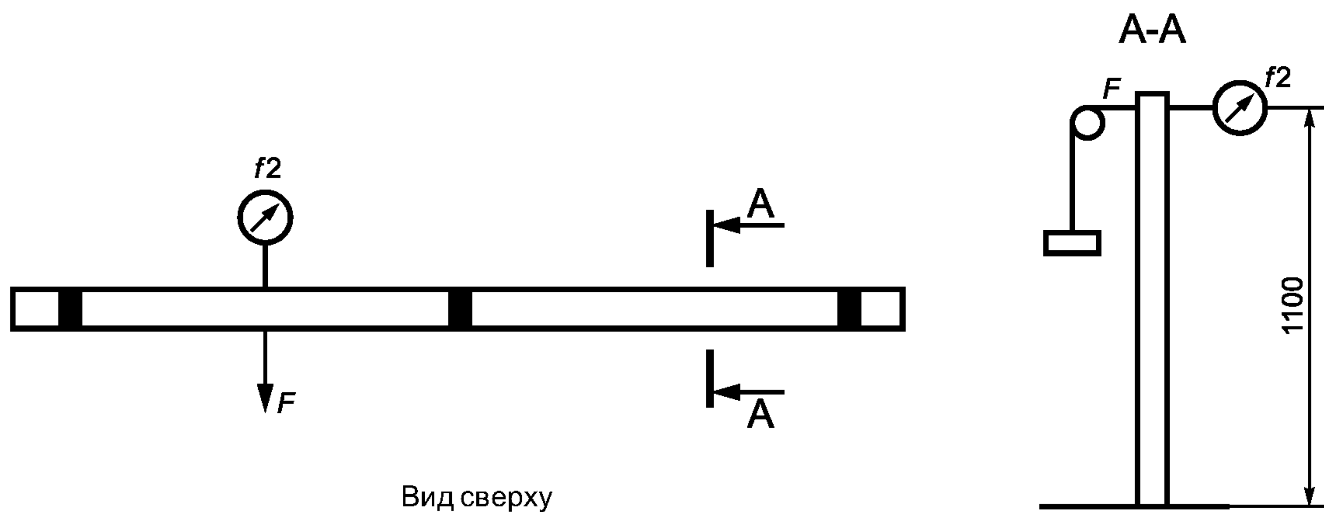
Рисунок 11 — Схема испытания поручней
