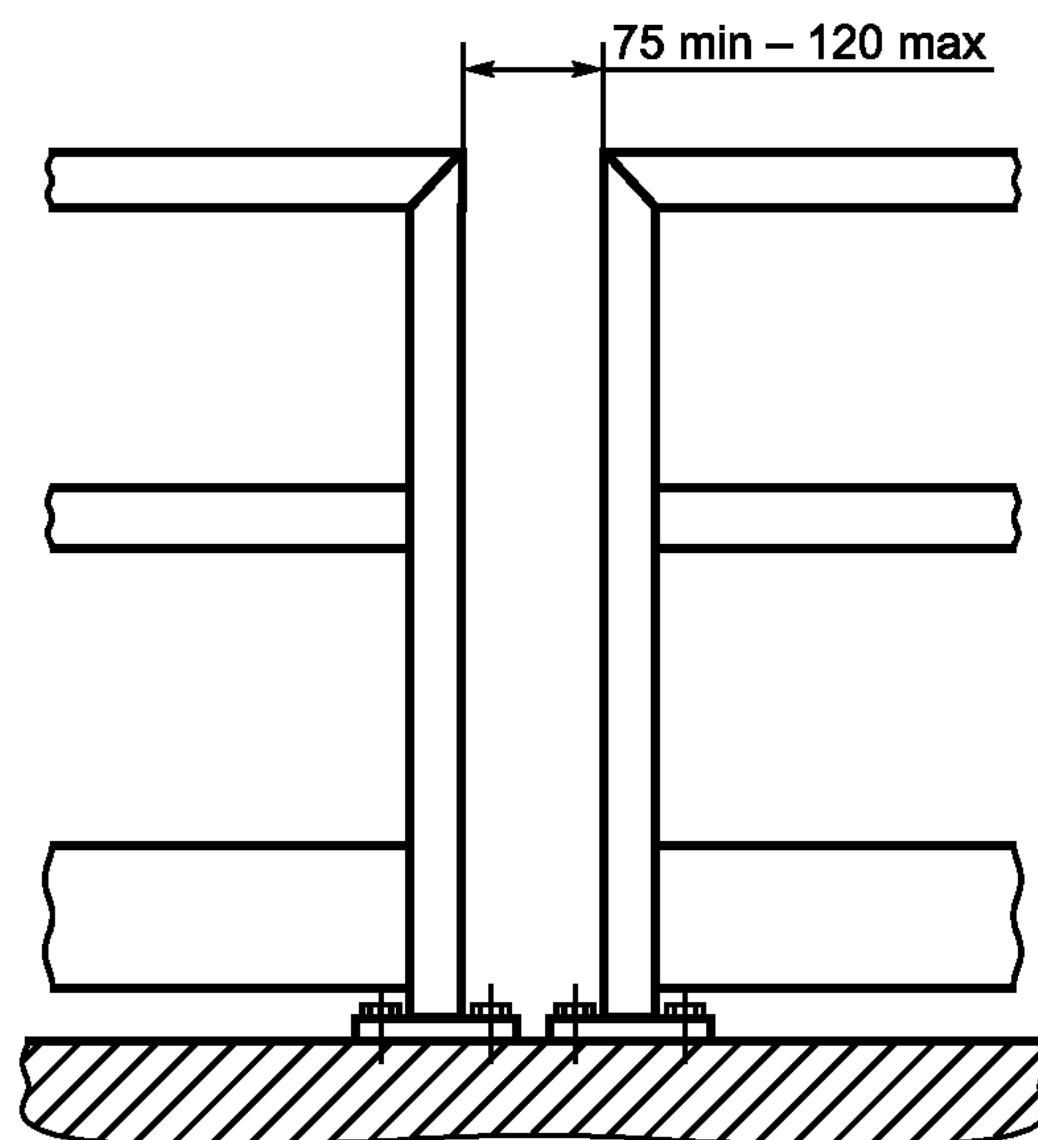
Рисунок 5 — Расстояние в свету между двумя сегментами перил
