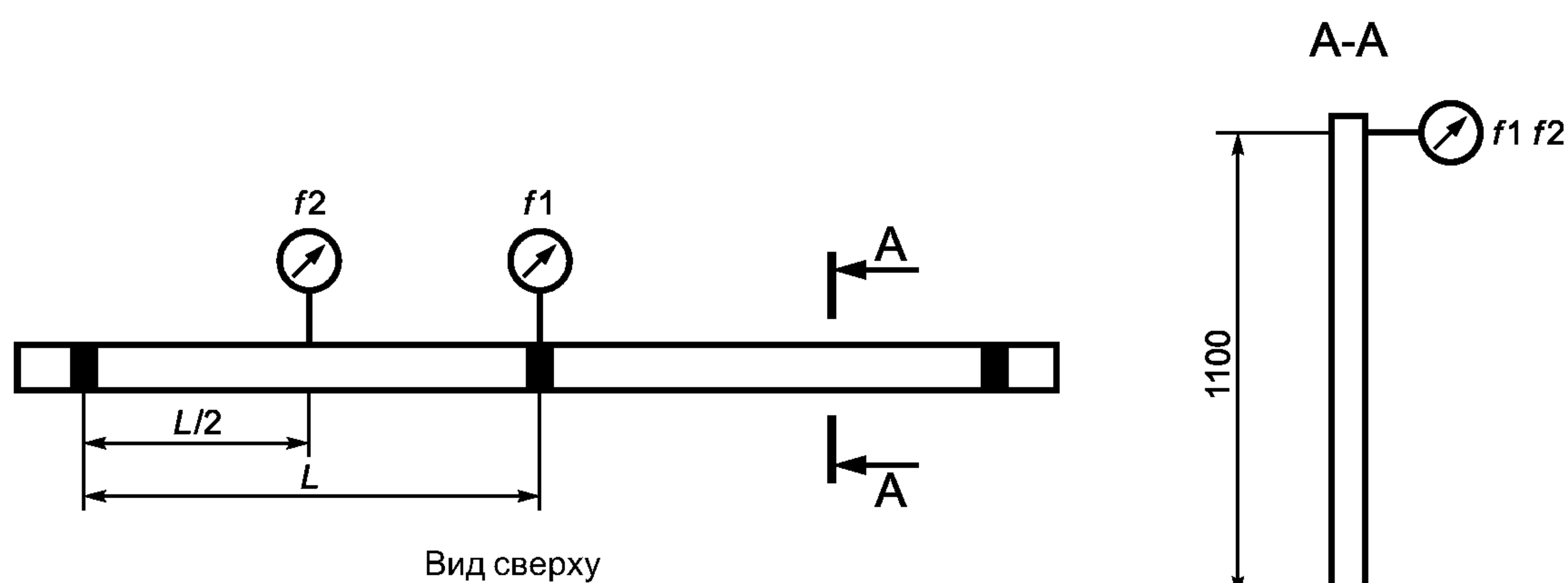
Рисунок 9 — Схема расположения прибора при измерении деформации
