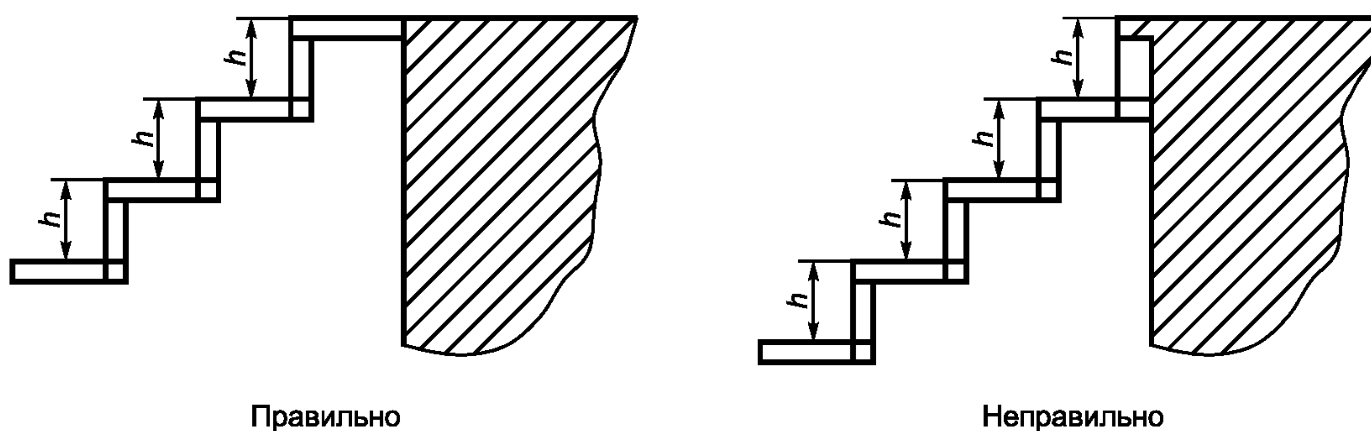
Рисунок 3 — Положение самой верхней ступени
