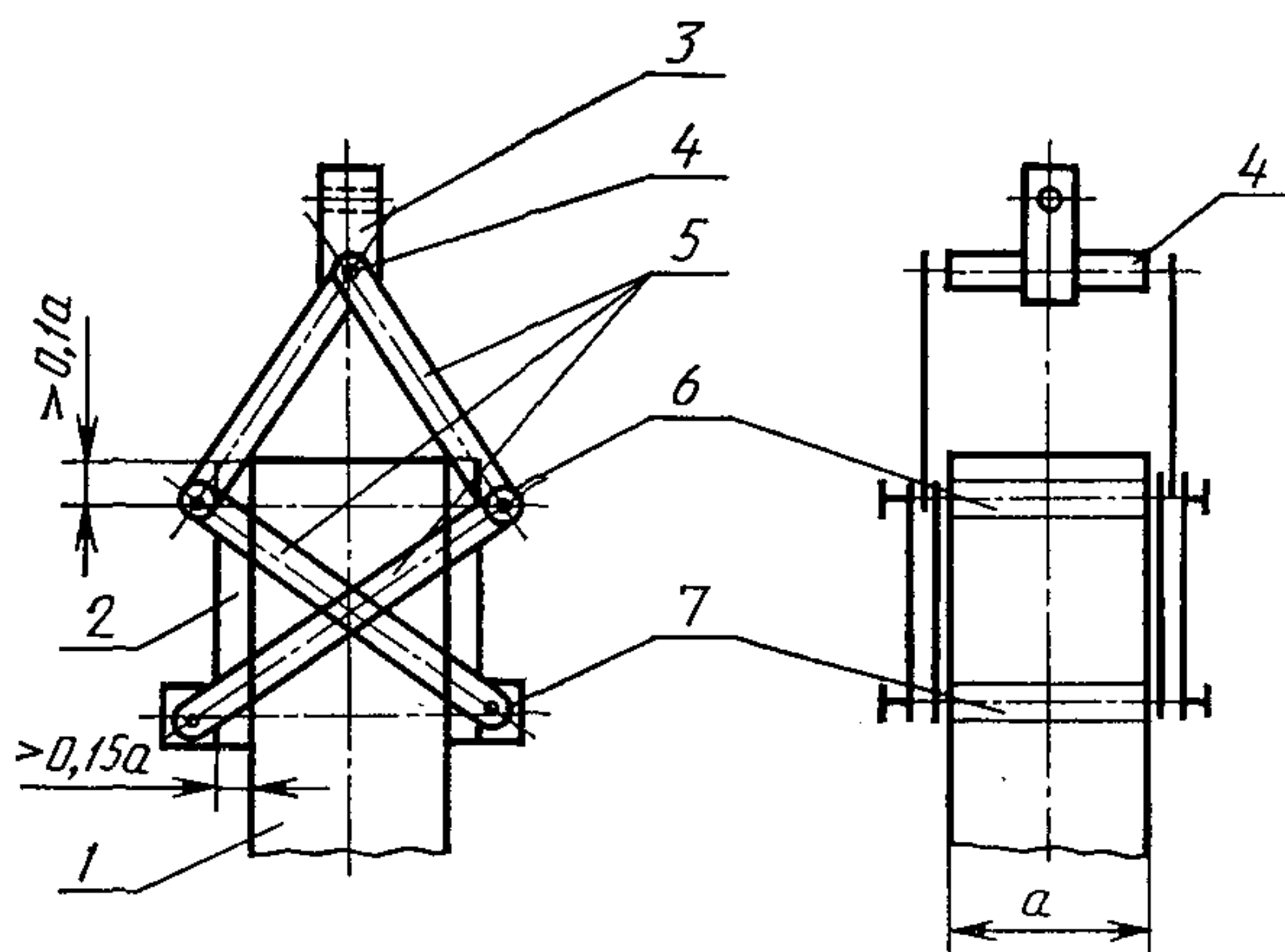
Рис. 4. Схемы съемного самозажимного захвата для образцов-призм:
