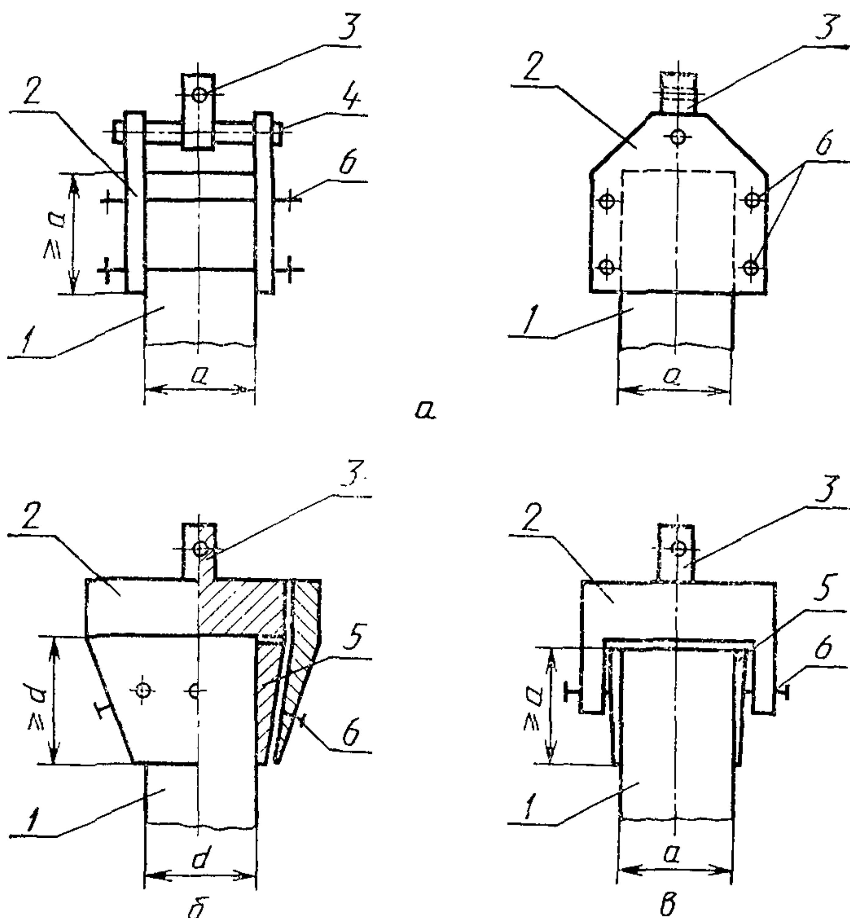
Рис. 3. Схемы съемных зажимных захватов:
