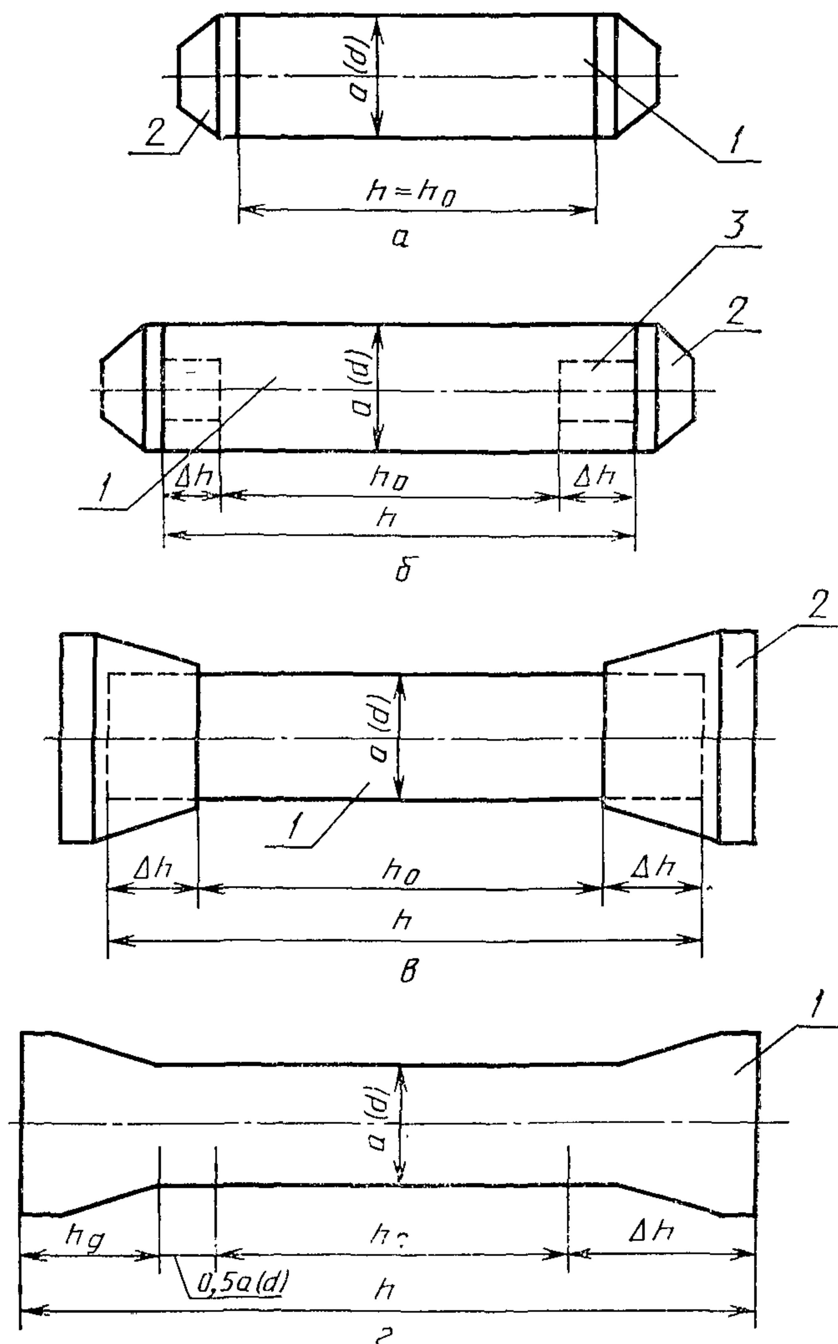
Рис. 1. Расположение зон однородного напряженного состояния ( h_0 ) и влияния захватов \Delta h при испытаниях с использованием приклеиваемых (а), анкерных (б), цанговых (в) захватов и на образцах с галтелями (г)
