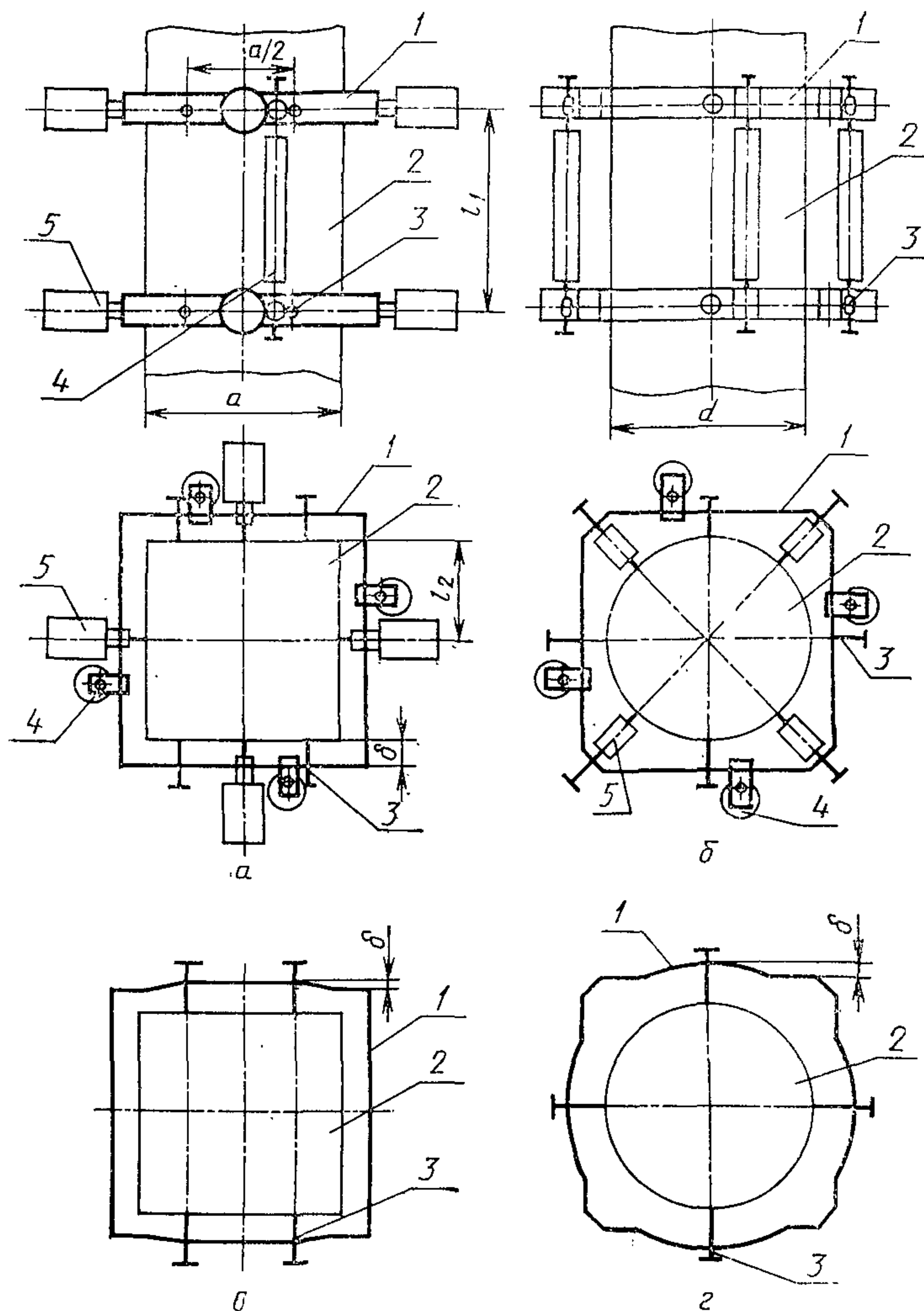
Рис. 3. Установка гибких рамок:
