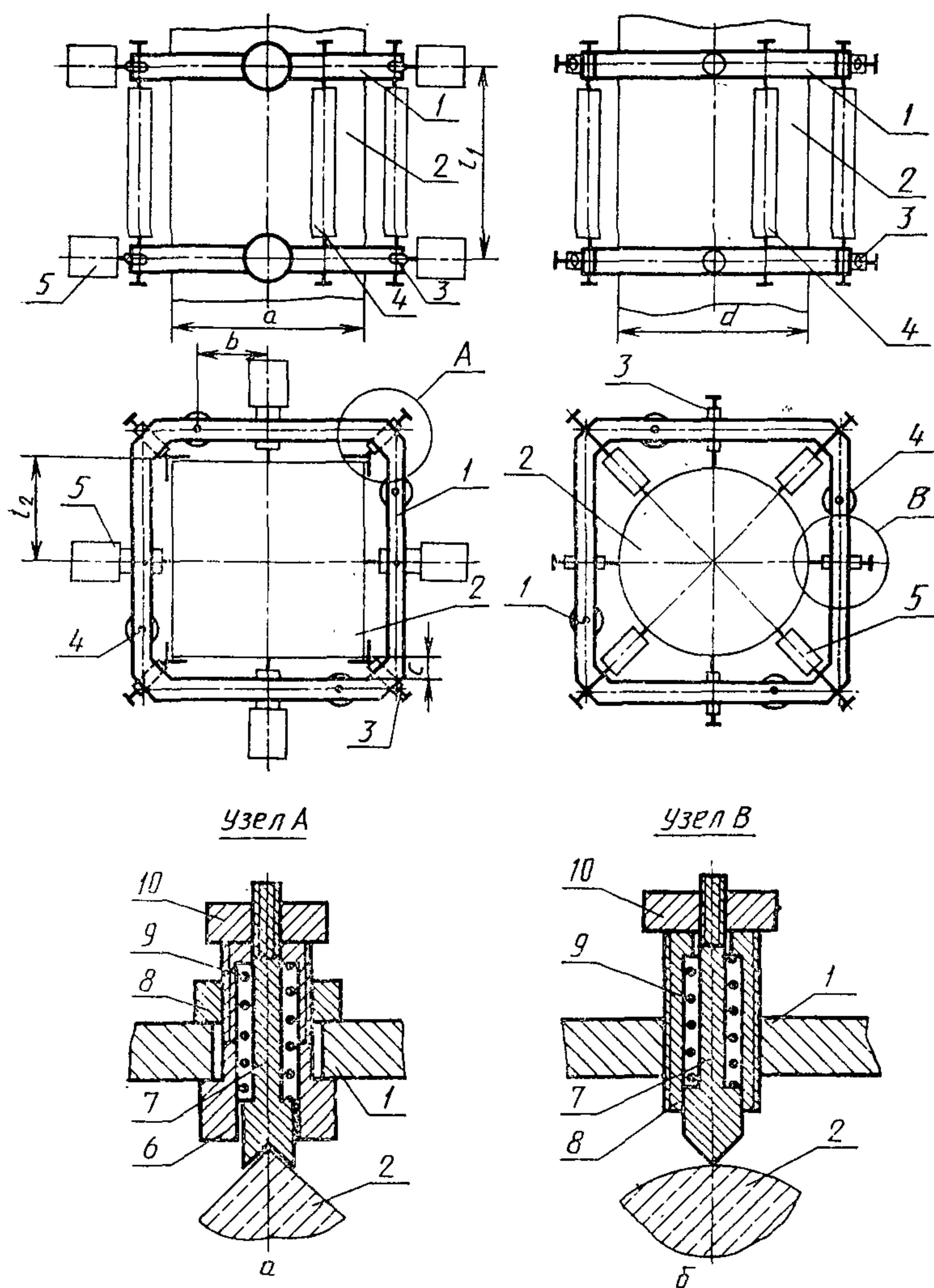
Рис. 1. Установка жестких квадратных рамок:
