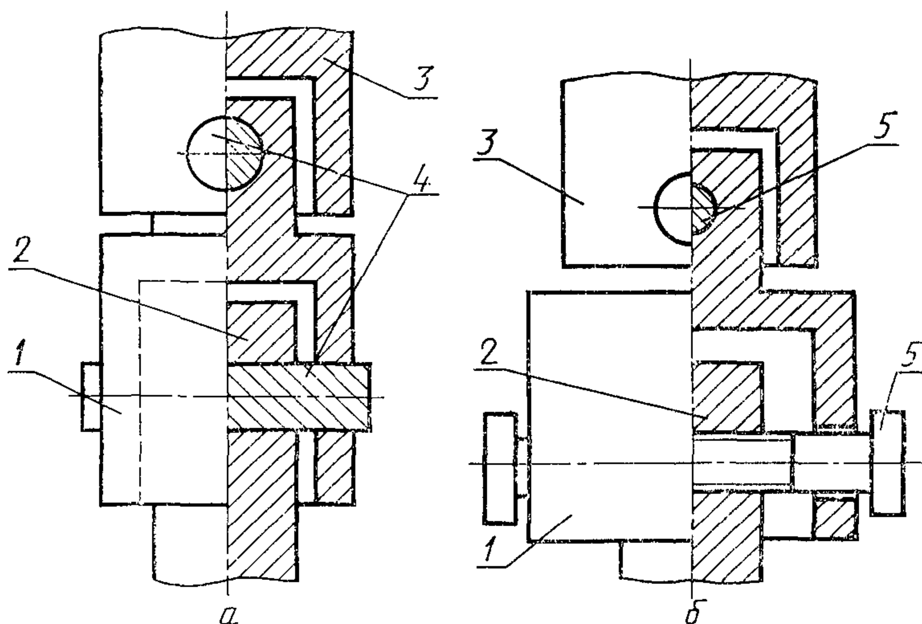
Рис. 5. Шарнир Гука:
