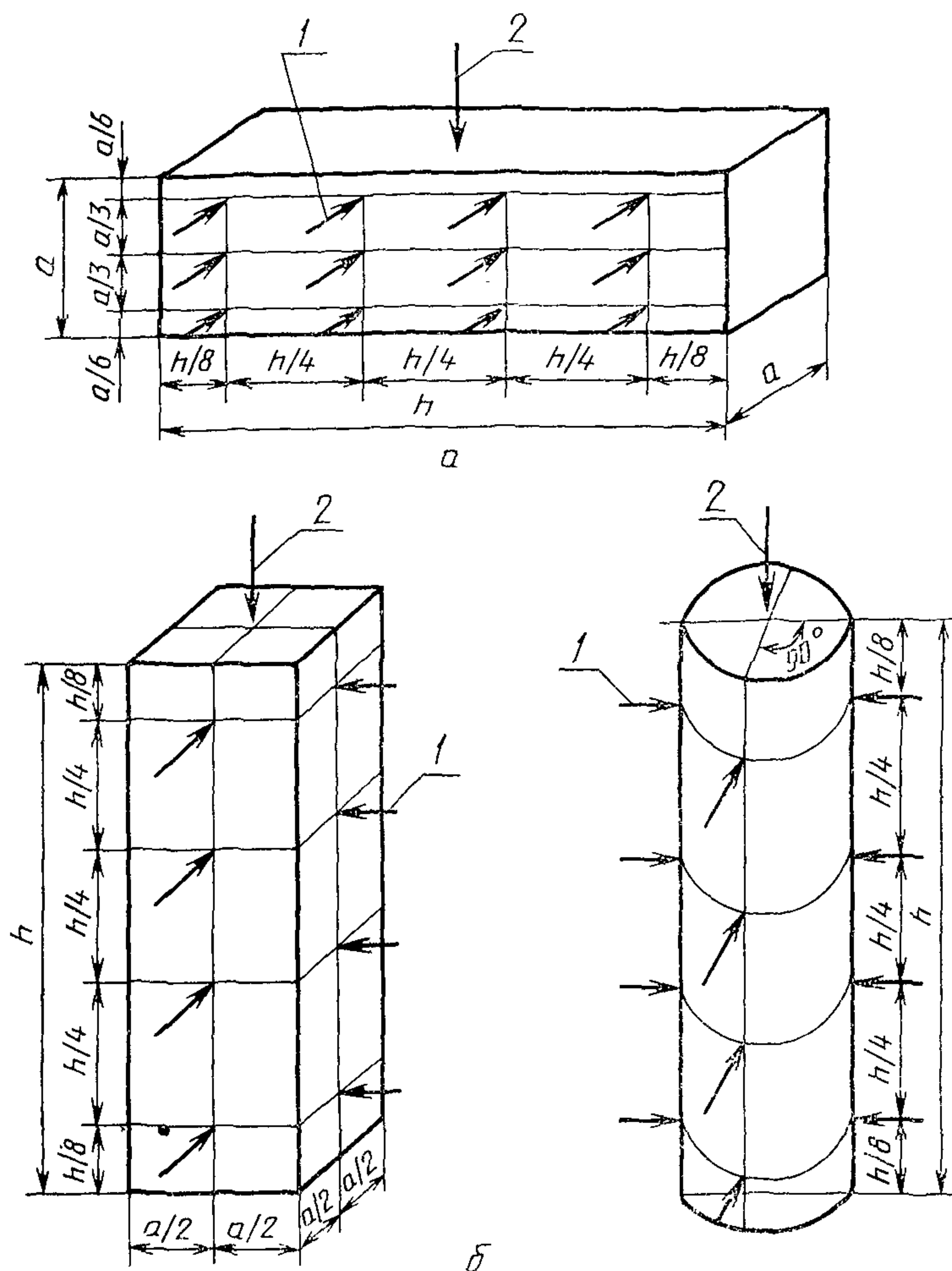
Рис. 2. Схемы прозвучивания при контроле акустической неоднородности бетона:
