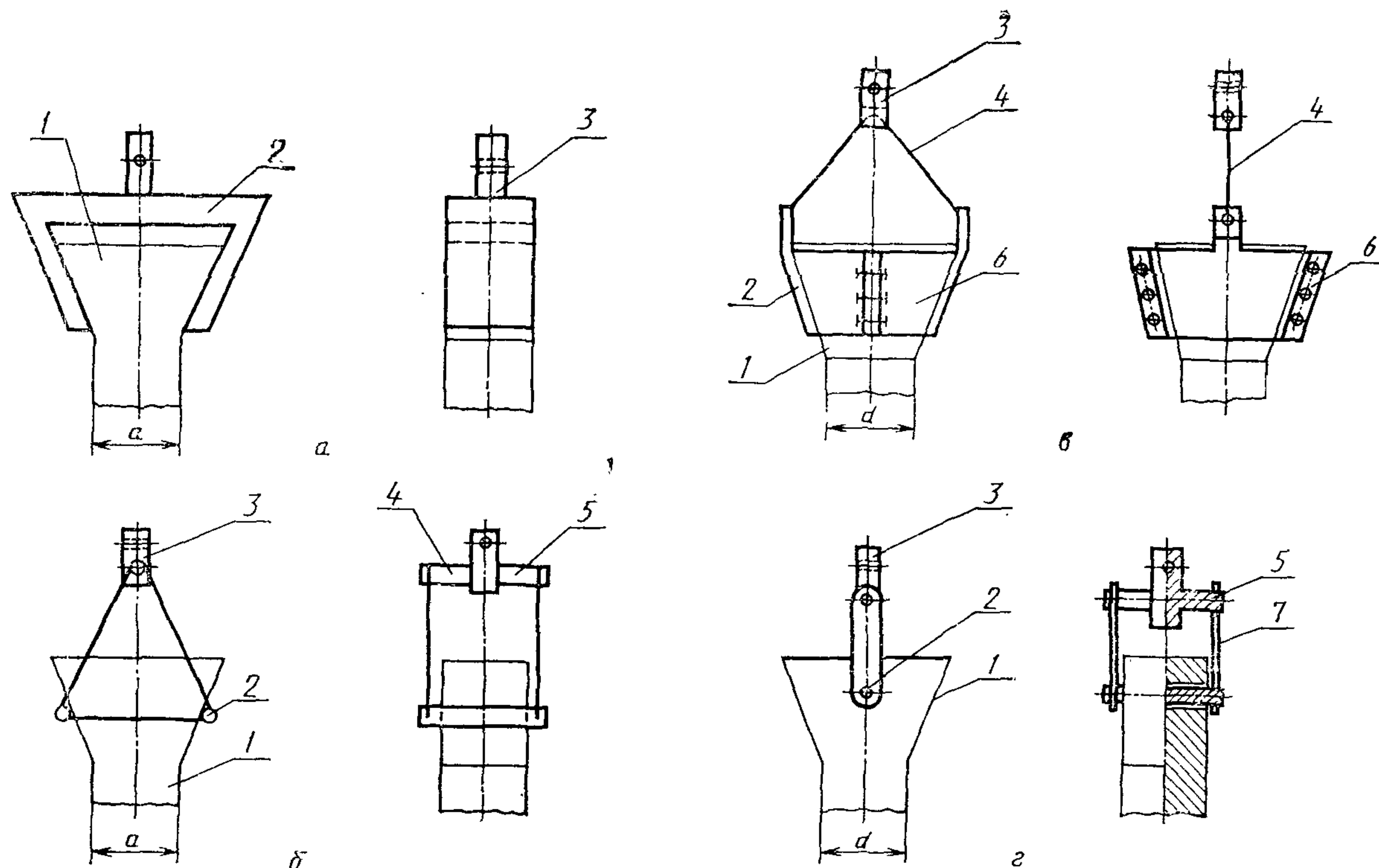
Рис. 1. Схемы захватов для образцов с галтелями:
