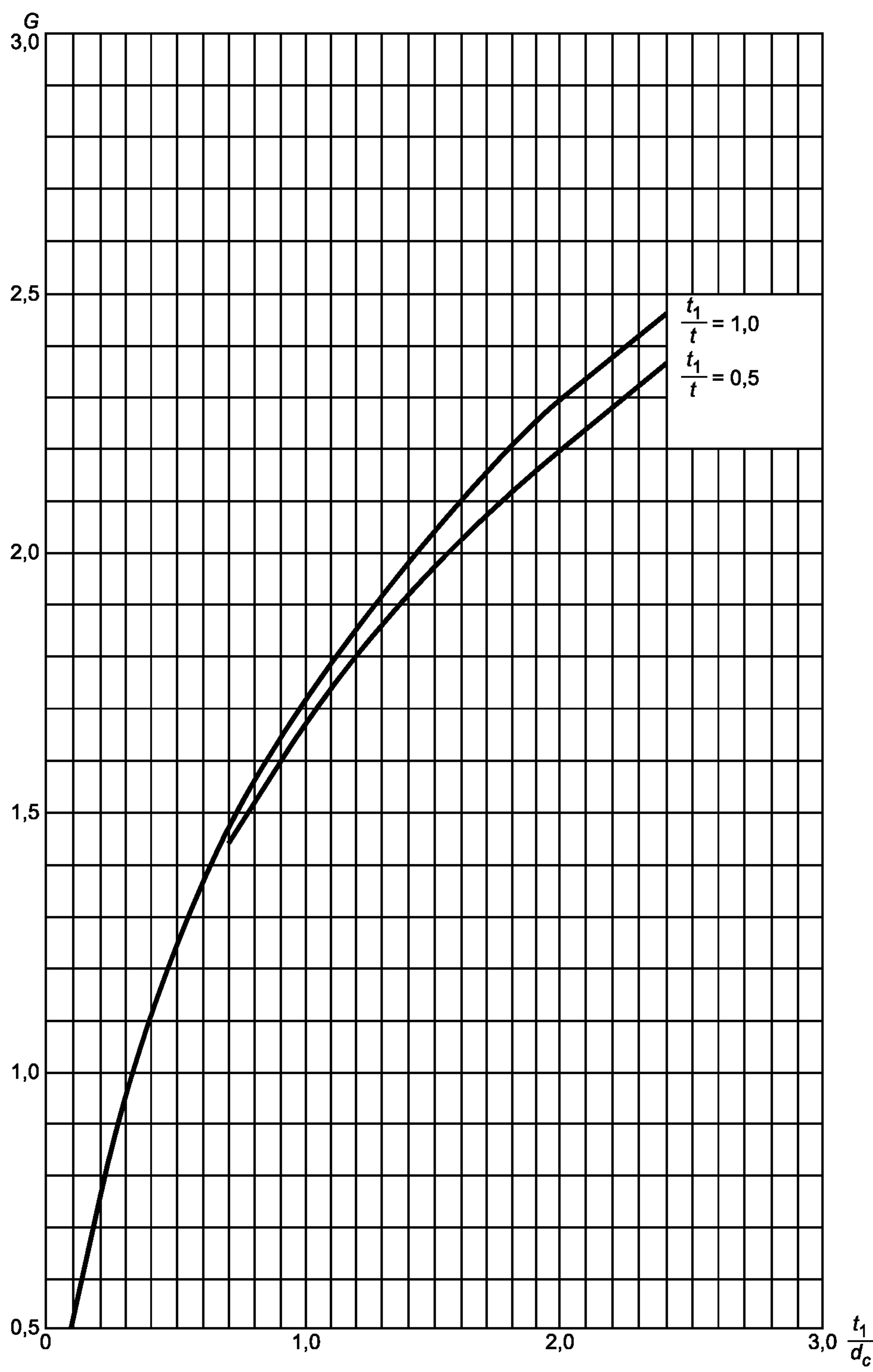
t — толщина изоляции между жилами; t_1 — толщина изоляции между жилой и оболочкой; d_c — диаметр жилы (круглой) Рисунок 2 — Геометрический фактор G для двужильного кабеля с поясной изоляцией и круглыми жилами (см. 2.1.2.1)
