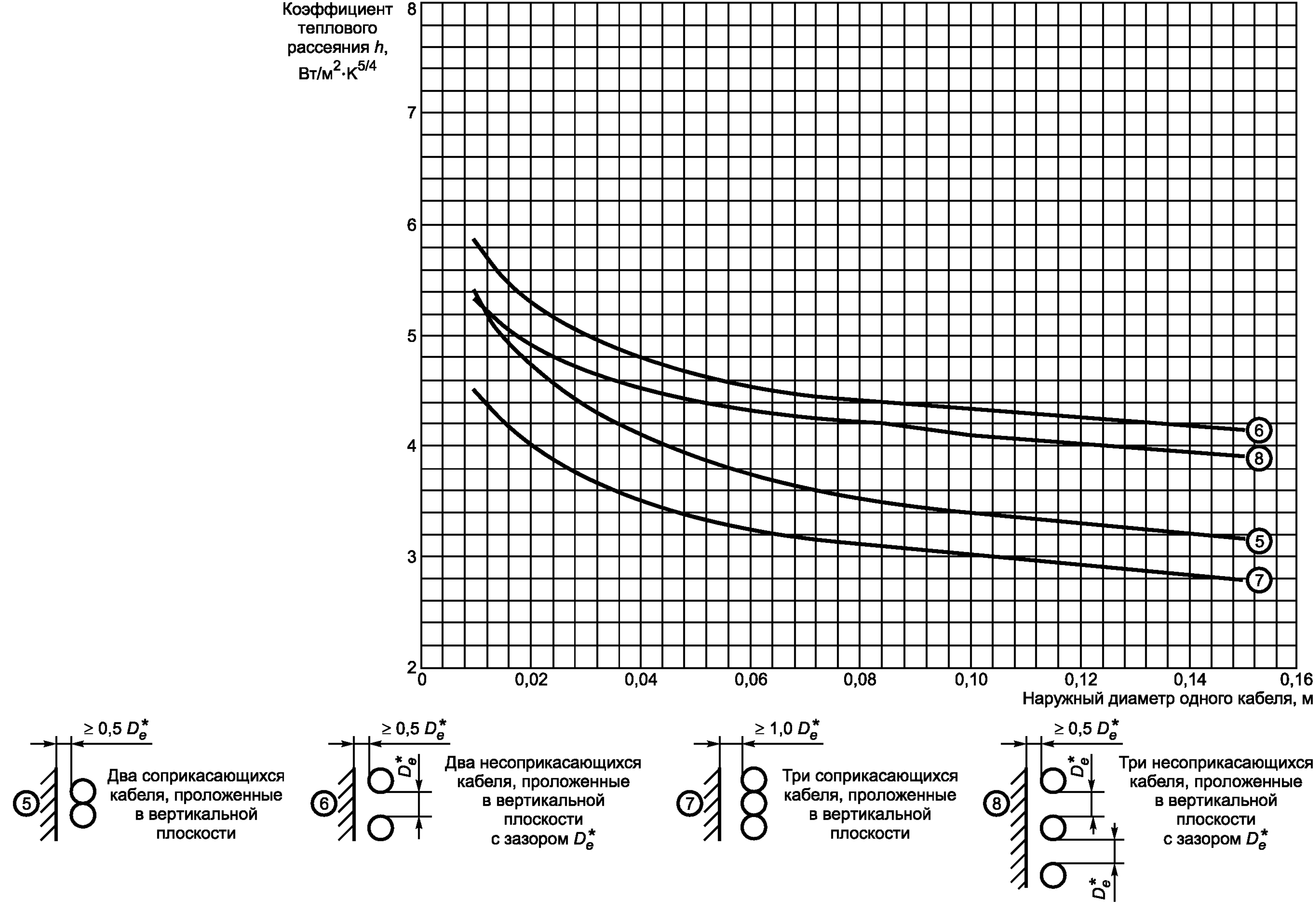
Рисунок 7b — Коэффициент теплового рассеяния для кабелей с черной поверхностью, проложенных на воздухе
