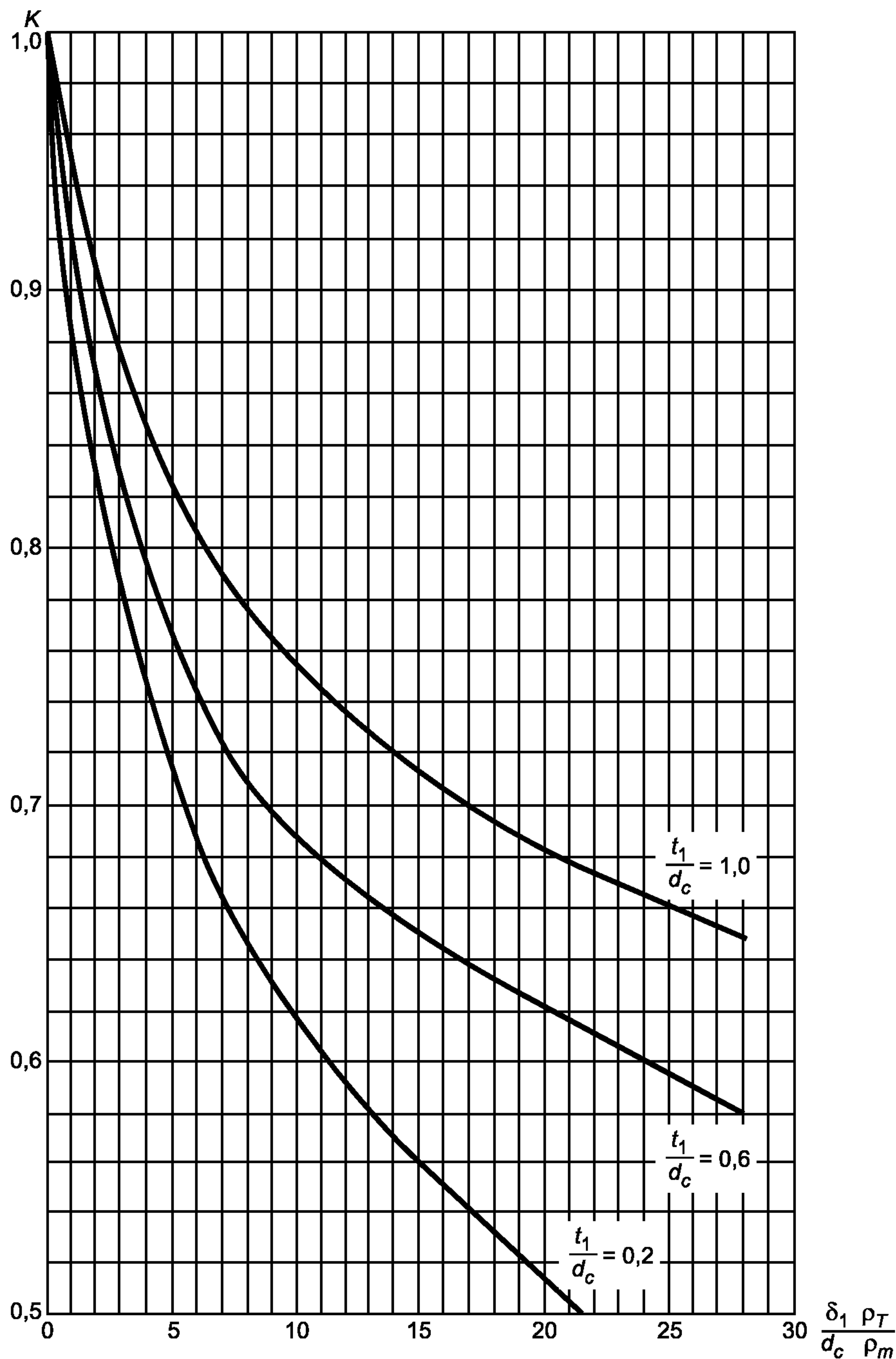
K — коэффициент экранирования; \delta_1 — толщина металлического экрана по изолированной жиле; \rho_T — удельное тепловое сопротивление изоляции; d_c — диаметр жилы (круглой); t_1 — толщина изоляции между жилой и экраном; \rho_m — удельное тепловое сопротивление экранирующего материала: 27 \cdot 10^{-4} \text{ К} \cdot \text{м/Вт} — для меди; 48 \cdot 10^{-4} \text{ К} \cdot \text{м/Вт} — для алюминия
