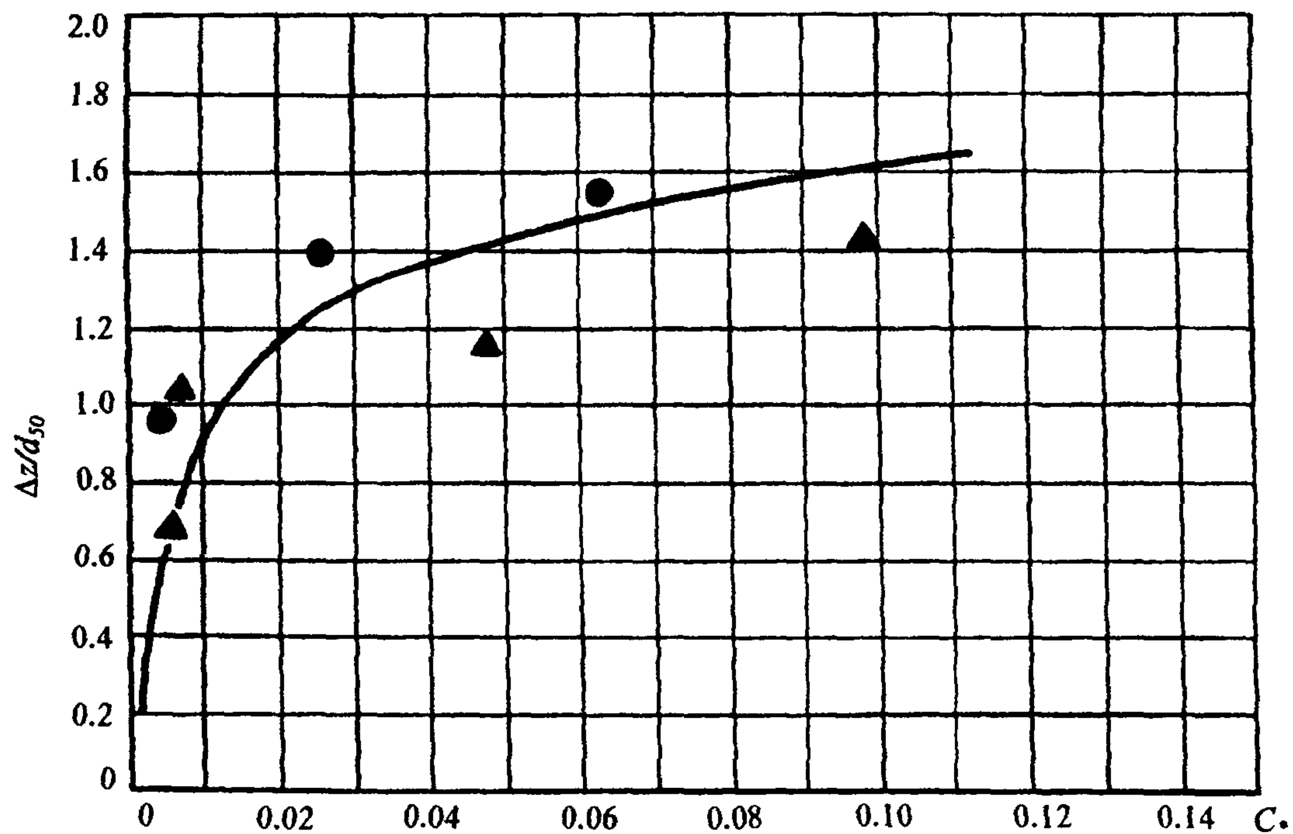
Диаграмма для определения C .
