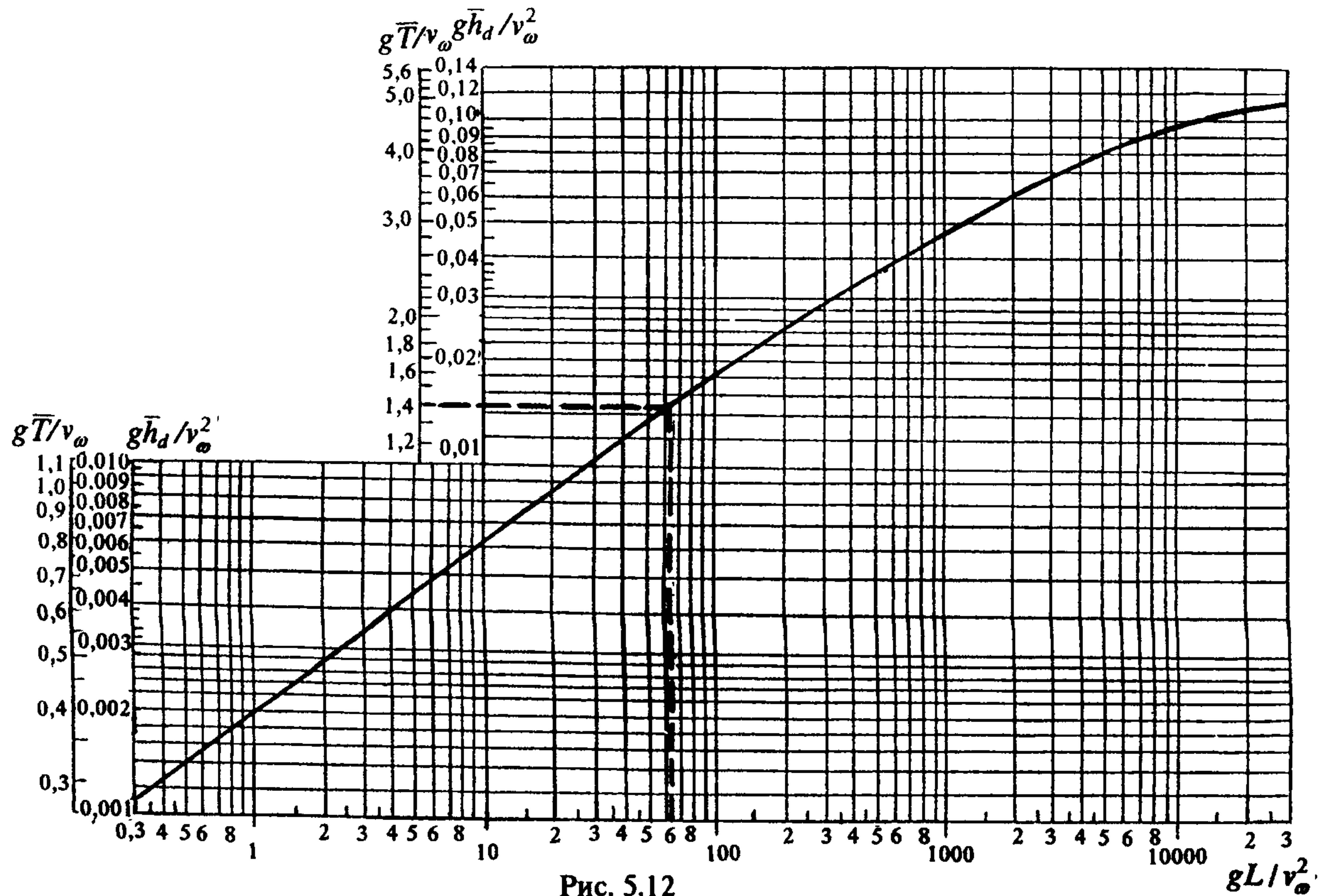
График для определения элементов ветровых волн в глубоководных зонах
