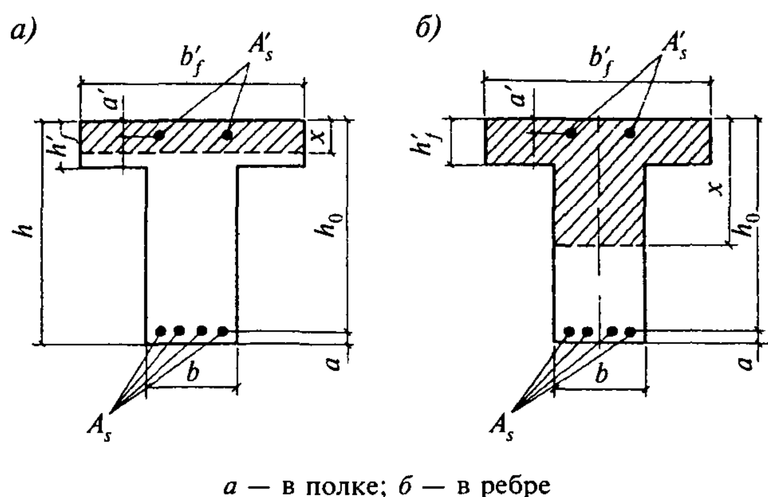
Рисунок 7.3 — Положение границы сжатой зоны в сечении изгибаемого железобетонного элемента
