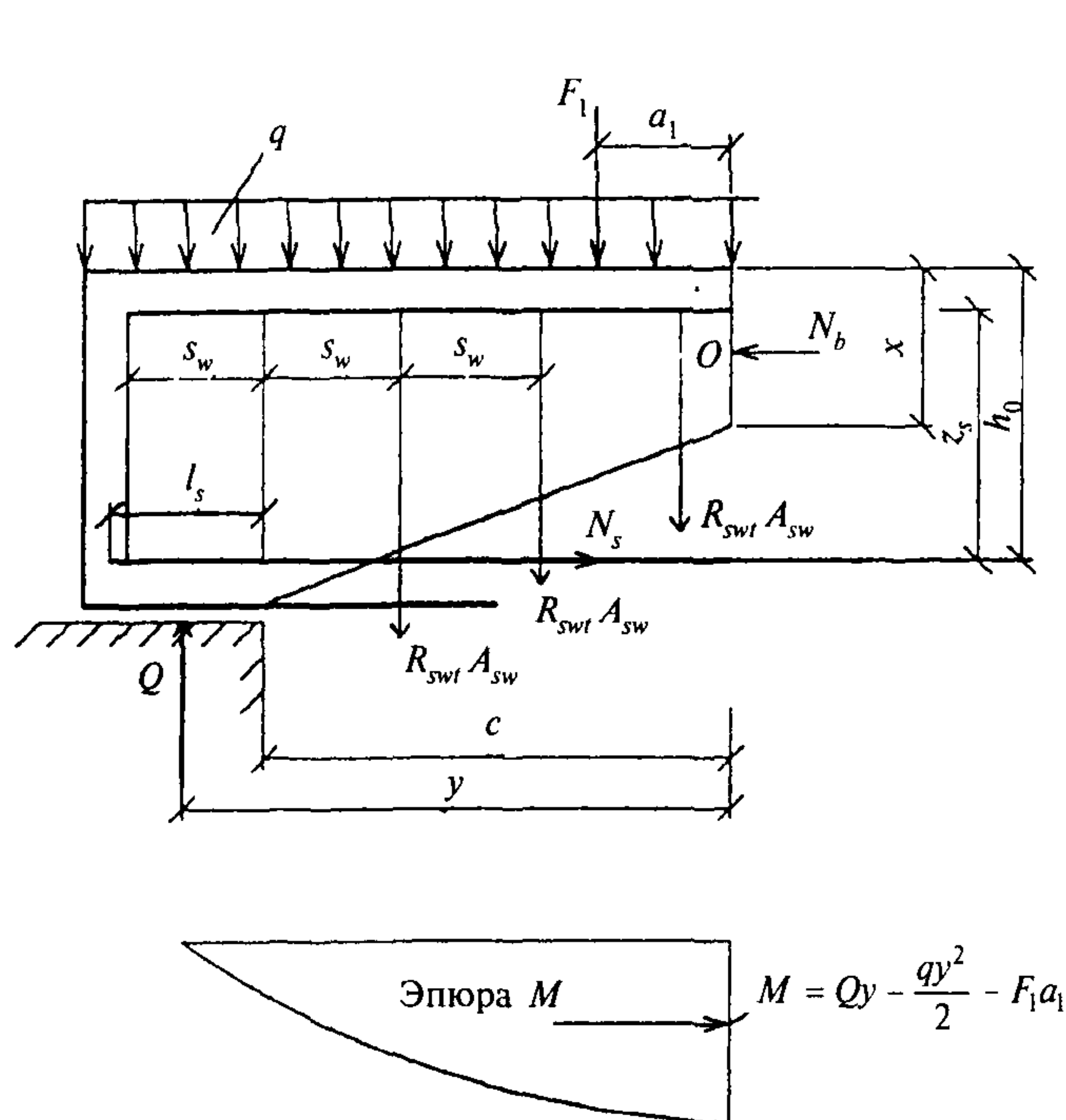
Рисунок 7.7 — Схема усилий в наклонном сечении элемента с хомутами при расчете на действие момента
