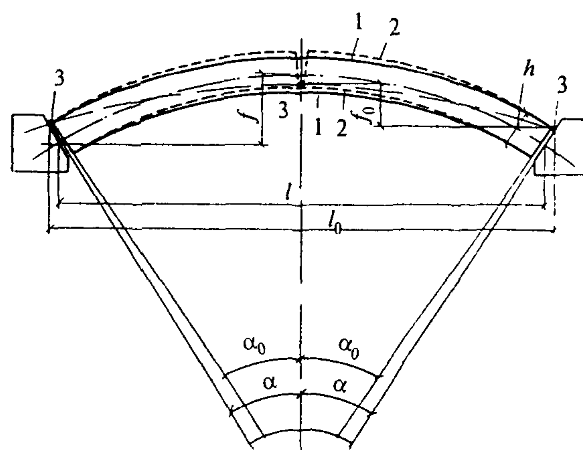
1 — свод до нагрева; 2 — свод нагретый; 3 — условный шарнир
