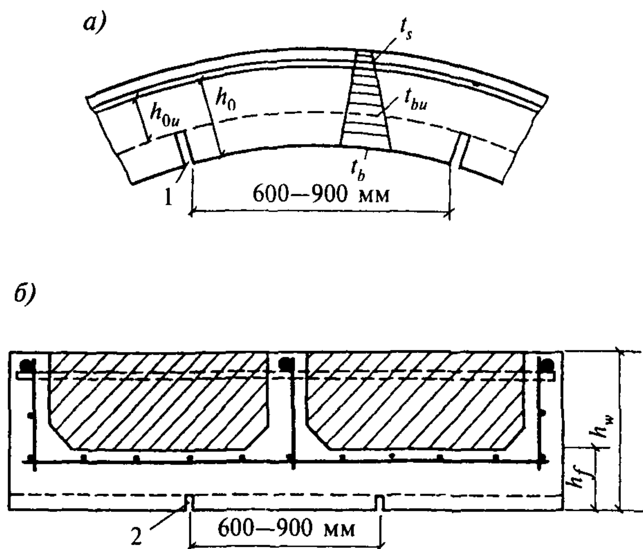
a — компенсационные; b — усадочные; 1 — компенсационный шов шириной 2—5 мм; 2 — усадочный шов глубиной 0,1h_f и шириной 2—3 мм
