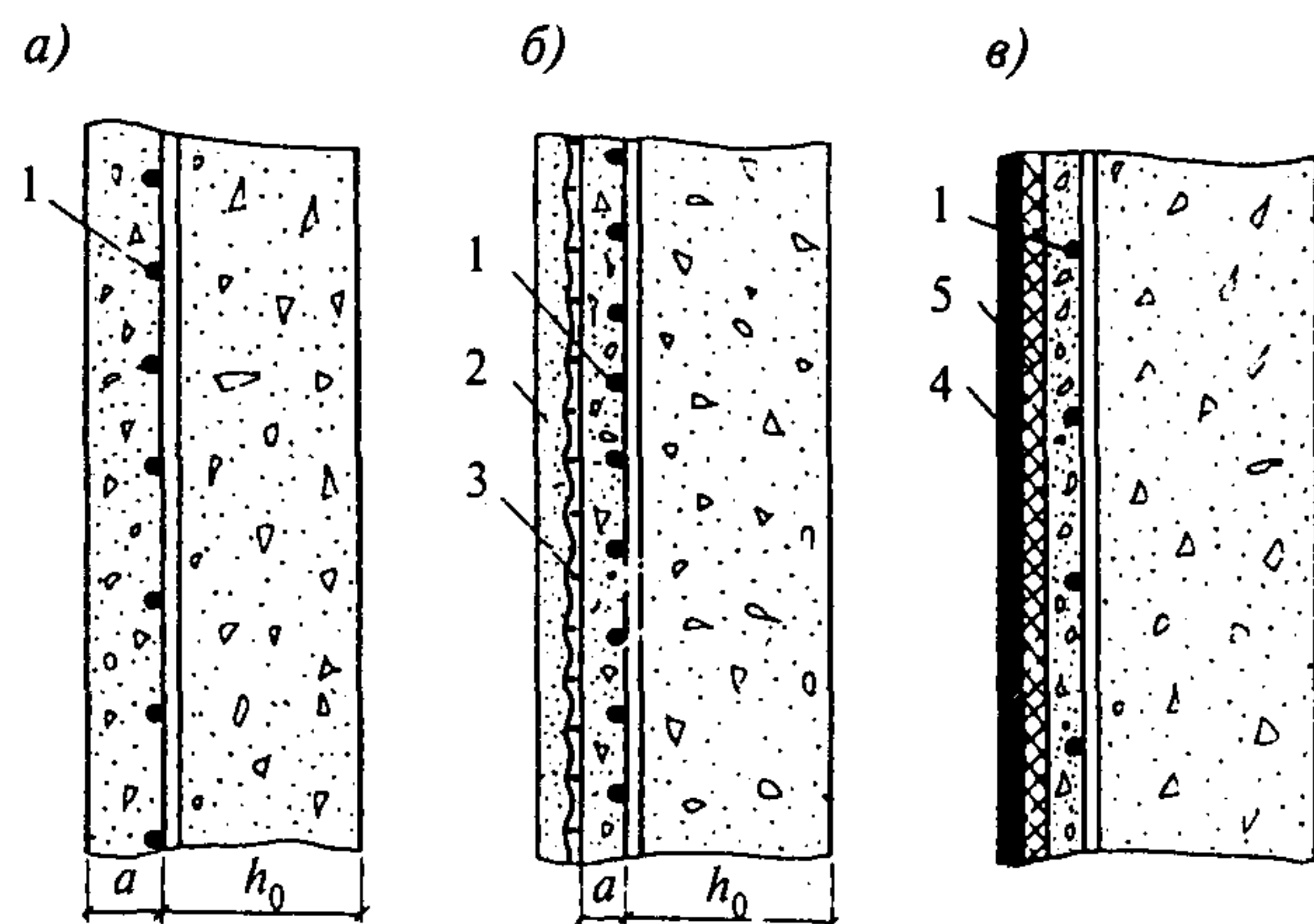
а — однослойная из сборного или монолитного железобетона; б — то же, с теплоизоляционной штукатуркой; в — то же, с теплоизоляцией и стальным кожухом; 1 — арматура; 2 — теплоизоляционная штукатурка; 3 — металлическая сетка; 4 — стальной кожух; 5 — теплоизоляция
