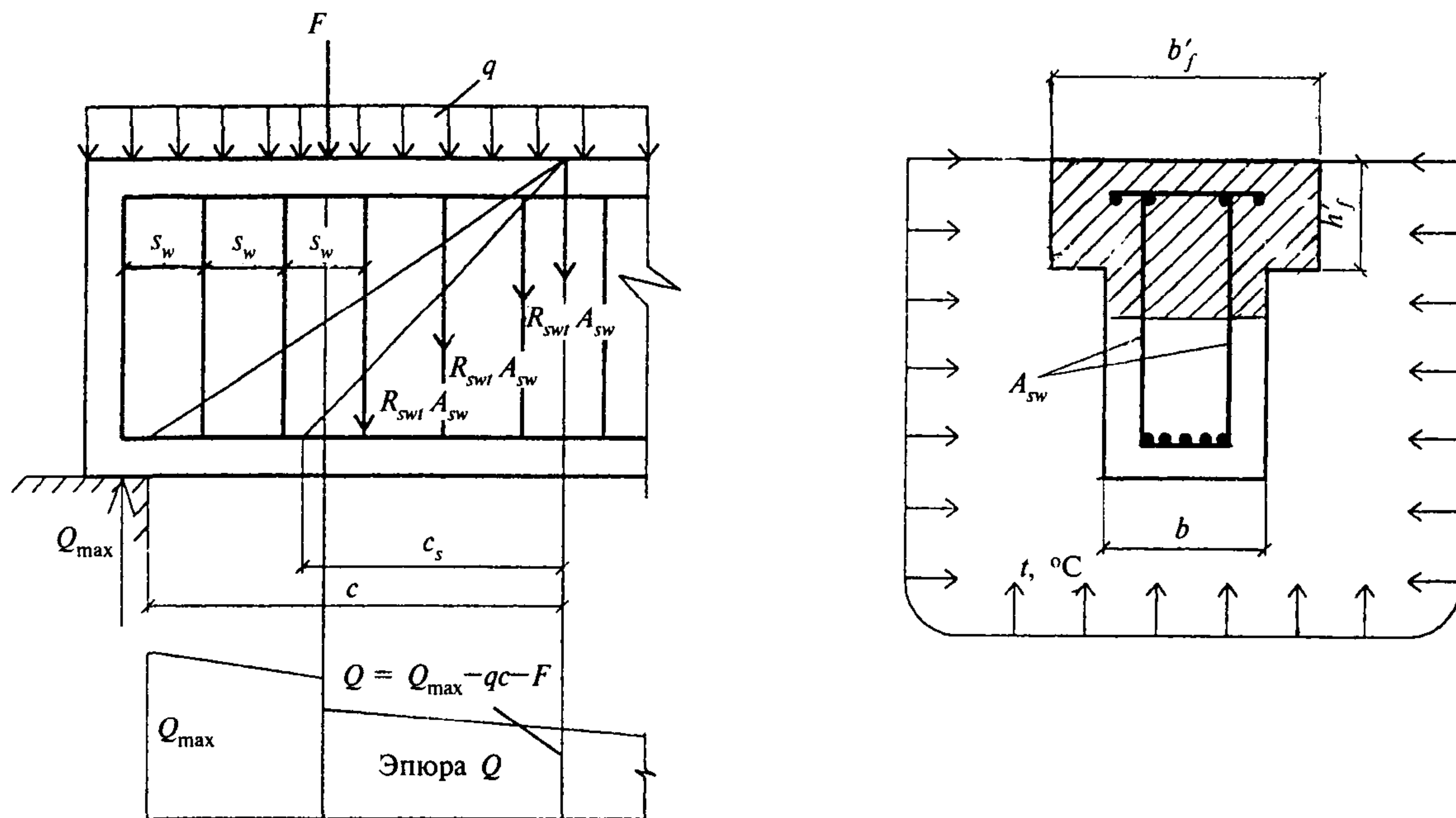
Рисунок 7.6 — Схема усилий в наклонном сечении элемента с хомутами при расчете на действие поперечных сил
