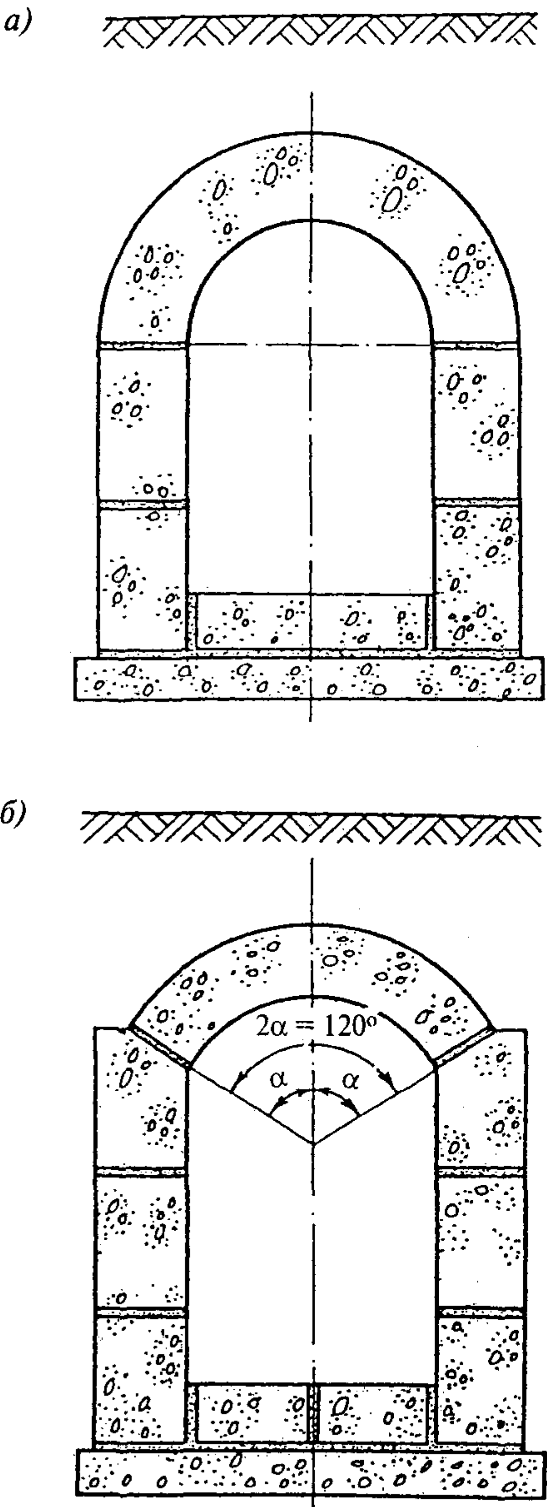
а — с цилиндрическим полициркульным сводом; б — с цилиндрическим лучковым сводом
