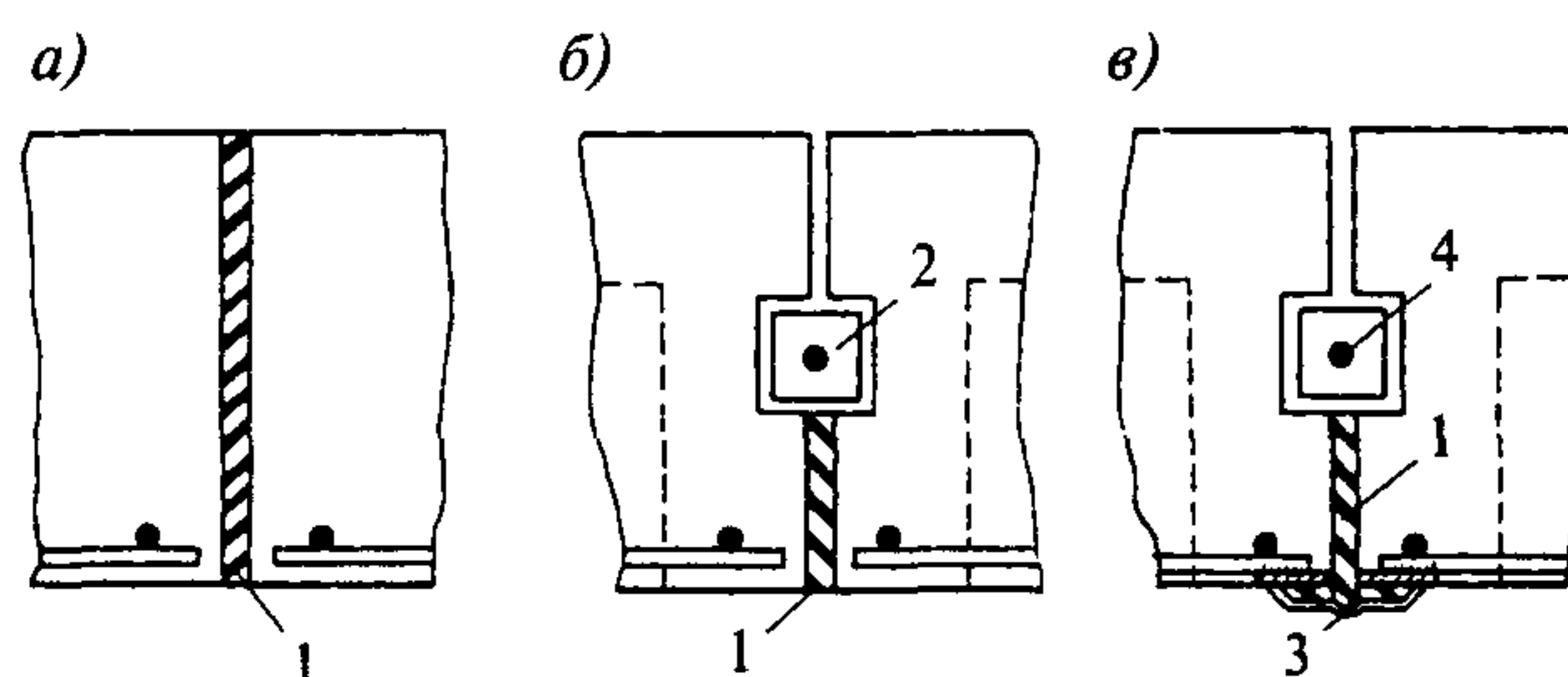
Рисунок 9.1 — Стыки элементов сборных конструкций из жаростойкого бетона
