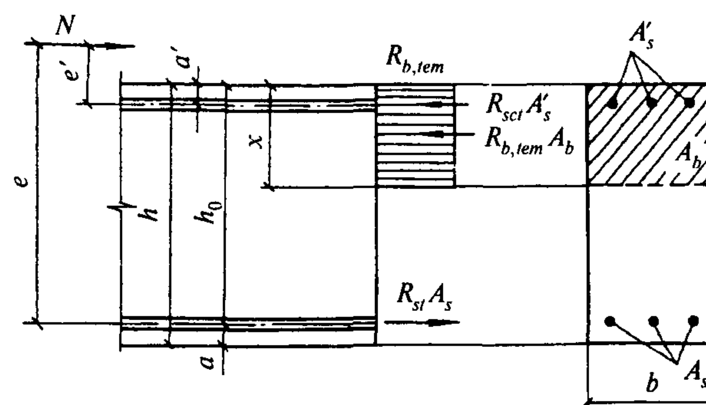
Рисунок 7.4 — Схема усилий и эпюра напряжений в сечении, нормальном к продольной оси внецентренно сжатого железобетонного элемента, при расчете его по прочности
