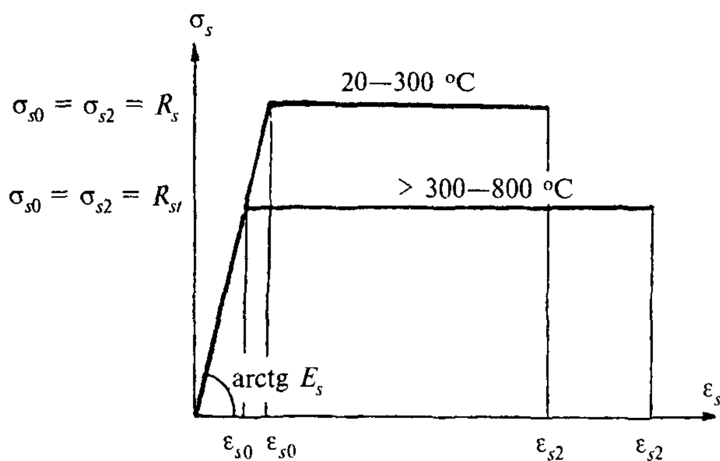
Рисунок 5.2 — Двухлинейная диаграмма растянутой арматуры
