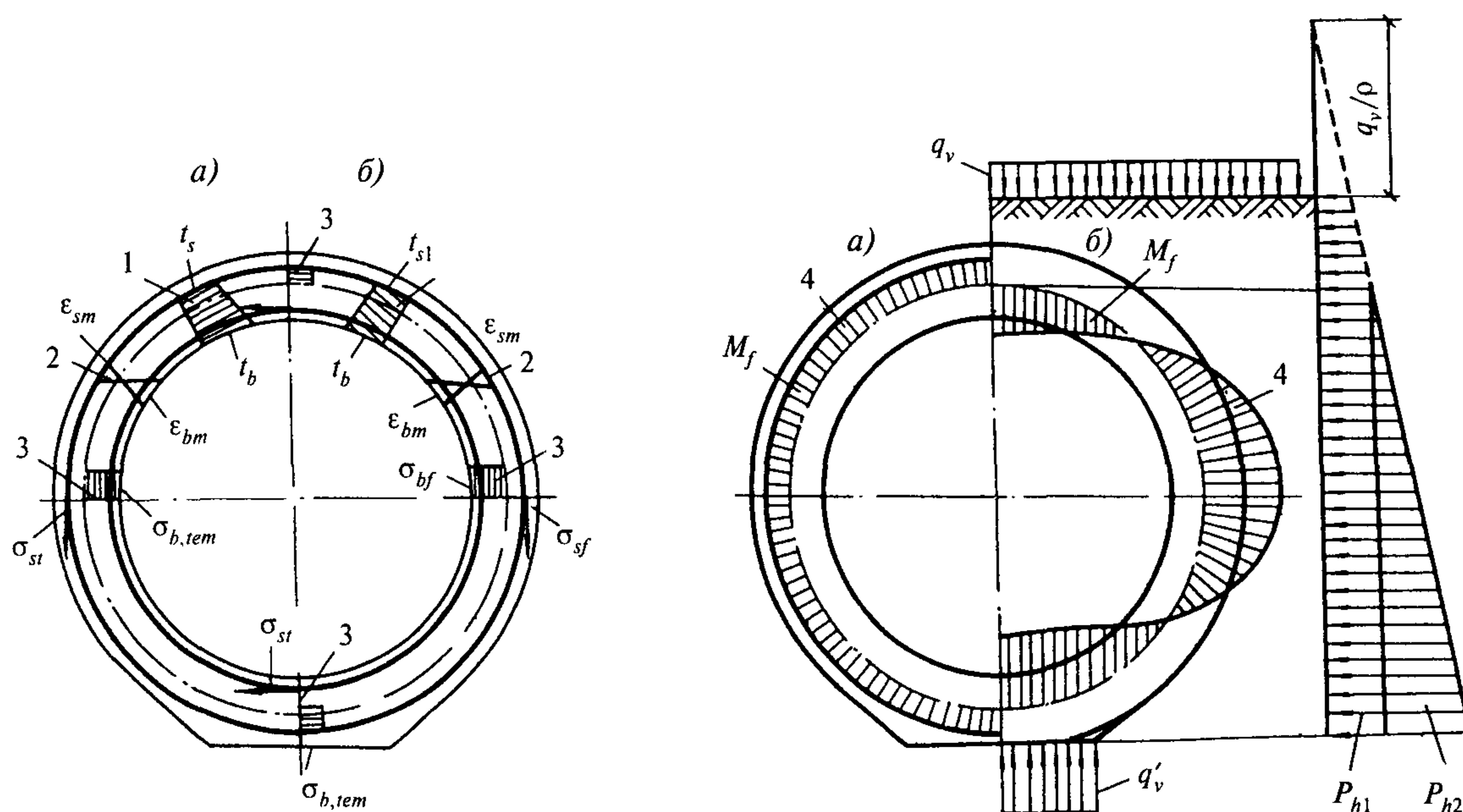
a — от воздействия температуры; б — от воздействия нагрузки; 1 — температур; 2 — деформаций; 3 — напряжений; 4 — усилий в подземном круглом железобетонном борове
