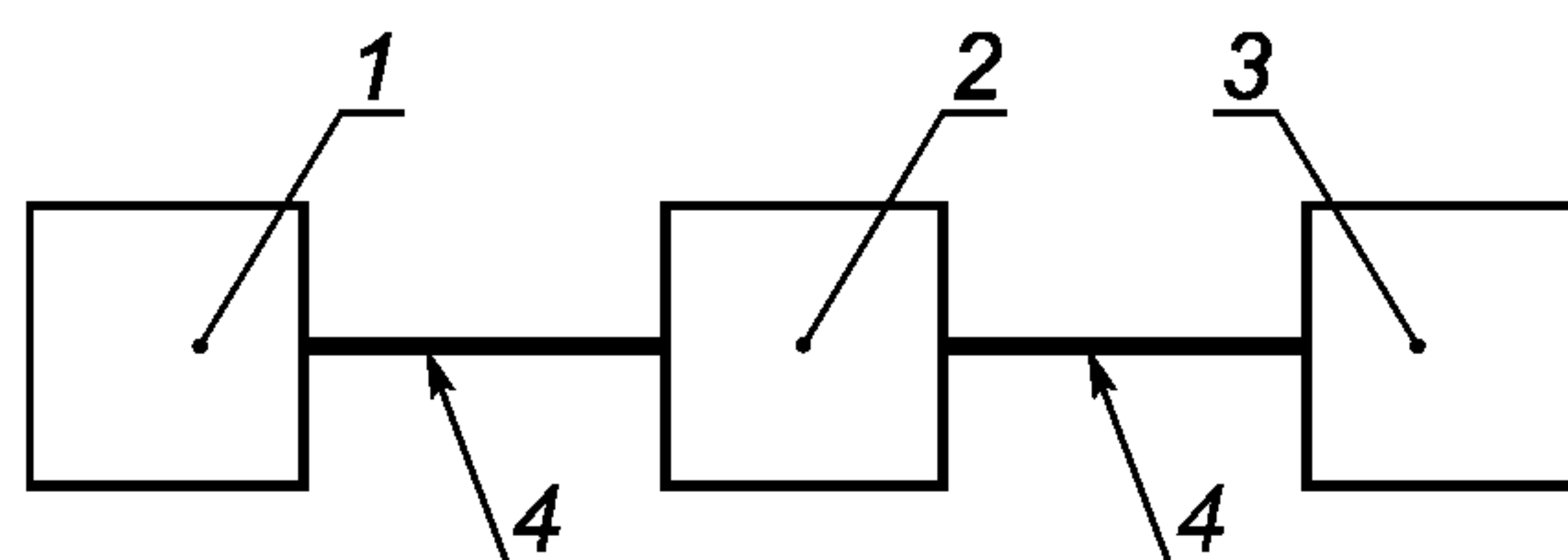
1 — измеряемая антенна с ВЧ фидером; 2 — блок питания; 3 — измеритель КСВН с индикатором; 4 — измерительный кабель
