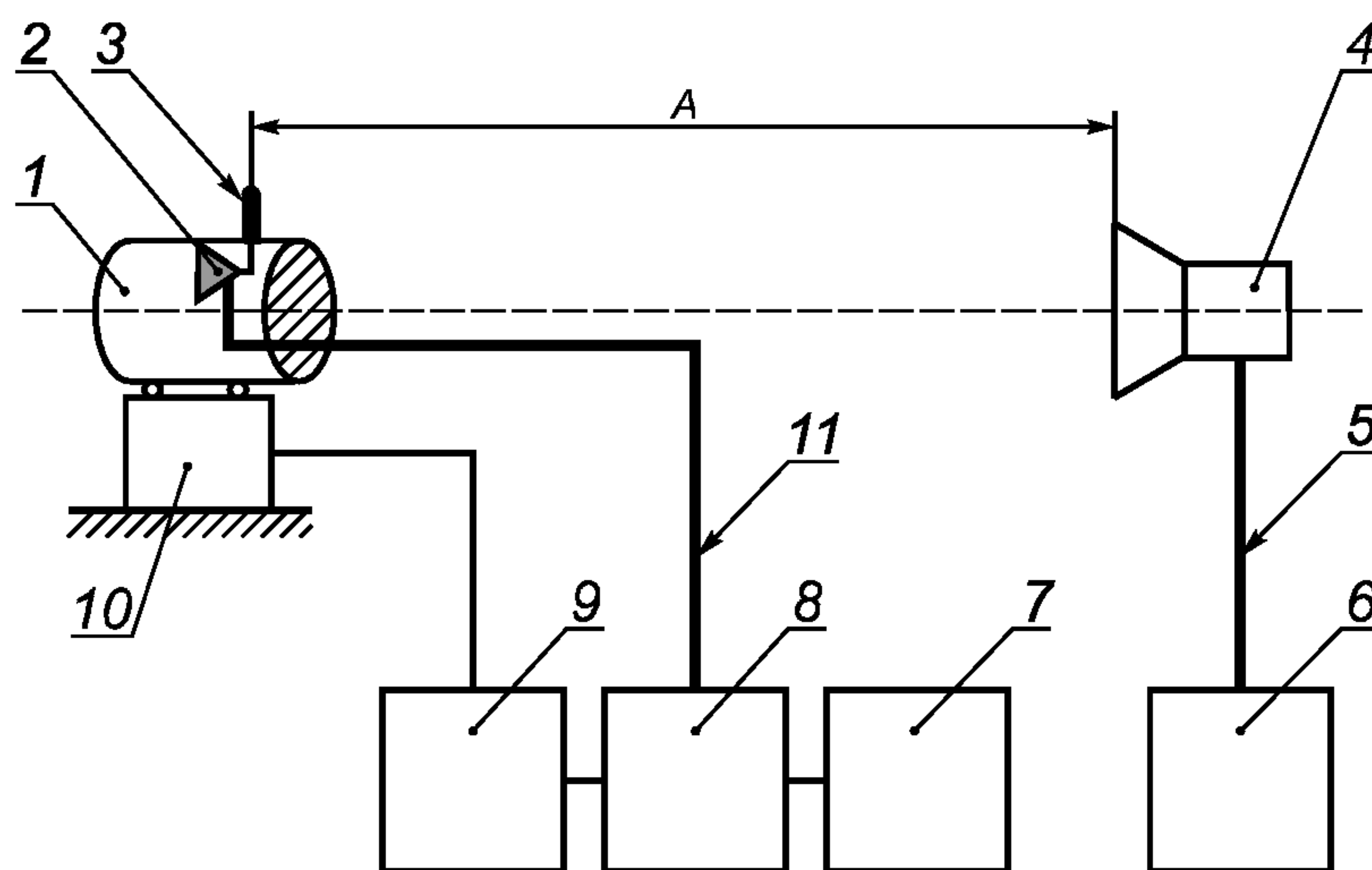
1 — фрагмент макета ВС; 2 — детекторная секция; 3 — измеряемая антенна; 4 — облучающая антенна; 5 — фидер питания; 6 — высокочастотный генератор; 7 — регистрирующее устройство (самописец, ПЭМВ+АЦП); 8 — усилитель; 9 — пульт управления; 10 — поворотное устройство; 11 — приемный тракт
