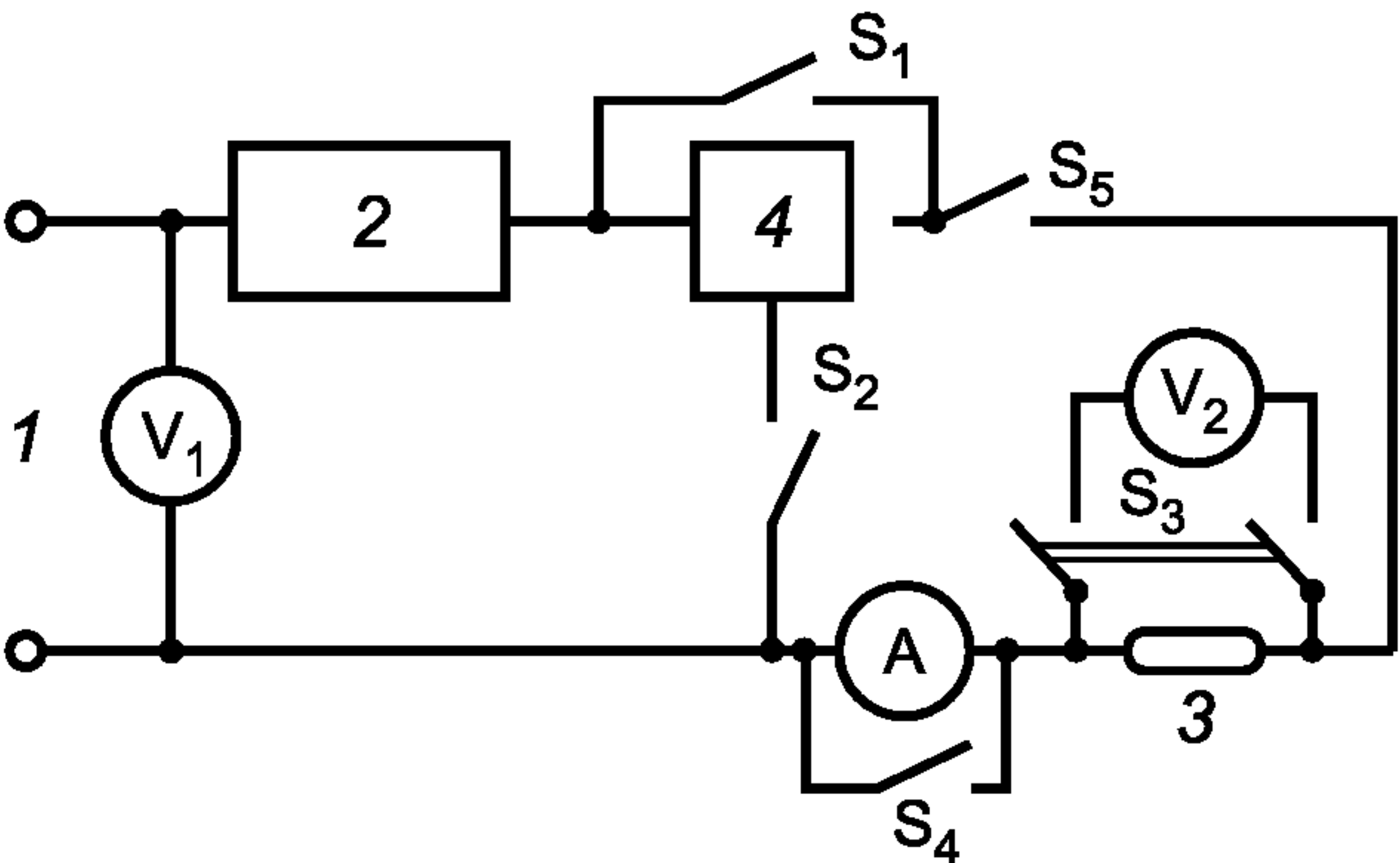
1 — синусоидальный источник питания; 2 — ДОИ; 3 — лампа; 4 — ЗУ
