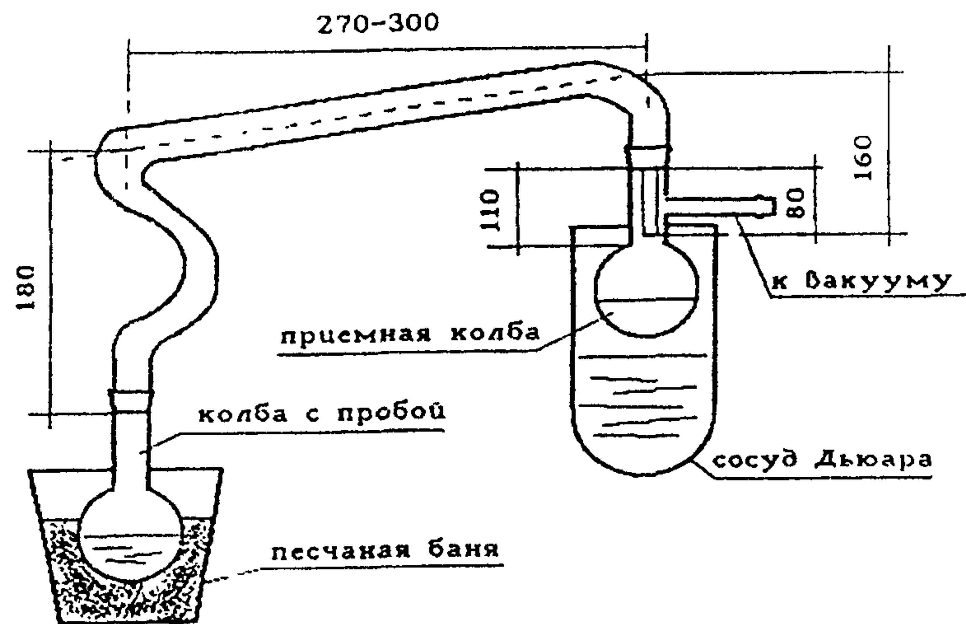
Рис. 2 СХЕМА ВАКУУМНОЙ УСТАНОВКИ.
