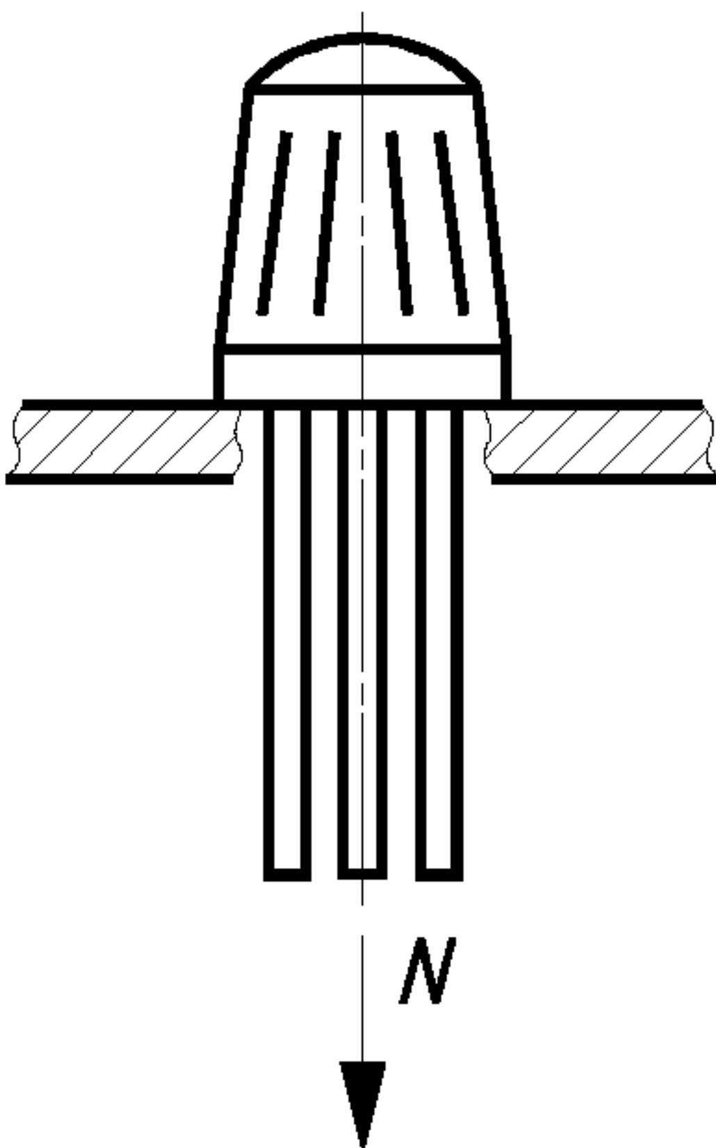
Рисунок 106 — Пример приложения усилия натяжения по оси зажима
