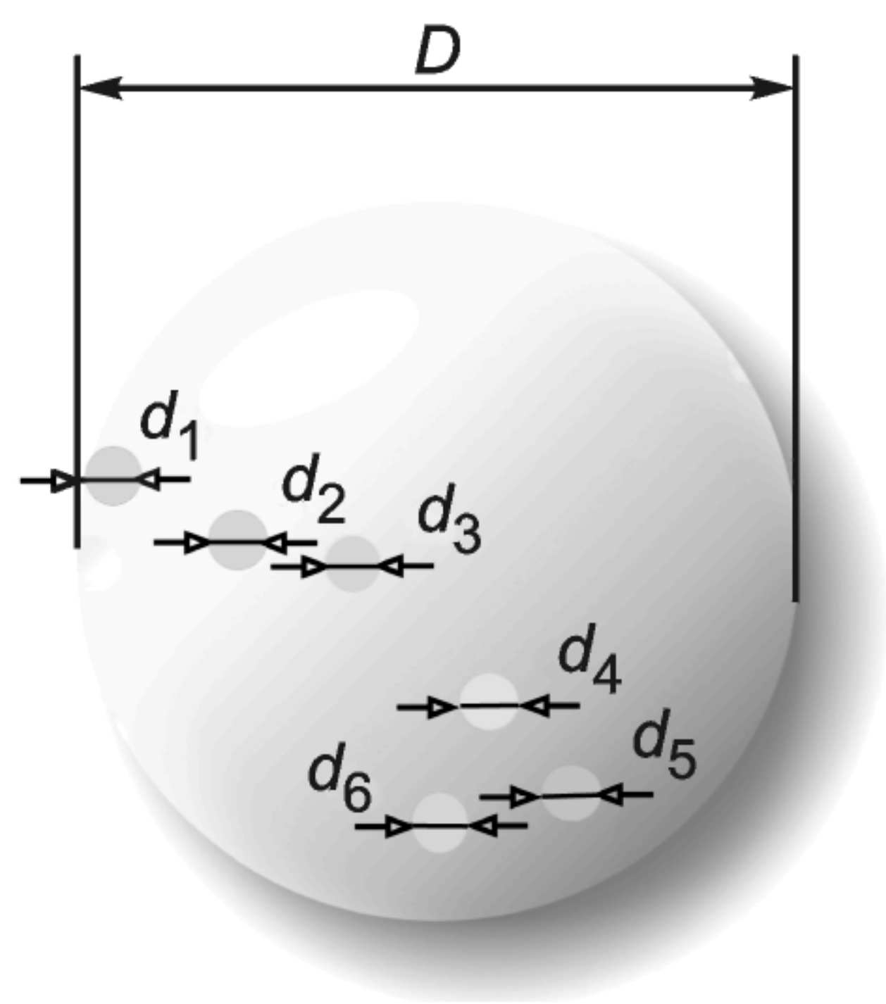
Примечание — МСШ считаются негодными при отношении (d_1 + d_2 + d_n)/D > 0,25 . Рисунок А.3 — Газообразные включения
