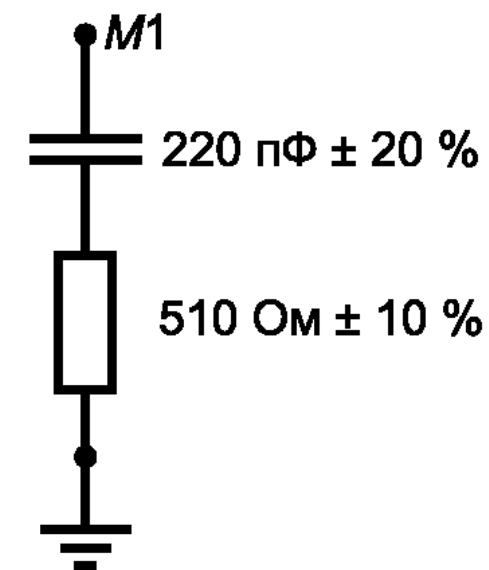
Рисунок 12 — Элемент RC для эквивалента руки (см. 7.4.2.3)
