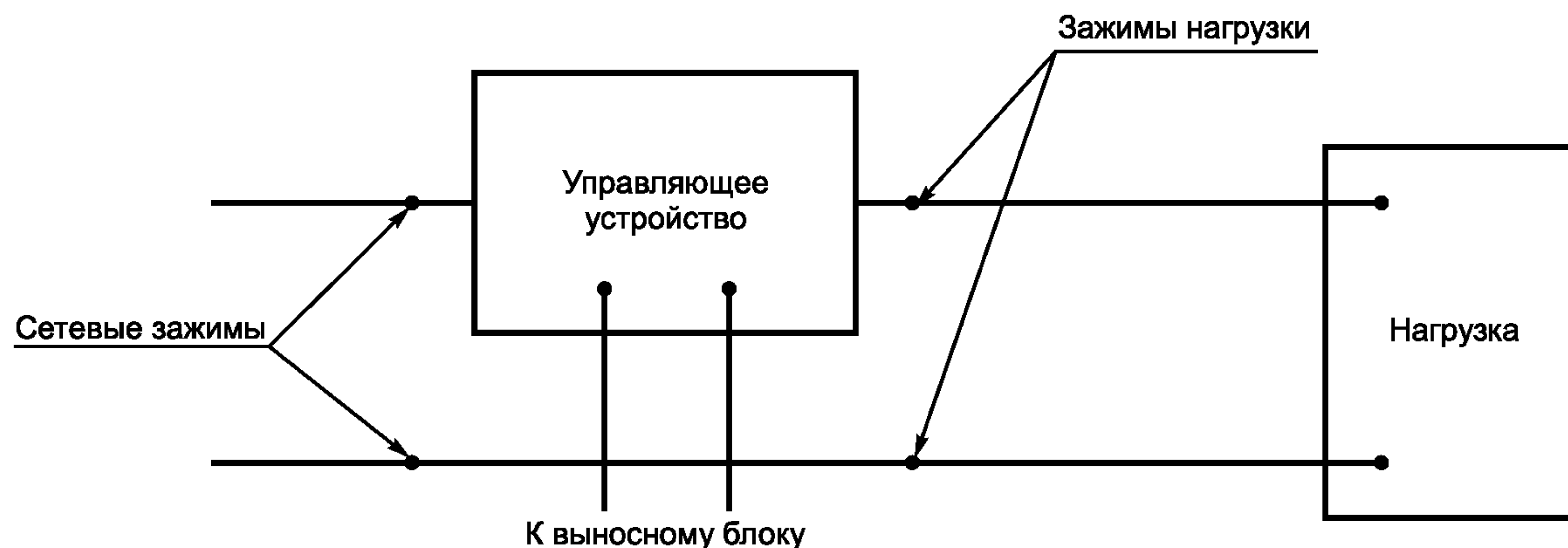
Рисунок 16а — Схема измерения для двухзажимных управляющих устройств
