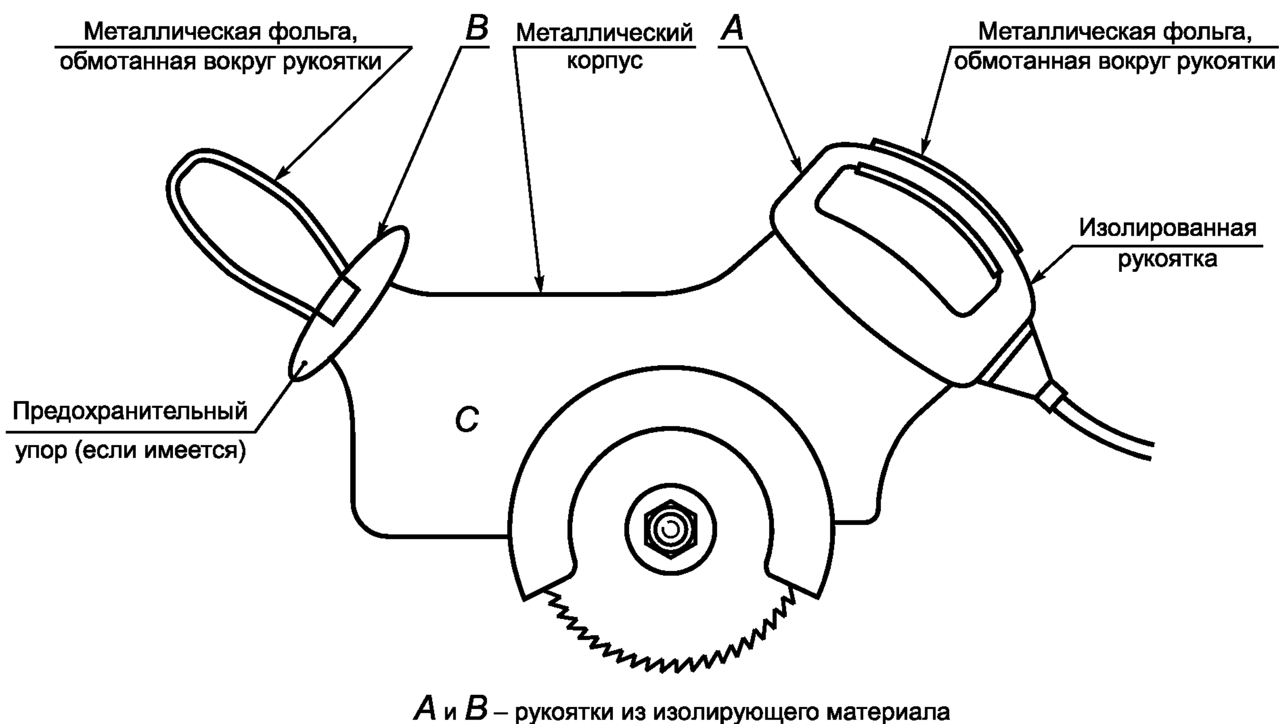
Рисунок 14 — Переносная электрическая пила с эквивалентом руки (см. 7.4.2.3)
