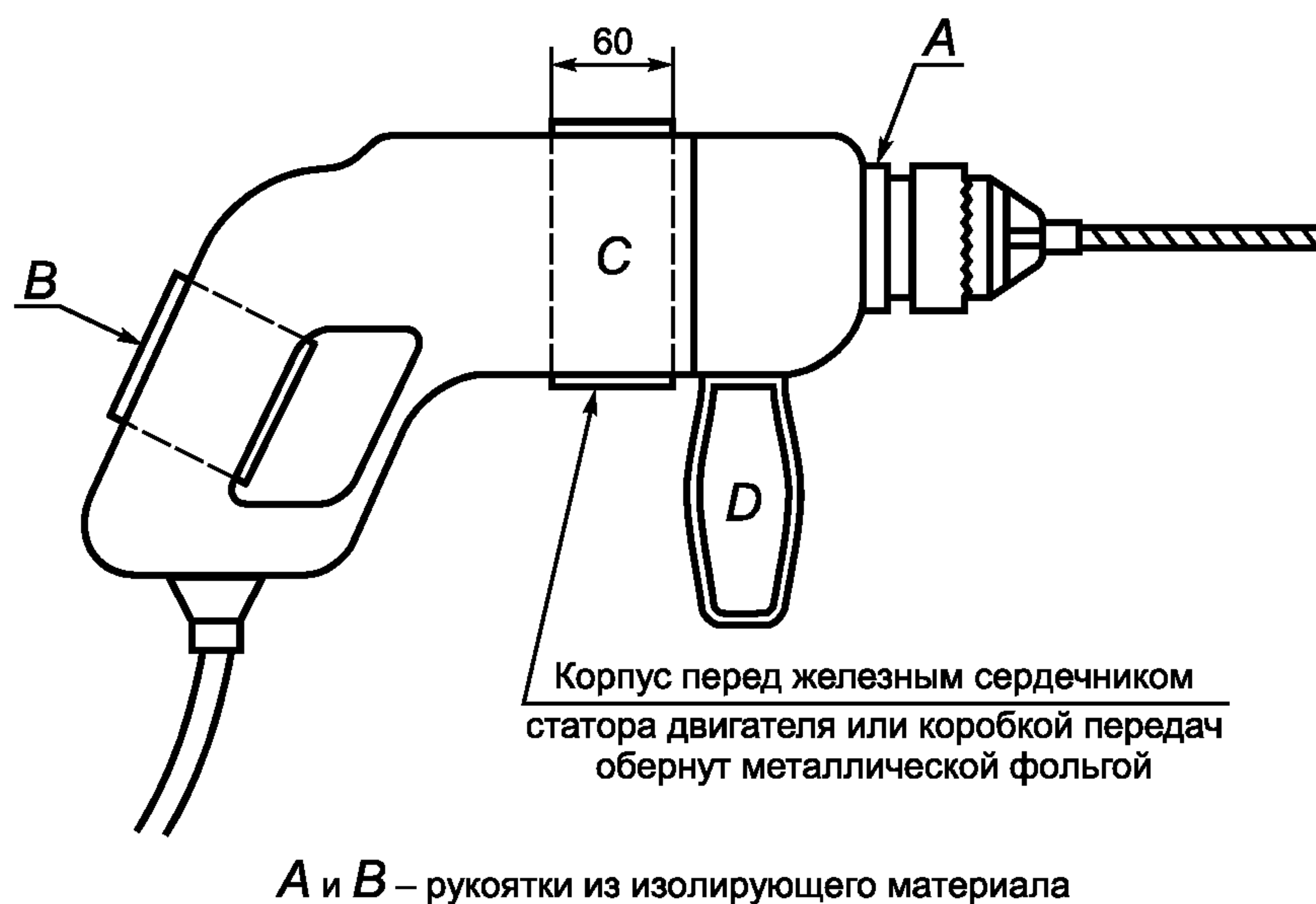
Рисунок 13 — Переносная электрическая дрель с эквивалентом руки (см. 7.4.2.3)
