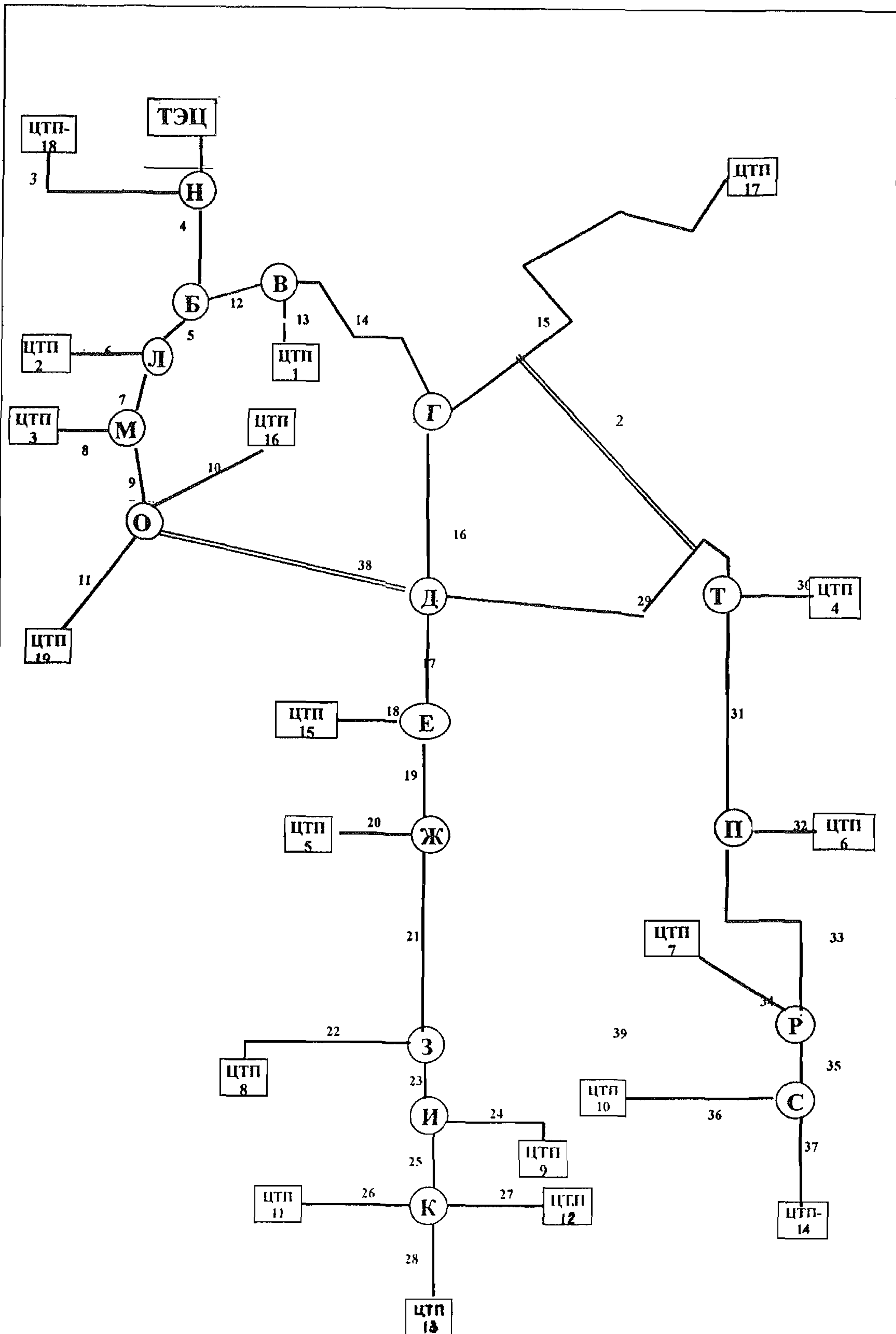
Рис. 6 Схема рекомендуемых распределительных тепловодов г. АРТЕМЬЕВСКА:
