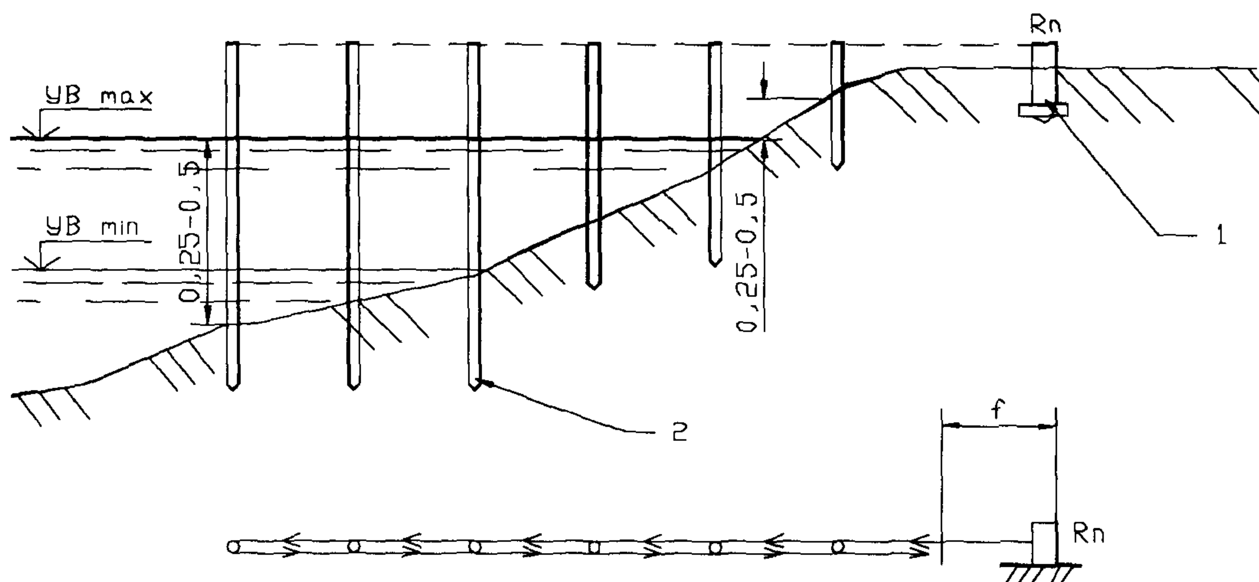
Рис. 1. Временный водомерный пост:
