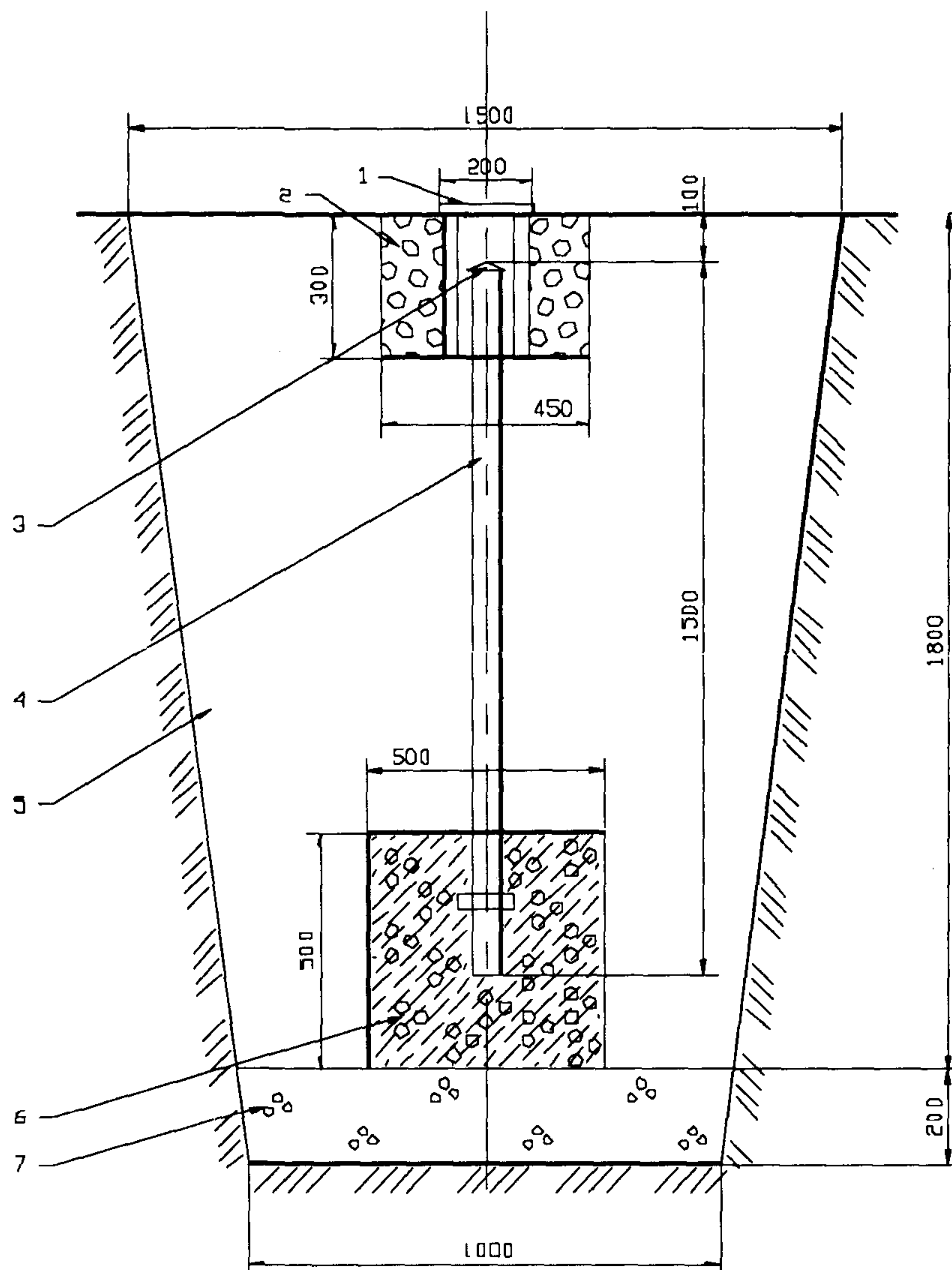
Рис. 1. Репер в виде бетонной тумбы:
