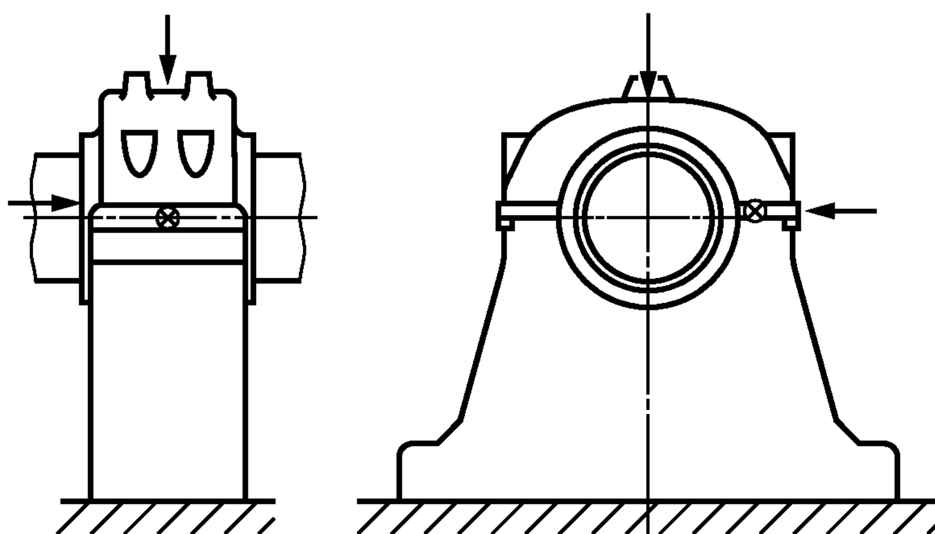
Рисунок 4 — Расположение датчиков у стояковых подшипников
