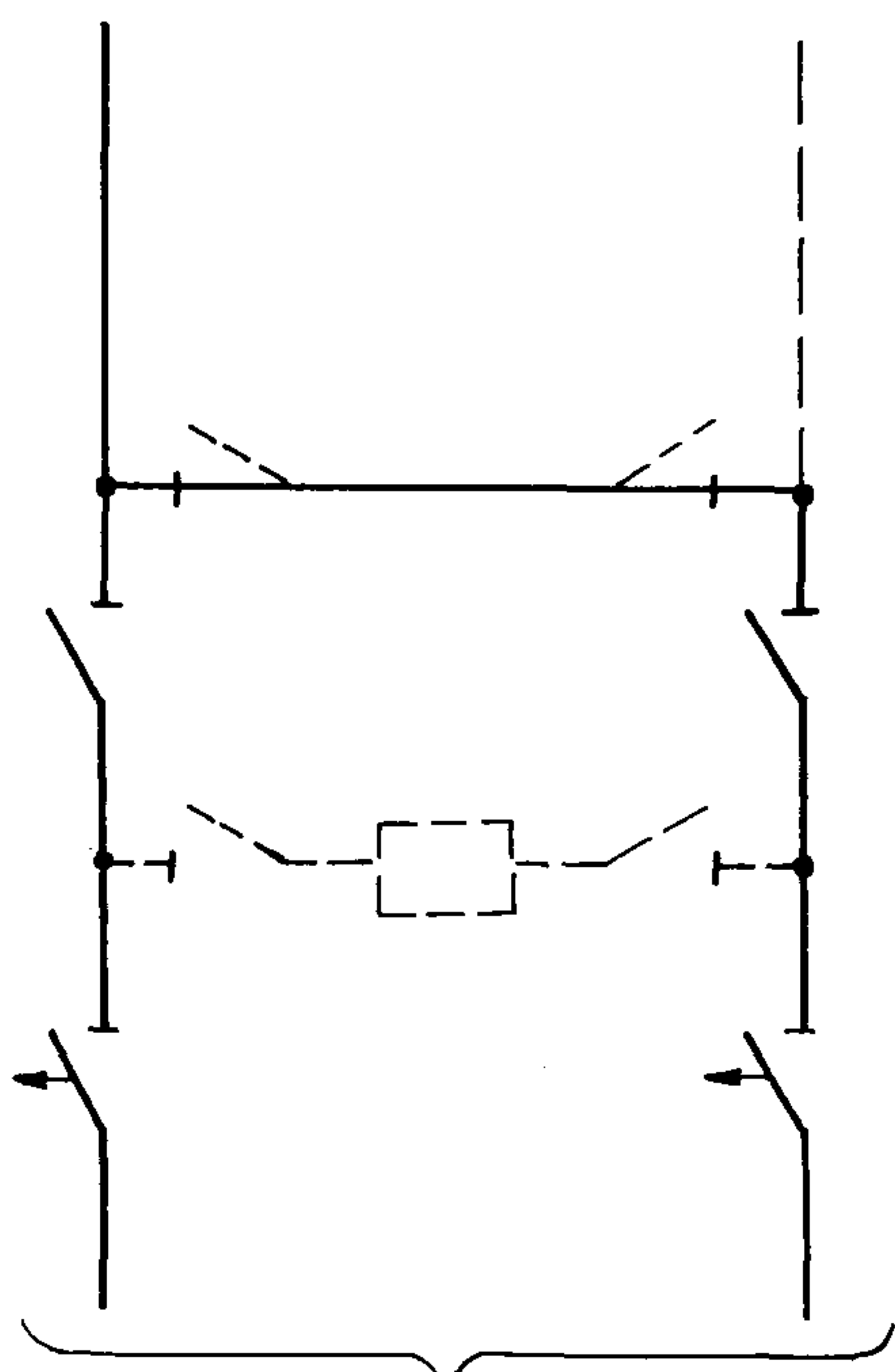
к трансформаторам а) схема 110, 220-5
