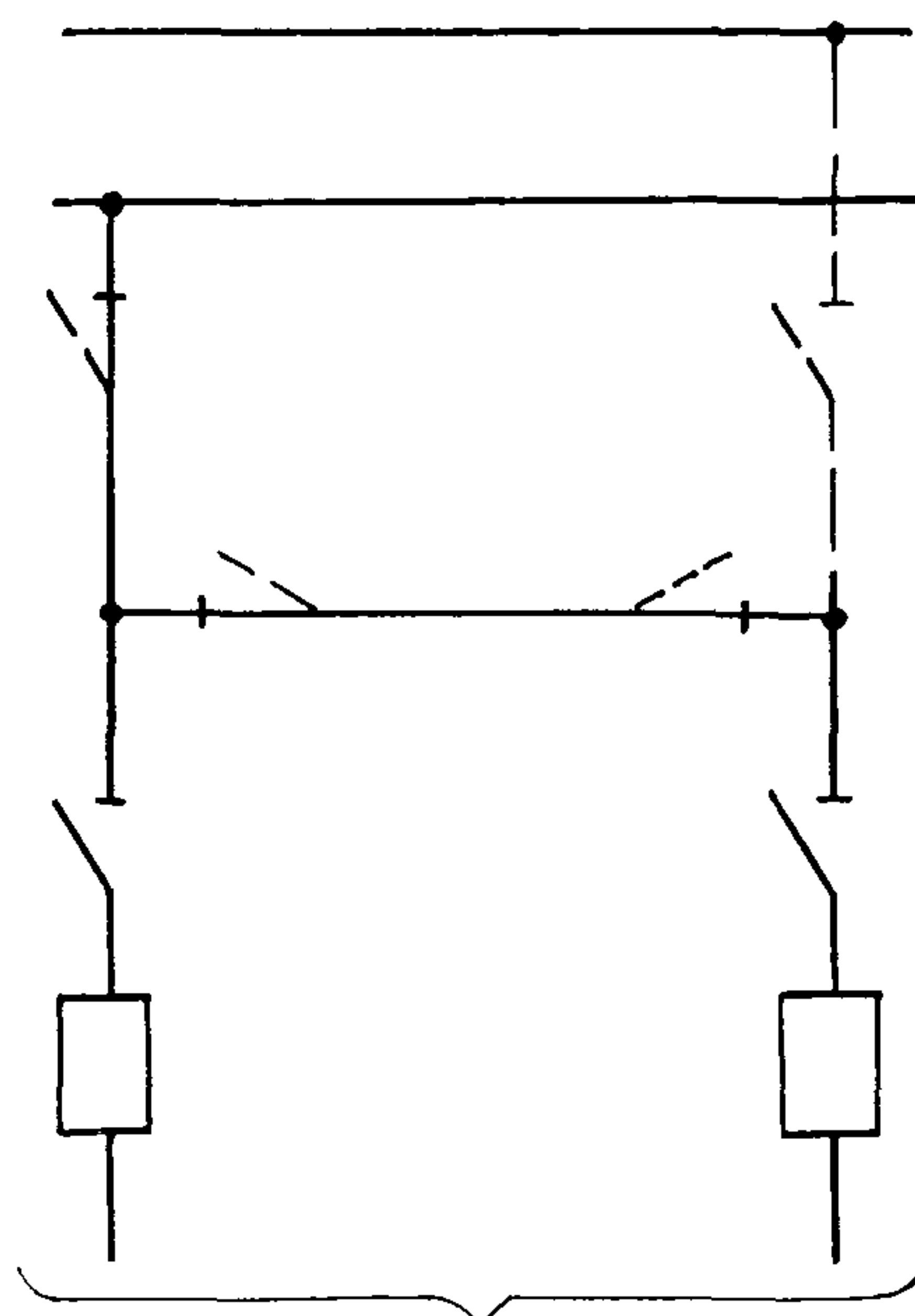
к трансформаторам б) схема 35-4Н
