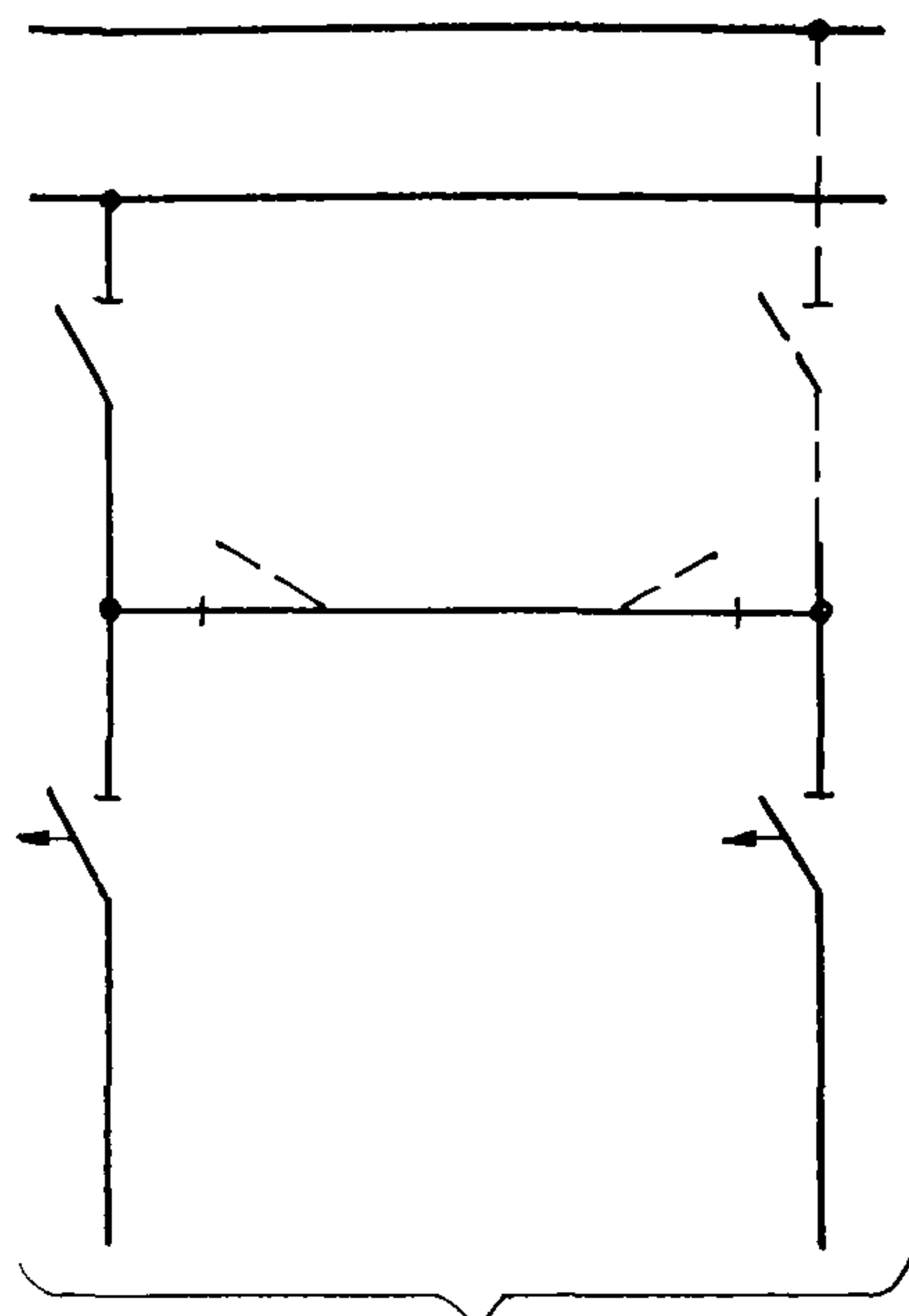
к трансформаторам а) схема 110, 220-4
