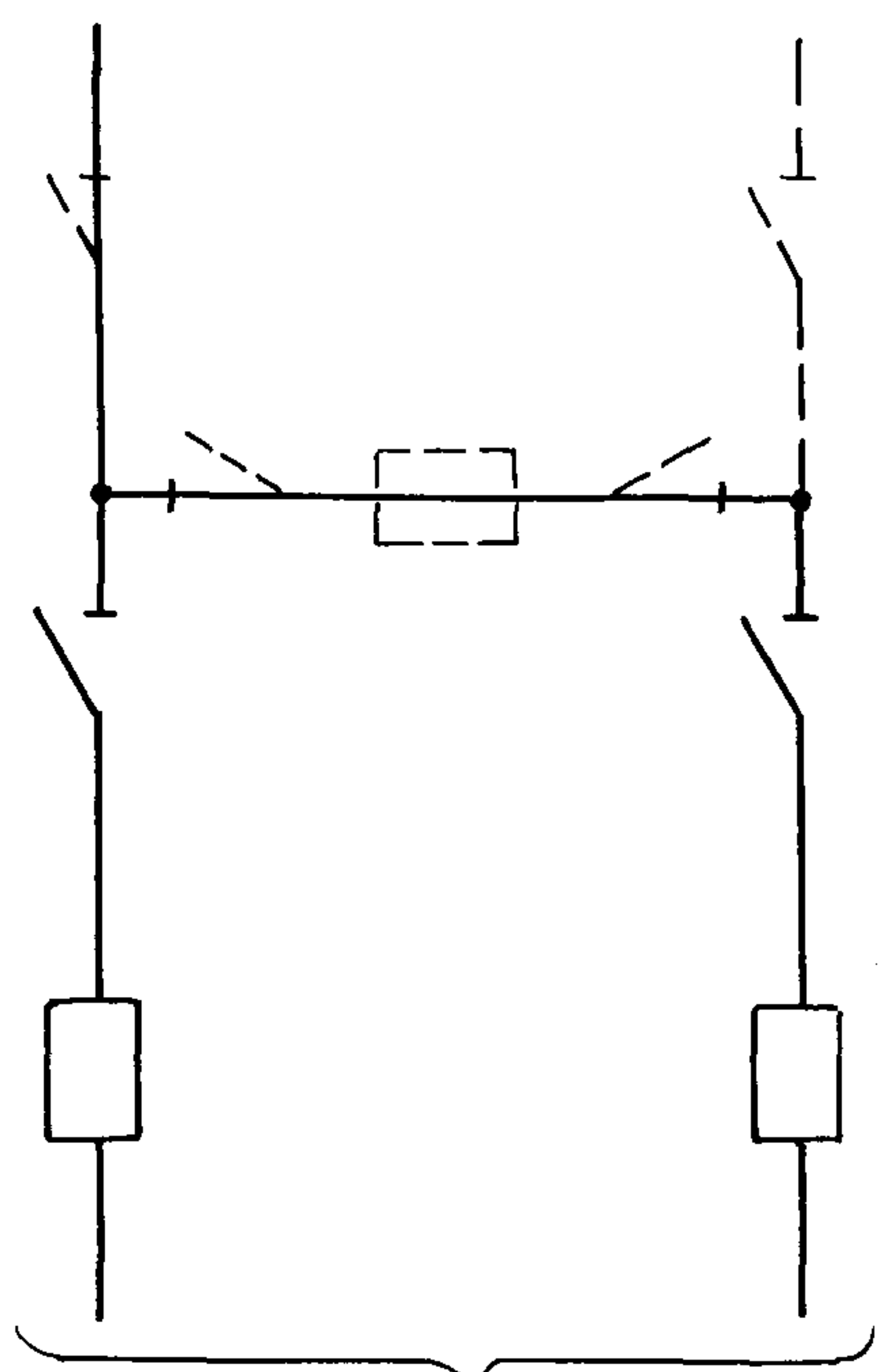
к трансформаторам б) схема 35-5АН
