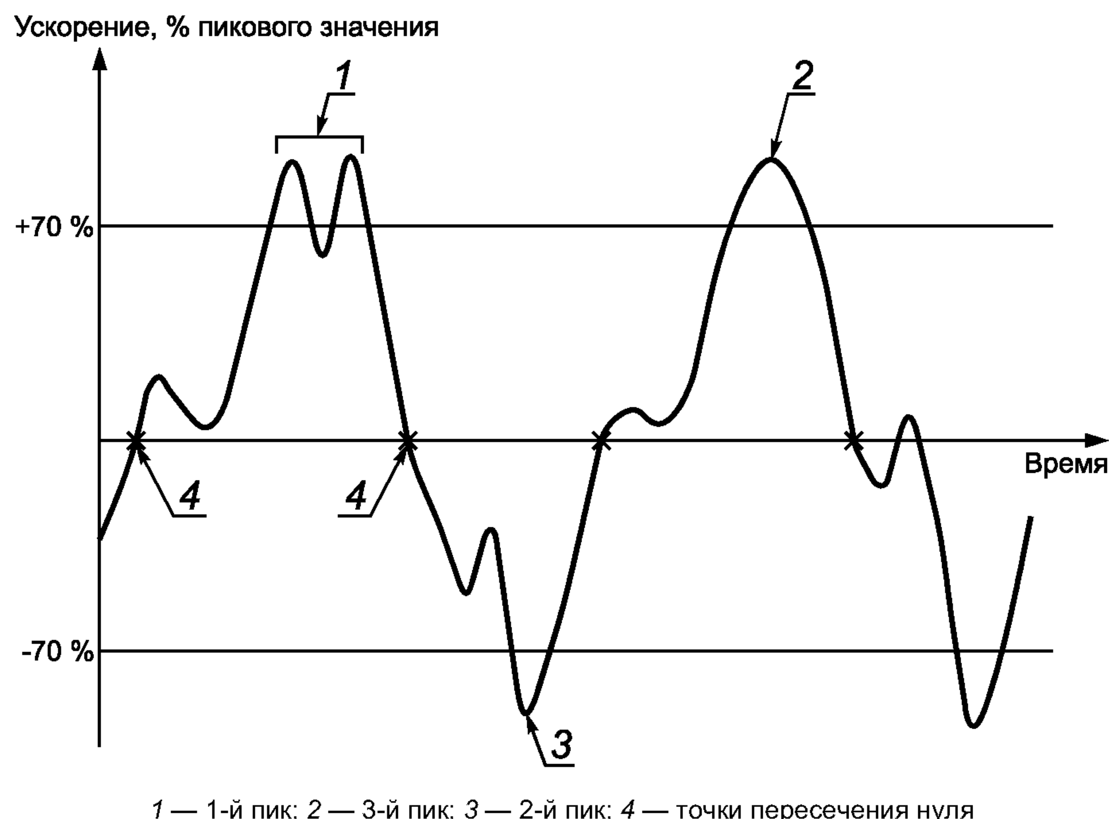
Рисунок 2 — Пример идентификации пиков отклика, превышающих пороговое значение (70 %)
