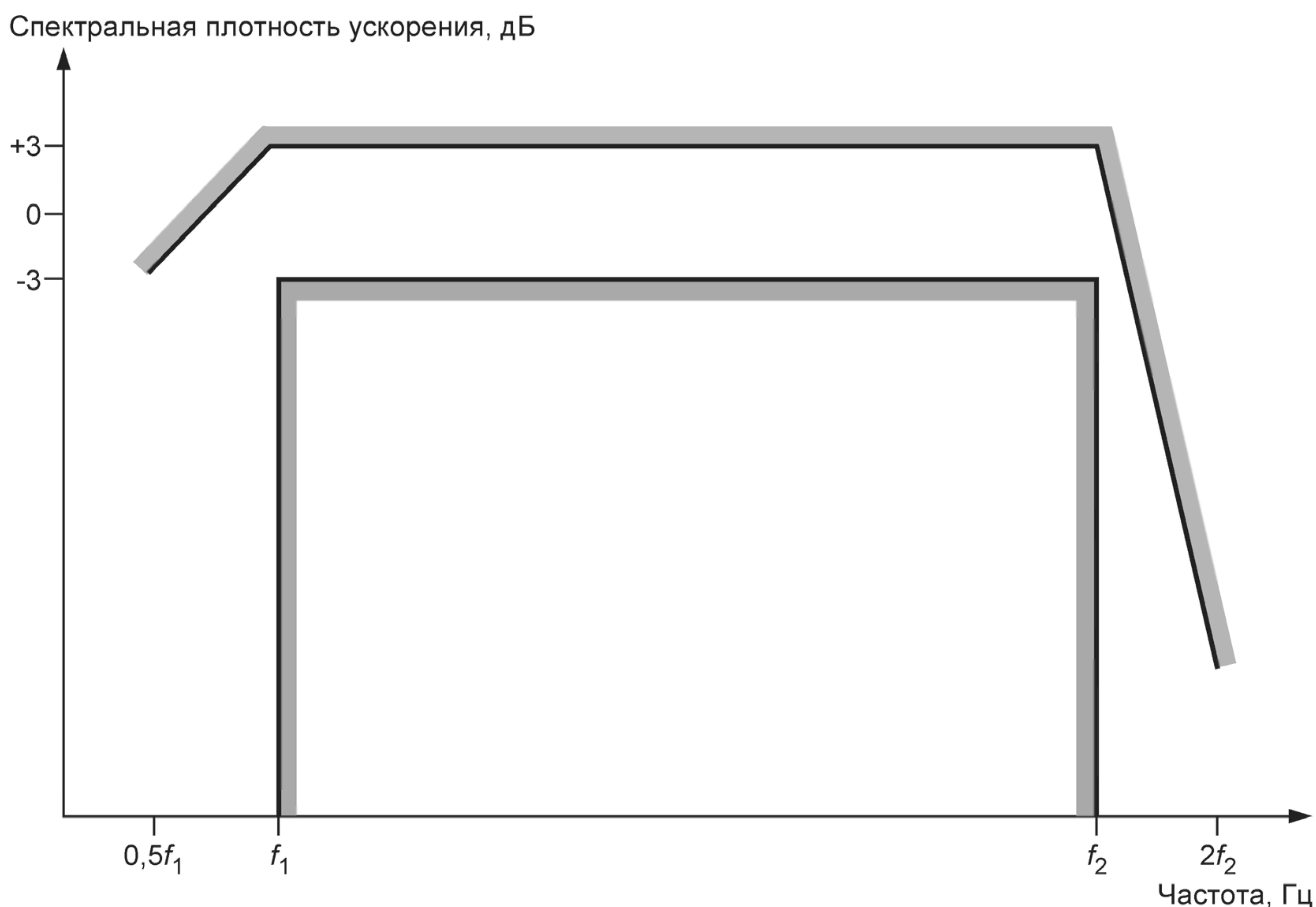
Рисунок 1 — Границы спектральной плотности ускорения (см. также 5.1.1)
