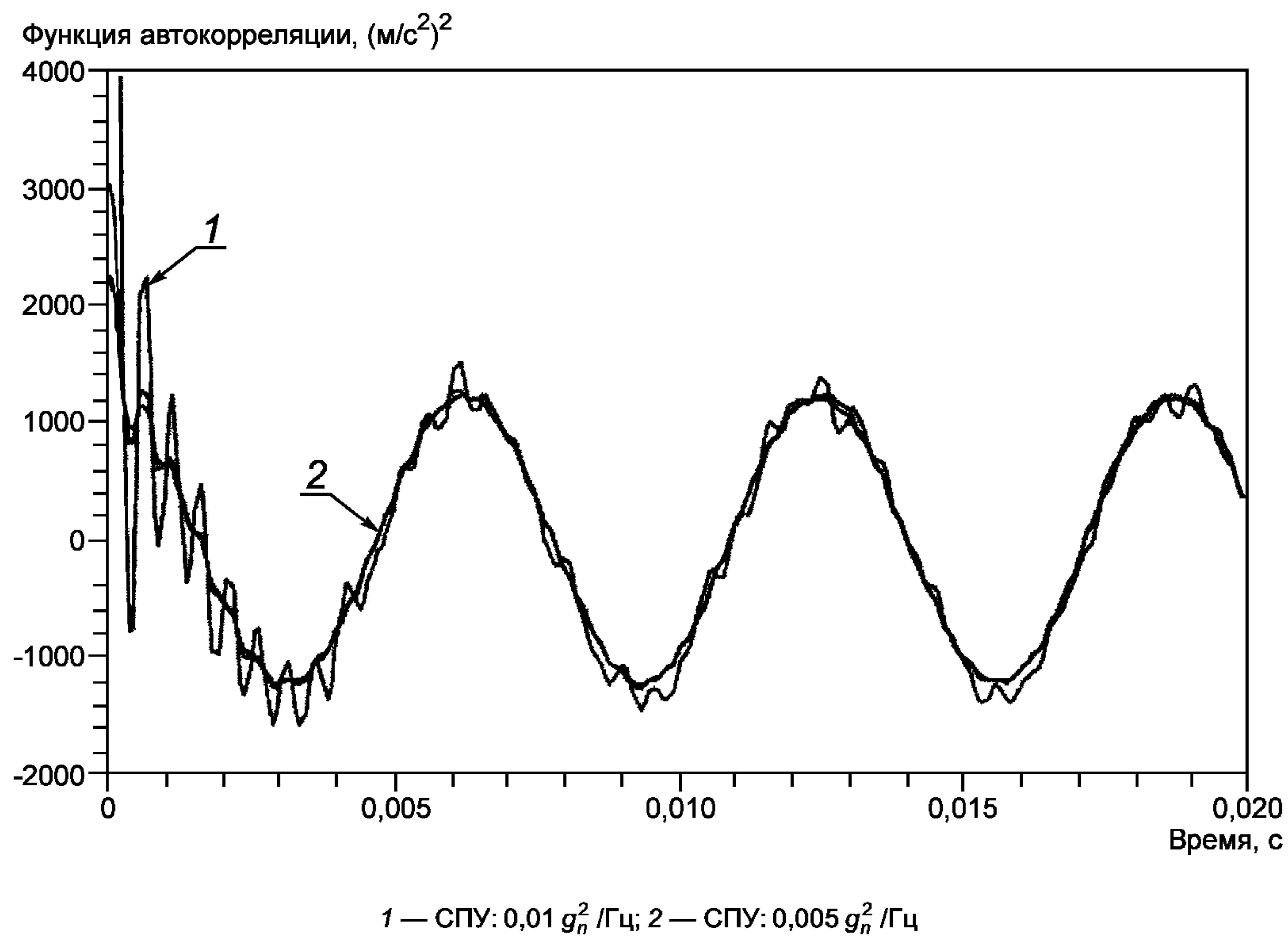
Рисунок А.3 — Автокорреляционная функция для смеси случайного шума с гармоническим сигналом на частоте 160 Гц
