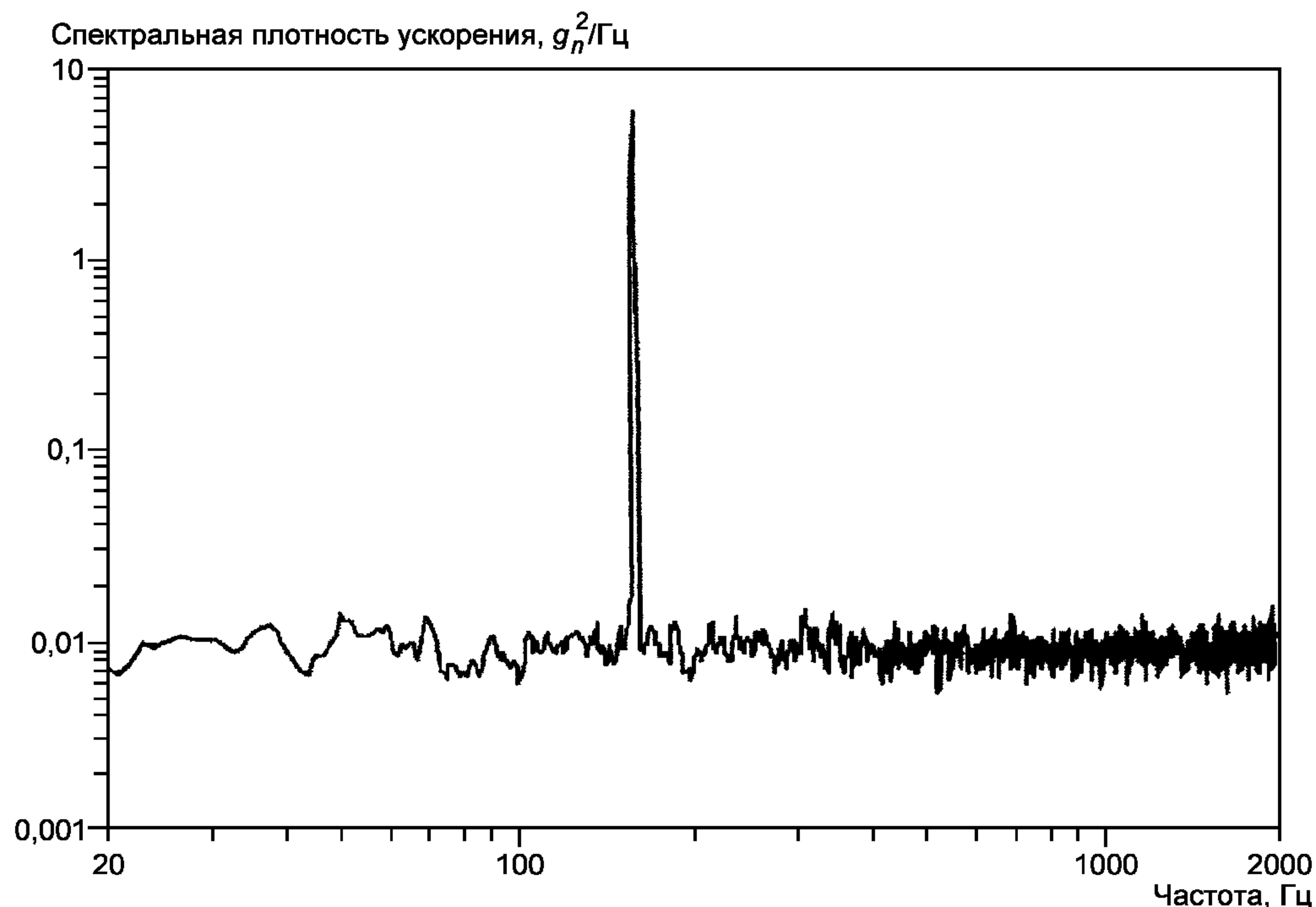
Рисунок А.1 — Гармонический сигнал на частоте 160 Гц
