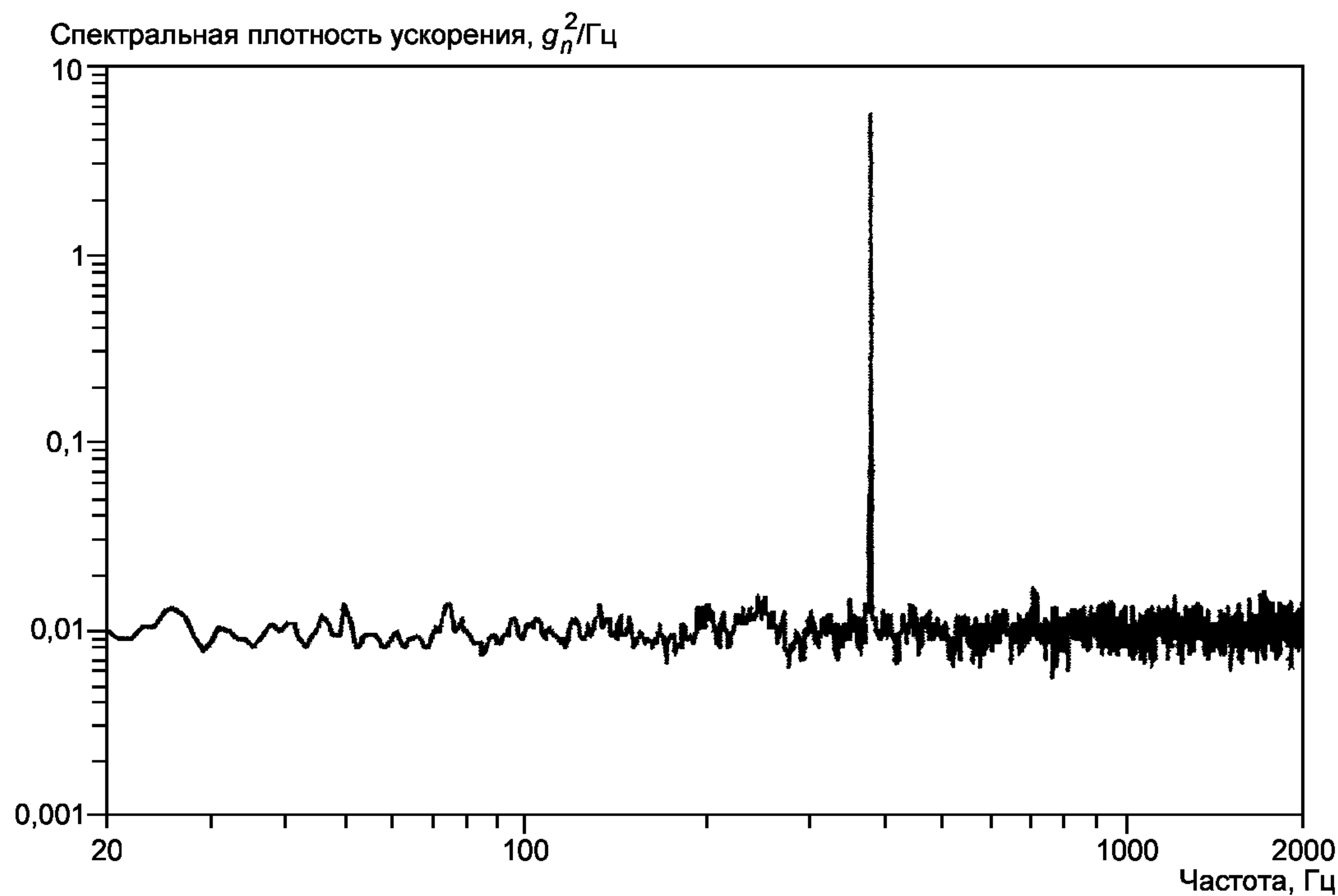
Рисунок А.2 — Гармонический сигнал на частоте 380 Гц
