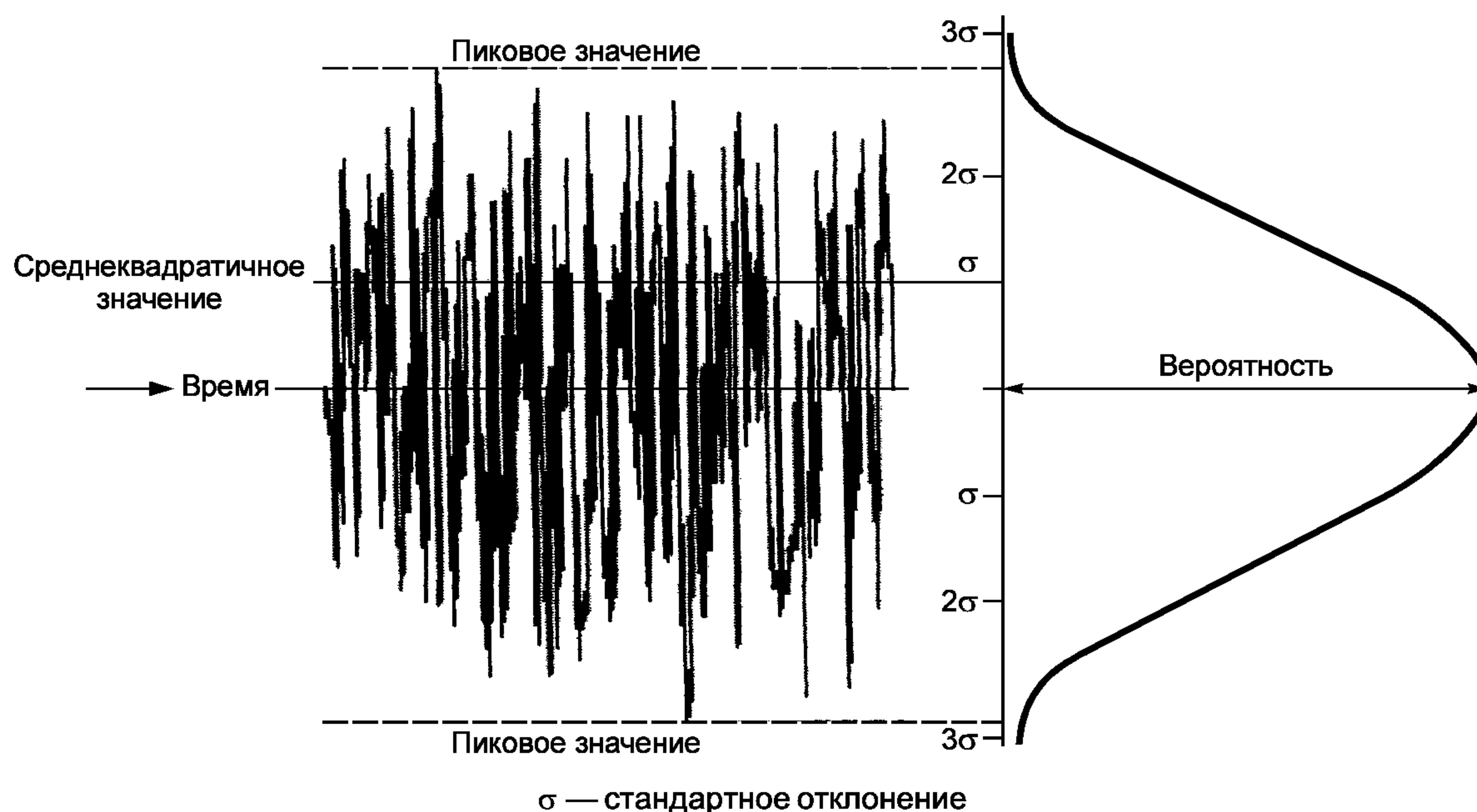
Рисунок 2 — Случайный сигнал, близкий к нормальному, с заданным уровнем отсечки
