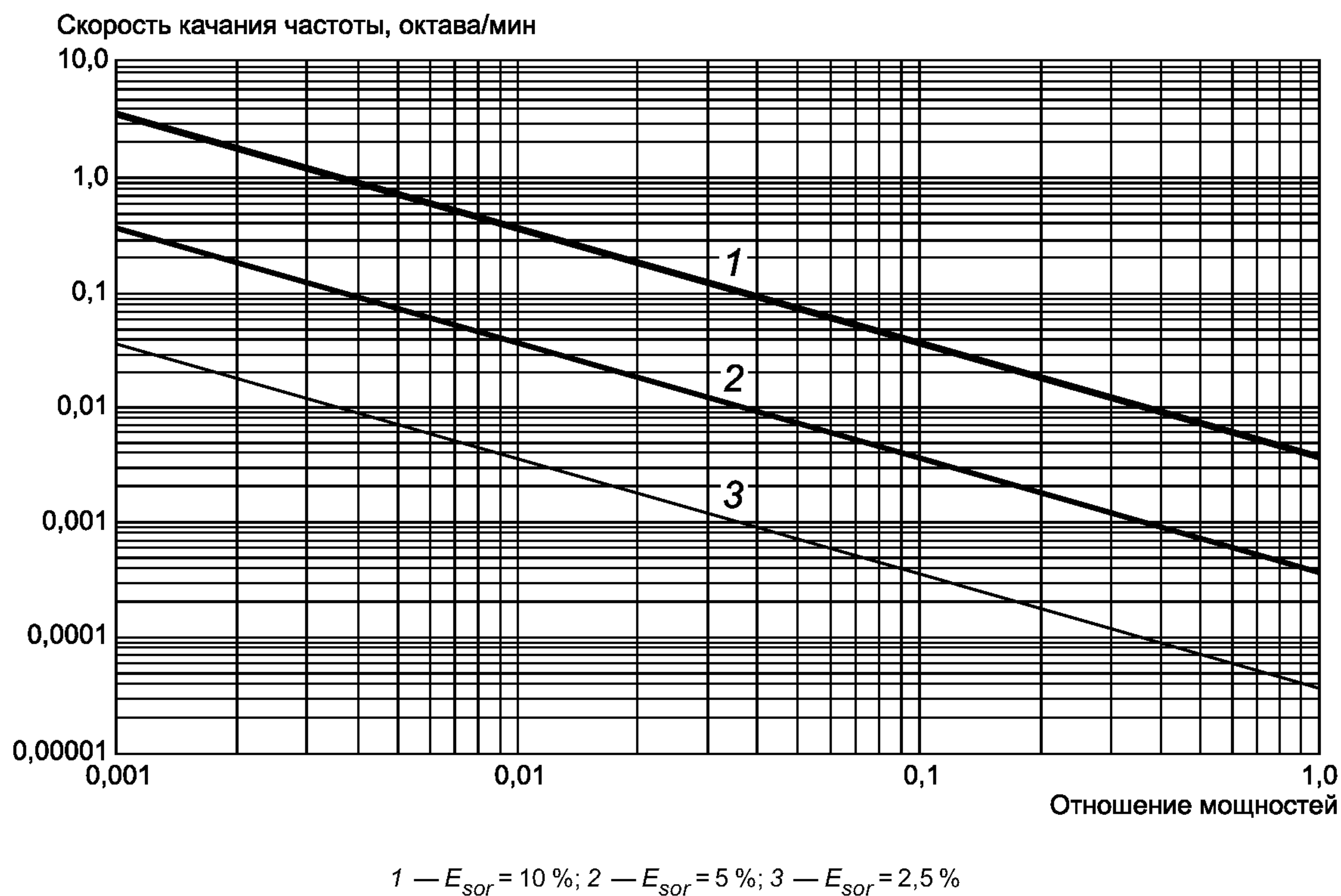
Рисунок 5 — Рекомендуемая скорость качания частоты в зависимости от отношения мощностей для разных значений E_{sor}
