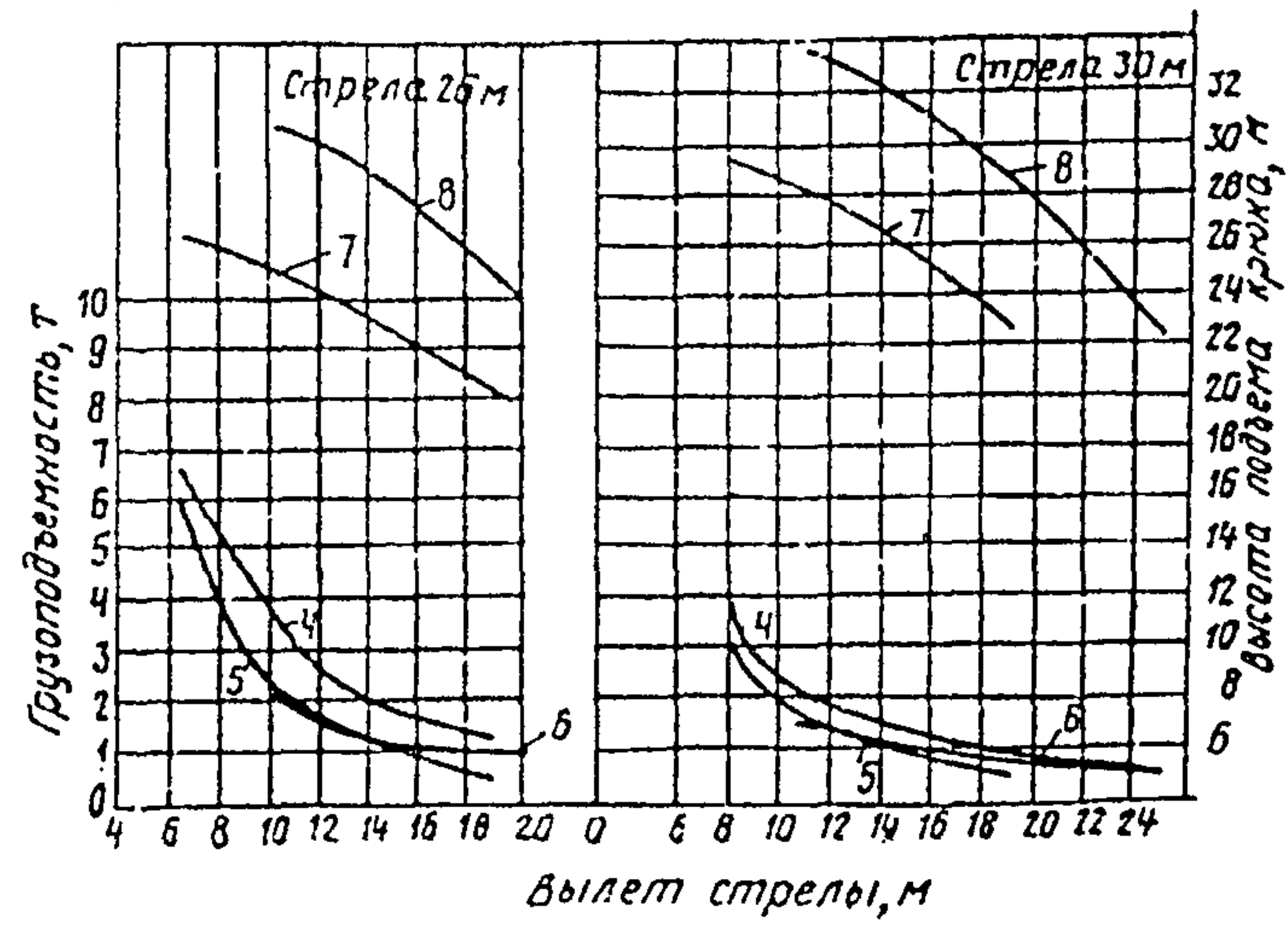
Грузовысотные характеристики крана КС-4562:
