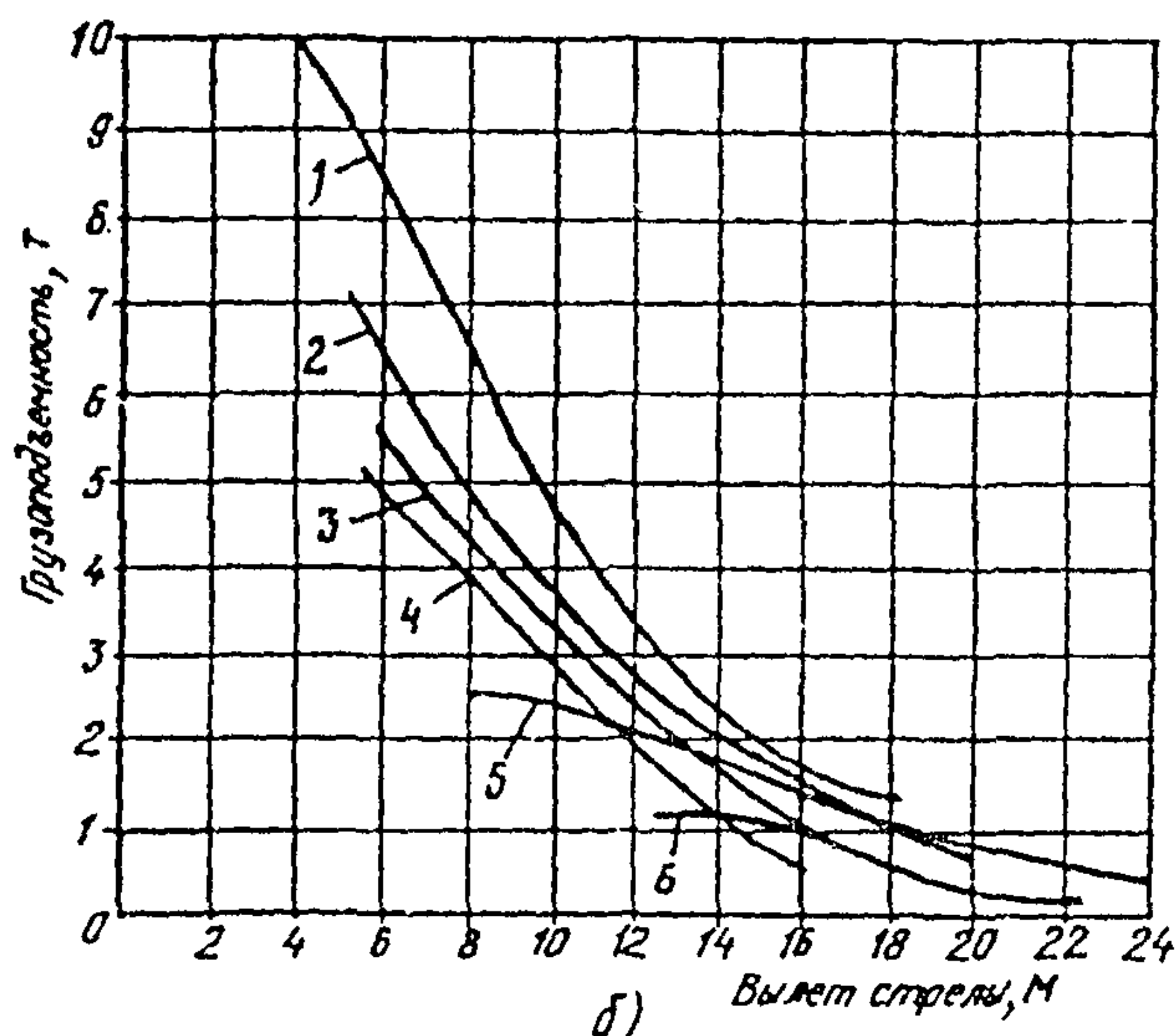
Кривые грузоподъемности крана КС-5473Б на выносных опорах (основной подъем):
