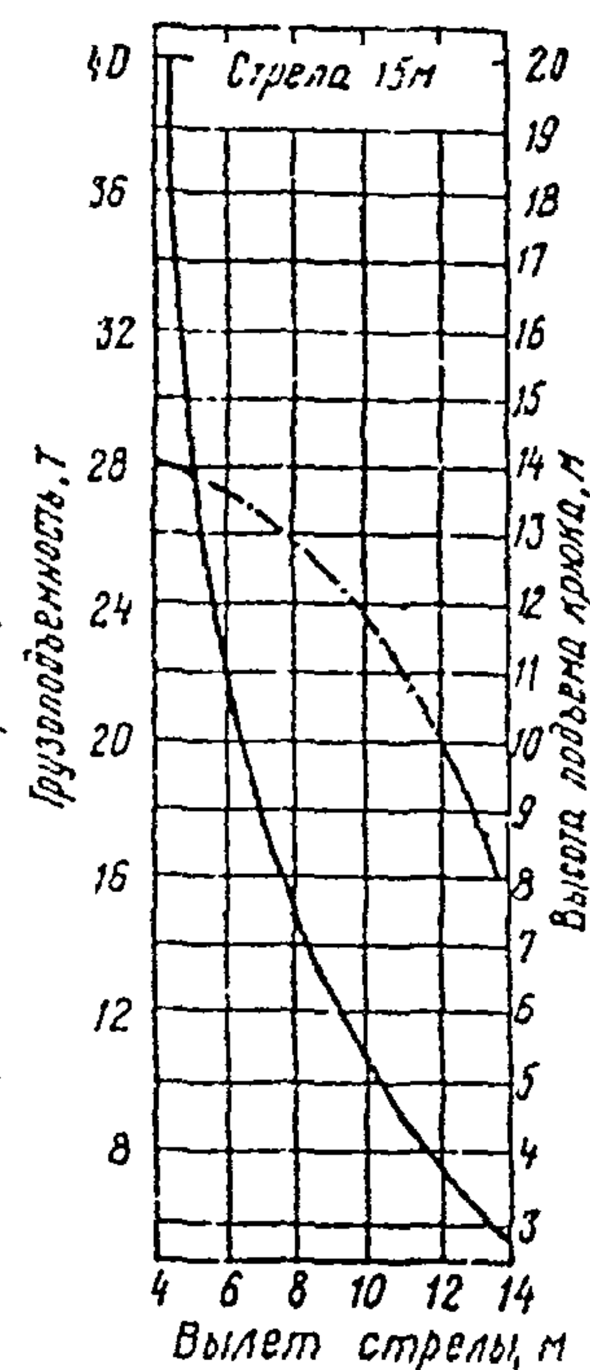
Грузовысотные характеристики крана КС-5363В с УПИ
