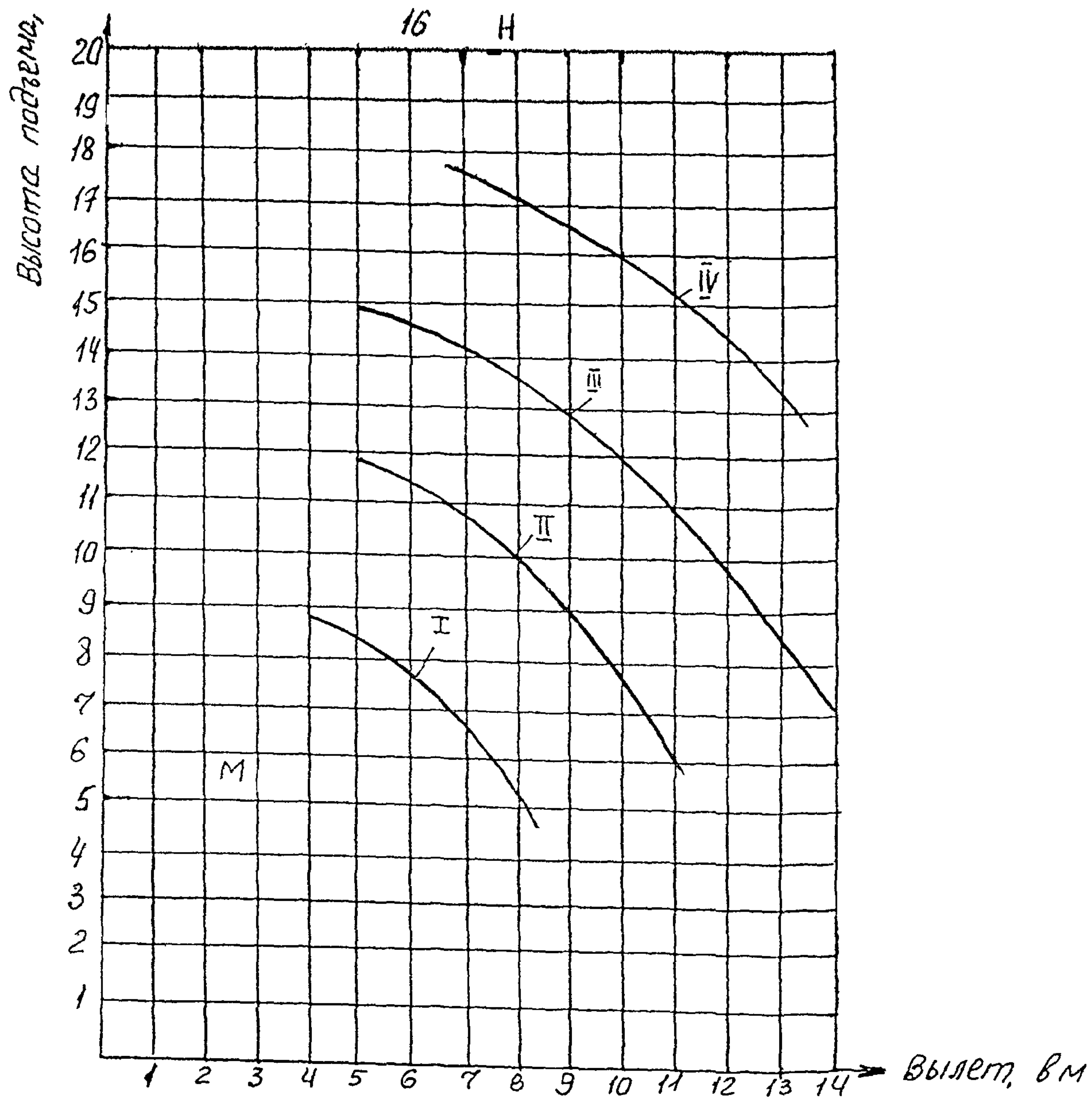
Рис.6. Диаграмма высотных характеристик стрелового крана СМК-101А I-стрела 8,6м; II-стрела 11,6м; III-стрела 14,6м; IV-стрела 17,6м; H-стрела 17,6м с гуськом; M-стрела 8,6м при перемещении с грузом.
