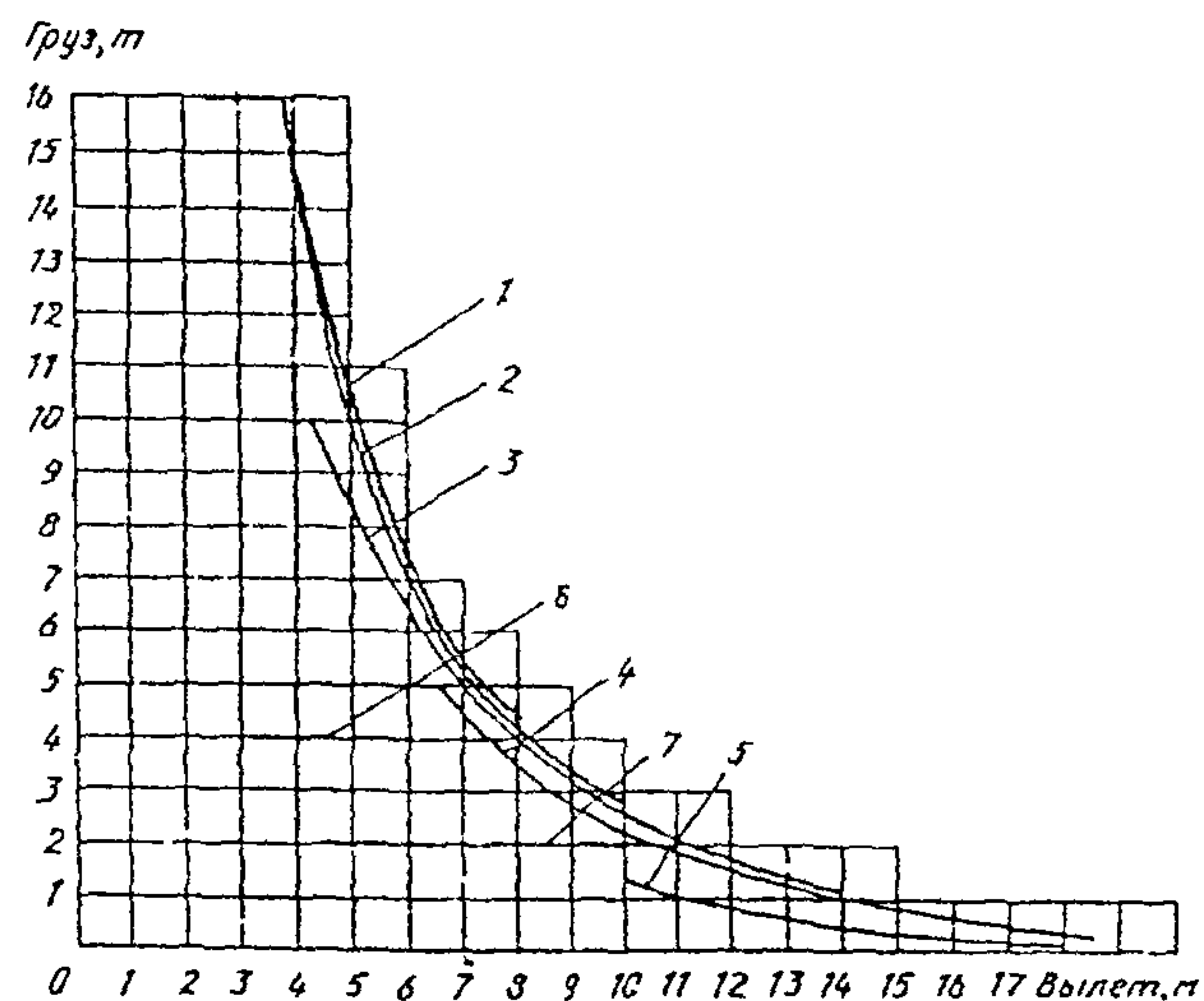
Кривые грузоподъемности крана КС-4572А на выносных опорах:
