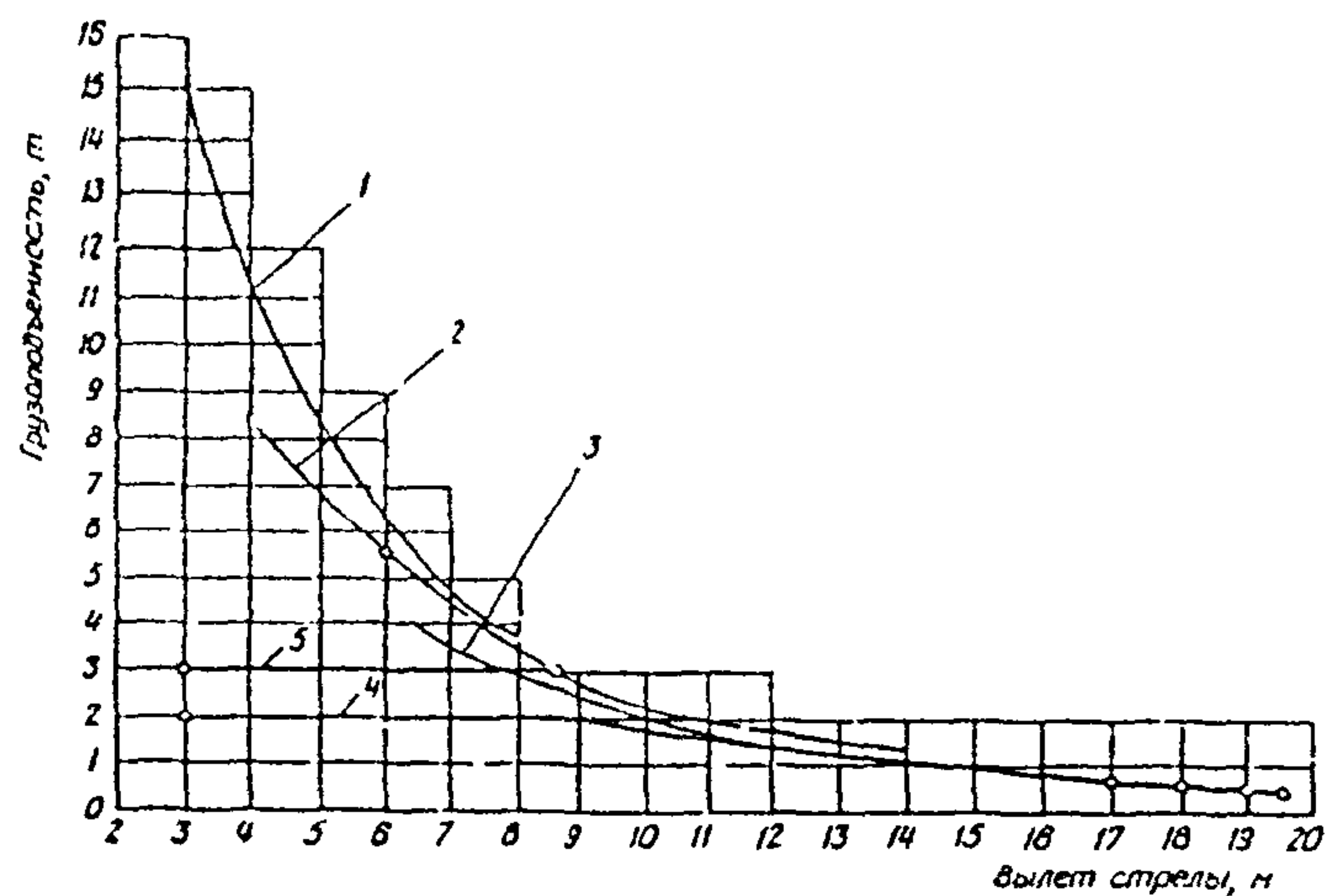
Кривые грузоподъемности крана КС-3578 на выносных опорах:
