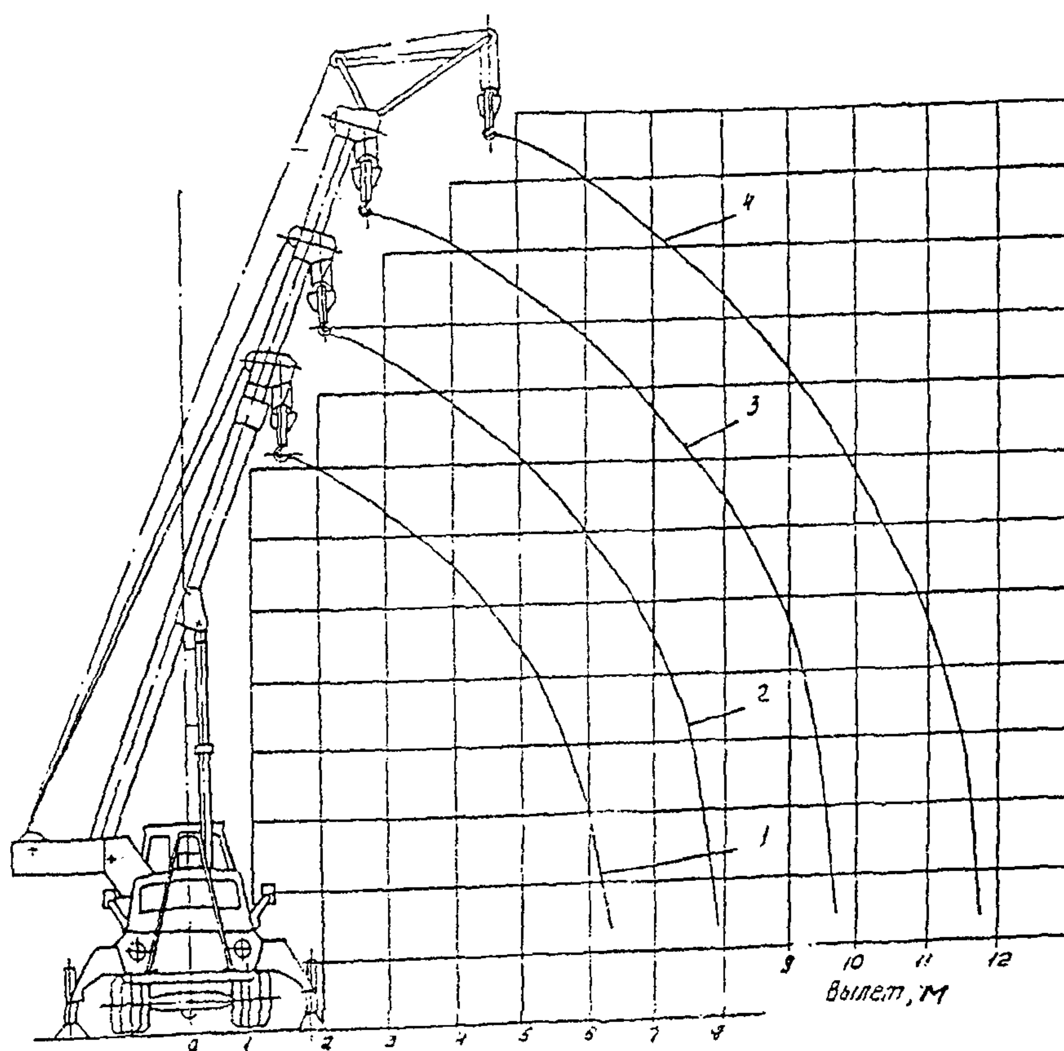
Кривые высоты подъема крюка крана КС-2571А-1: 1 — на стреле 7,3 м; 2 — на стреле 9 м; 3 — на стреле 10,8 м; 4 — на стреле 10,8 м с гуськом 2,2 м
