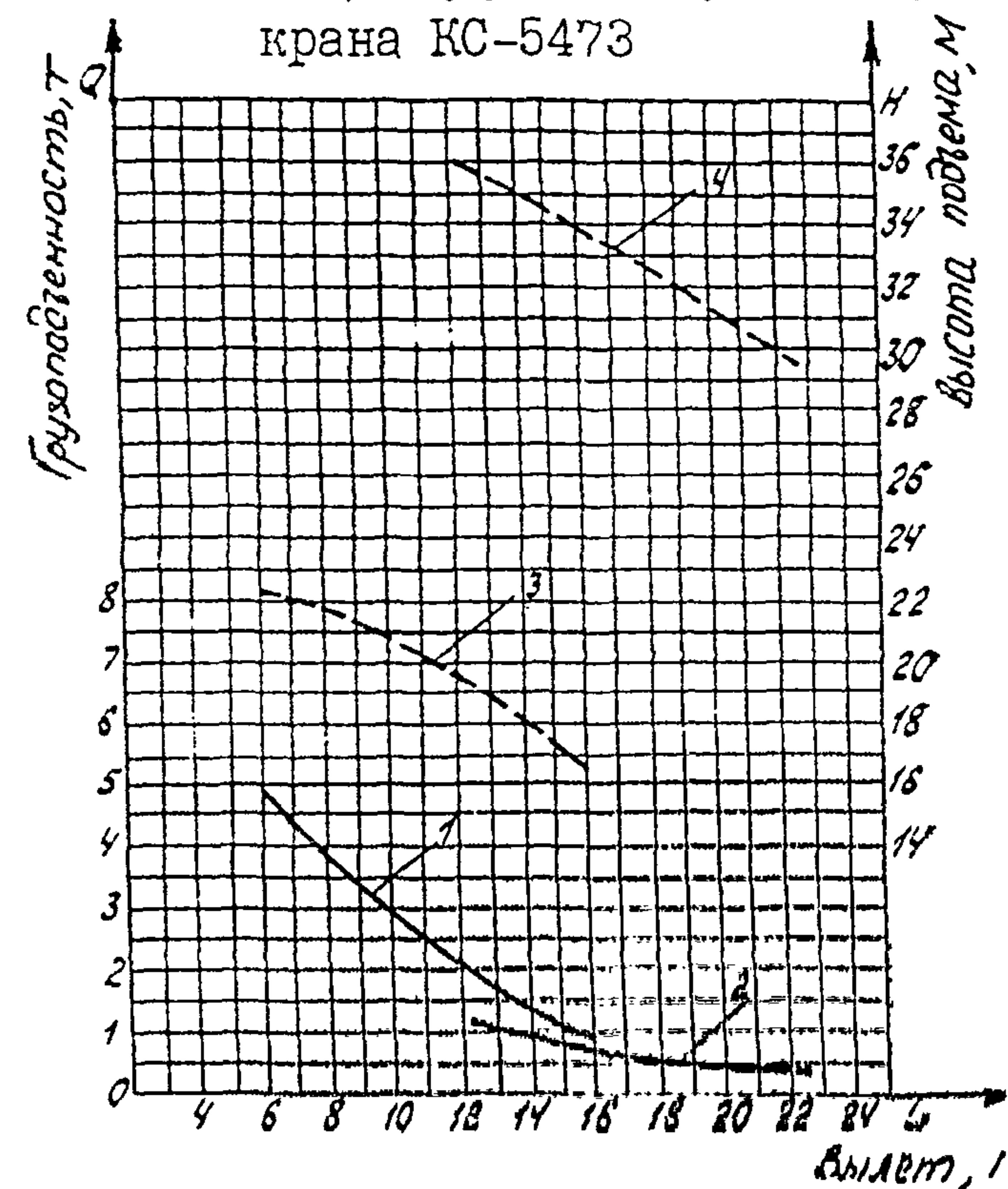
Грузовысотные характеристики (Диаграмма грузоподъемности и высоты подъема для стрелы с удлинителем 8 м ( \alpha = 0^\circ ) и неуправляемым гуськом 1 м ( \alpha = 30^\circ ))
