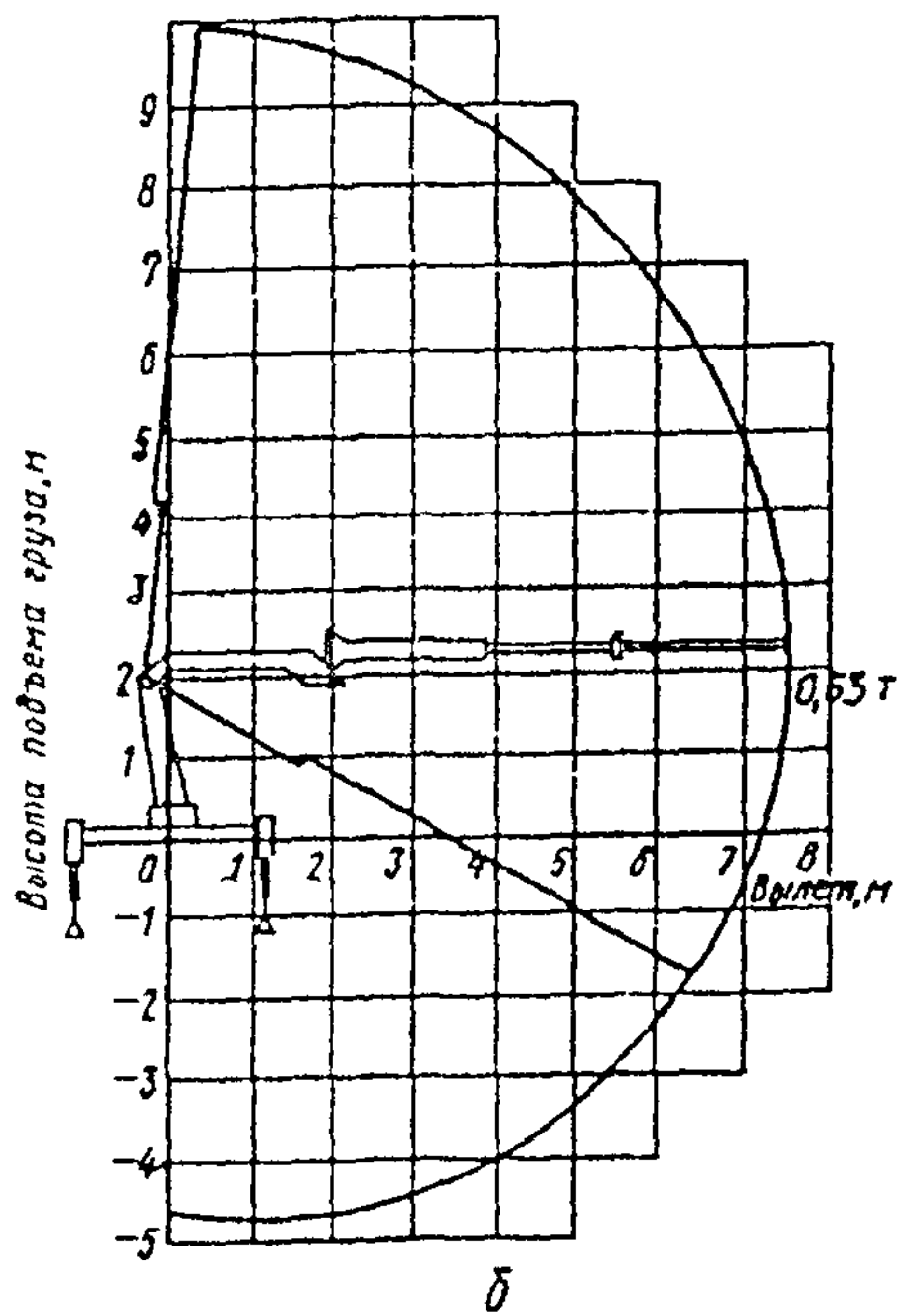
Грузовые характеристики бортового манипулятора МКС-4531: а — для основной стрелы (в скобках приведены данные при работе без выносных опор); б — для стрелы с удлинителем
