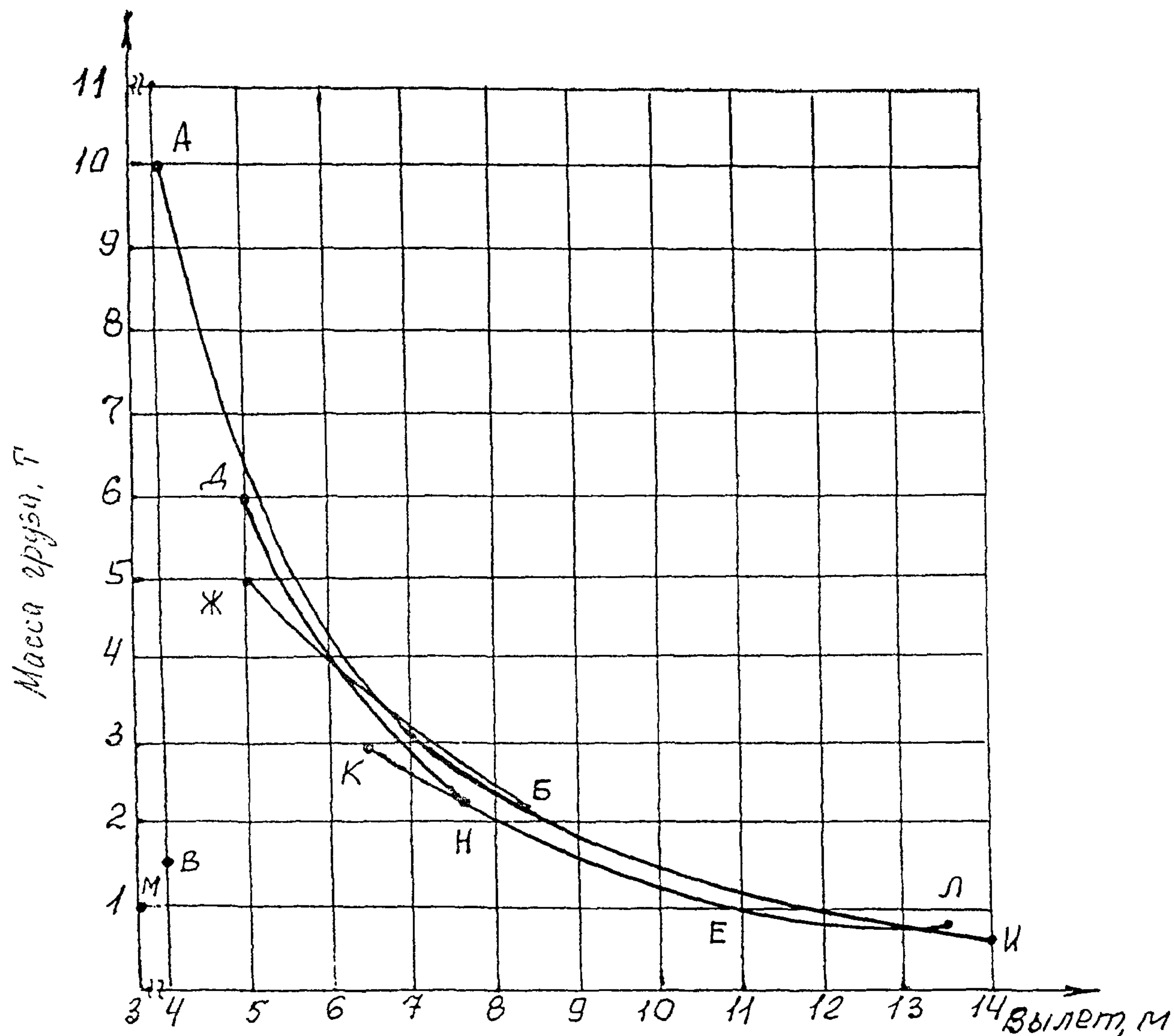
Рис. 5. Диаграмма грузовых характеристик стрелового крана СМК-101А
