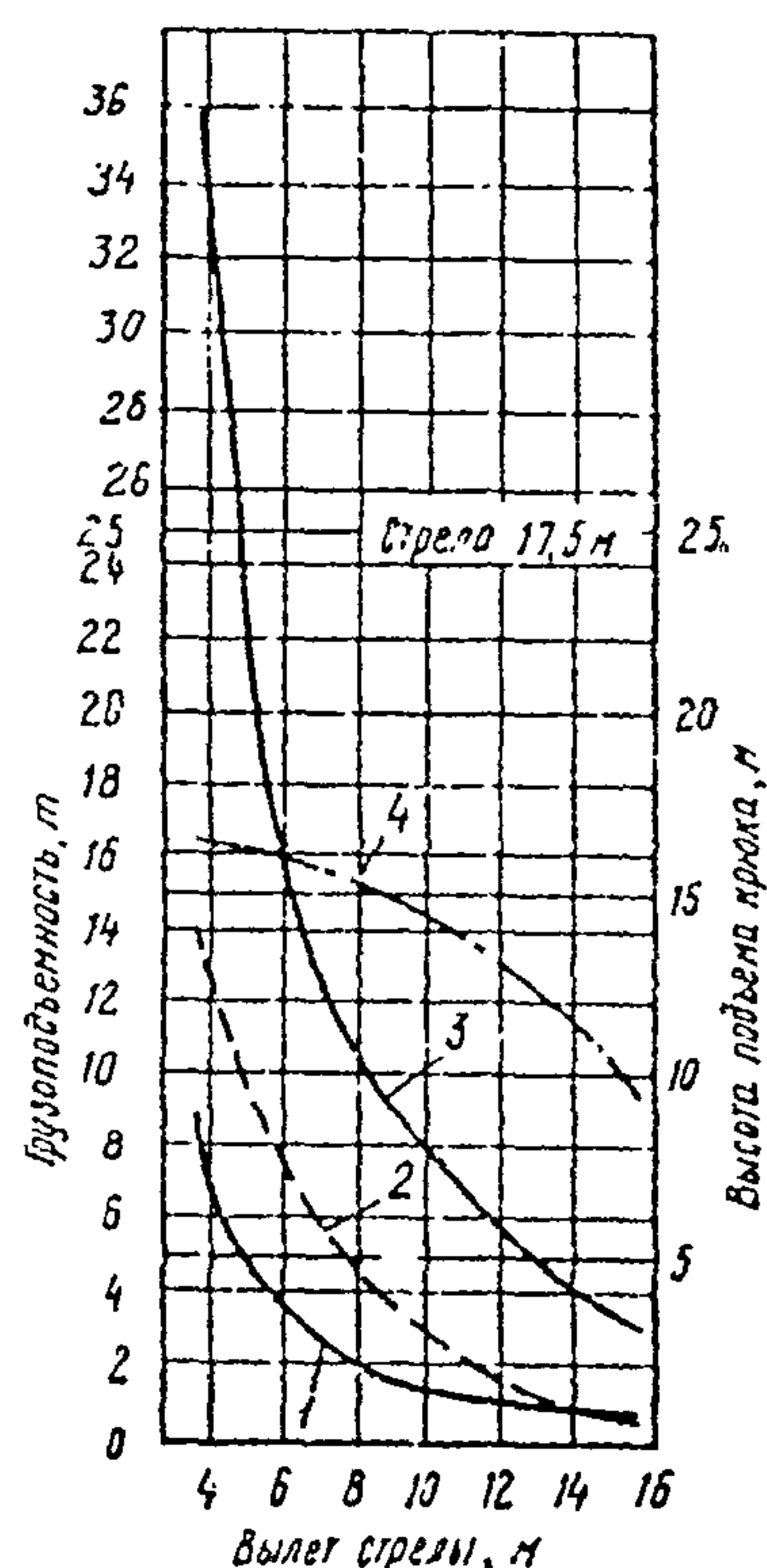
Грузовысотные характеристики крана КС-5363В на минимальных (1, 2, 3) и максимальной стрелах:
