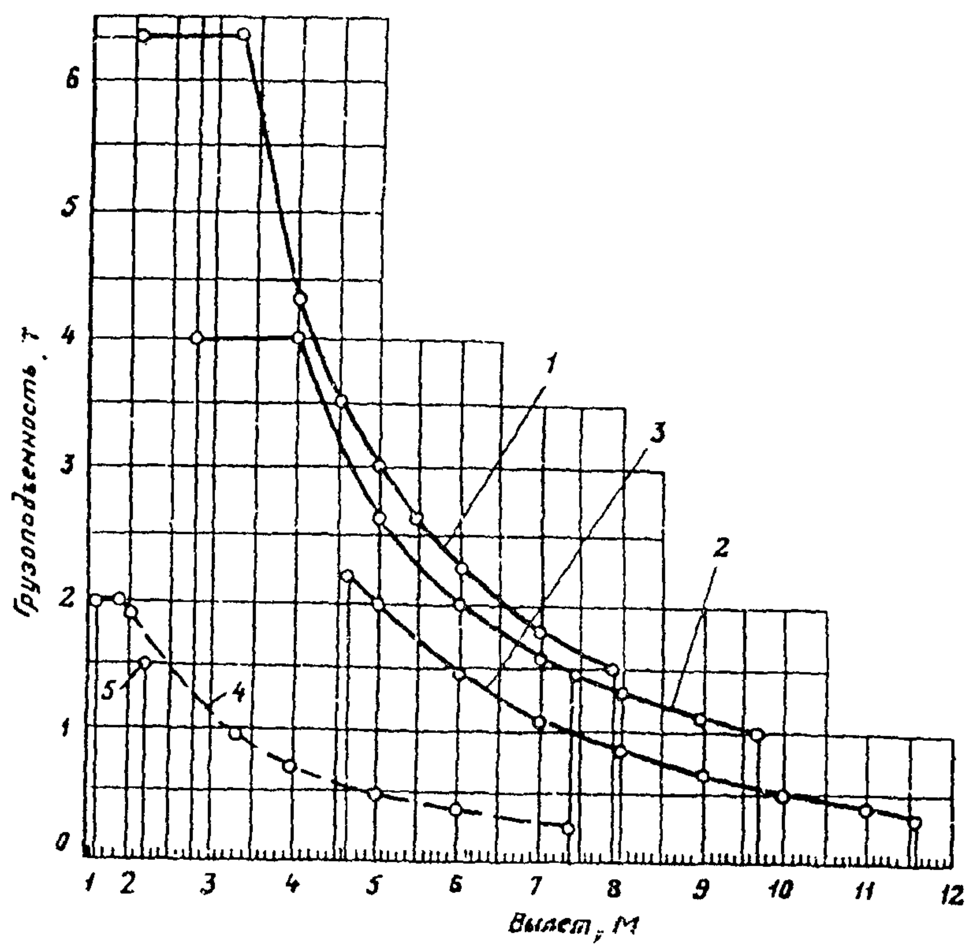
Р-К .. Кривые грузоподъемности крана КС-2571А-1: в точках: 1 — на стреле 9 м; 2 — на стреле 10,8 м; 3 — на стреле 10,8 м с гуськом 2,2 м; без опор на стреле 7,3 м; 4 — в статичном положении; 5 — при передвижении с грузом на крюке
