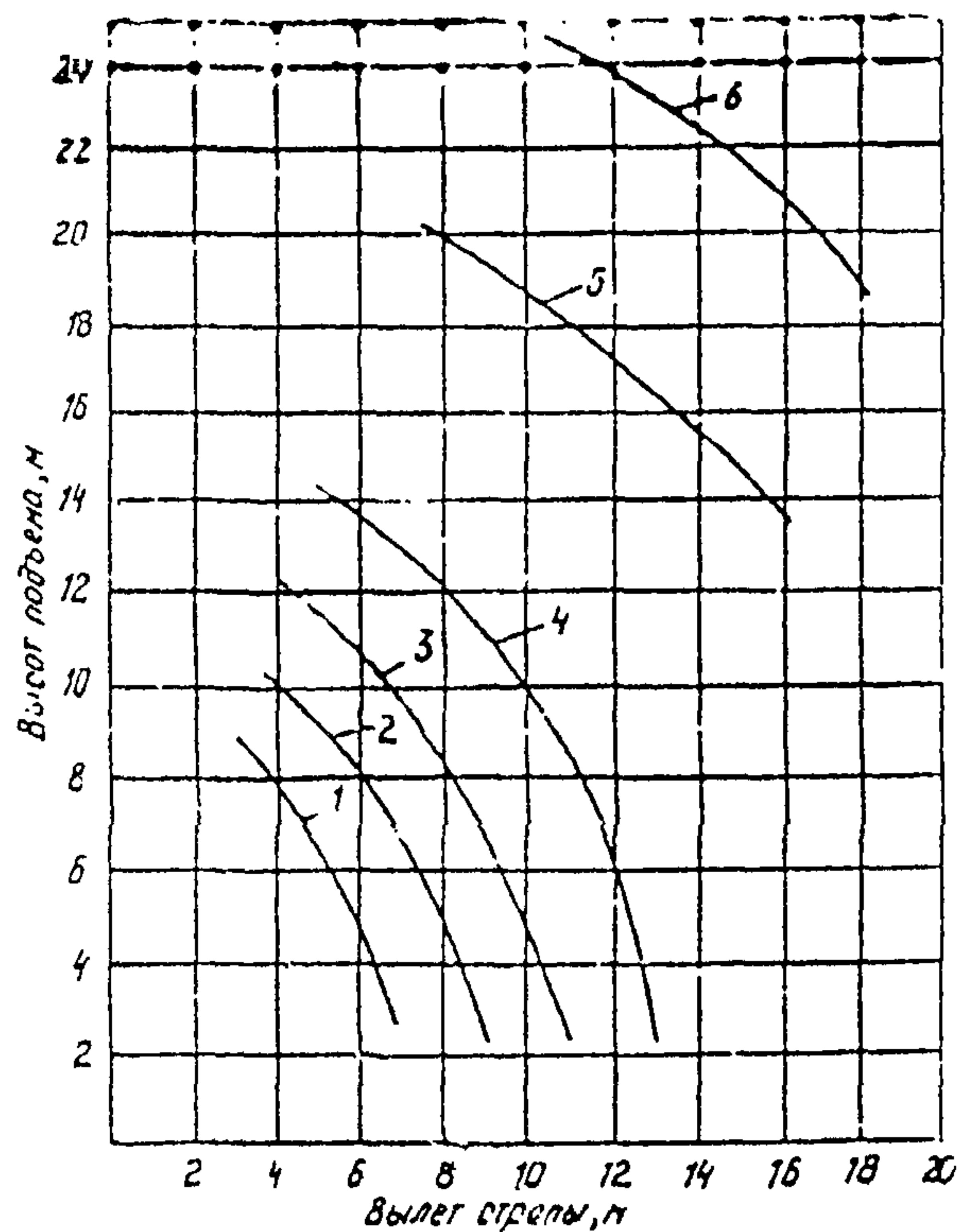
Кривые высоты подъема крюка крана КС-3577 (КС-3577-3-1). 1 — на стреле 8 м; 2 — на стреле 10 м; 3 — на стреле 12 м; 4 — на стреле 14 м; 5 — на стреле 14 м с гуськом 7 м; 6 — на стреле 14 м с гуськом 7 м и вставкой 4,5 м
