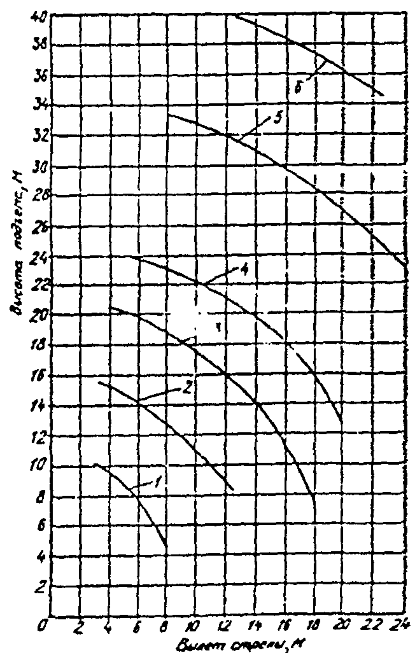
Кривые высоты подъема крюка крана КС-5473Б на выносных опорах (основной подъем):
