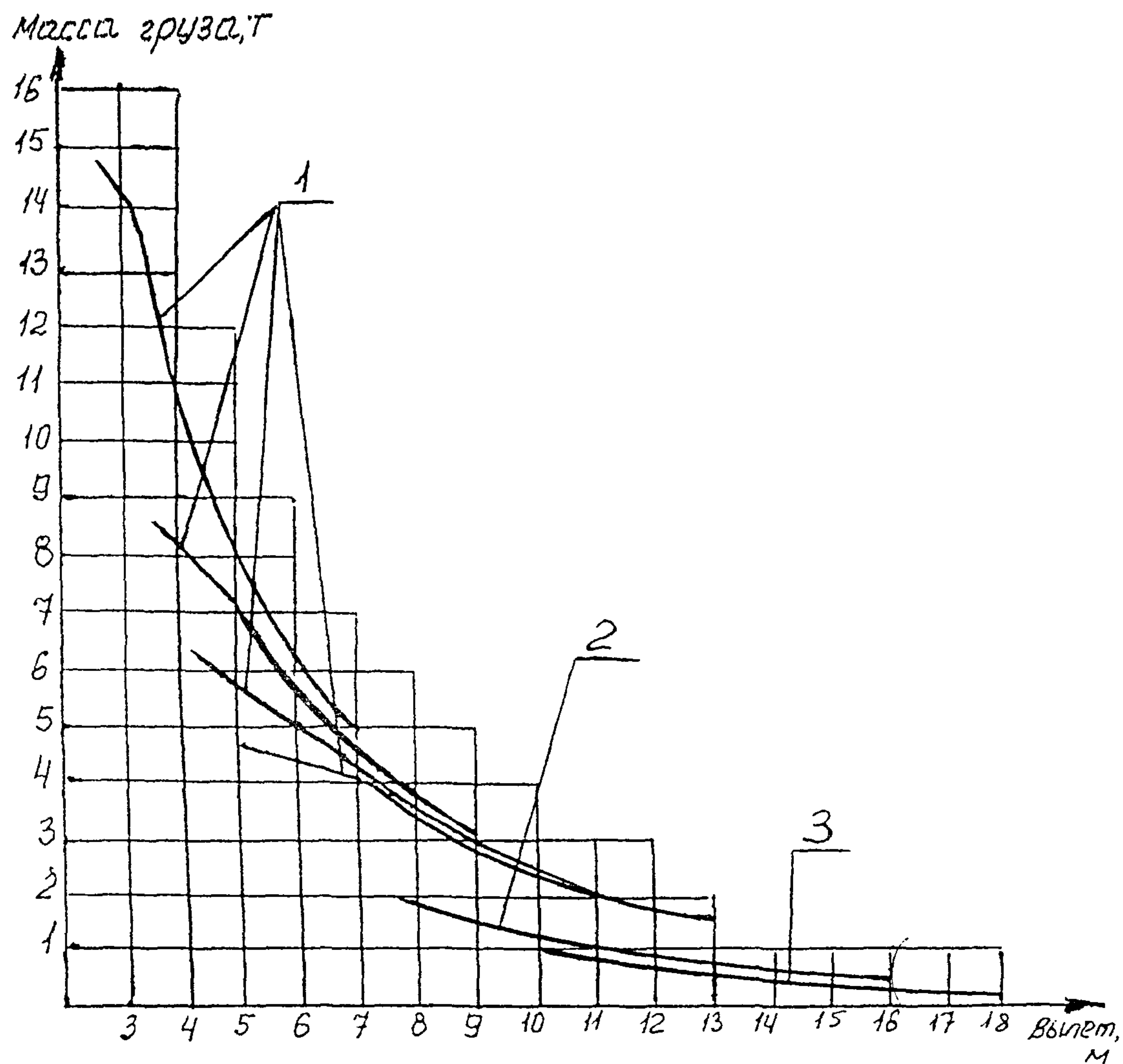
Рис.7. Диаграмма грузовых характеристик крана КС-3577-4
