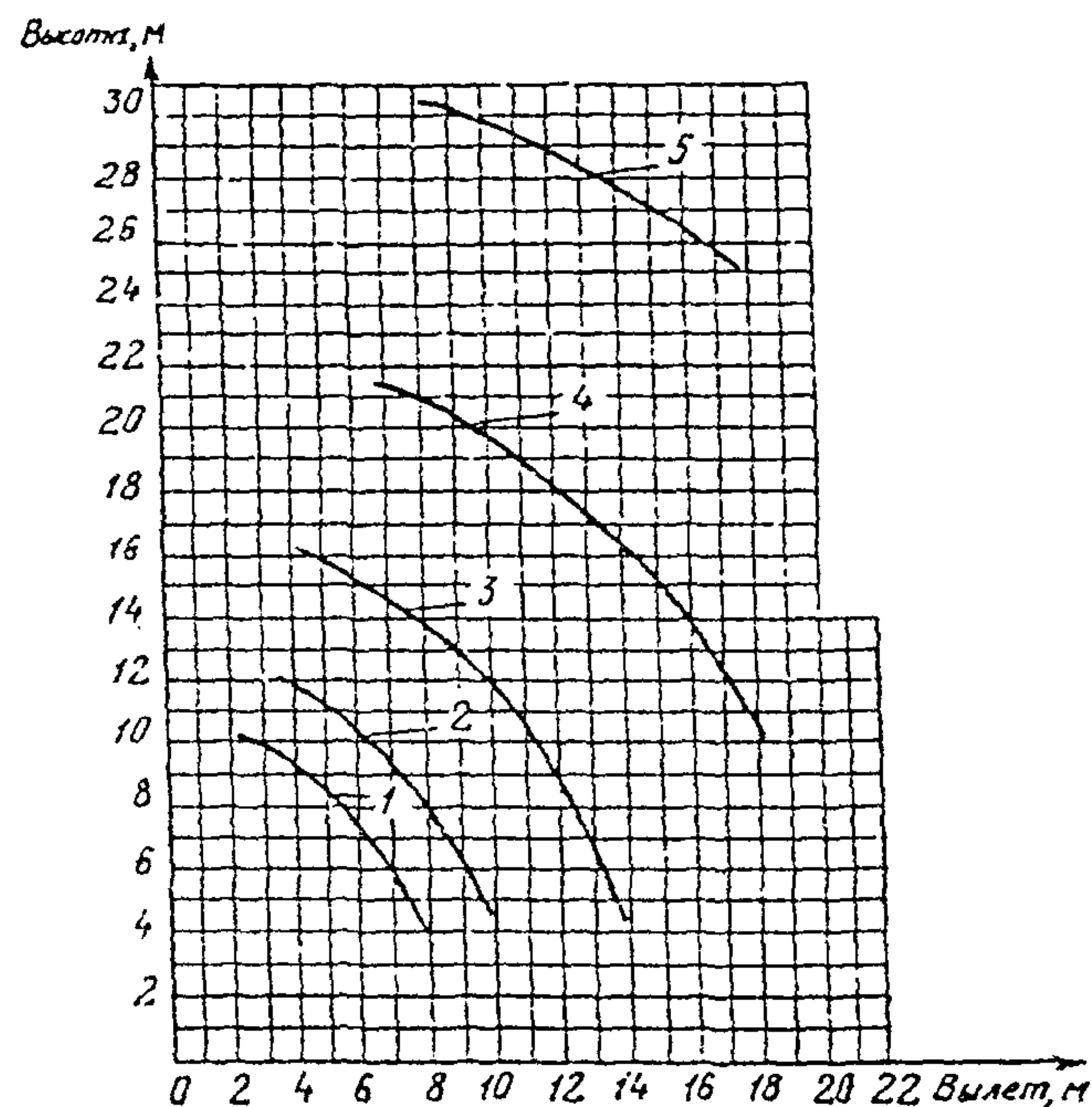
Кривые высоты подъема крюка крана КС-4572А:
