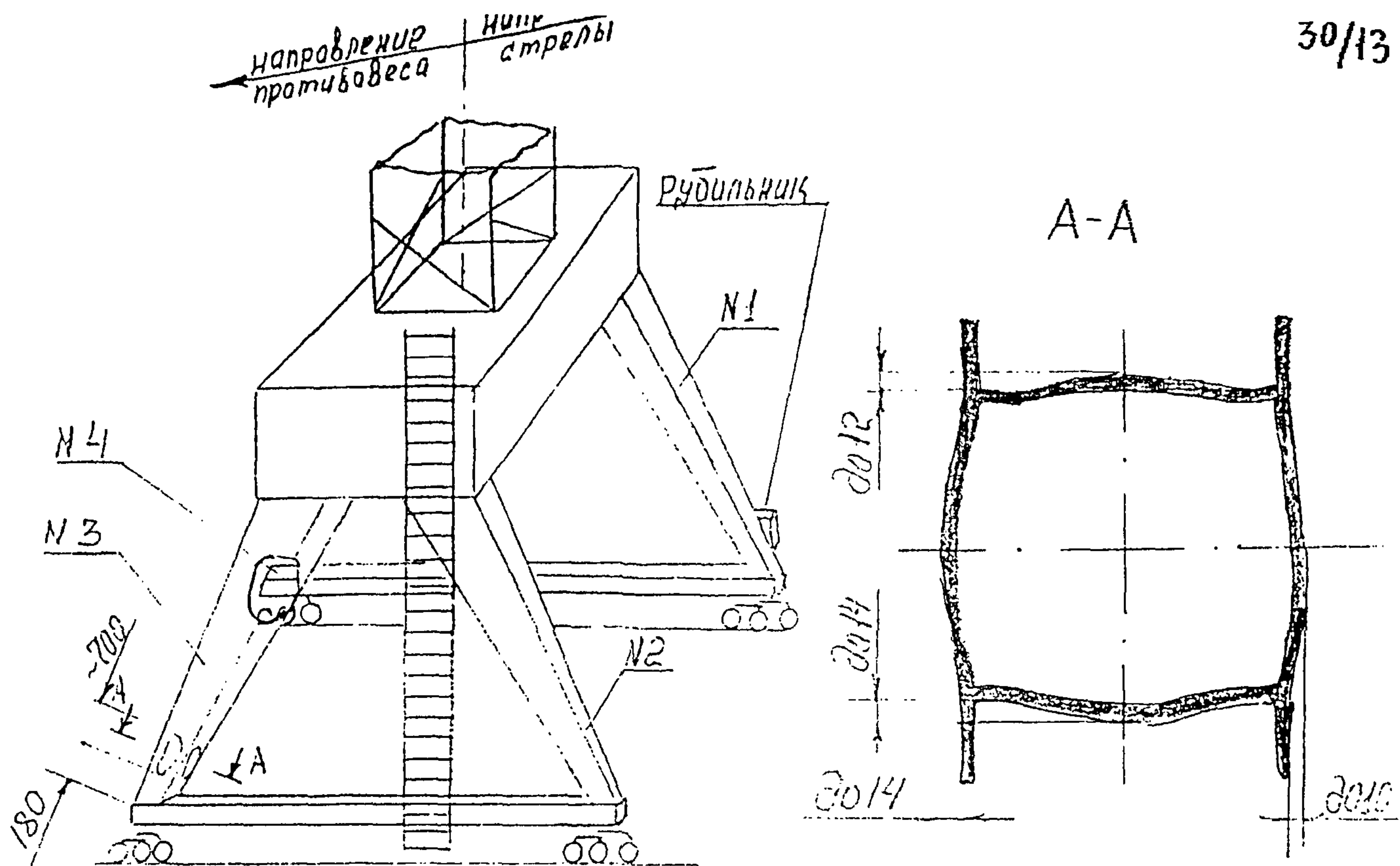
Рис. 1. Схема расположения дефектной стойки портала.
