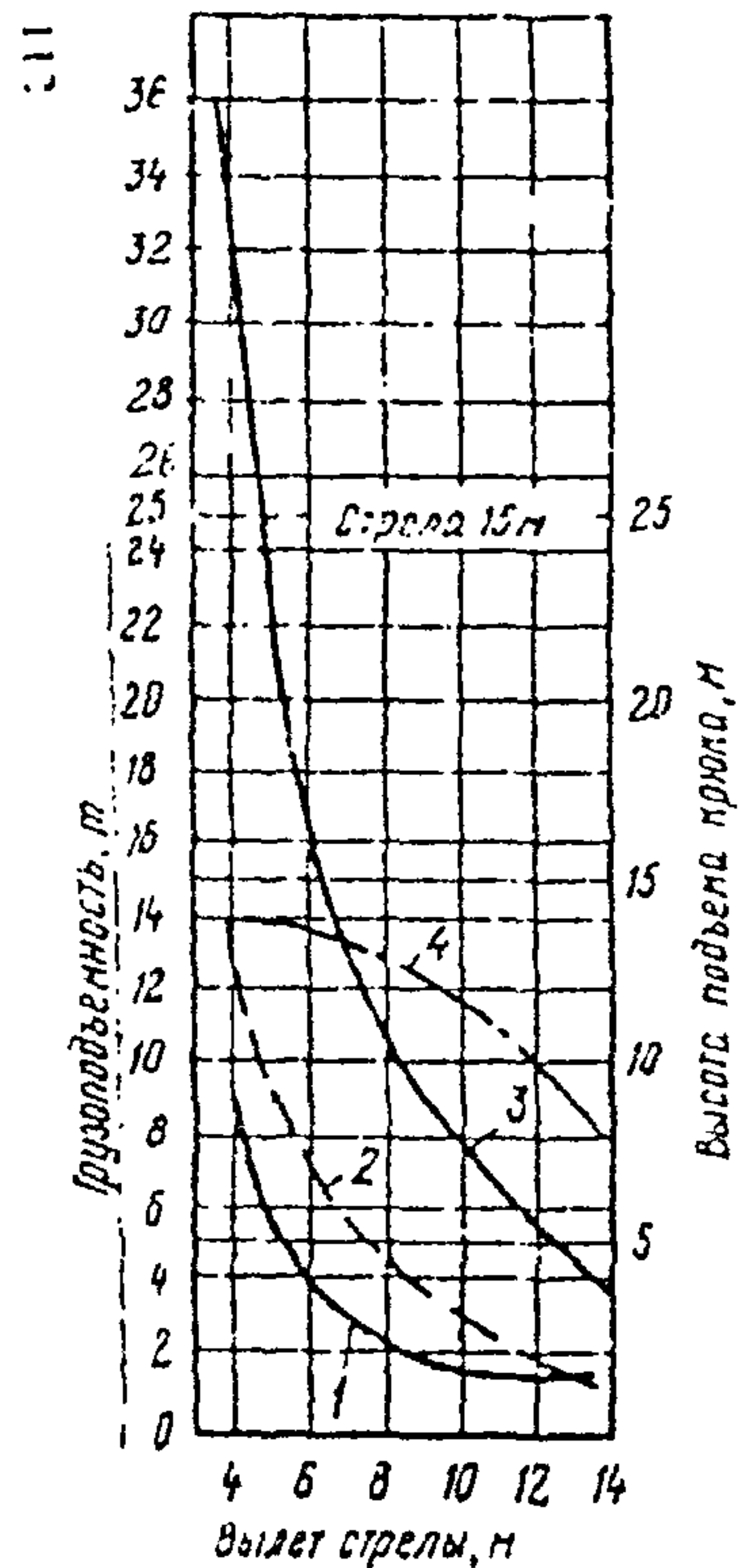
Грузовысотные характеристики крана КС-5363В на минимальных (1, 2, 3) и максимальной стрелах:
