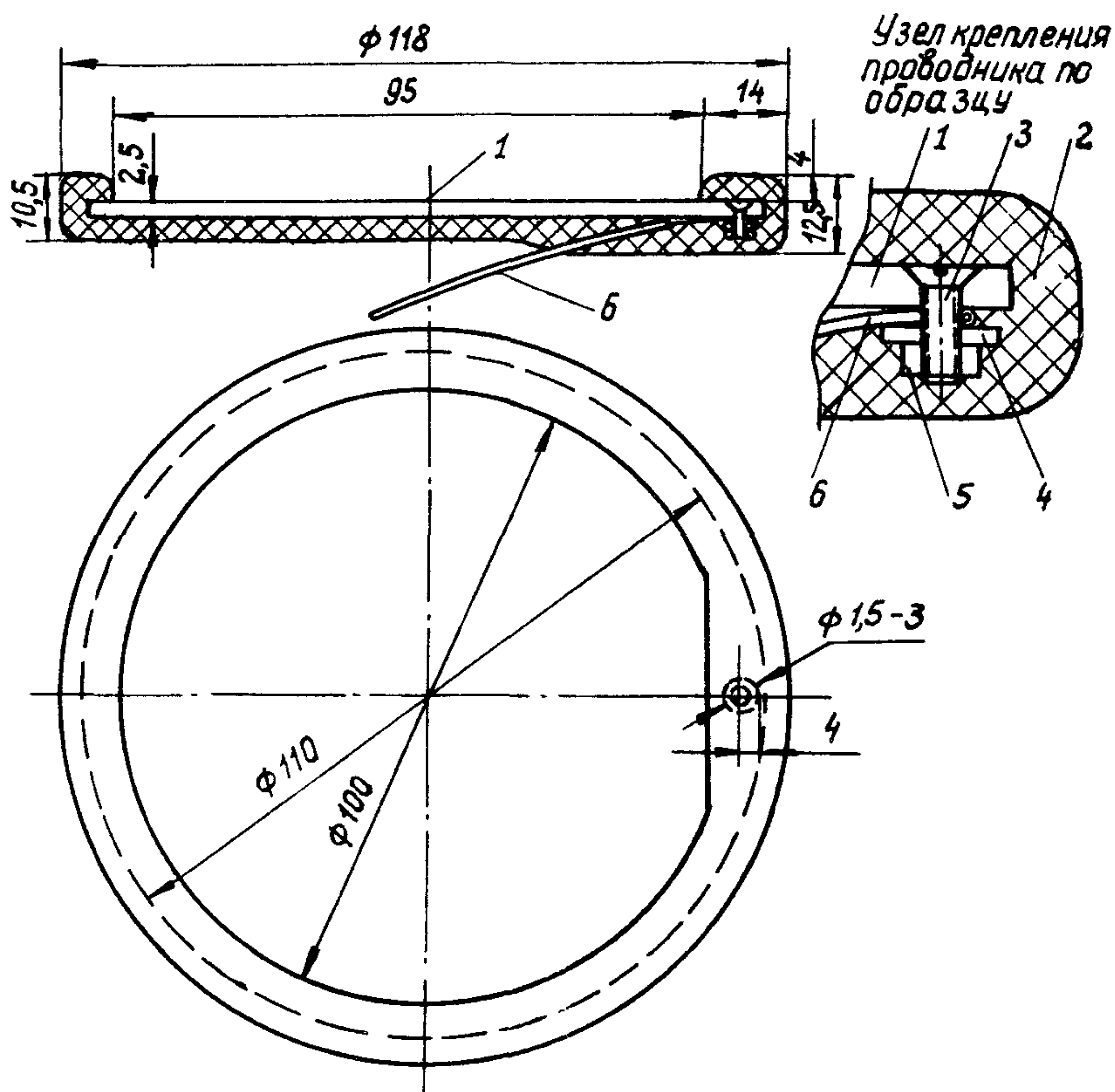
Рис.1. Модель образца, имитирующая дефект диаметром 100 мм: 1 - образец; 2 - битумная изоляция; 3 - болт ( \ell \approx 7-10 мм, диаметр 1,5-3 мм); 4 - шайба (диаметр 1,5-3 мм); 5 - гайка (диаметр 1,5-3 мм); 6 - проводник
