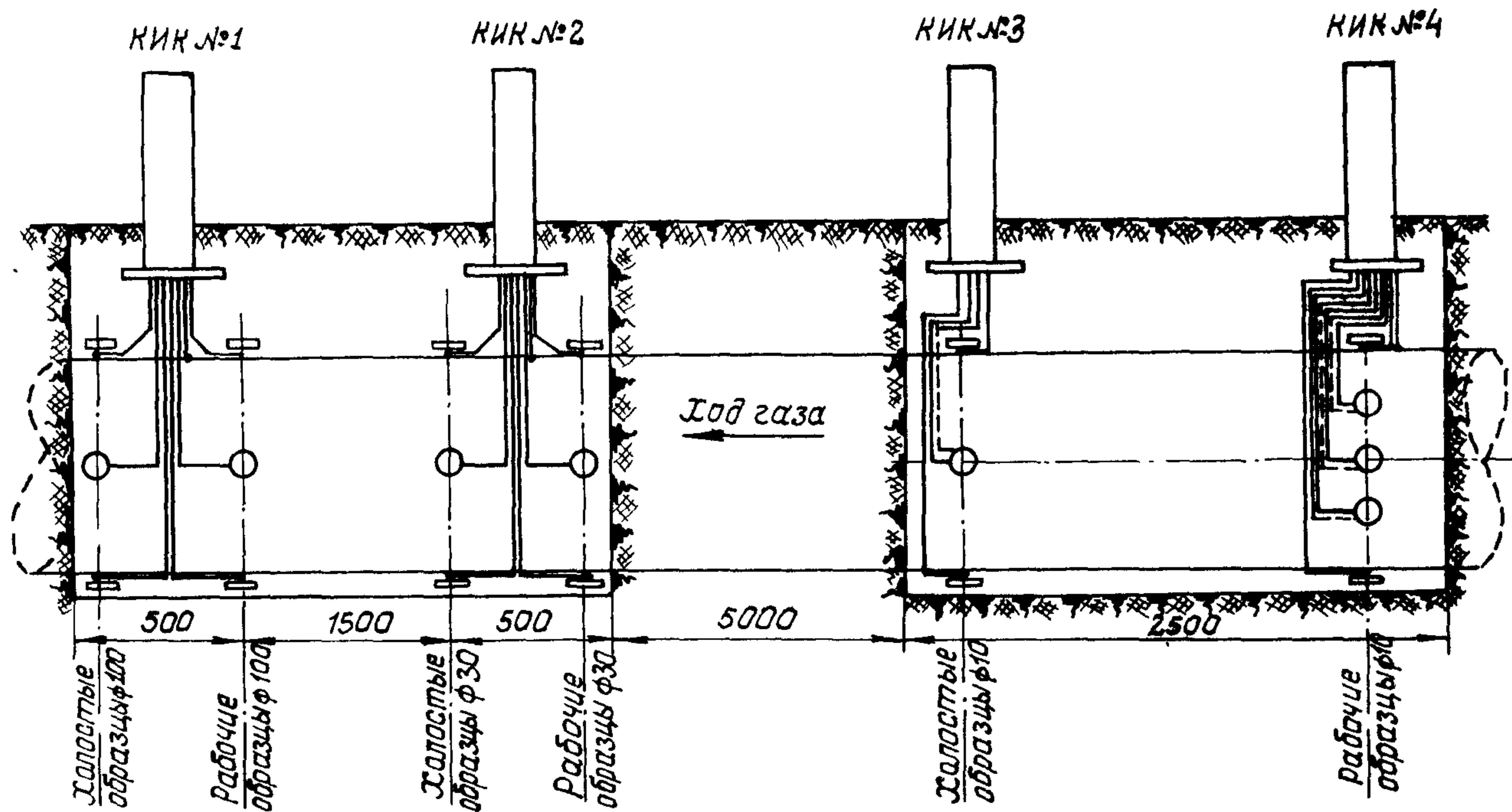
Рис.4. Схема установки для определения эффективности электрохимической защиты трубопровода
