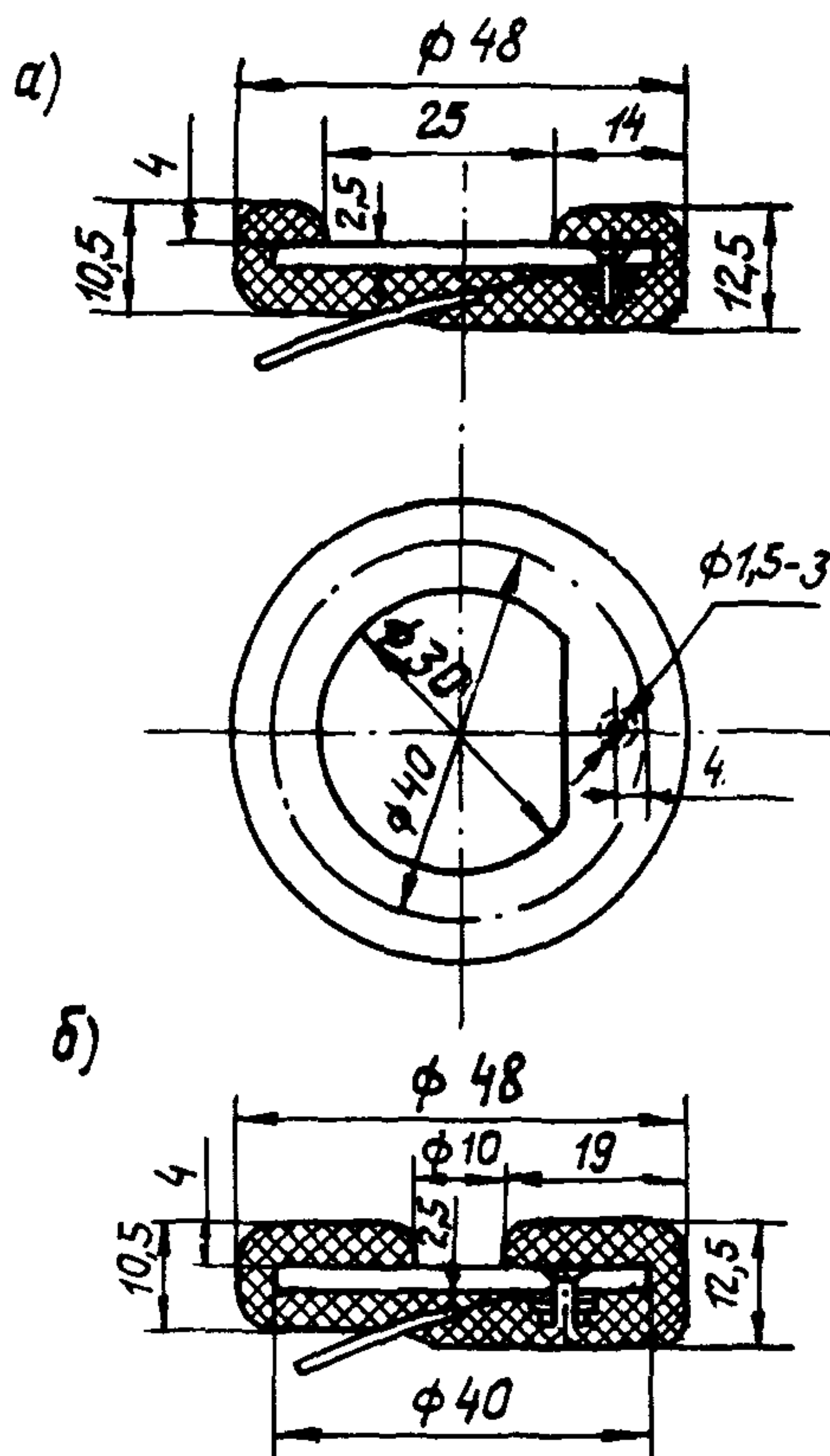
Рис.2. Модели образцов, имитирующие дефекты диаметром:
