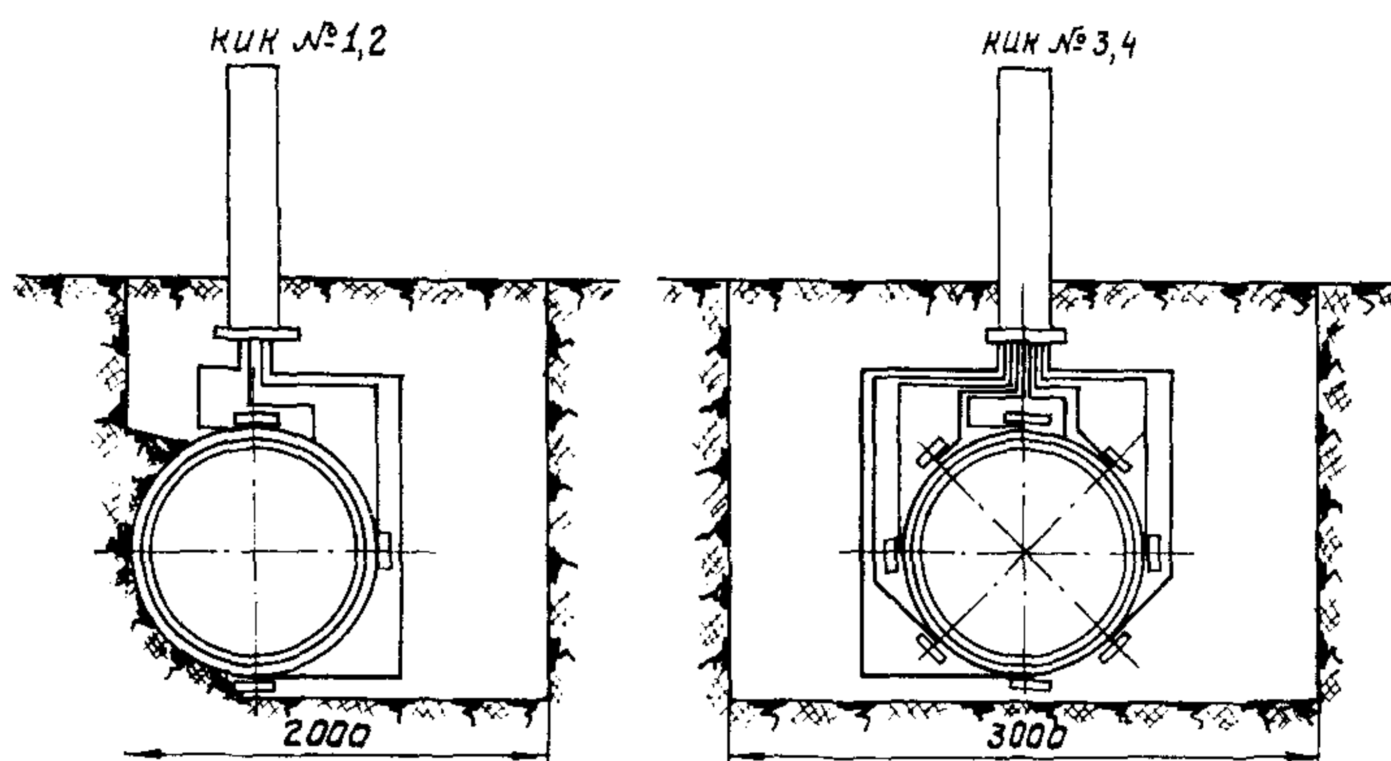
Рис.5. Схема укладки образцов в грунт
