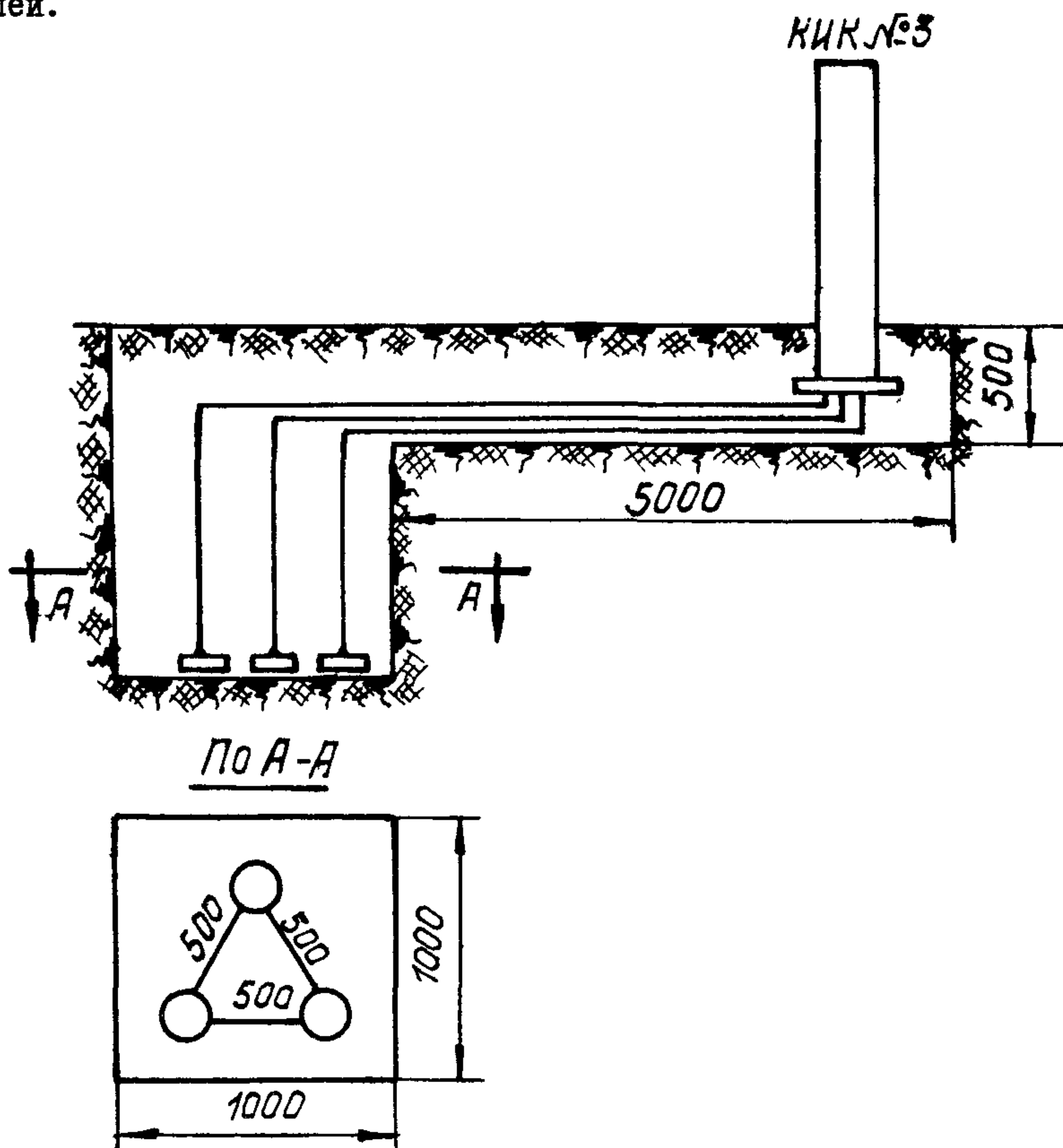
Рис.6. Схема отдельного шурфа для холостых образцов
