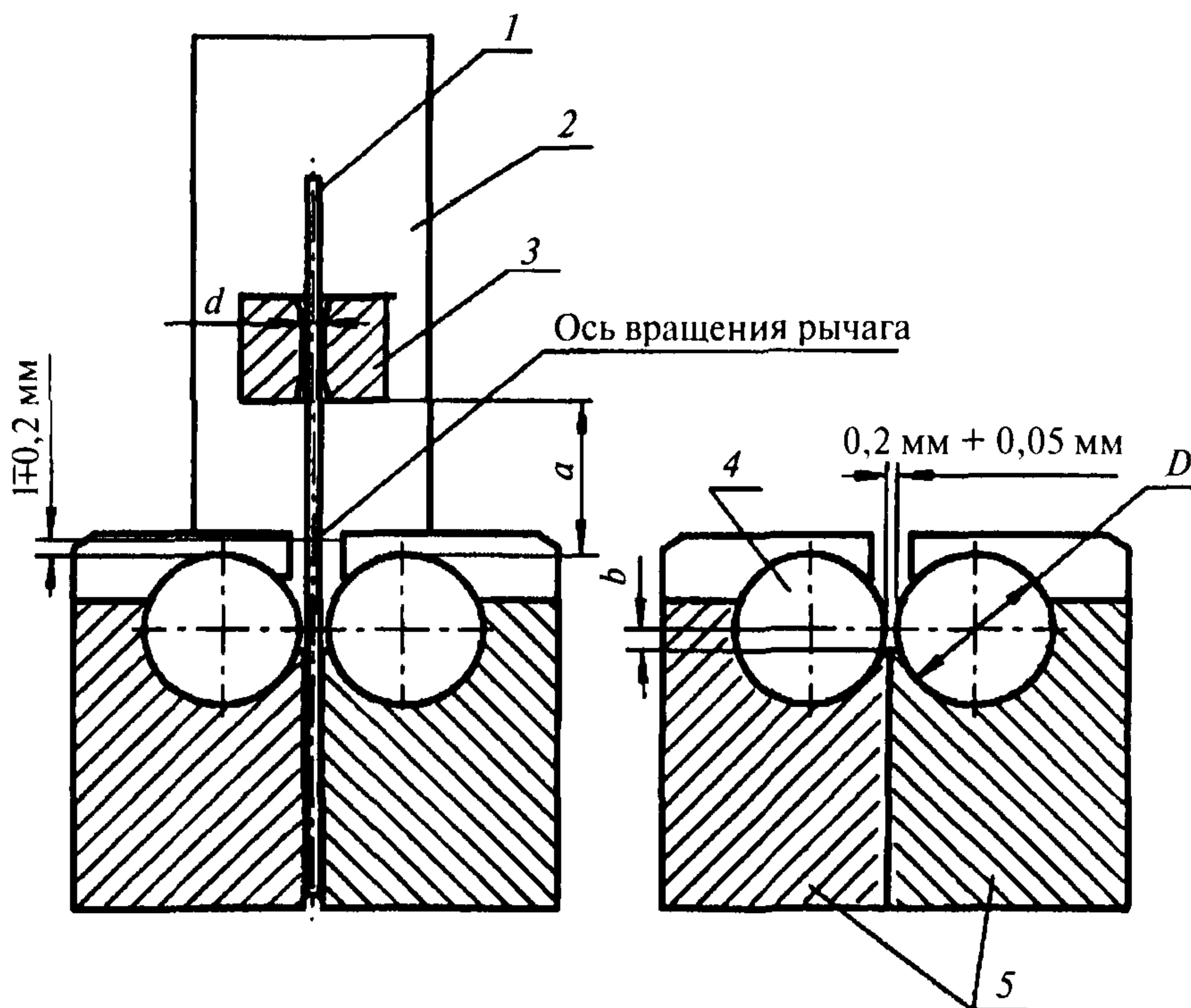
Рис. 1. Прибор для испытания проволоки на перегиб: 1 — испытуемый образец; 2 — изгибающий рычаг; 3 — поводок; 4 — цилиндрические валики; 5 — зажимные губки; a — расстояние от нижней поверхности поводка до верхней образующей валиков; b — расстояние от поверхности губок до линии, соединяющей центры валиков; D — диаметр валиков; d — диаметр поводка
