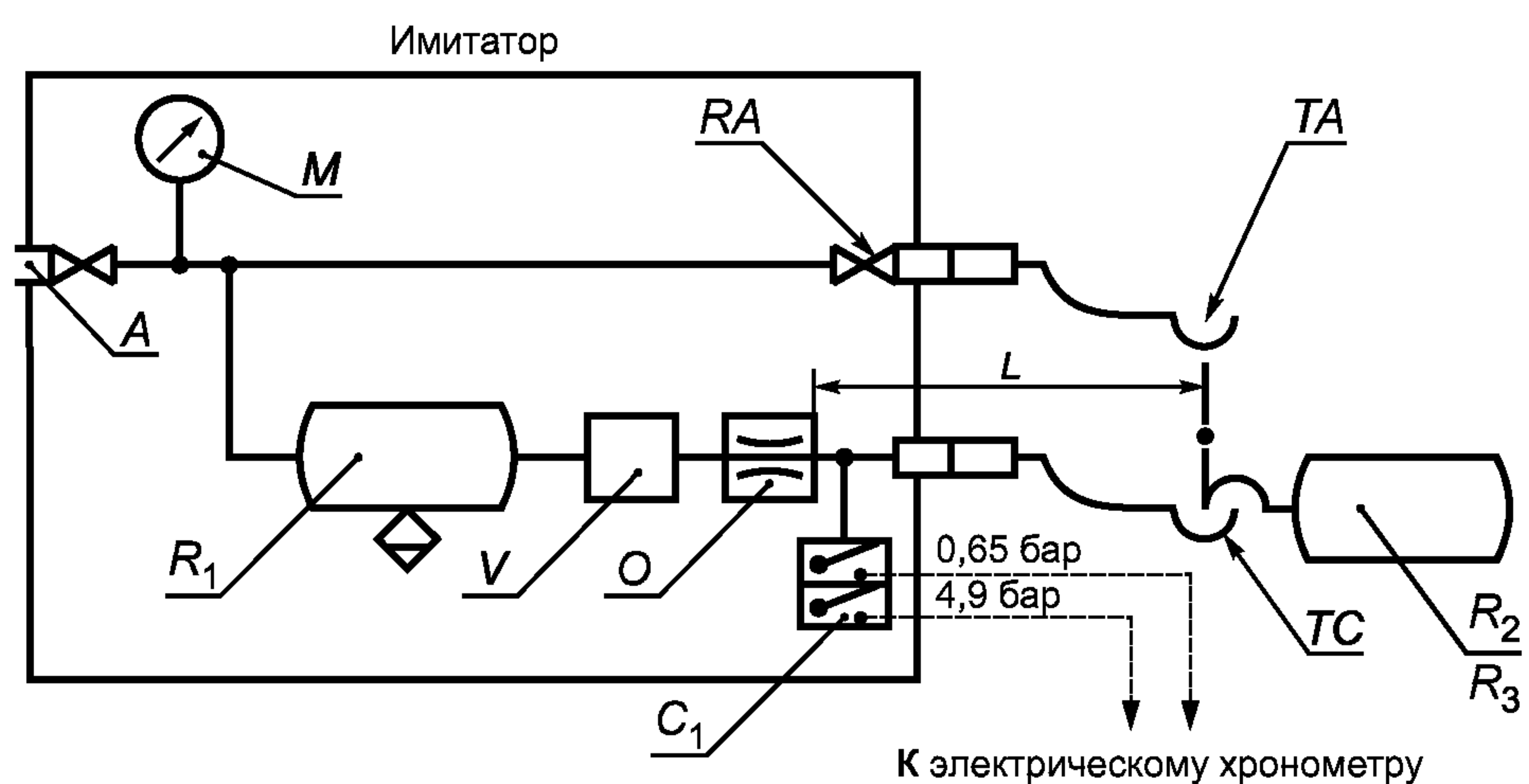
Рисунок Д.1 — Схема настройки имитатора
