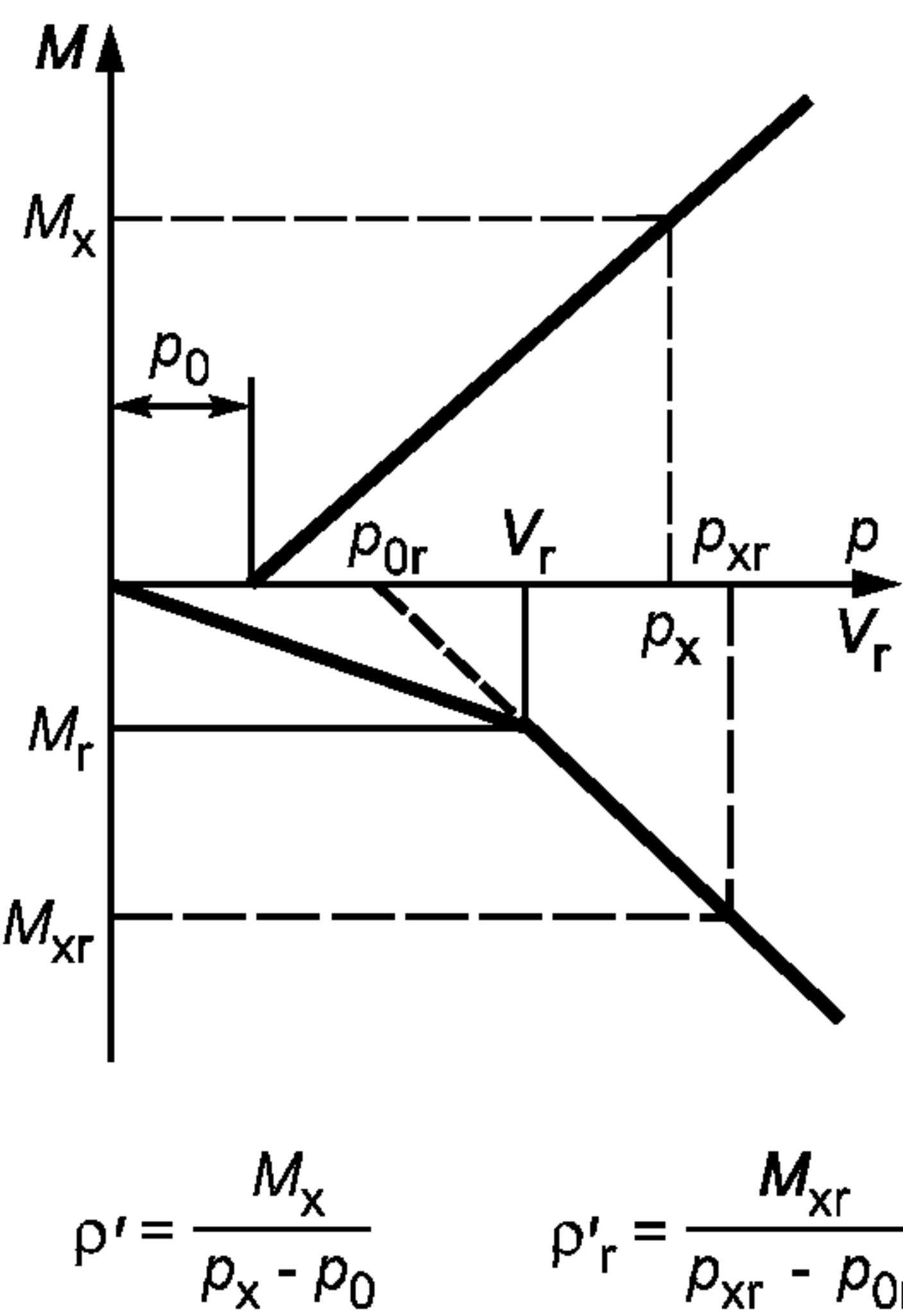
Рисунок М.7 — Характеристики инерционных тормозов с гидравлическим приводом
