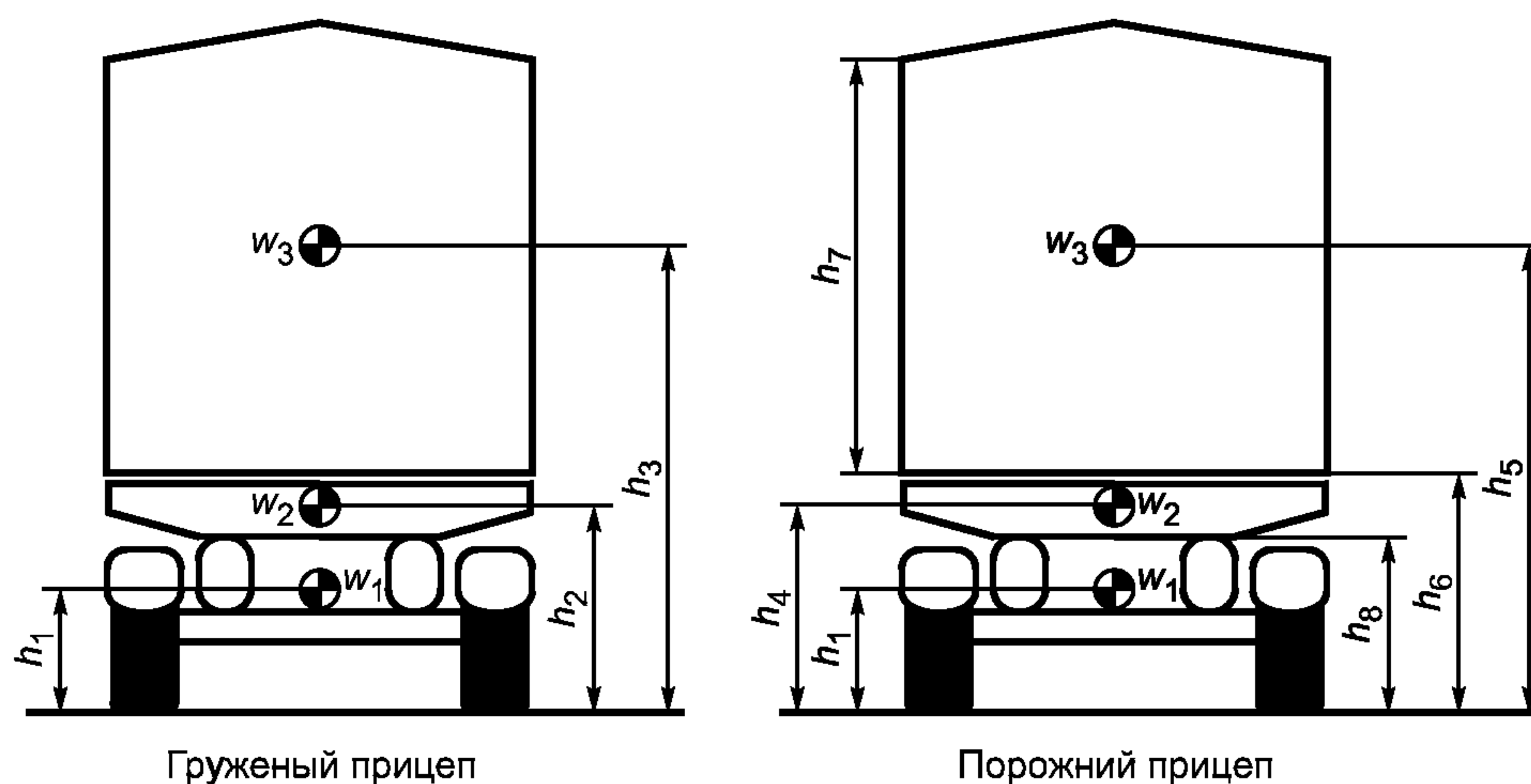
Рисунок X.1 — Расположение центров масс отдельных элементов прицепа
