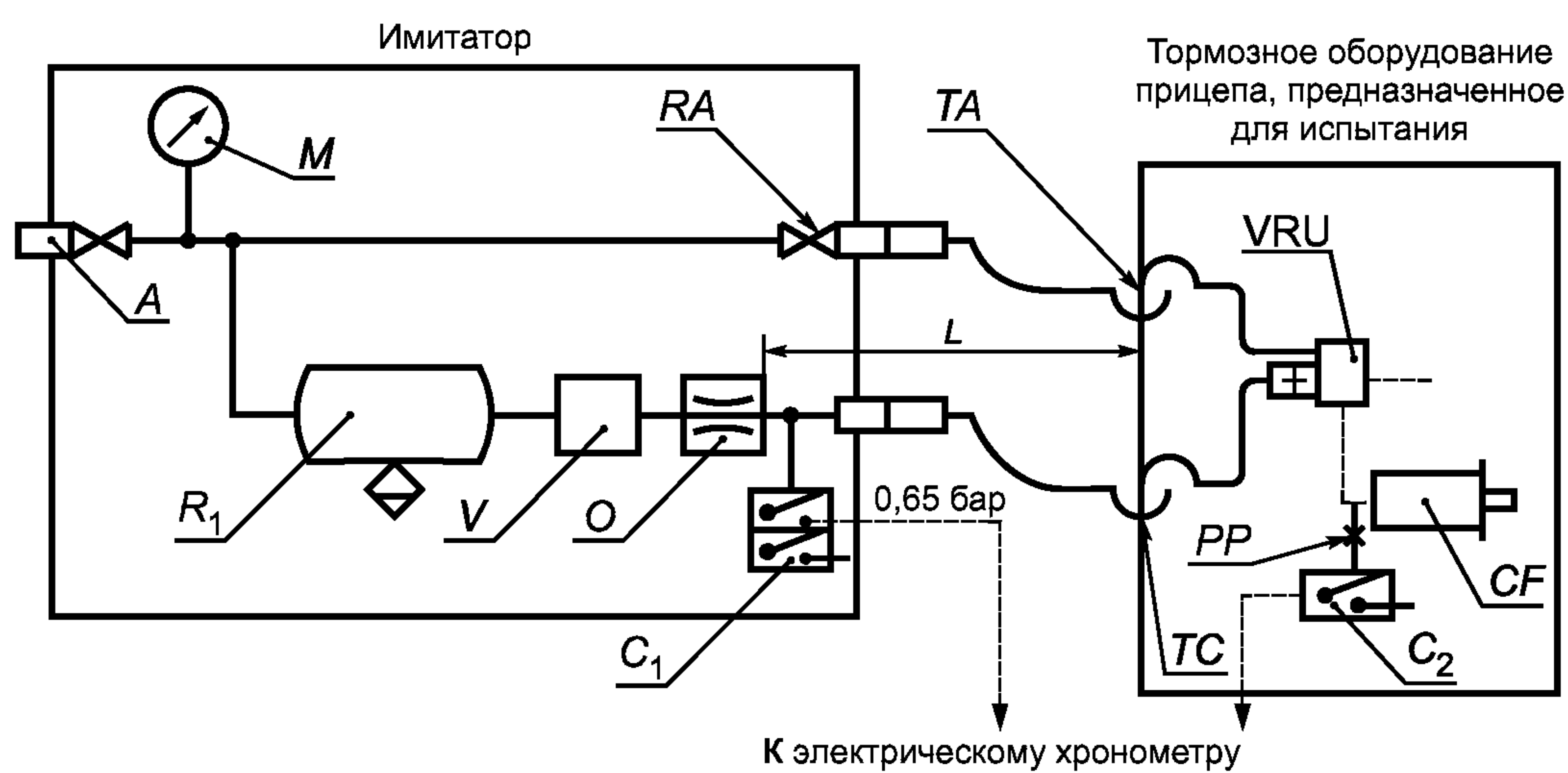
Рисунок Д.2 — Схема испытания прицепа
