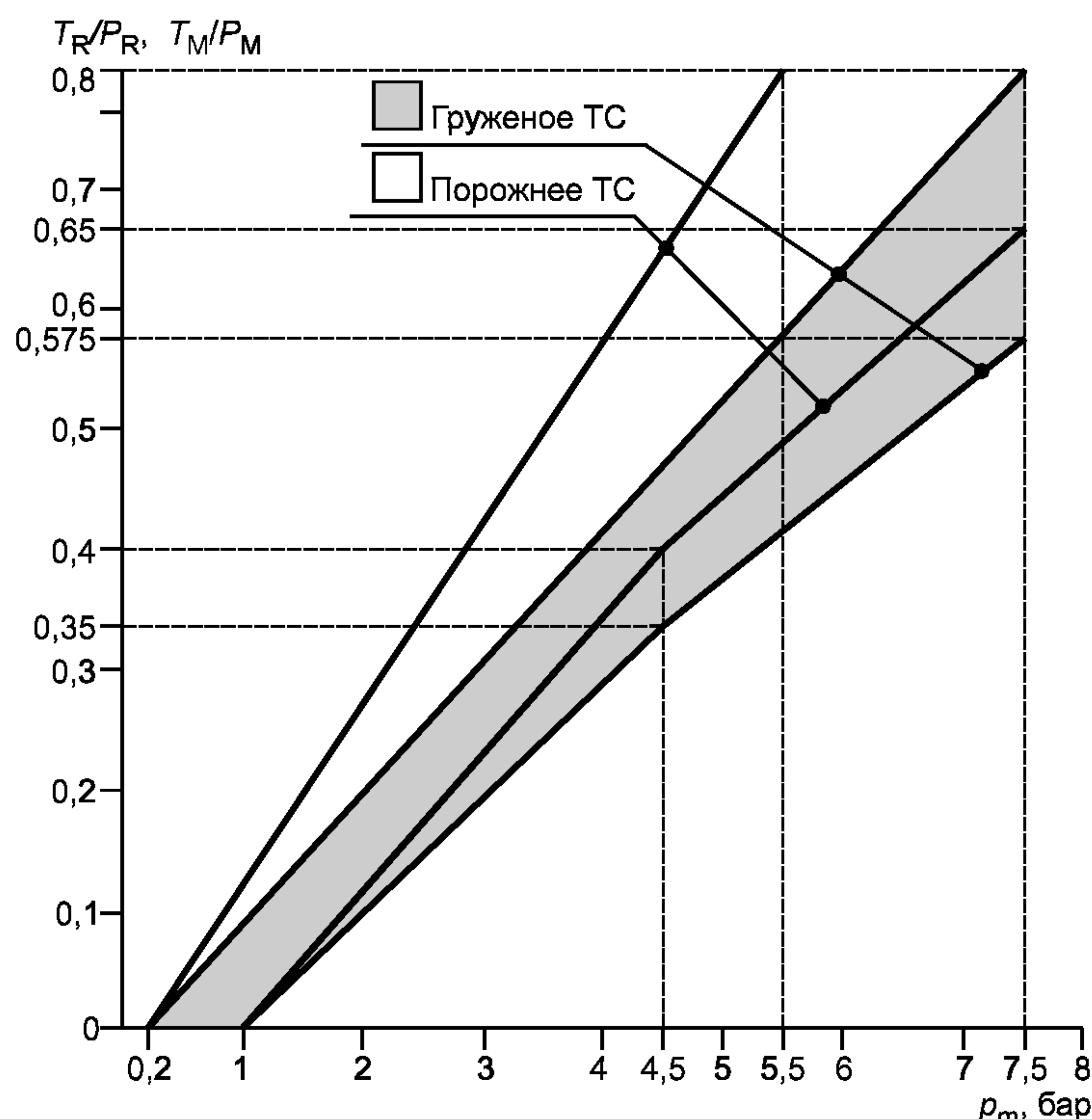
Рисунок К.4 — Области совместимости значений удельных тормозных сил и давления в соединительной головке управляющей магистрали для буксирующих транспортных средств и прицепов, за исключением тягачей для полуприцепов (седельных тягачей) и полуприцепов
