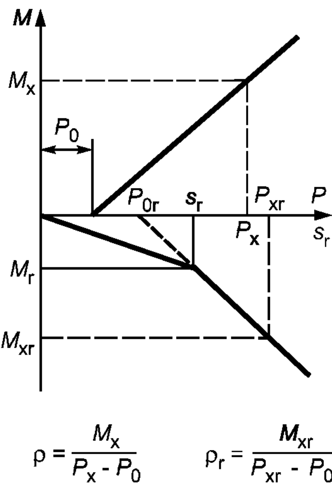
Рисунок М.6 — Характеристики инерционных тормозов с механическим приводом (см. раздел М.2)
