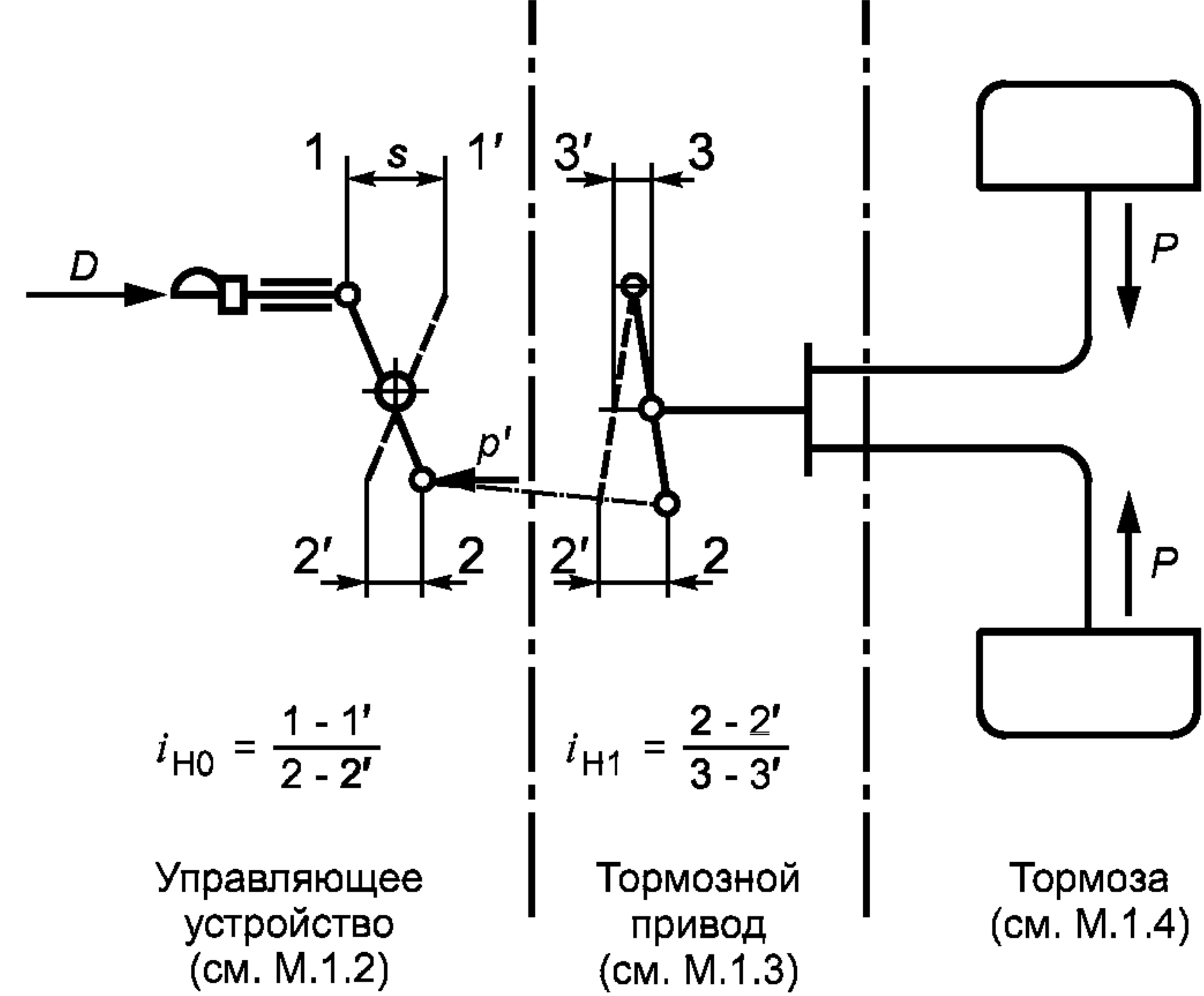
Рисунок М.5 — Схема инерционной тормозной системы с механическим приводом (см. М.2.3)
