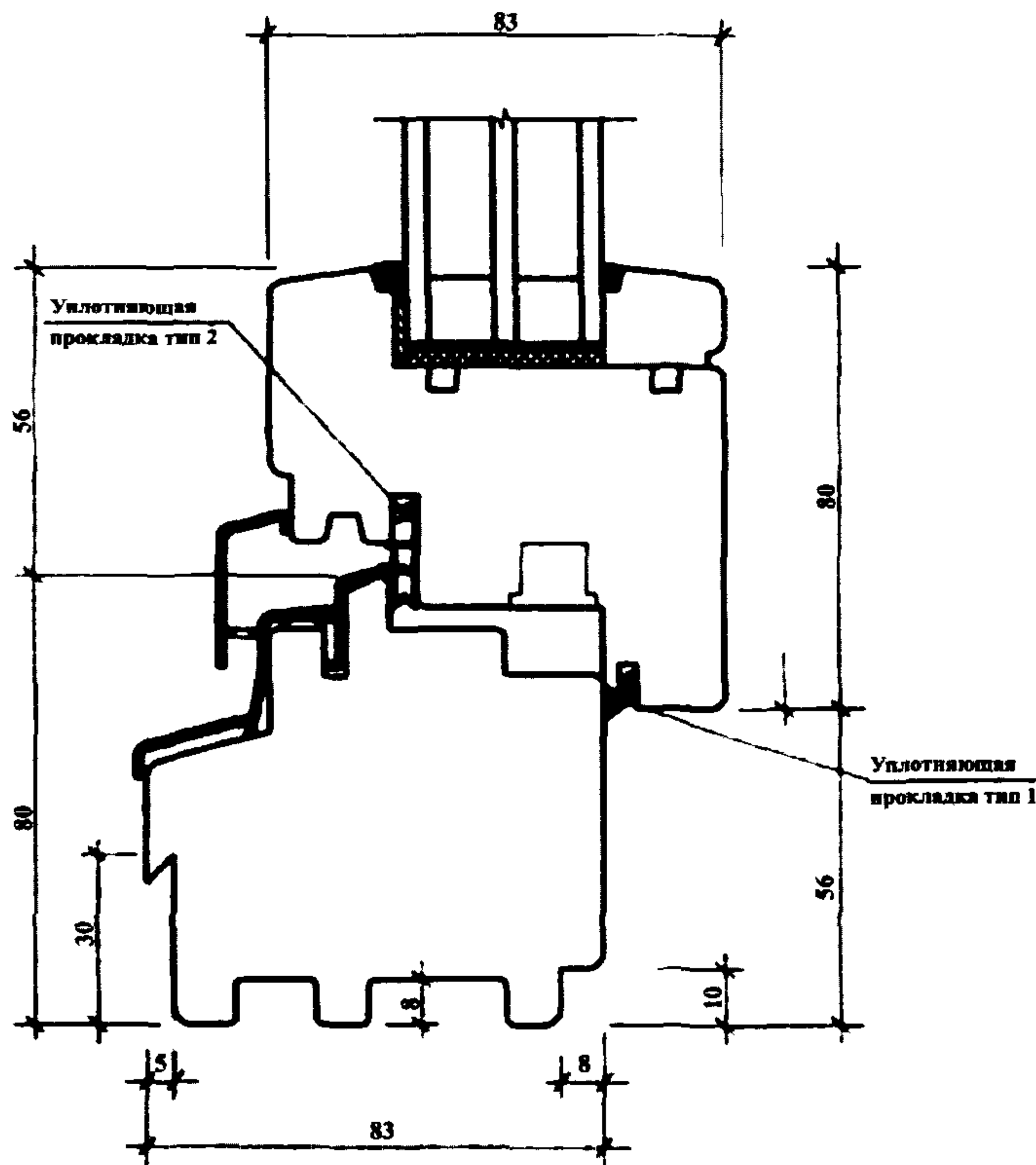
в) сечение 2-2
