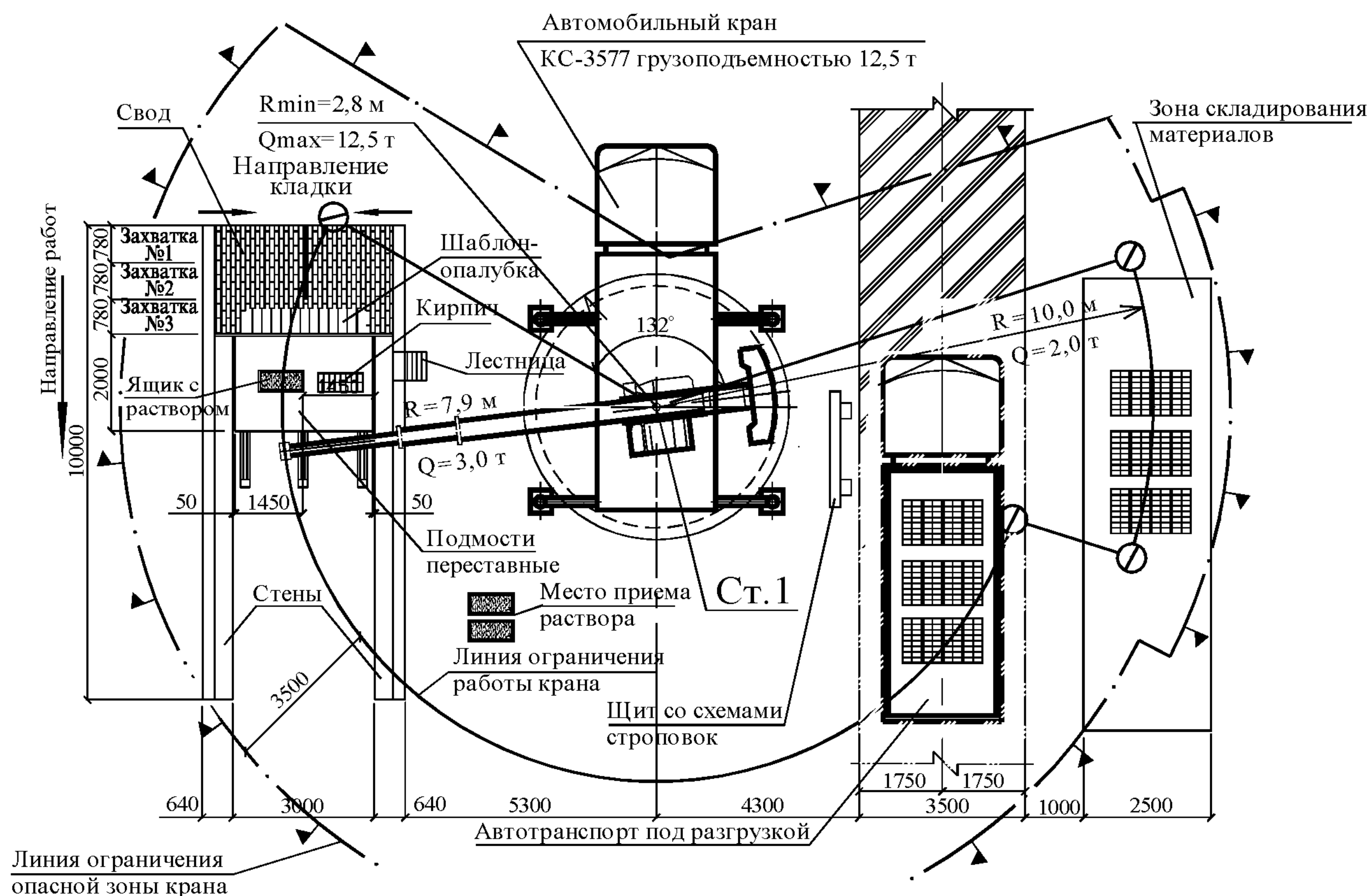
Рисунок 4 – Схема организации работ
