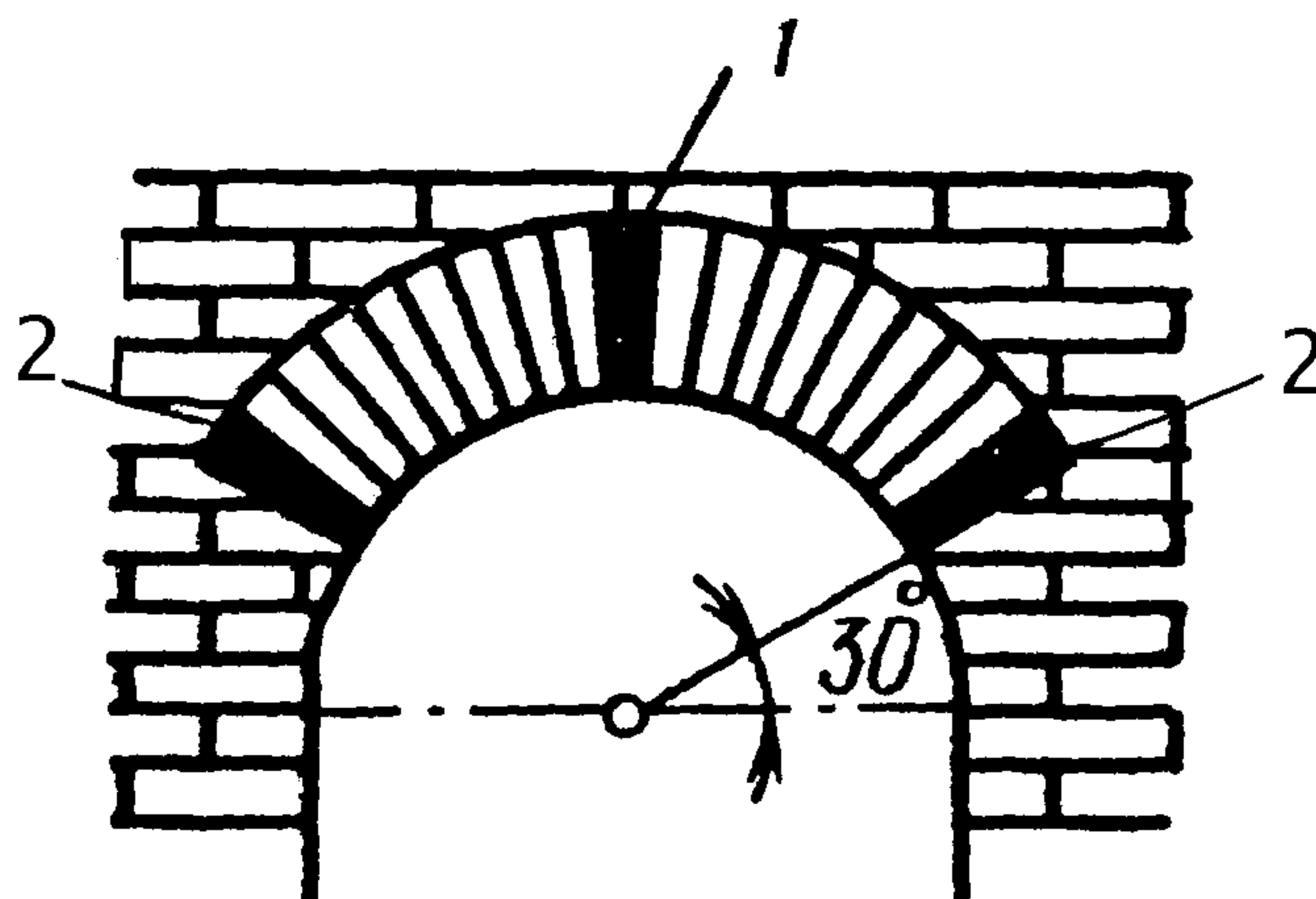
1 – замок; 2 – пята
