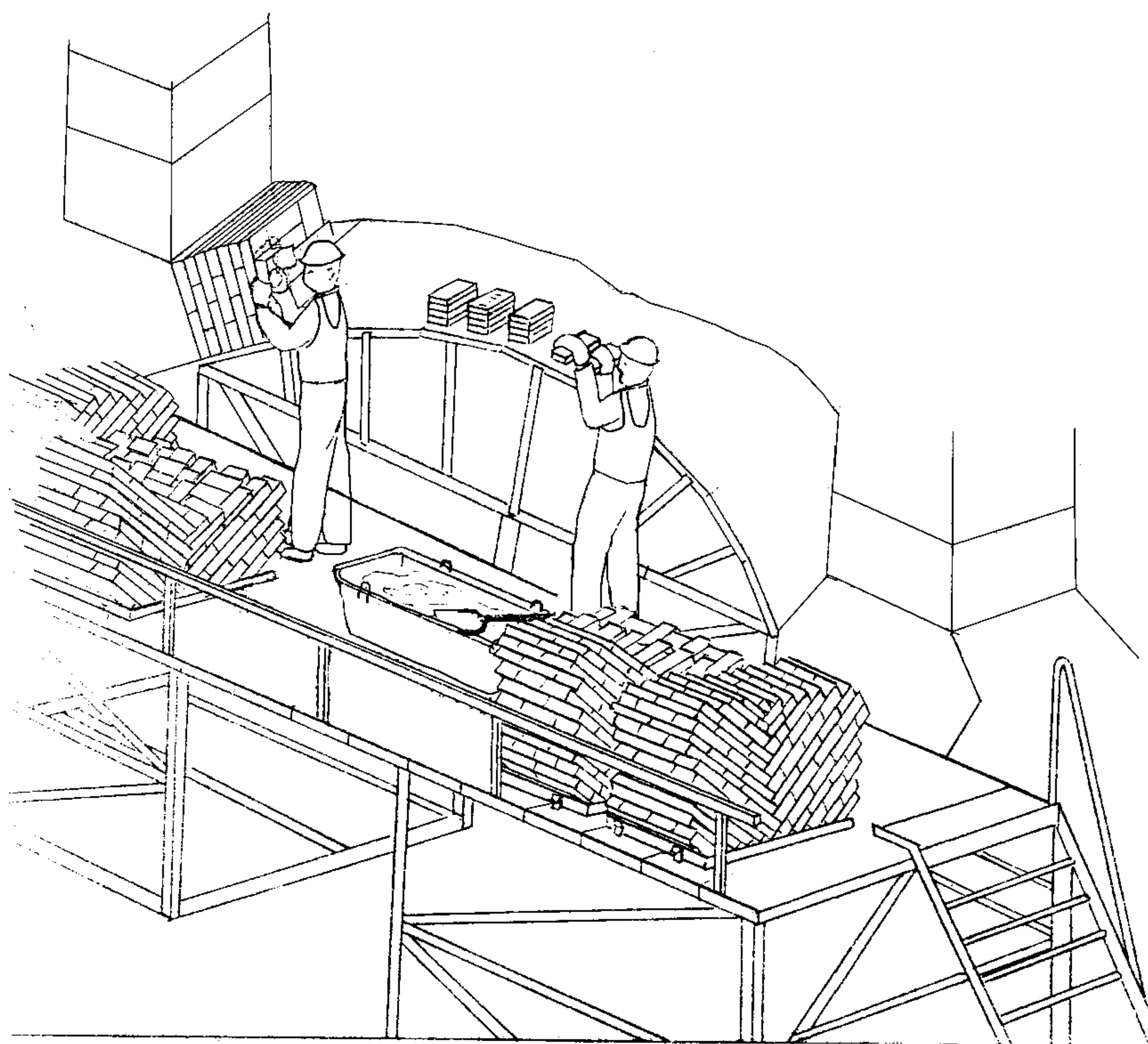
Рисунок 8 – Кладка арки (свода)
