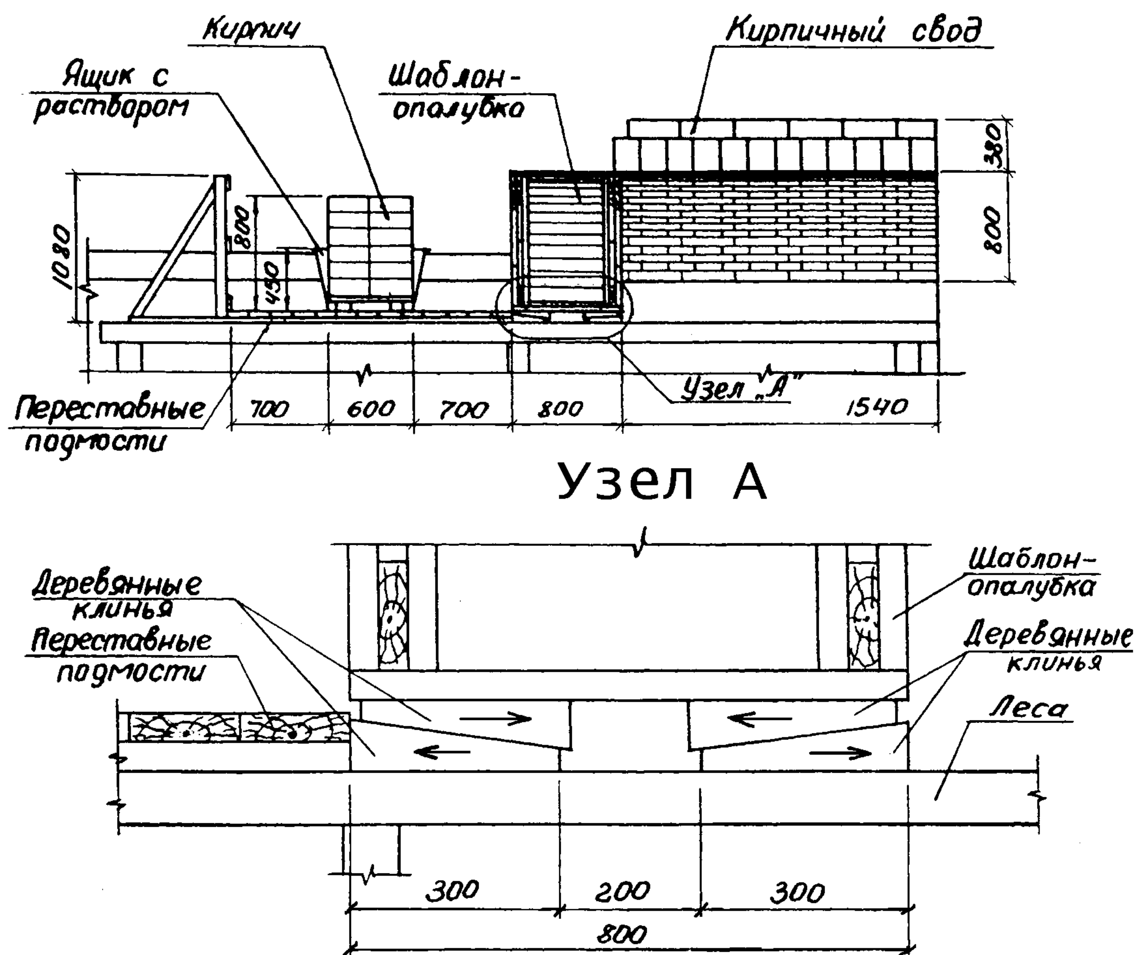
Рисунок 6 – Схема установки и демонтажа шаблона-опалубки
