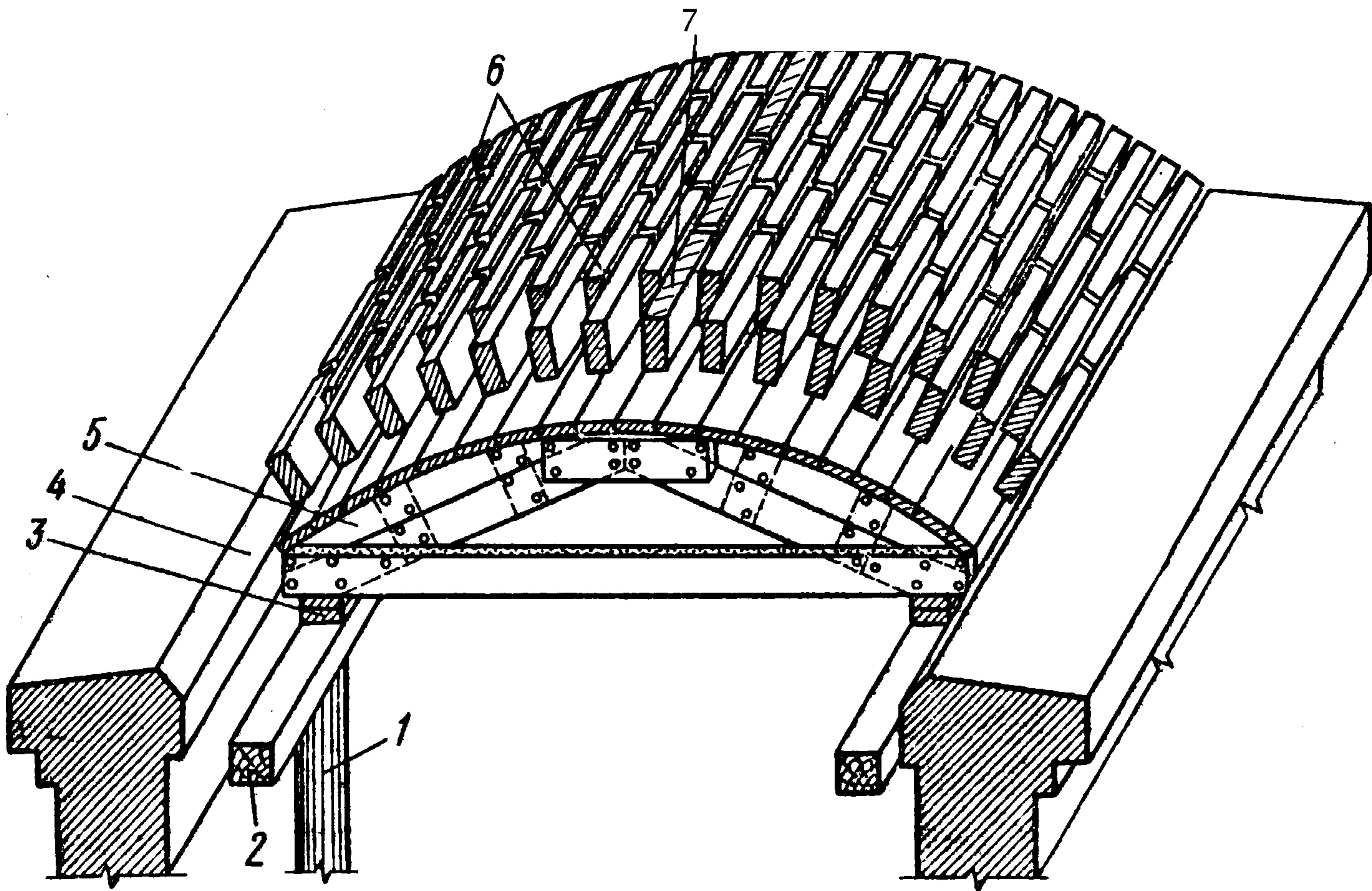
1 – стойка; 2 – горизонтальный брус, поддерживающий опалубку; 3 – клинья; 4 – пятa; 5 – круглая опалубка; 6 – ряды, образующие свод; 7 – замковый ряд
