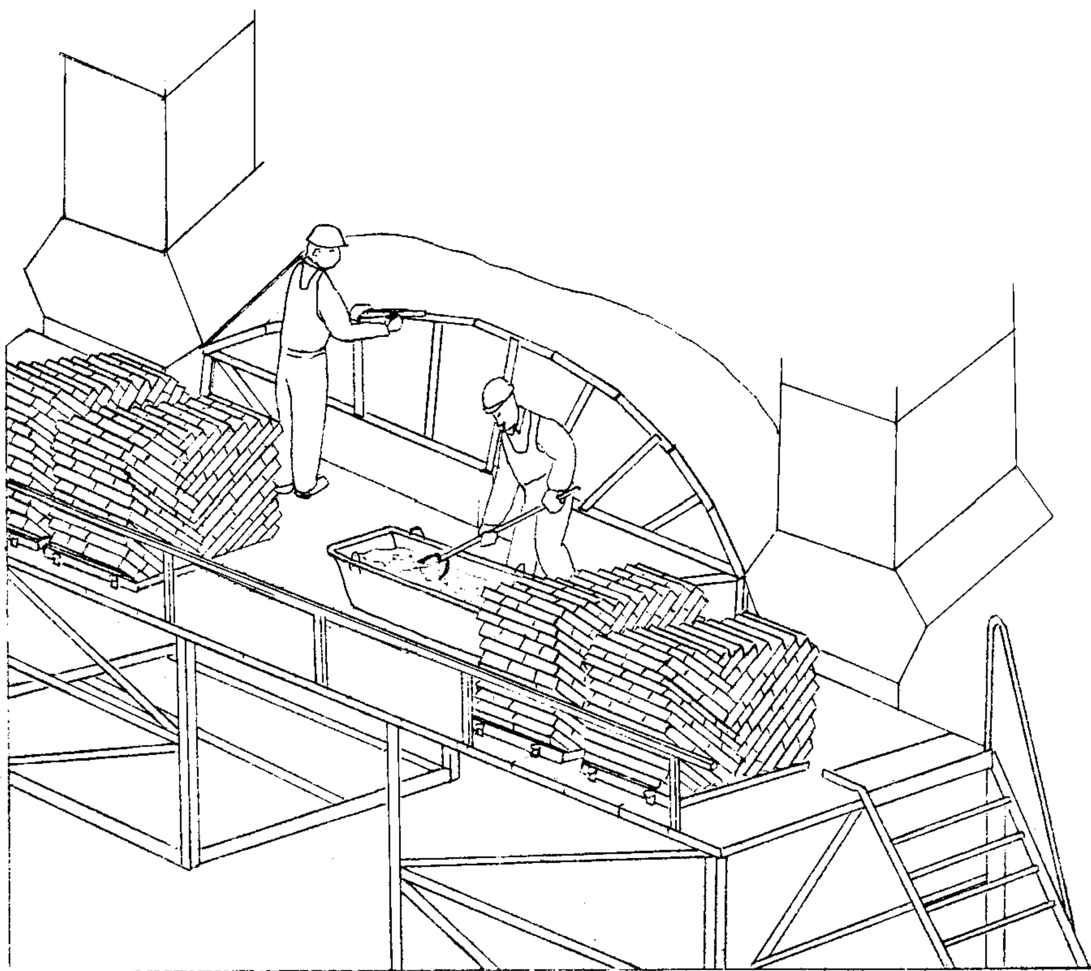
Рисунок 7 – Разметка места укладки кирпичей по опалубке
