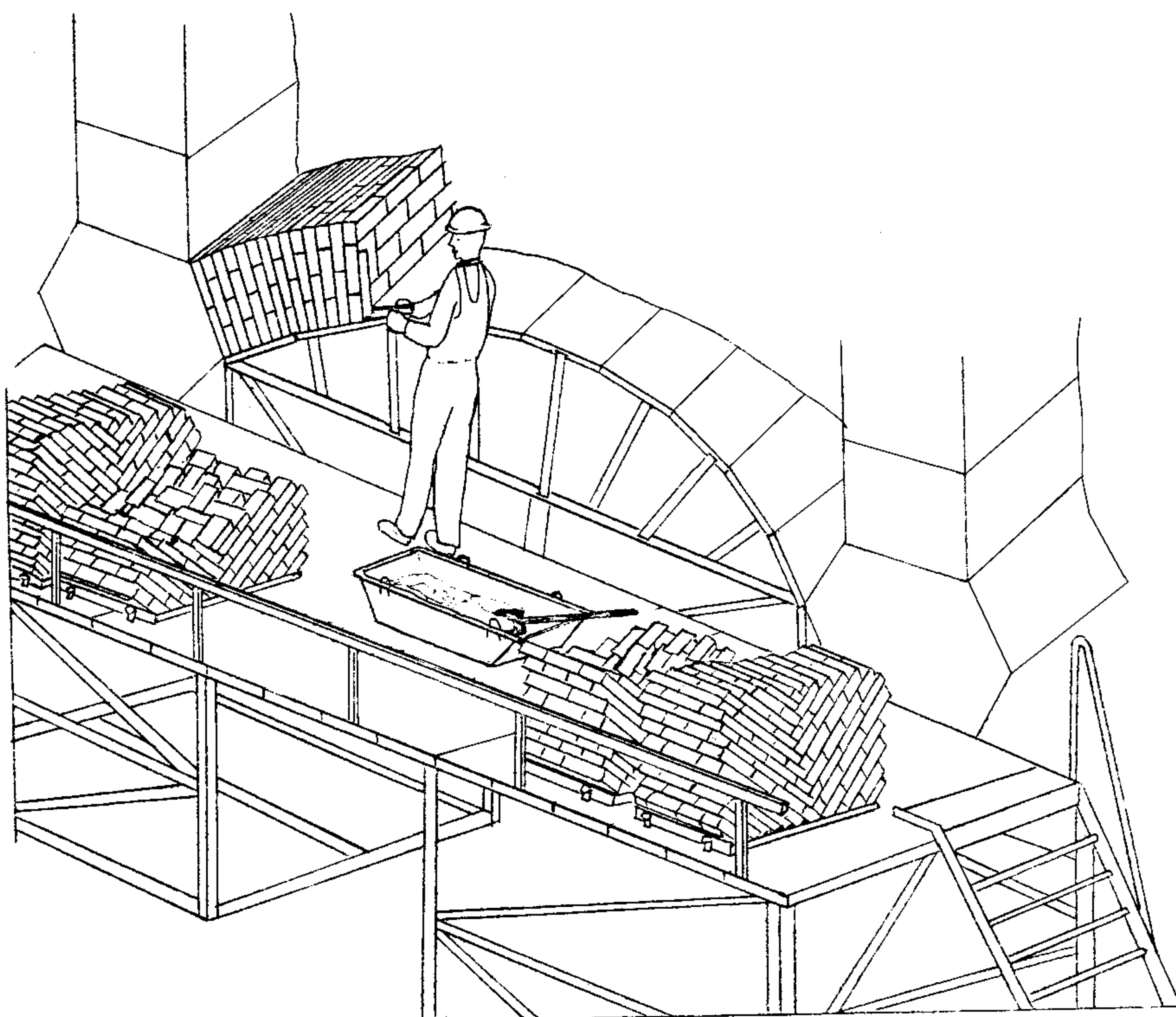
Рисунок 9 – Выверка кладки
