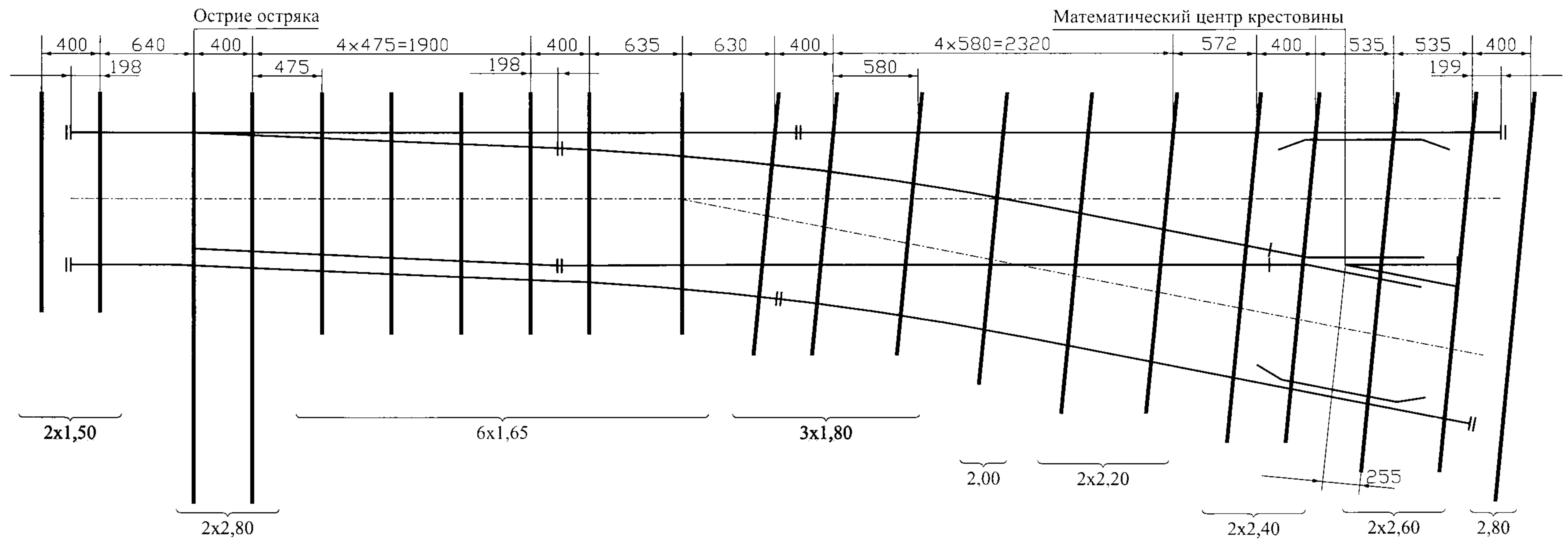
Схема укладки стрелочного перевода т.Р24 м.1/5 пр. 9245.000.00
