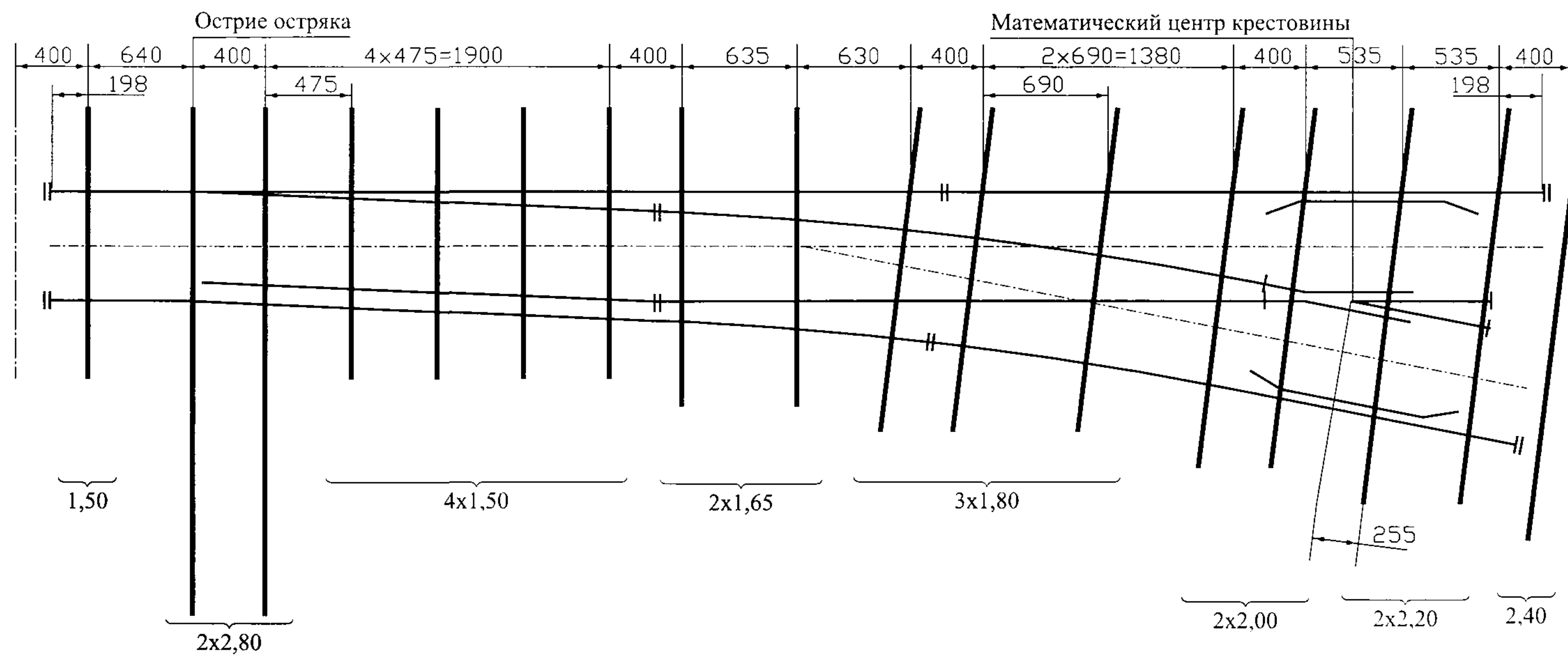
Схема укладки стрелочного перевода т.Р24 м.1/5 пр. 6245.00.000
