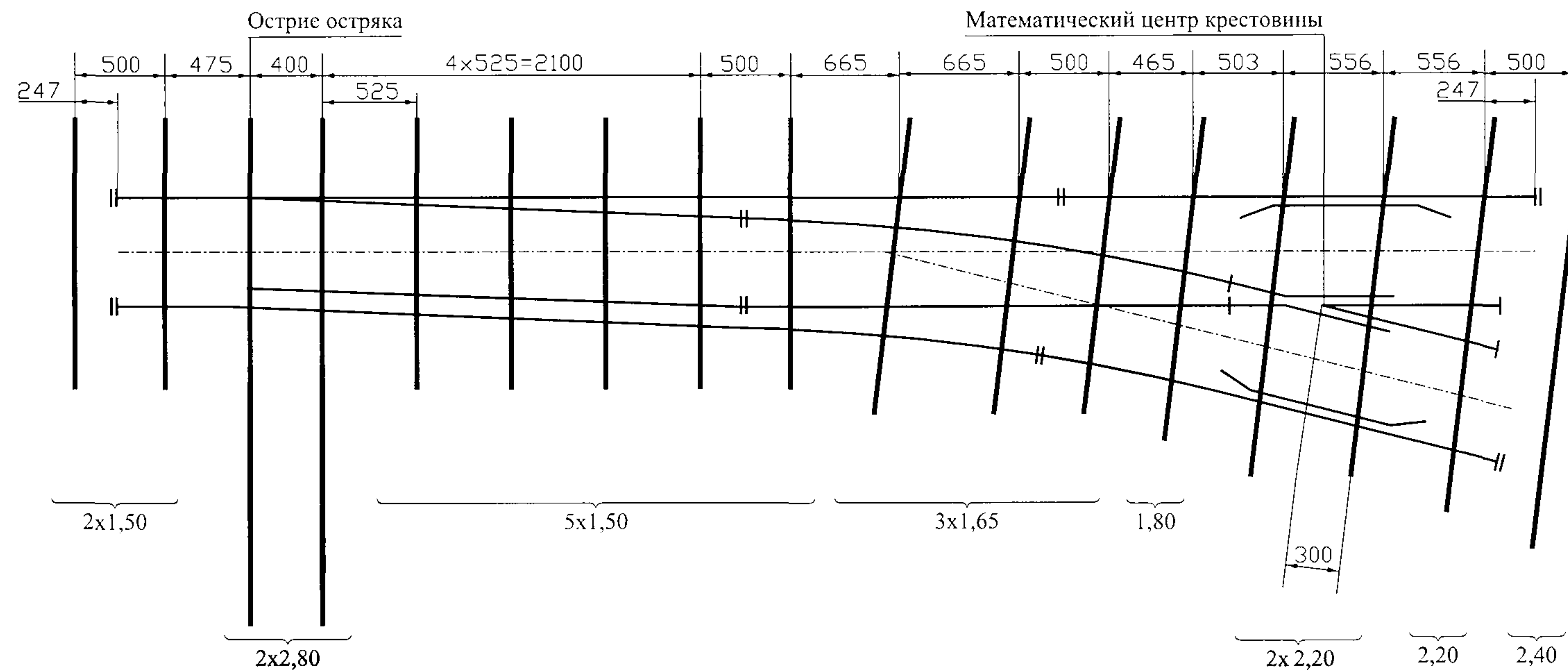
Схема укладки стрелочного перевода т.РЗЗ м.1/4 пр. 6334.000.00
