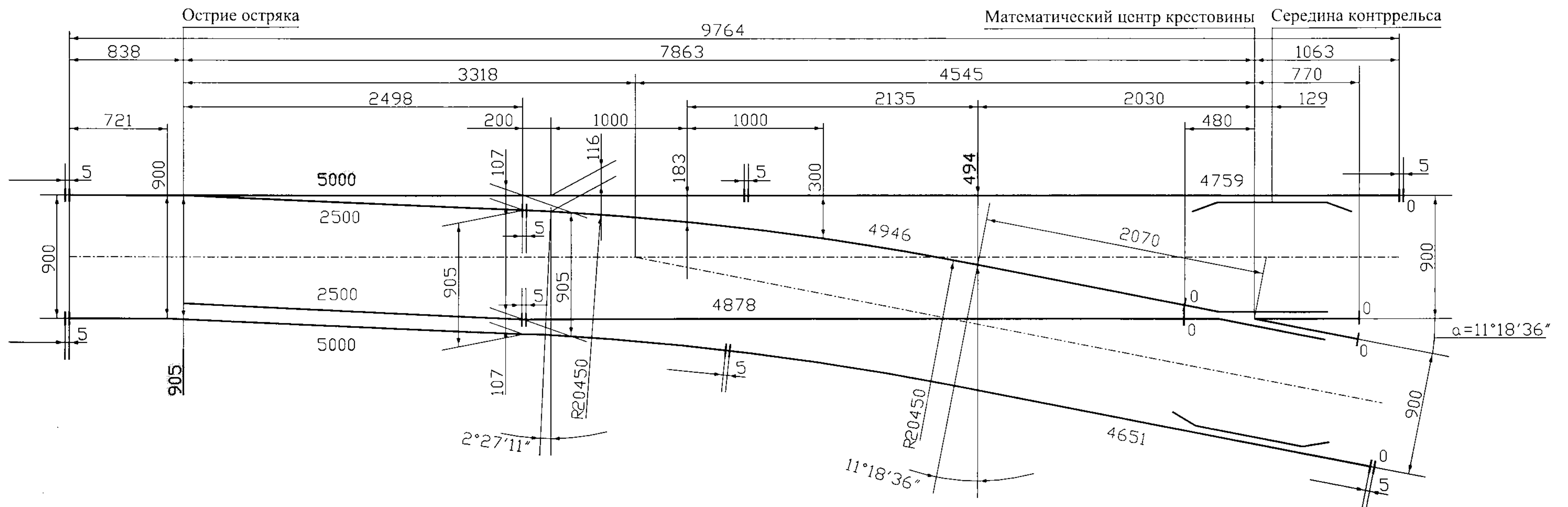
Схема геометрических размеров стрелочного перевода т.Р24 м.1/5 пр. 9245.000.00
