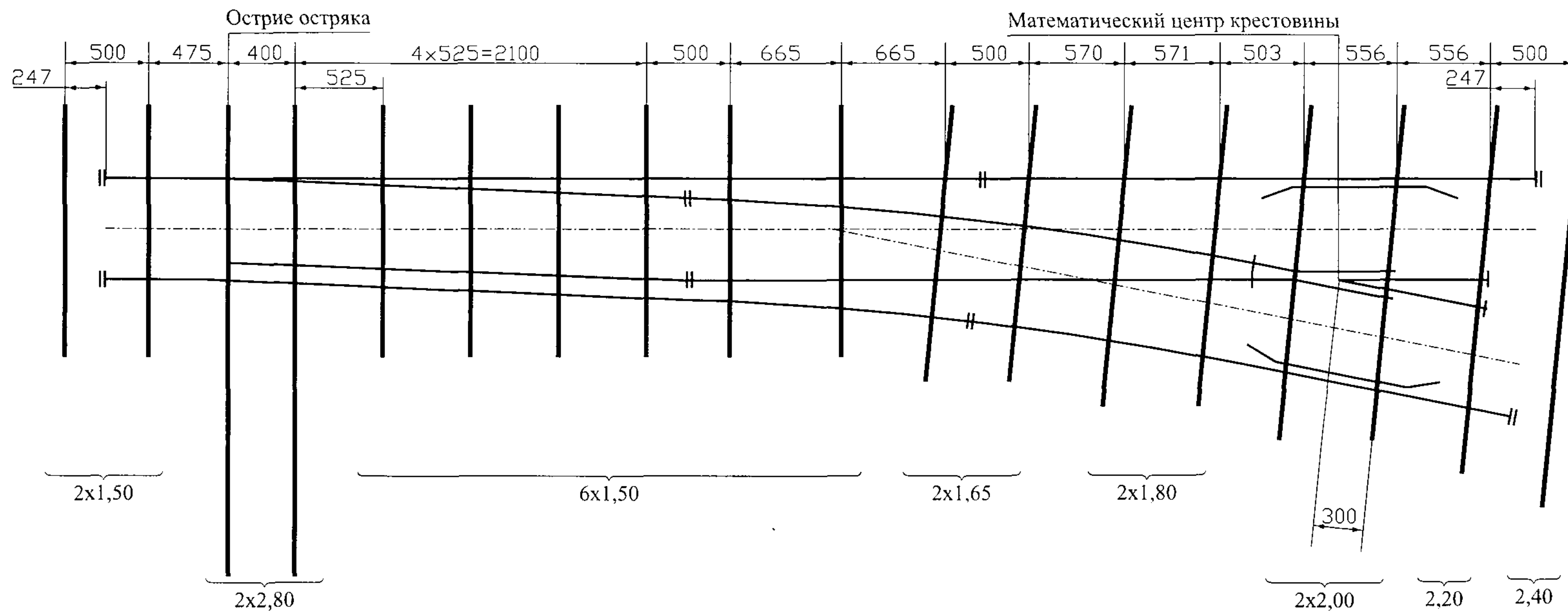
Схема укладки стрелочного перевода т.РЗЗ м.1/5 пр. 6335.000.00
