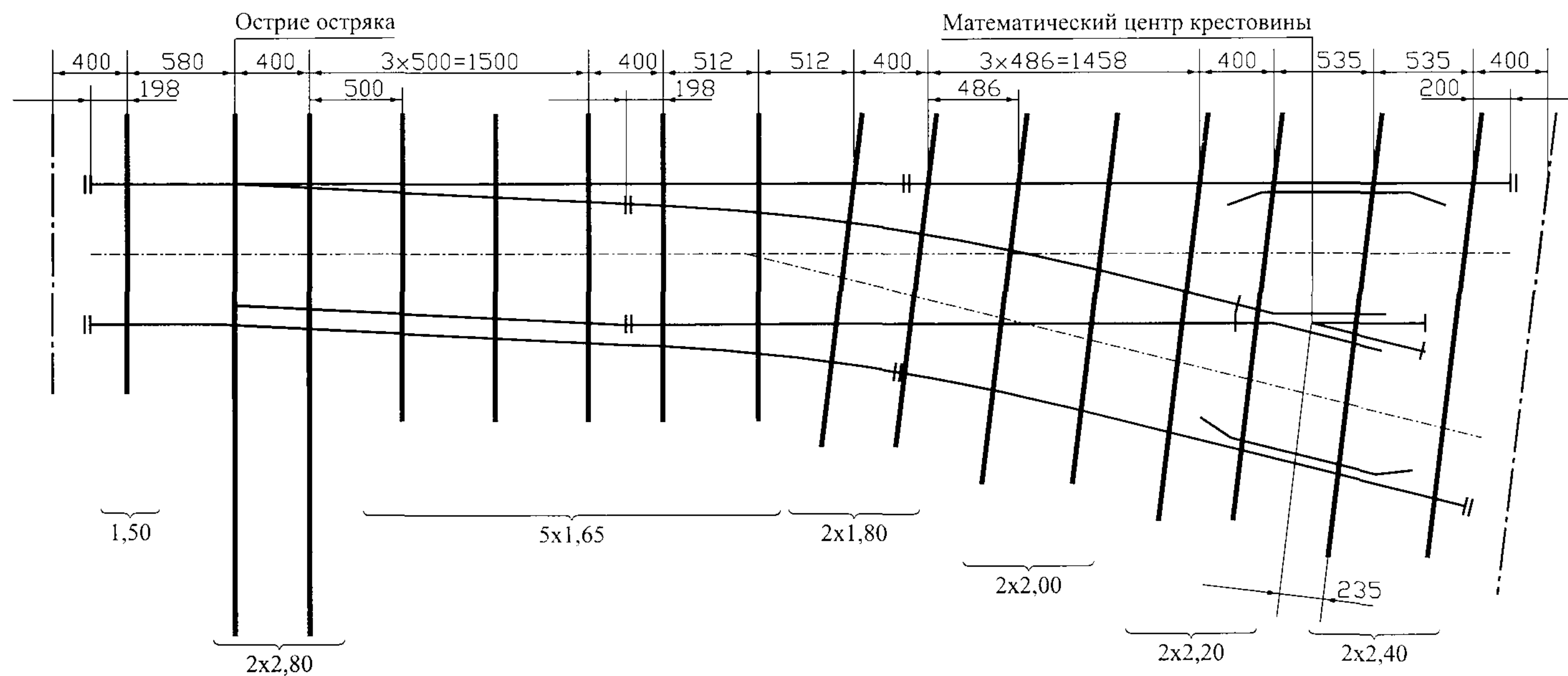
Схема укладки стрелочного перевода т.Р24 м.1/4 пр. 7244.00.000
