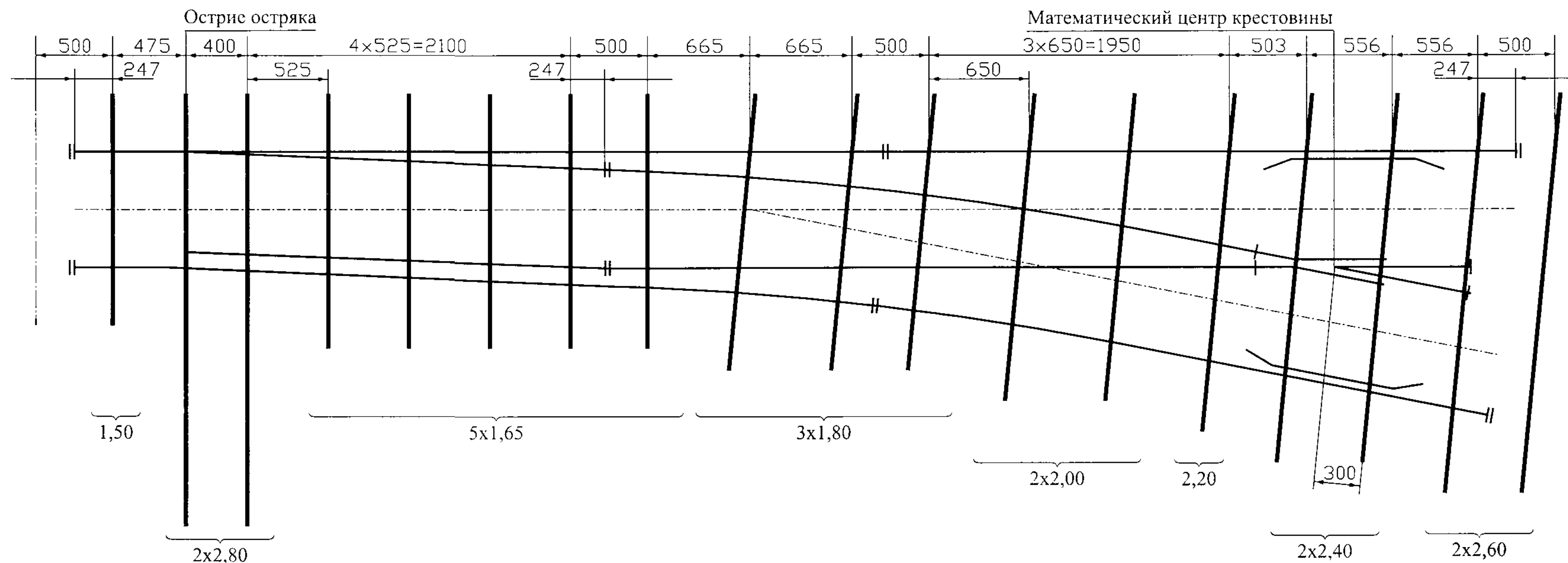
Схема укладки стрелочного перевода т.РЗЗ, марка 1/5 Проект 7335.000.00
