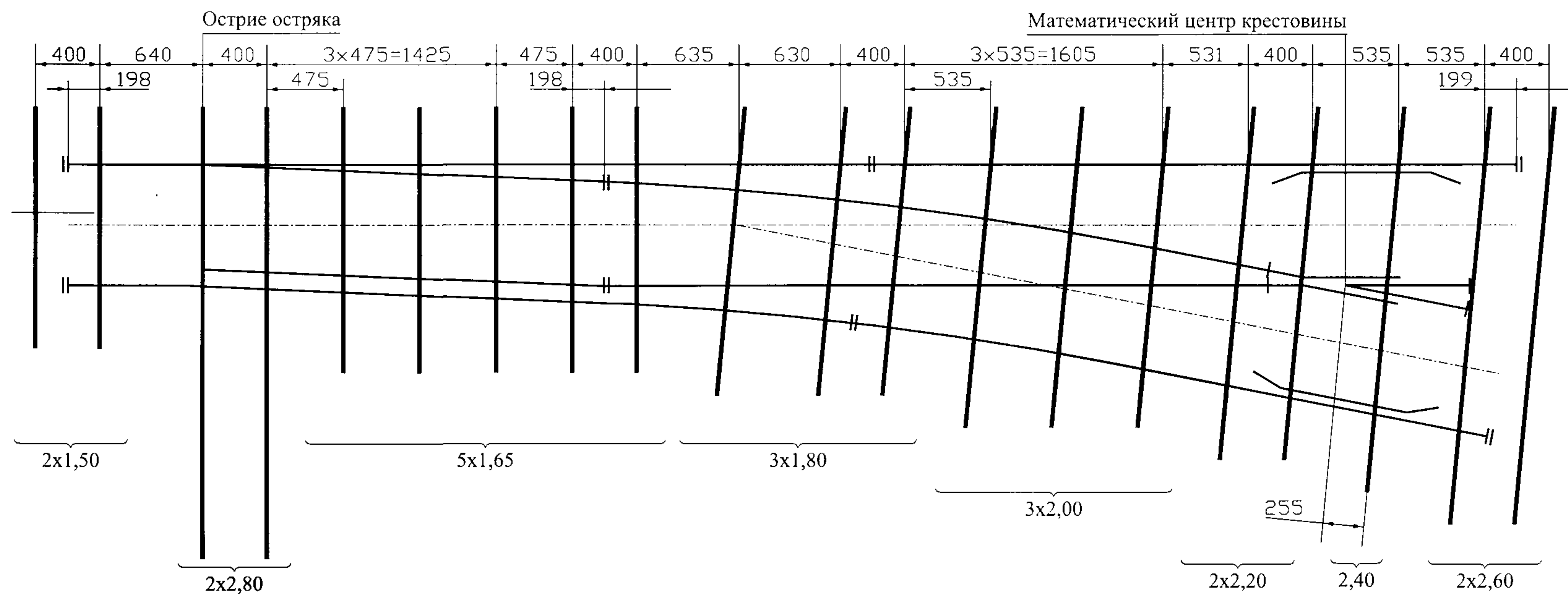
Схема укладки стрелочного перевода т.Р24 м.1/5 пр. 7245.00.000
