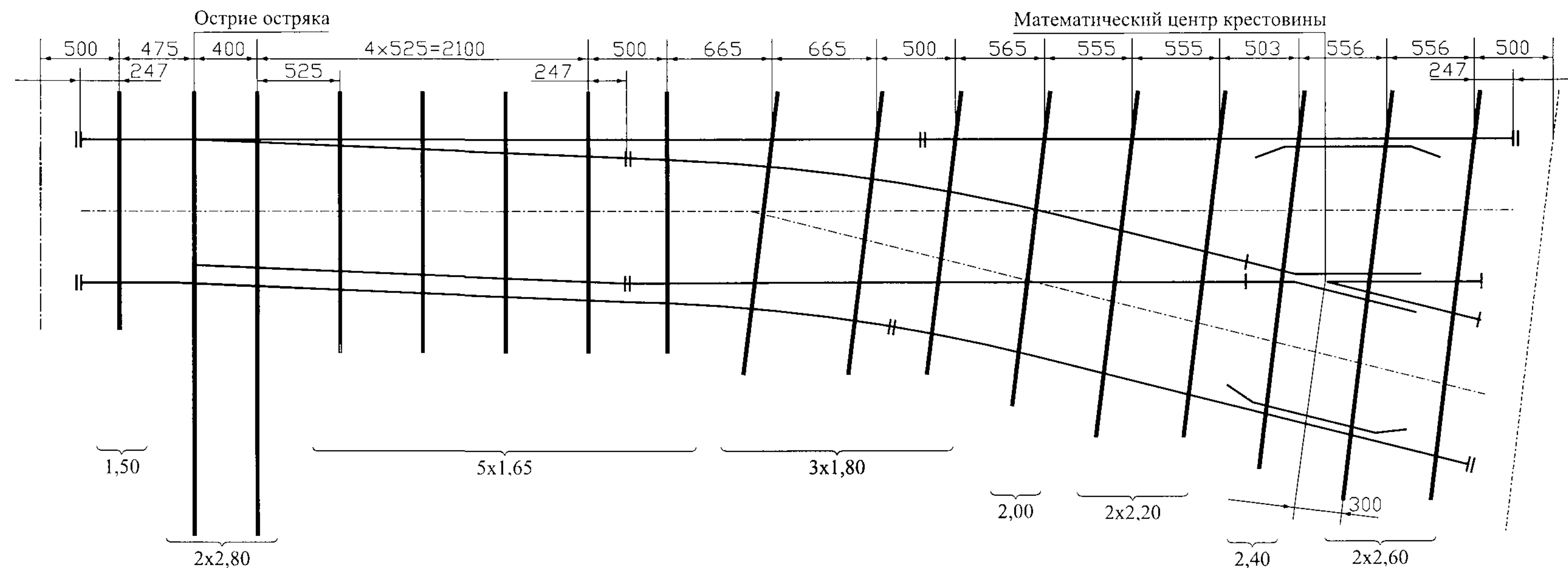
Схема укладки стрелочного перевода т.РЗЗ м.1/4 пр. 9334.000.00
