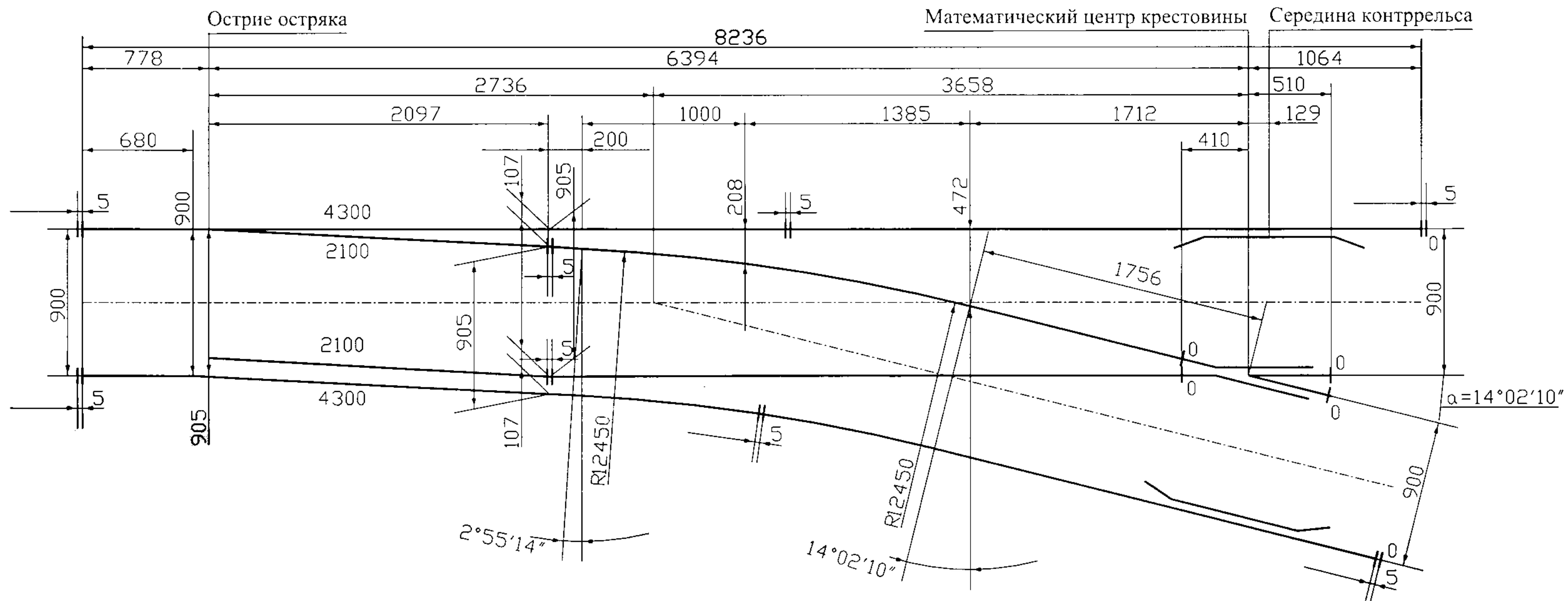
Схема геометрических размеров стрелочного перевода т.Р24 м.1/4 пр. 9244.000.00
