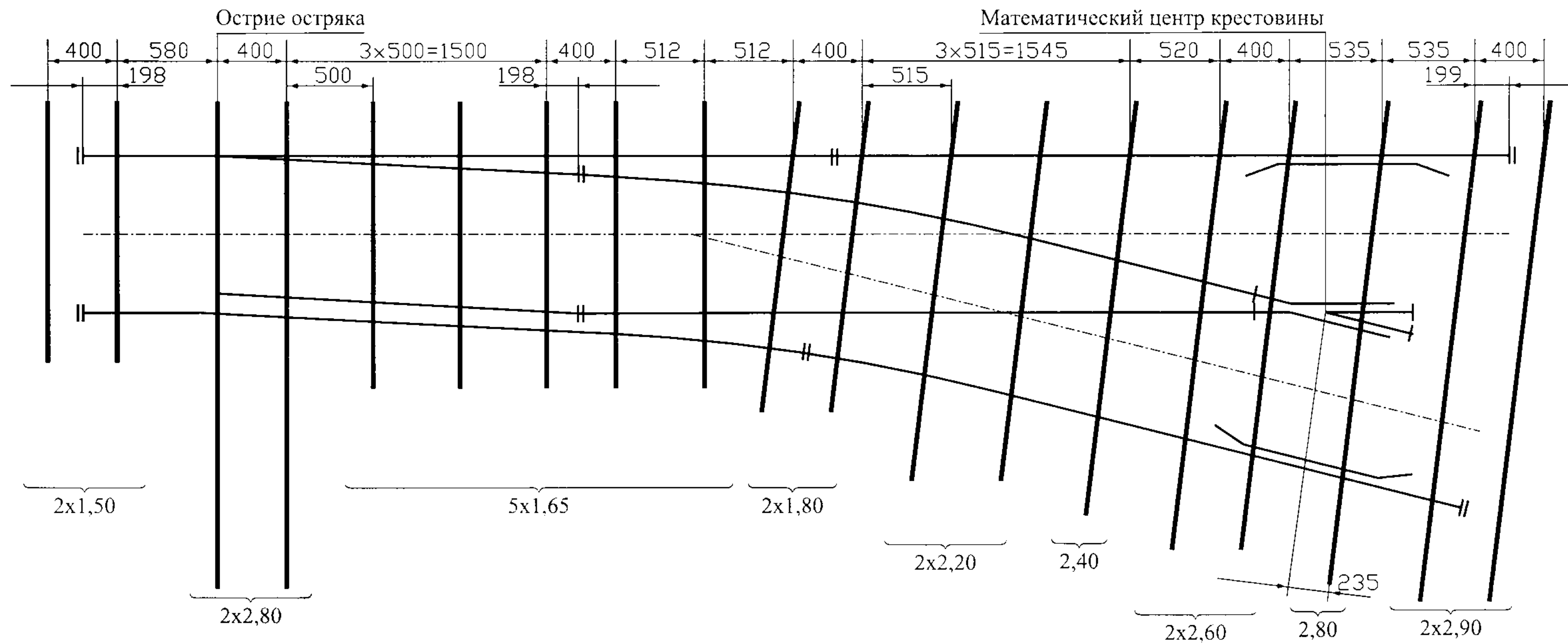
Схема укладки стрелочного перевода т.Р24 м.1/4 пр. 9244.000.00
