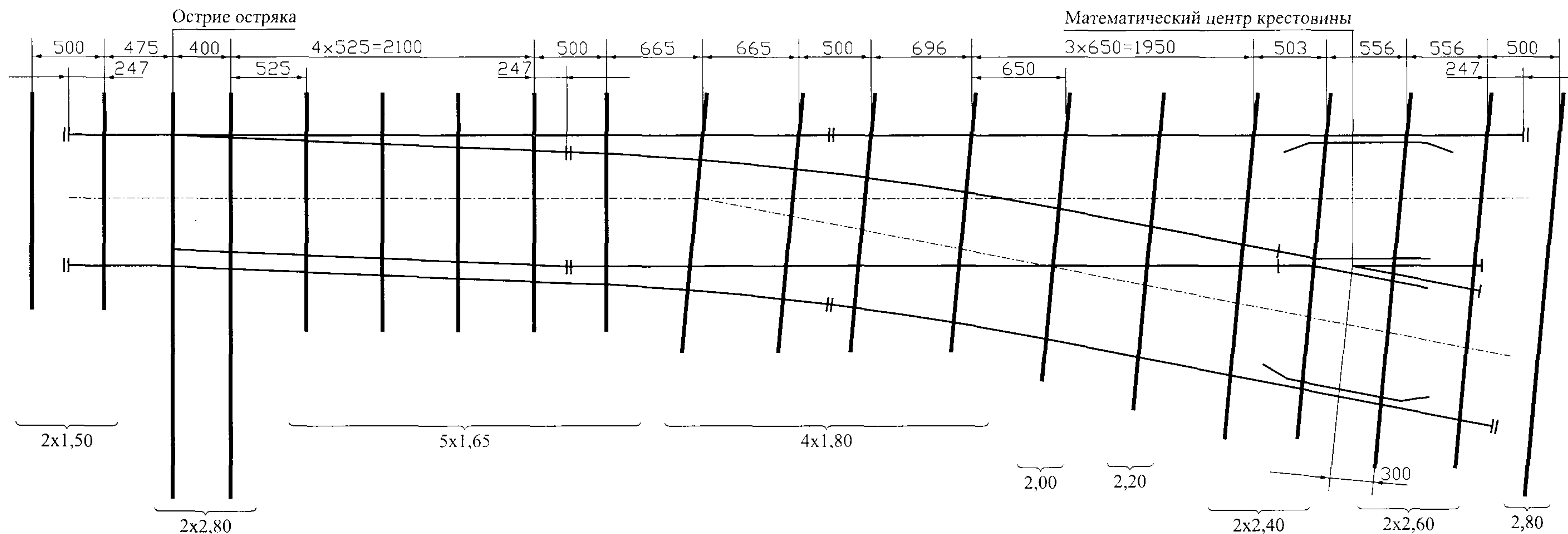
Схема укладки стрелочного перевода т.РЗЗ м.1/5 пр. 9335.000.00
