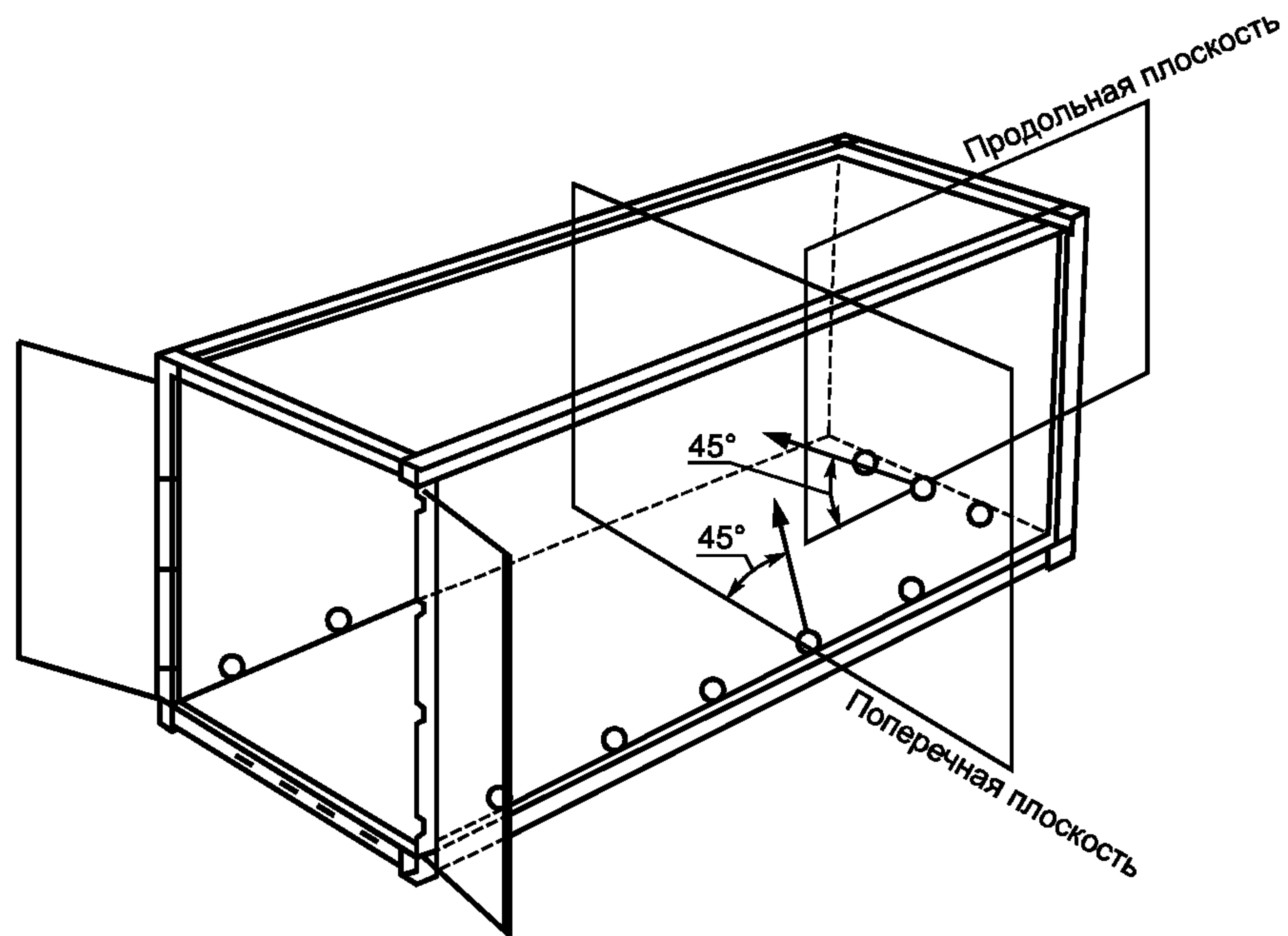
Рисунок Е.1 — Схема приложения испытательных нагрузок
