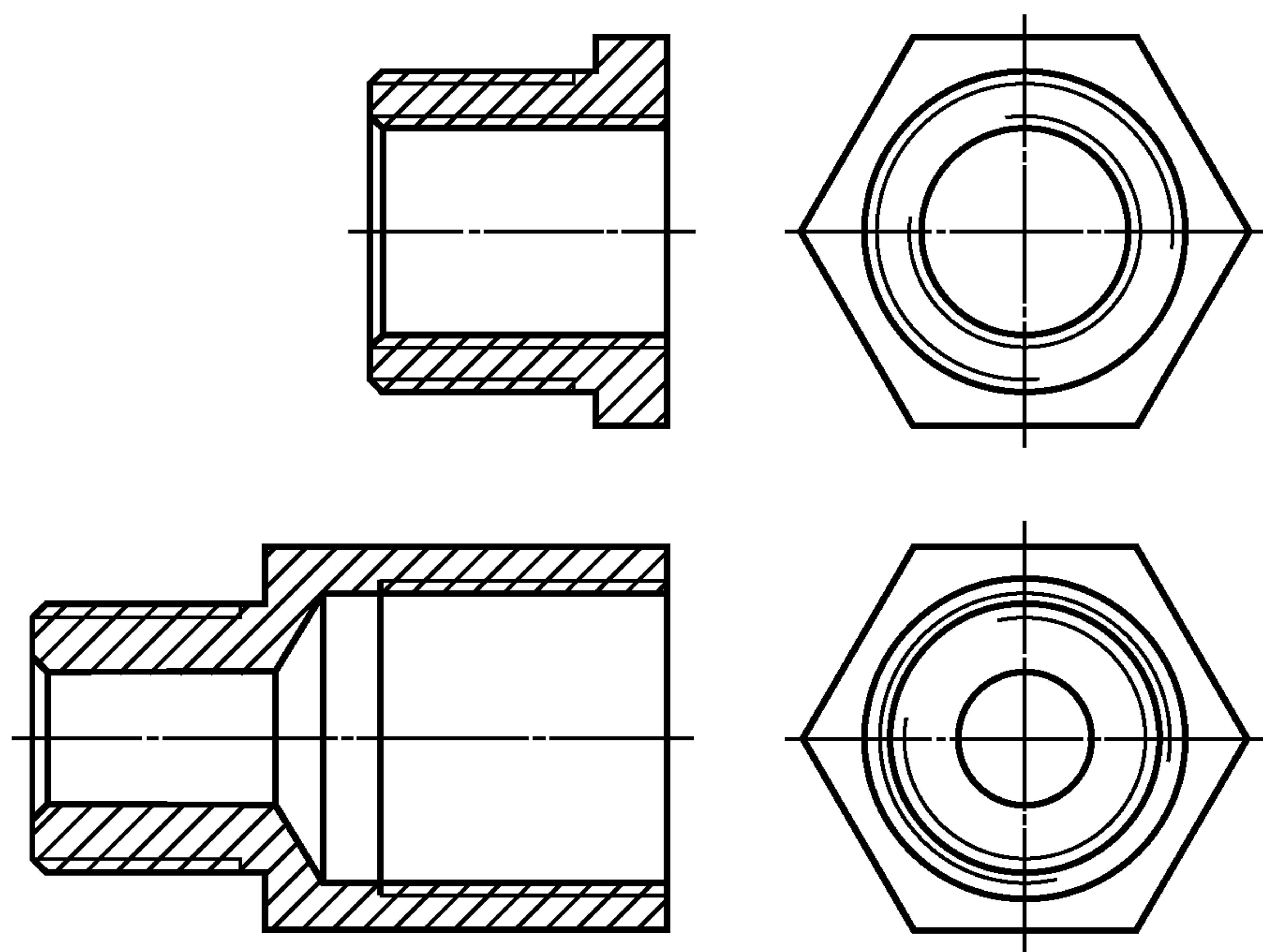
Рисунок С.2 — Примеры Ex-переходников
