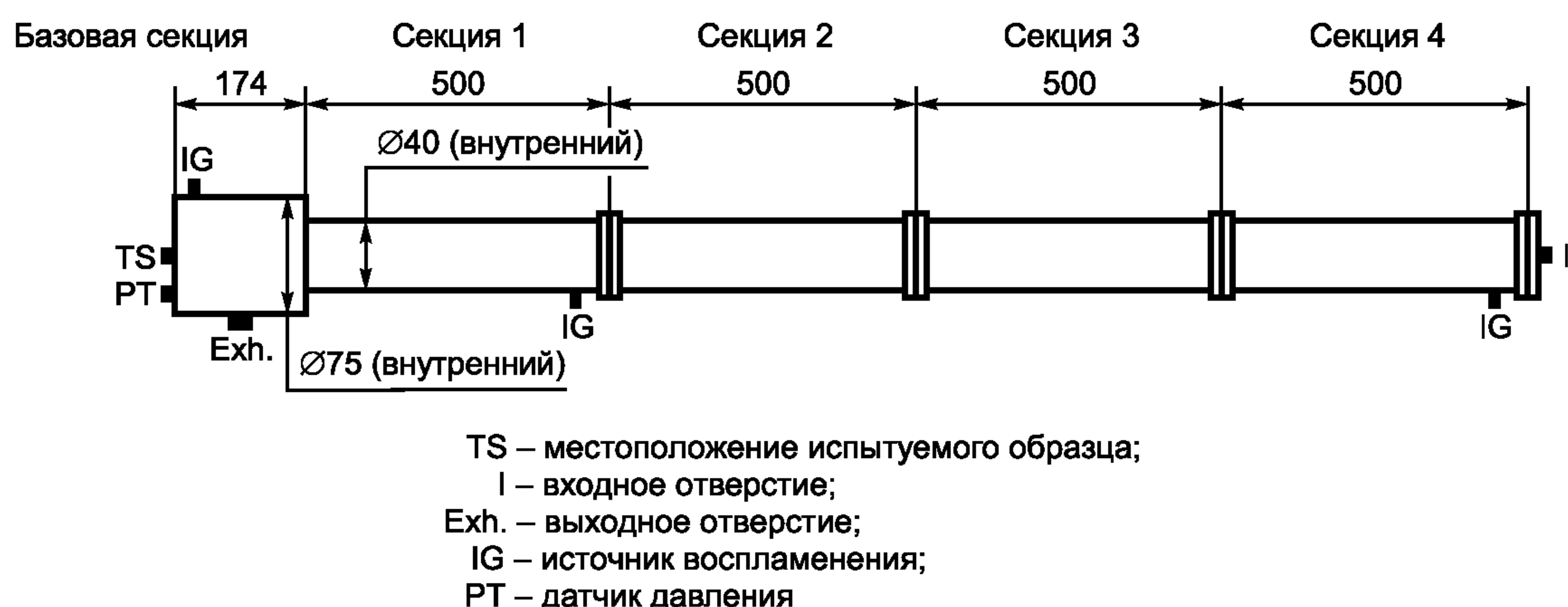
Рисунок 21 — Установка для испытаний дыхательных и дренажных устройств
