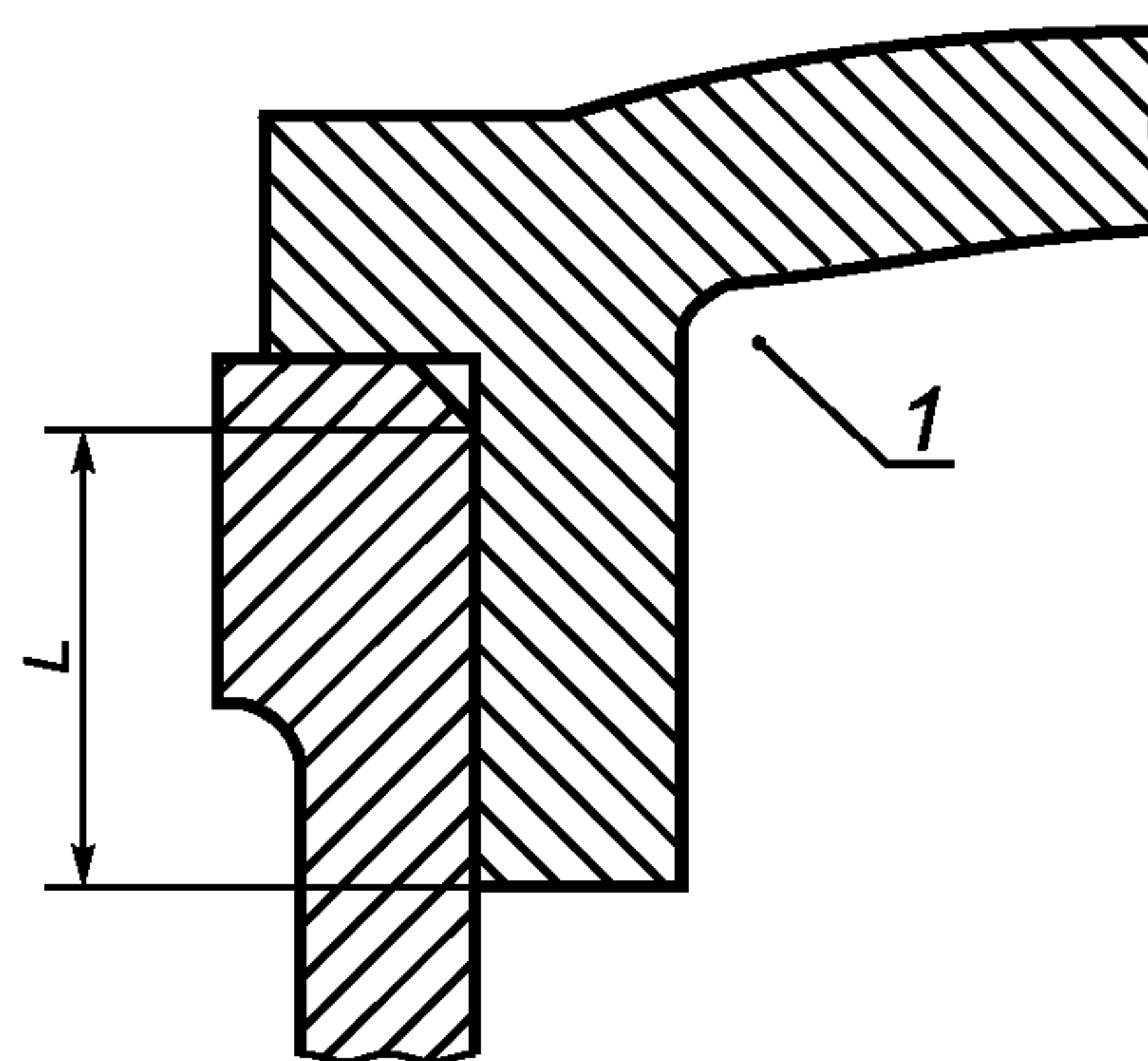
Рисунок 2б — Только цилиндрическая часть
