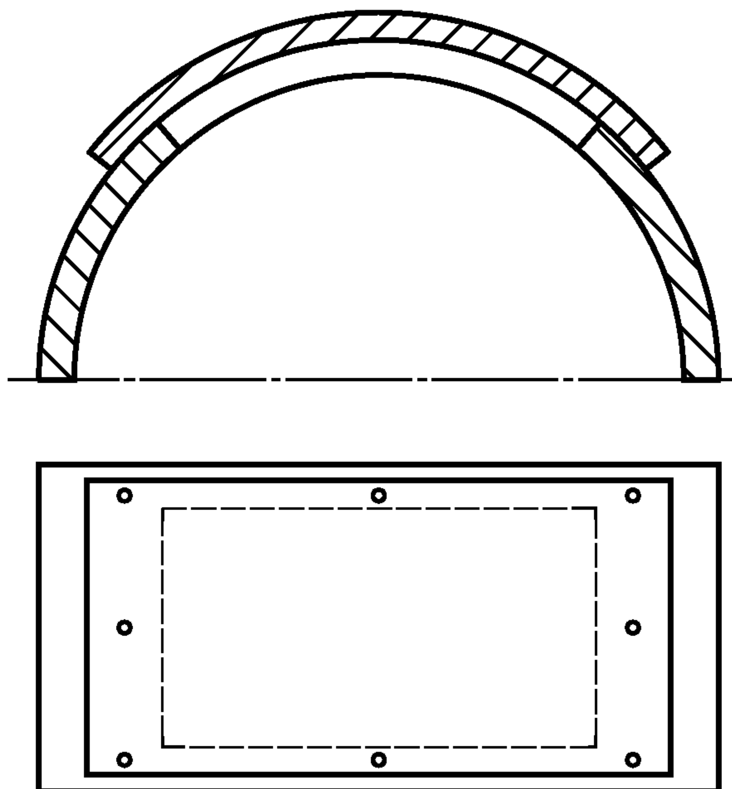
Рисунок 9а — Пример соединения с частично цилиндрическими поверхностями
