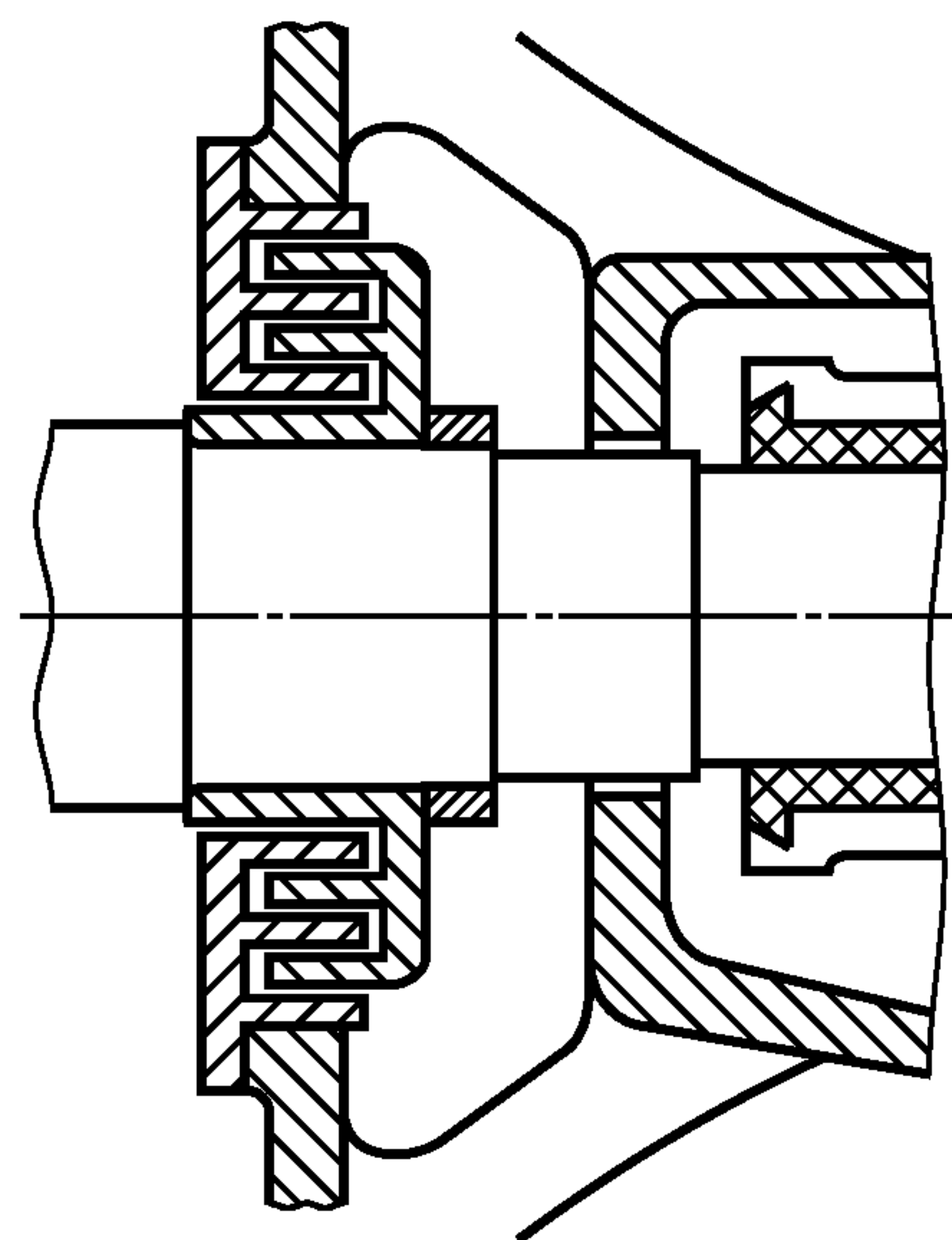
Рисунок 18 — Лабиринтное соединение для валов вращающихся электрических машин
