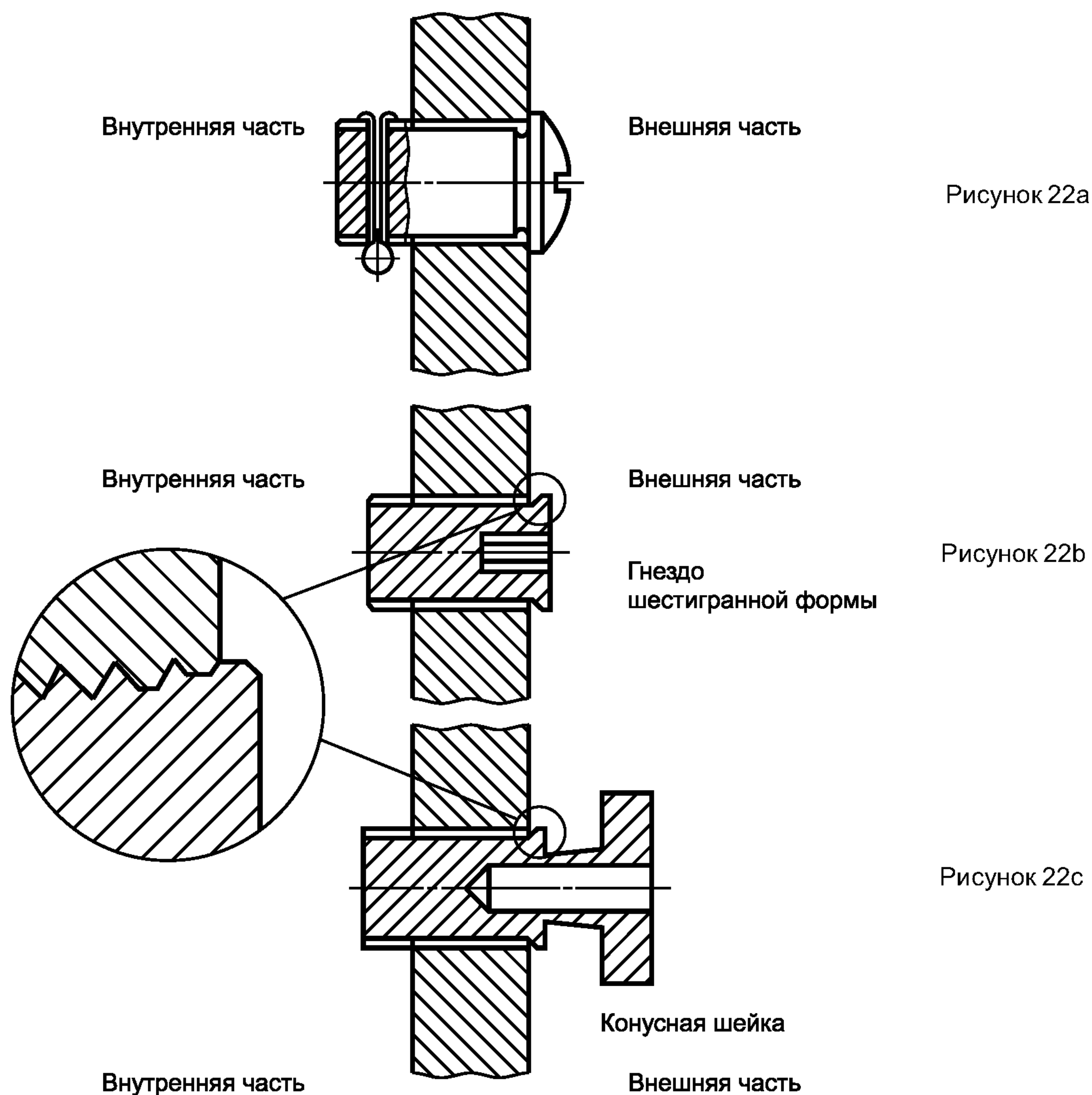
Рисунок 22 — Примеры заглушек для неиспользованных отверстий
