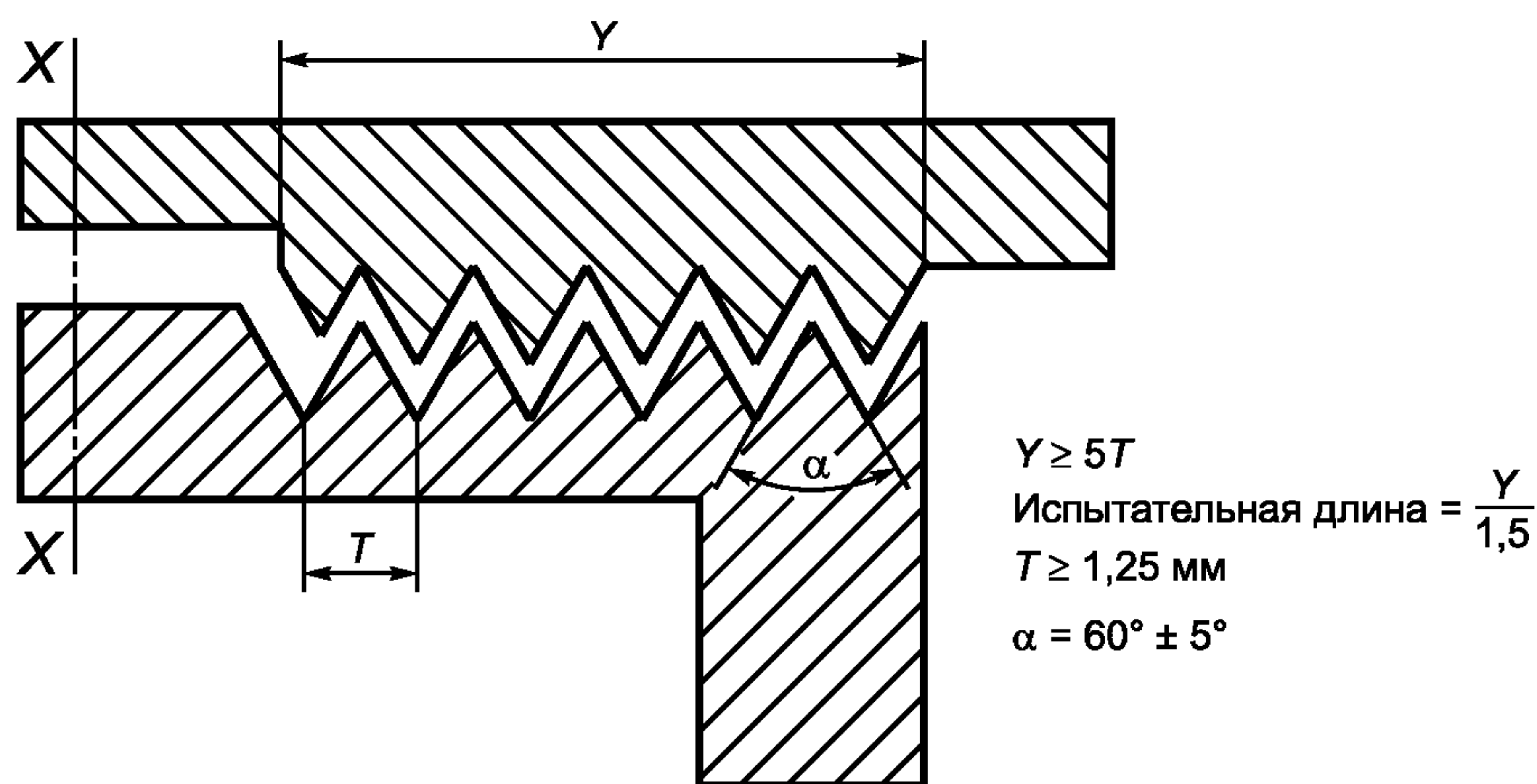
Рисунок 9b — Пример зубчатого соединения
