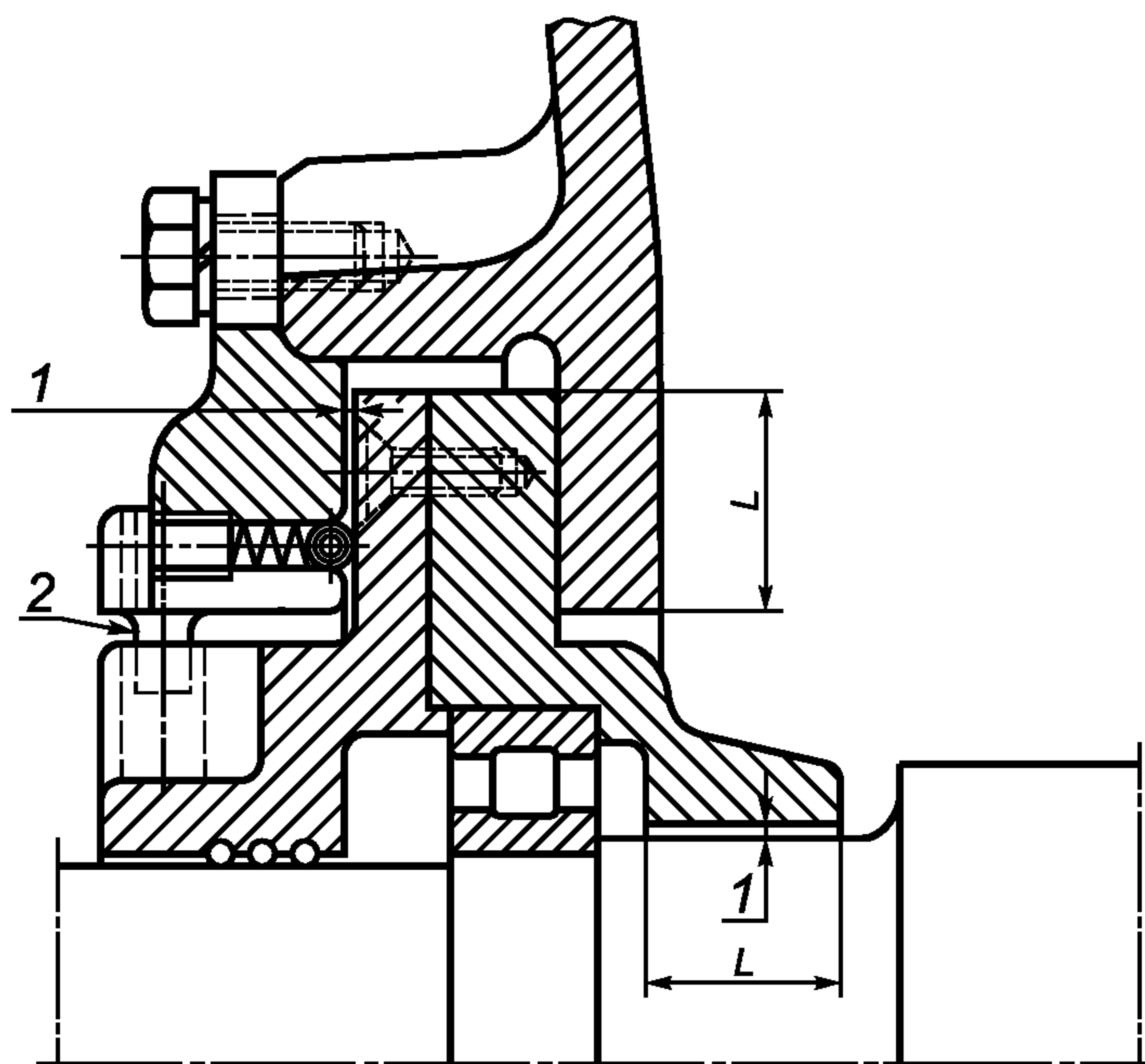
1 — зазор; 2 — стопор для предотвращения проворачивания втулки
