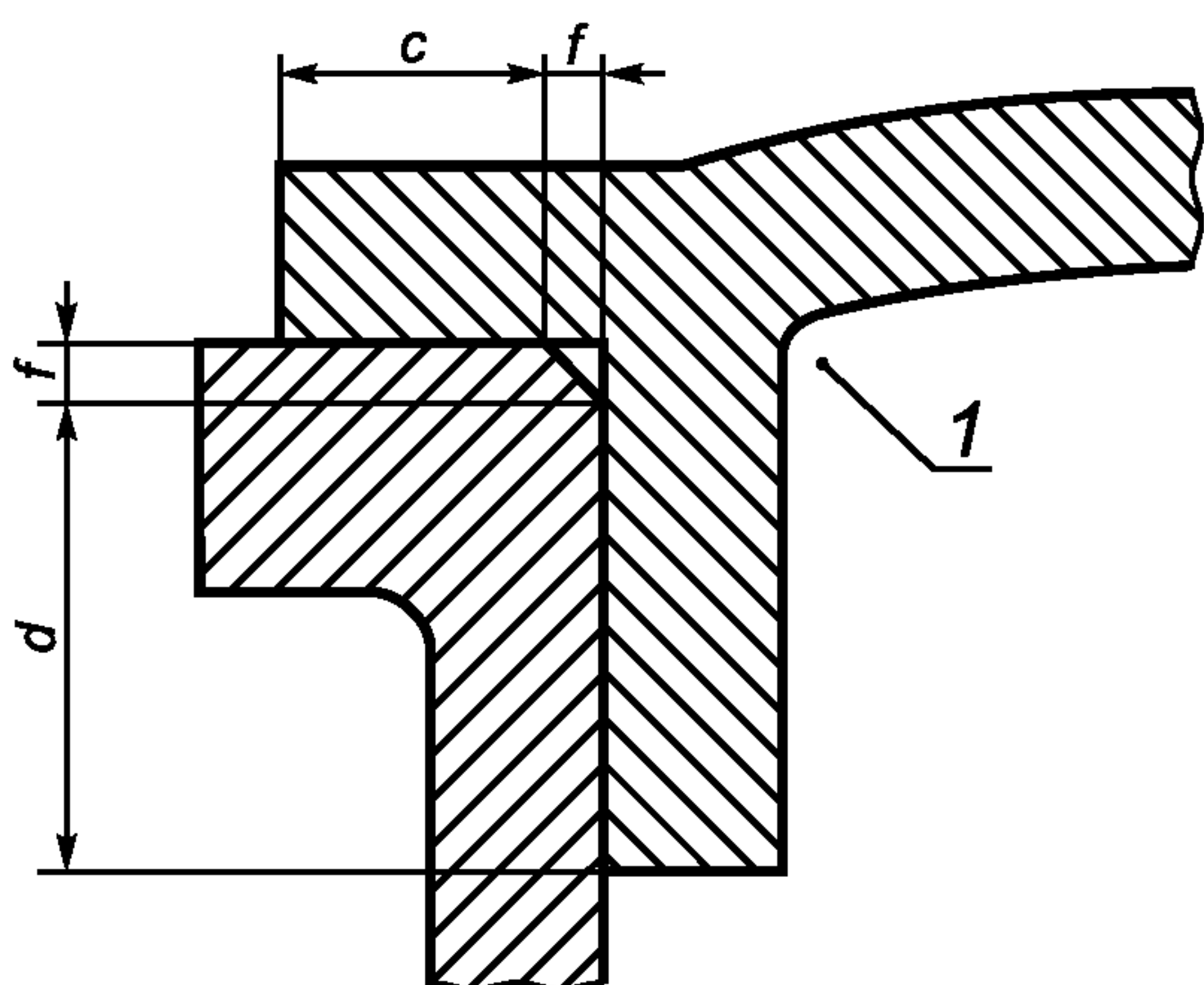
Рисунок 2а — Цилиндрическая и плоская части
