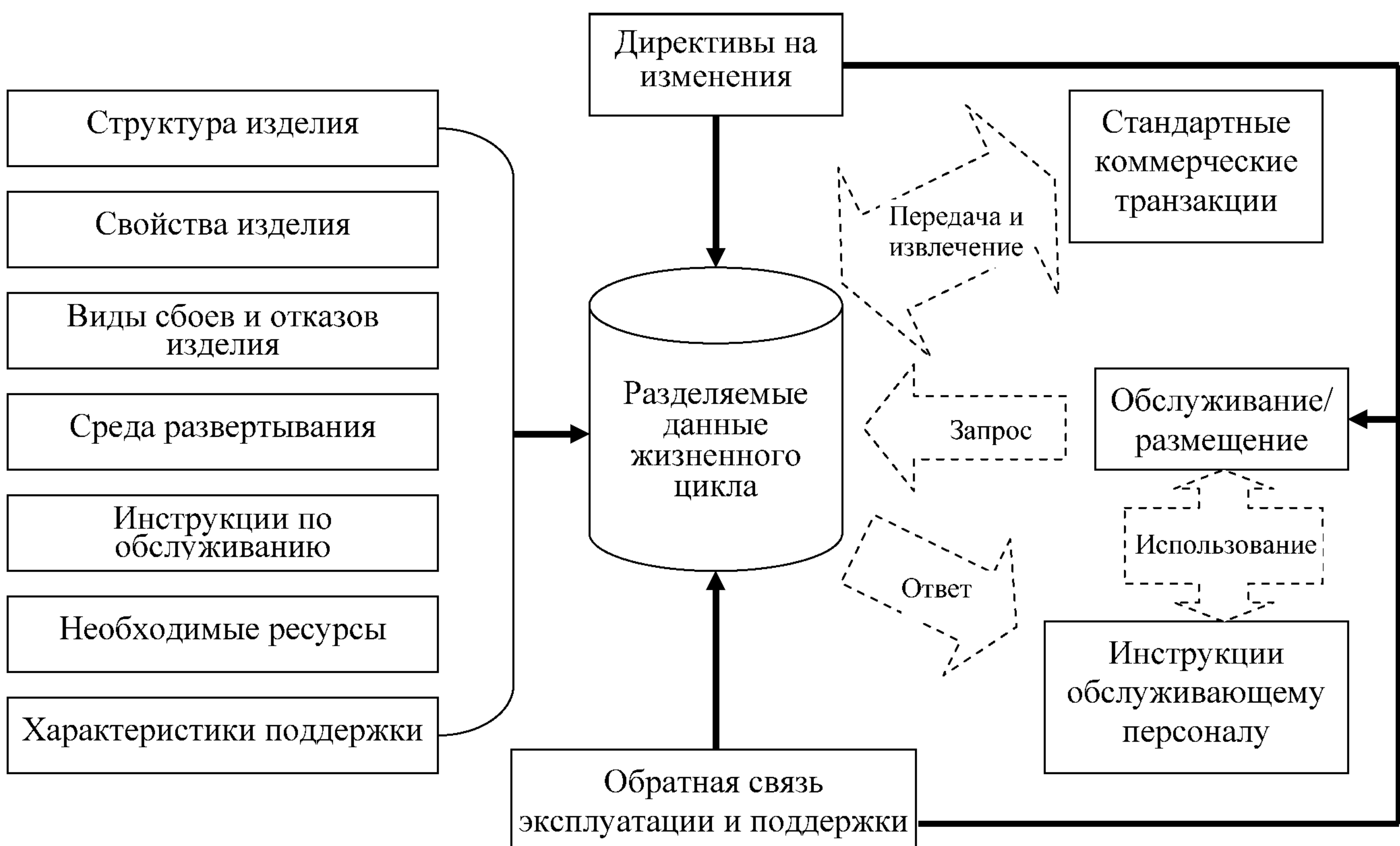
Рисунок 1 — Визуальное представление ПЖЦИ
