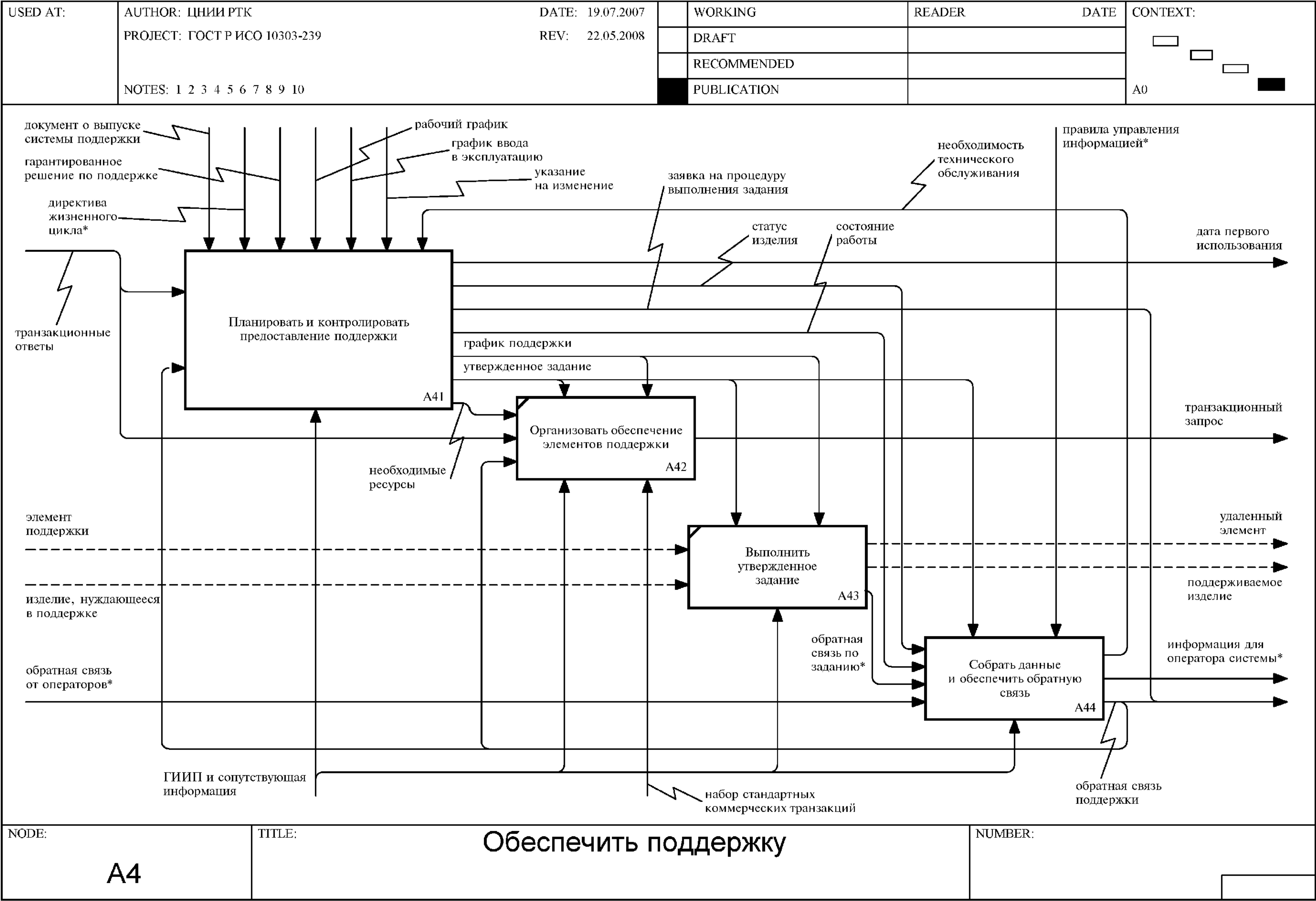
Рисунок F.37 — Диаграмма A4: Обеспечить поддержку
