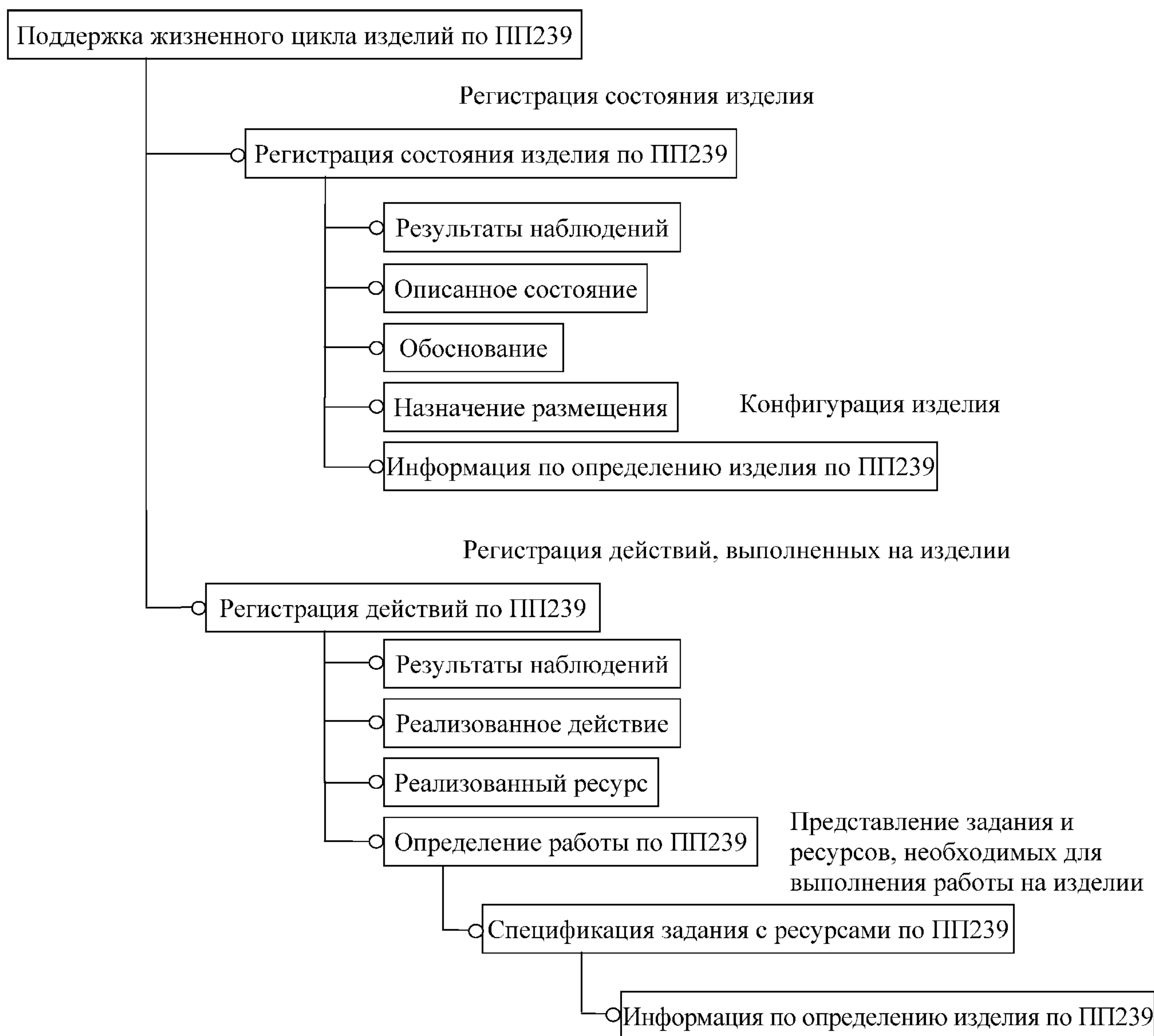
Рисунок 6 — Выделенная часть иерархии модулей прикладного протокола AP239_product_life_cycle_support
