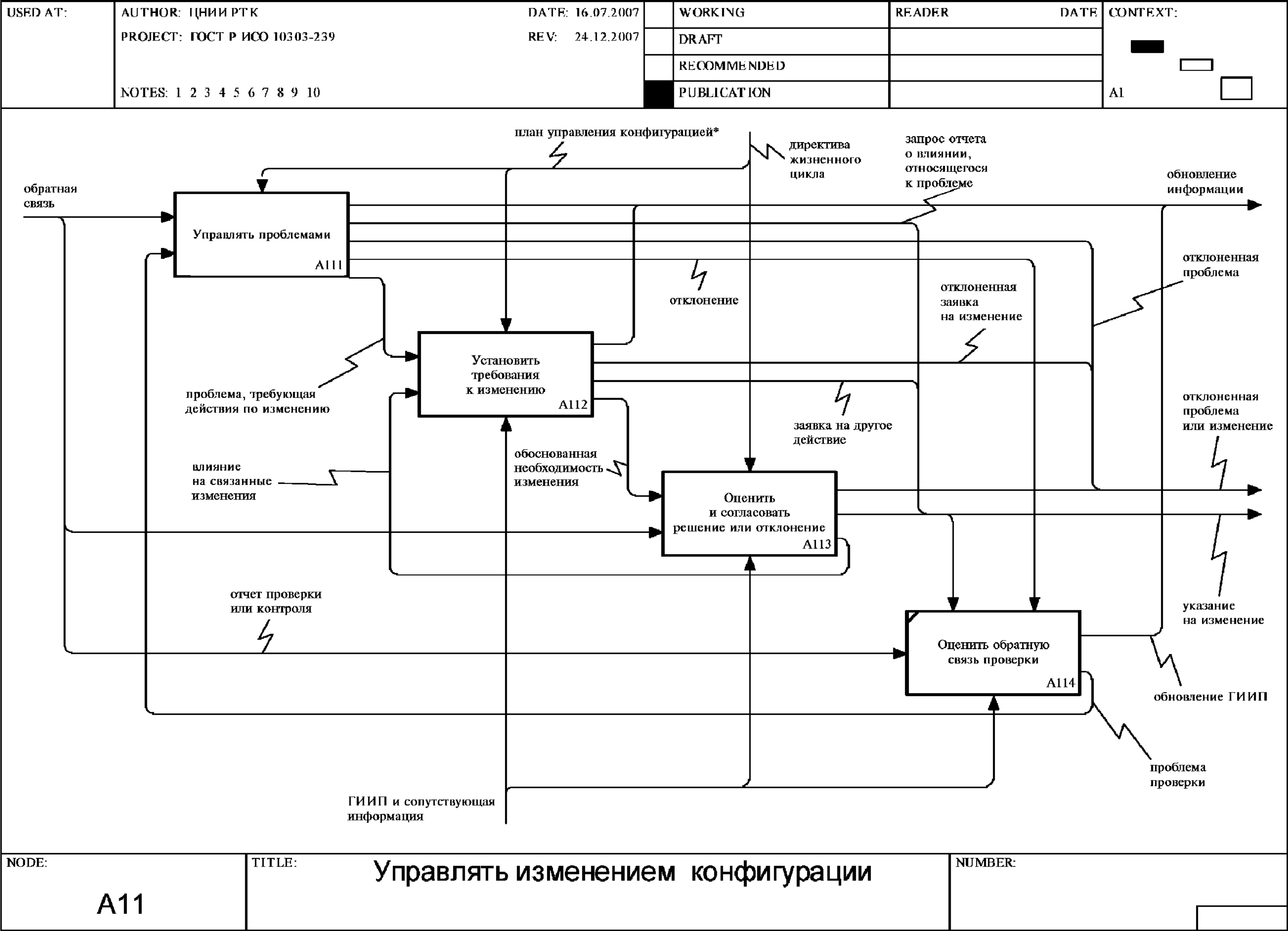
Рисунок F.4 — Диаграмма A11: Управлять изменением конфигурации
