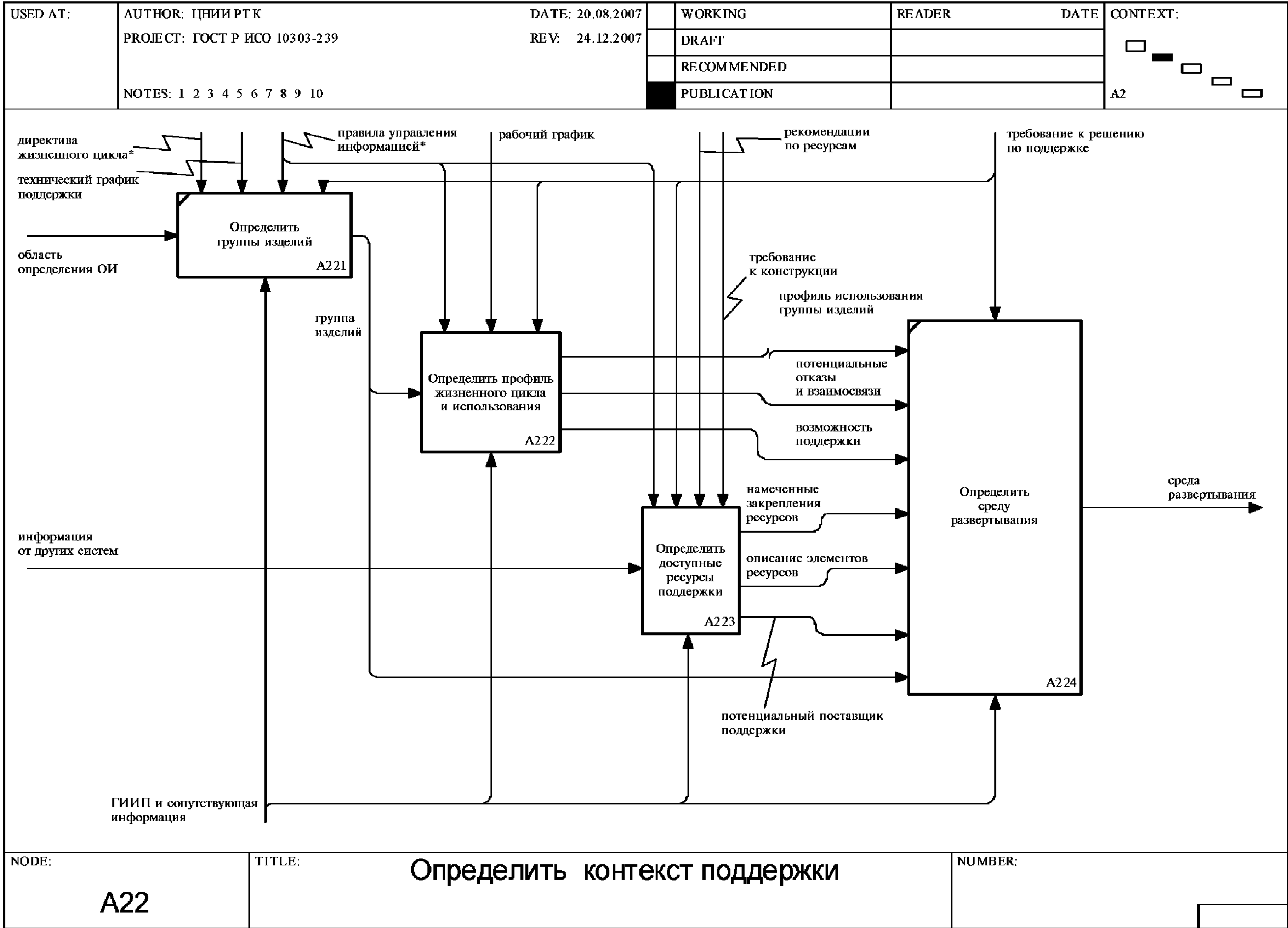
Рисунок F.21 — Диаграмма A22: Определить контекст поддержки
