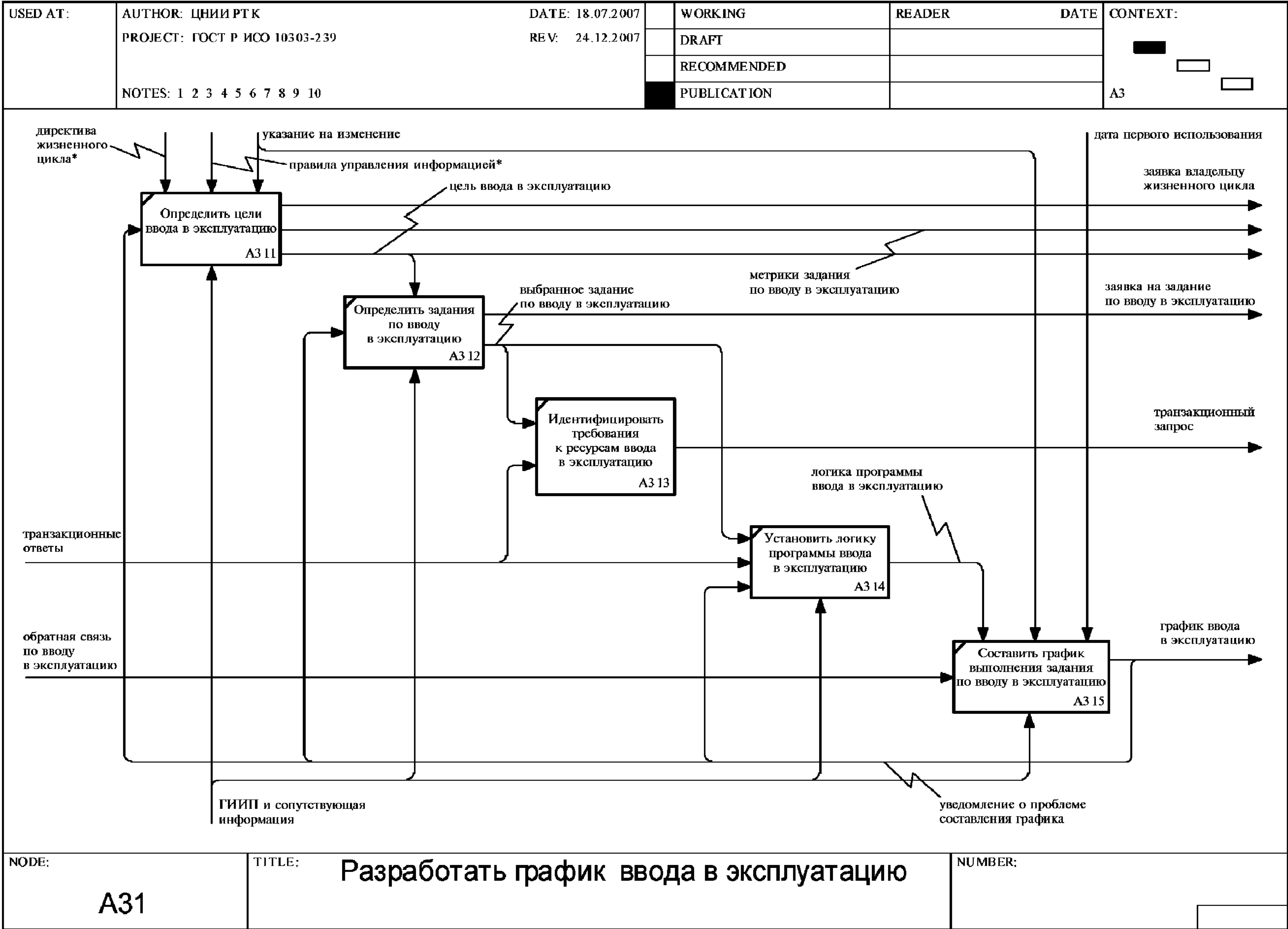
Рисунок F.36 — Диаграмма A31: Разработать график ввода в эксплуатацию
