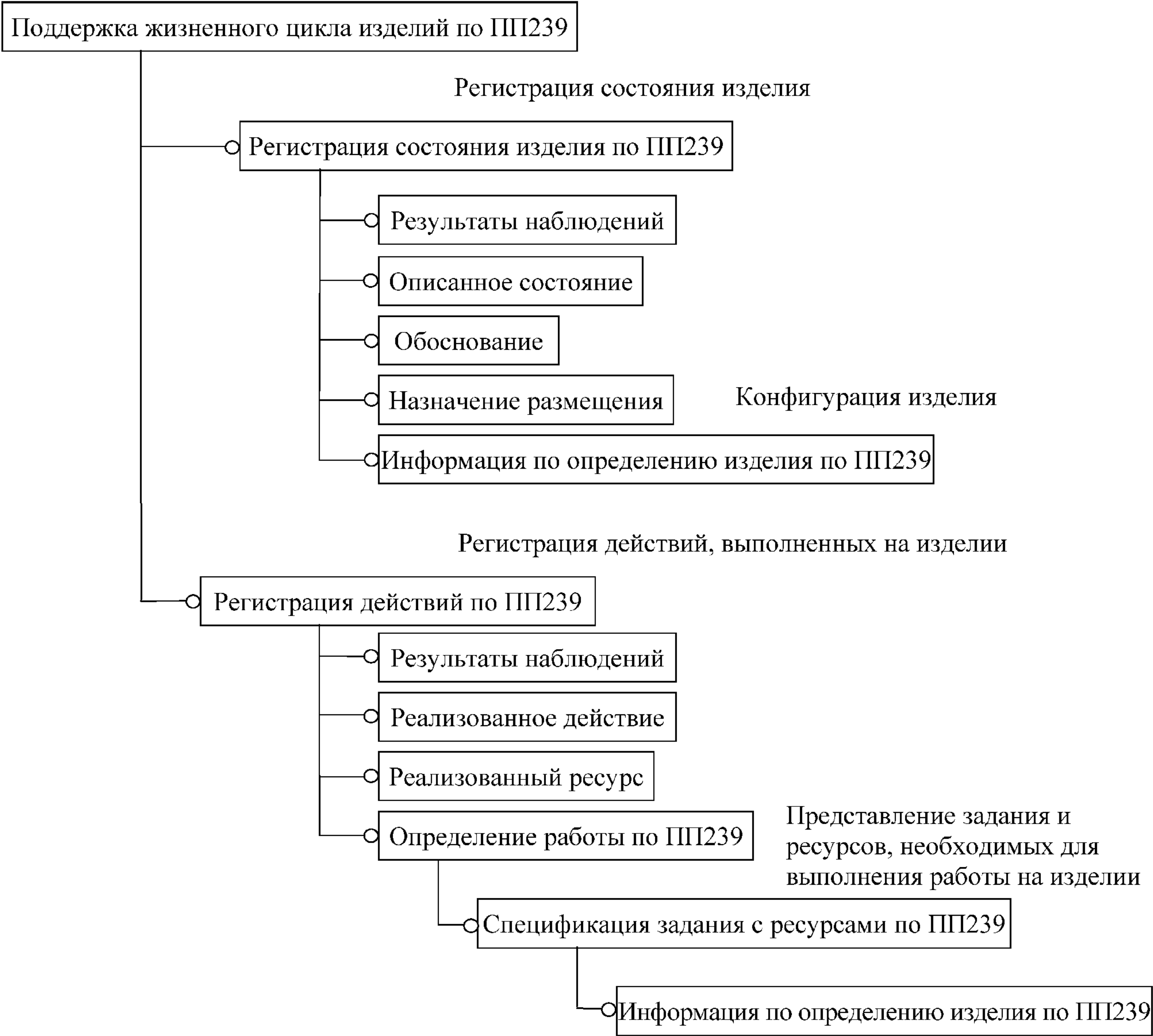
Рисунок 4 — Выделенная часть иерархии модулей
