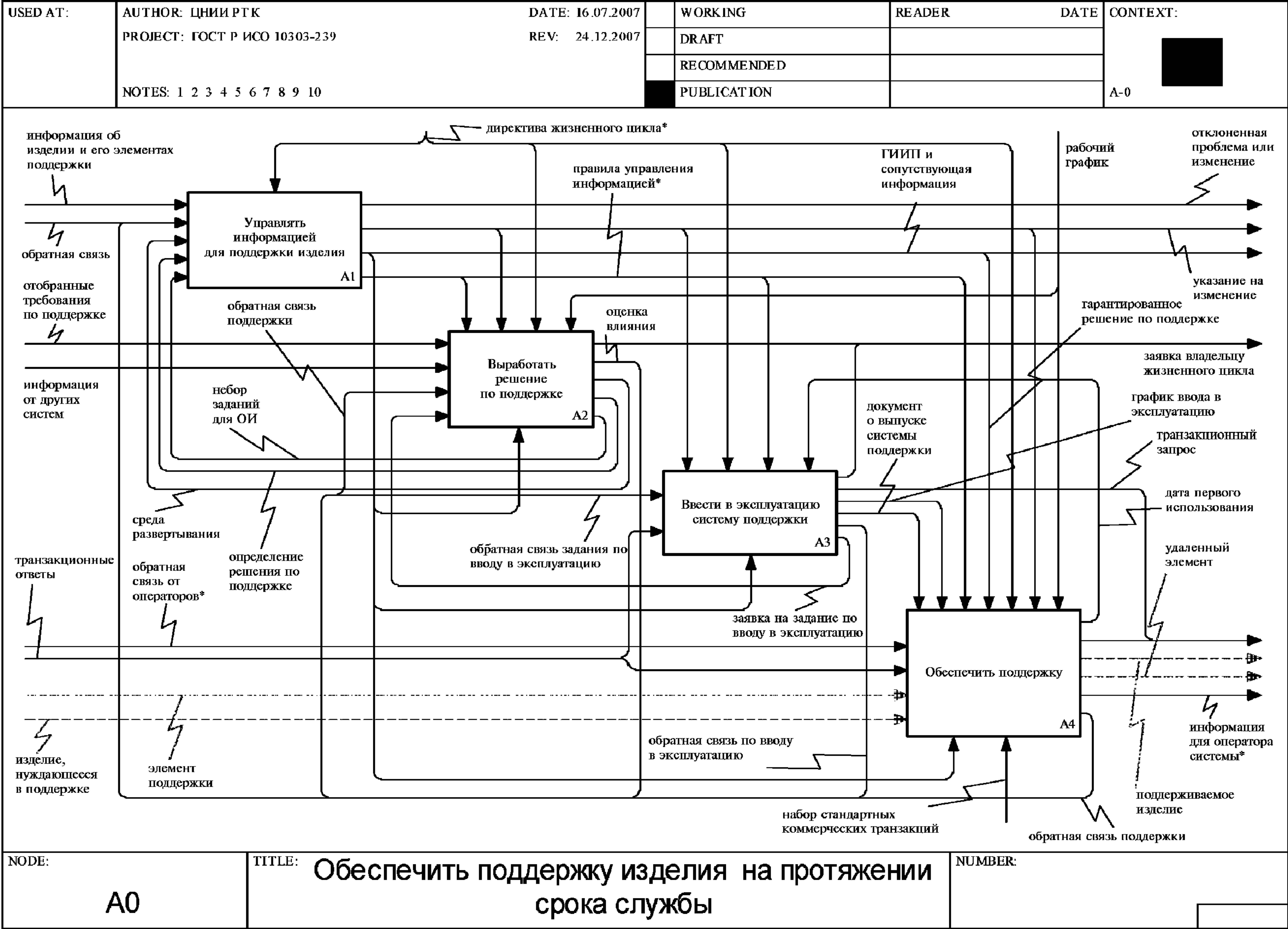
Рисунок F.2 — Диаграмма A0: Обеспечить поддержку изделия на протяжении срока службы
