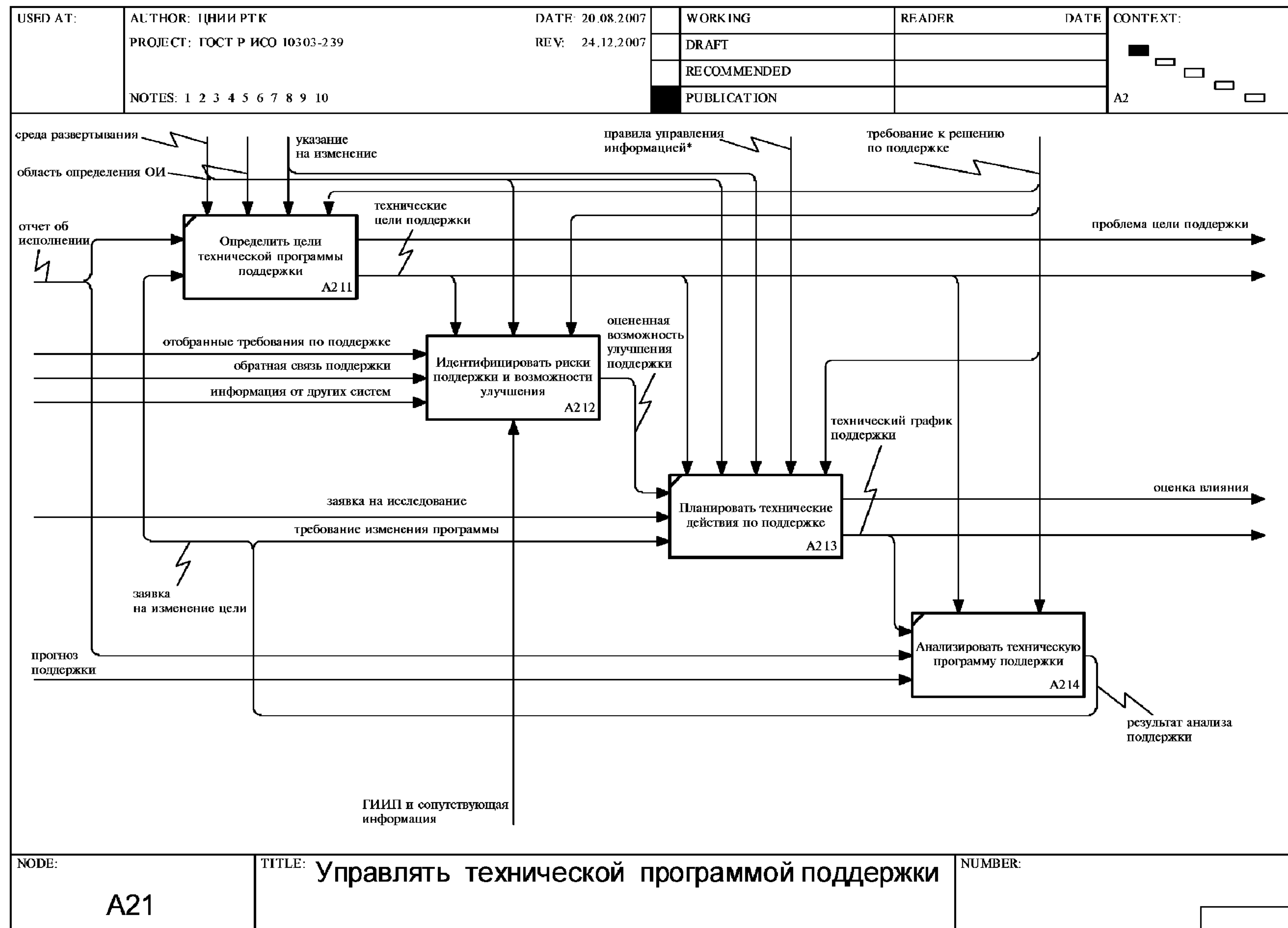
Рисунок F.19 — Диаграмма A21: Управлять технической программой поддержки
