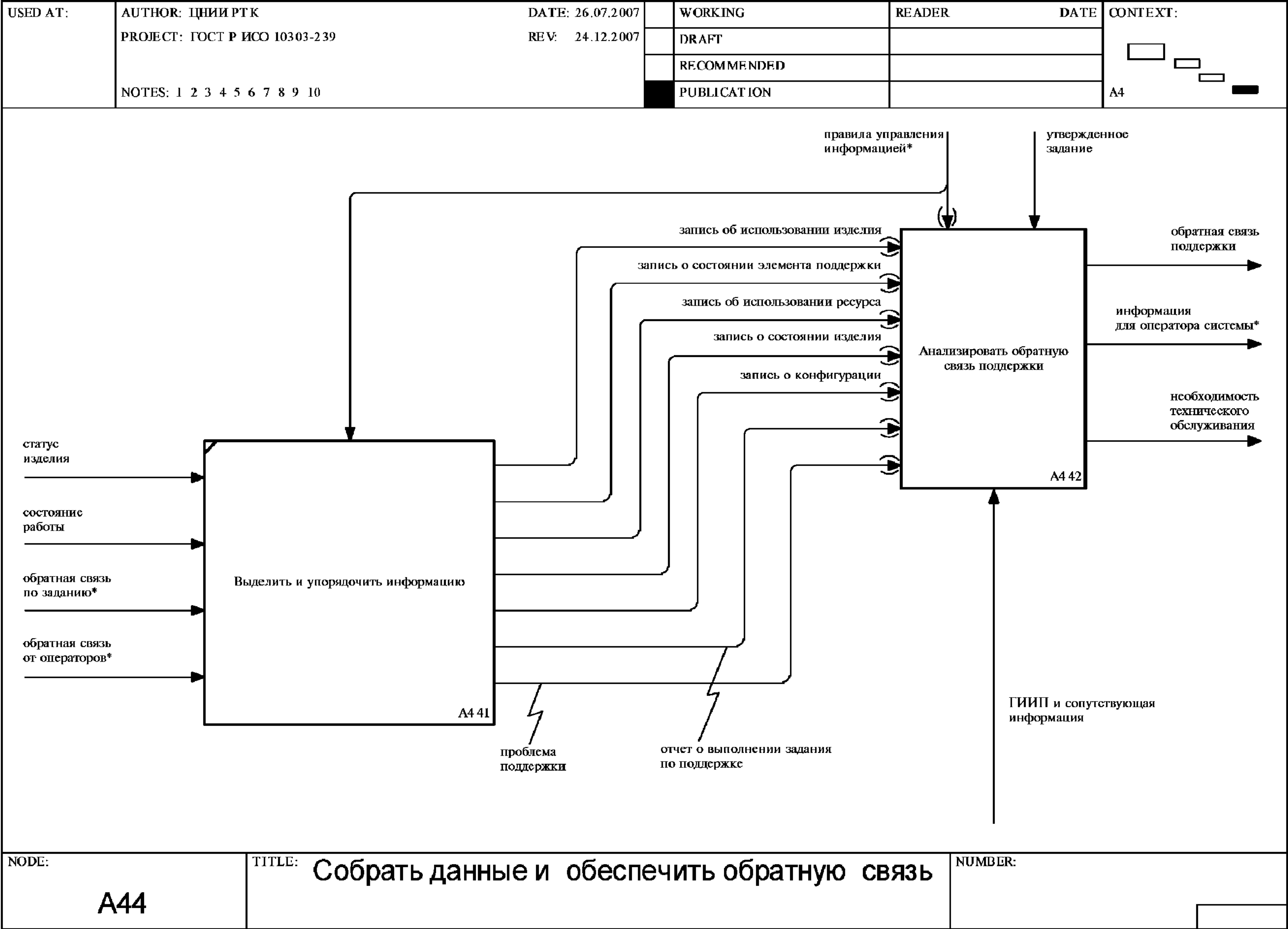
Рисунок F.43 — Диаграмма A44: Собрать данные и обеспечить обратную связь
