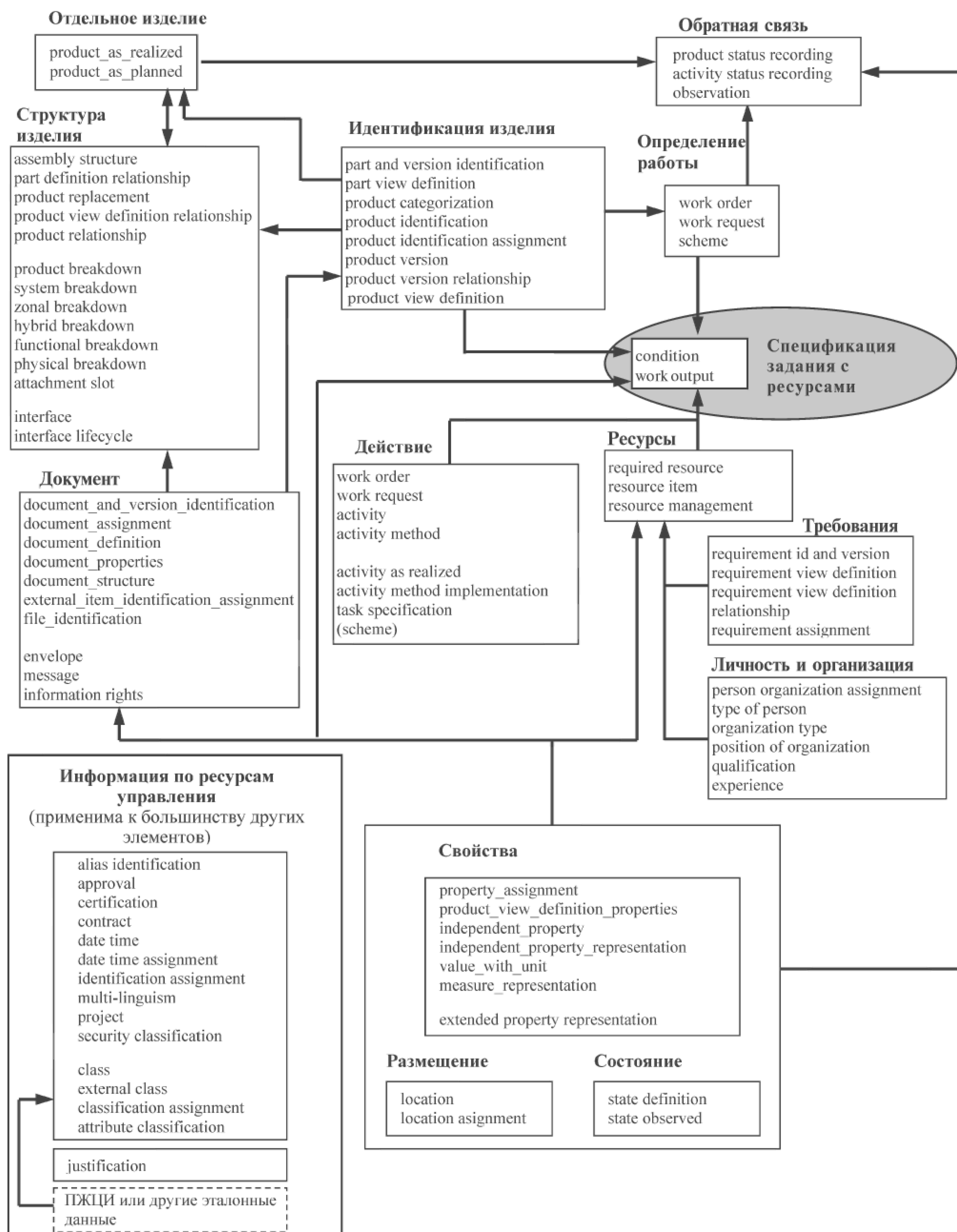
Рисунок 5 — Модель планирования данных
