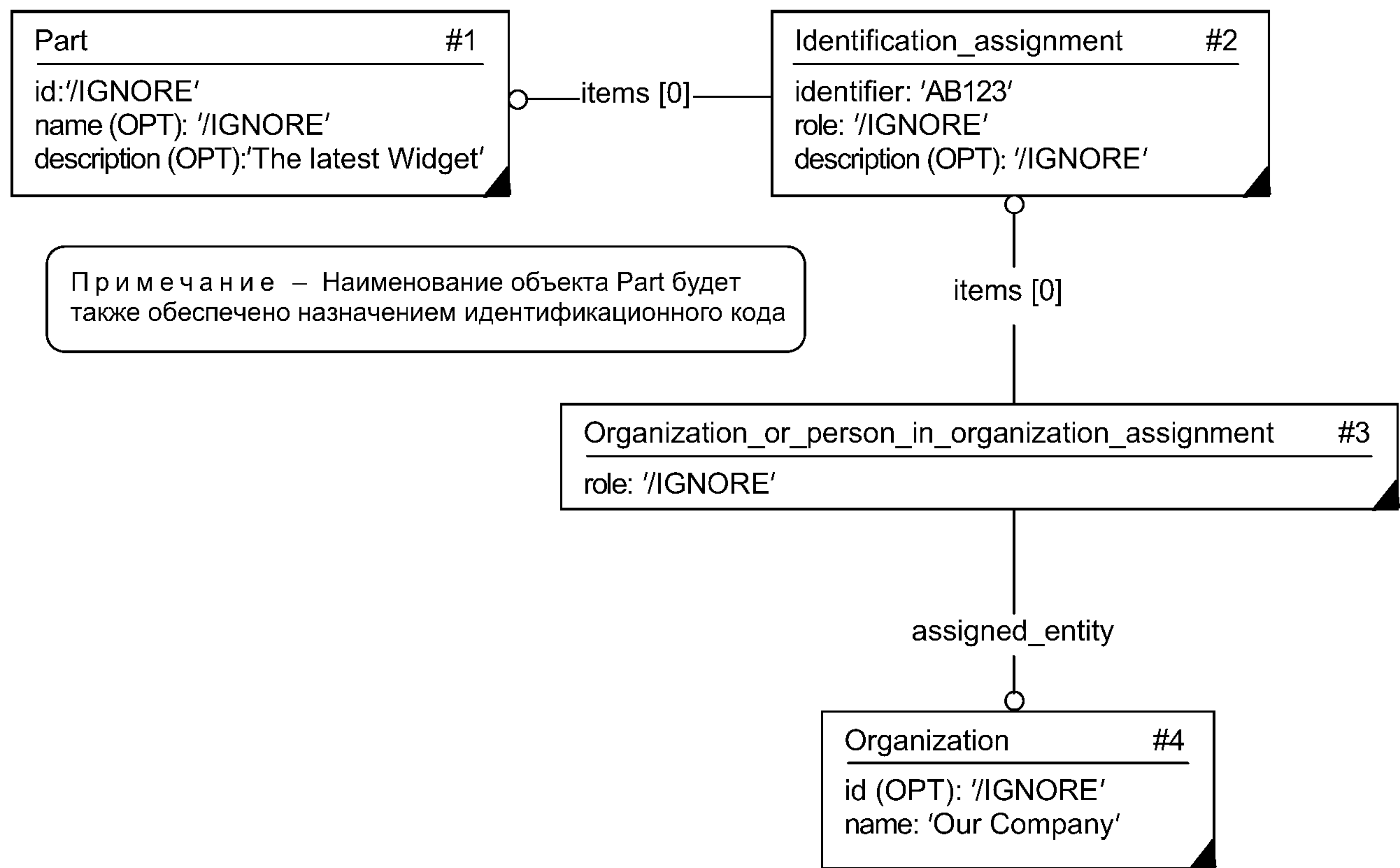
Рисунок I.1 — Пример назначения идентификационного кода
