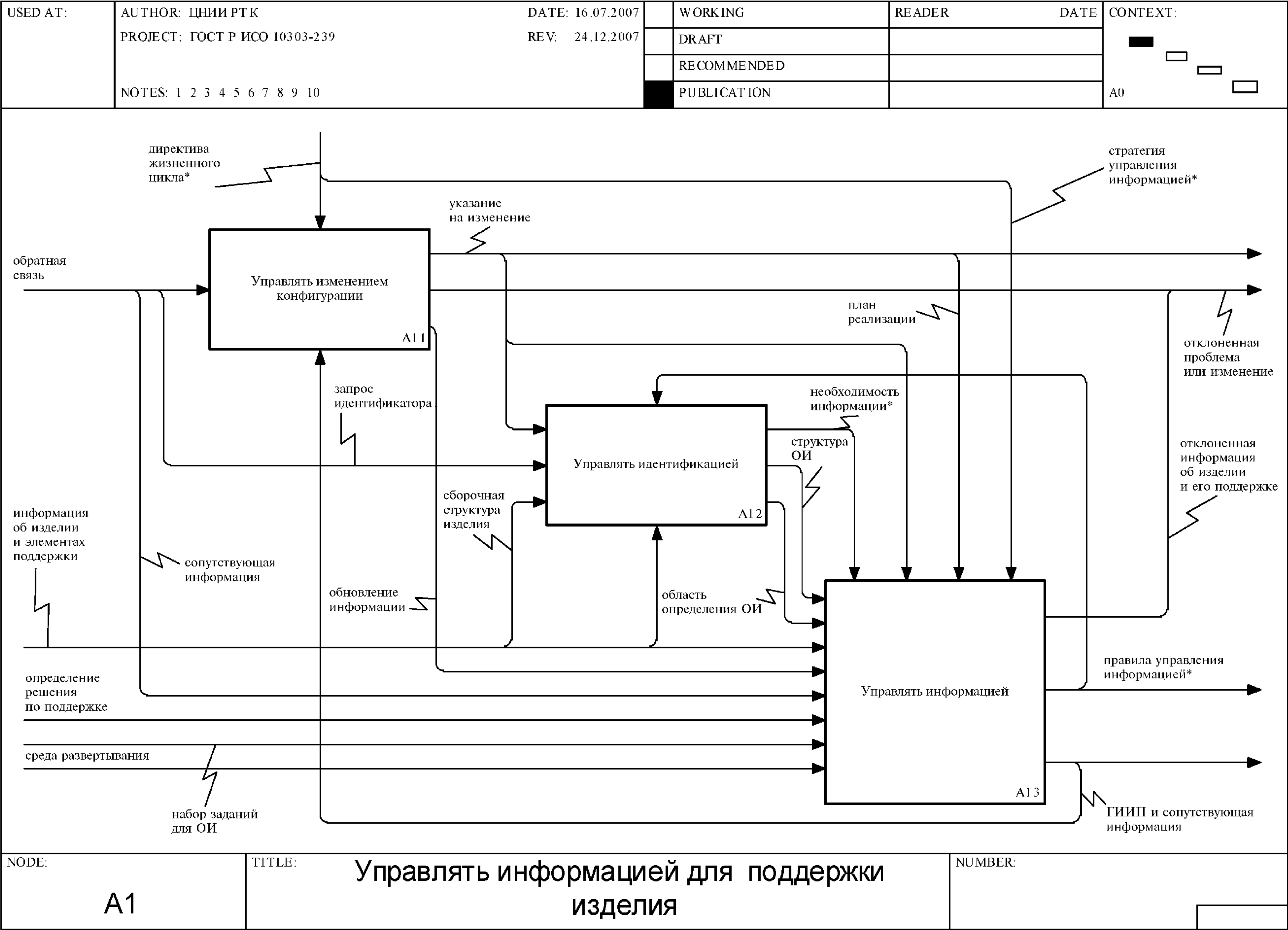
Рисунок F.3 — Диаграмма A1: Управлять информацией для поддержки изделия
