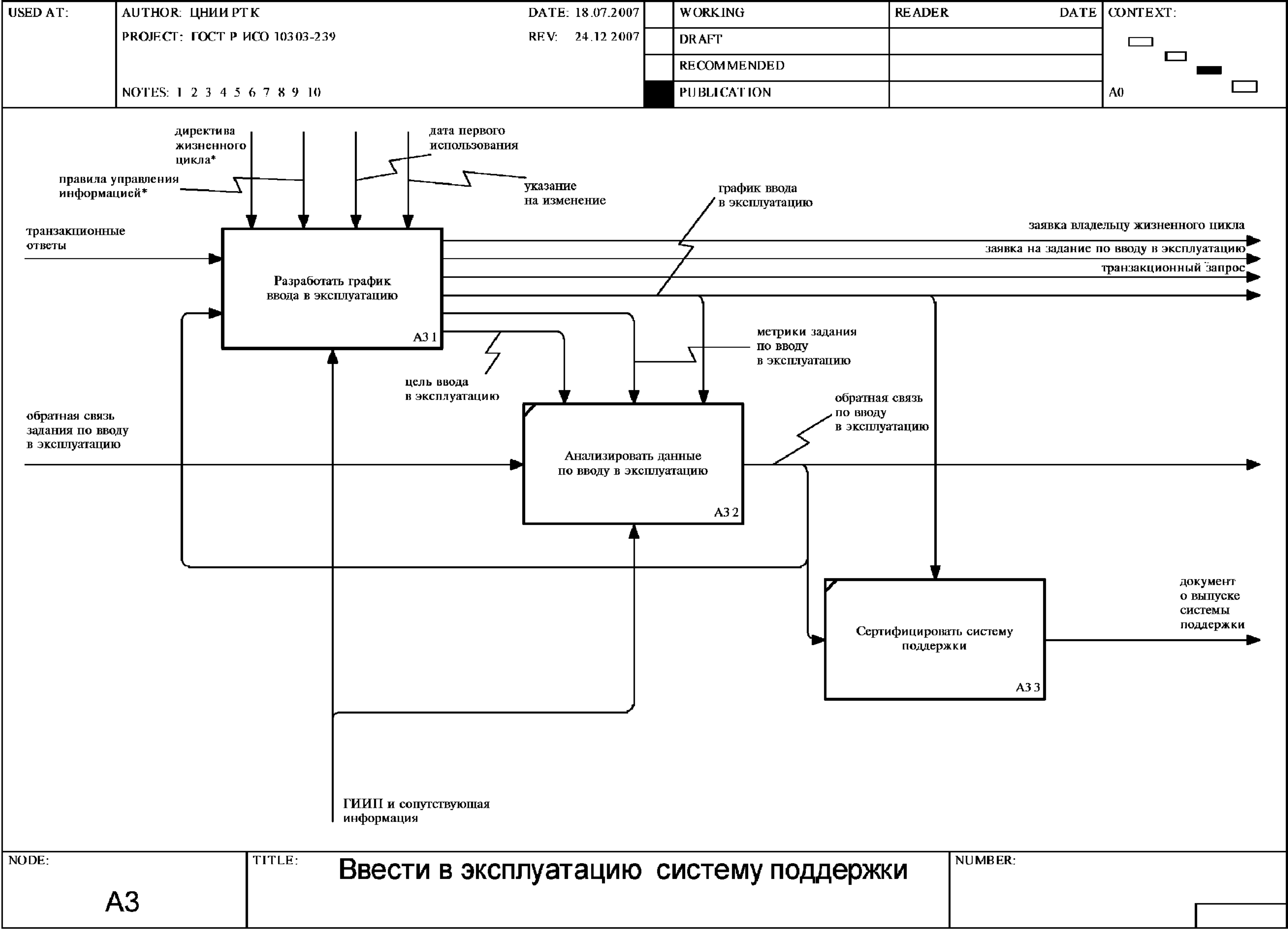
Рисунок F.35 — Диаграмма A3: Ввести в эксплуатацию систему поддержки
