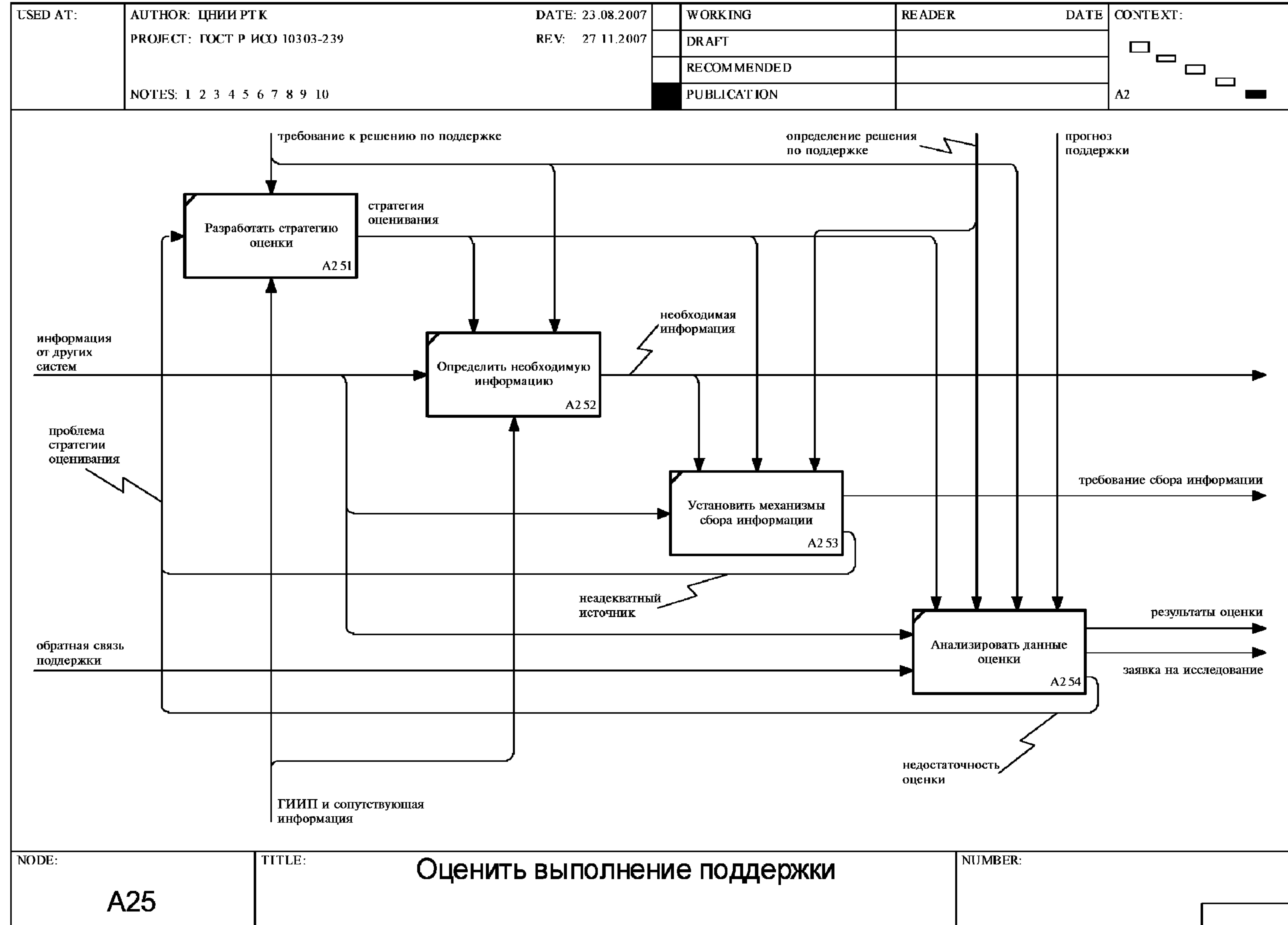
Рисунок F.34 — Диаграмма A25: Оценить выполнение поддержки
