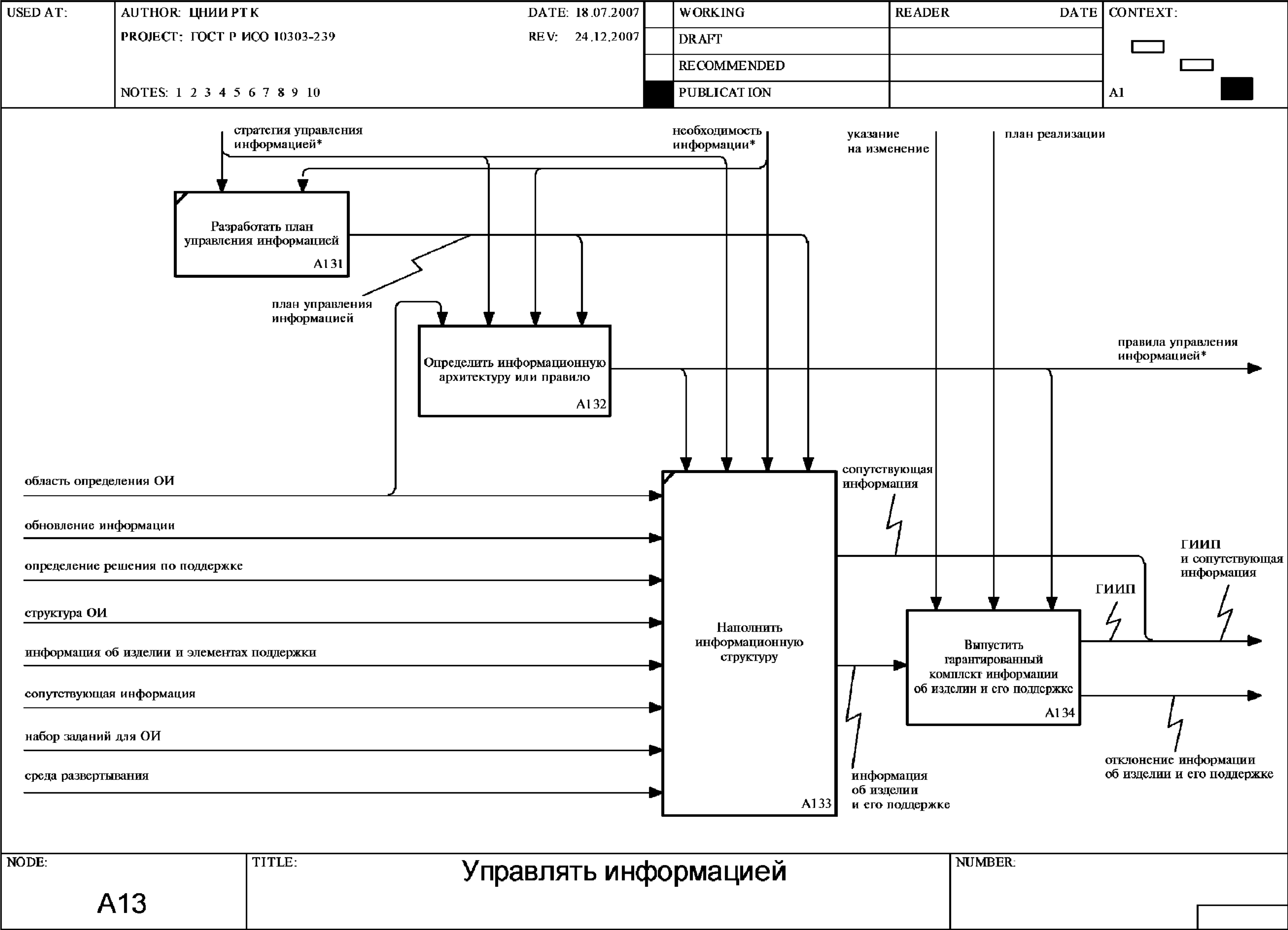
Рисунок F.15 — Диаграмма A13: Управлять информацией
