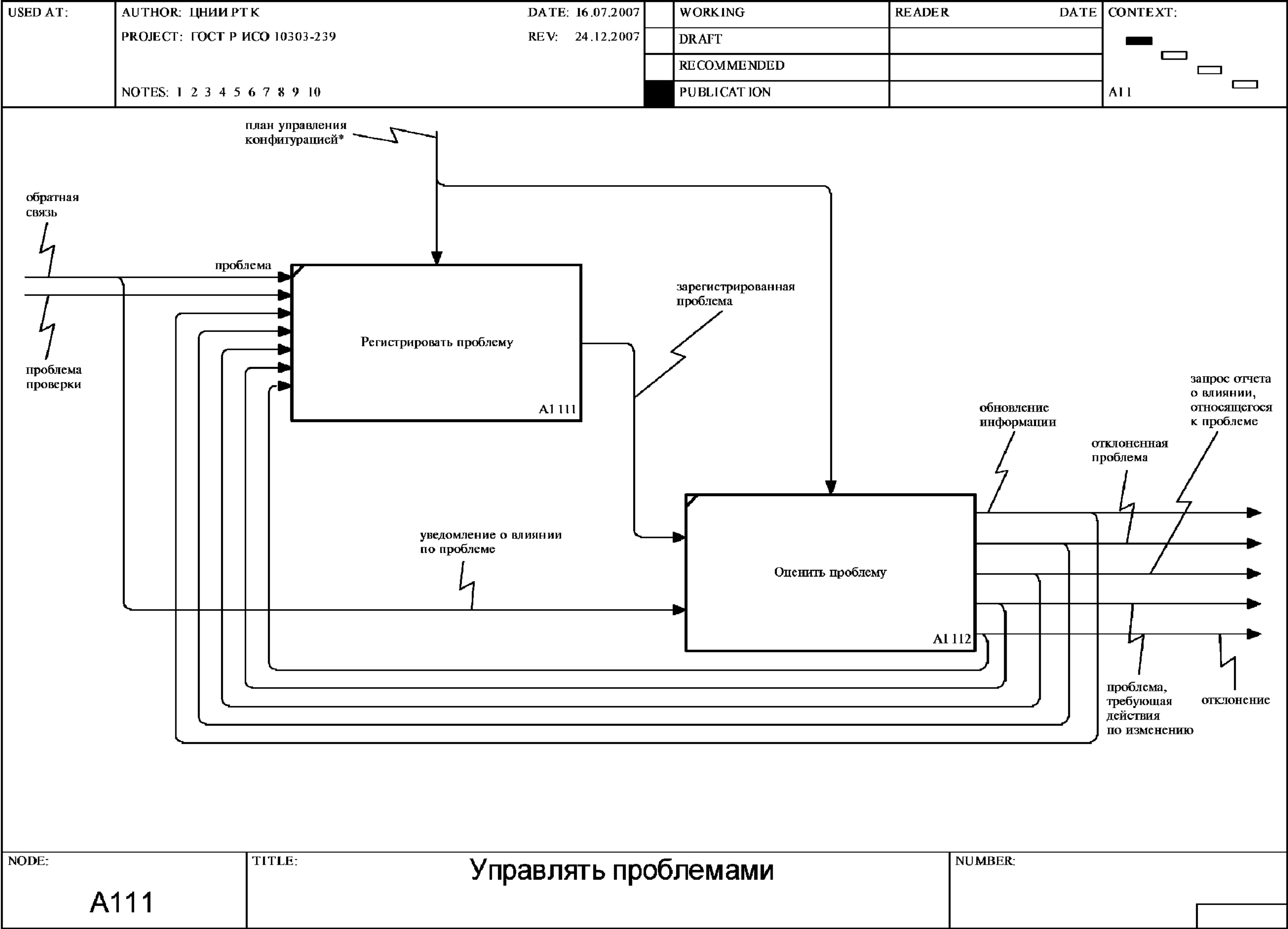
Рисунок F.5 — Диаграмма A111: Управлять проблемами
