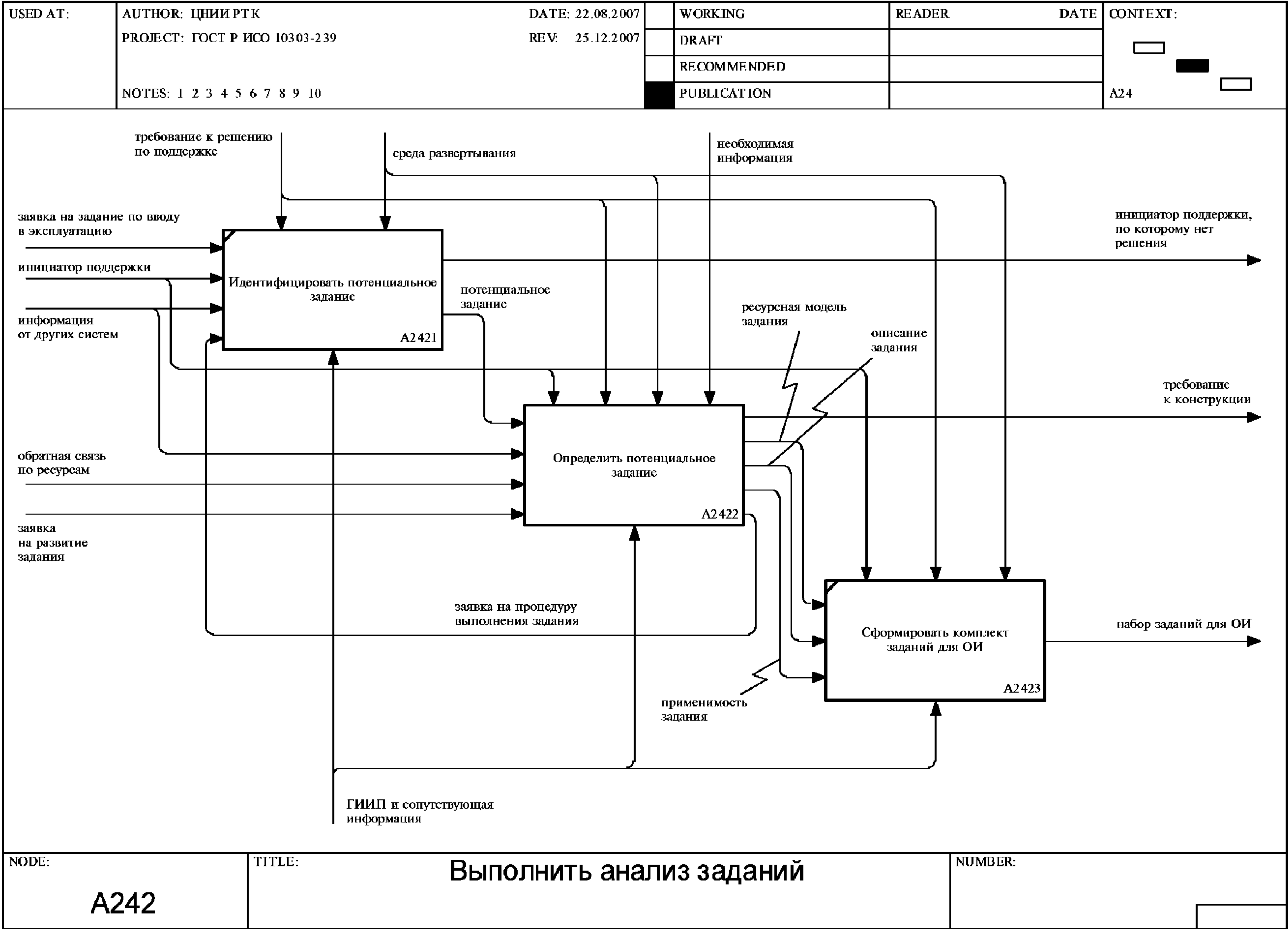
Рисунок F.28 — Диаграмма A242: Выполнить анализ заданий
