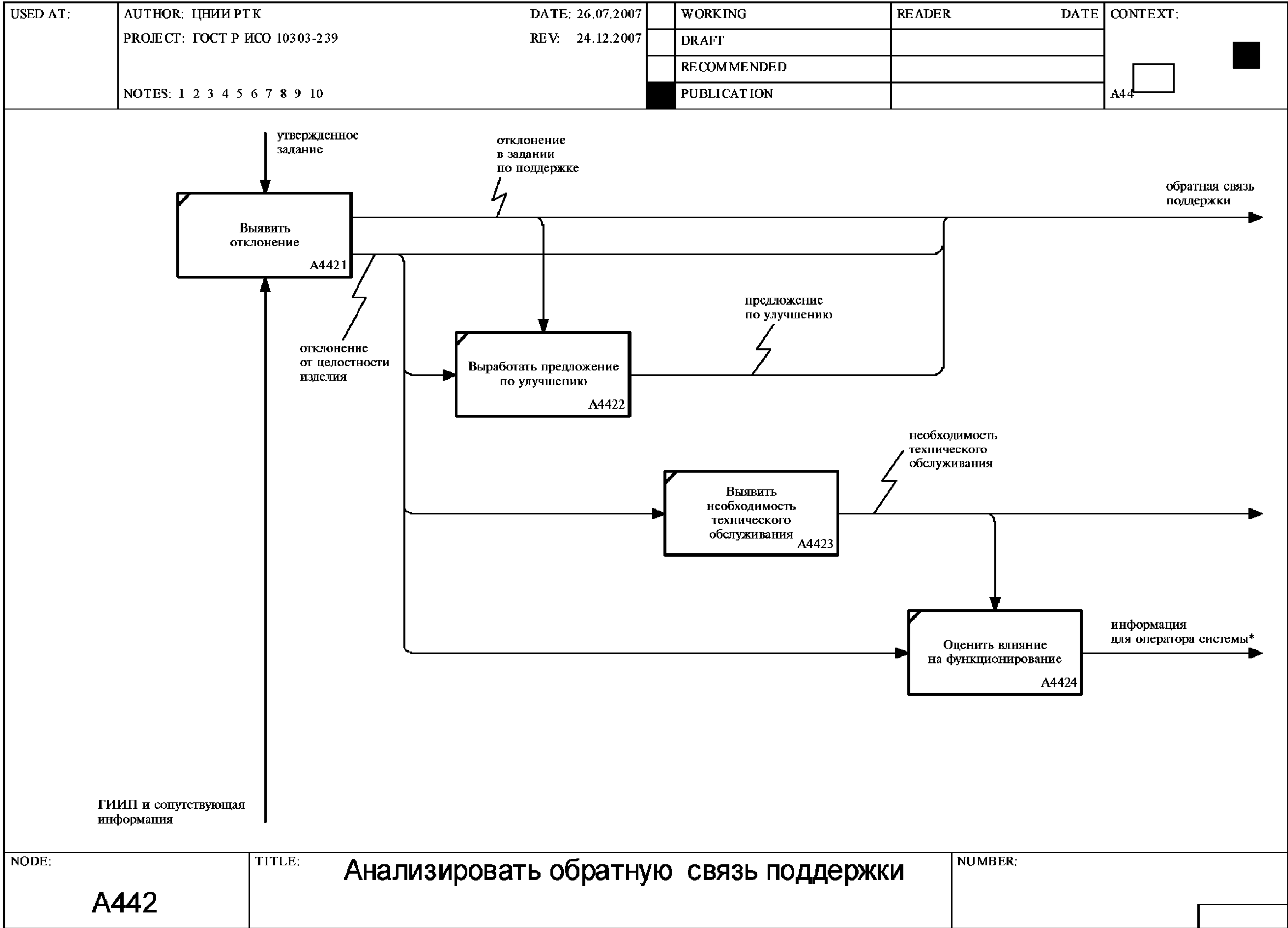
Рисунок F.44 — Диаграмма A442: Анализировать обратную связь поддержки
