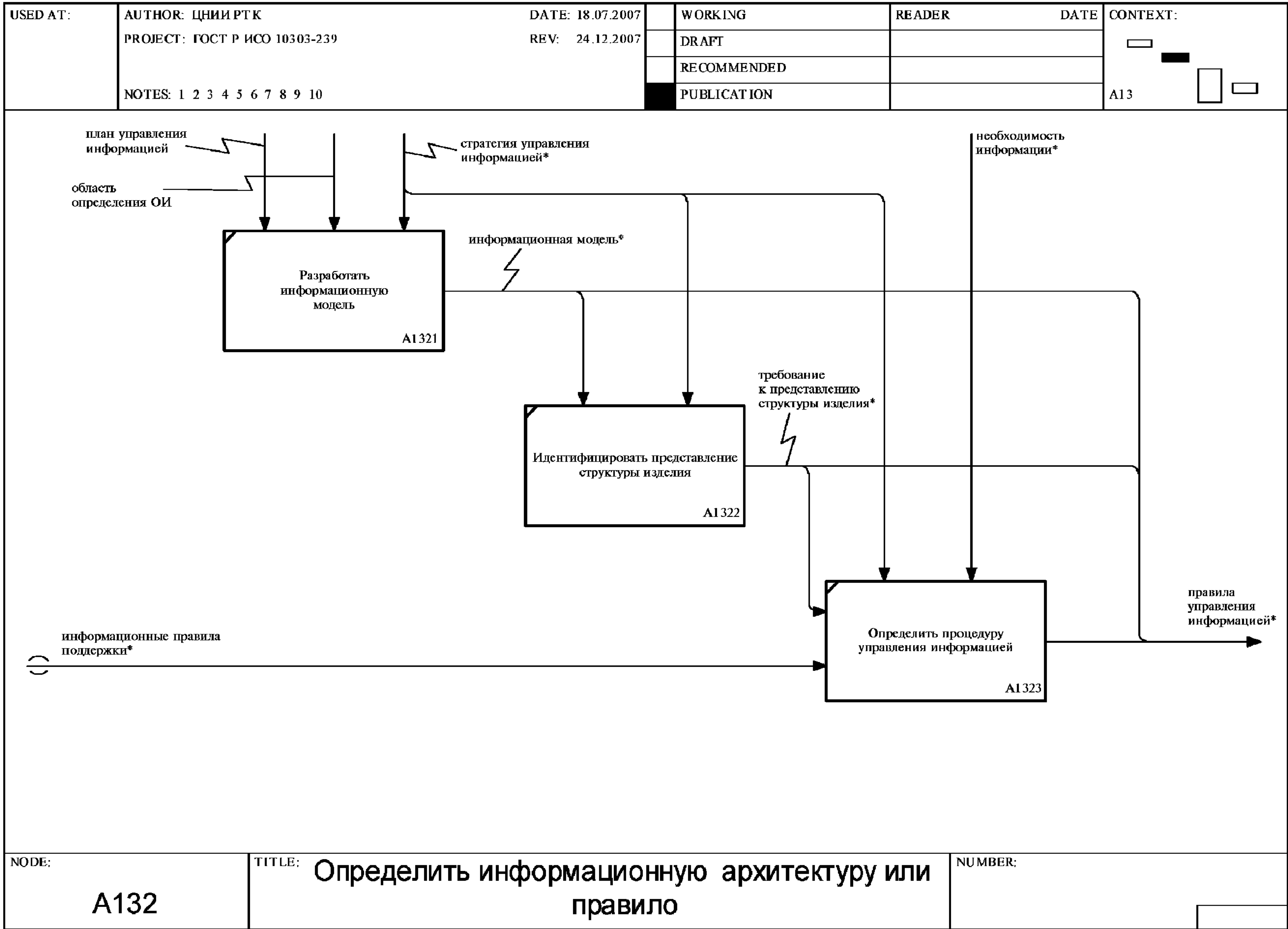
Рисунок F.16 — Диаграмма A132: Определить информационную архитектуру или правило
