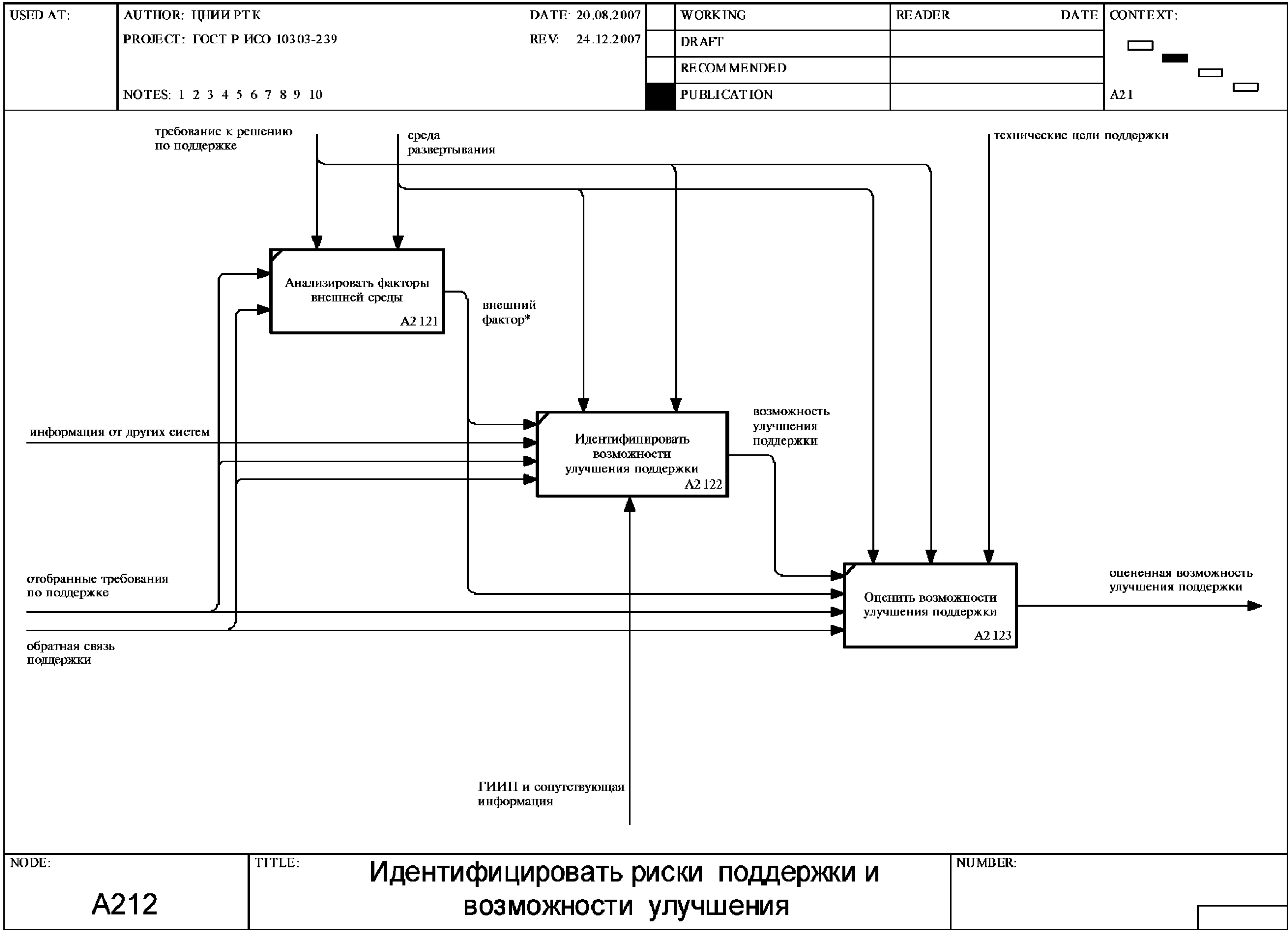
Рисунок F.20 — Диаграмма A212: Идентифицировать риски поддержки и возможности улучшения
