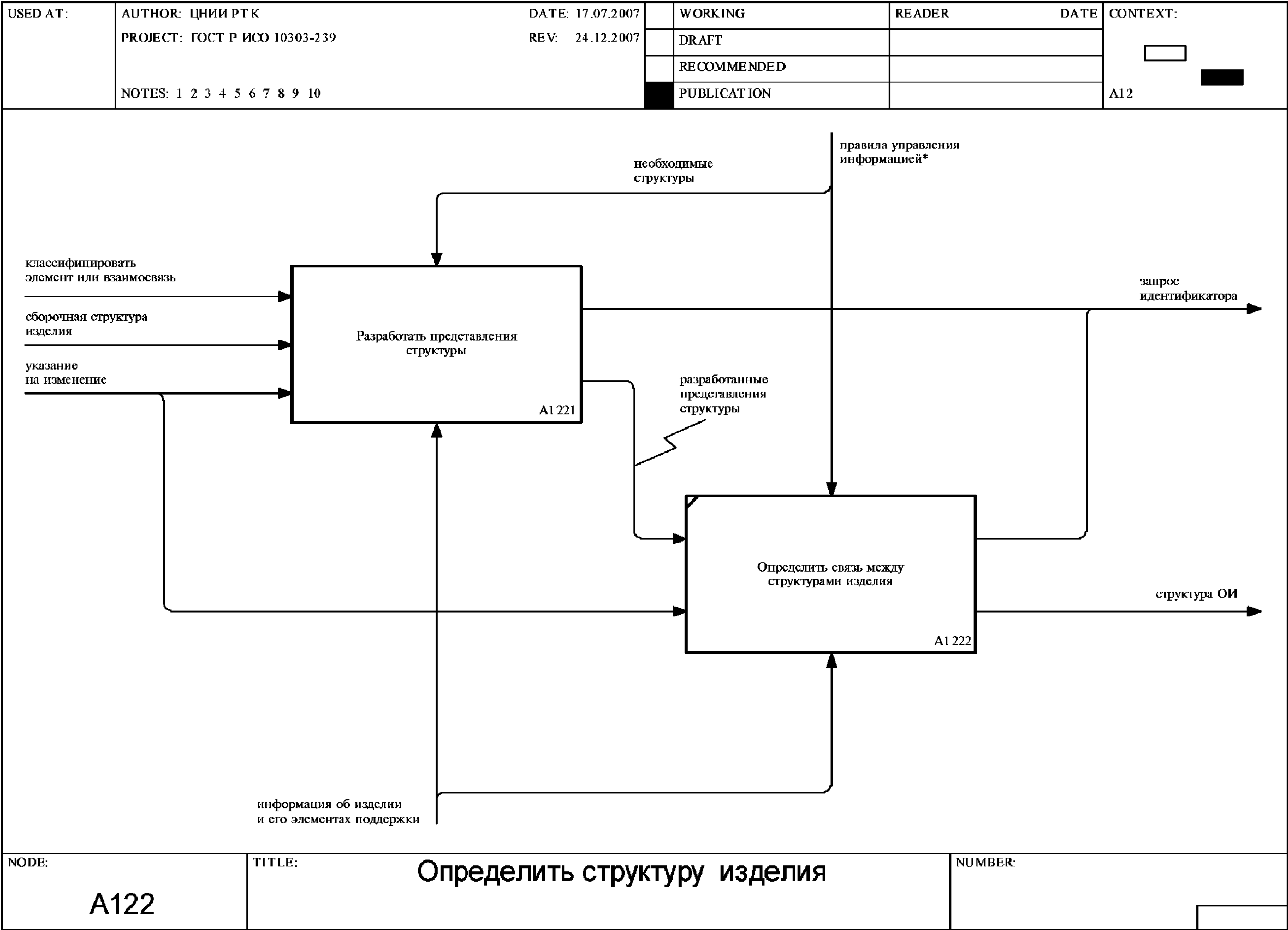
Рисунок F.13 — Диаграмма A122: Определить структуру изделия
