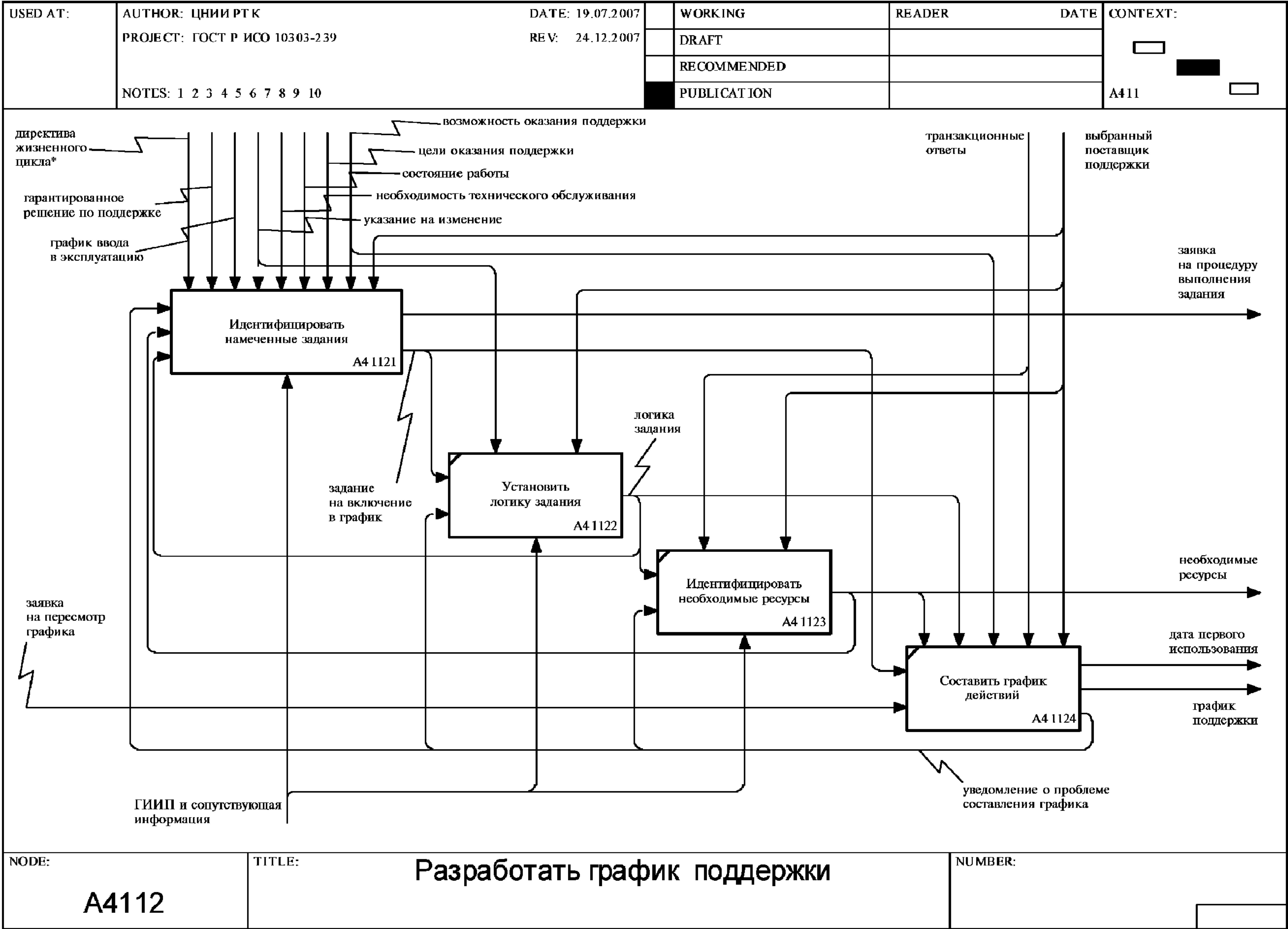
Рисунок F.40 — Диаграмма A4112: Разработать график поддержки
