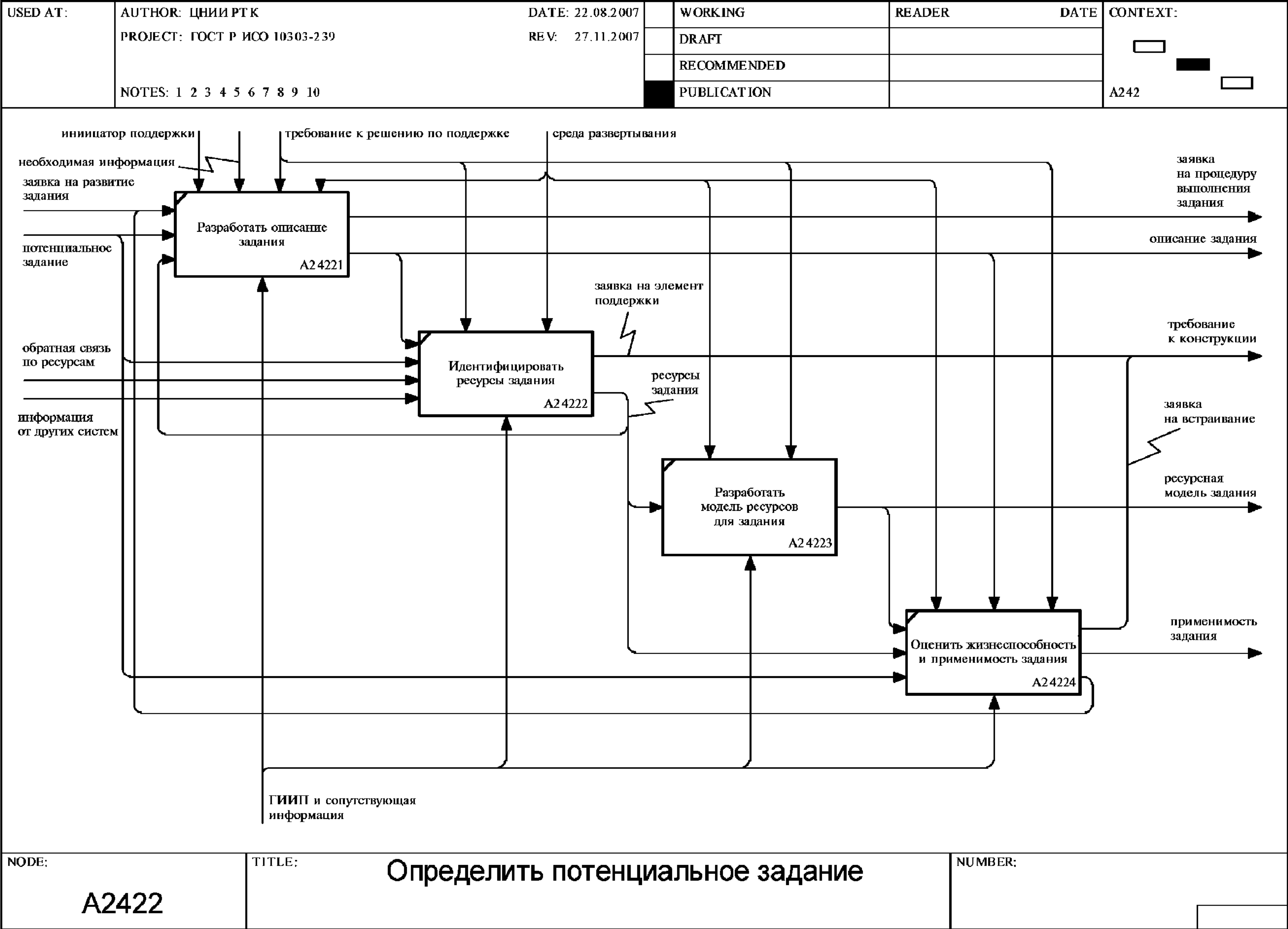
Рисунок F.29 — Диаграмма A2422: Определить потенциальное задание
