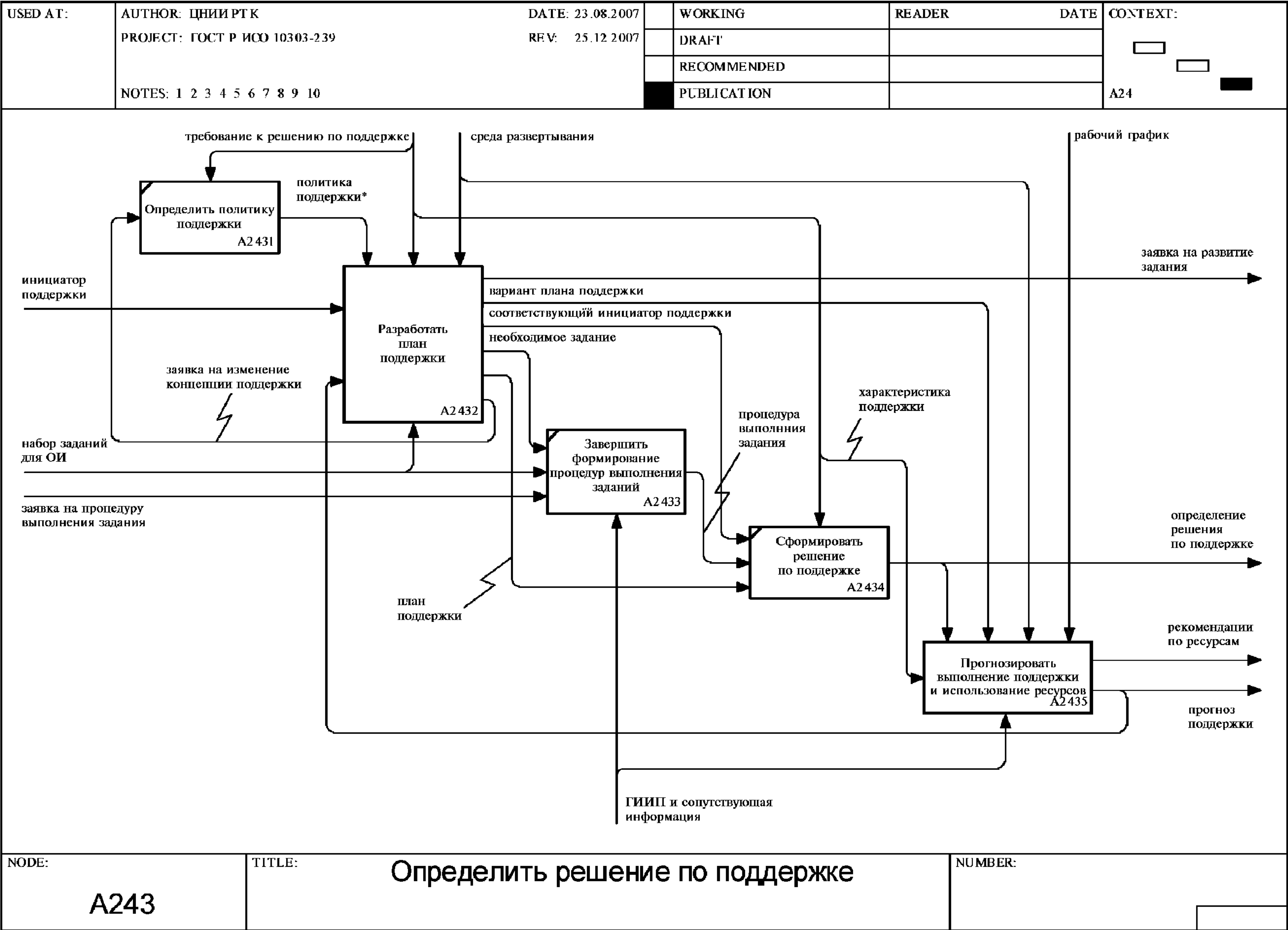
Рисунок F.30 — Диаграмма A243: Определить решение по поддержке
