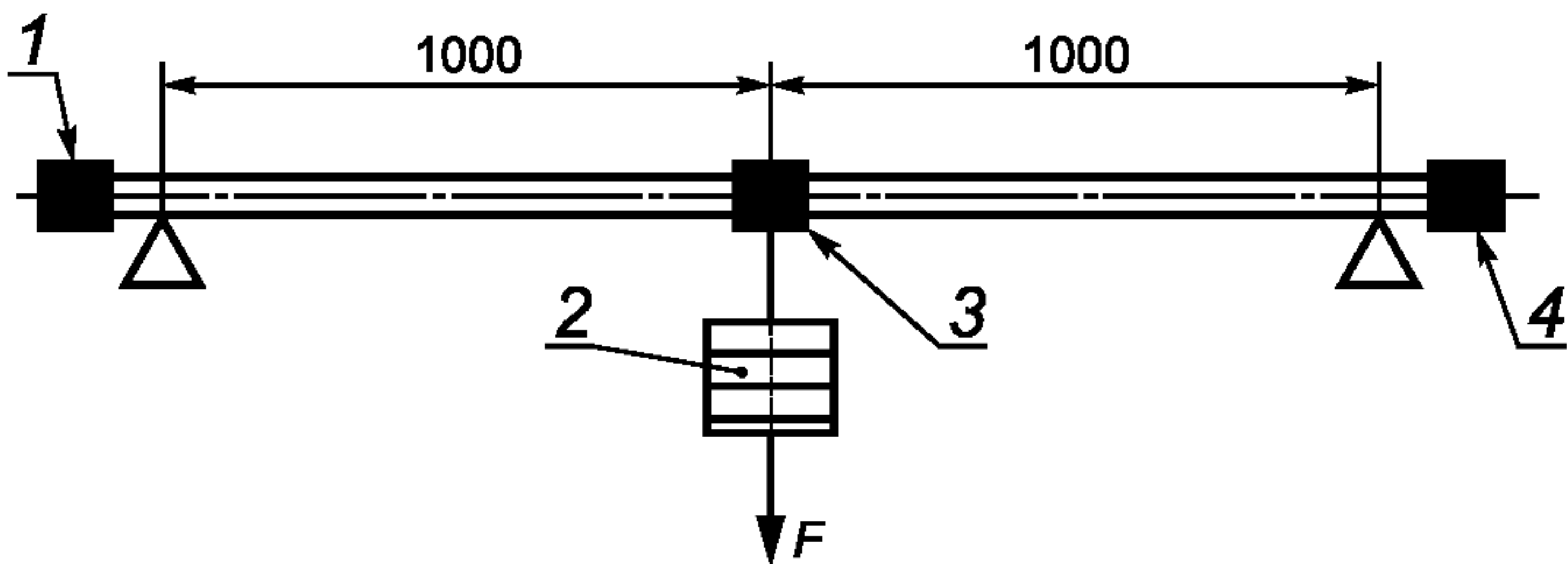
1 — пробка; 2 — вес; 3 — фитинг; 4 — подача
