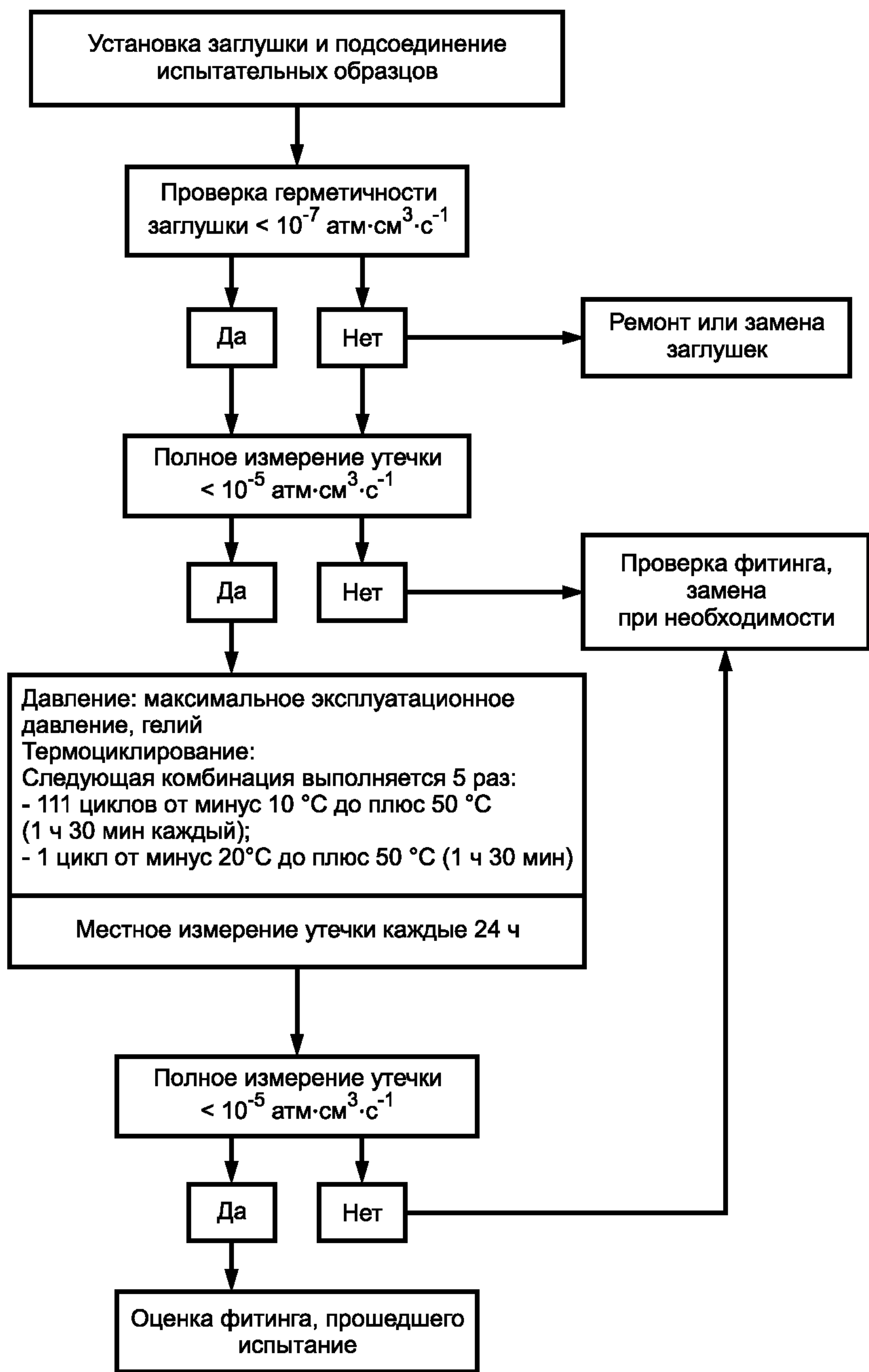
Рисунок И.1 — Испытание фитинга на герметичность
