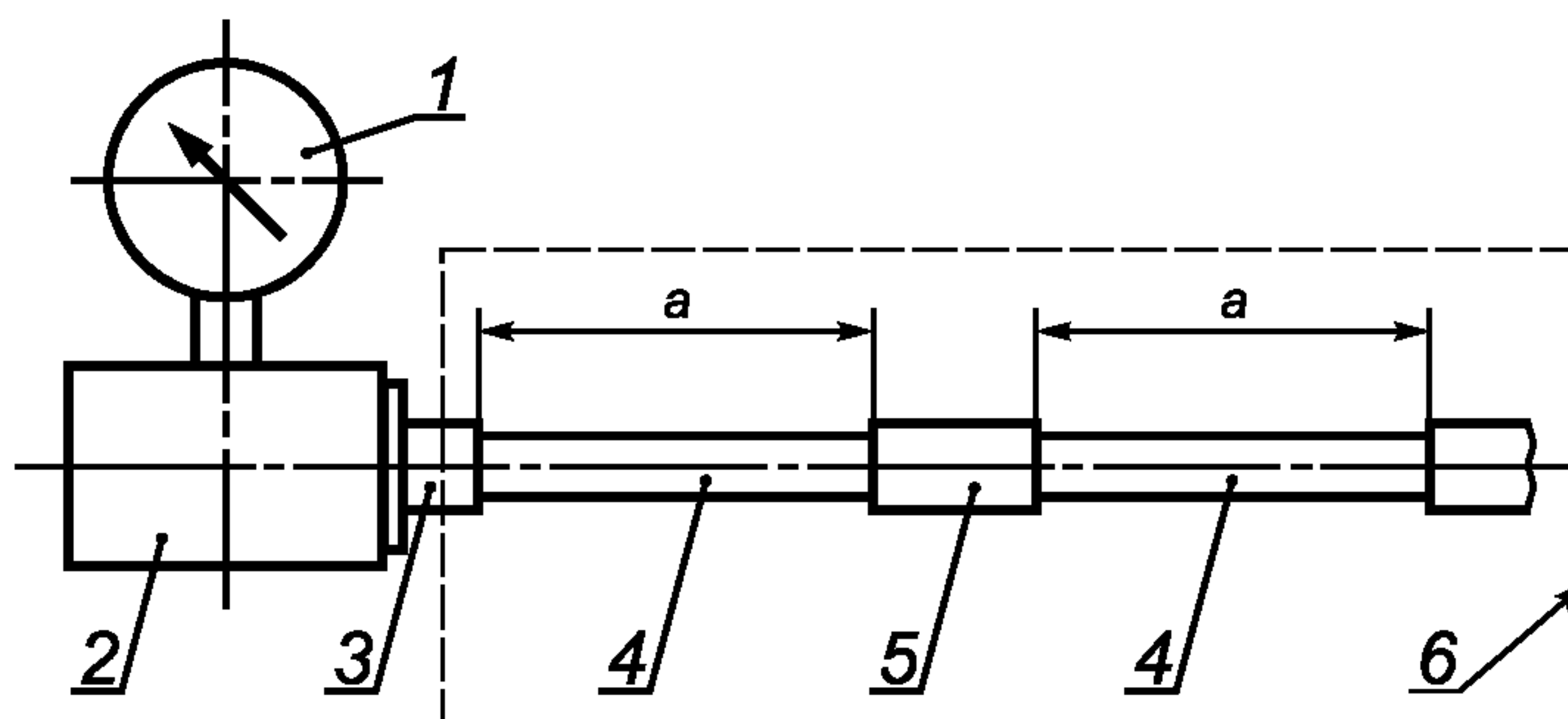
1 — манометр для измерения давления; 2 — нагнетательный насос; 3 — соединение насоса; 4 — труба; 5 — испытуемый фитинг; 6 — емкость с водой; a — размеры (таблица 9)
