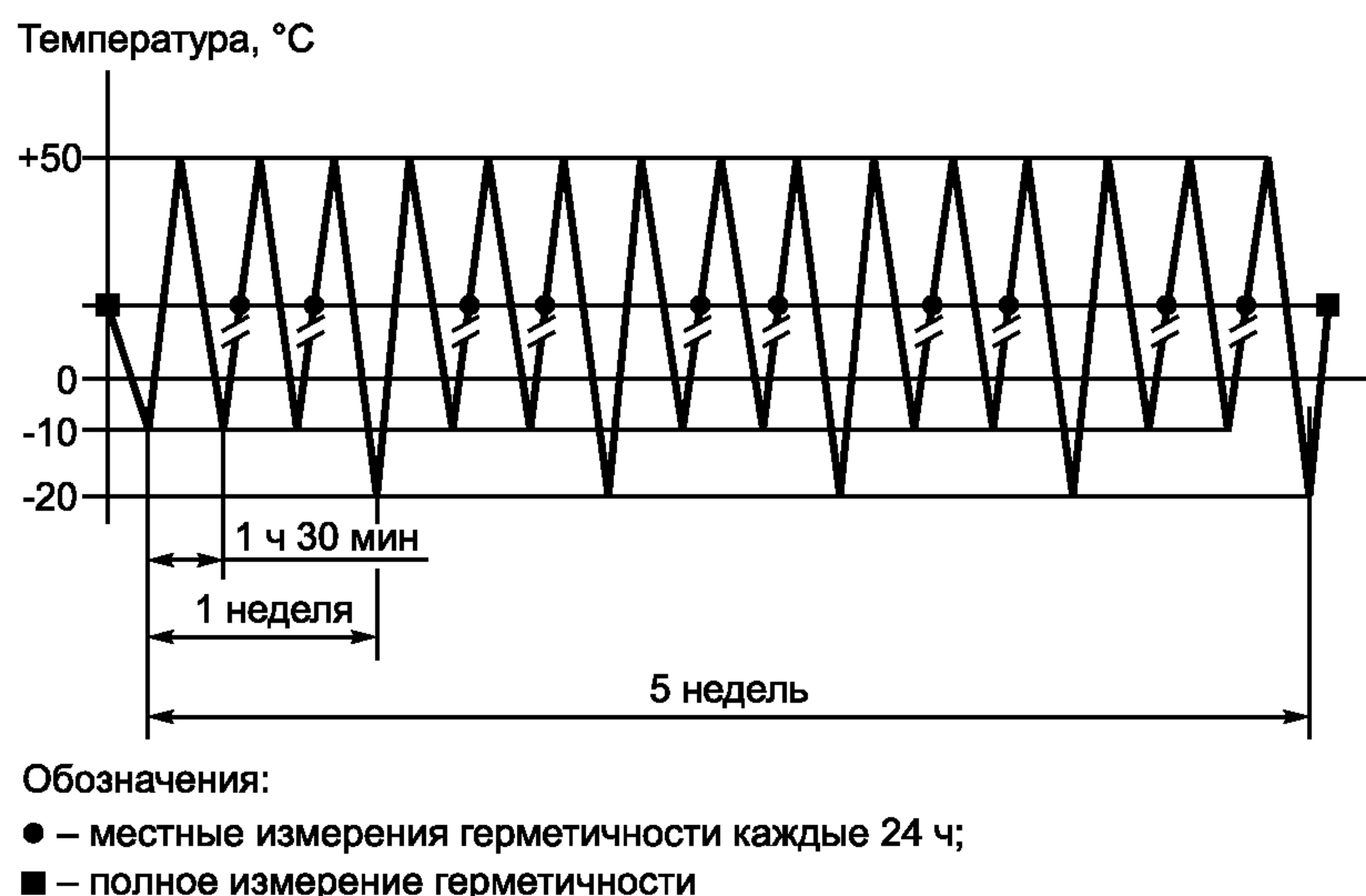
Рисунок И.2 — Термоциклирование
