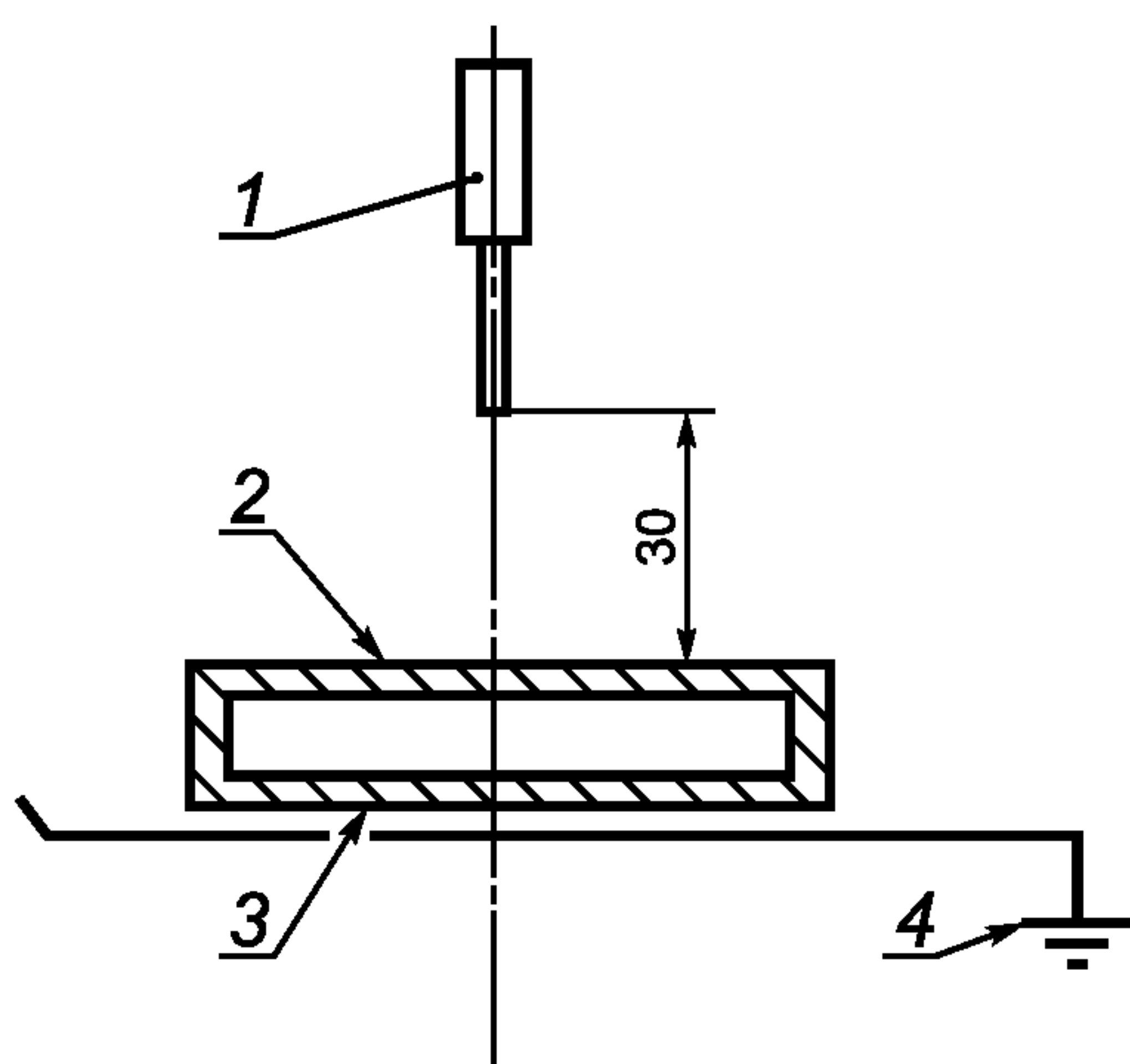
Рисунок 8 — Электризация корпуса в электрическом поле источника высокого напряжения постоянного тока
