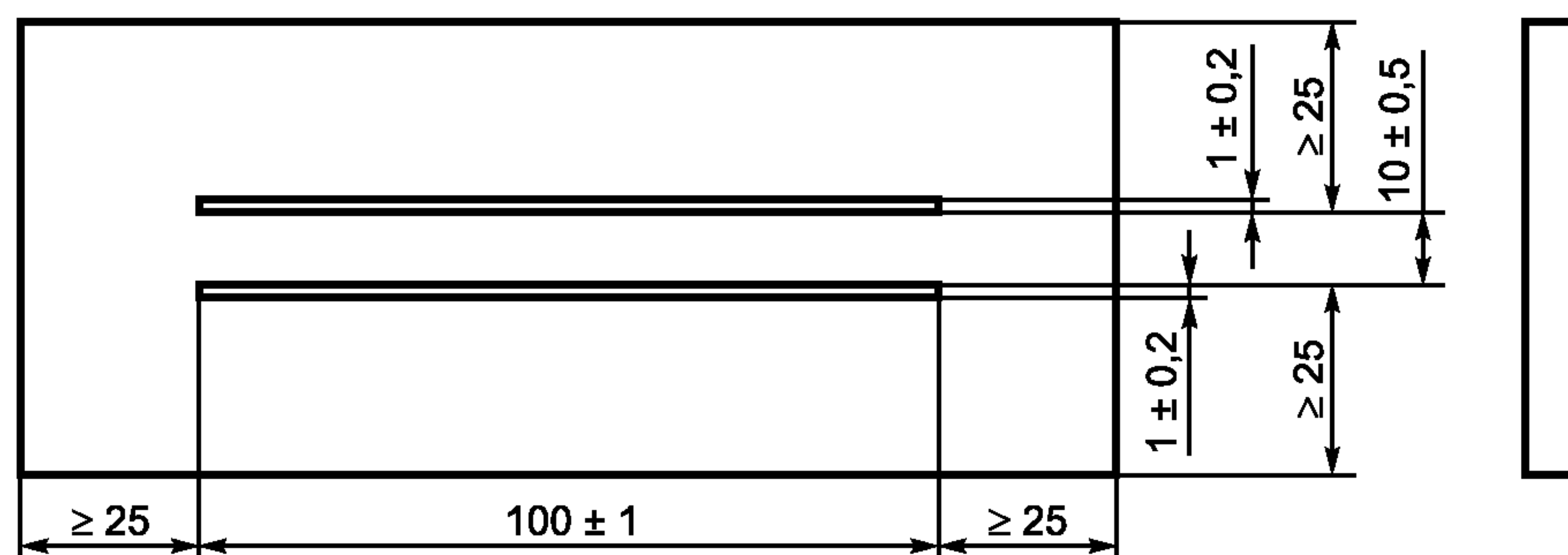
Рисунок 5 — Испытуемый образец с электродами из проводящей краски
