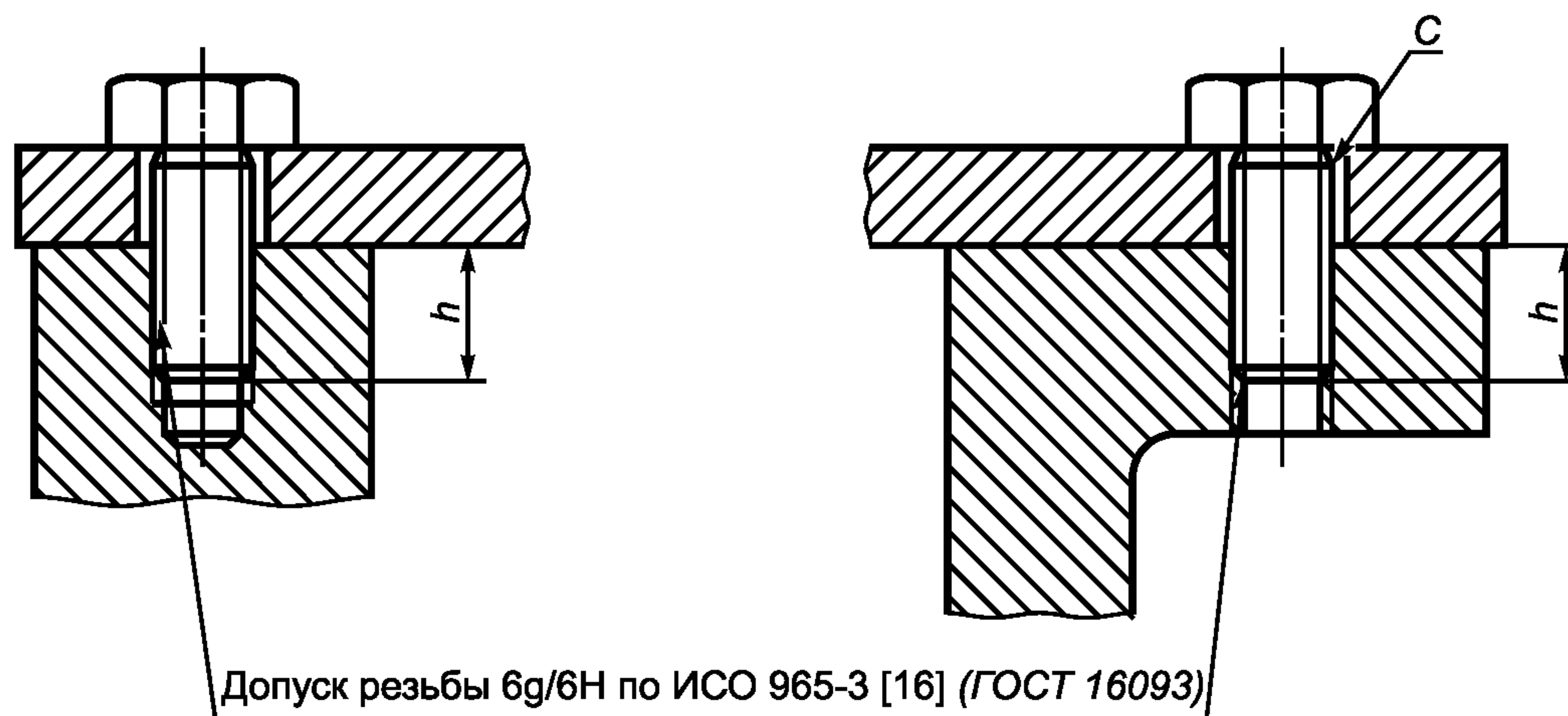
Рисунок 1 — Допуски и зазор для резьбовых крепежных деталей
