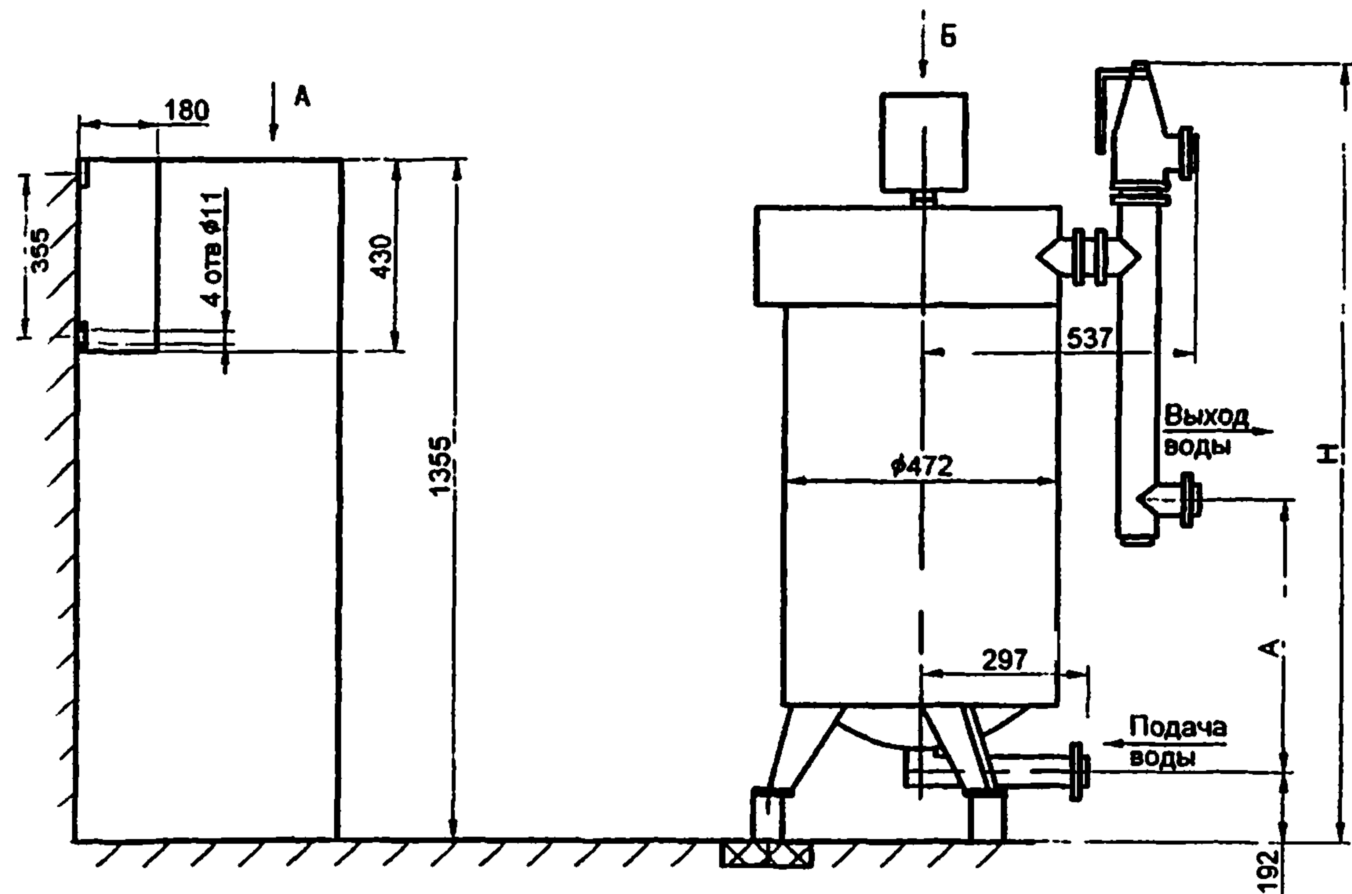
Габаритные, установочные, присоединительные размеры и масса электронагревателей ЭПЗ-ИЗМ и шкафов управления
