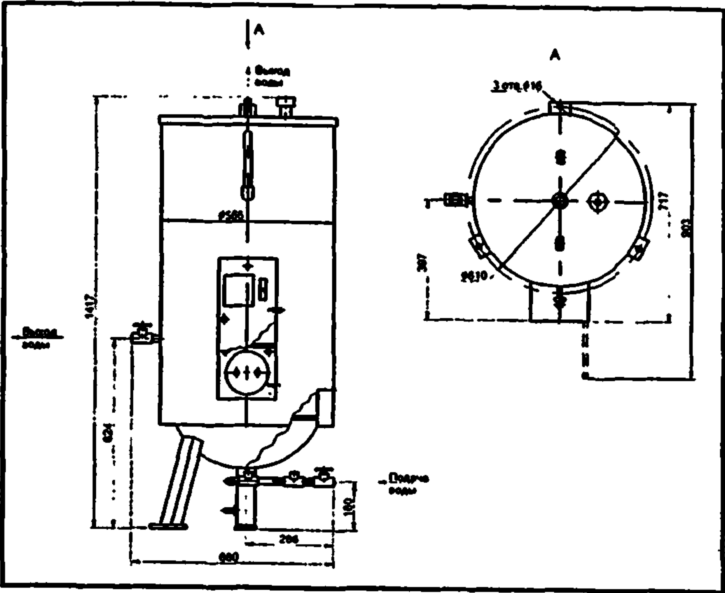
Габаритные и установочные размеры электроводонагревателя САОС-200/90И1
