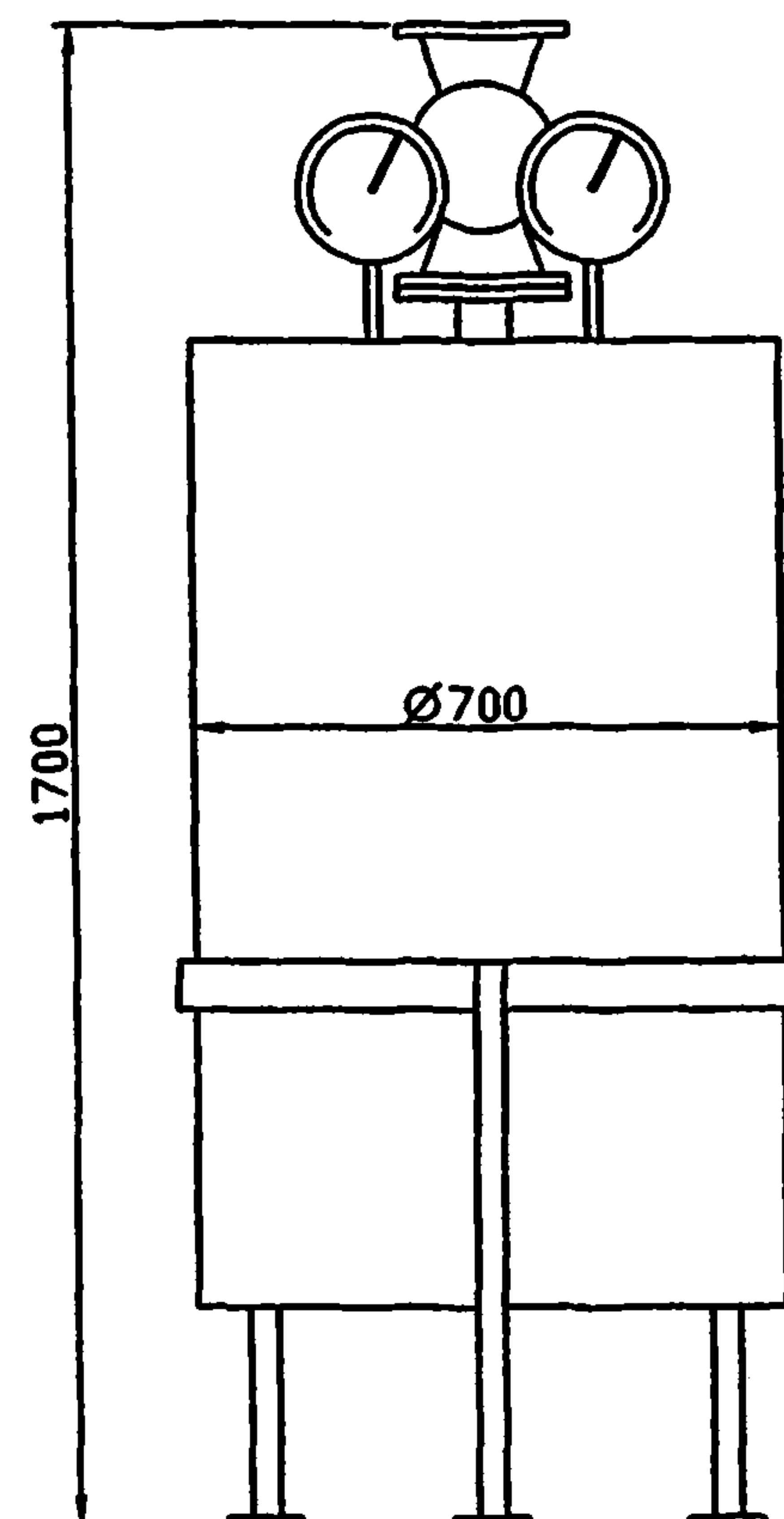
Общий вид эл.котла КЭП
