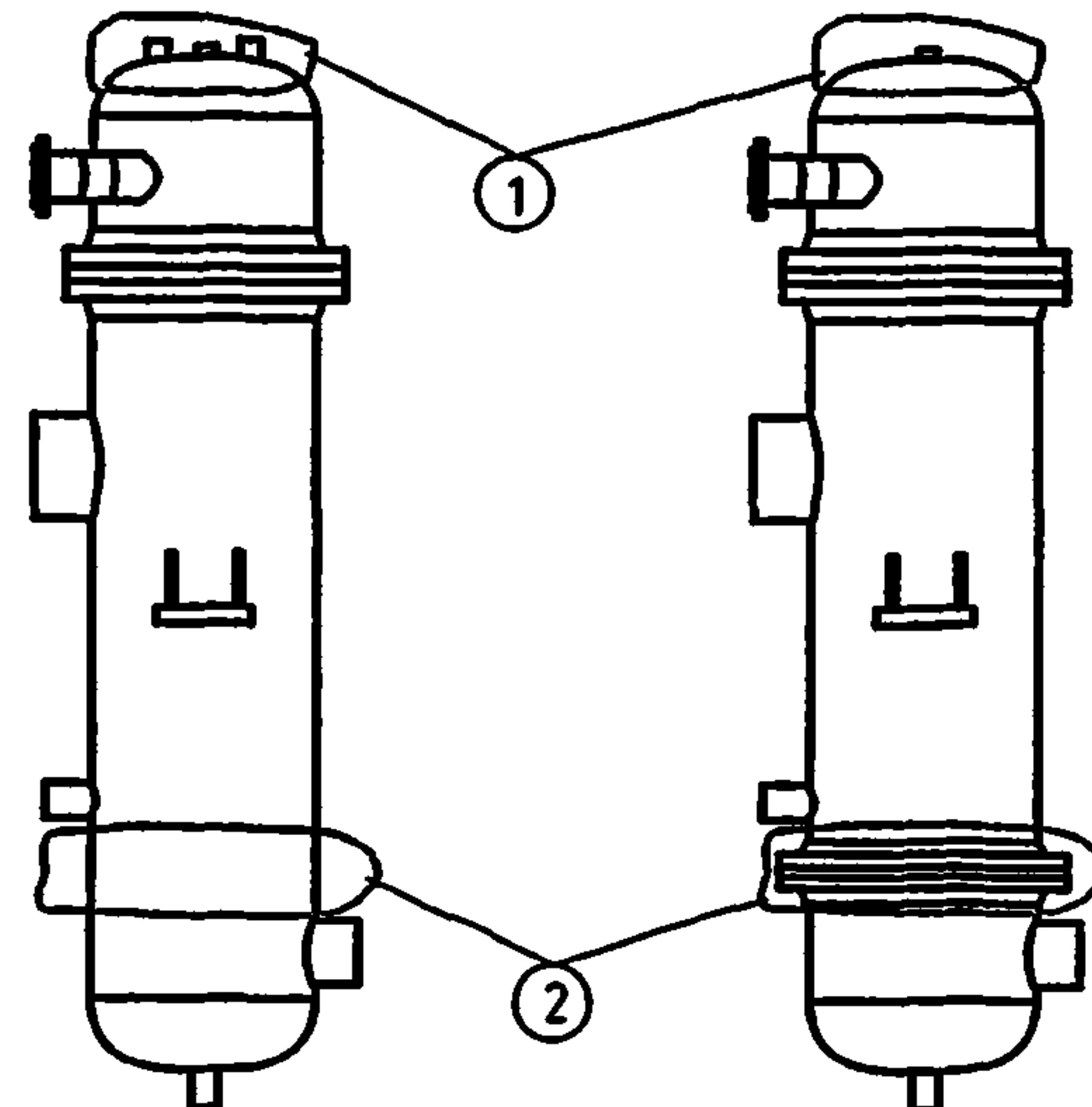
рис. Пример подогревателей ПСВ 1 — исключение анкерных связей; 2 — дополнительный фланцевый разъём для осмотра и трубной системы без её выема из корпуса;
