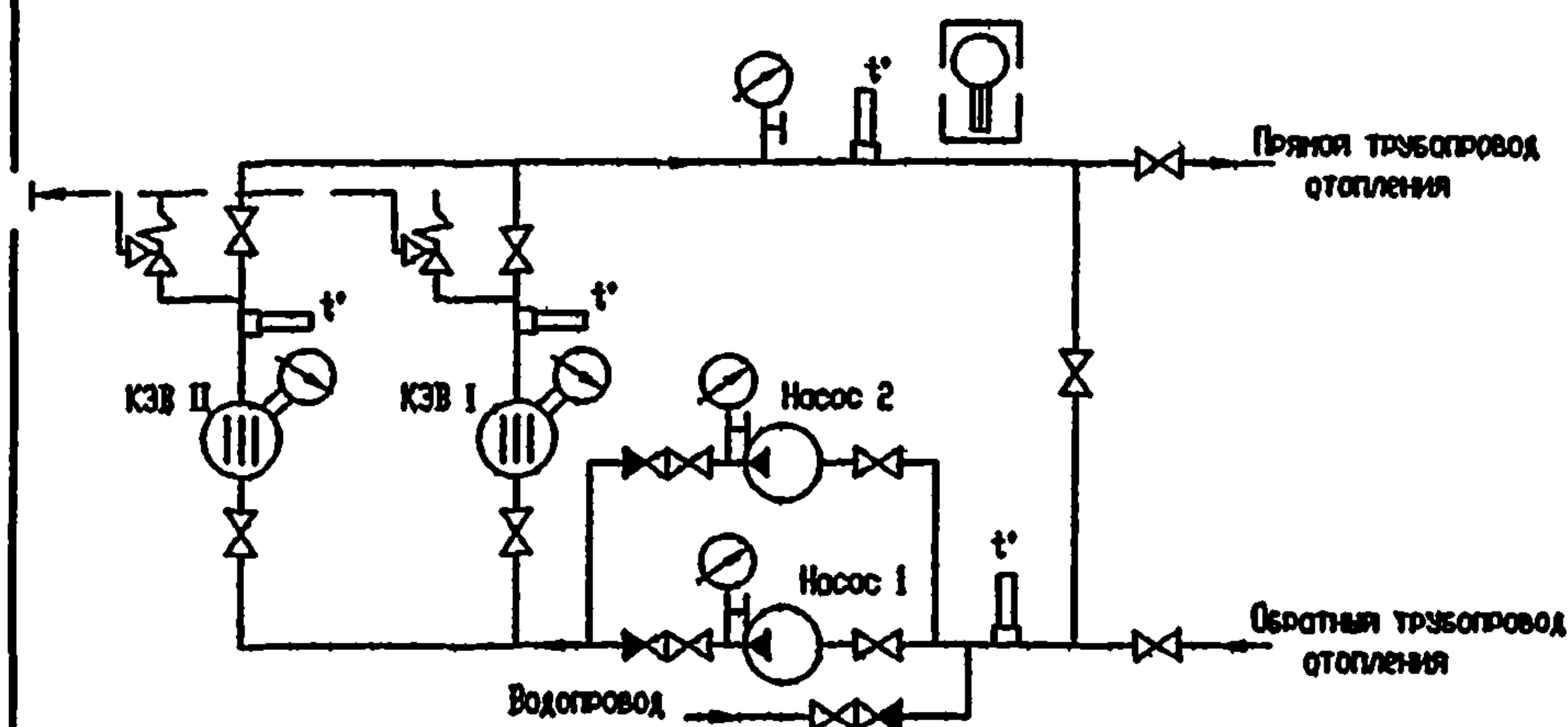
Принципиальная тепловая схема электрокотельной отопления
