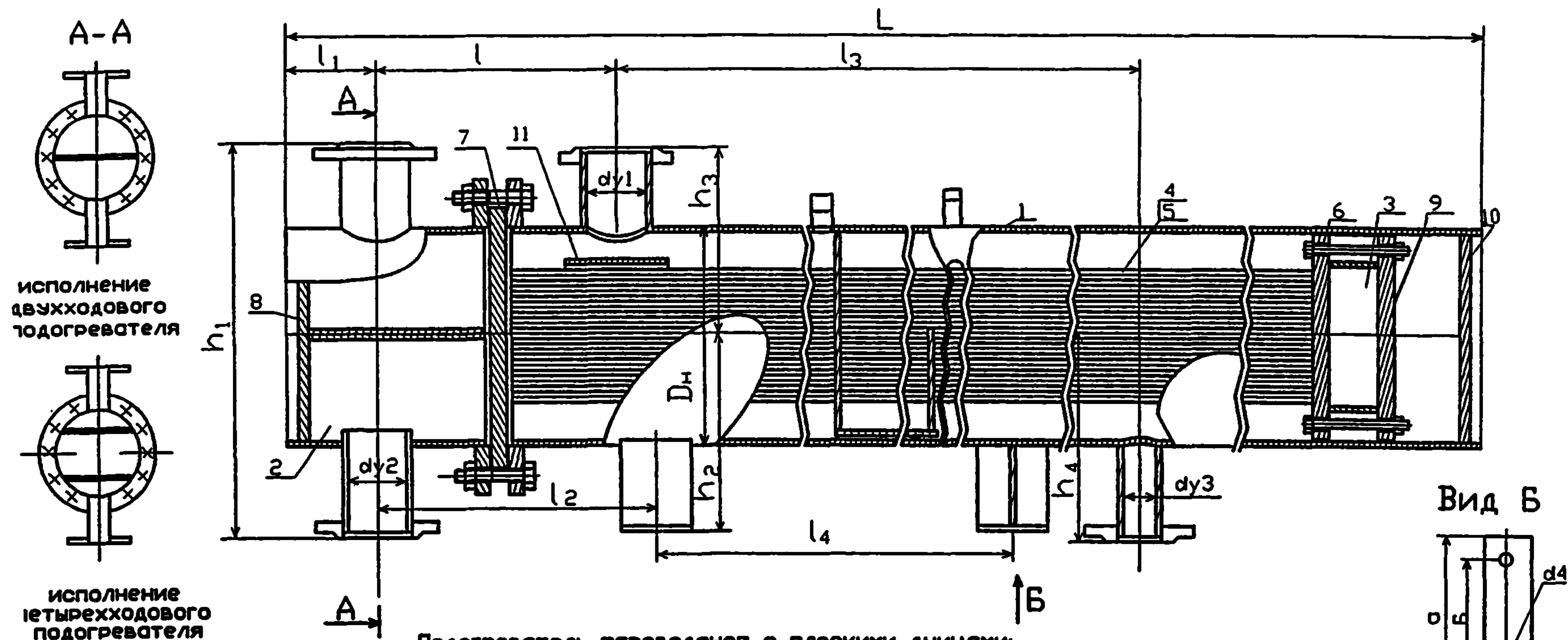
Подогреватель пароводяной с плоскими днищами.
