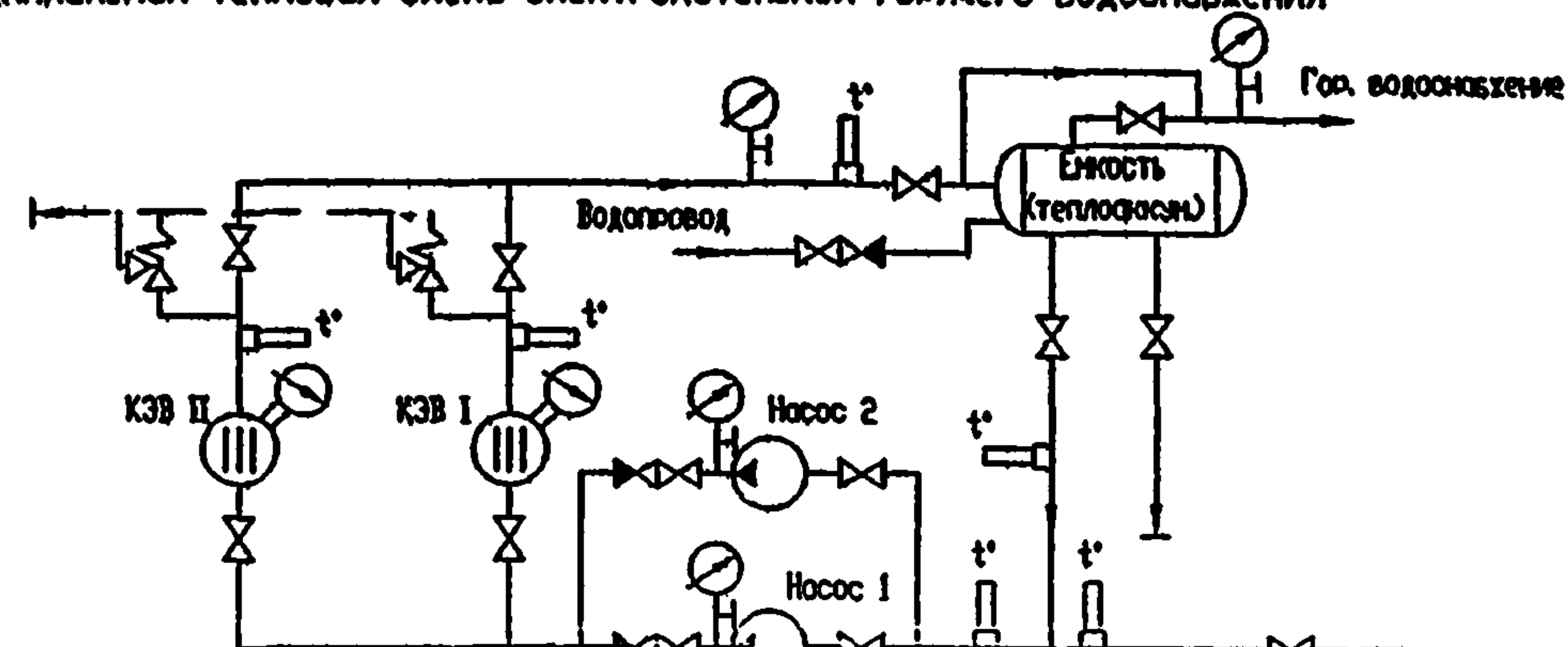
Принципиальная тепловая схема электрокотельной горячего водоснабжения
