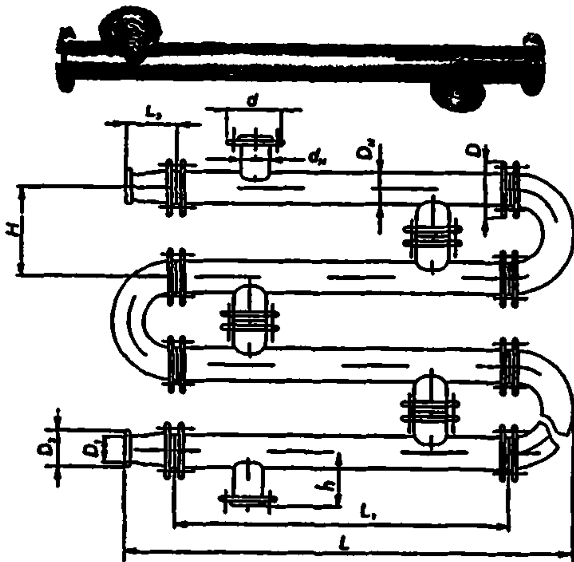
Габаритные и присоединительные размеры, мм
