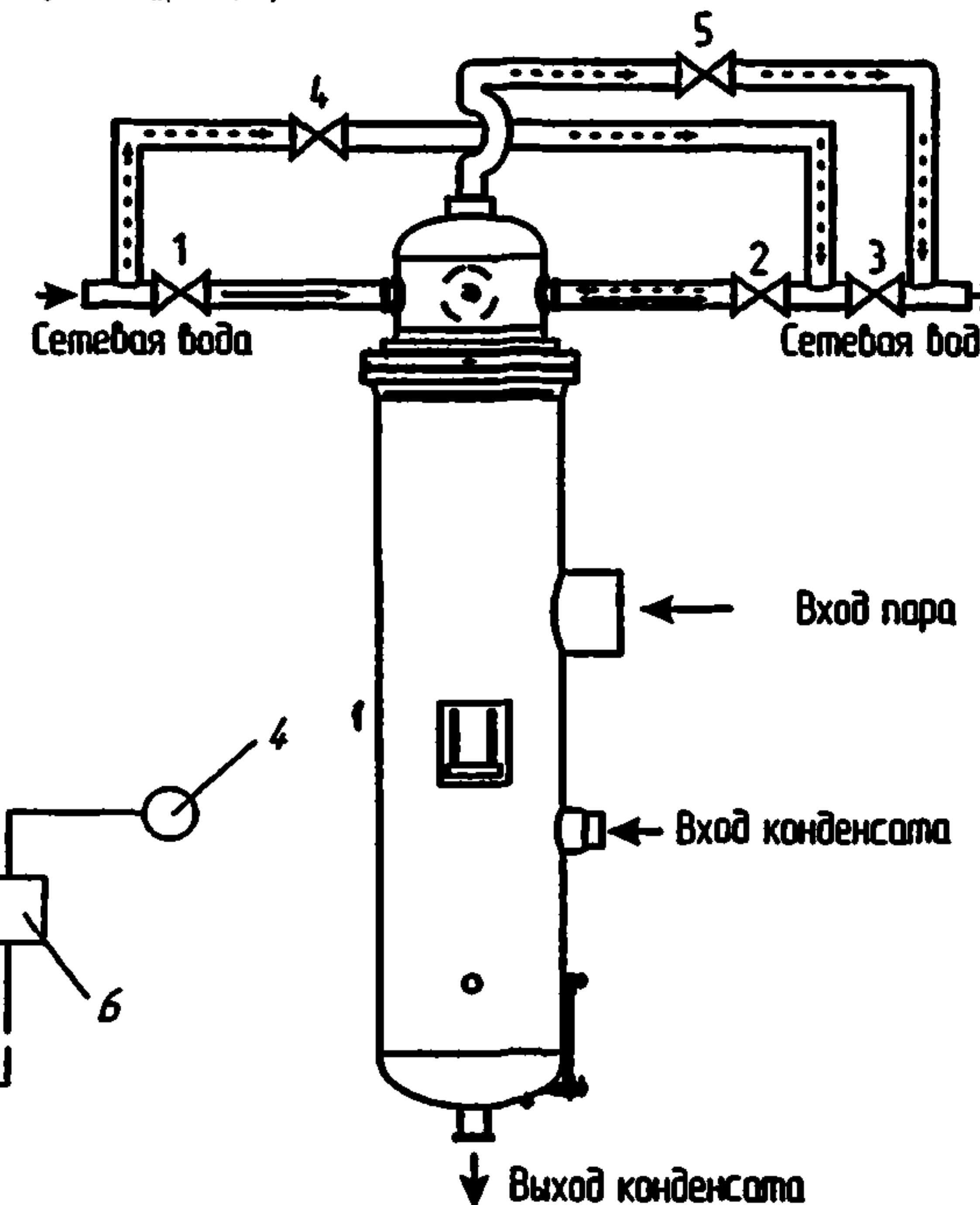
Схема включения подогревателя ПСВ-300-14-23
