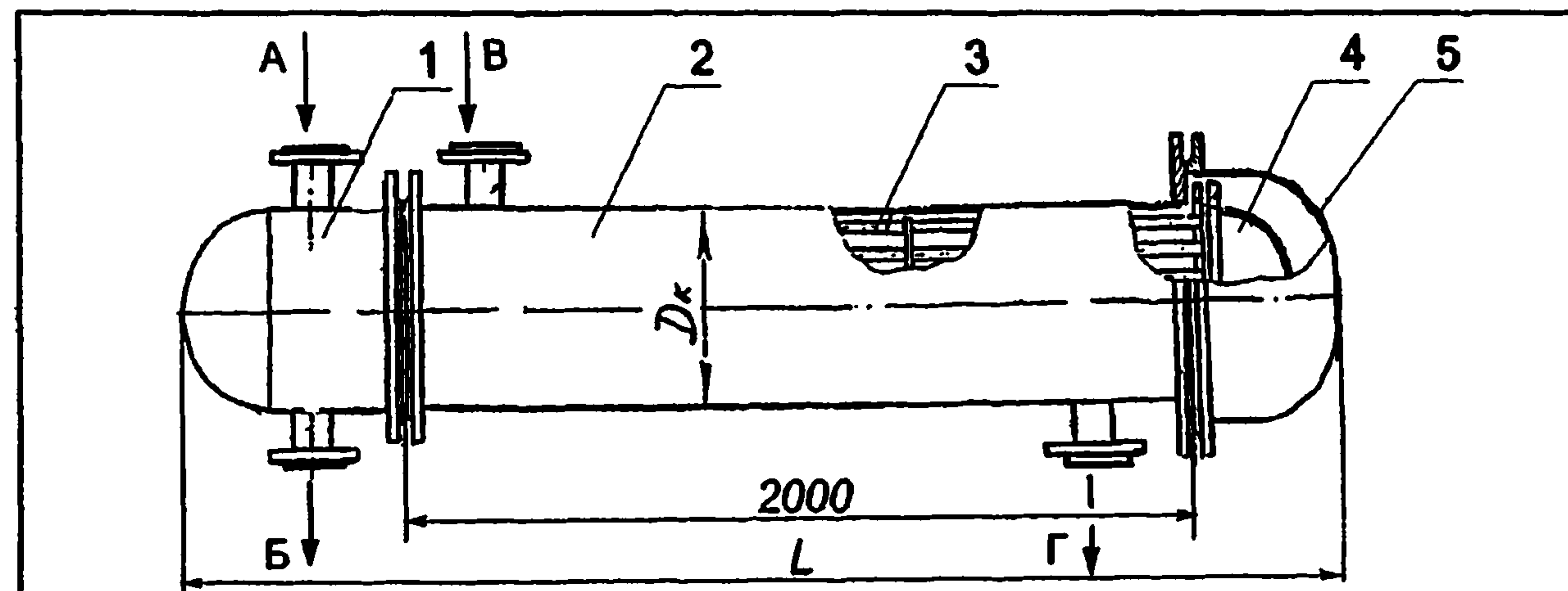
Рис. 1. ВОДОПОДОГРЕВАТЕЛЬ ТИПА ВПМР
