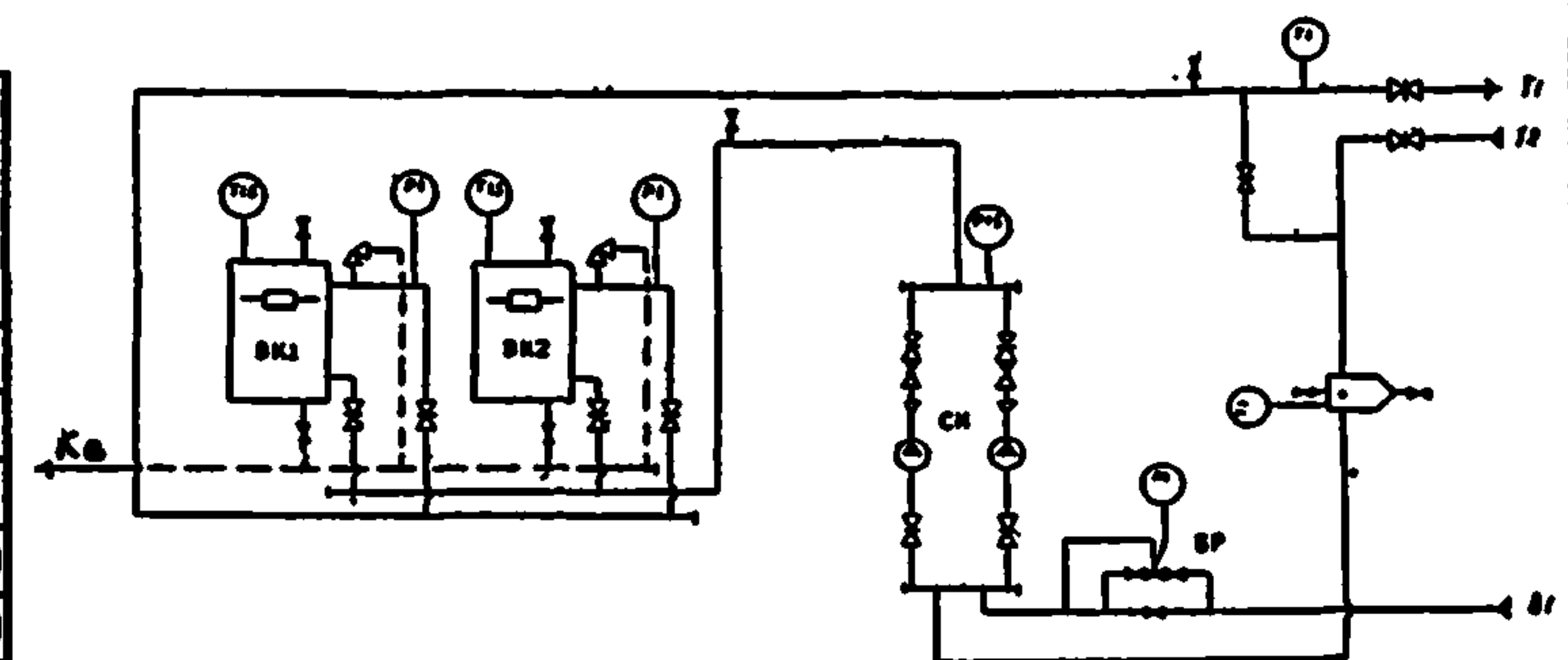
Принципиальная тепловая схема электростанции с двумя электродными котлами для закрытой системы отопления.
