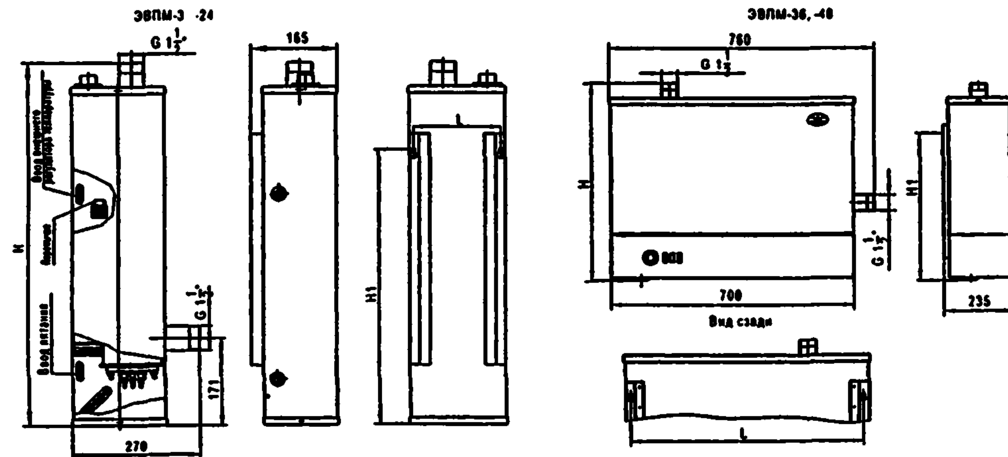
Электроводонагреватели ЭВПМ-3...-48. Габаритный чертеж
