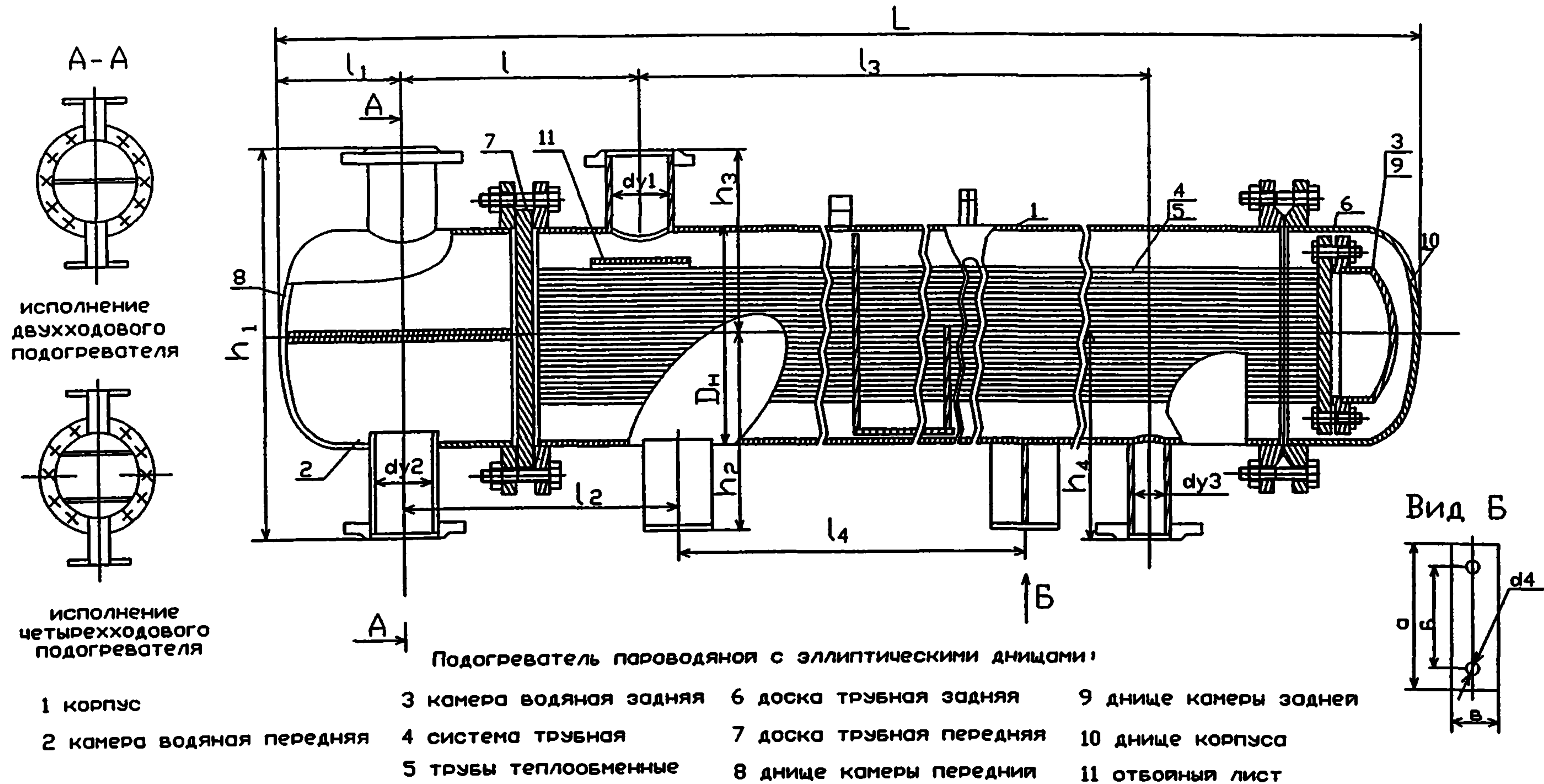
Габаритные и присоединительные размеры
