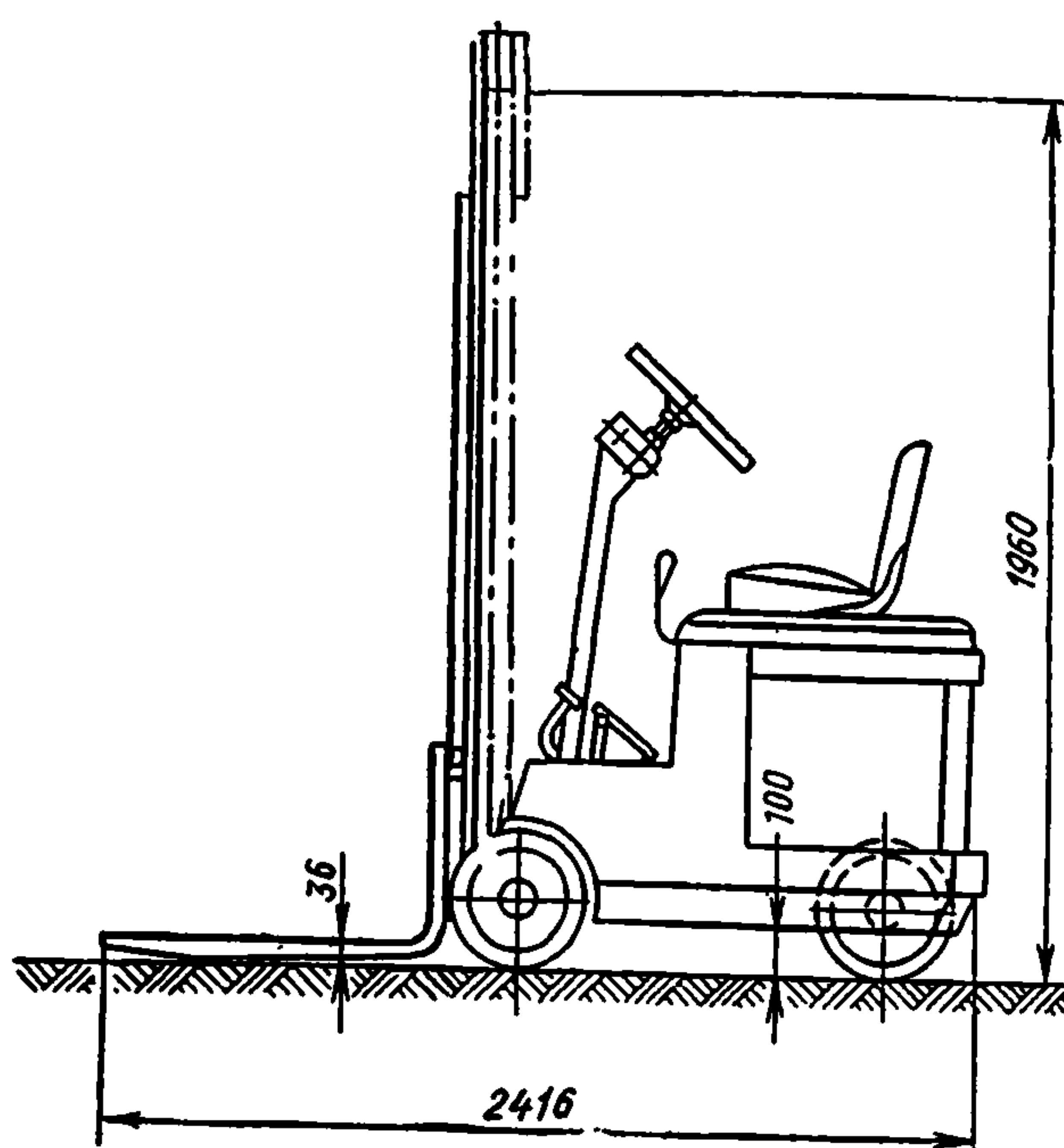
Рис. 35. Электропогрузчик ЭП-1201
