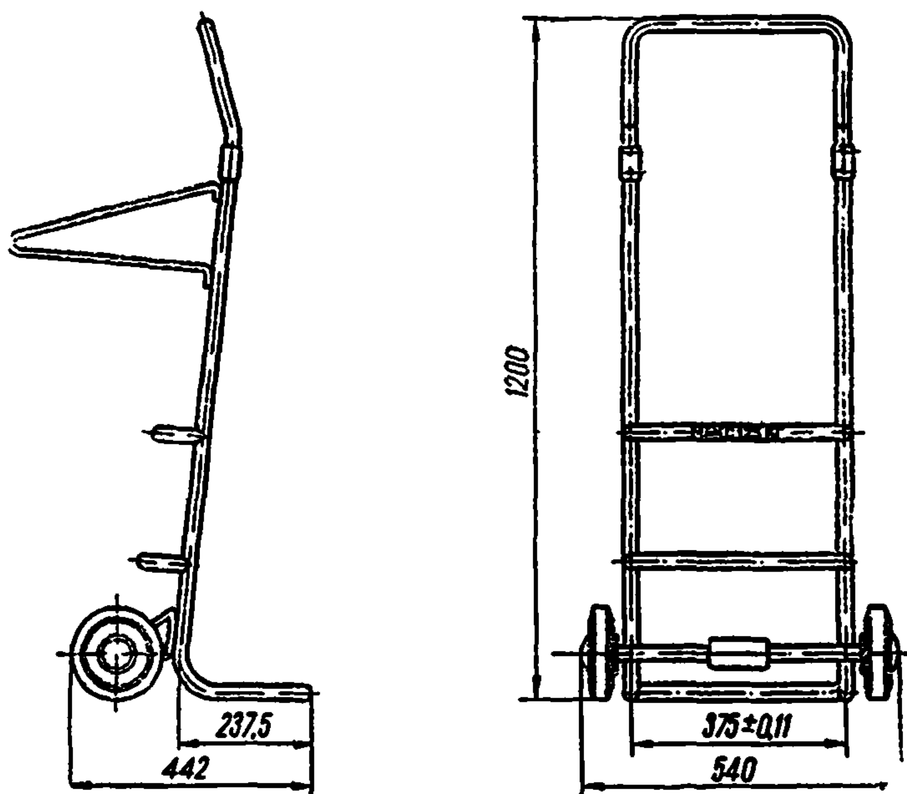
Рис. 39. Тележка ручная ТГМ-125
