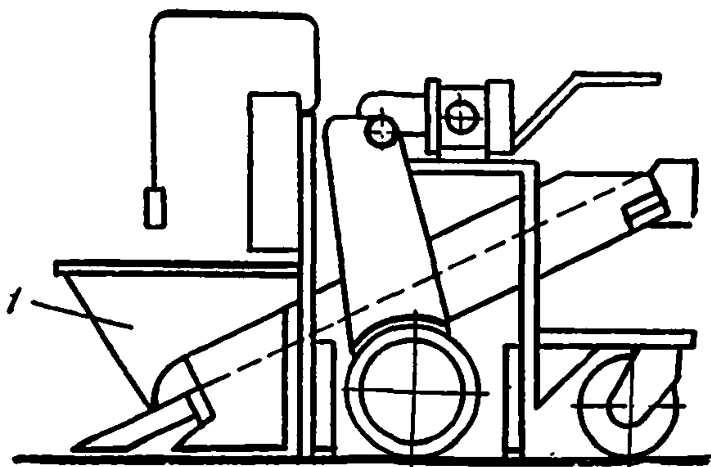
Рис. 4. Подборщик с бункером: 1 — бункер
