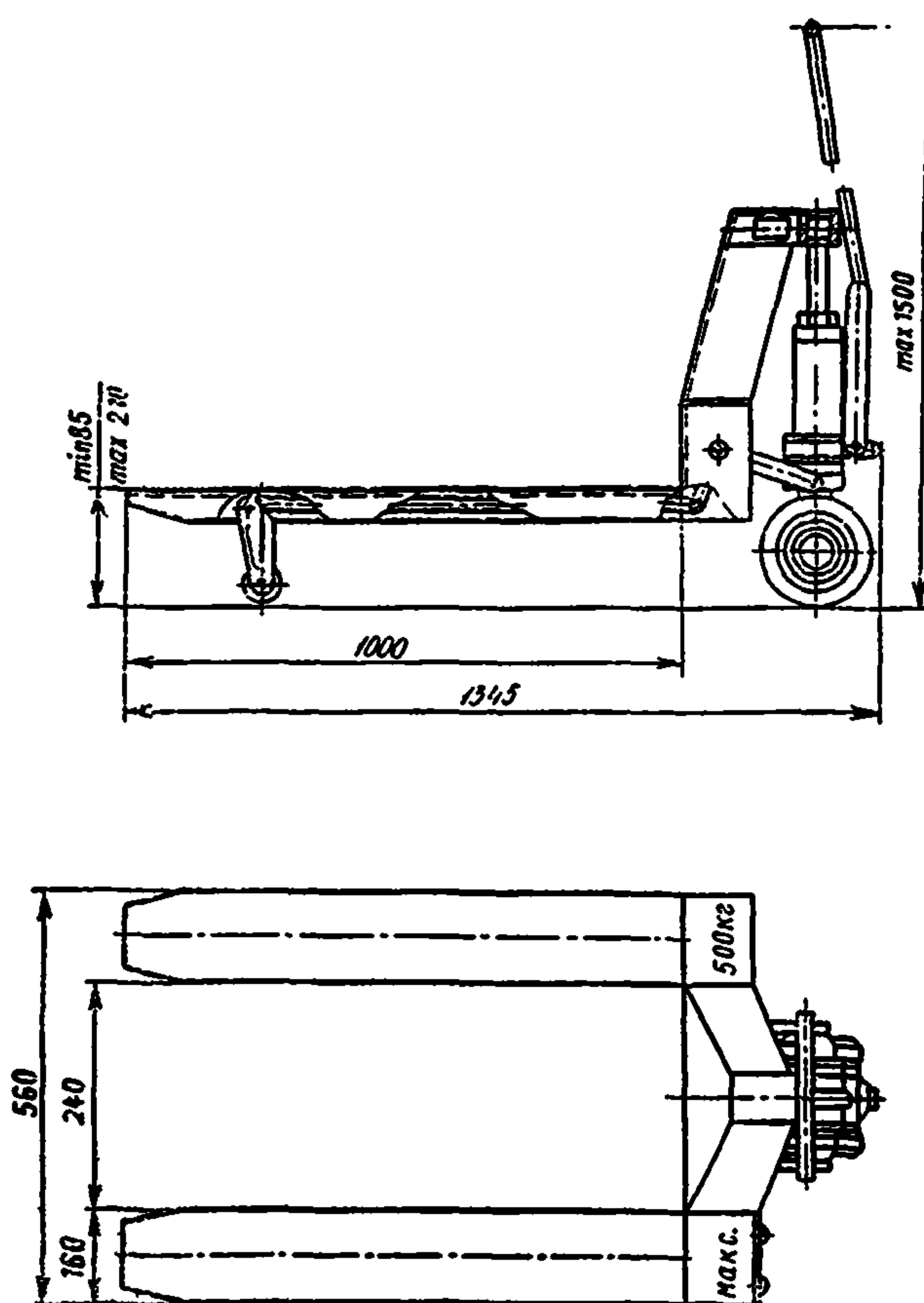
Рис. 41. Гидравлическая тележка с подъемными вилами ТГП-500
