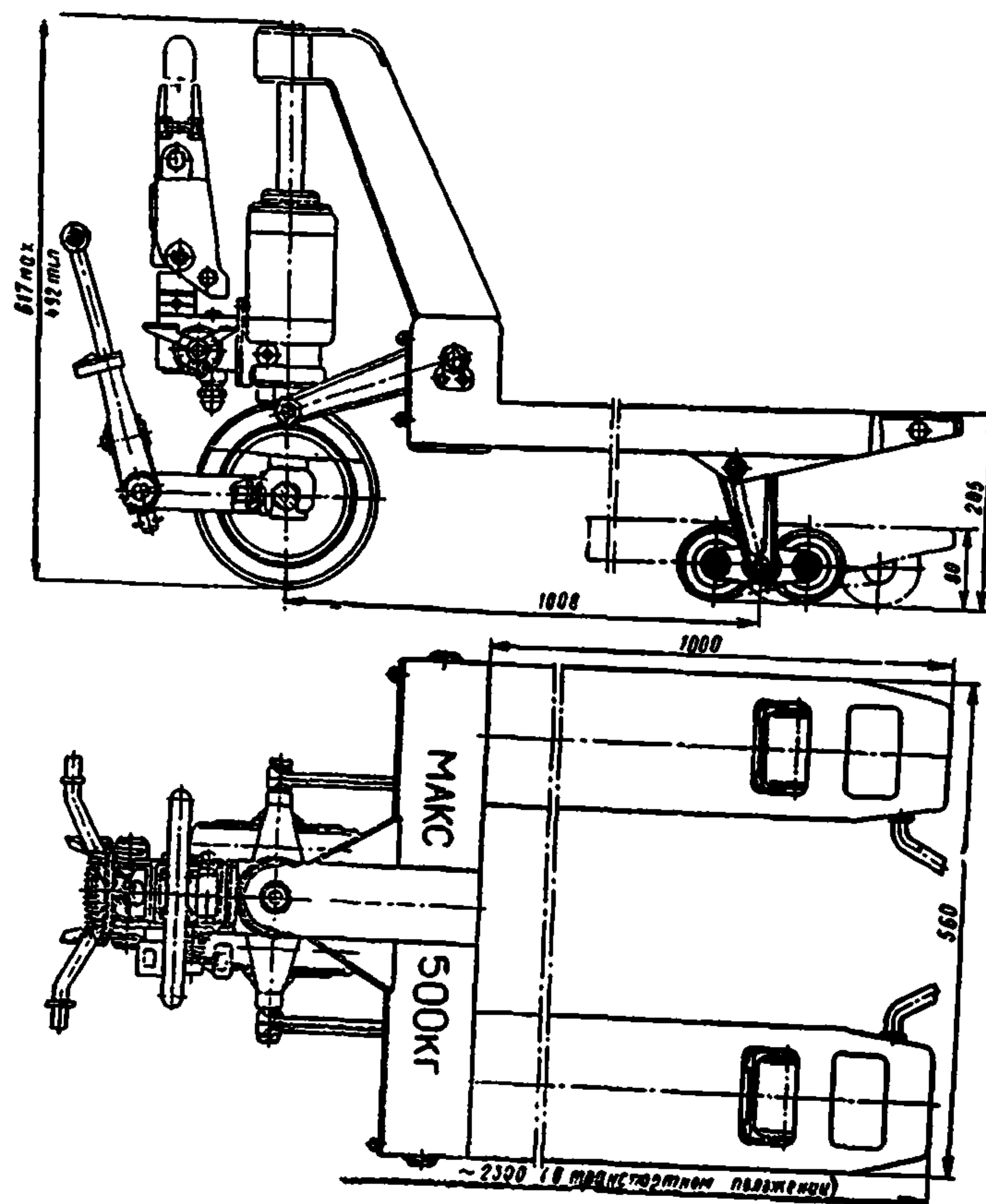
Рис. 42. Гидравлическая тележка с подъемными вилами ТГВ-500 М
