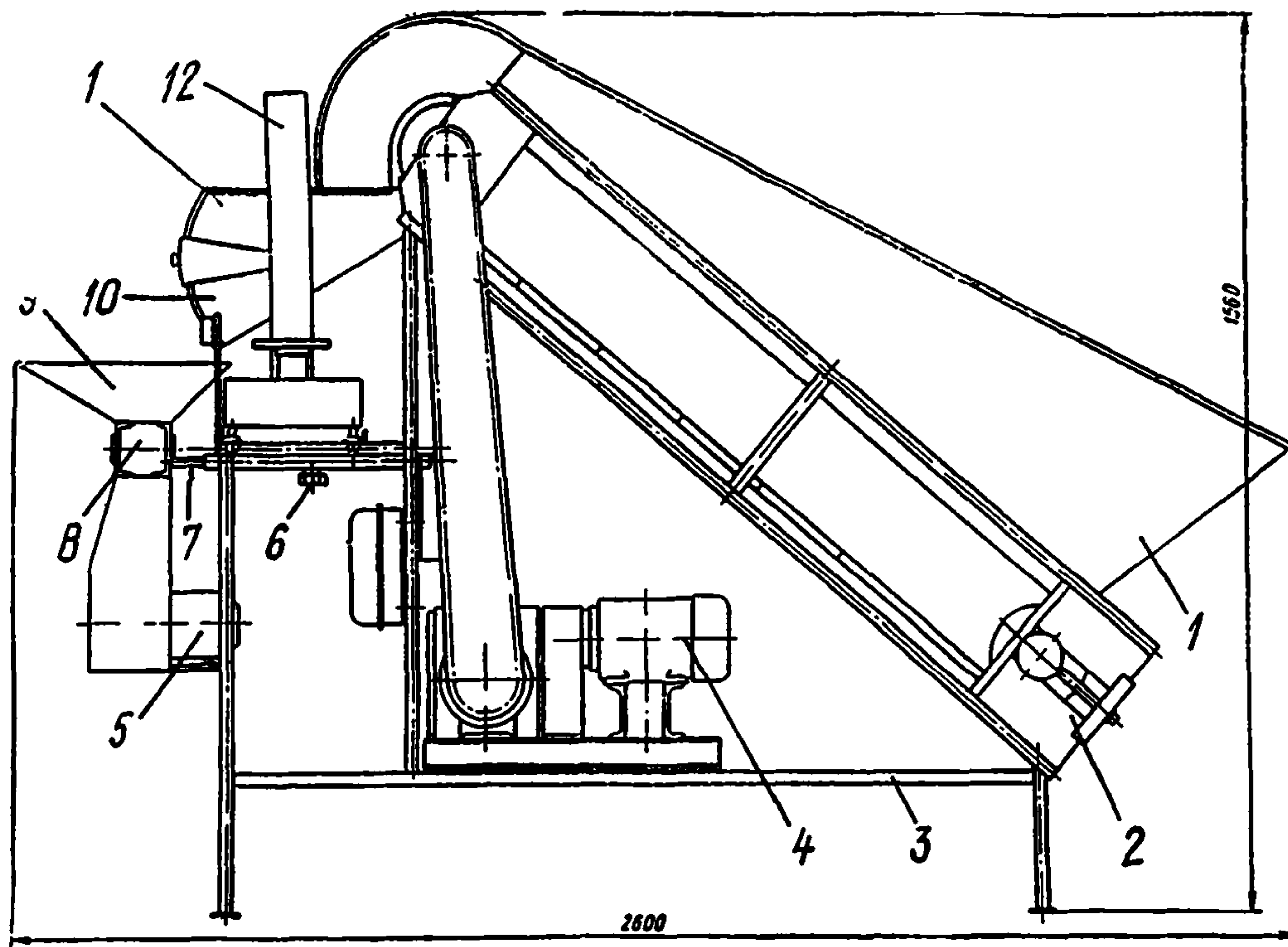
Рис. 50. Установка для фасования УФ-79:
