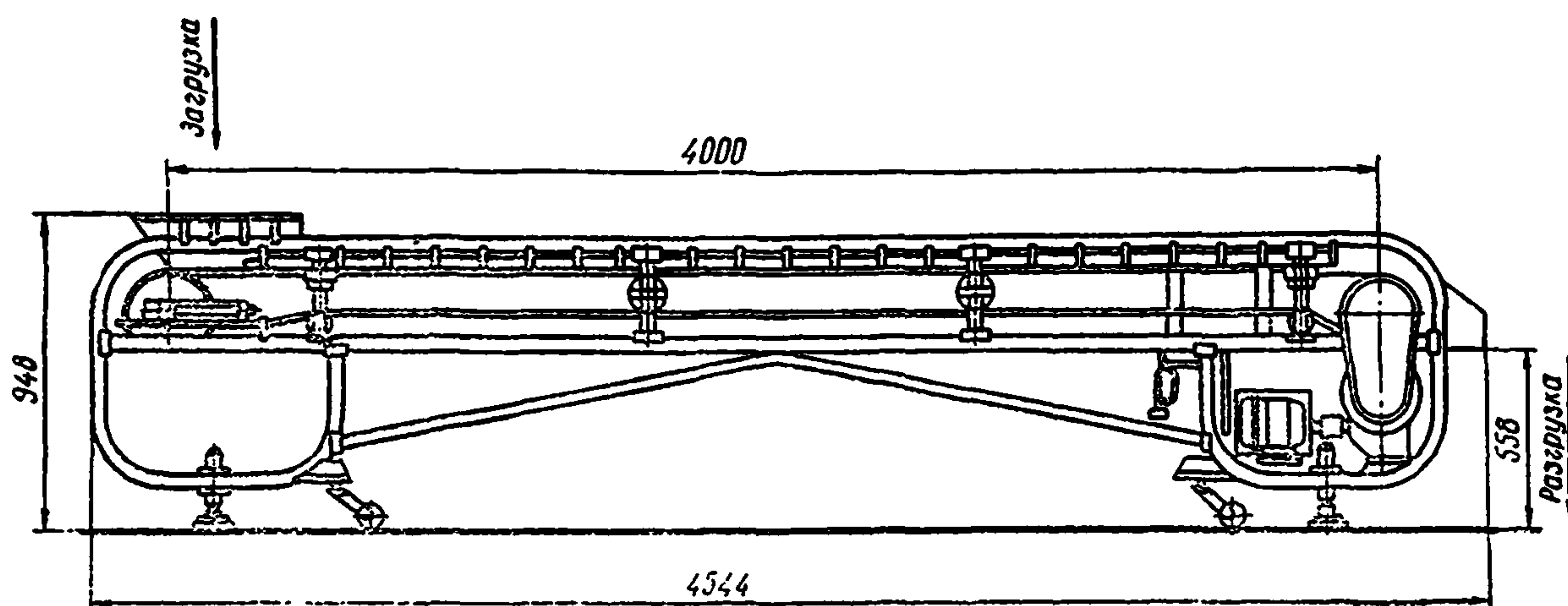
Рис. 49. Транспортёр сортировочно-инспекционный ТСИ
