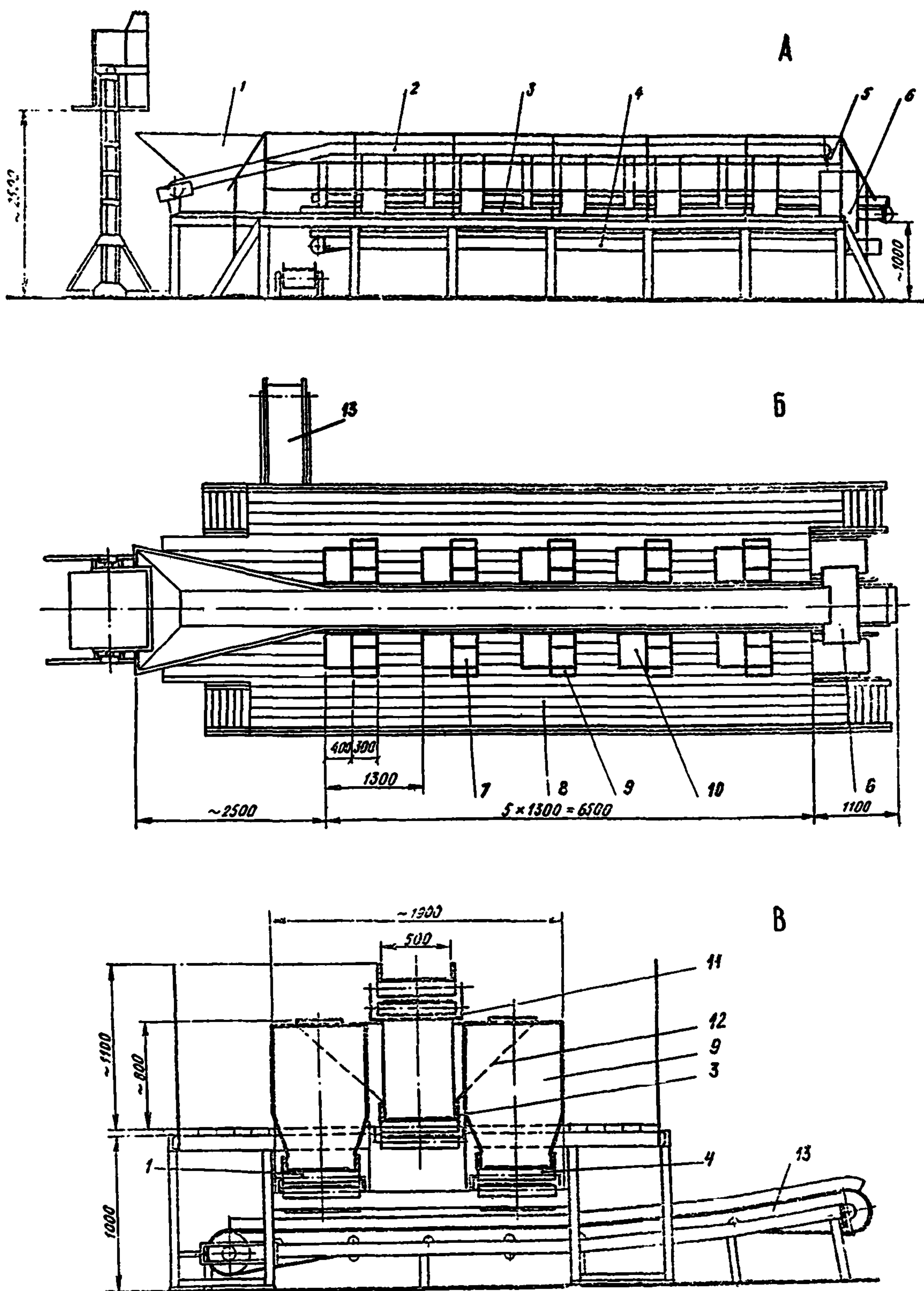
Рис. 61. Рациональная схема участка зачистки кочанов: А—вид сбоку, Б—вид сверху, В—разрез. 1—приемный бункер; 2—конвейер для незачищенных кочанов; 3—конвейер для зачищенных кочанов; 4—конвейер для отходов; 5—очищающий скребок; 6—двускатный лоток; 7—стол для зачистки; 8—площадка; 9—окна шахты для отходов; 10—люк для зачищенных кочанов; 11—поддон; 12—наклонный склиз; 13—поперечный конвейер для отходов
