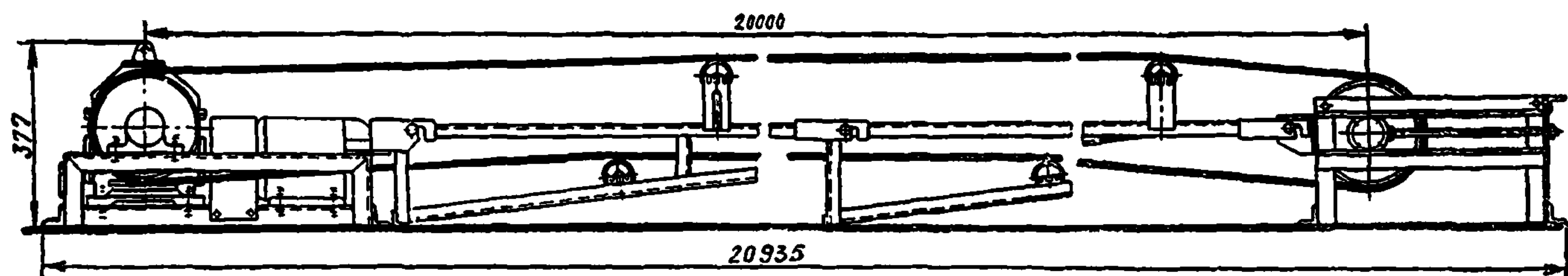
Рис. 14. Конвейер ленточный 20-метровый КЛ-500-20
