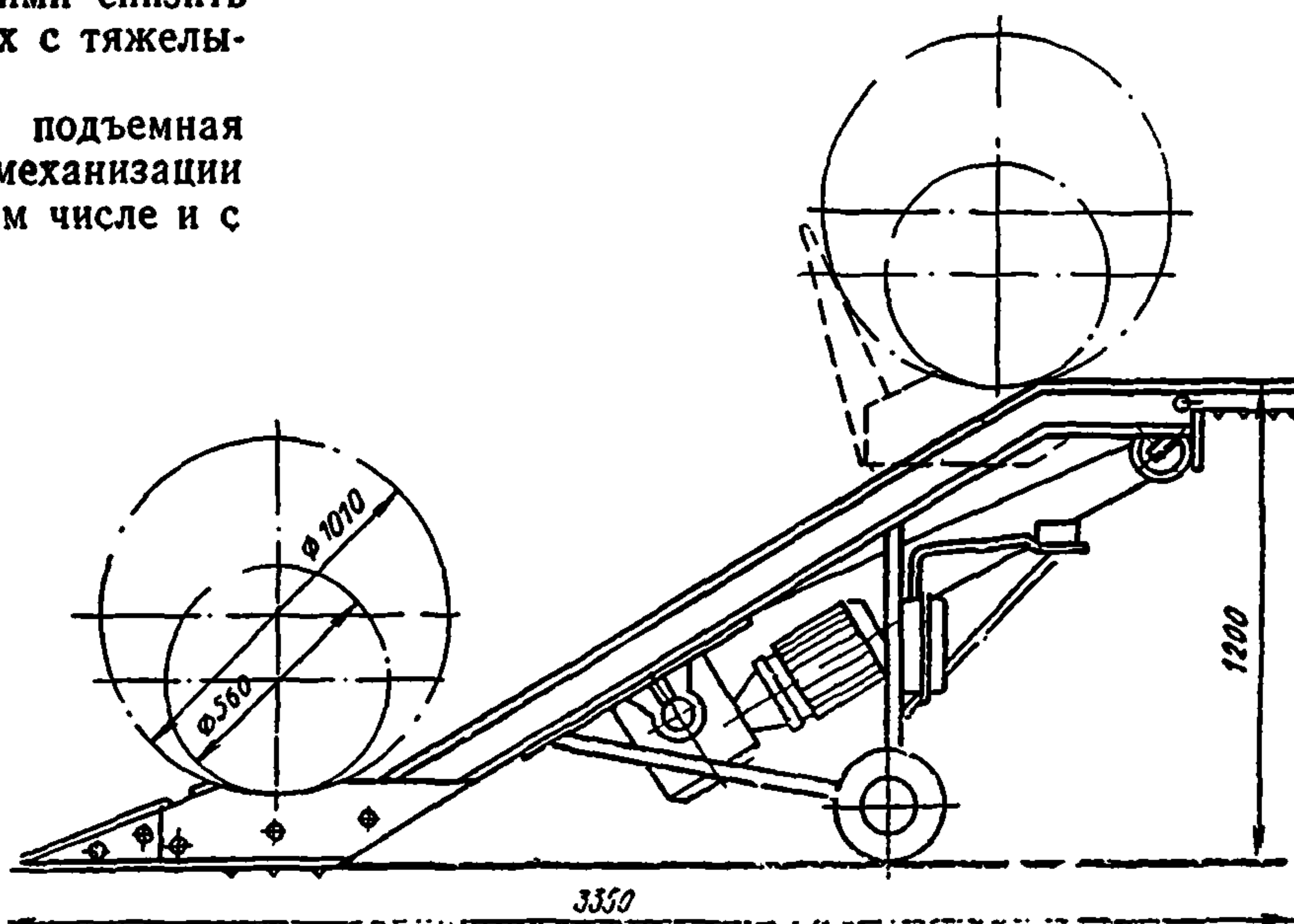
Рис. 27. Бочкопогрузчик М8-ВБП-100
