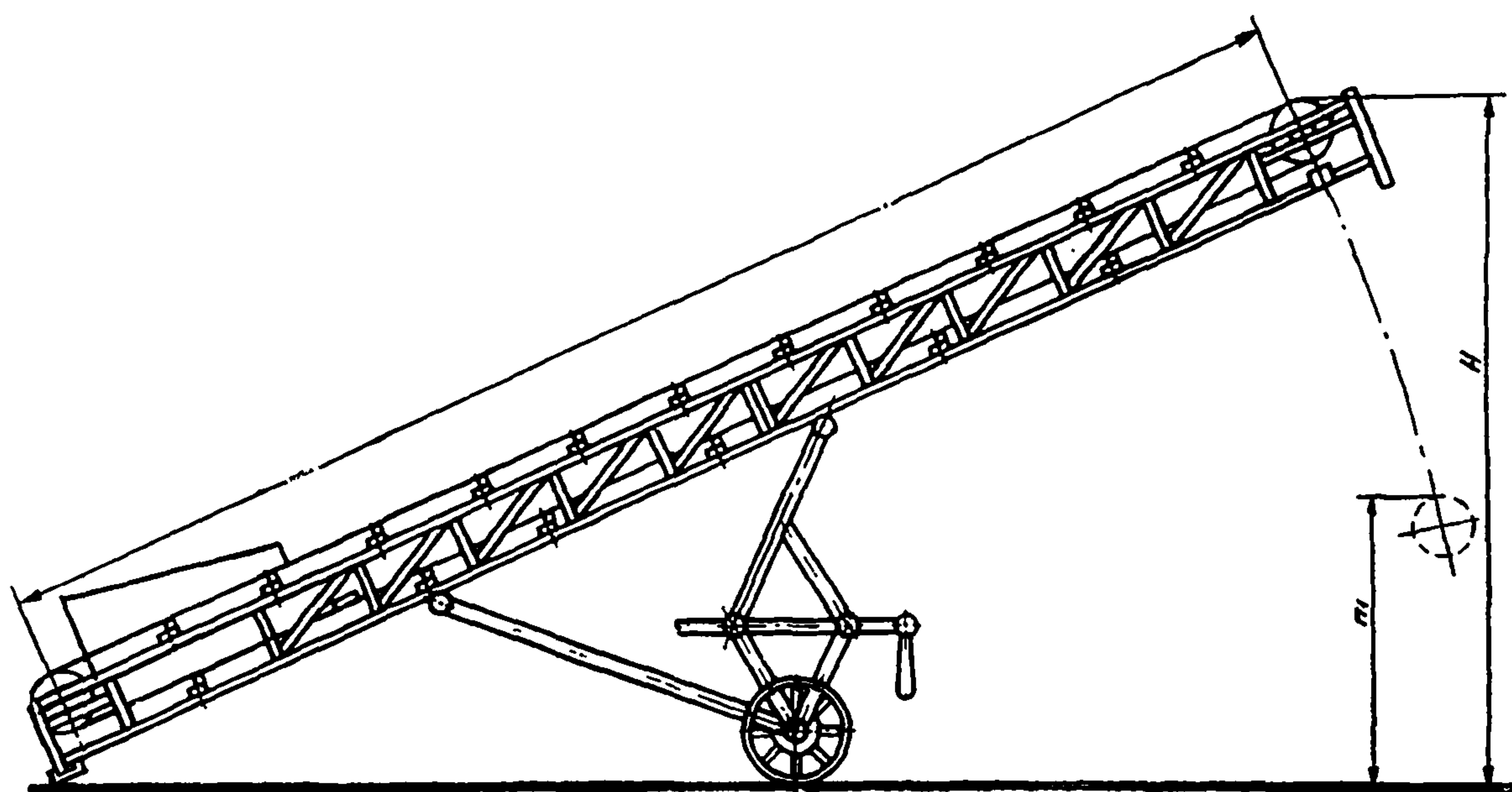
Рис. 15. Конвейер ленточный передвижной 10 и 15-метровый КЛП-500-10, КЛП-500-15
