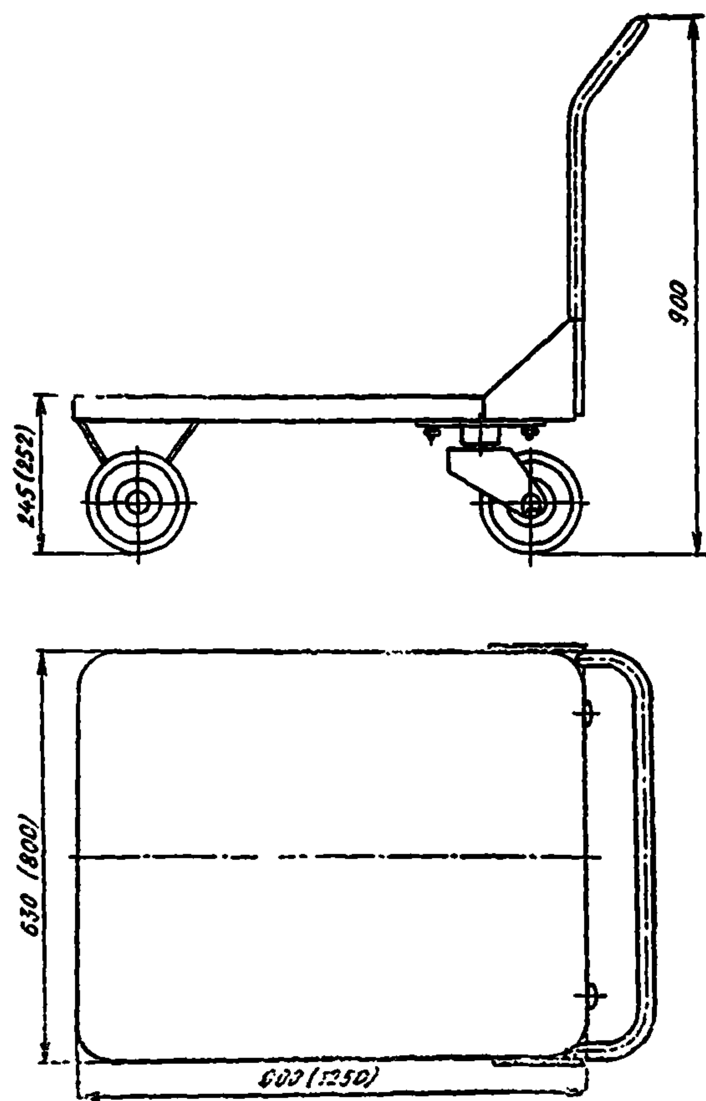
Рис. 38. Тележка ручная ТГ-125 (250)
