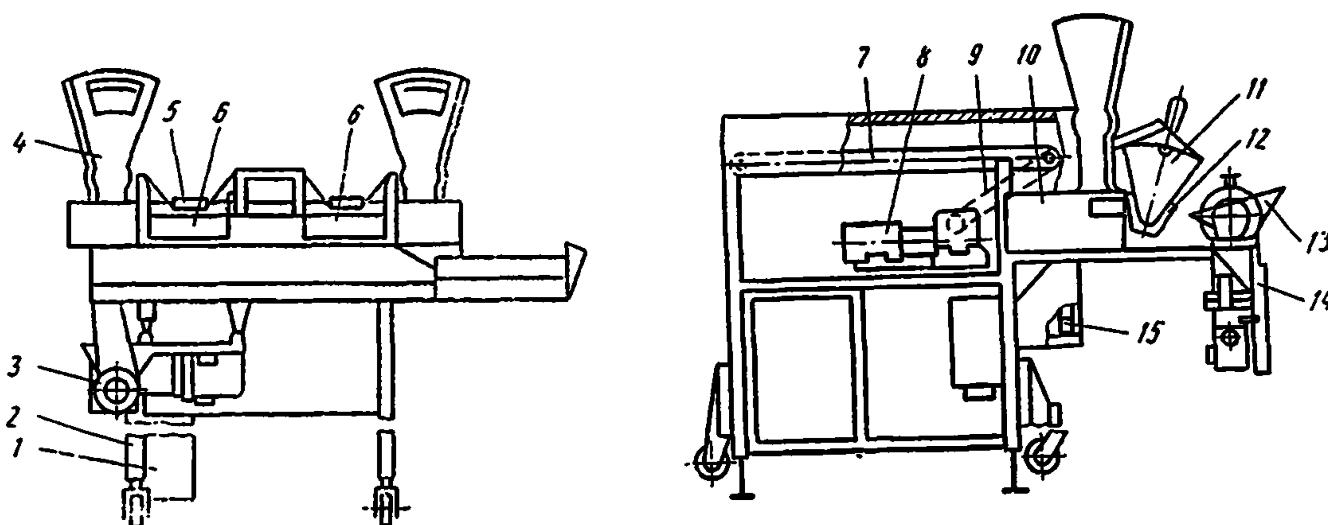
Рис. 51. Весы полуавтоматические ДОФ-5:
