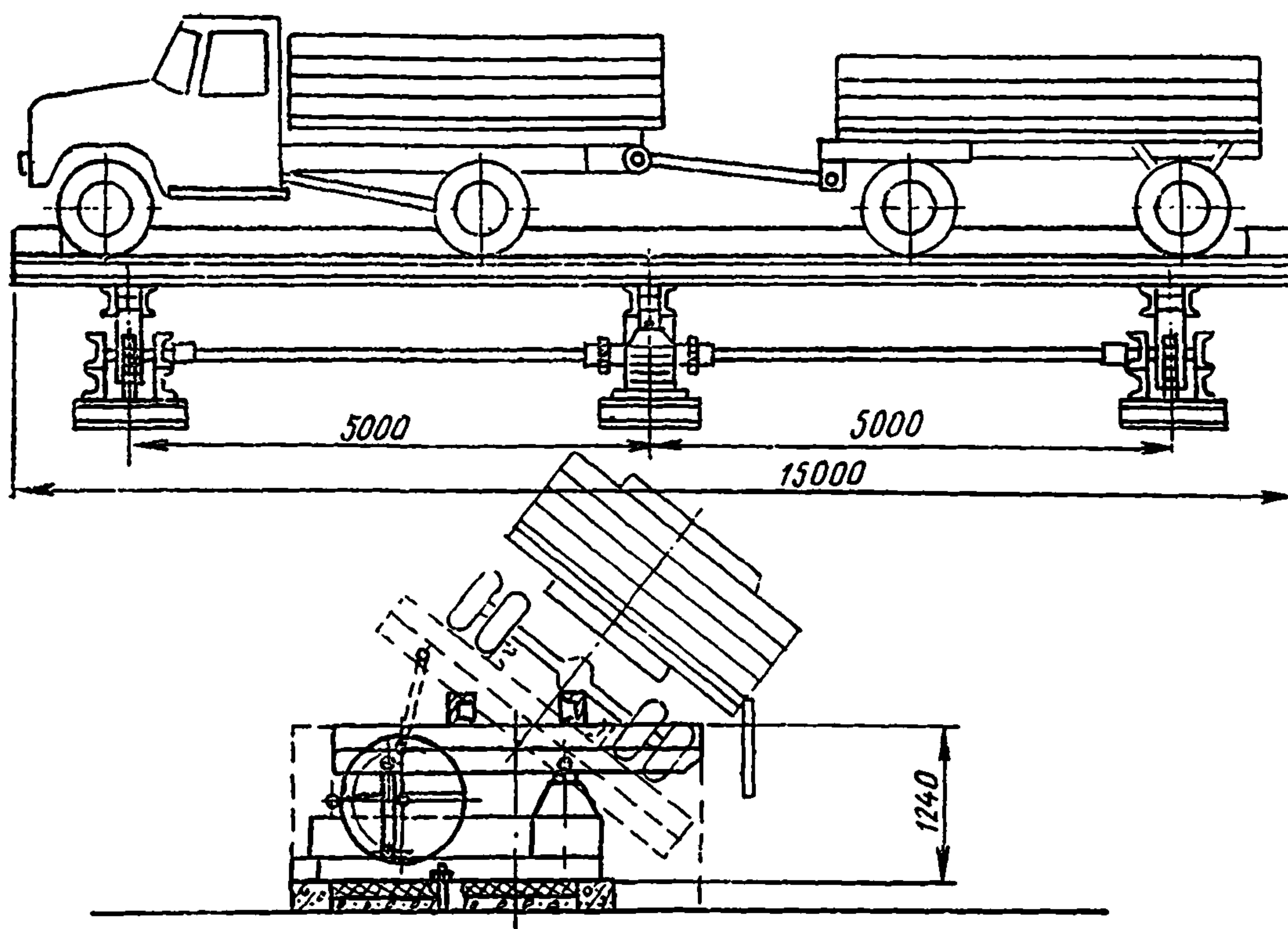
Рис. 8. Автомобилеразгрузчик АВС-50М
