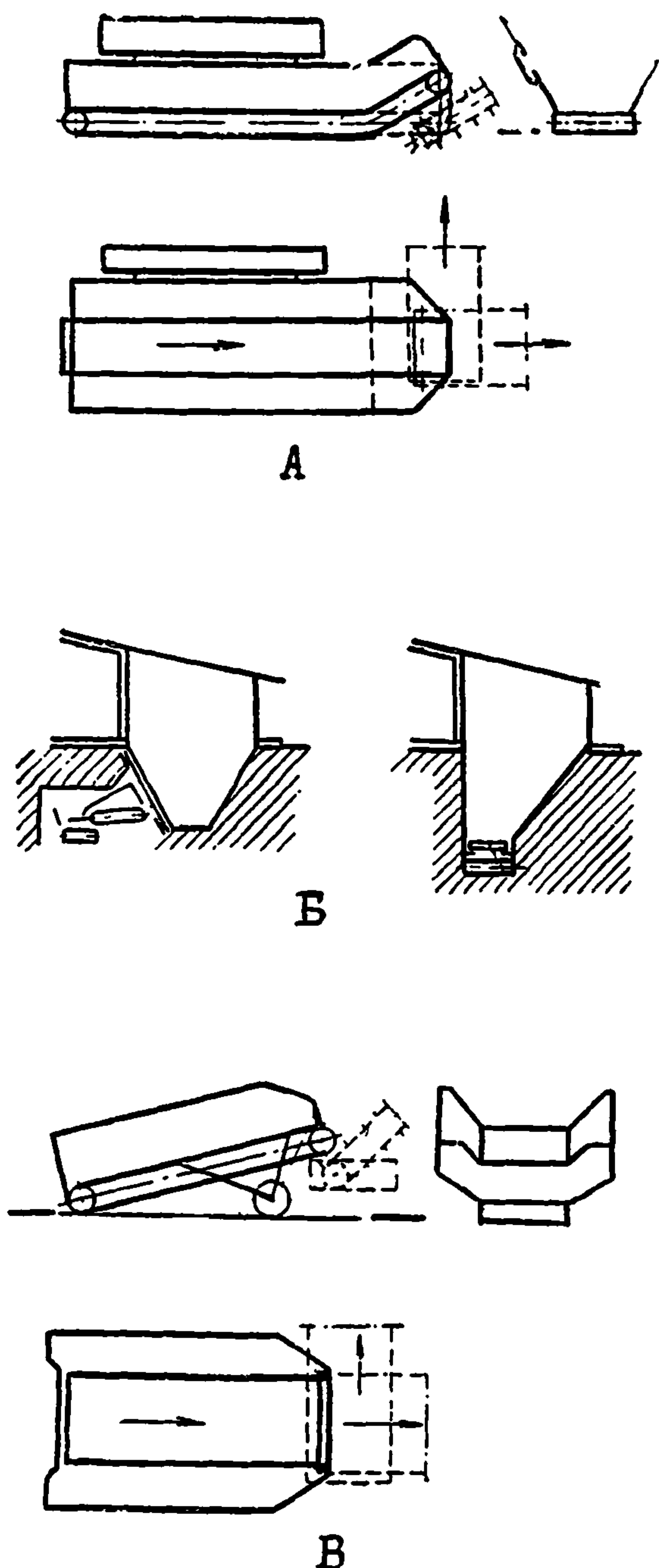
Рис. 11. Конструктивные схемы приемных бункеров
