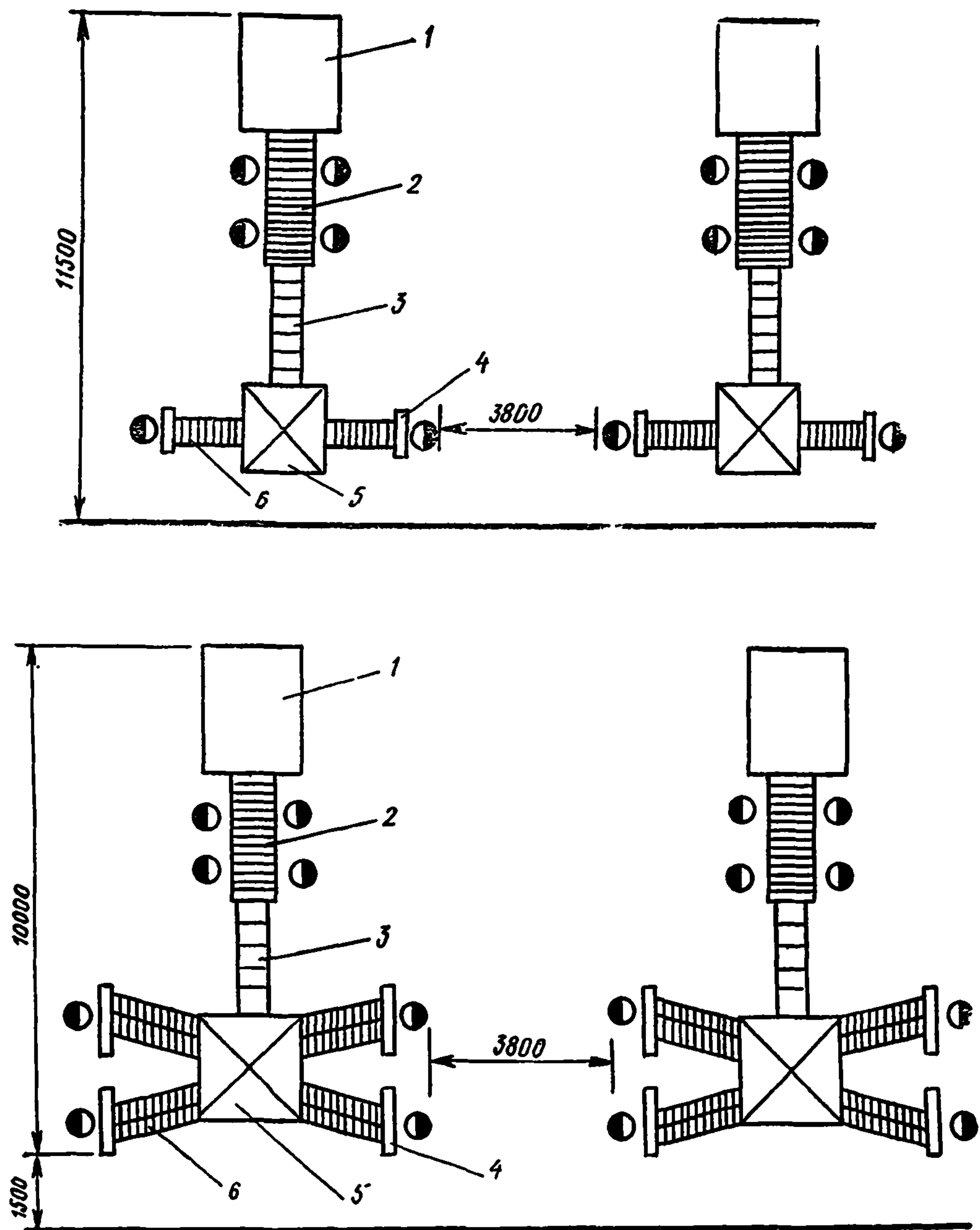
Рис. 59. Варианты расстановки оборудования на участке товарной обработки и фасовки овощей:
