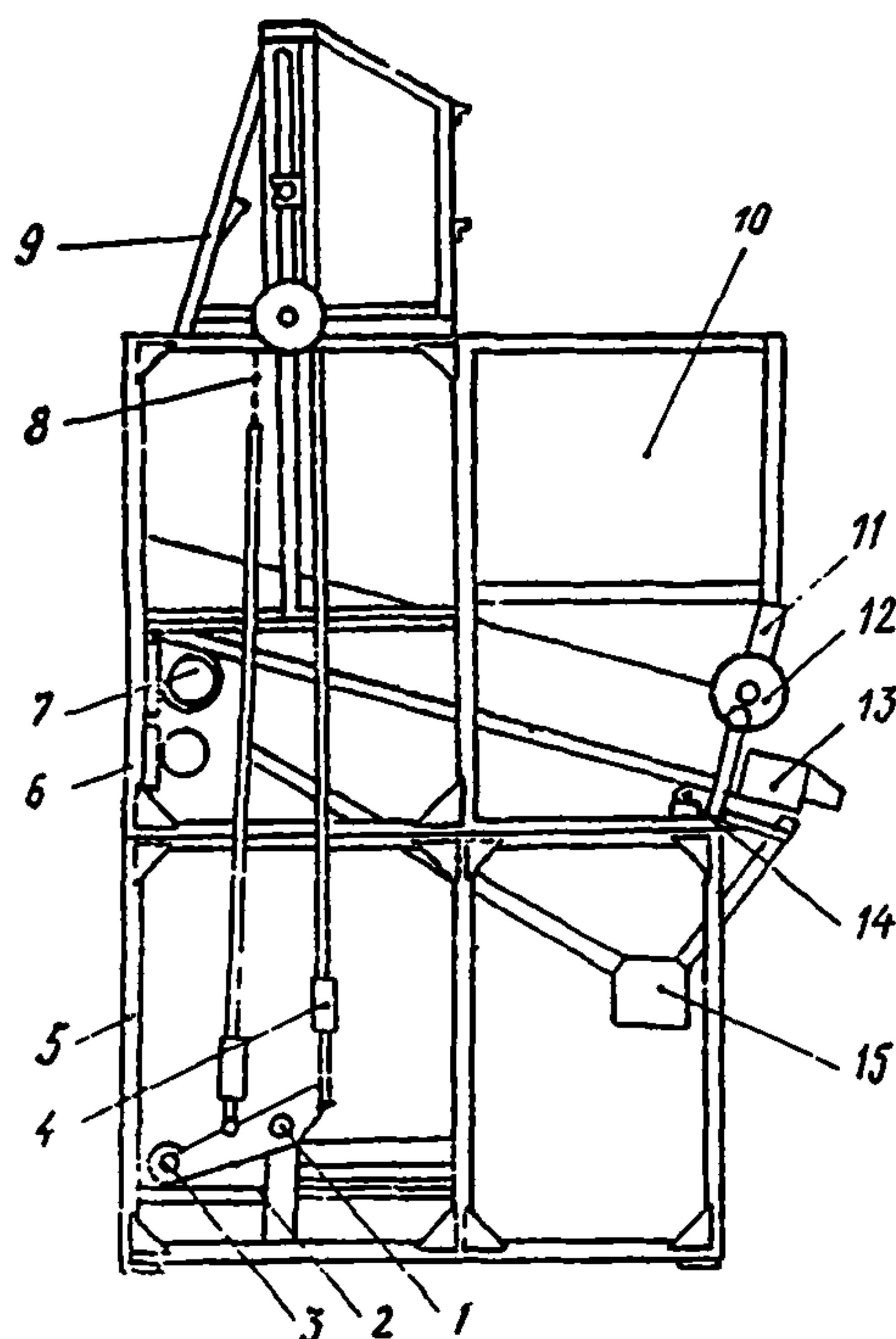
Рис. 44. Контейнероопрокидыватель КУП-1000:
