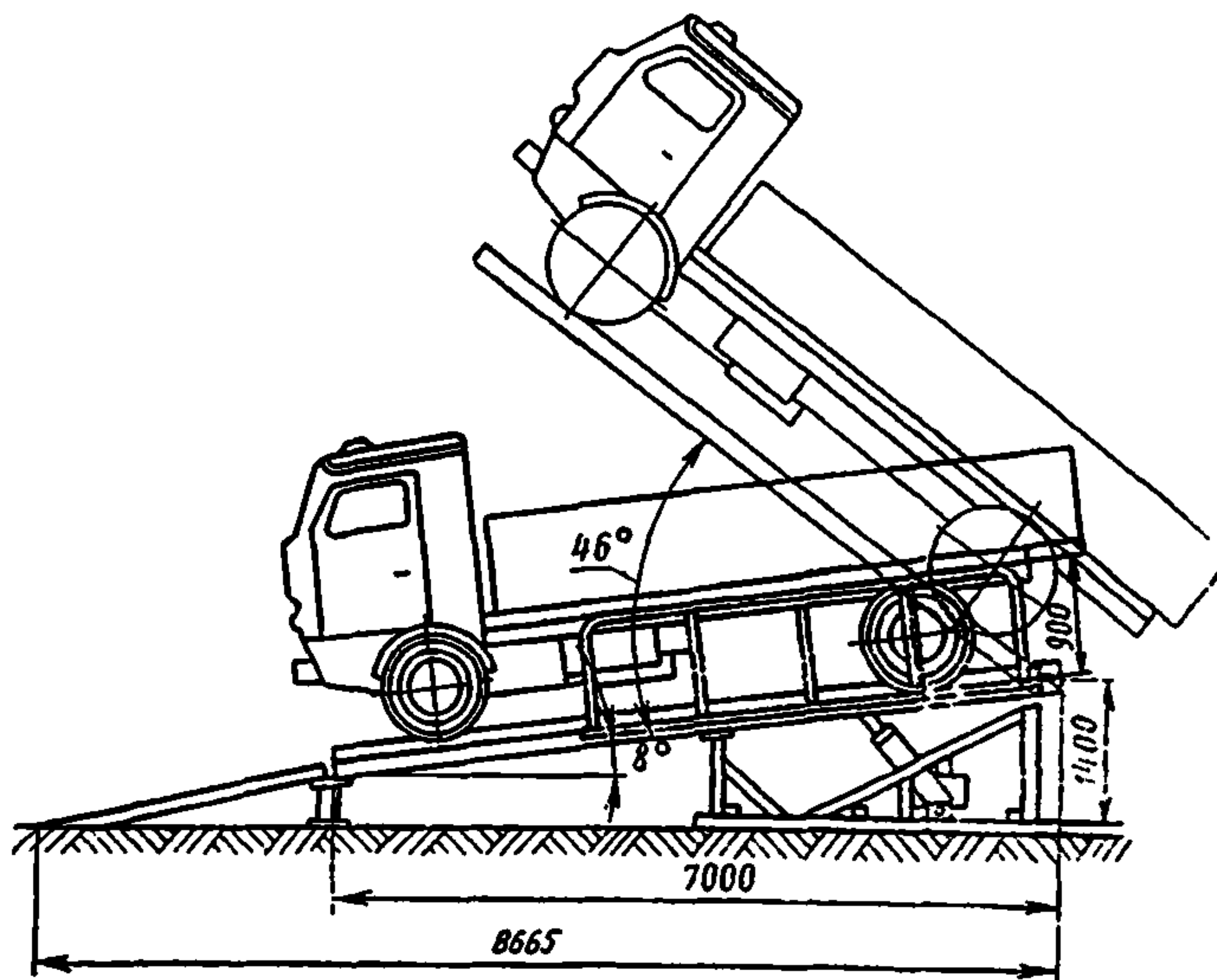
Рис. 10. Автомобилеразгрузчик ГУАР-15Н (П)
