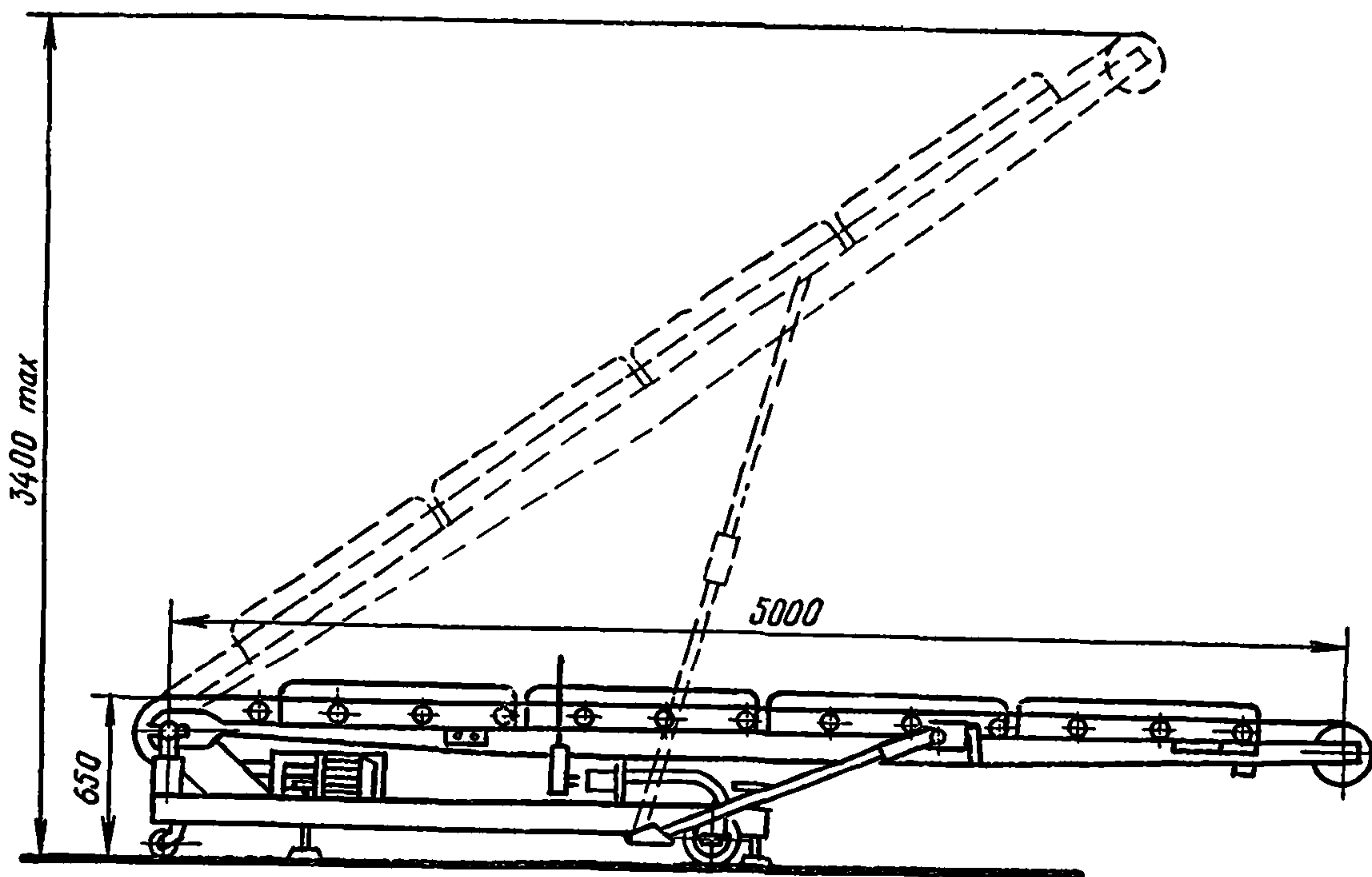
Рис. 25. Конвейер наклонный передвижной КНП-5
