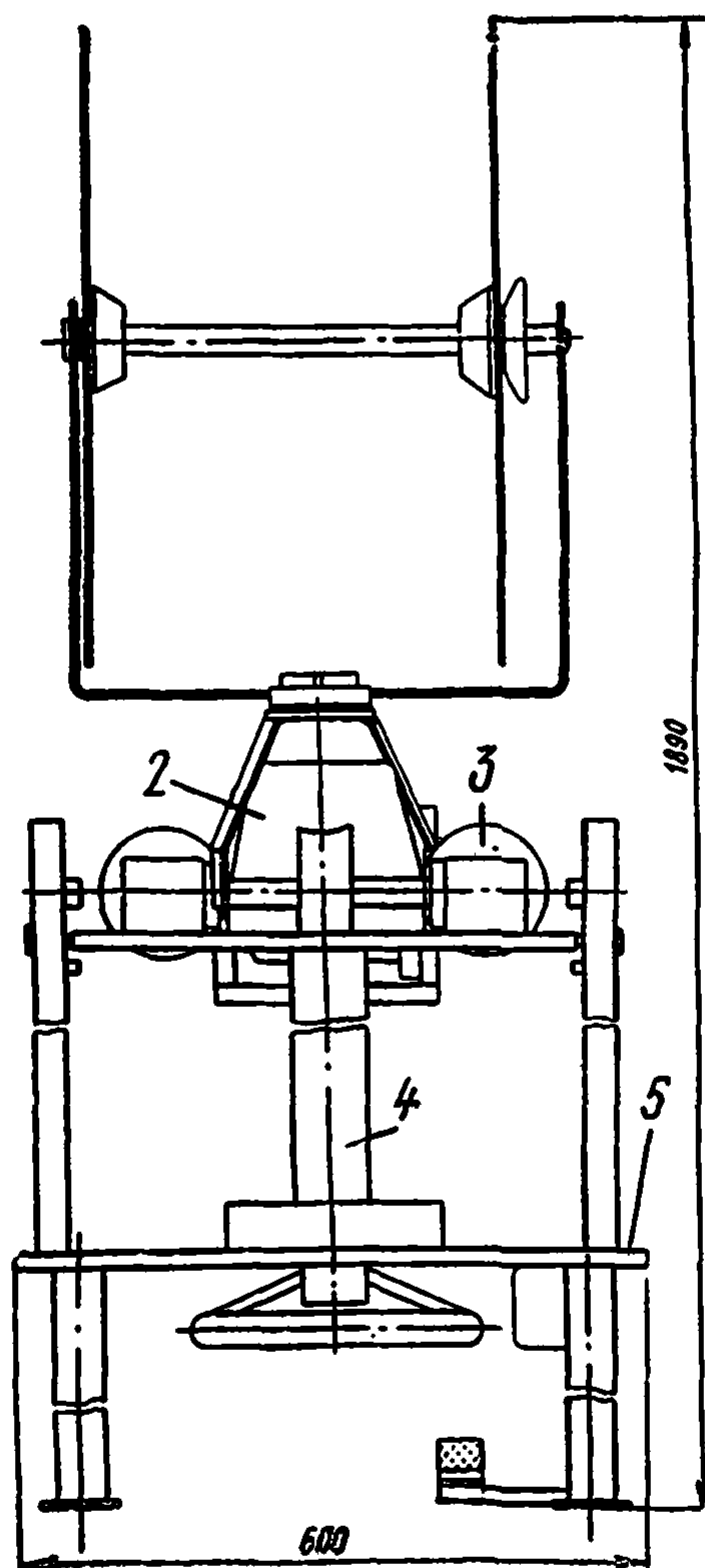
Рис. 54. Приспособление ПСП-3:
