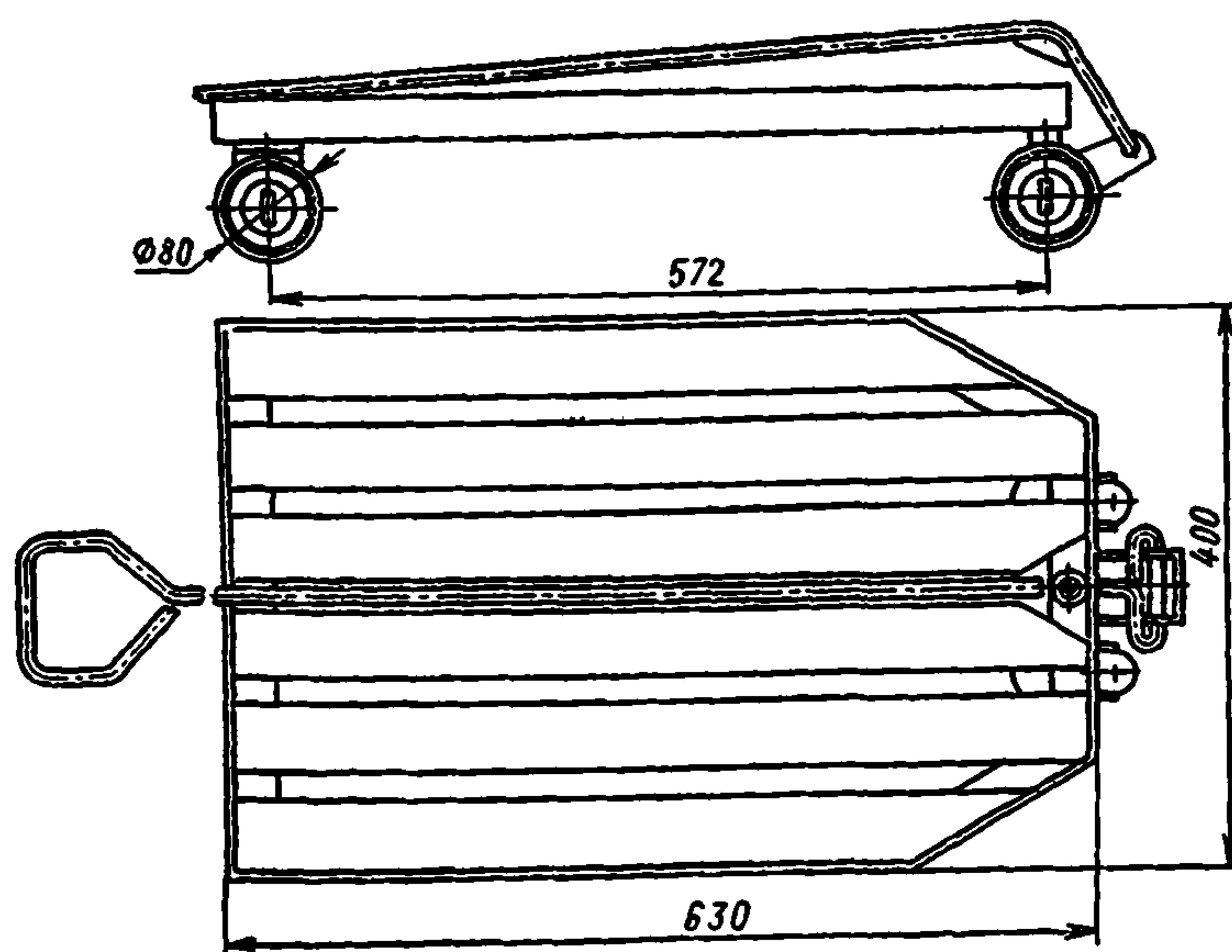
Рис. 37. Тележка ручная ТГ-50
