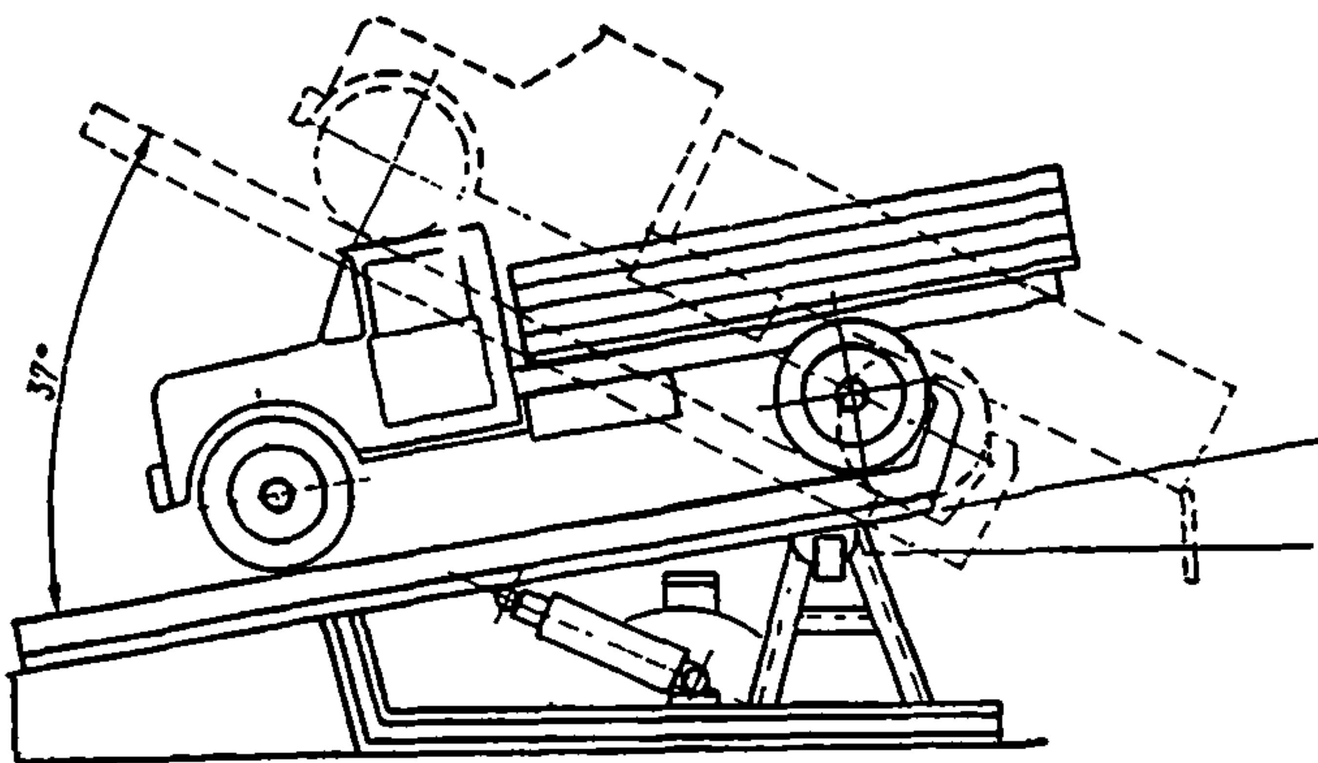
Рис. 9. Автомобилеразгрузчик ГАП-2Ц
