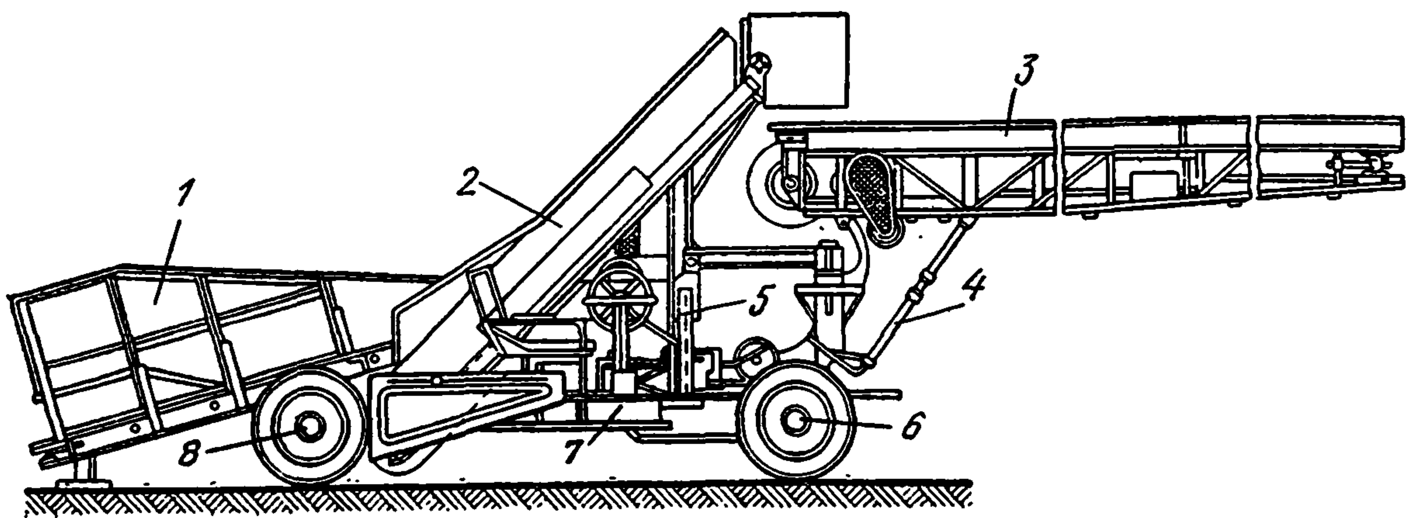
Рис. 18. Транспортер-эзгрузчик ТЗК-30;
