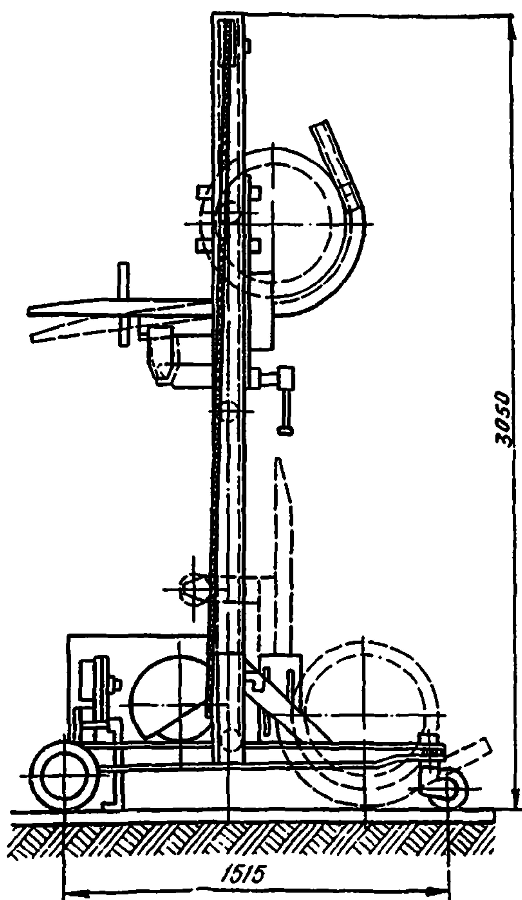
Рис. 28. Универсальный бочкоподъемник К-43216
