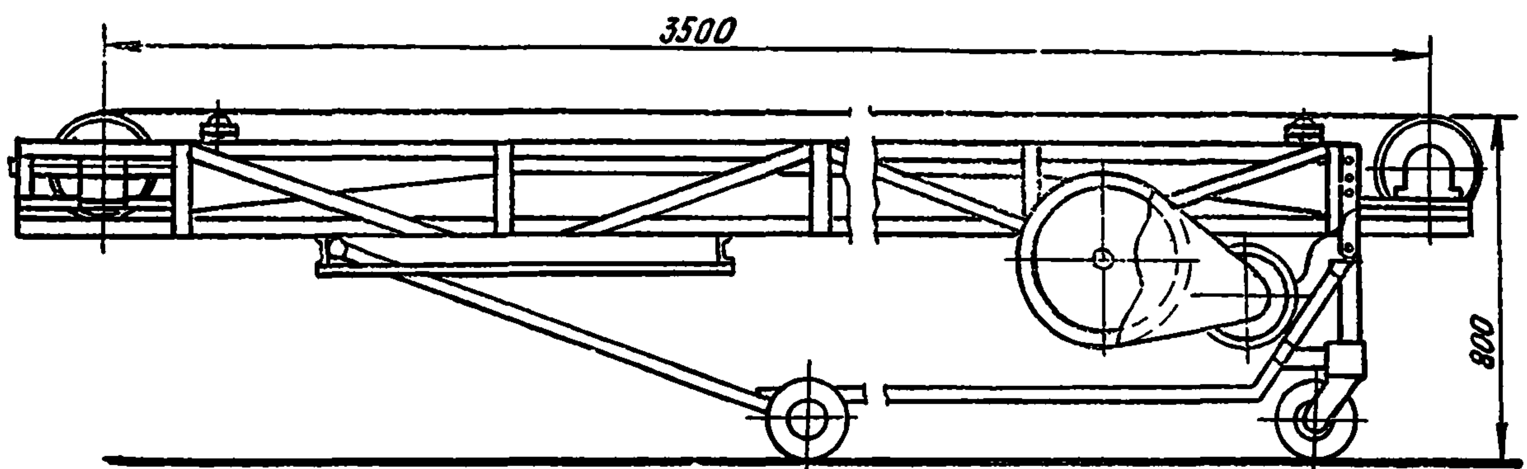
Рис. 17. Транспортер ленточный передвижной с переменным углом наклона ТПУ
