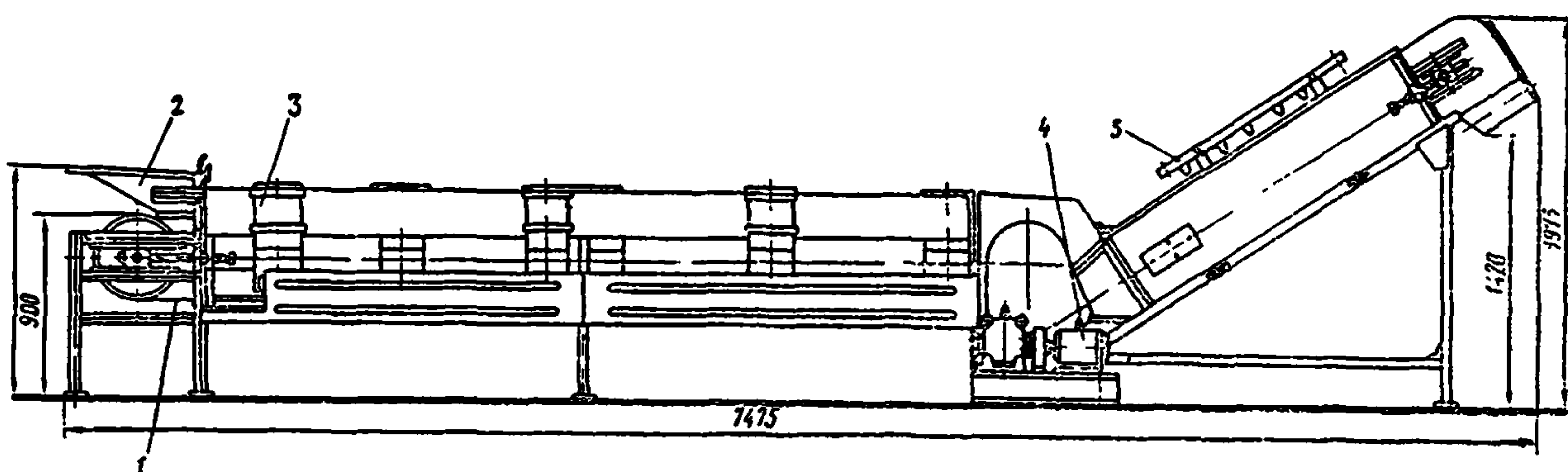
Рис. 48. Конвейер инспекционный ленточный Т1-КИ2Т:
