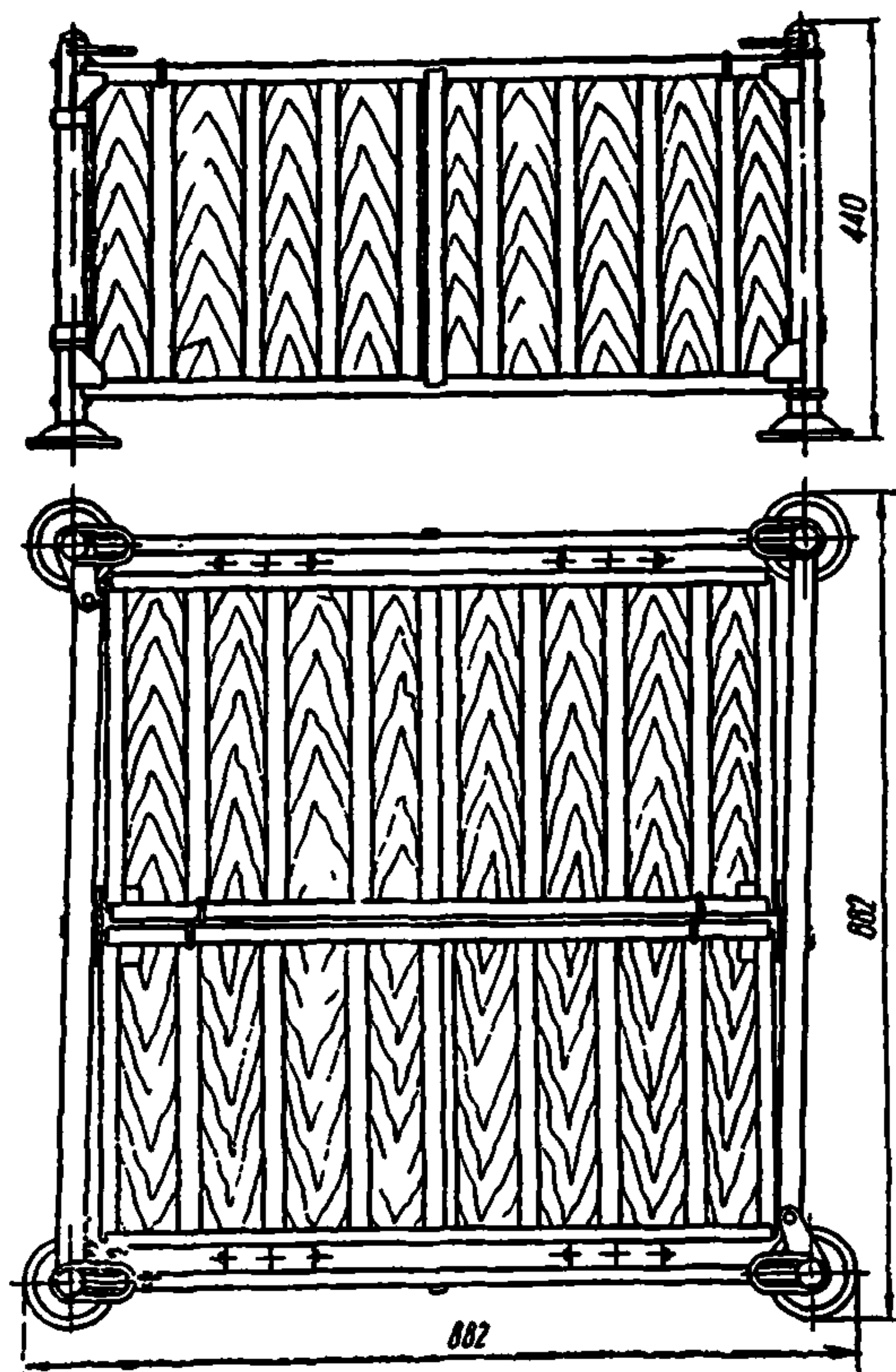
Рис. 30. Контейнер универсальный складной КУС-01/2
