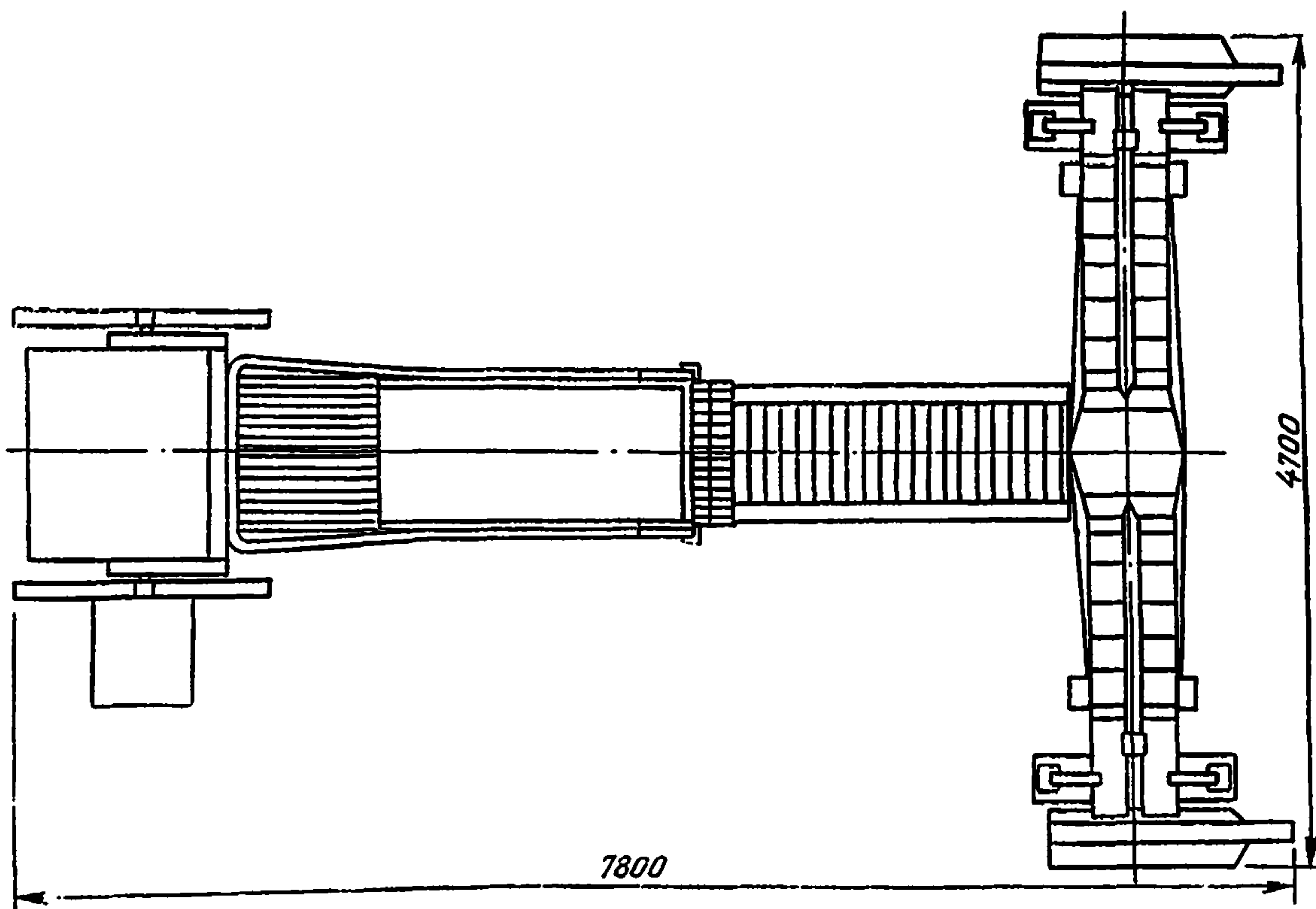
Рис. 56. Фасовочно-переборочная линия ФПЛ-2000
