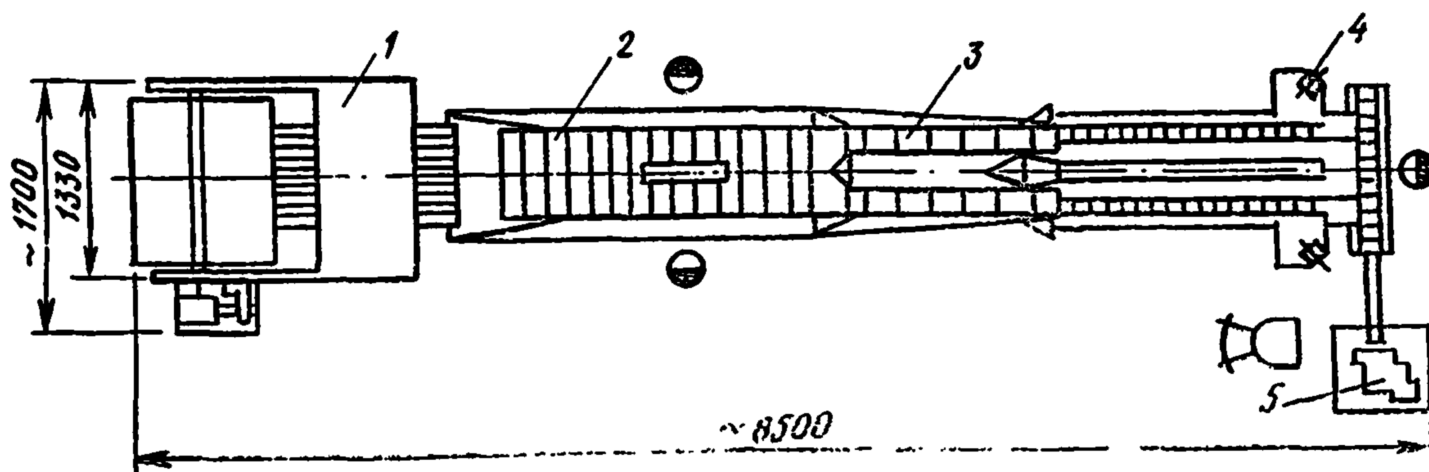
Рис. 57. Схема размещения оборудования линии товарной обработки и фасования картофеля ЛФК-1000В: 1 — контейнероопрокидыватель; 2 — переборочная машина; 3 — транспортер-питатель; 4 — весы полуавтоматические; 5 — упаковочная машина
