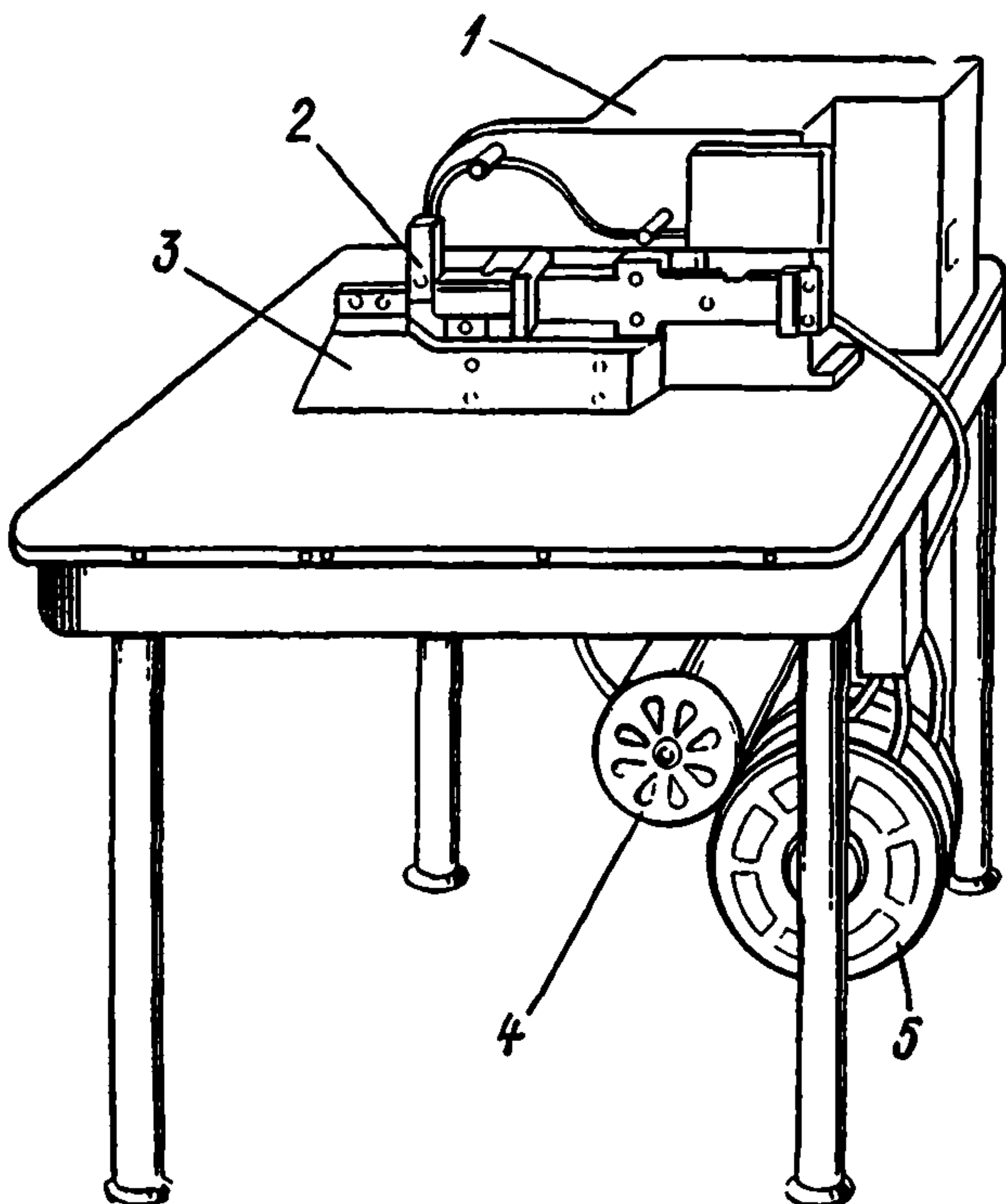
Рис. 53. Машина для упаковки овощей и фруктов МУ:
