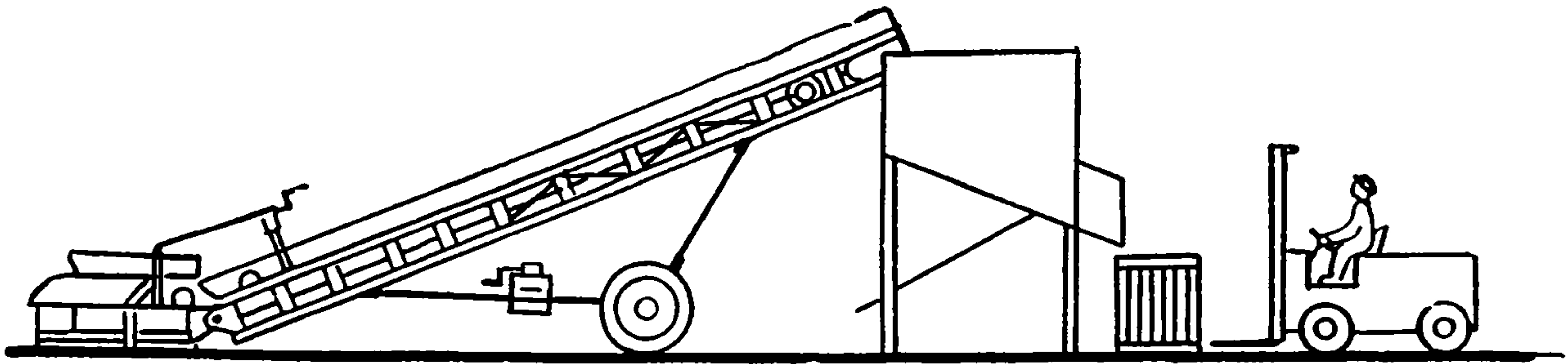
Рис. 21. Схема организации загрузки контейнеров с использованием ТПЛ-30
