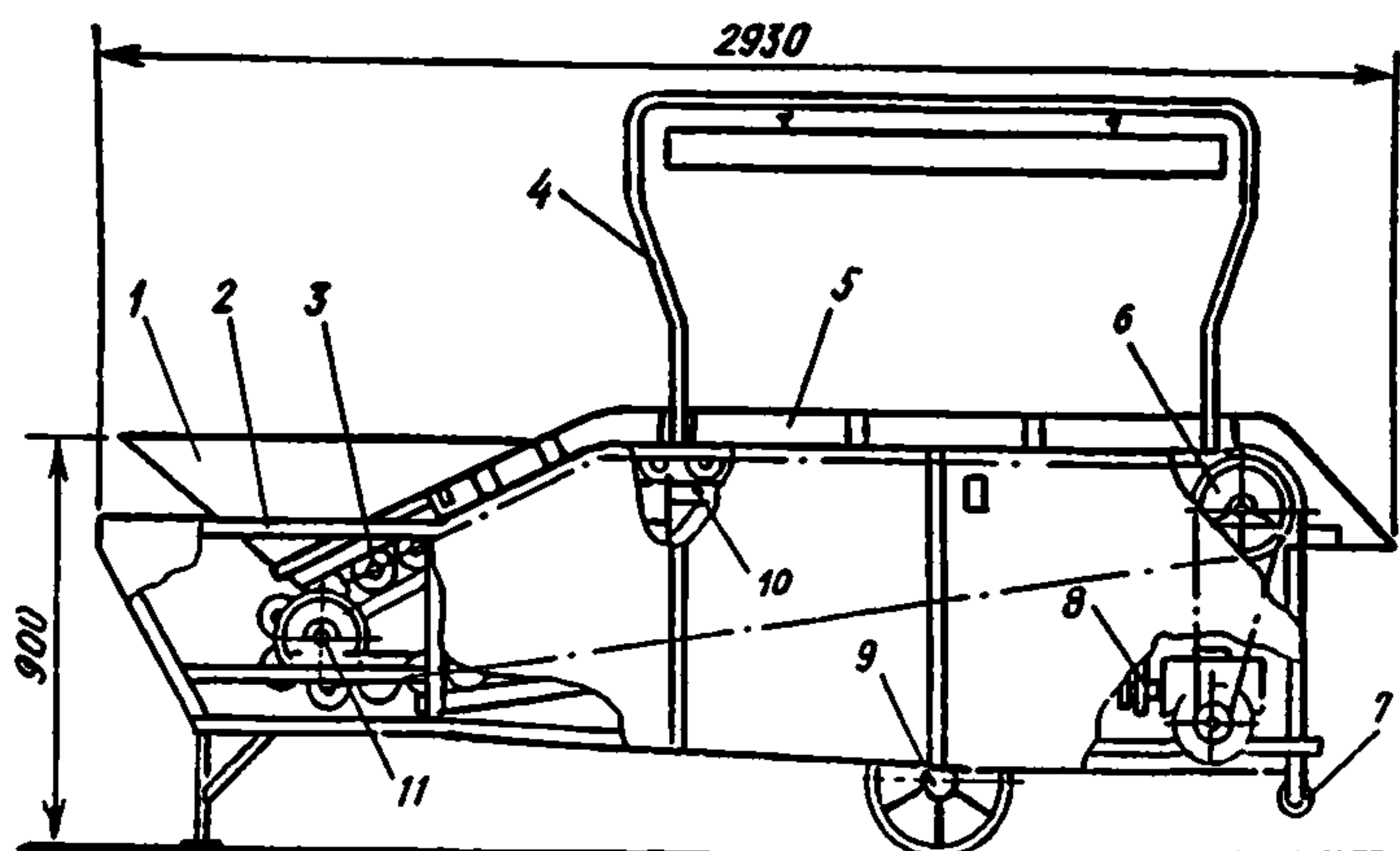
Рис. 45. Машина для переборки картофеля МПК-2:
