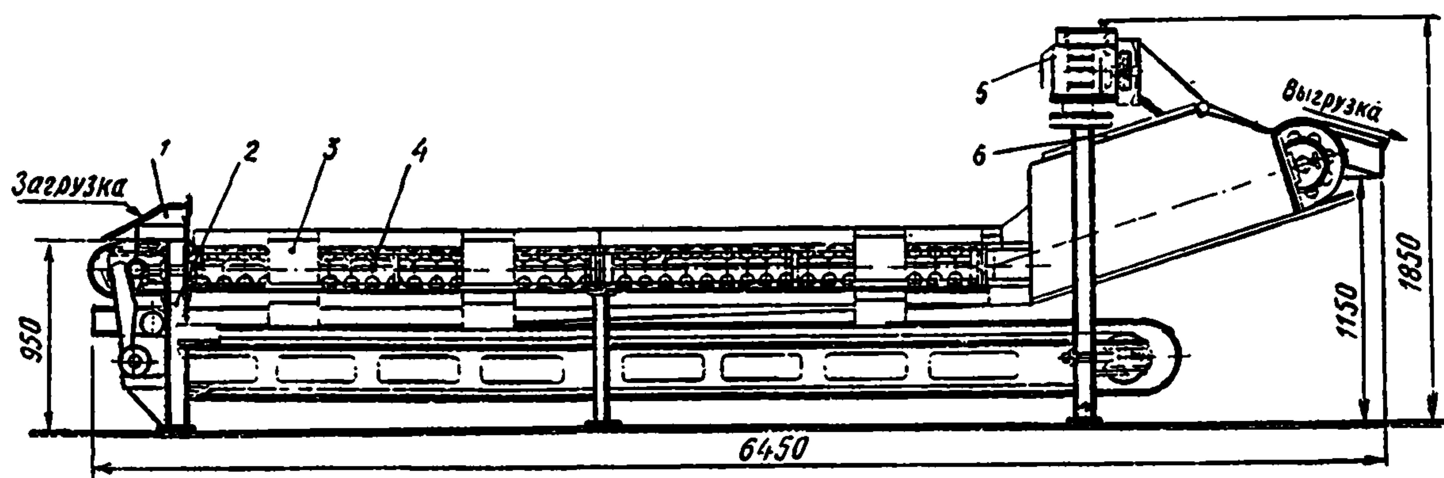
Рис. 47. Конвейер инспекционный роликовый Т1-КТ2В:
