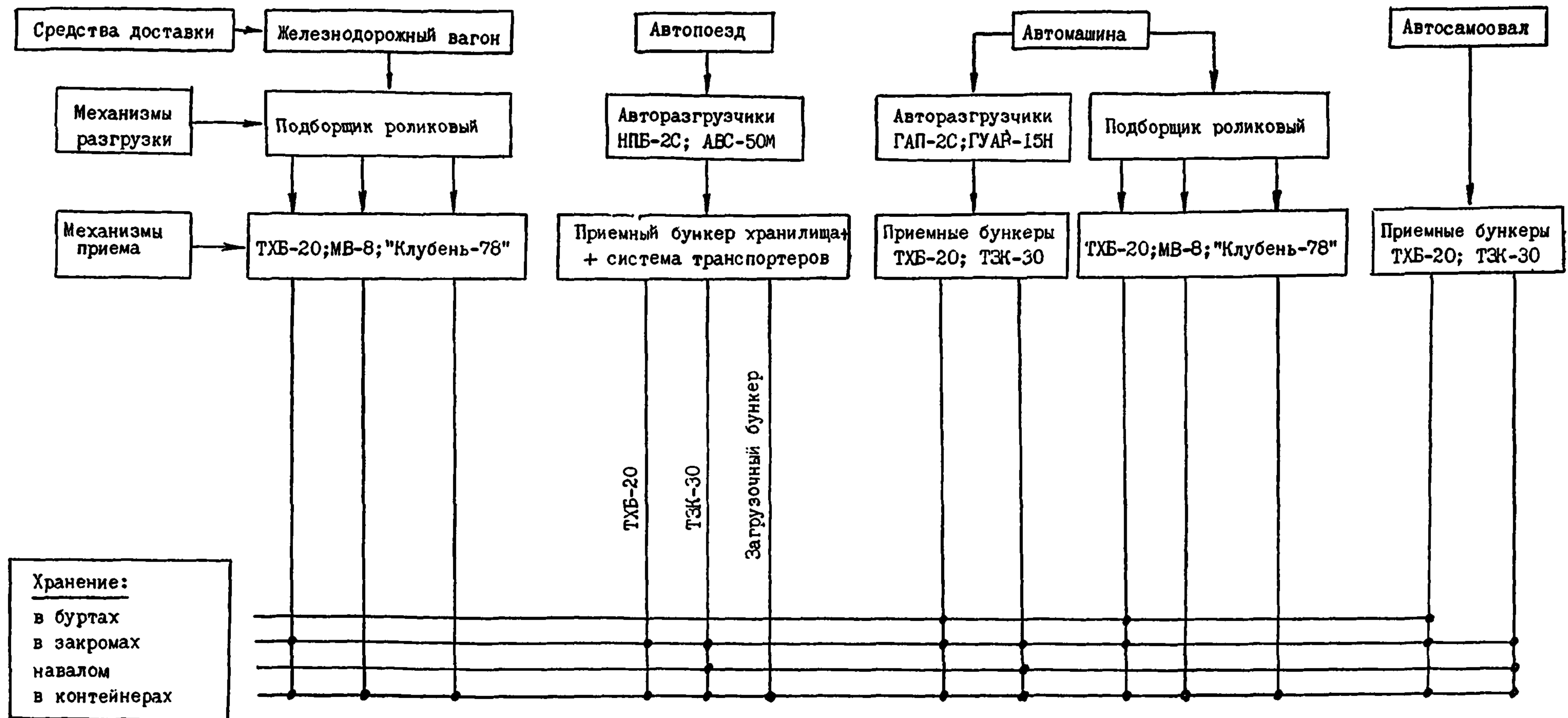
Рис. 20. Схема применения машин и механизмов для выгрузки навалочной продукции из различных видов транспорта и обеспечения способов хранения
