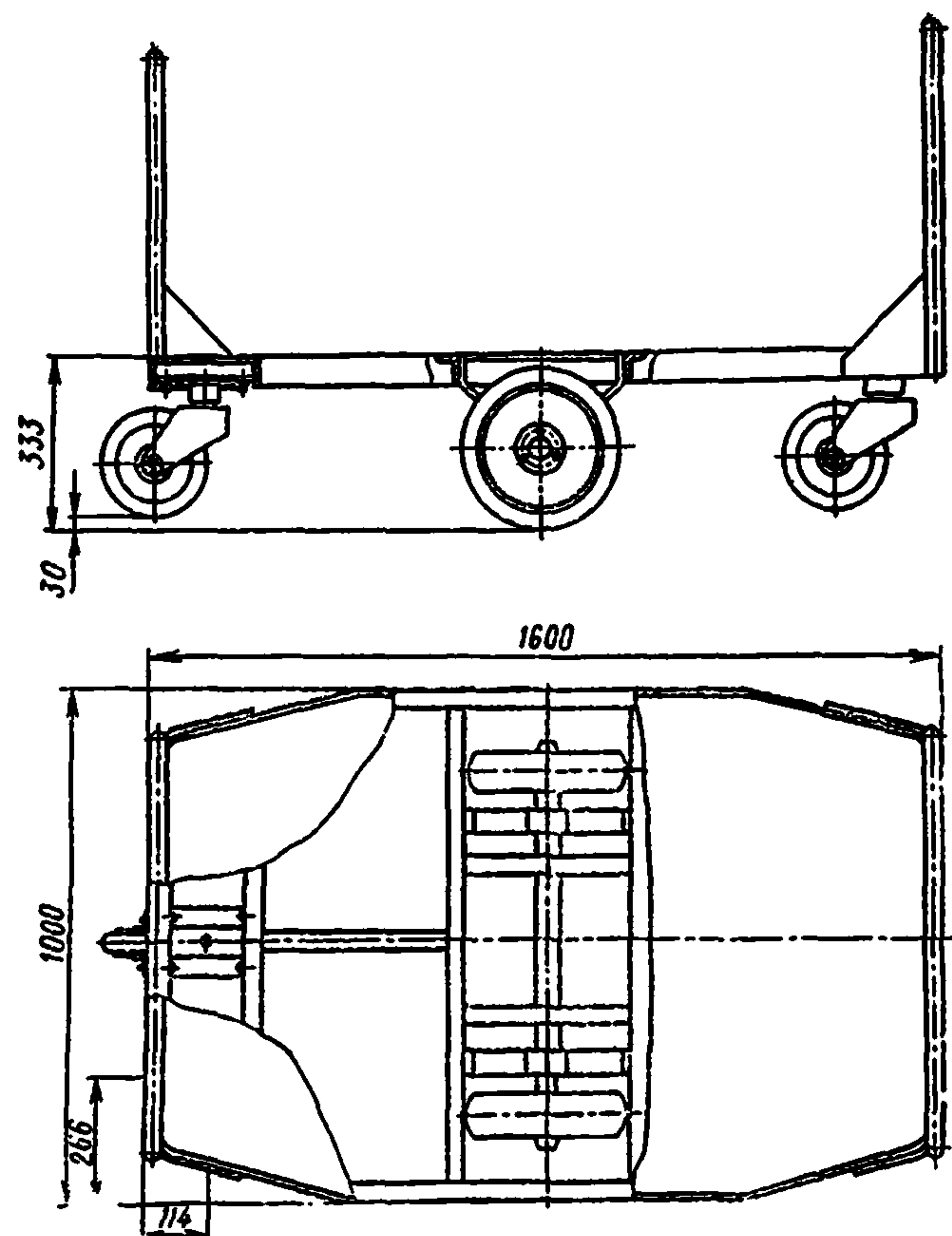
Рис. 40. Тележка ручная ТГМ-1000 М
