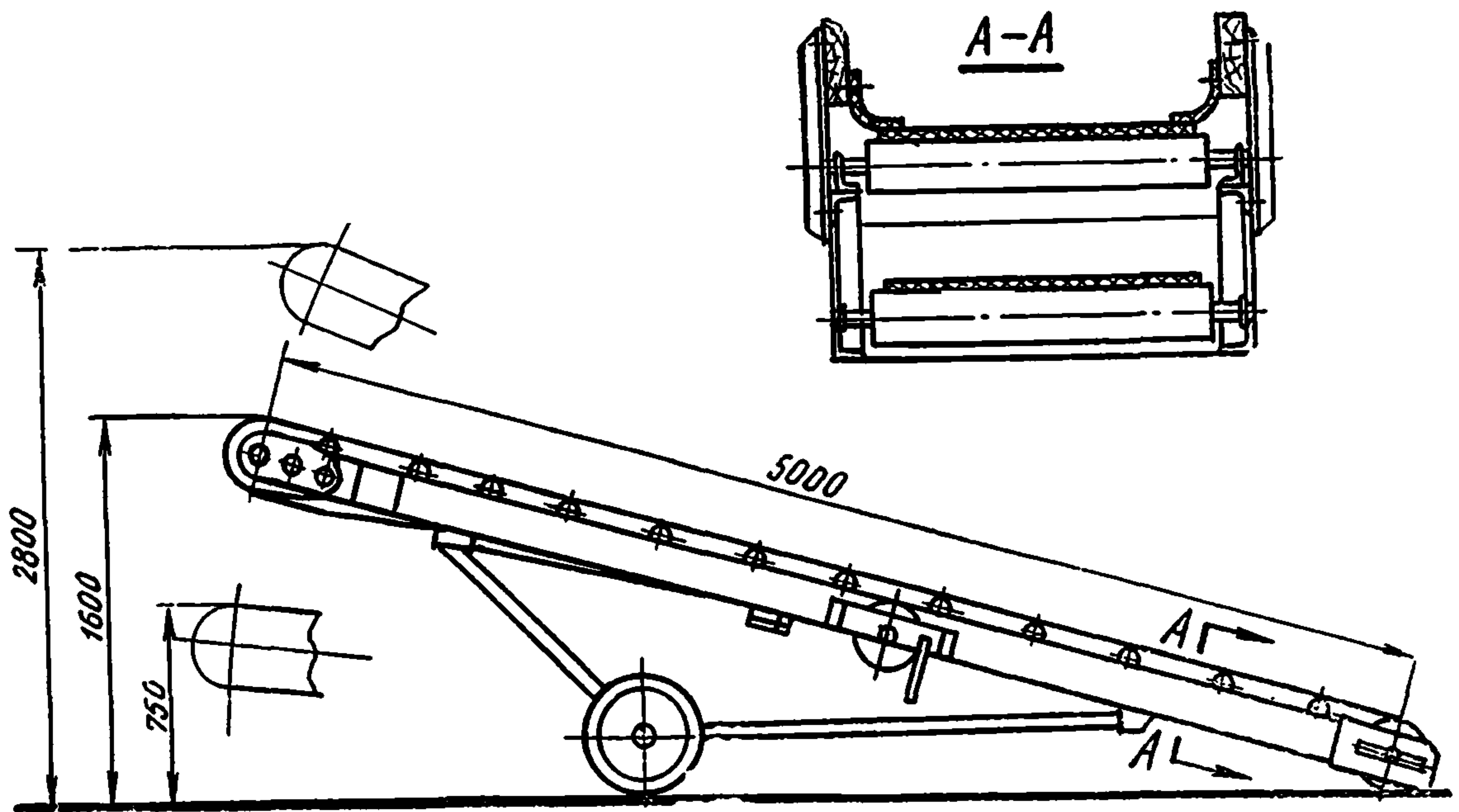
Рис. 16. Транспортер ленточный ЦТ-76
