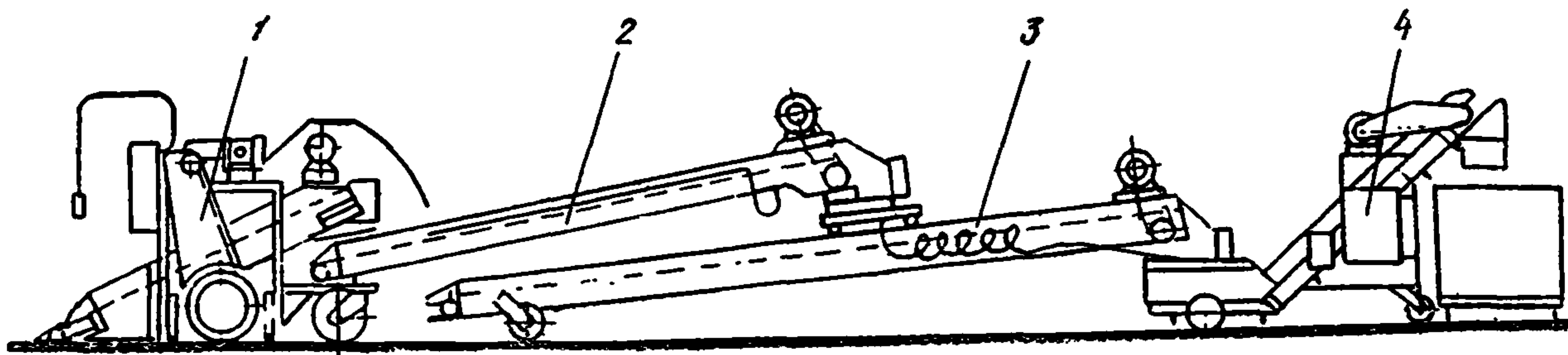
Рис. 2. Комплект механизмов МВ-8:
