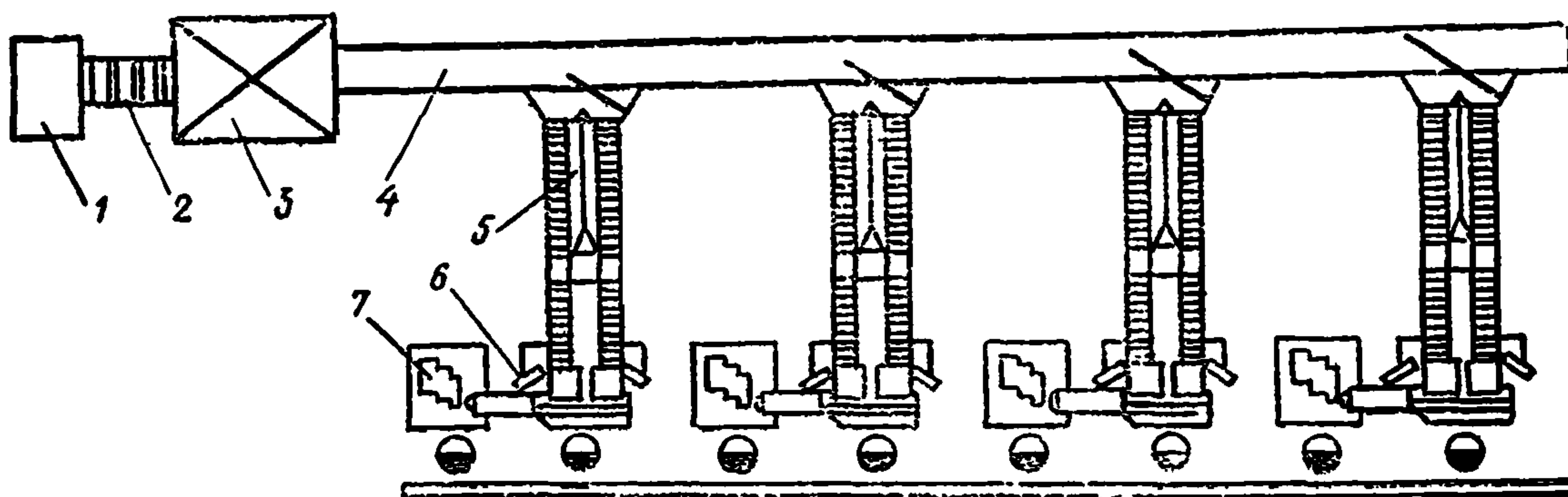
Рис. 58. Схема размещения оборудования фасовочной линии производительностью 24—25 т/смену: 1 — контейнероопрокидыватель; 2 — переборочная машина; 3 — бункер; 4 — распределительный транспортер; 5 — транспортер-питатель; 6 — весы полуавтоматические; 7 — упаковочная машина
