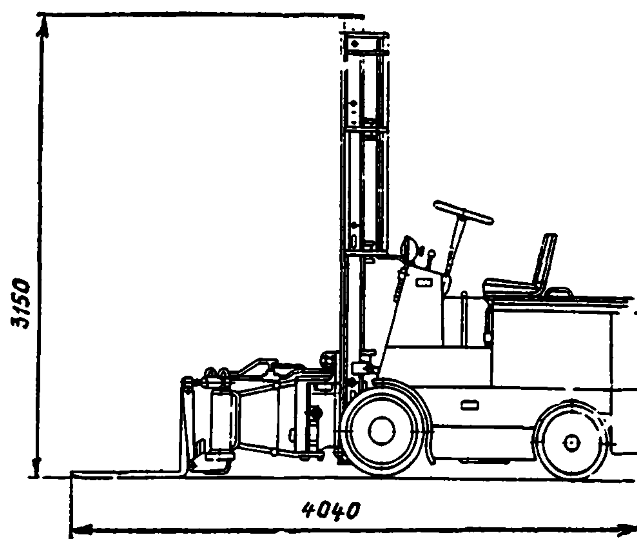
Рис. 36. Электропогрузчик ЭП-201 (205)
