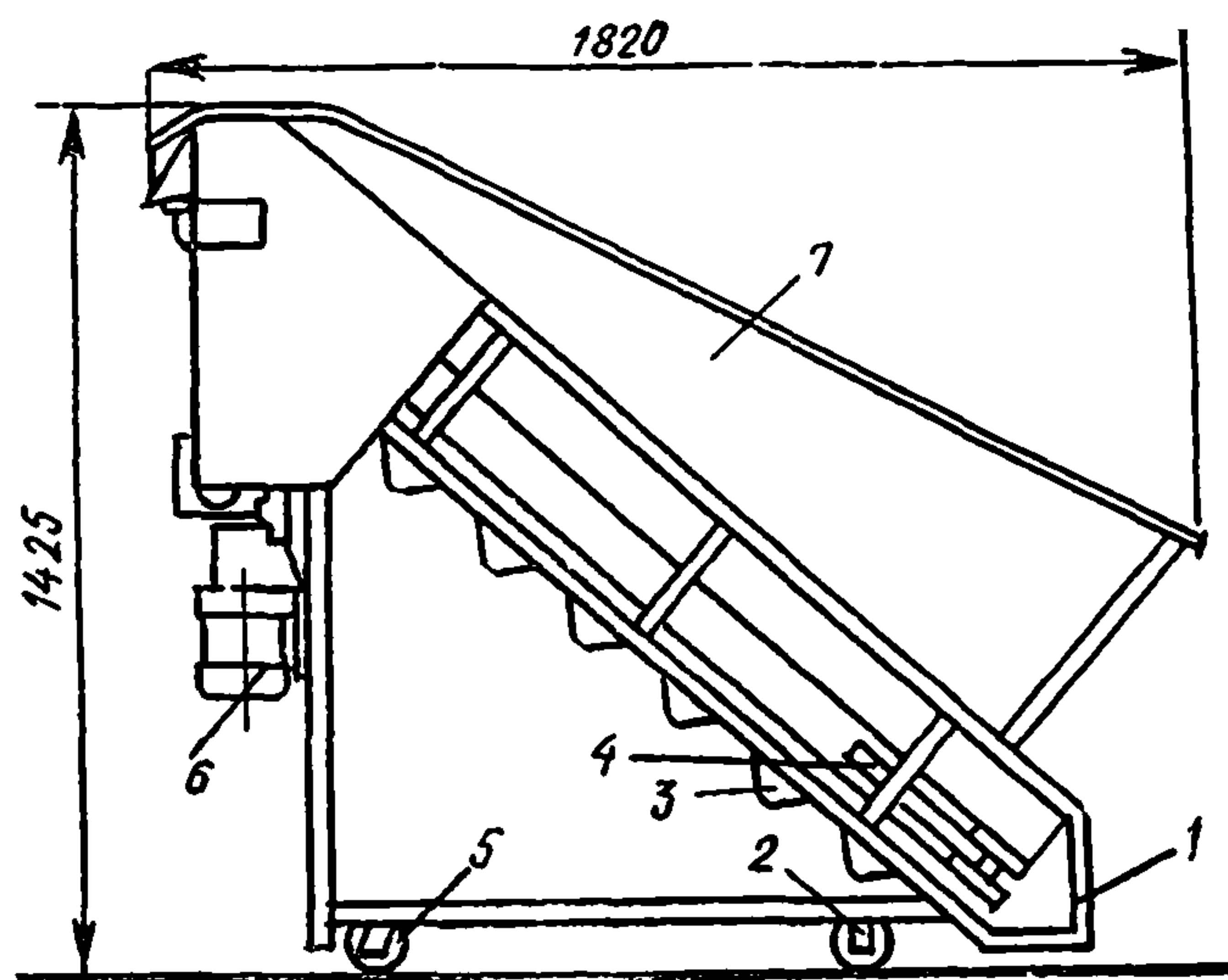
Рис. 52. Транспортер-питатель ЛФК-9
