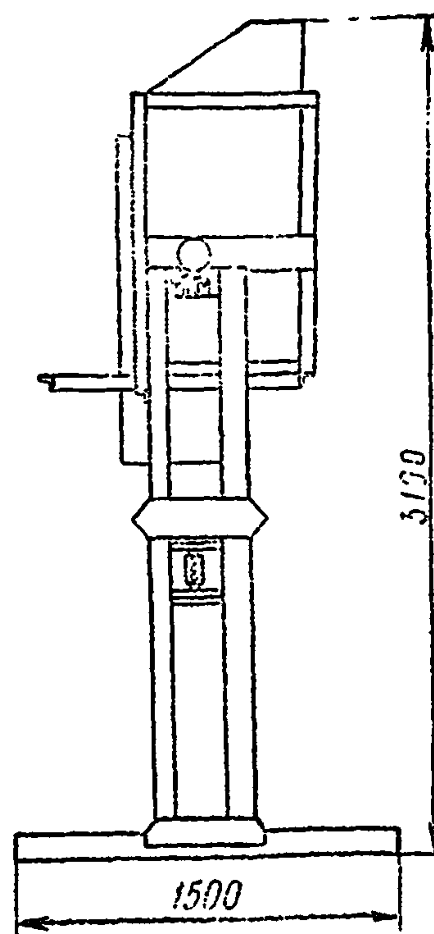
Рис. 43. Контейнероопрокидыватель КО-8
