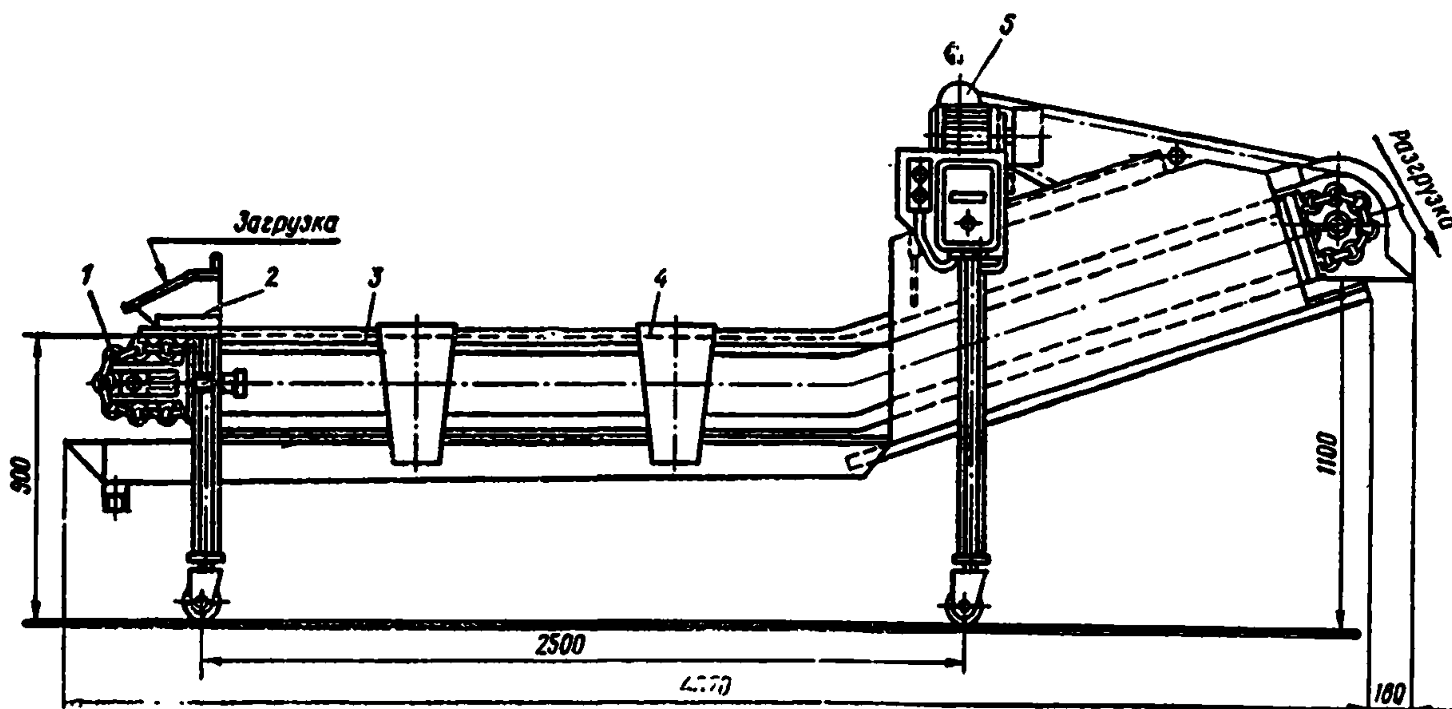
Рис. 46. Транспортер инспекционный роликовый КТО:
