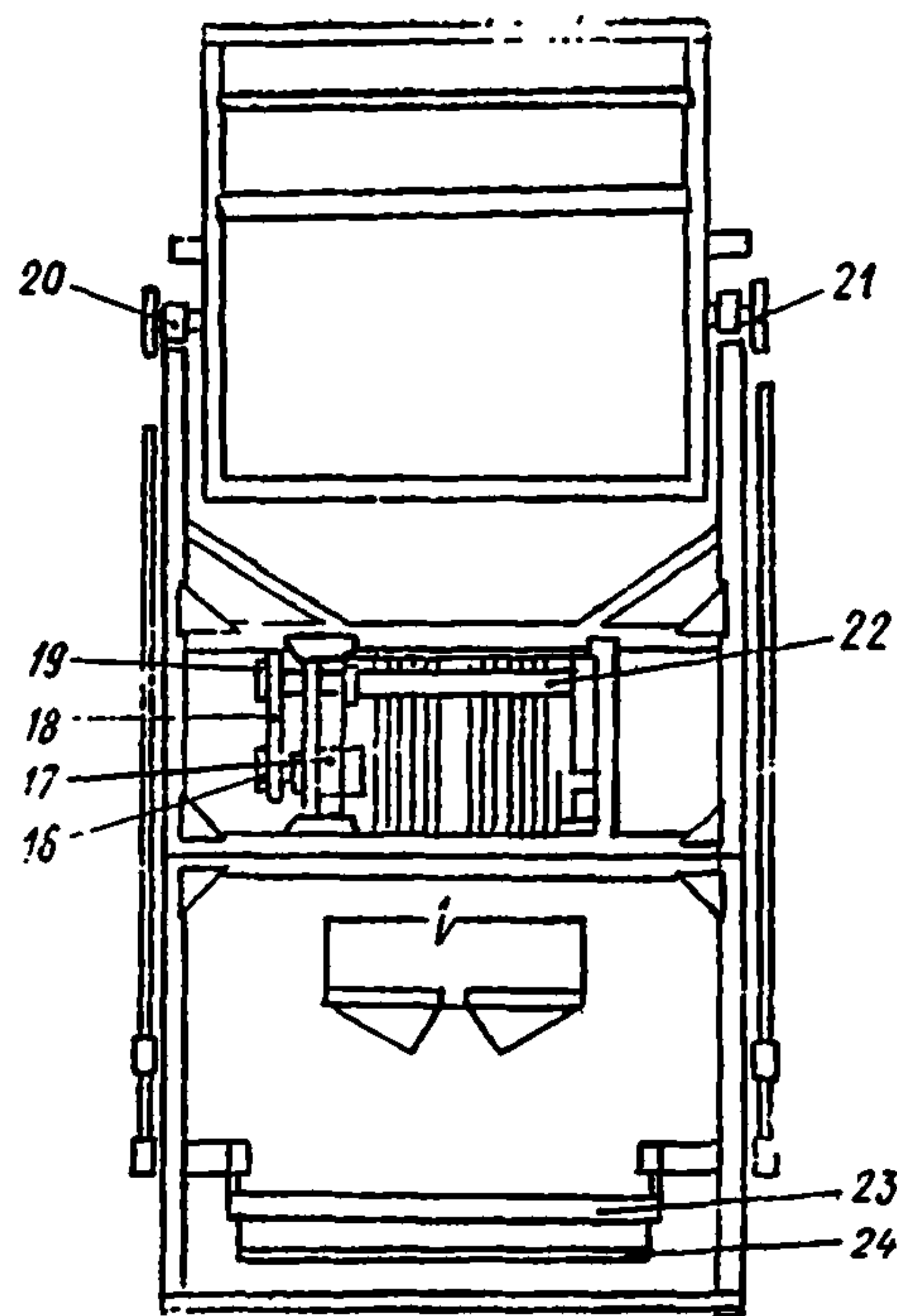
Рис. 44. Контейнероопрокидыватель КУП-1000:
