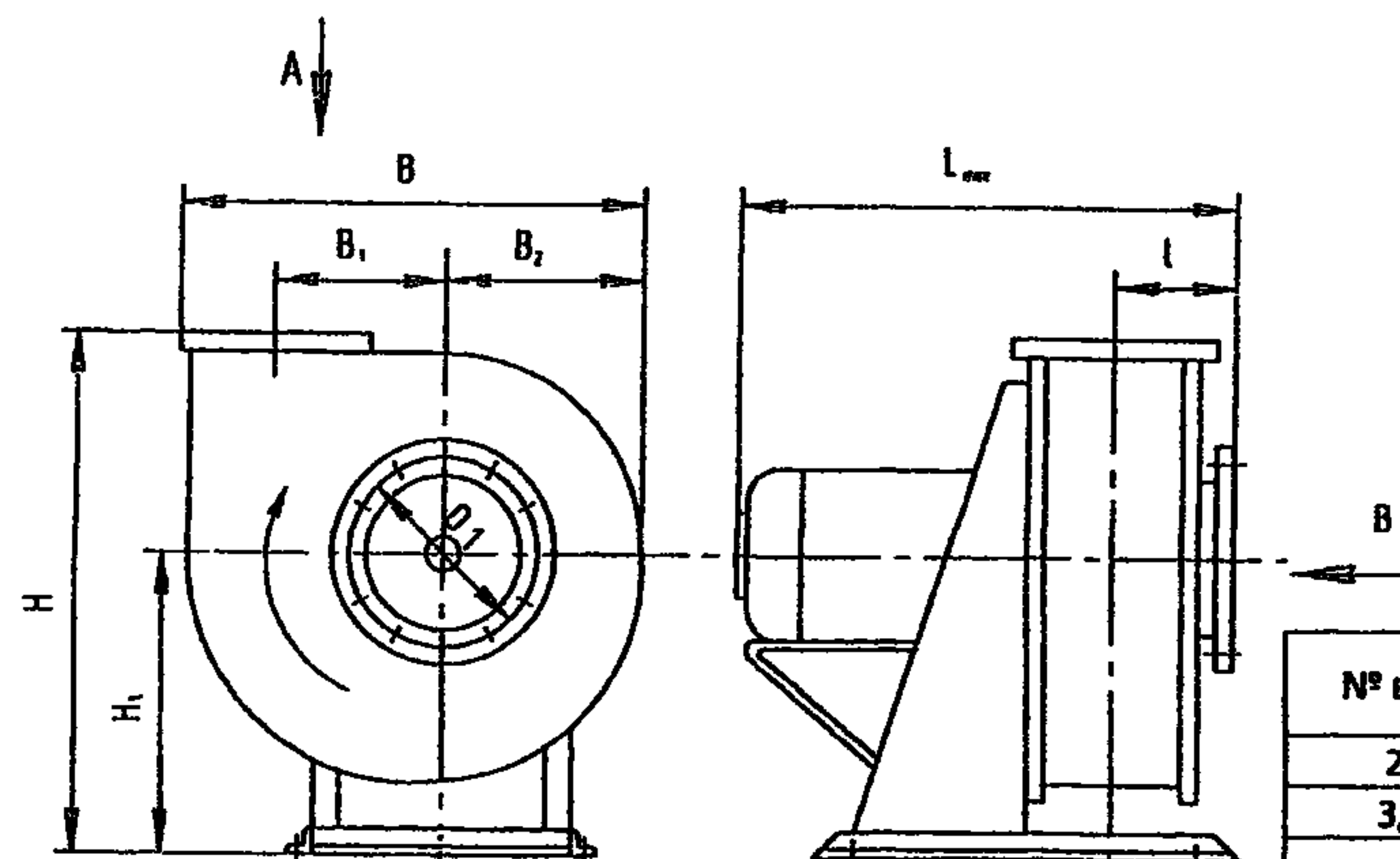
Вентиляторы низ. дав. ВР80-75 (ВЦ4-75), и. 1
