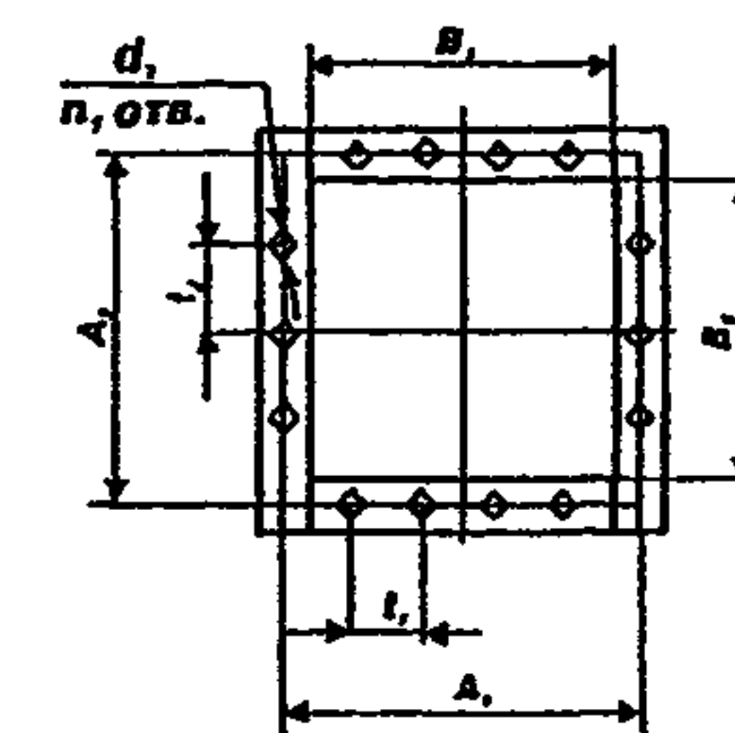
Фланец выходной
