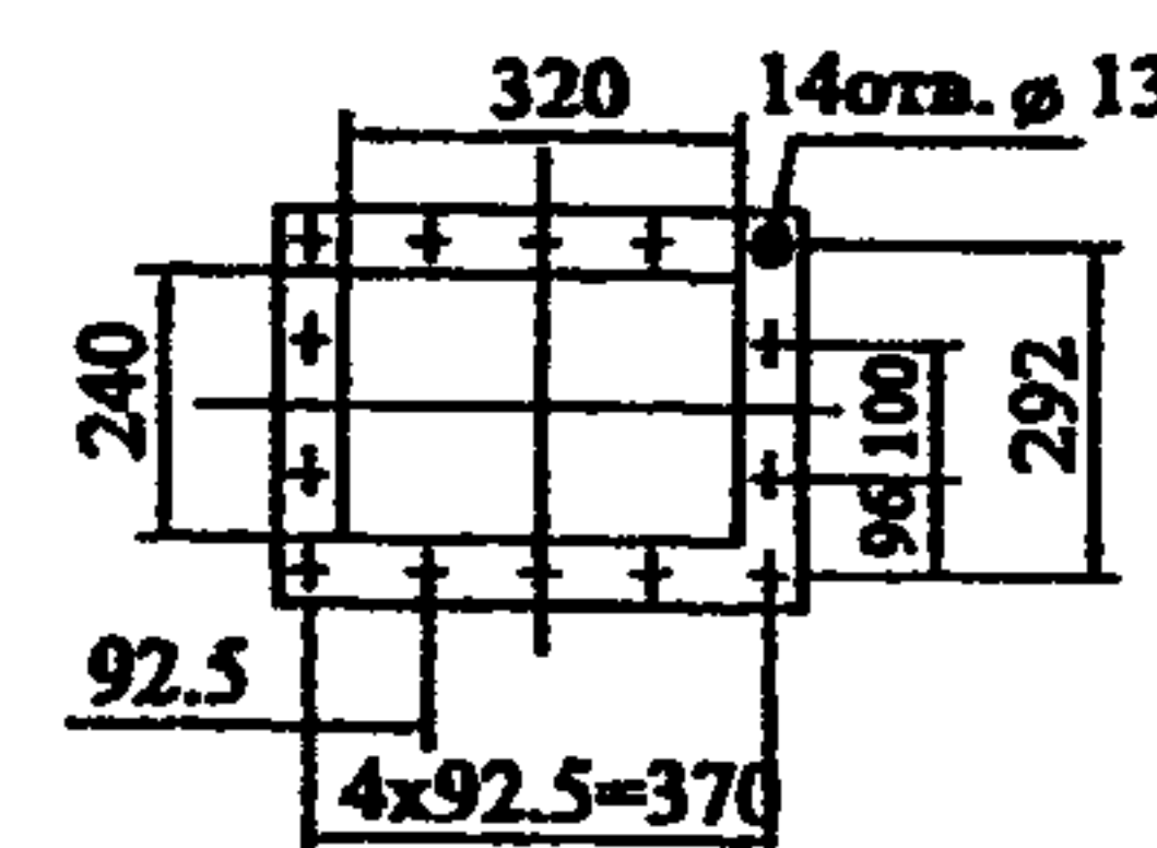
Выходной фланец
