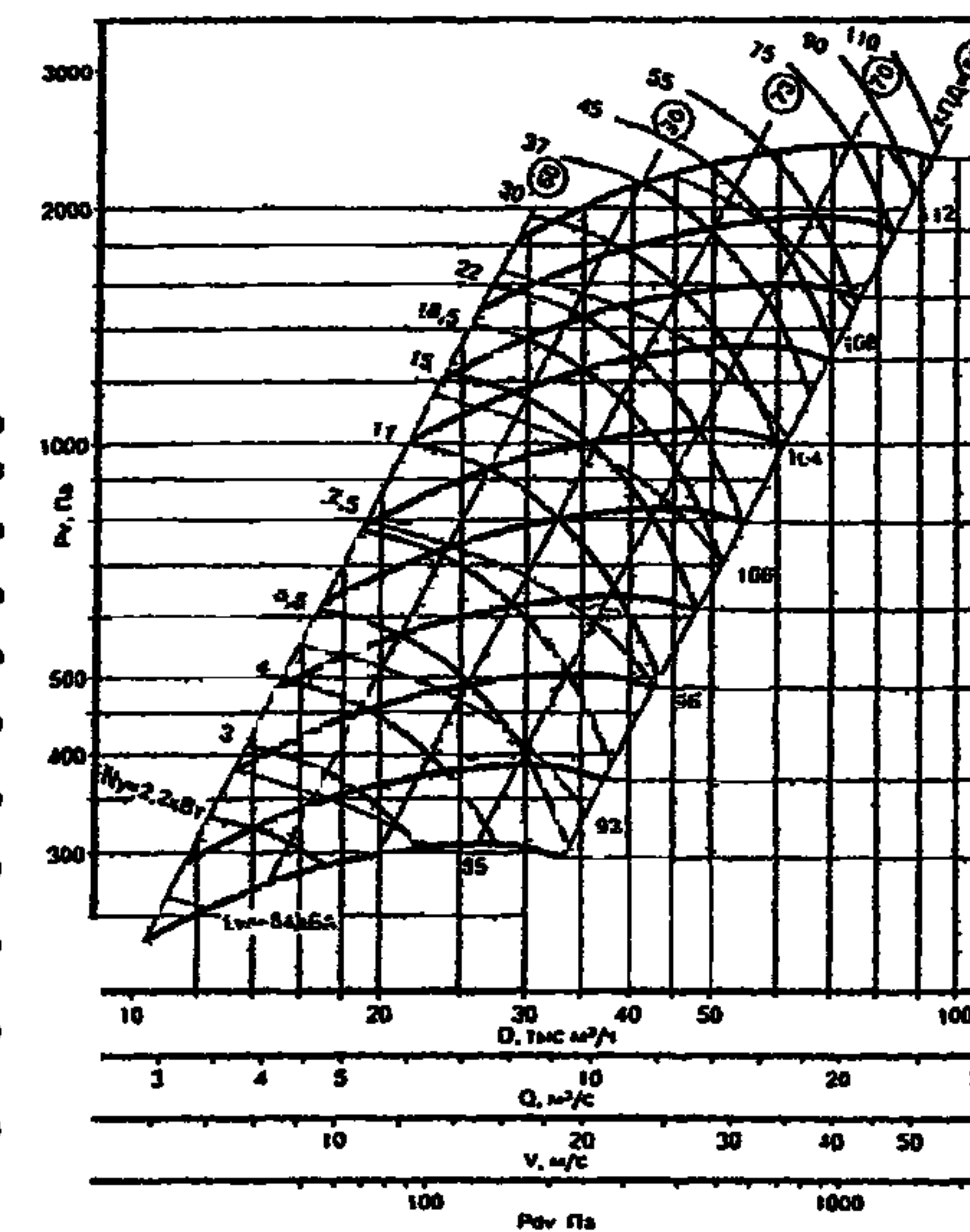
ВЦ 14-46-10 исполнение 5
