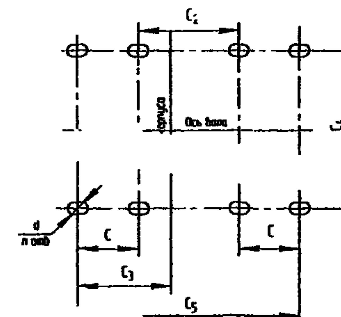
№ 8 - № 10
