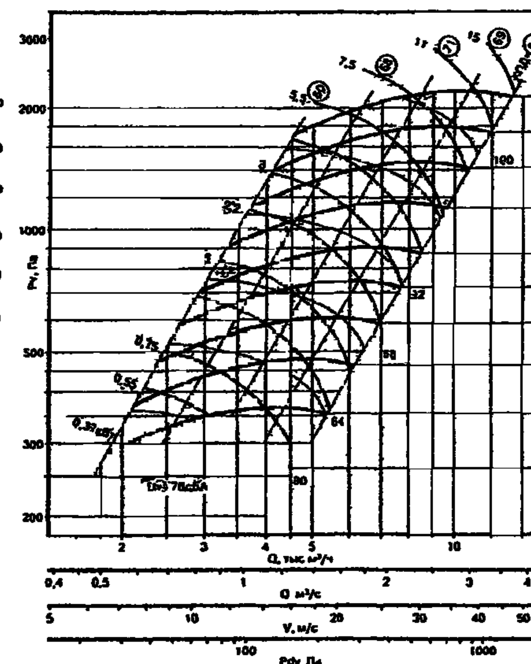
ВЦ 14-46-4 исполнение 5
