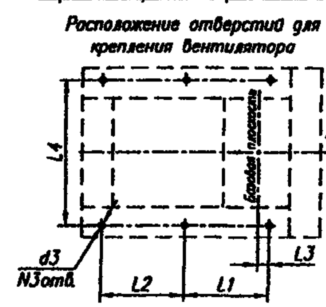
Вентилятор типа ВР 132-30 (исполнение 1).
