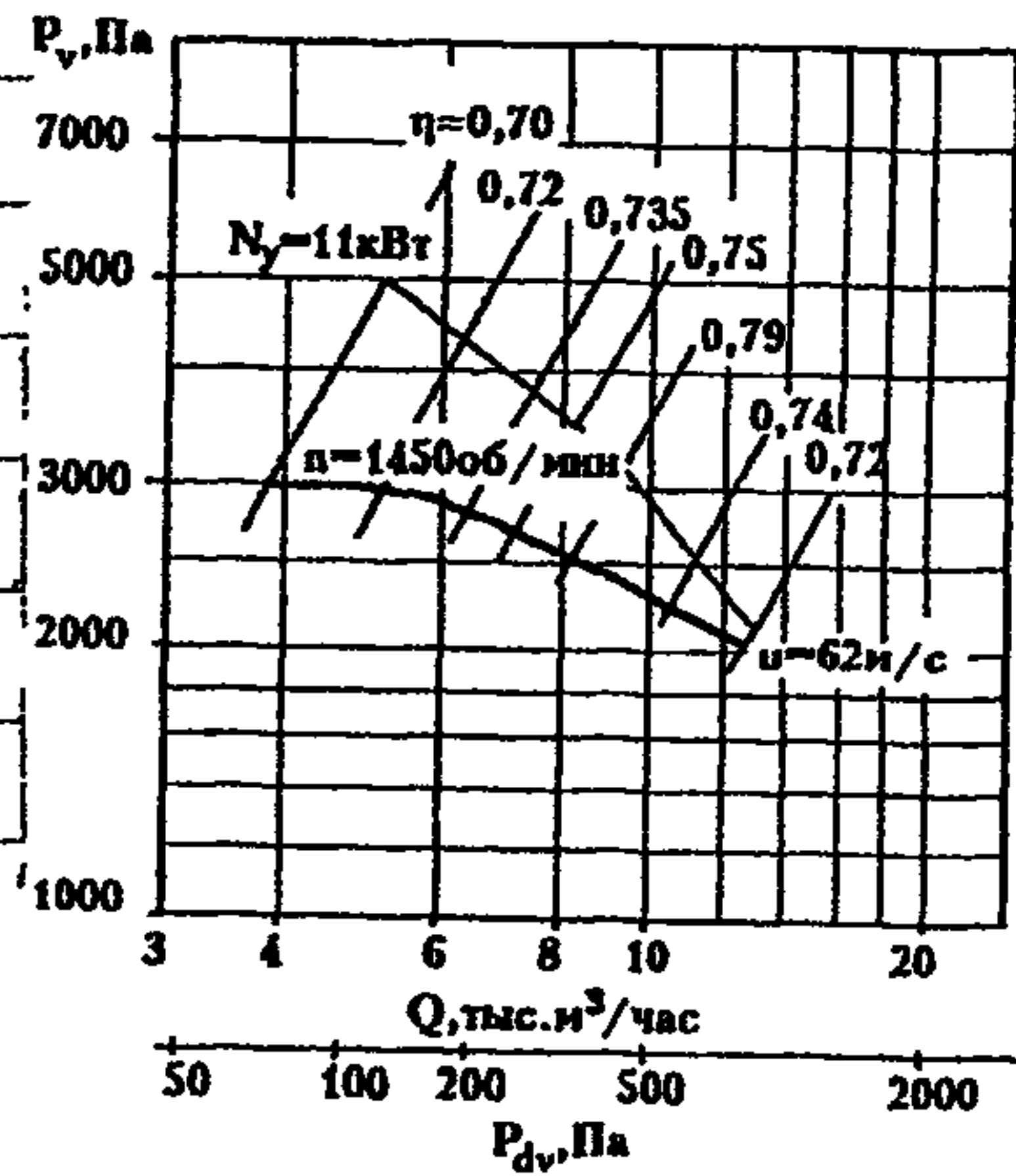
В.Ц5-35-8.01
