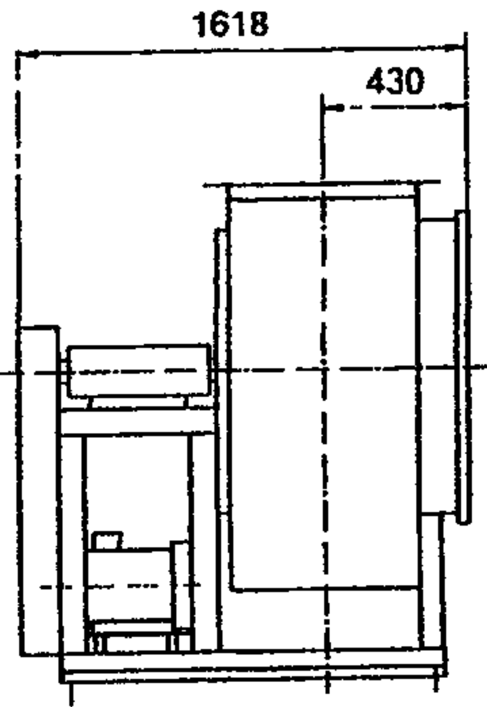
ВР-80-70-12.5-01
