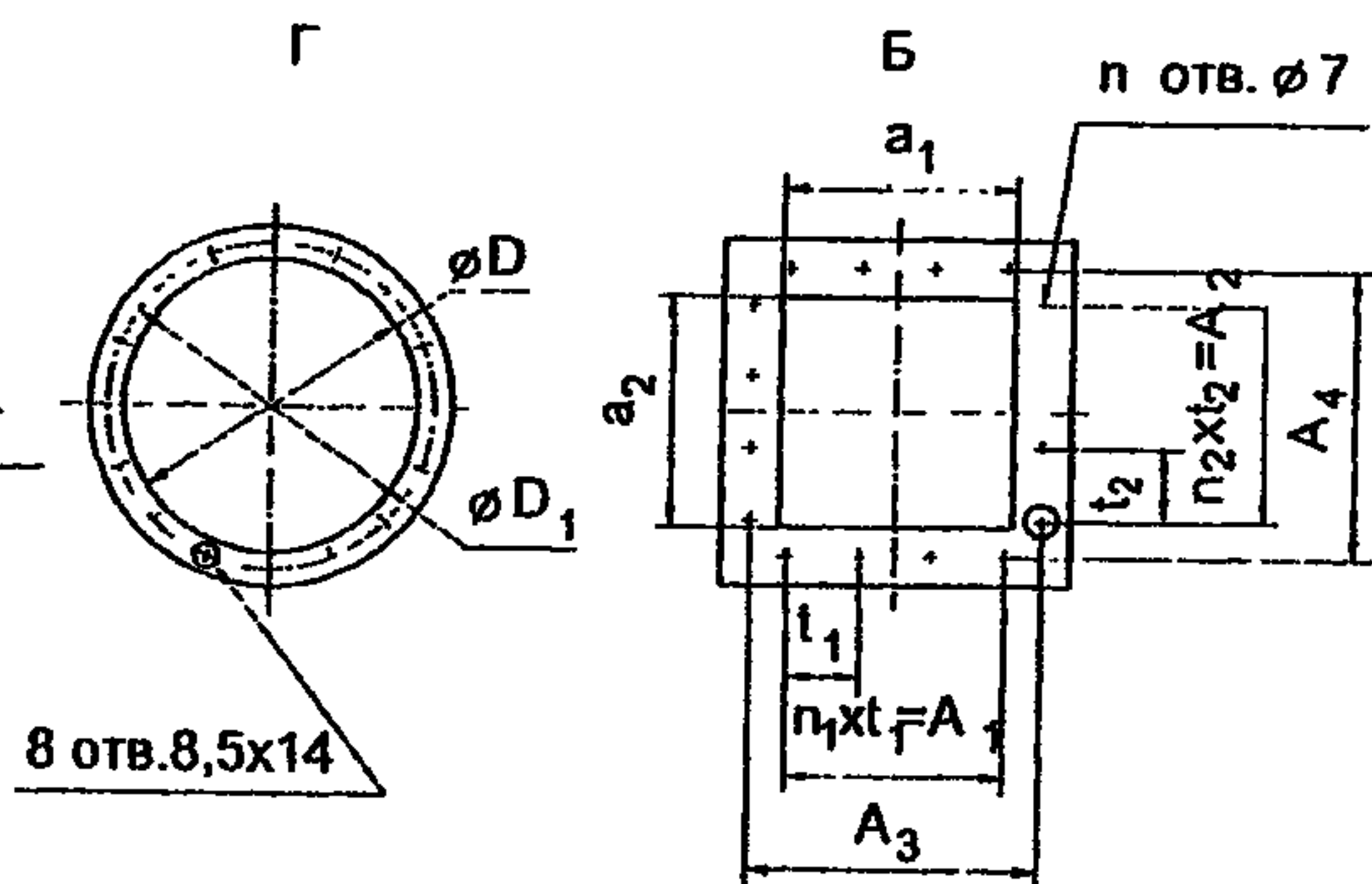
Расположение отверстий для крепления вентилятора ВР-300-45-2,5; -3,15; -4
