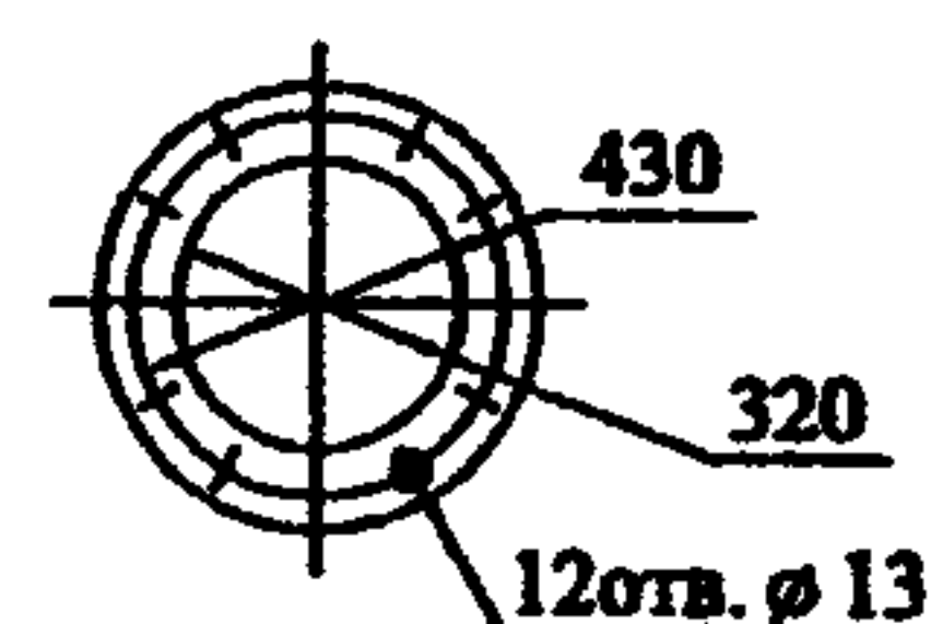
Входной фланец
