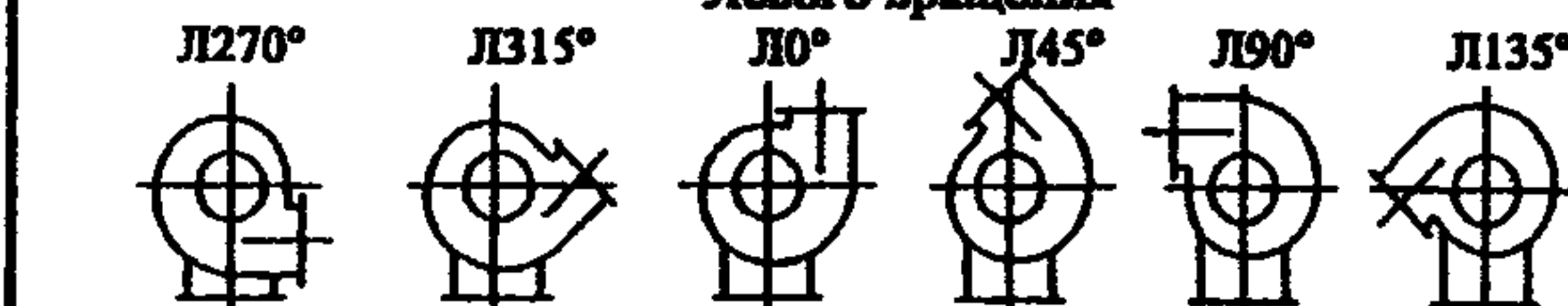
Левого вращения
