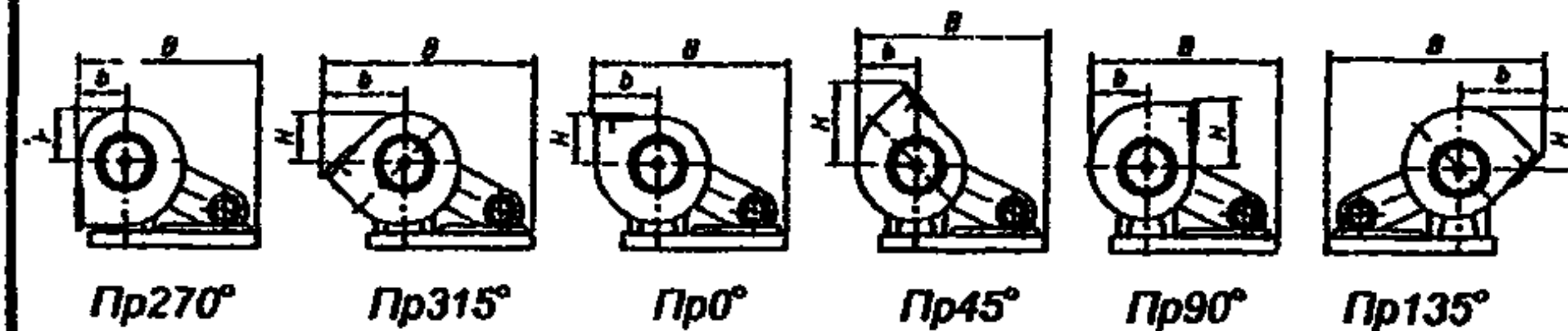
Вентилятор типа ВР 132-30 (исполнение 5).
