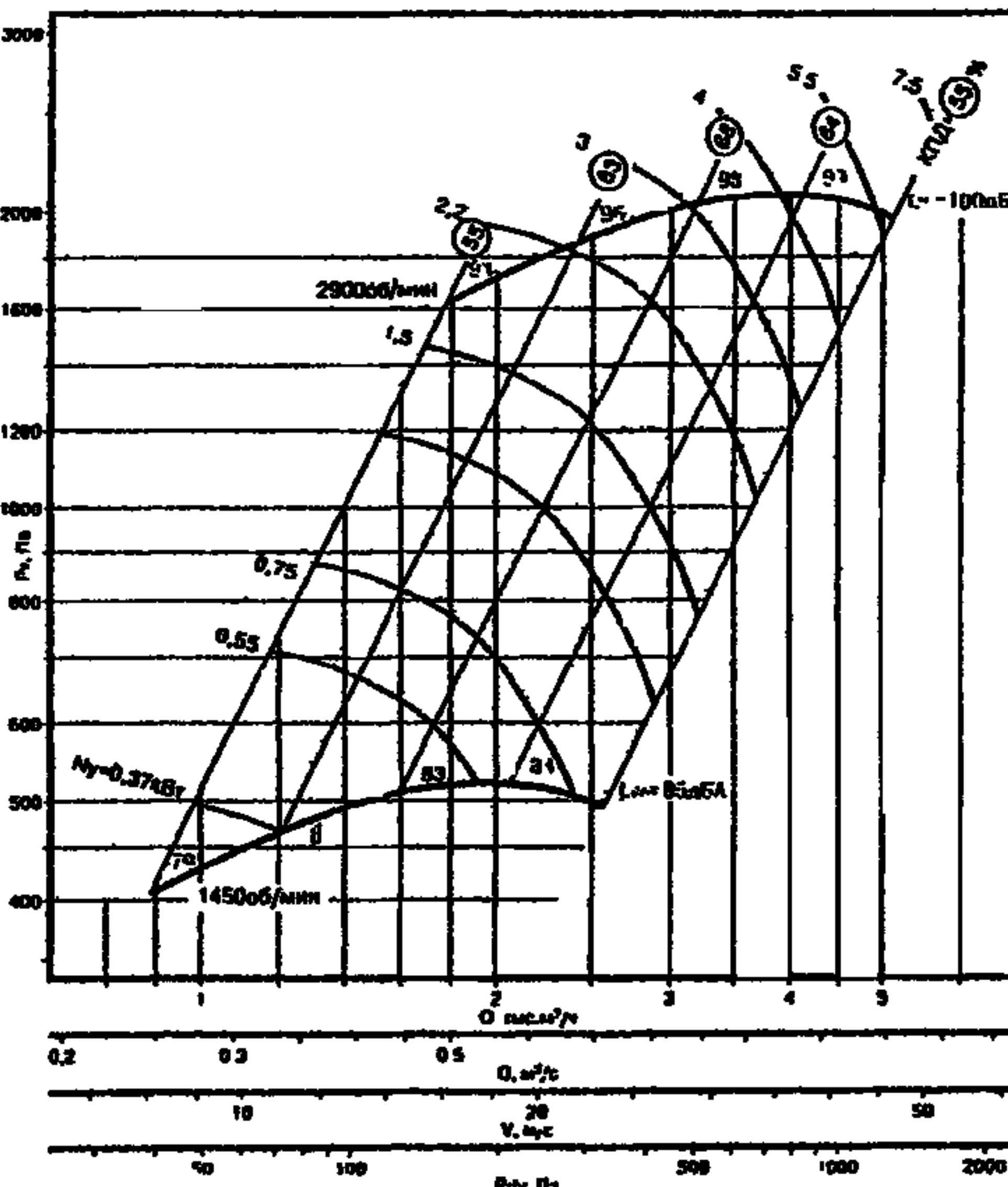
ВЦ 14-46-2,5 исполнение 1
