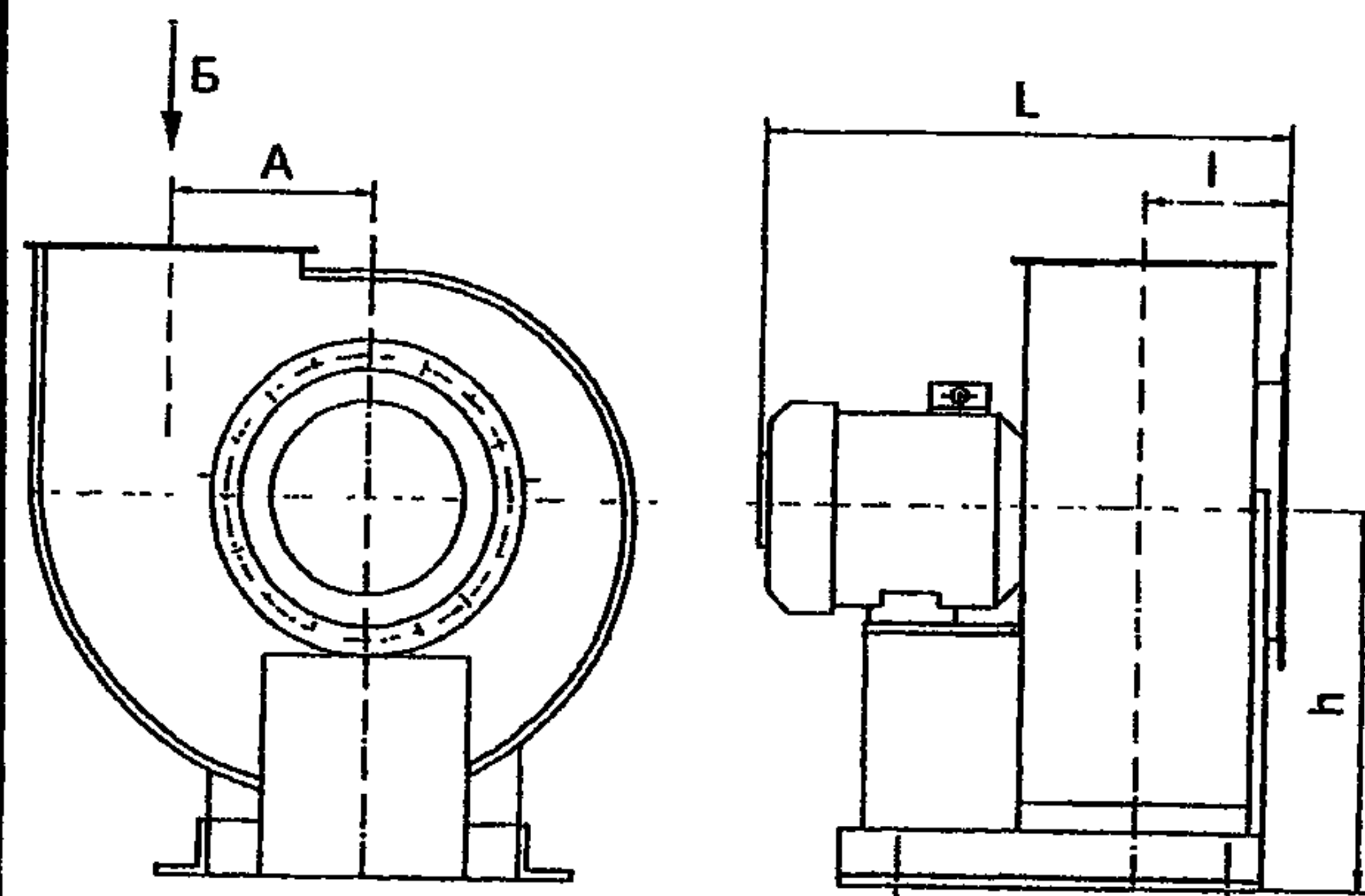
Расположение отверстий для крепления вентилятора ВР-300-45-2
