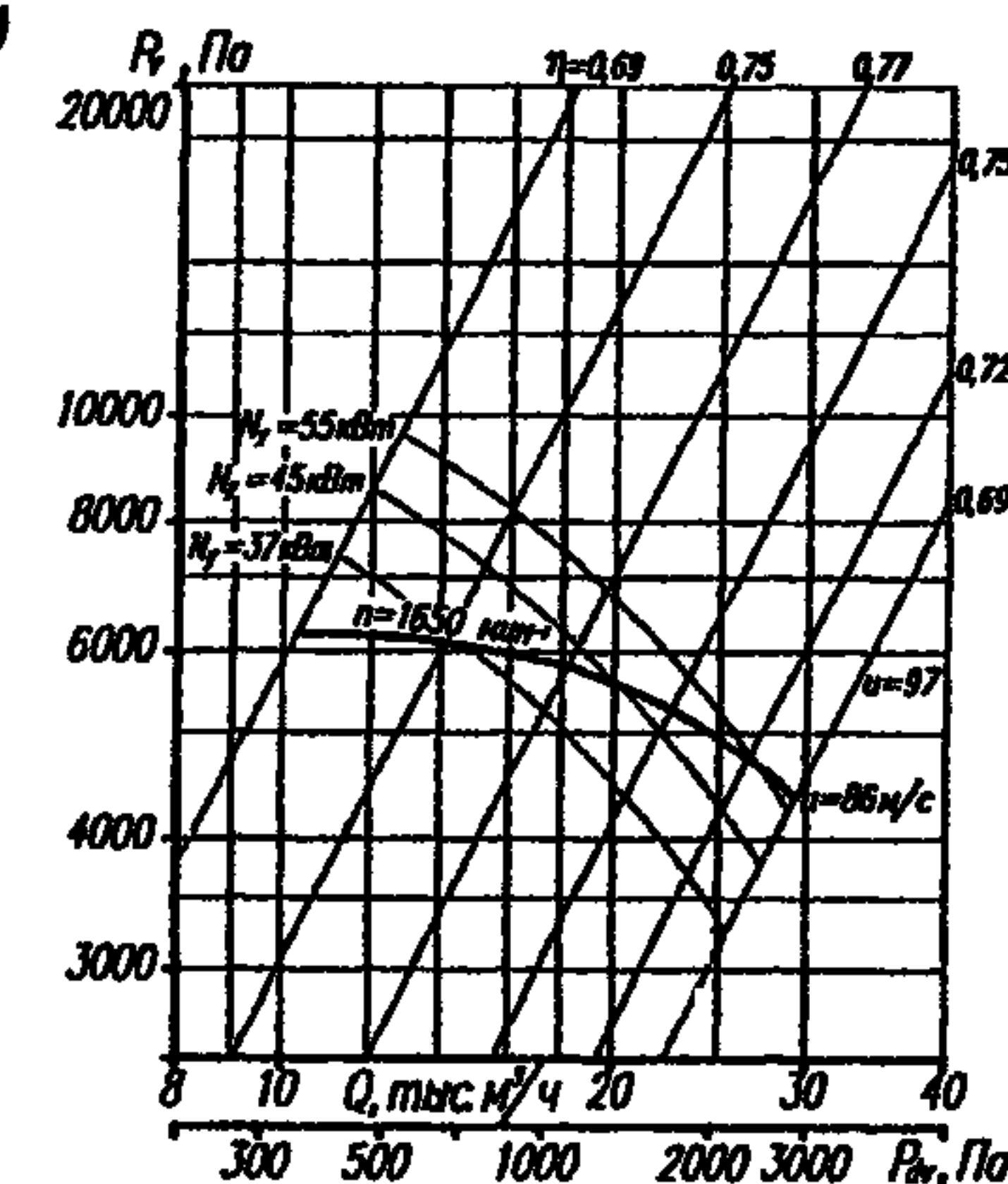
Аэродинамическая характеристика ВР 132-30 №10 (5 исполнение)
