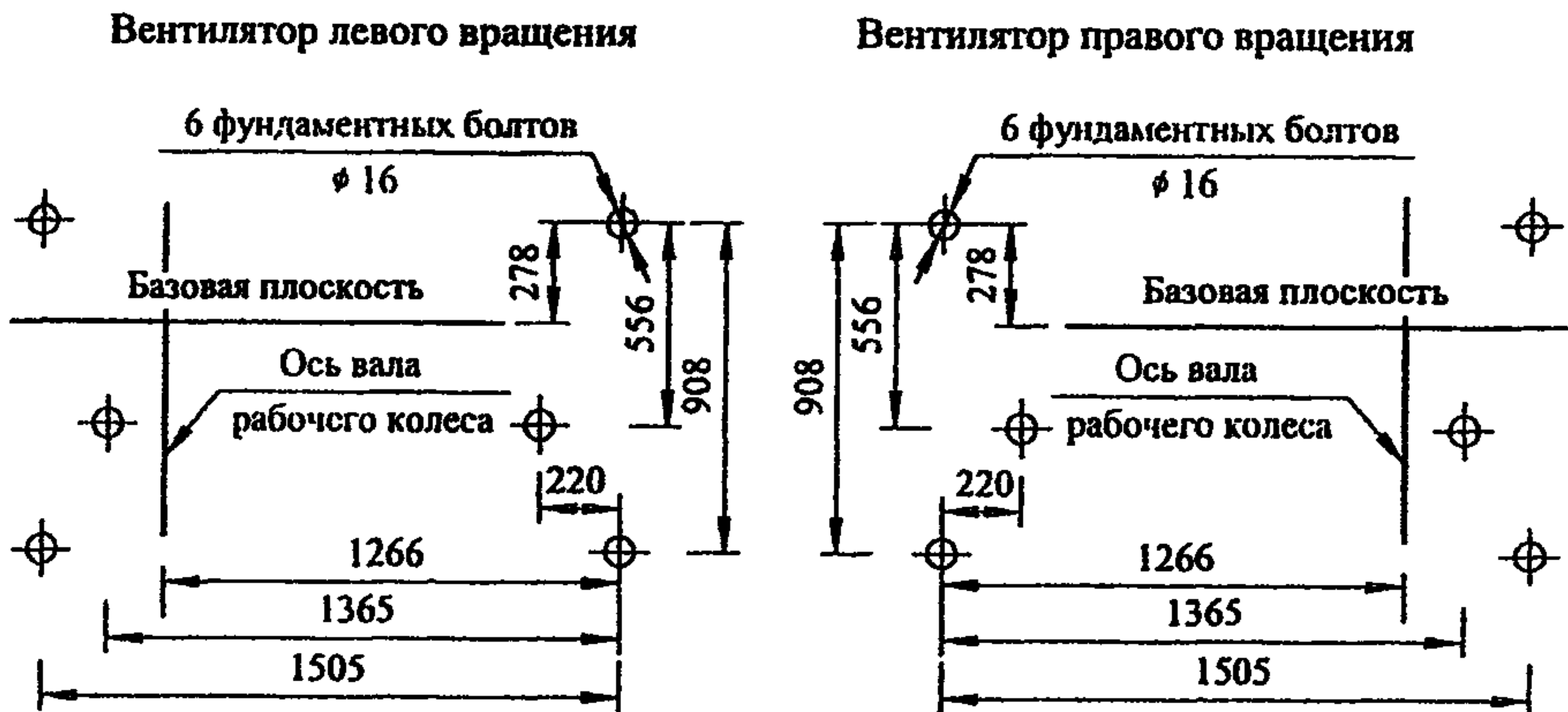
Схема разметки под фундаментные болты вентилятора ВРП-100-45-10.
