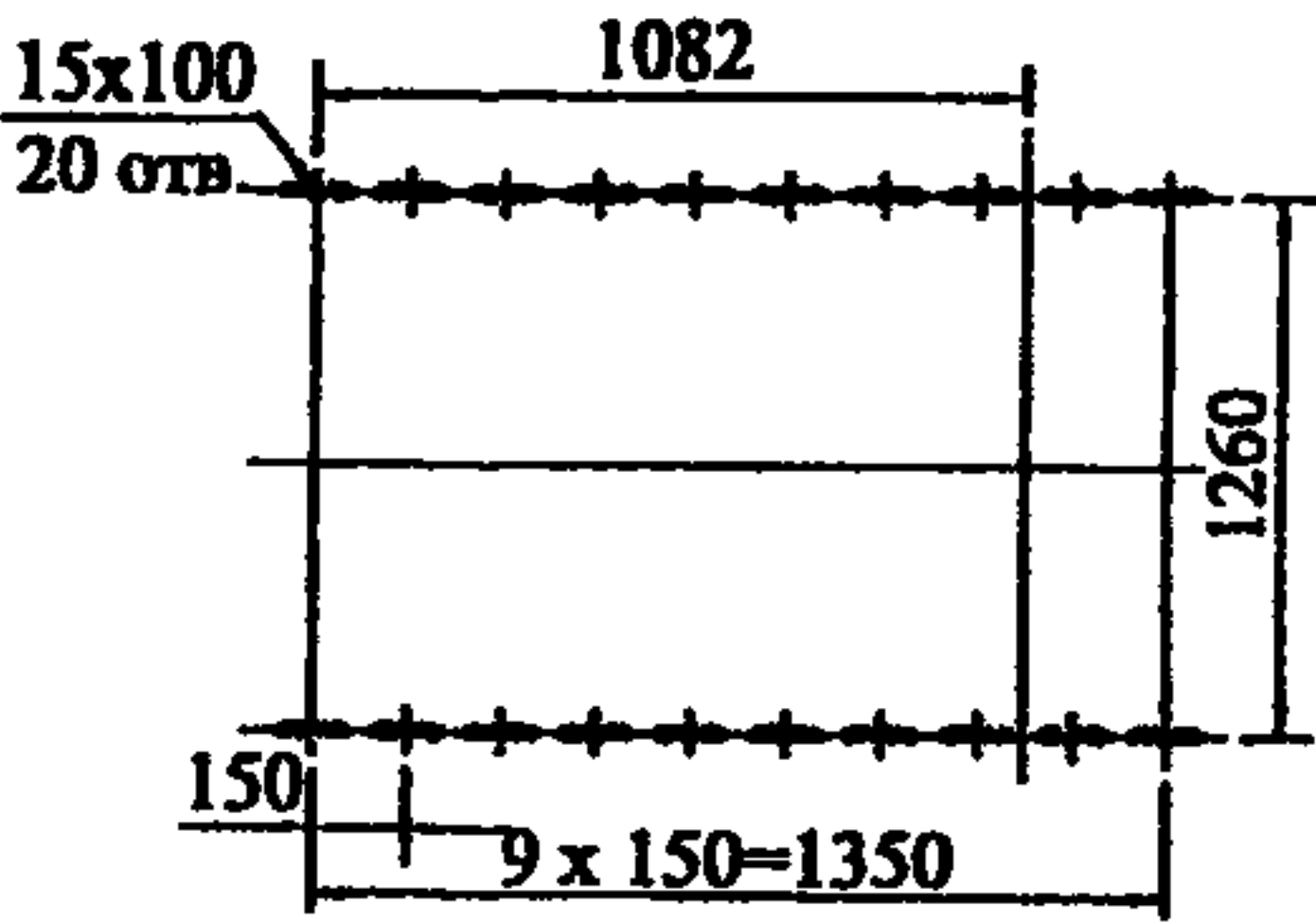
ВР-80-70-12.5
