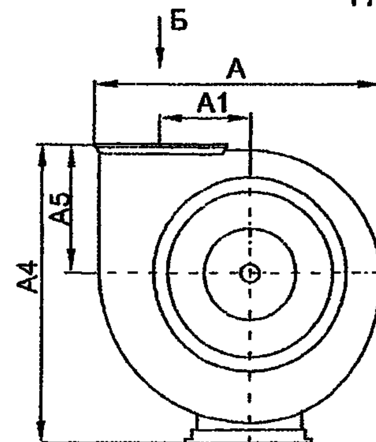
Схема расположения отверстий для крепления вентиляторов ВЦ4-70-6,3И1
