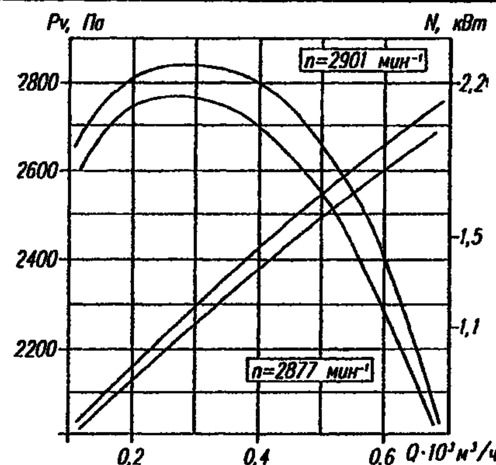
Аэродинамическая характеристика ВР 132-30 №4 (1 исполнение).
