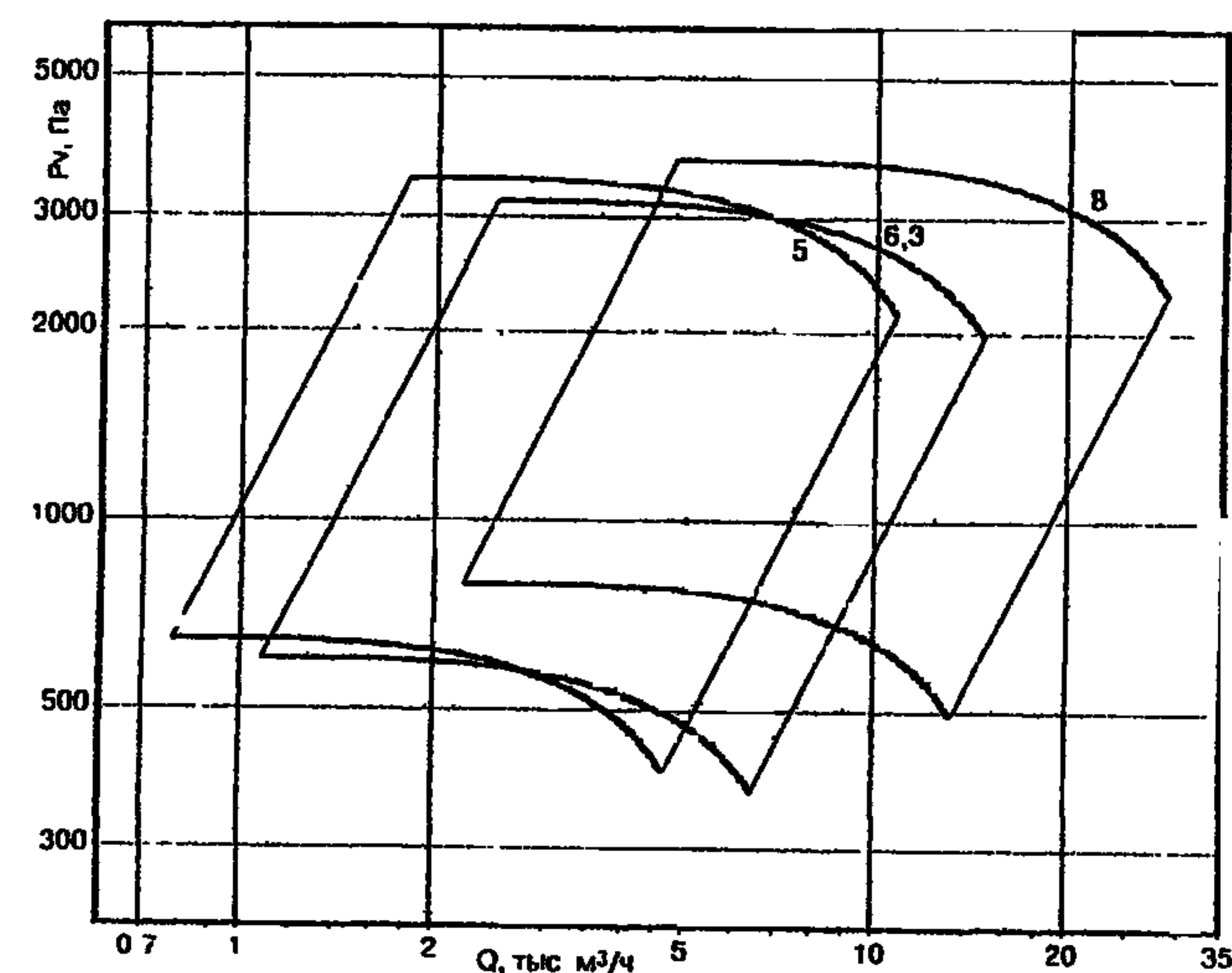
Область аэродинамических параметров
