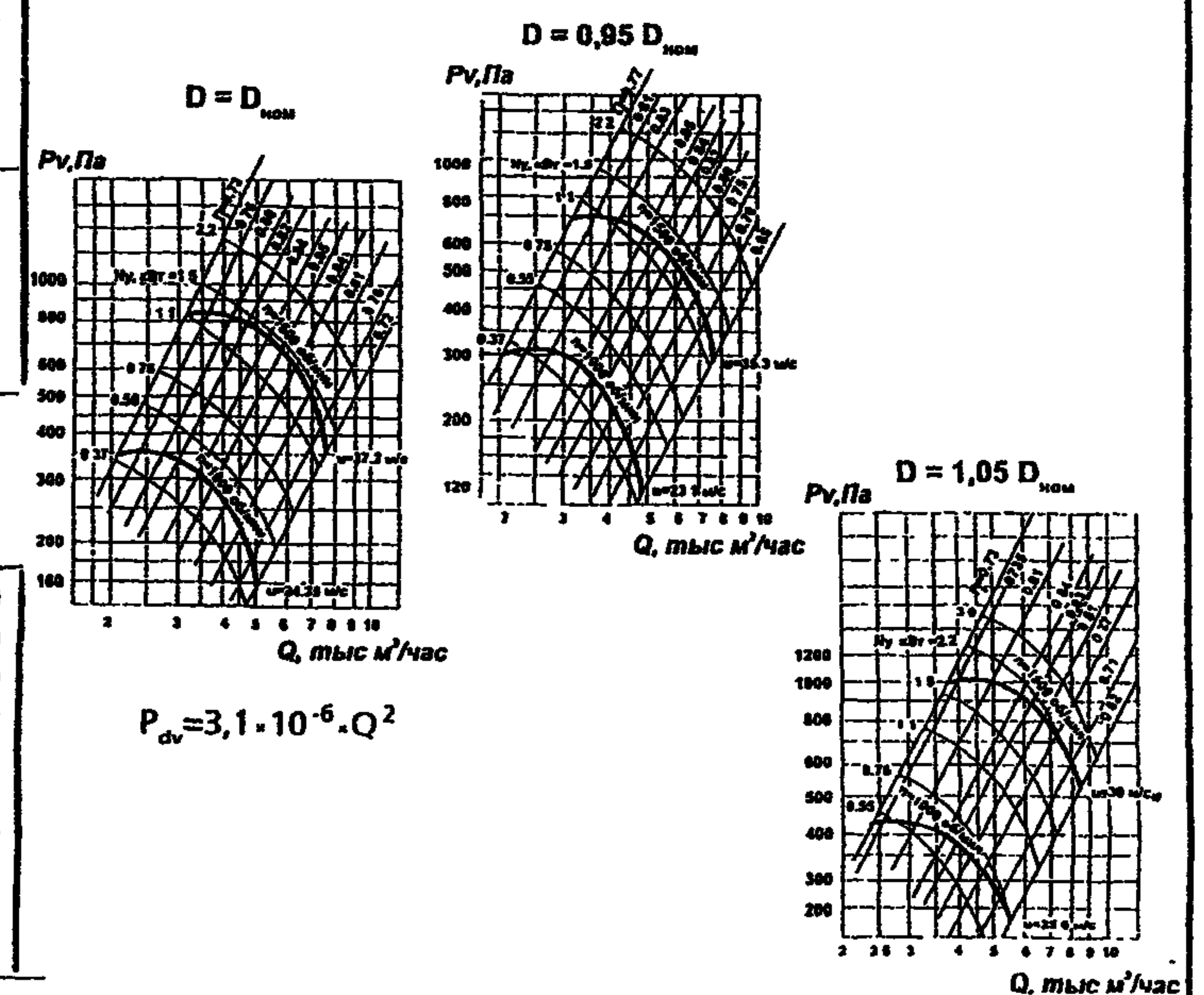
ВР80-75 (ВЦ 4 - 75) исп. 1 № 5
