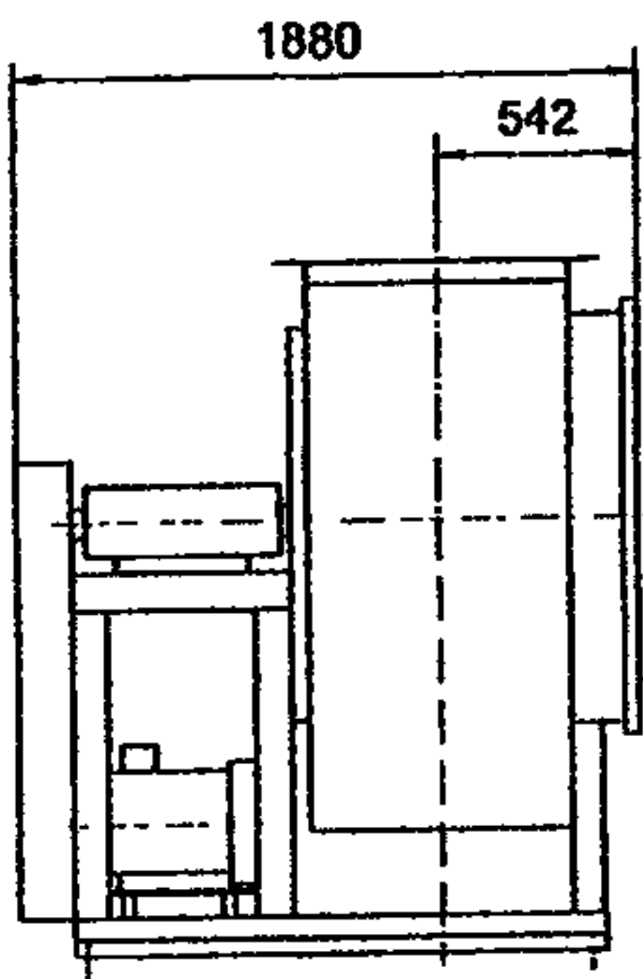
ВР-80-70-12.5-01
