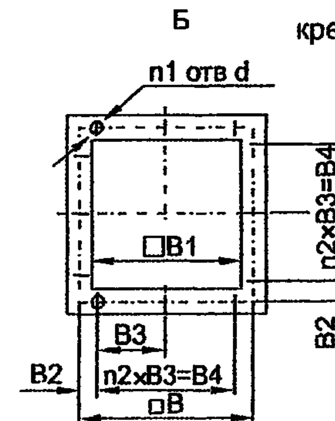
Схема расположения отверстий для крепления вентиляторов ВЦ4-70-8(К)
