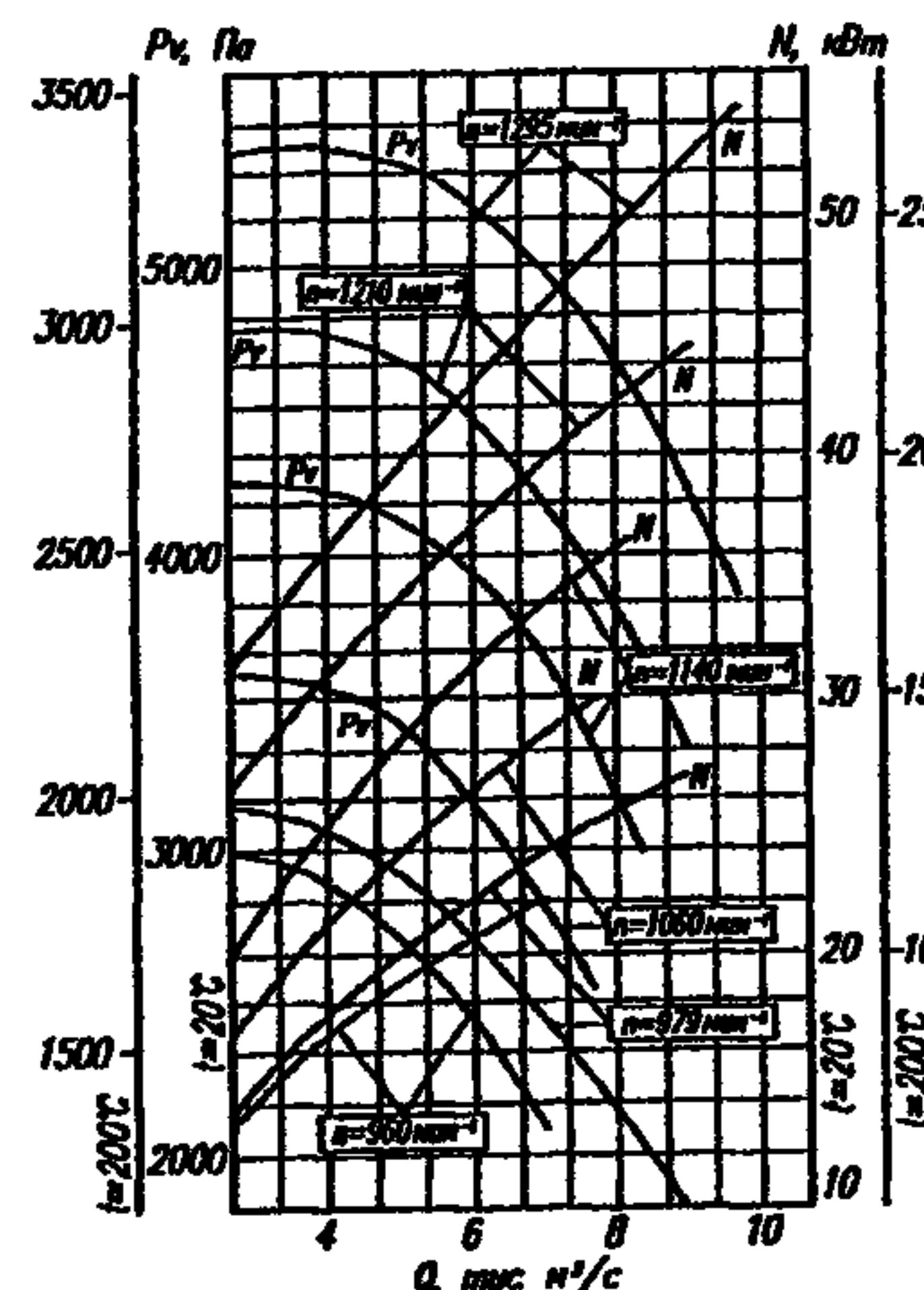
Аэродинамическая характеристика ВР 132-30 №4 (1 исполнение).
