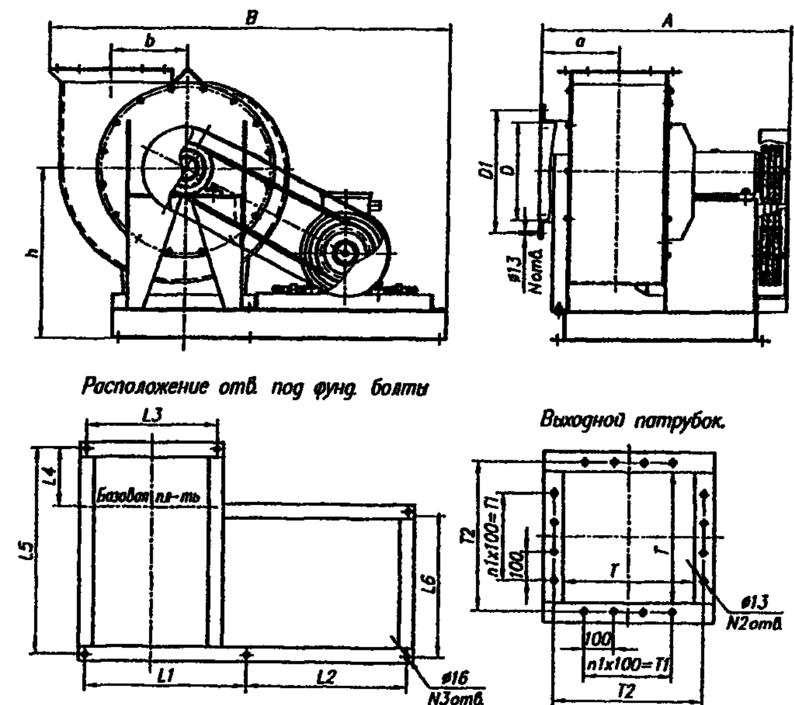
Габаритные и присоединительные размеры вентилятора ВР 140-40 №5-8.
