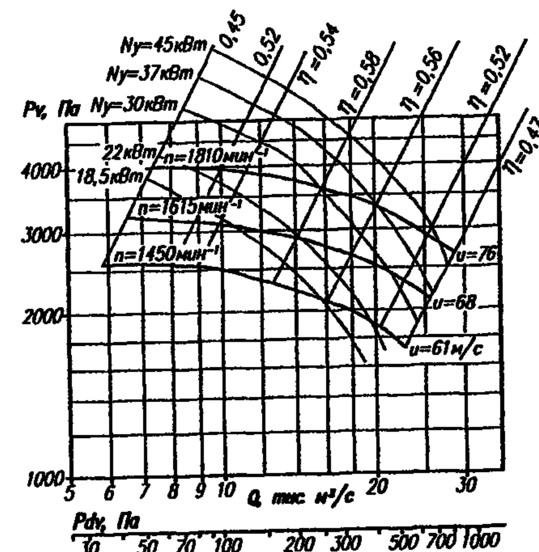
Аэродинамическая характеристика вентилятора ВР 140-40 № 8
