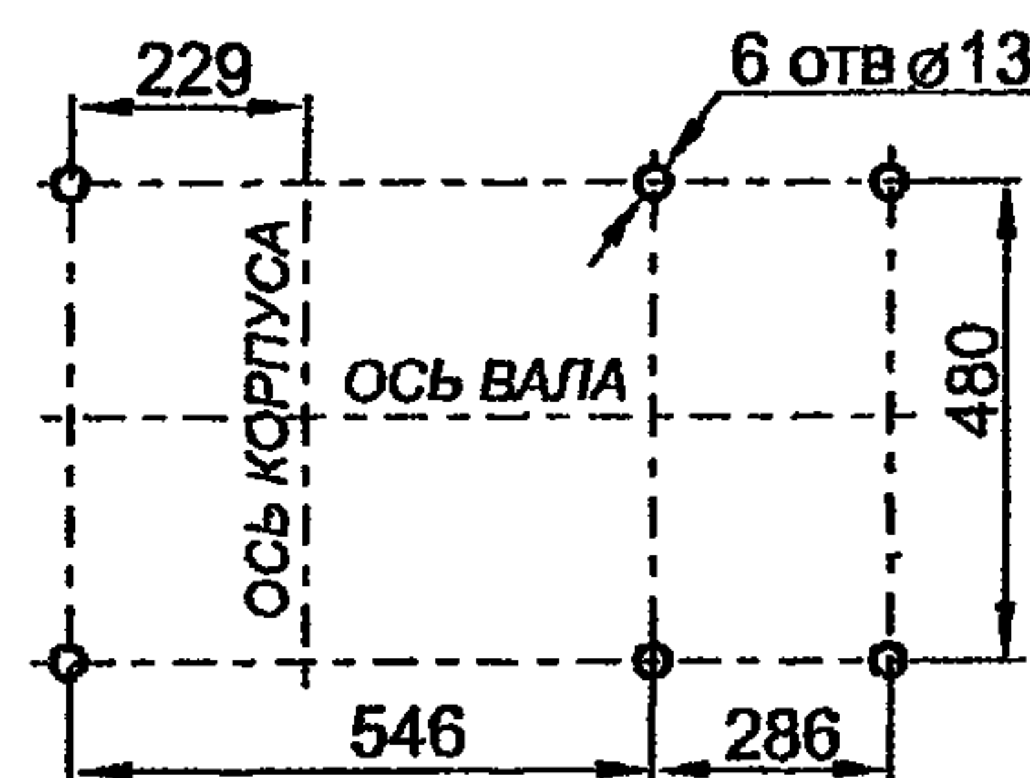
Схема расположения отверстий для крепления вентиляторов ВЦ4-70-6,3И1
