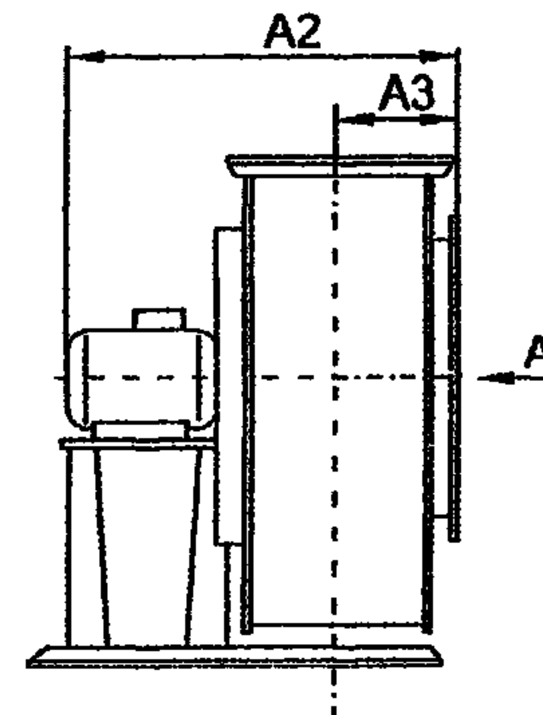
Схема расположения отверстий для крепления вентиляторов ВЦ4-70-6,3И1
