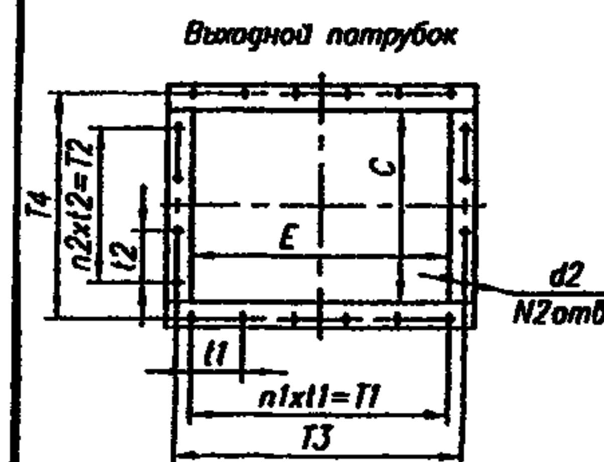
Вентилятор типа ВР 132-30 (исполнение 1).
