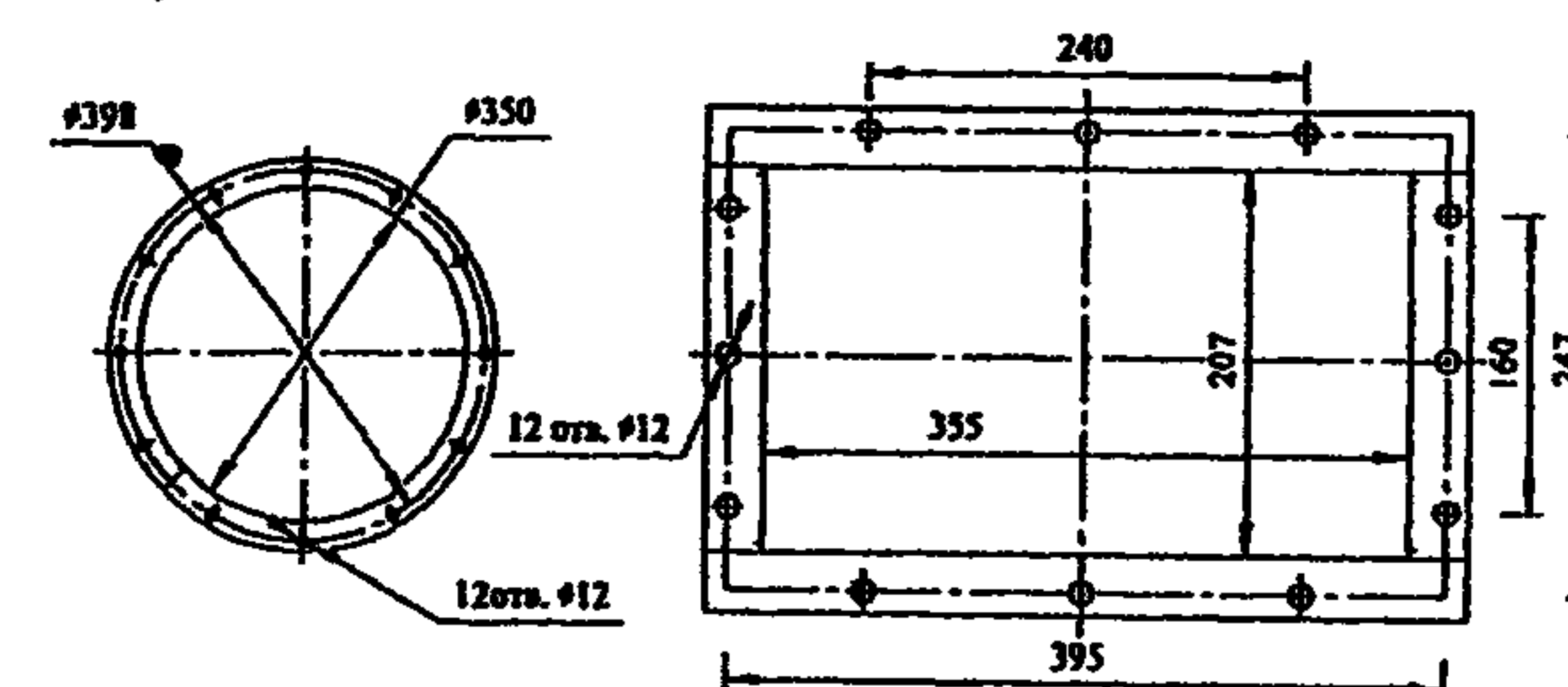
ПРИСОЕДИНИТЕЛЬНЫЕ РАЗМЕРЫ
