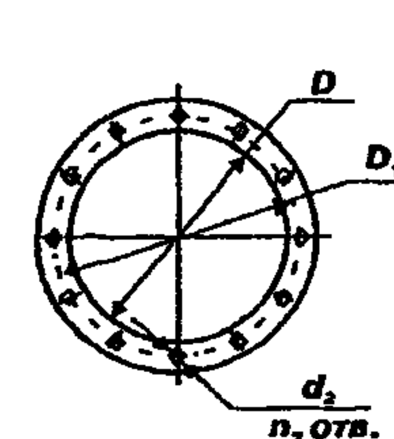
Фланец входной
