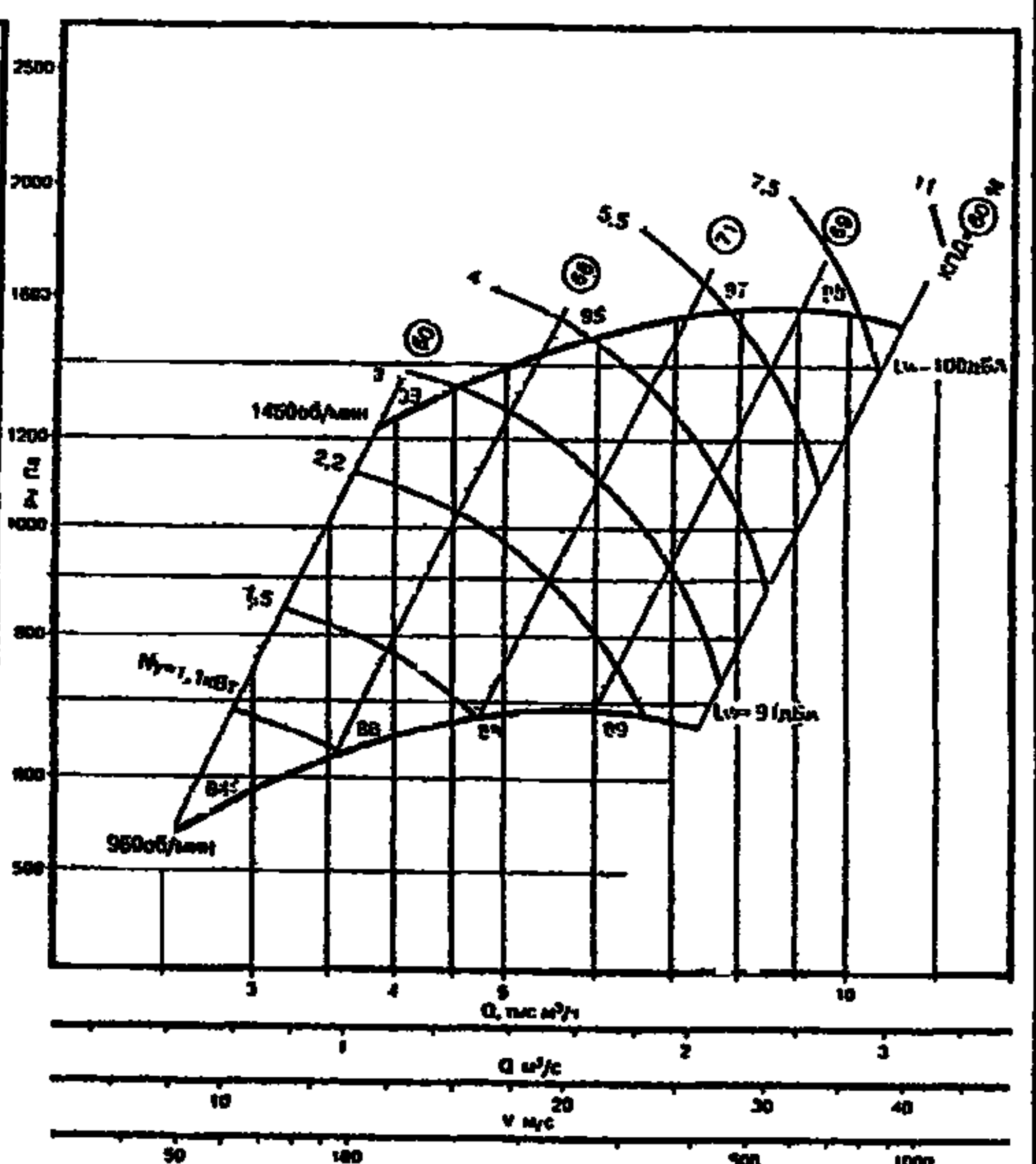
ВЦ 14-46-4 исполнение 1
