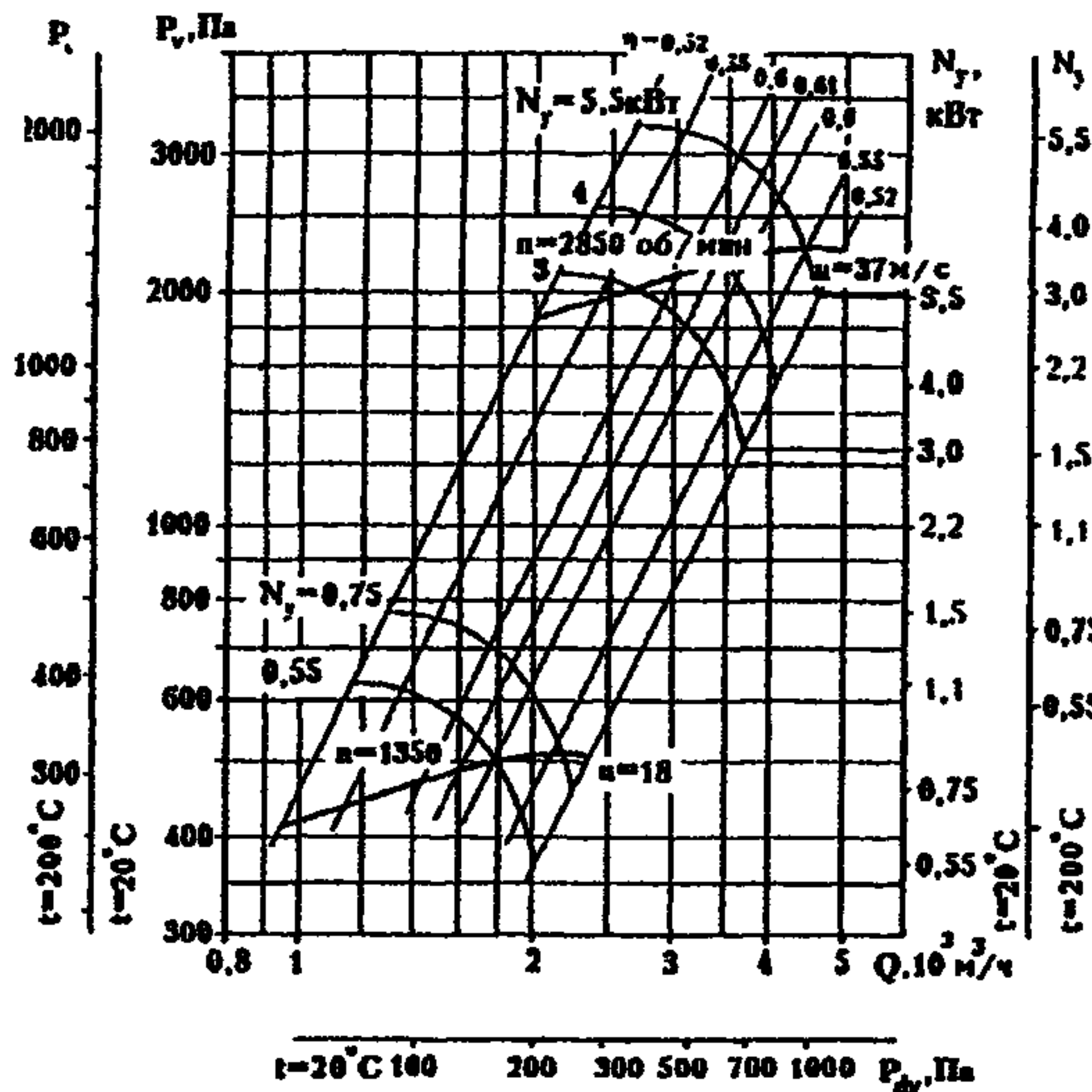
ВР-300-45-2,5
