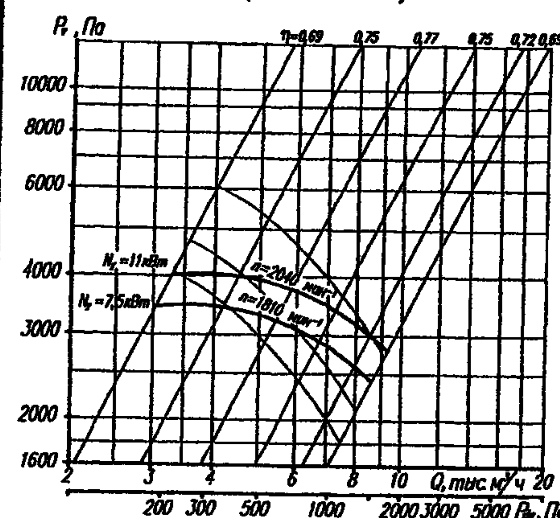
Аэродинамическая характеристика ВР 132-30 №6,3 (5 исполнение)
