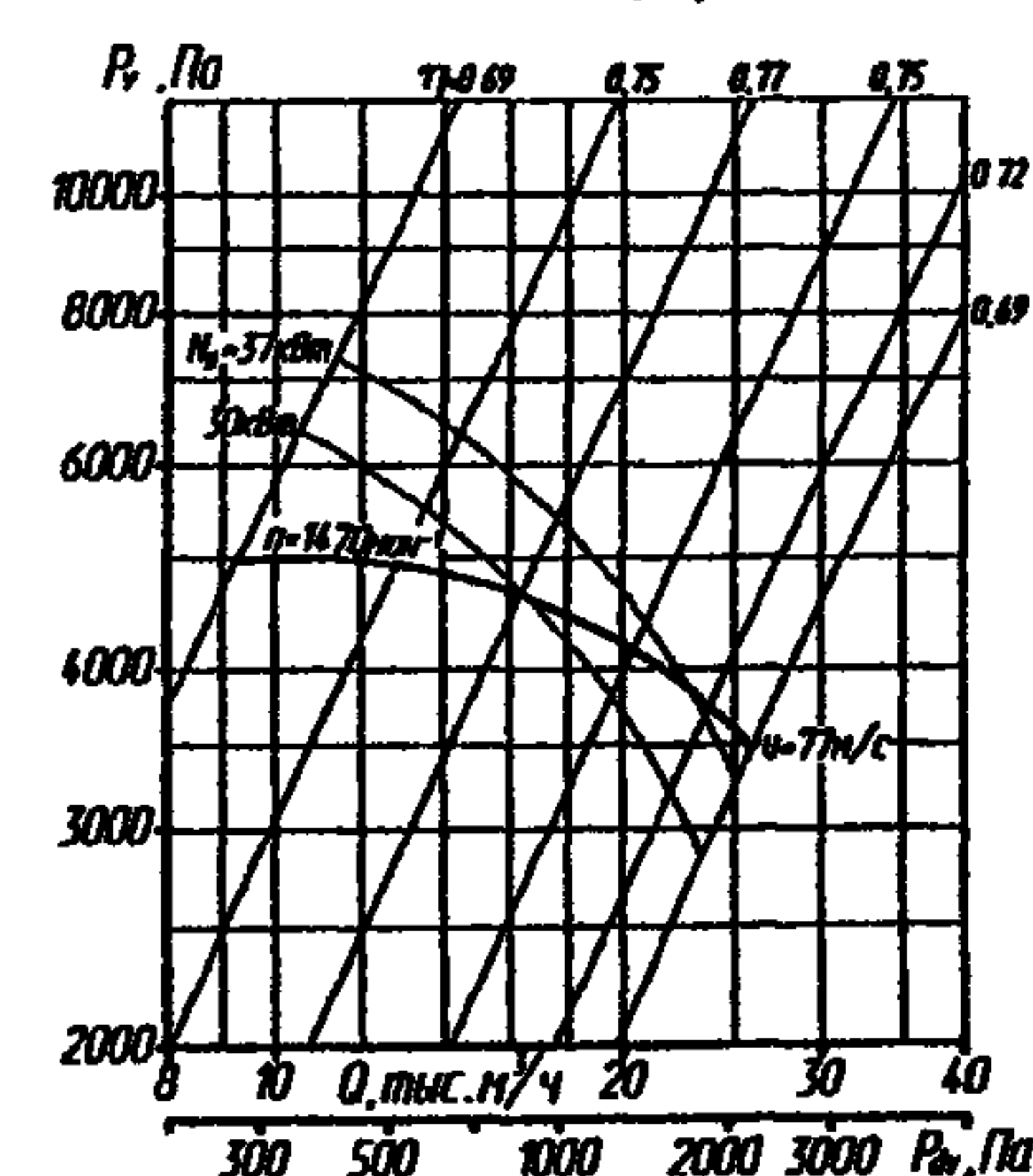
Аэродинамическая характеристика ВР 132-30 №10 (1 исполнение).
