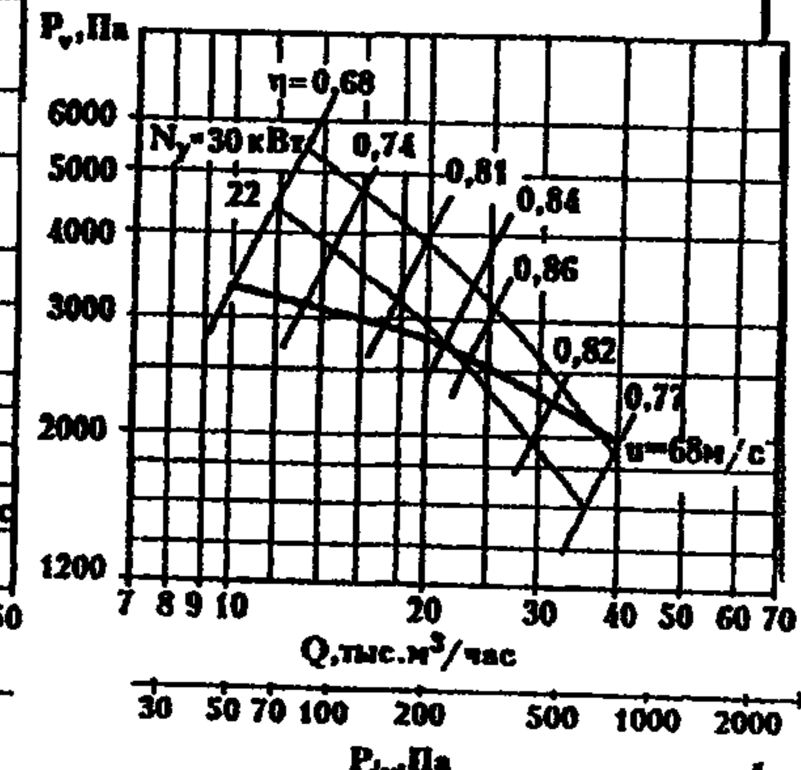
В.Ц5-50-9.01
