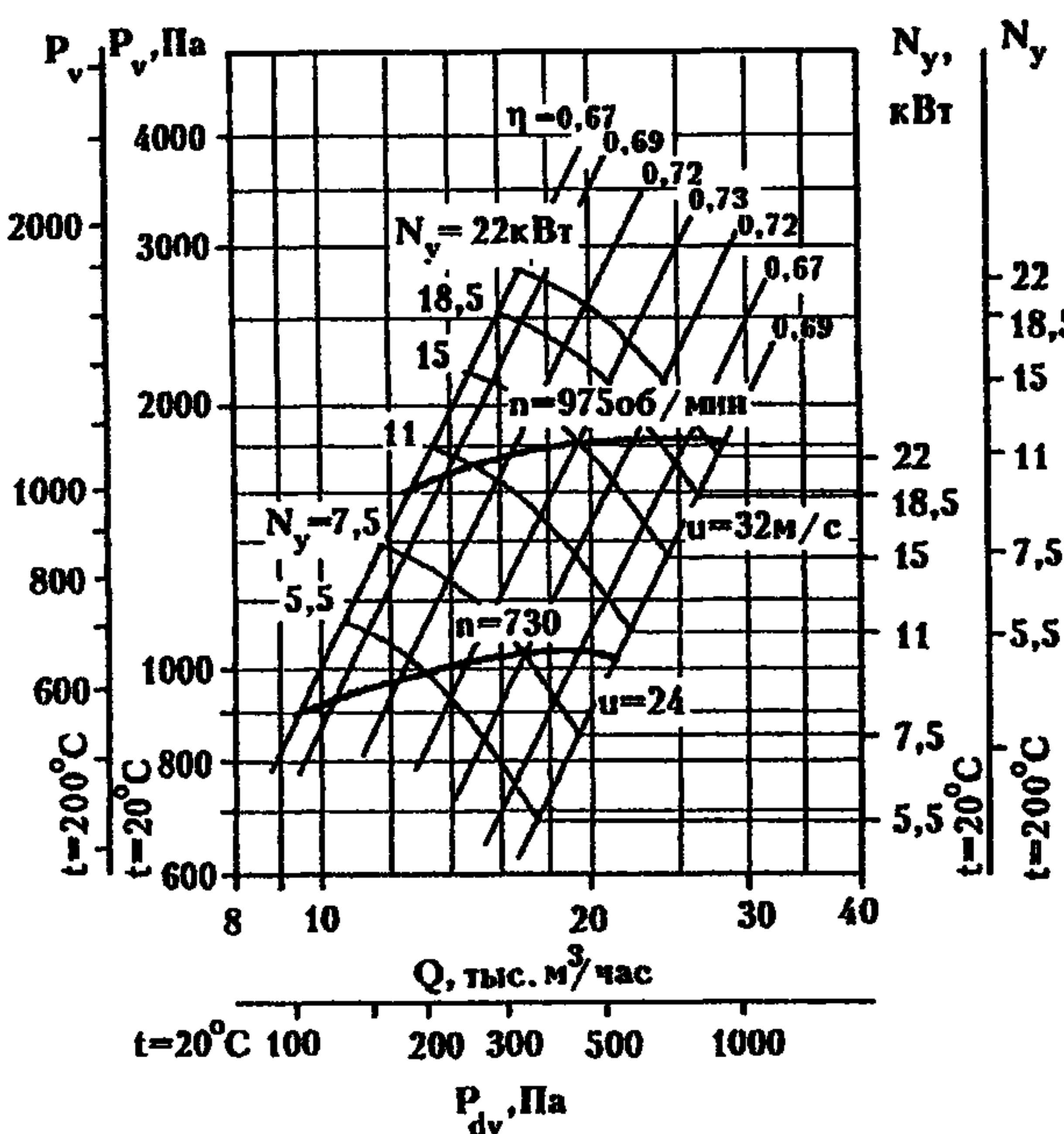
В-Ц14-46-6,3
