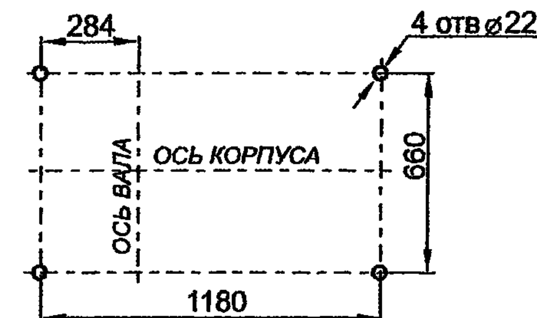
Схема расположения отверстий для крепления вентиляторов ВЦ4-70-8И1
