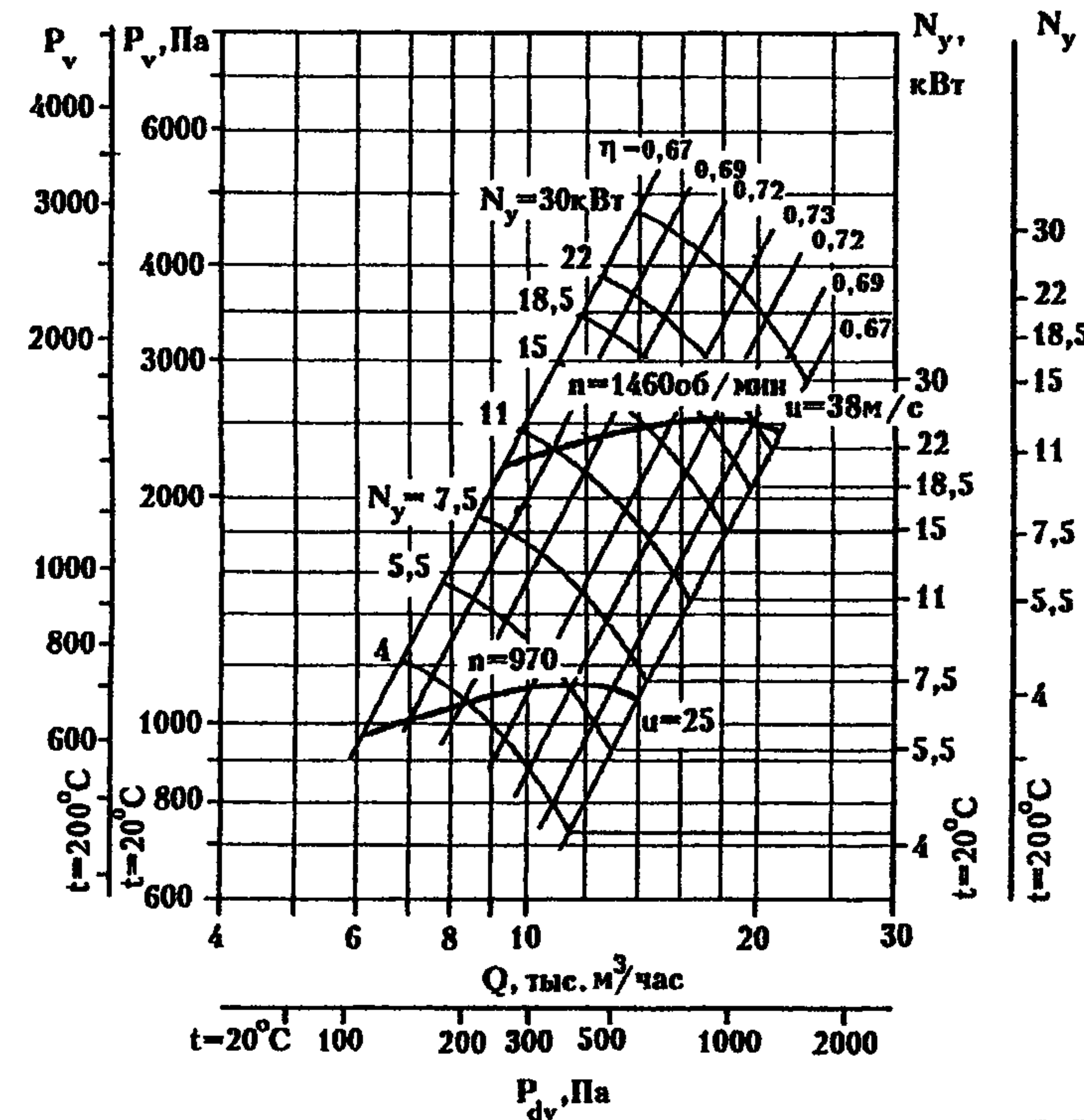
В-Ц14-46-5
