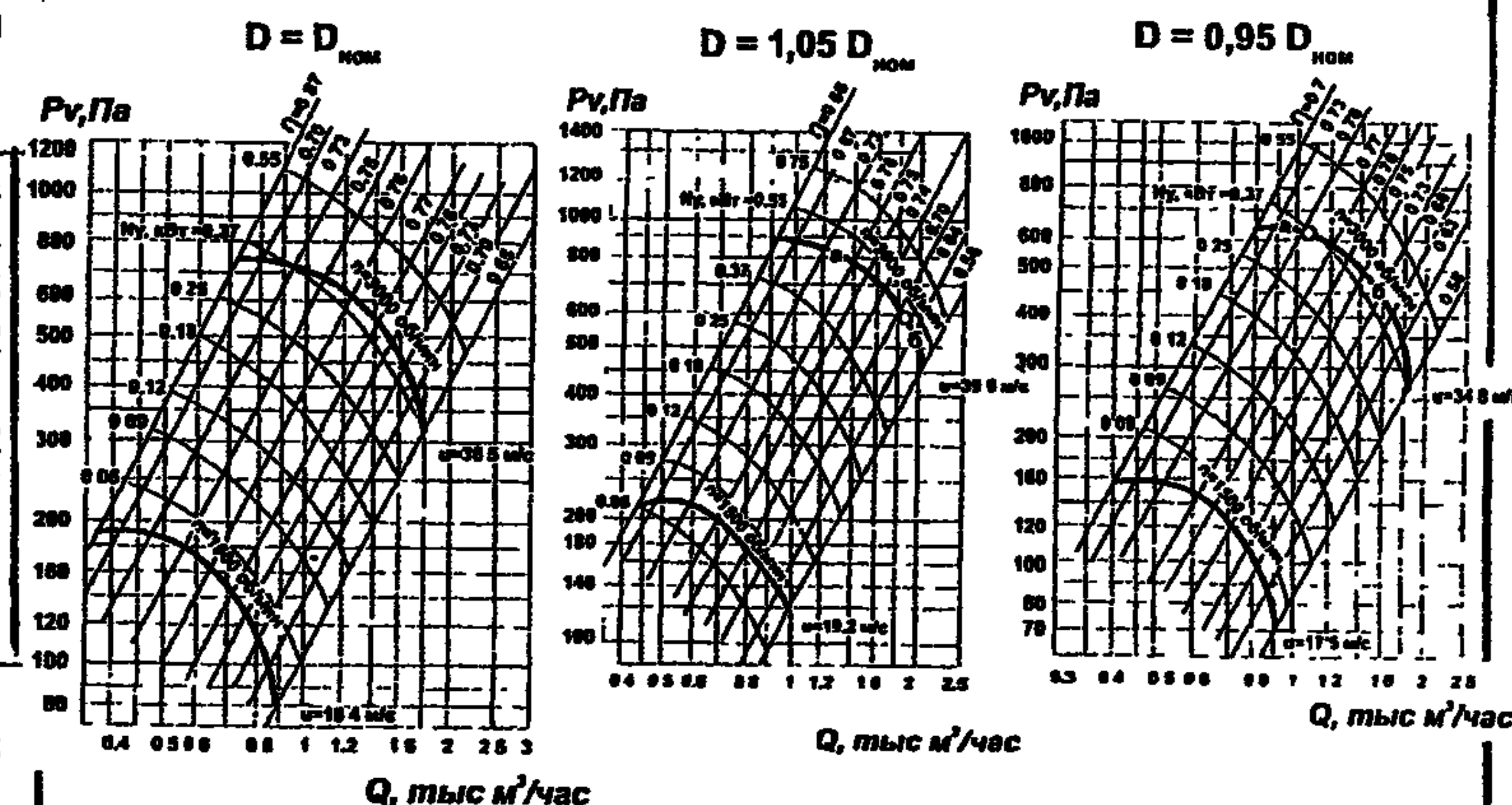
ВР80-75 (ВЦ 4 – 75) исп. 1 № 2,5
