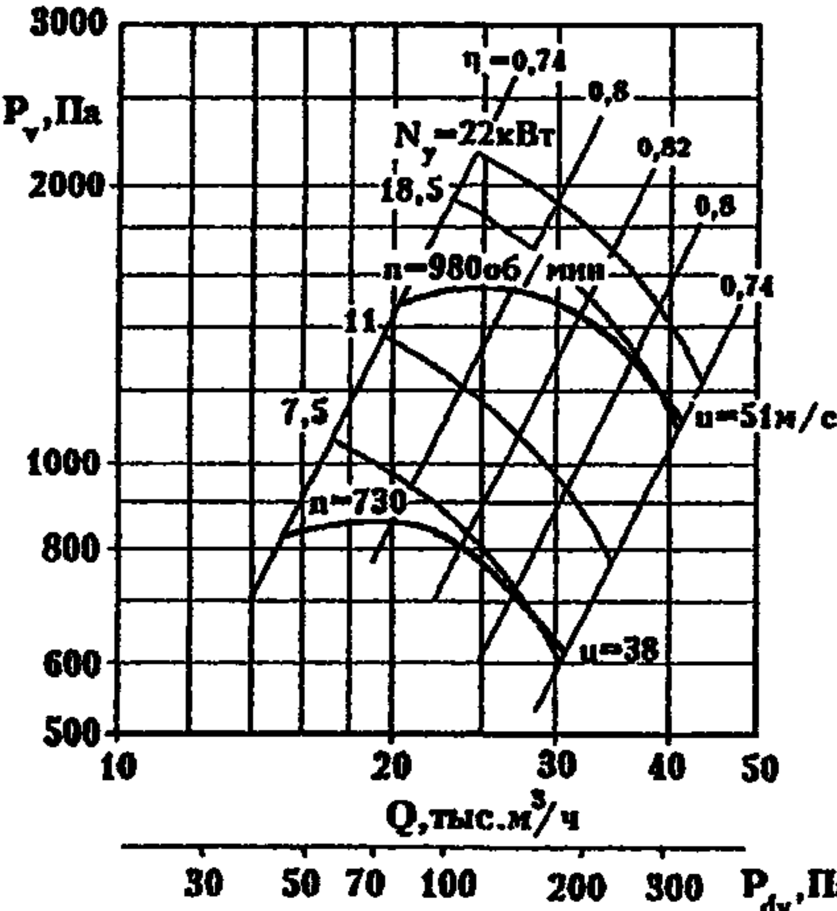
ВР-80-70-10-02
