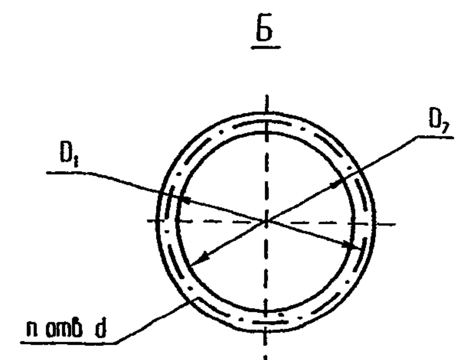
Габаритные и присоединительные размеры
