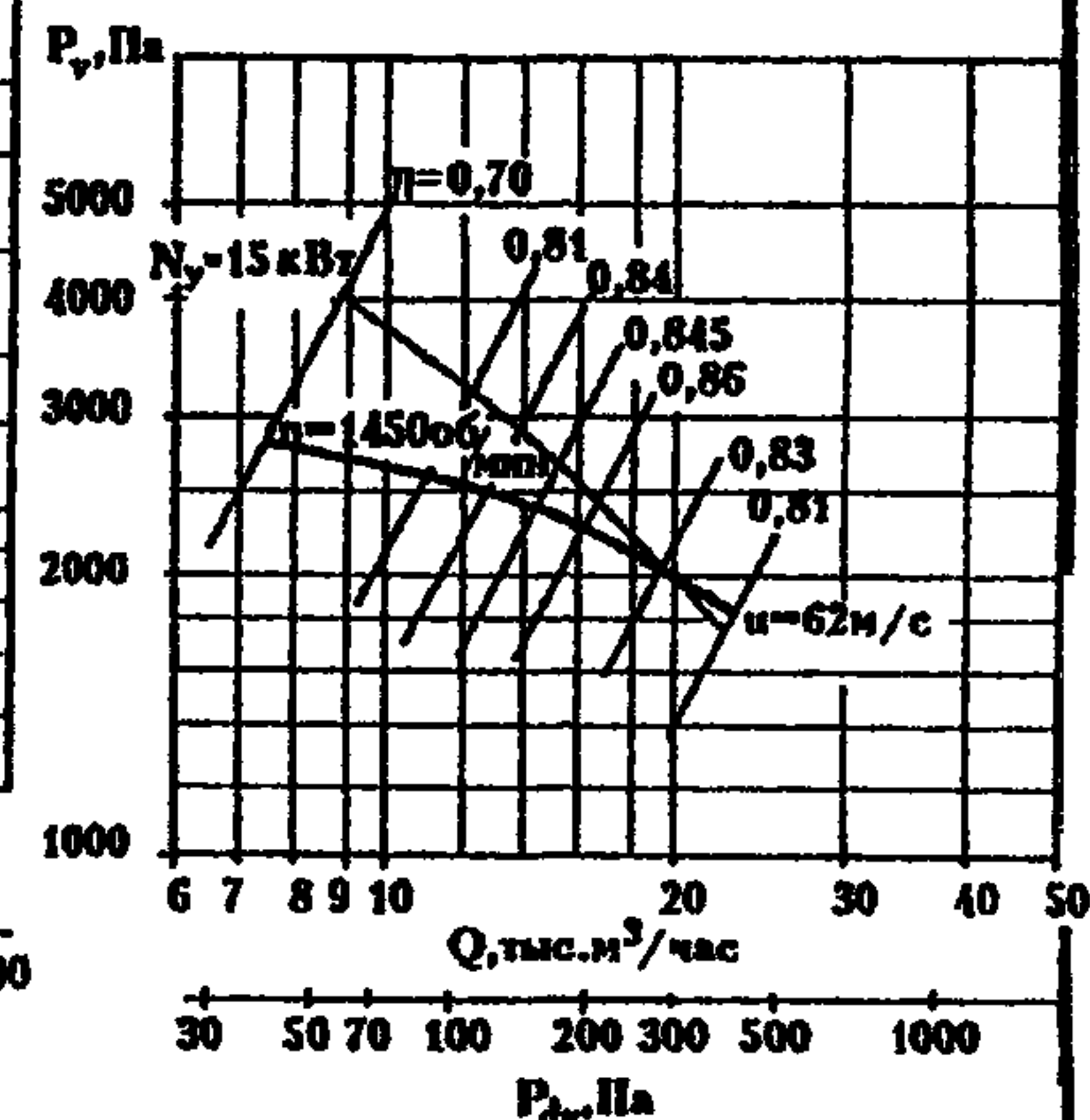
В.Ц5-50-9.01
