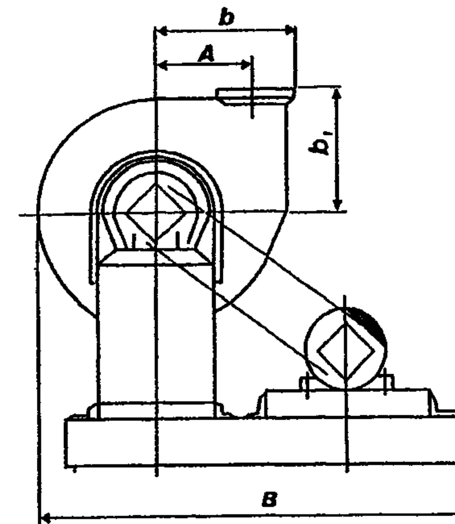
ВР-125-28 исполнение 5
