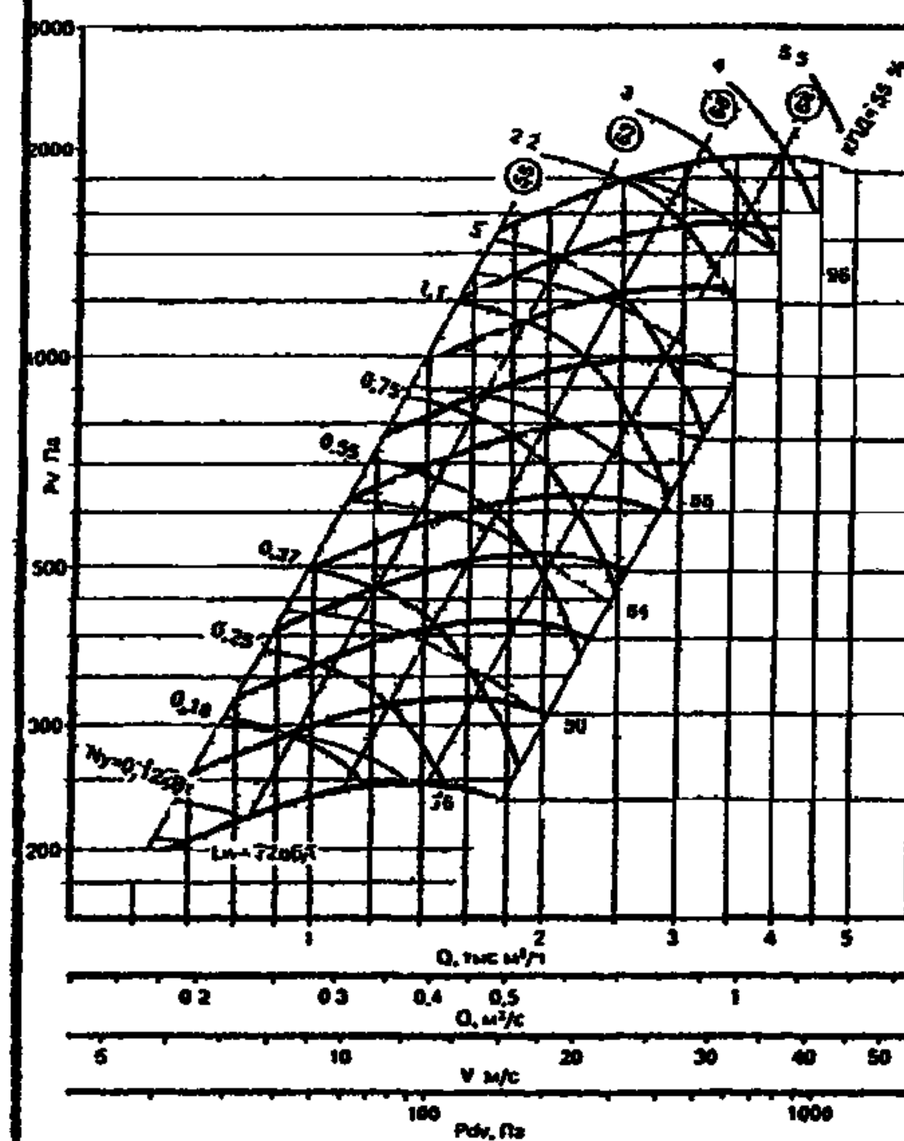
ВЦ 14-46-2,5 исполнение 5
