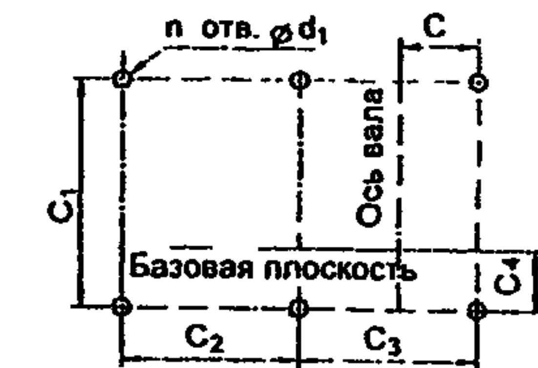
Расположение отверстий для крепления вентилятора
