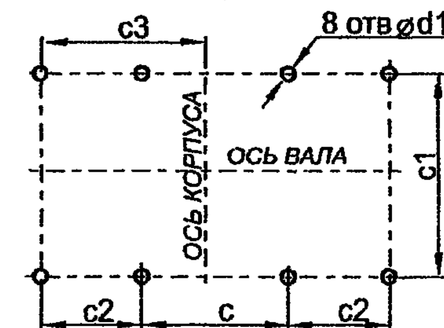
Схема расположения отверстий для крепления вентиляторов ВЦ4-70-2,5...5И1
