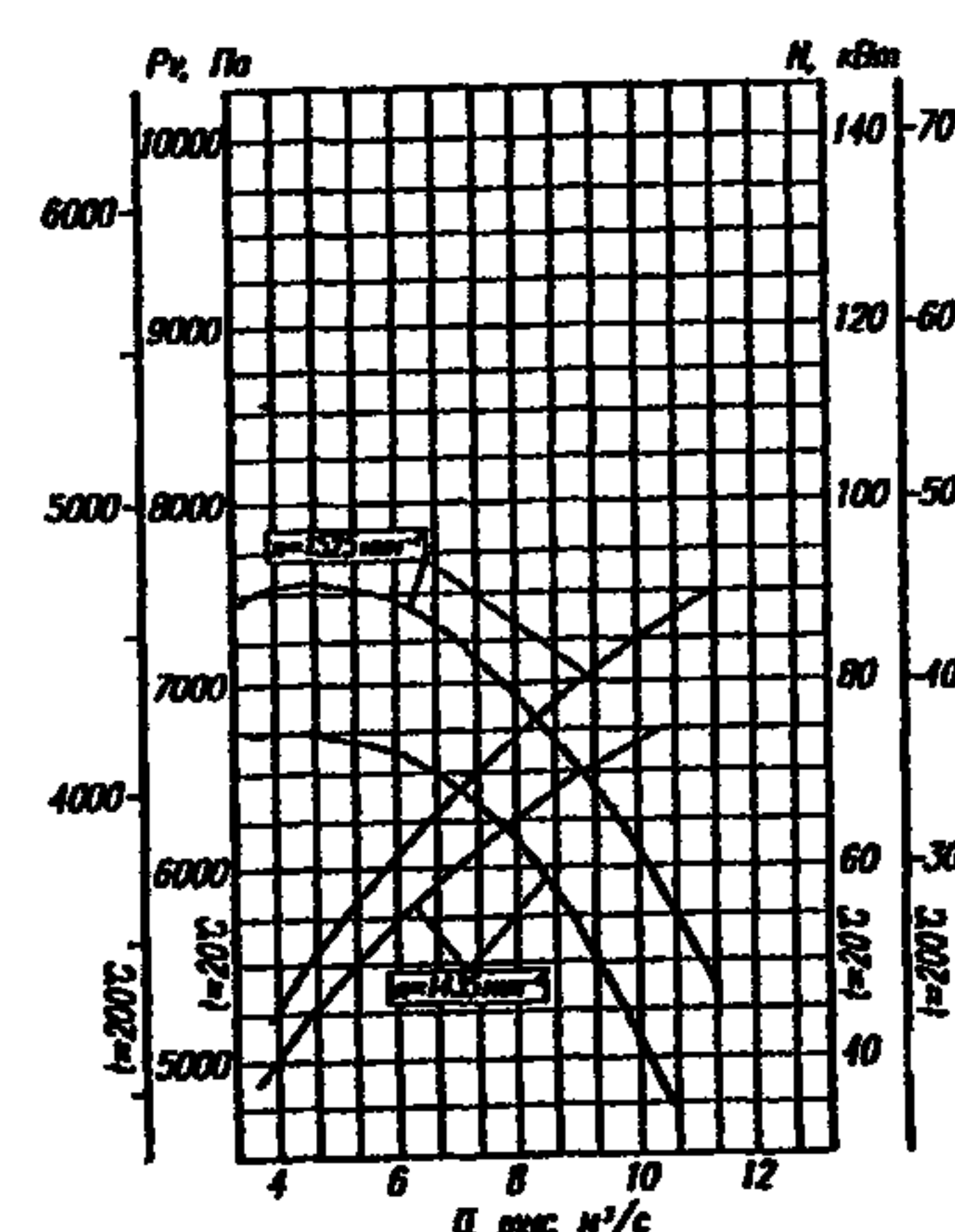
Аэродинамическая характеристика ВР 132-30 №12,5 (исполнение 5).
