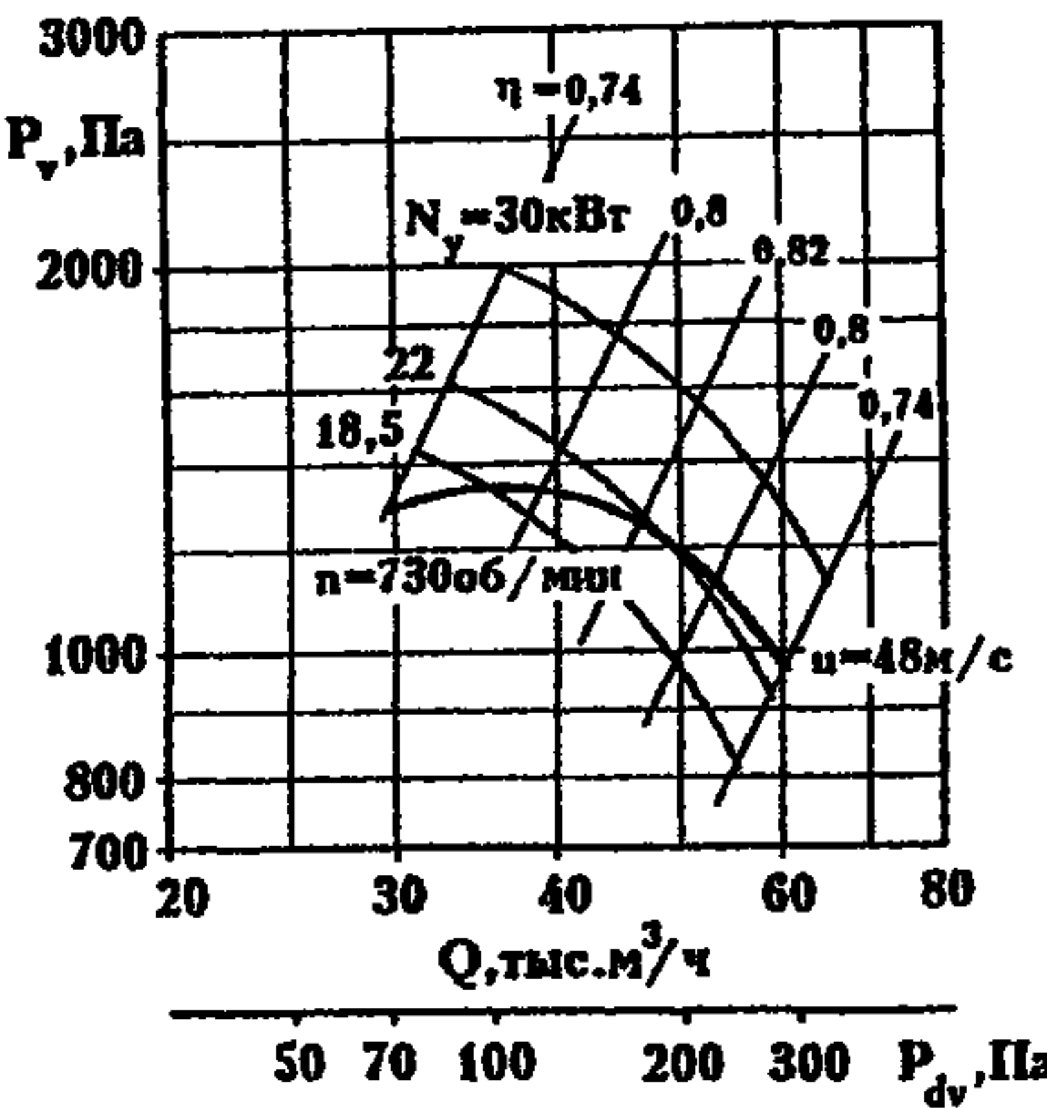
ВР-80-70-12.5-02
