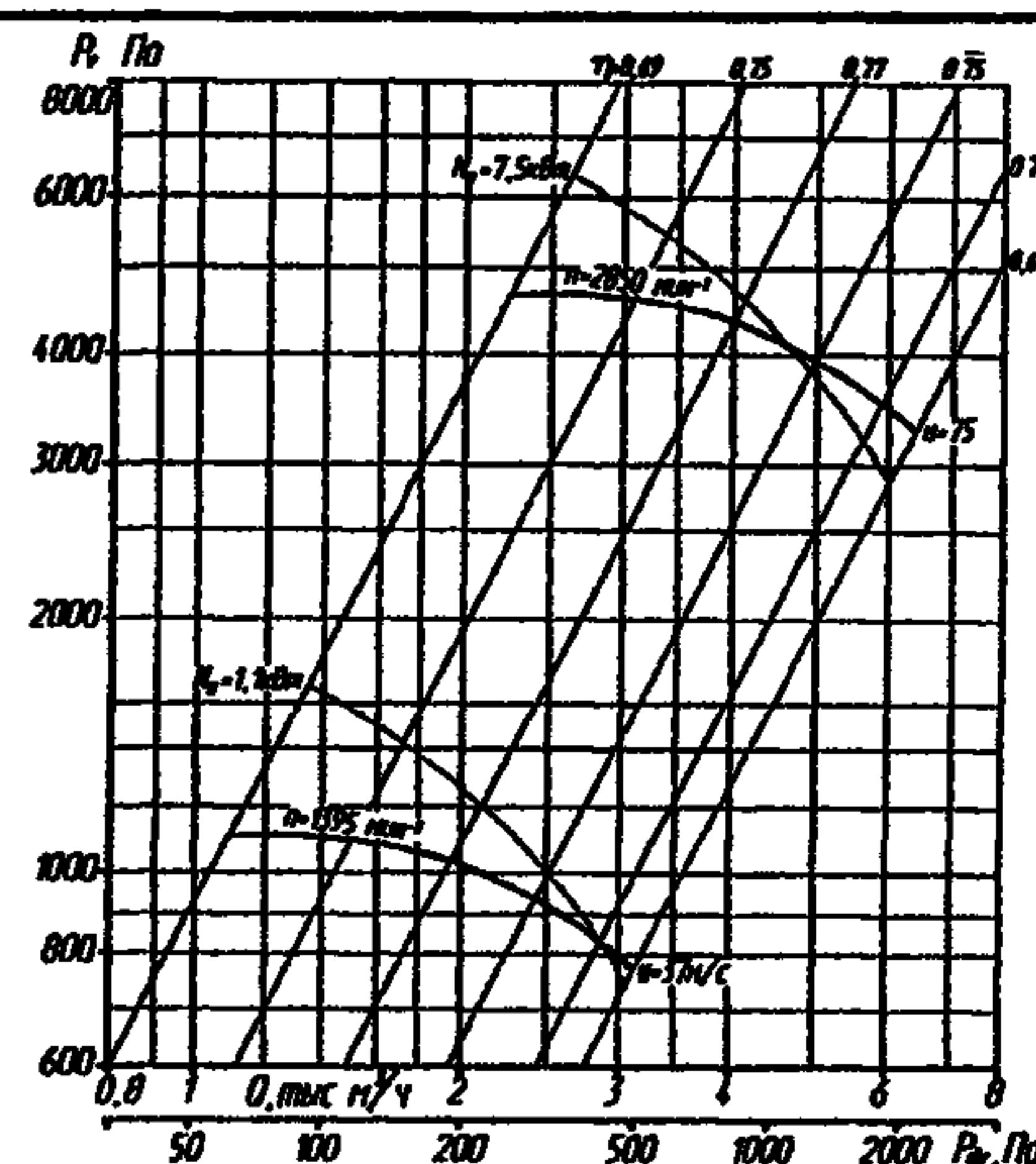
Аэродинамическая характеристика ВР 132-30 №5 (1 и 5 исполнение).
