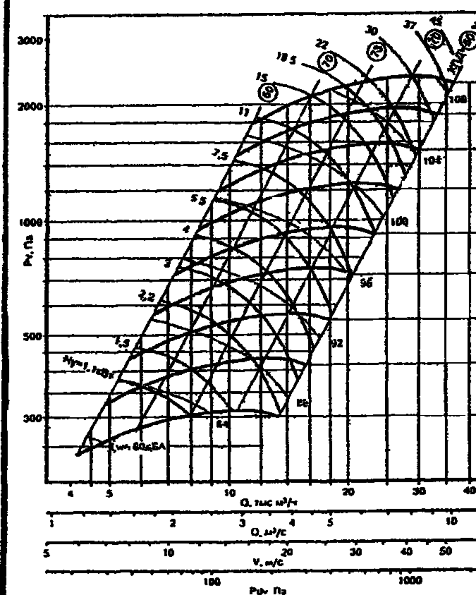
ВЦ 14-46-6,3 исполнение 5
