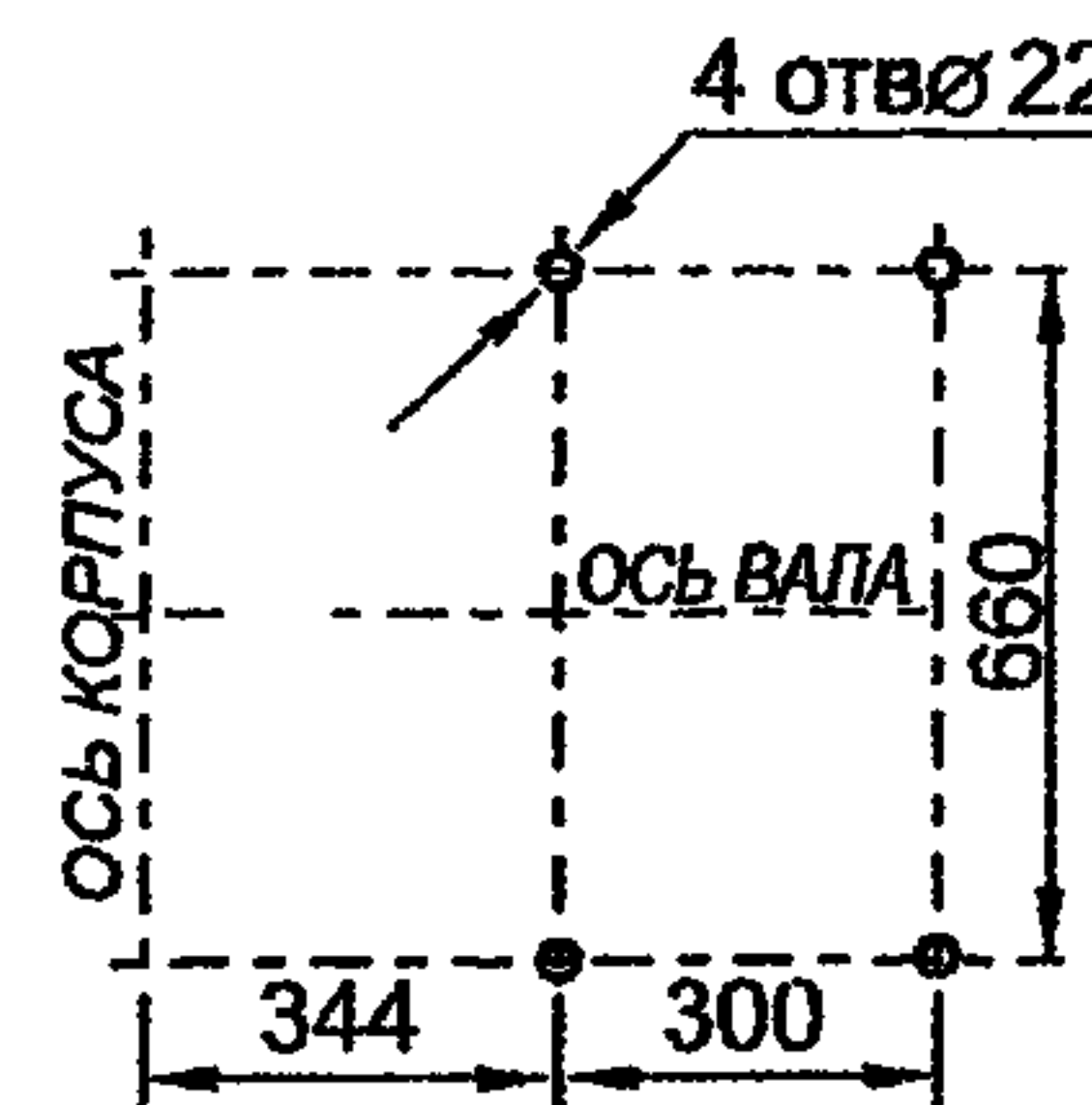
Схема расположения отверстий для крепления вентиляторов ВЦ4-70-8(К)
