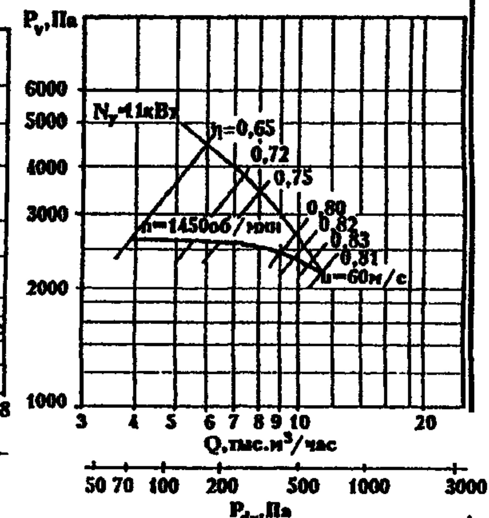
В.Ц5-45-8.01
