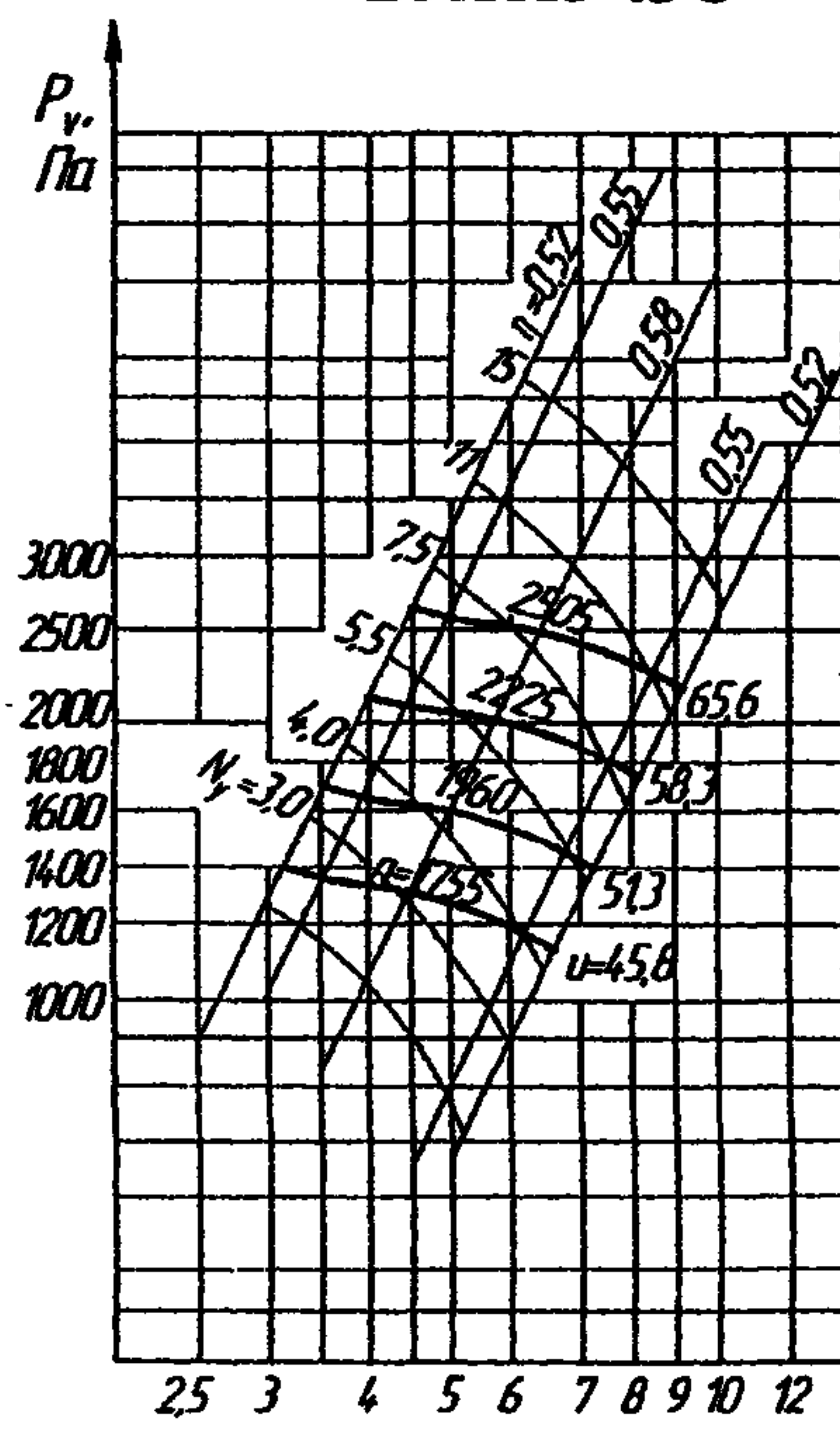
ВРП115-45-5
