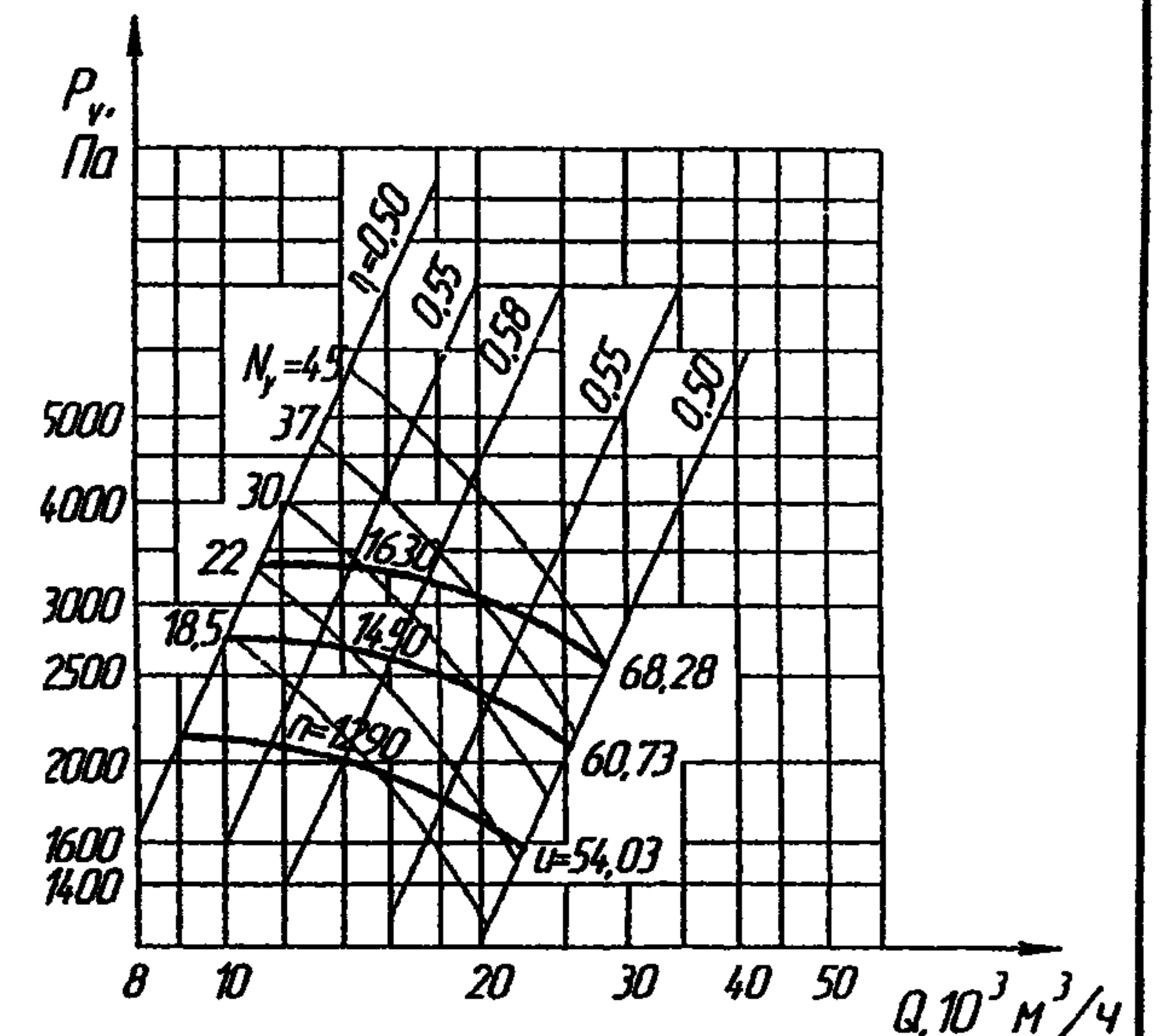
ВРП115-45-8
