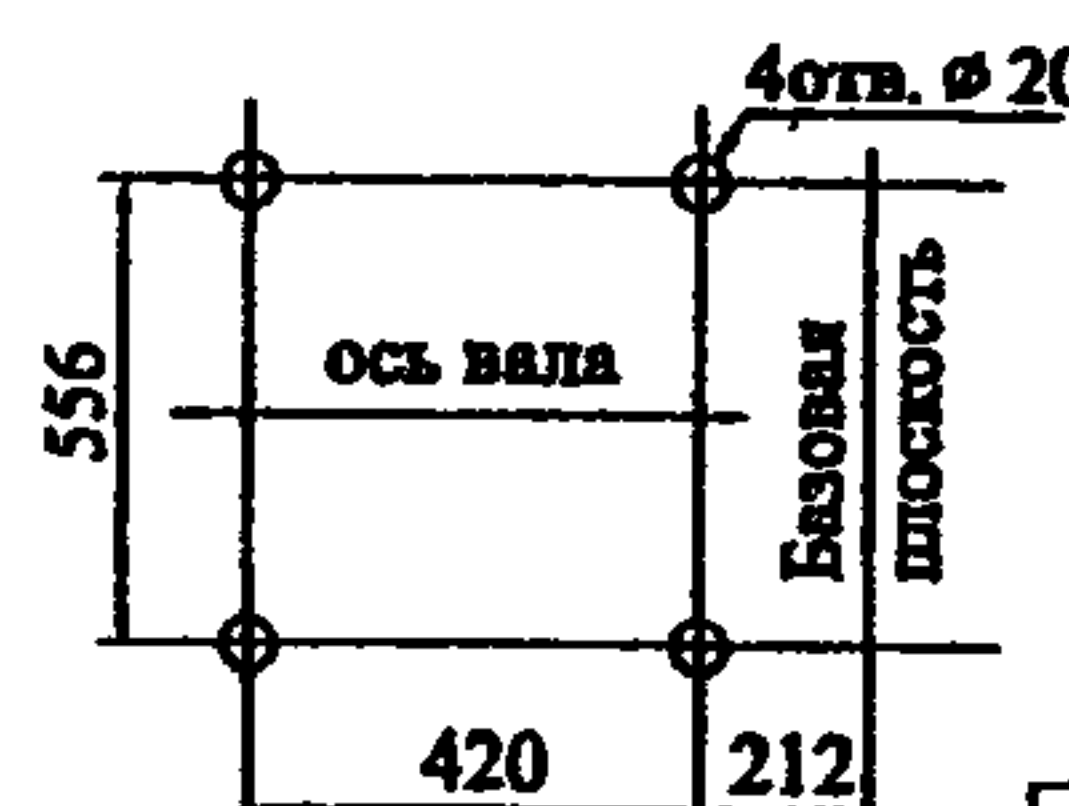
Расположение отверстий для крепления вентилятора
