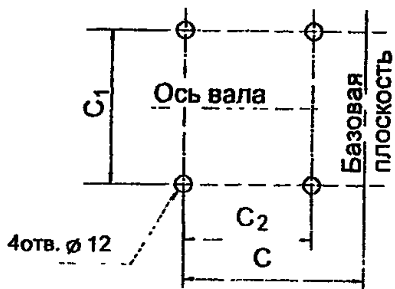
Расположение отверстий для крепления вентилятора ВР-300-45-2
