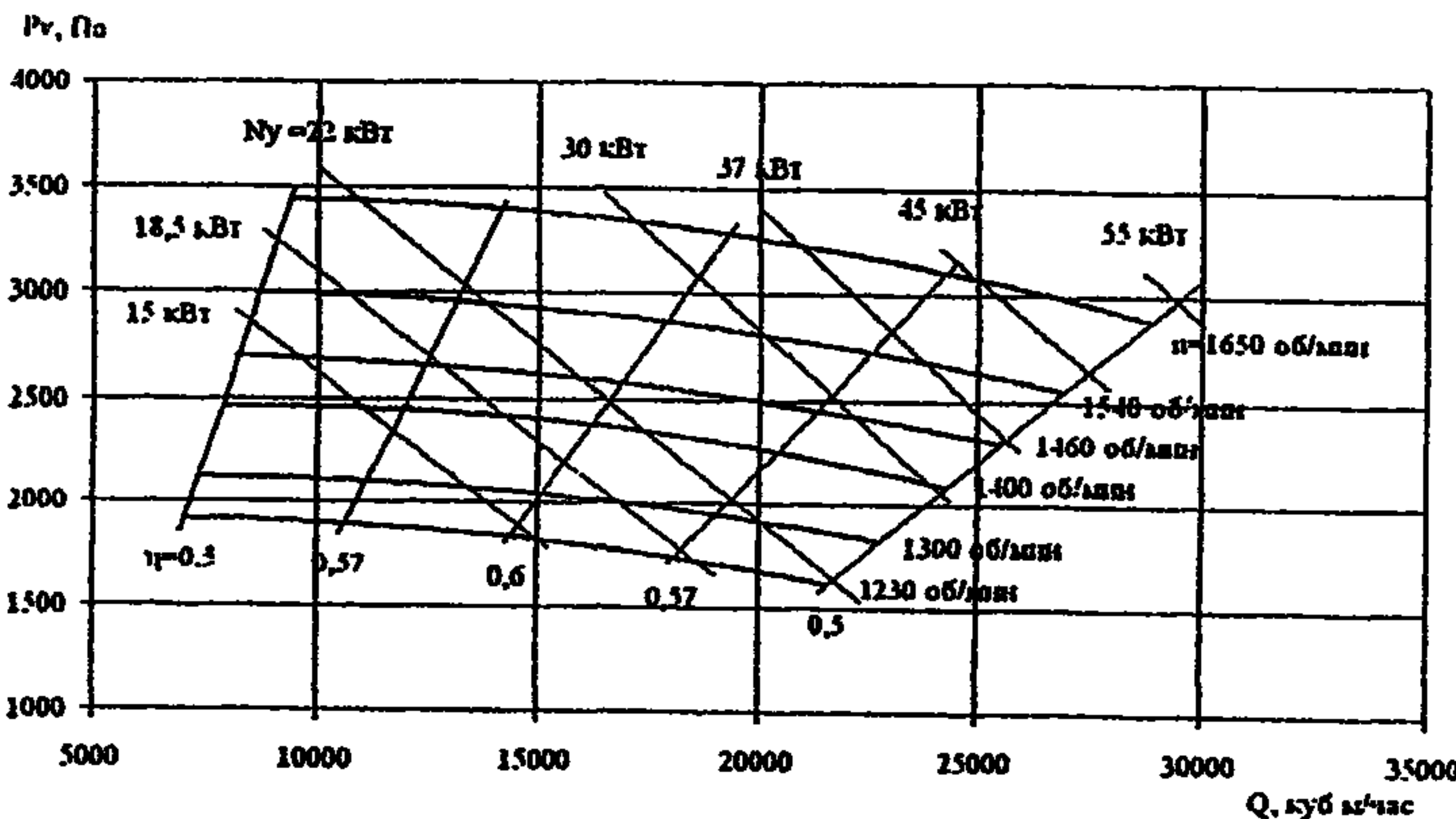
Аэродинамическая характеристика вентилятора ВРП-115-49-8.
