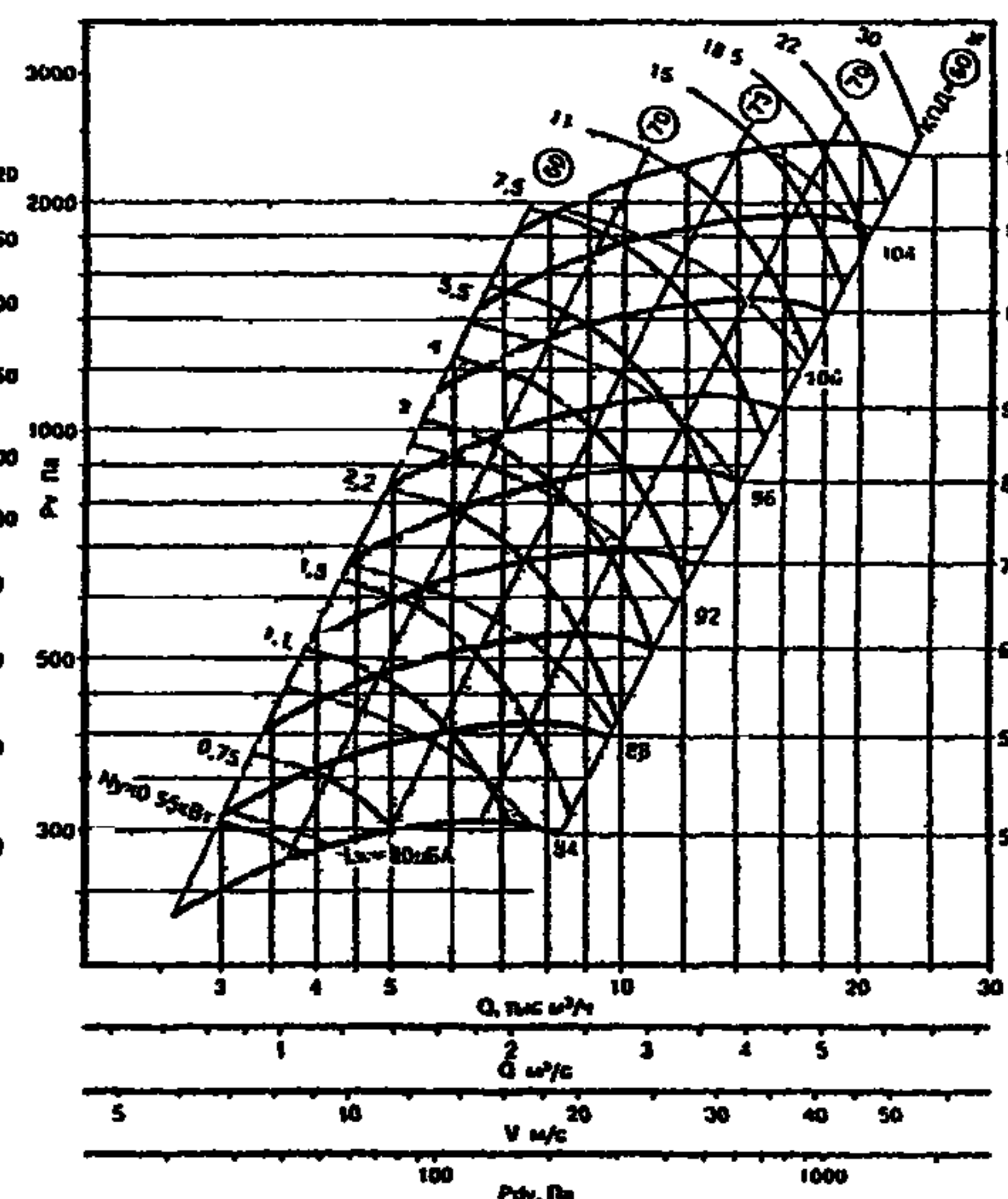
ВЦ 14-46-5 исполнение 5
