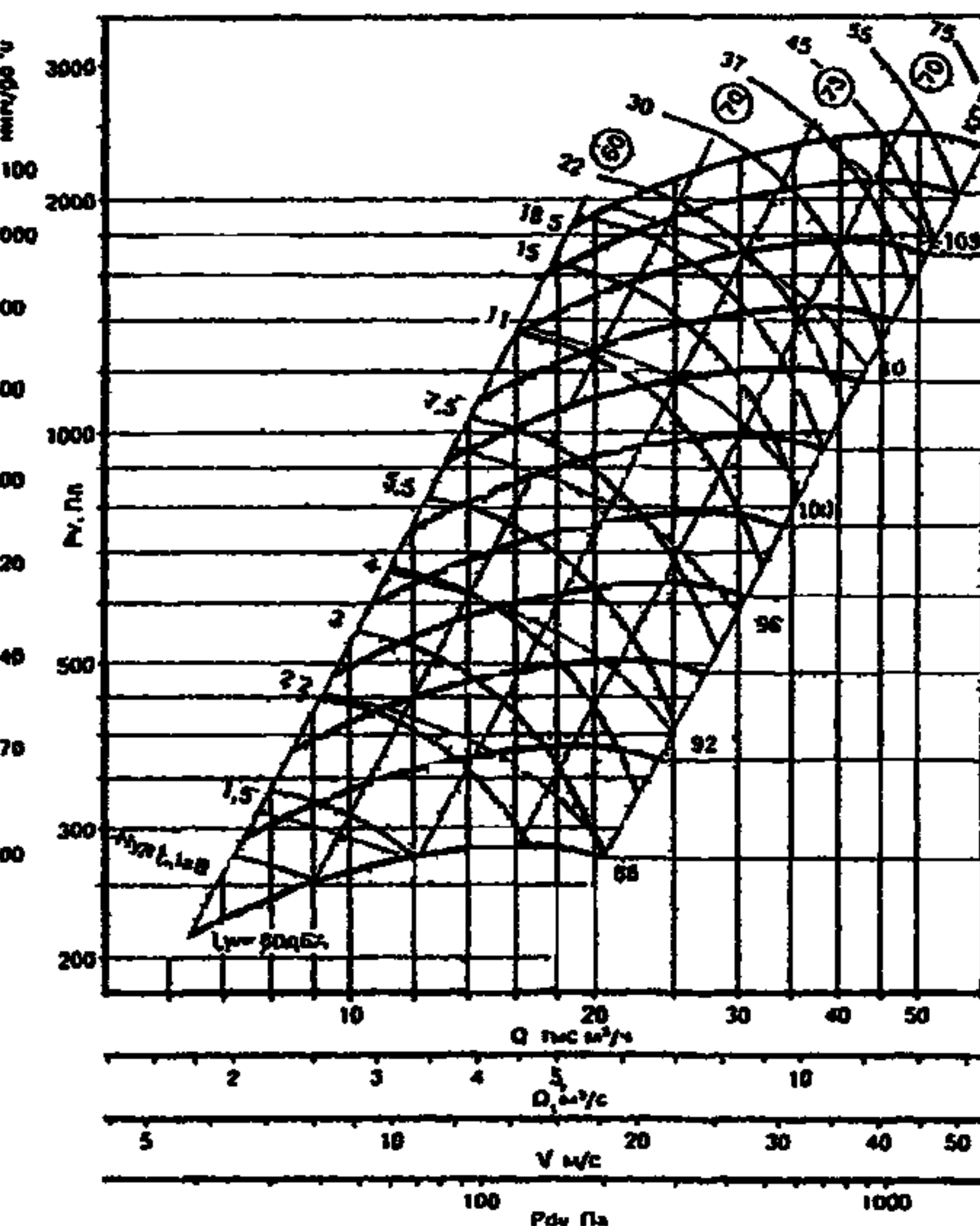
ВЦ 14-46-8 исполнение 5
