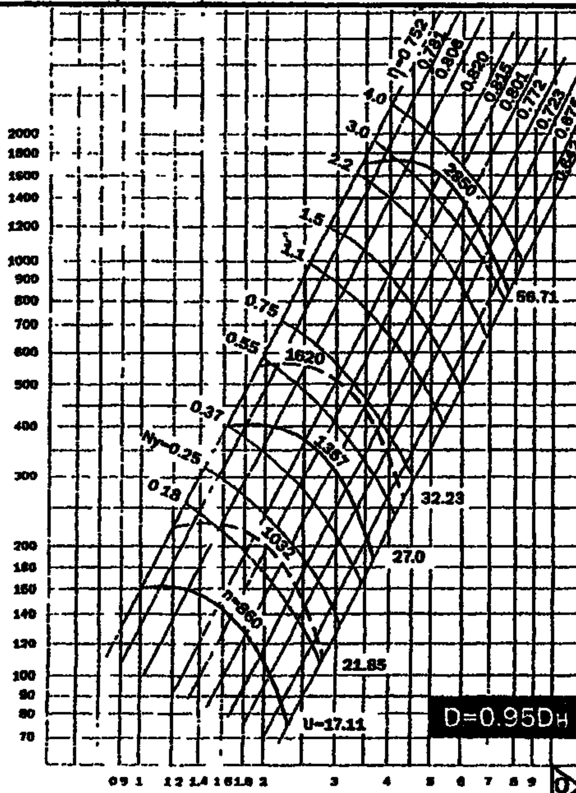
Аэродинамические характеристики вентилятора ВР-88-72-6.3
