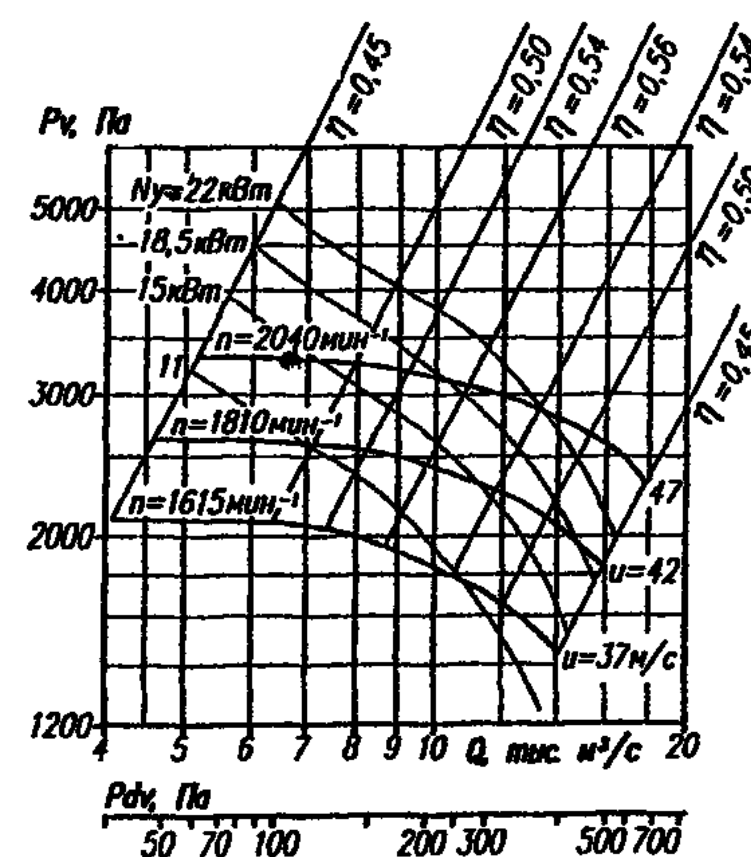
Аэродинамическая характеристика вентилятора ВР 140-40 № 6,3
