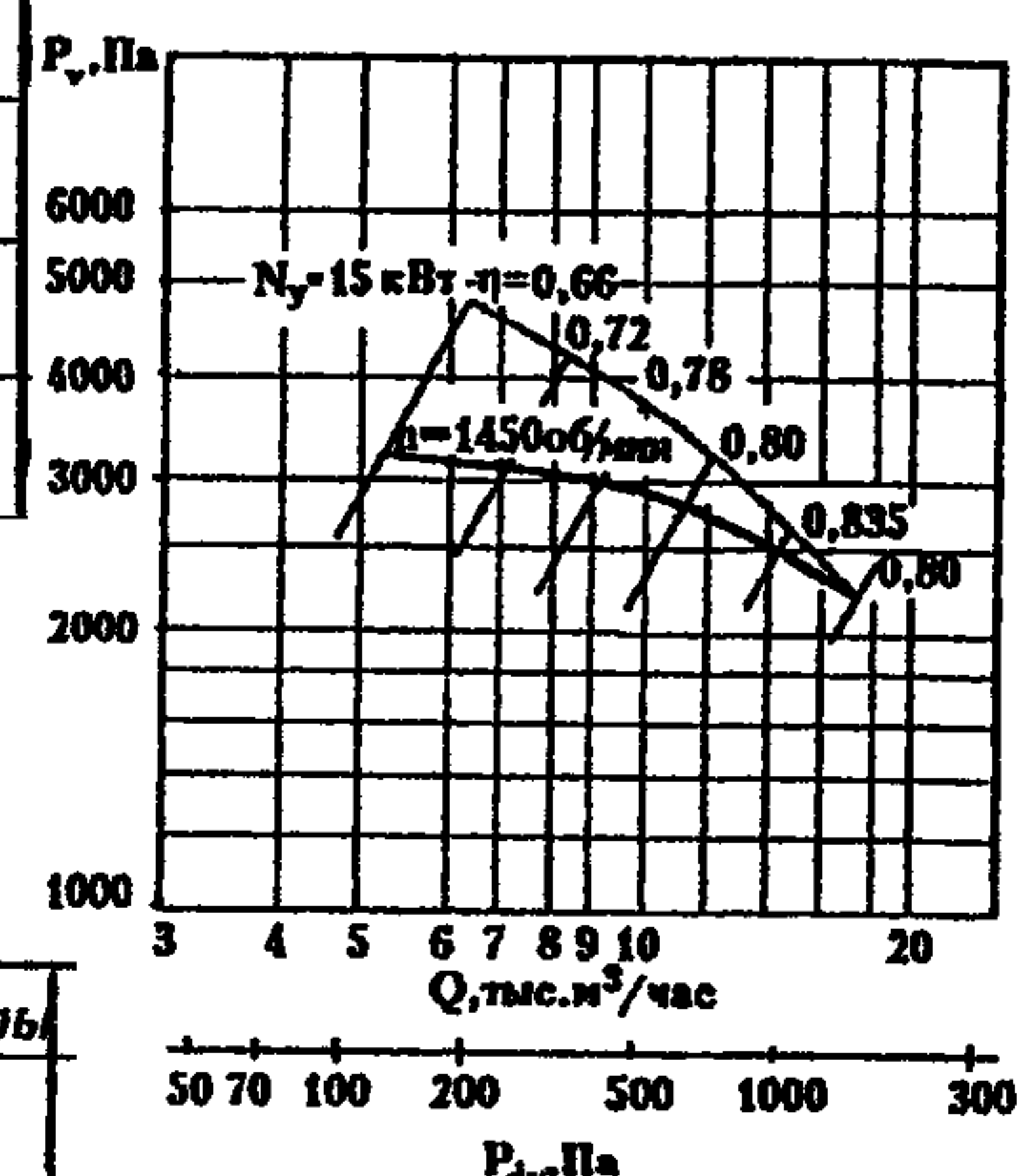
В.Ц5-50-8.02
