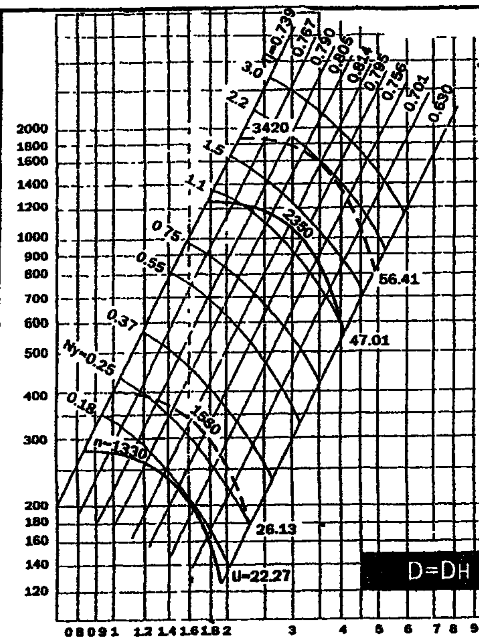
ВР-88-72-3.15
