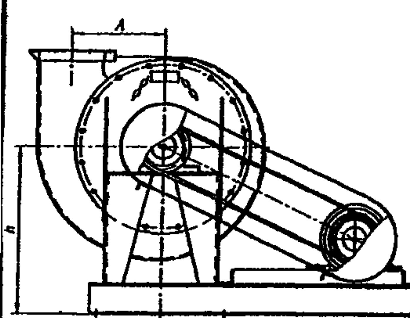
Расположение отверстий для крепления вентилятора
