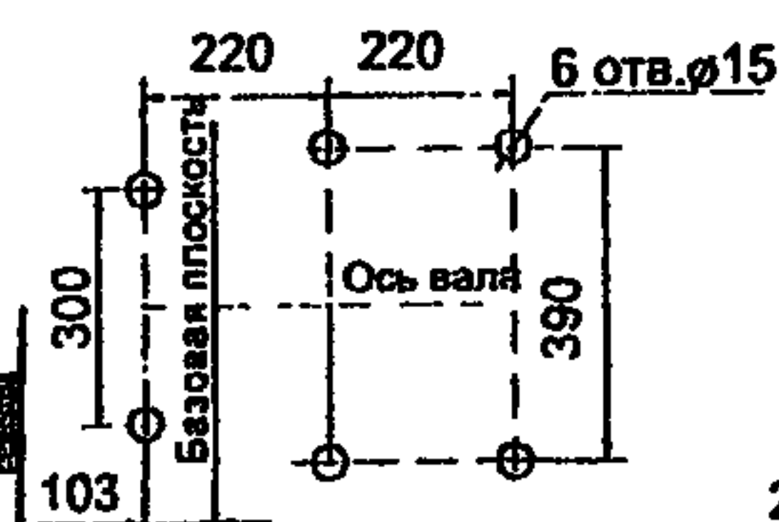
ВР132-30-5-02
