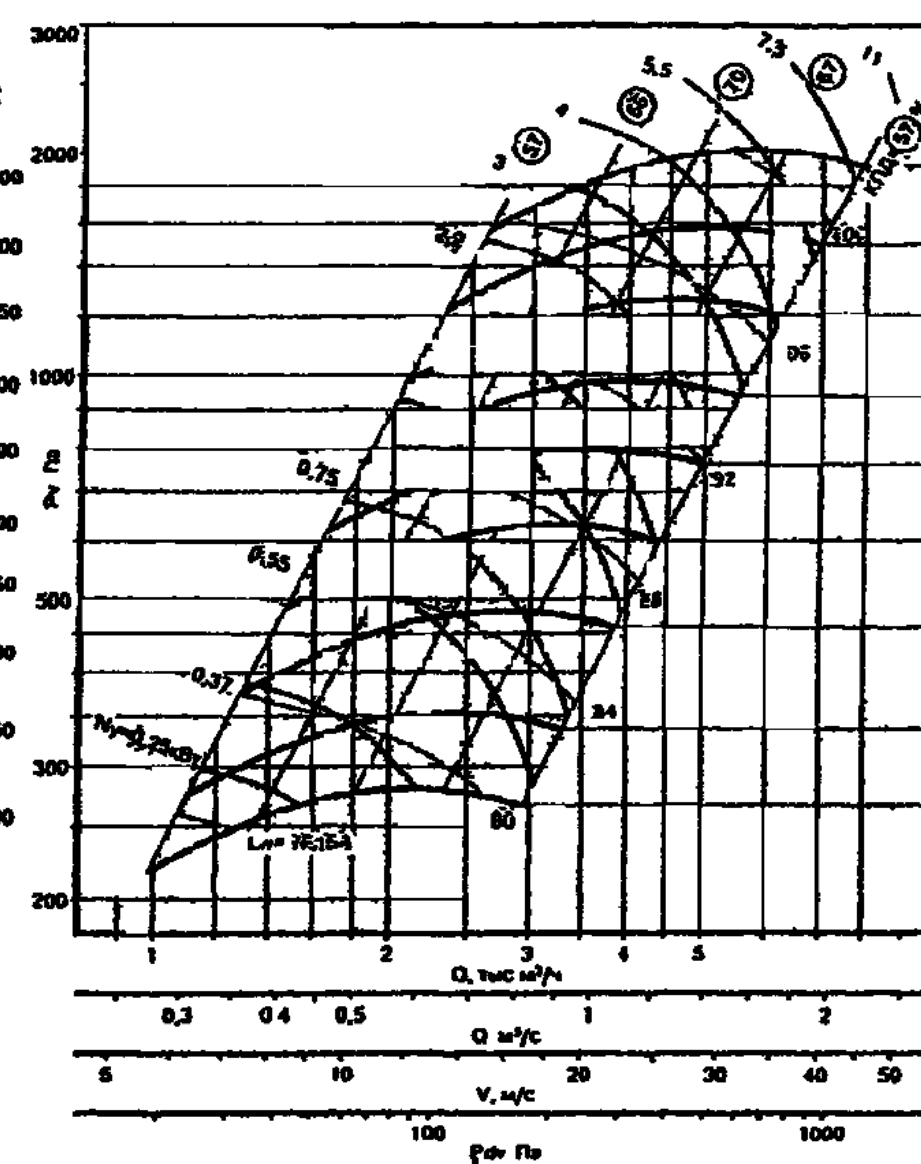
ВЦ 14-46-3,15 исполнение 5
