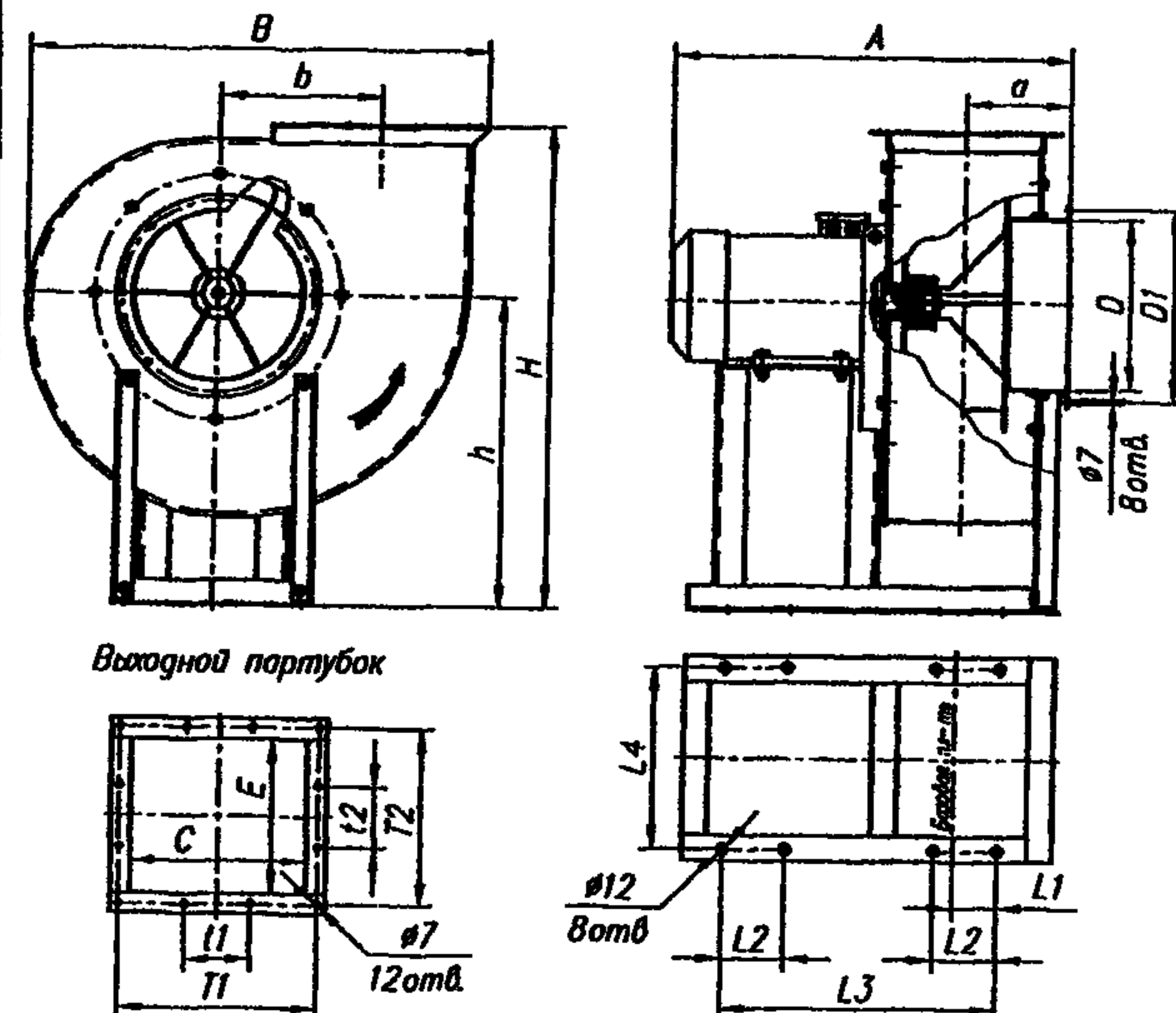
Габаритные и присоединительные размеры вентилятора ВР 140-40 №2,5-4.
