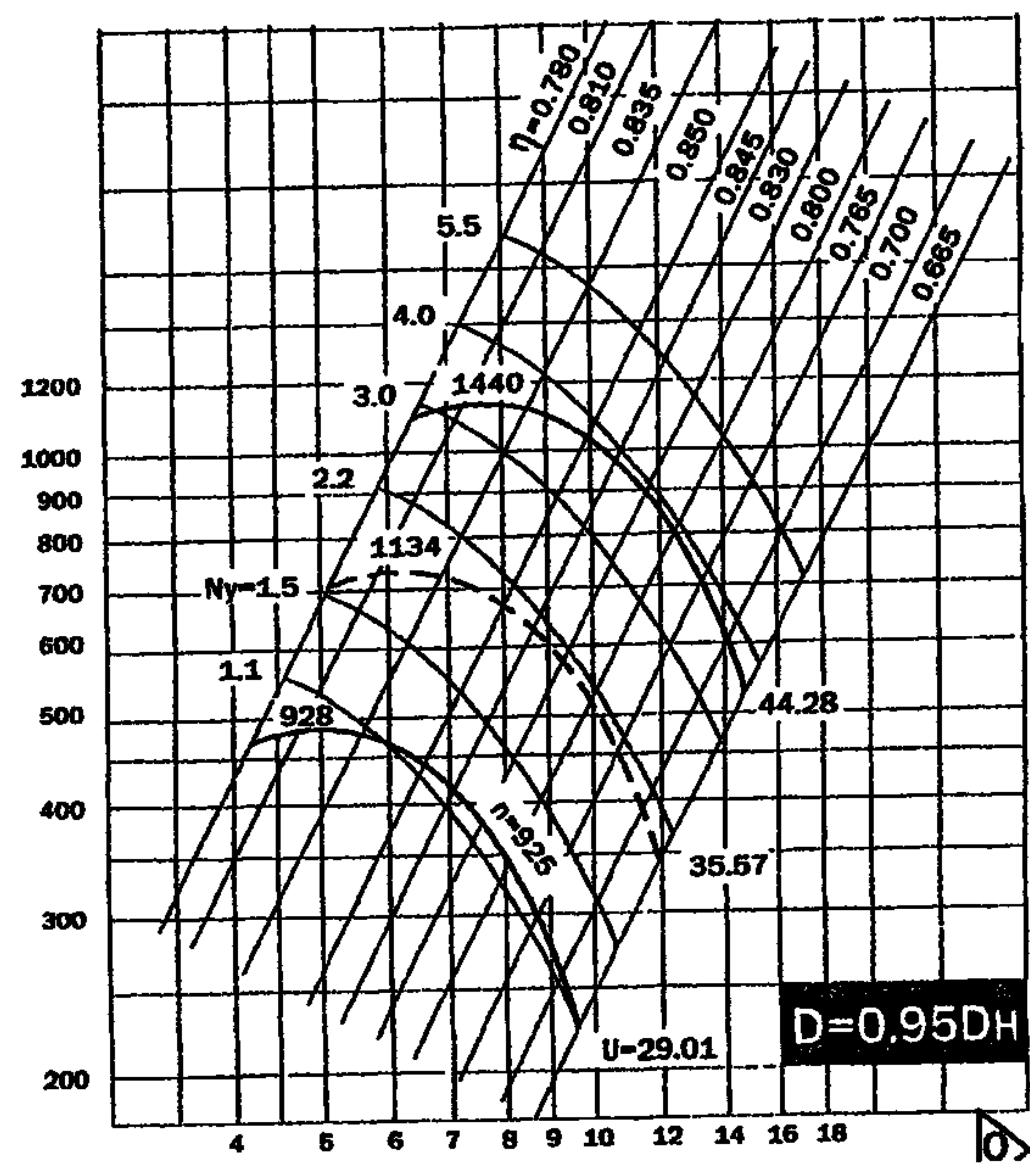
Аэродинамические характеристики вентилятора ВР-88-72-6.3
