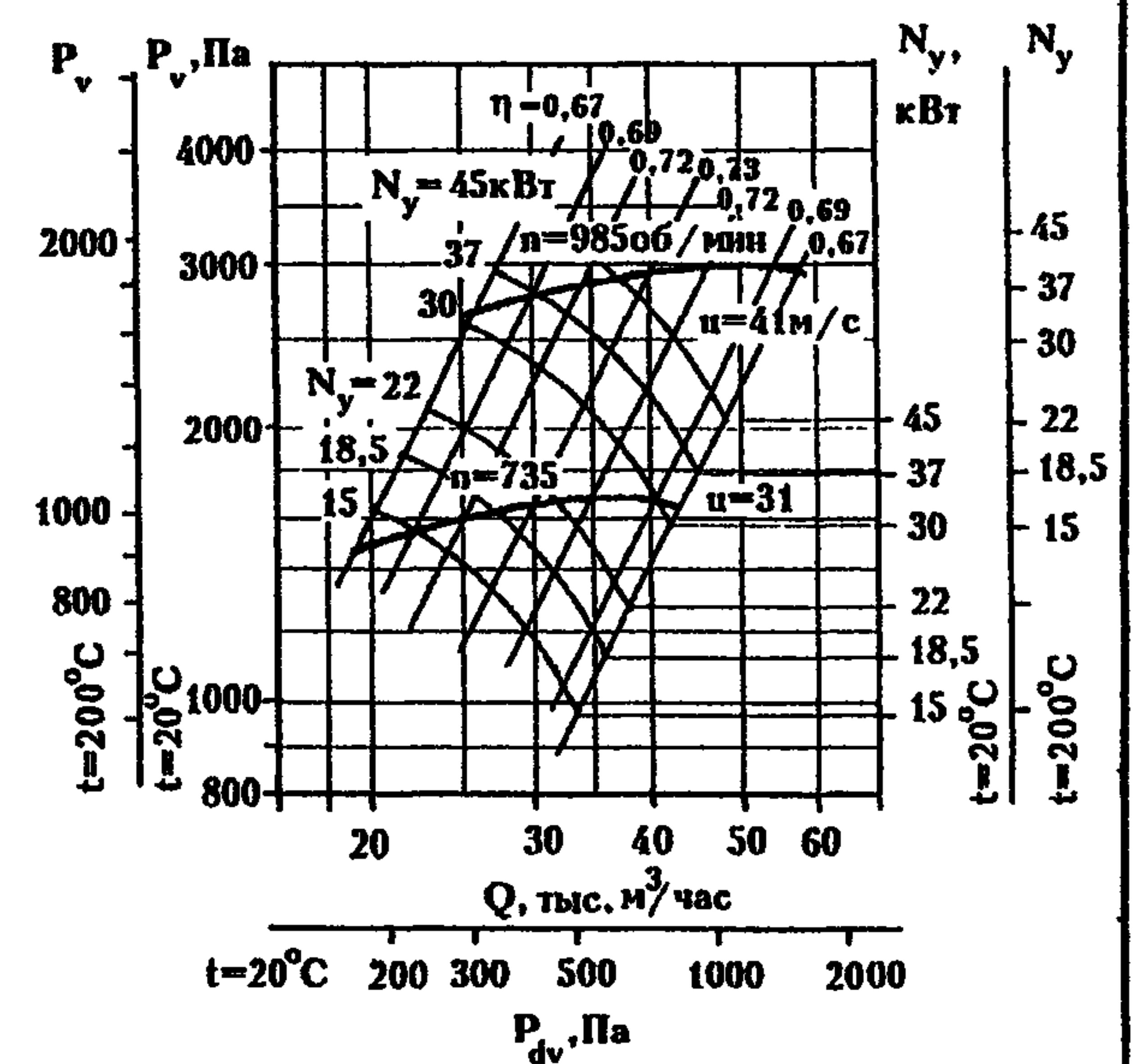
В-Ц14-46-8
