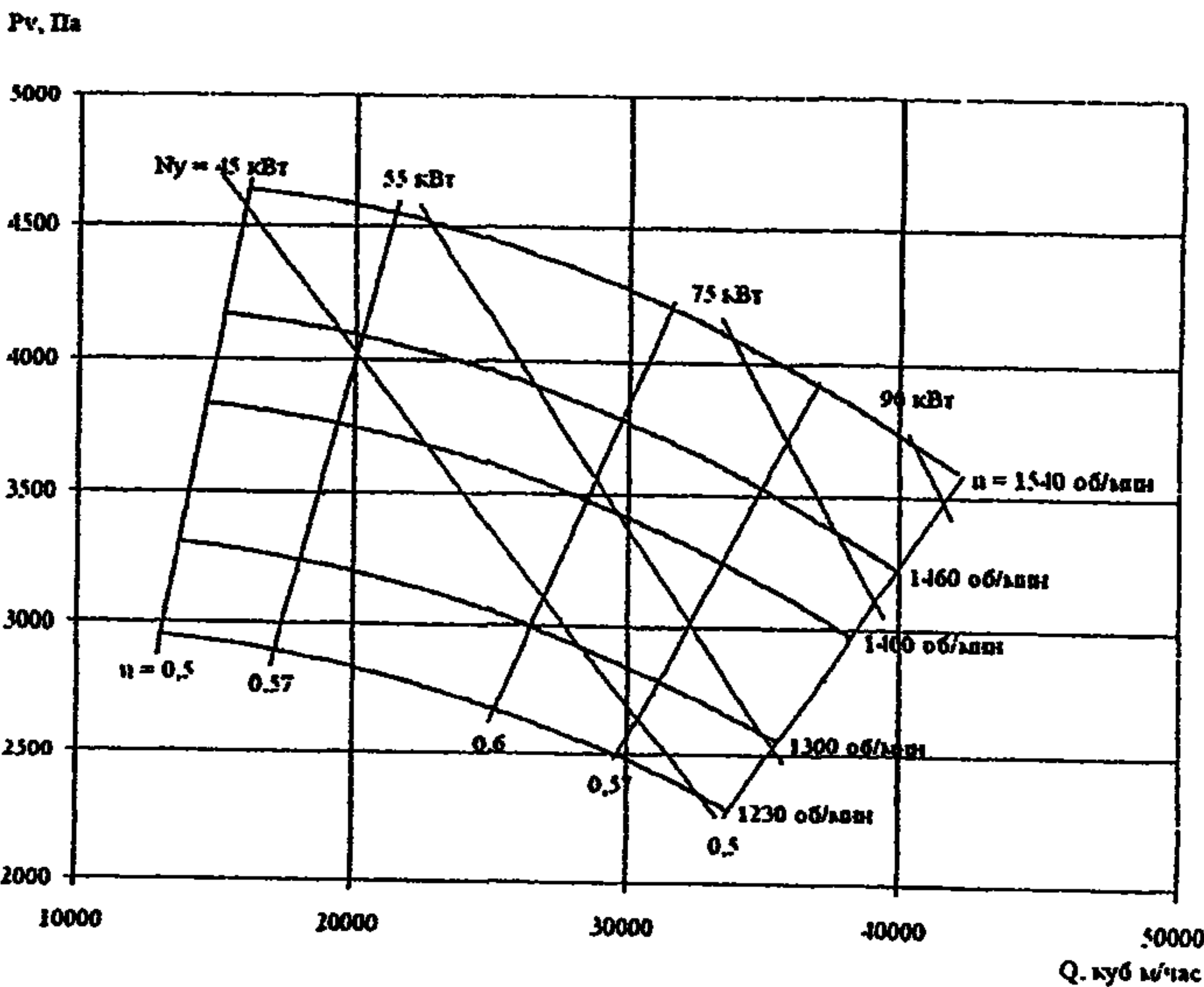
Аэродинамическая характеристика вентилятора ВРП-100-45-10
