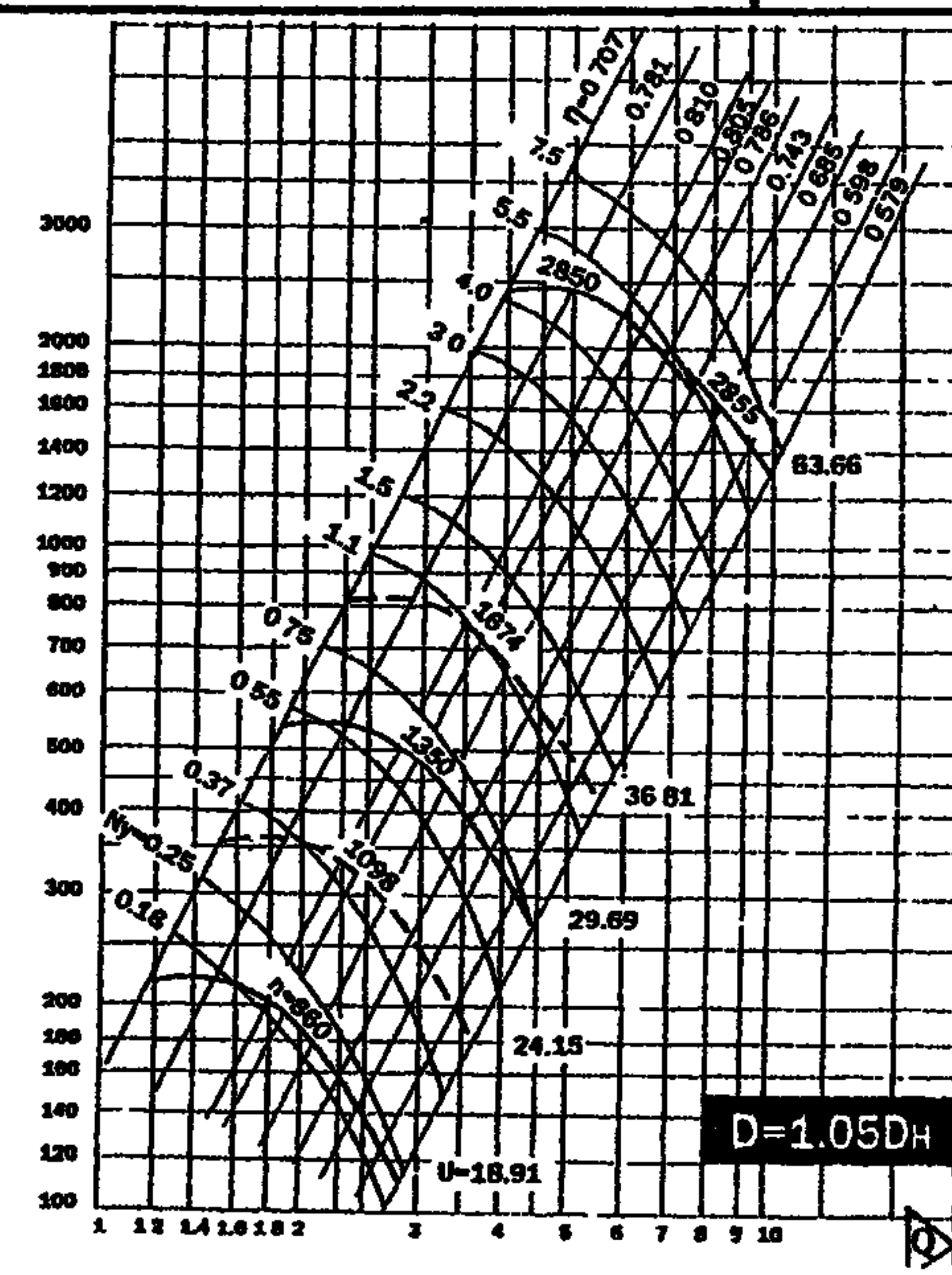
Аэродинамические характеристики вентилятора ВР-88-72-6.3
