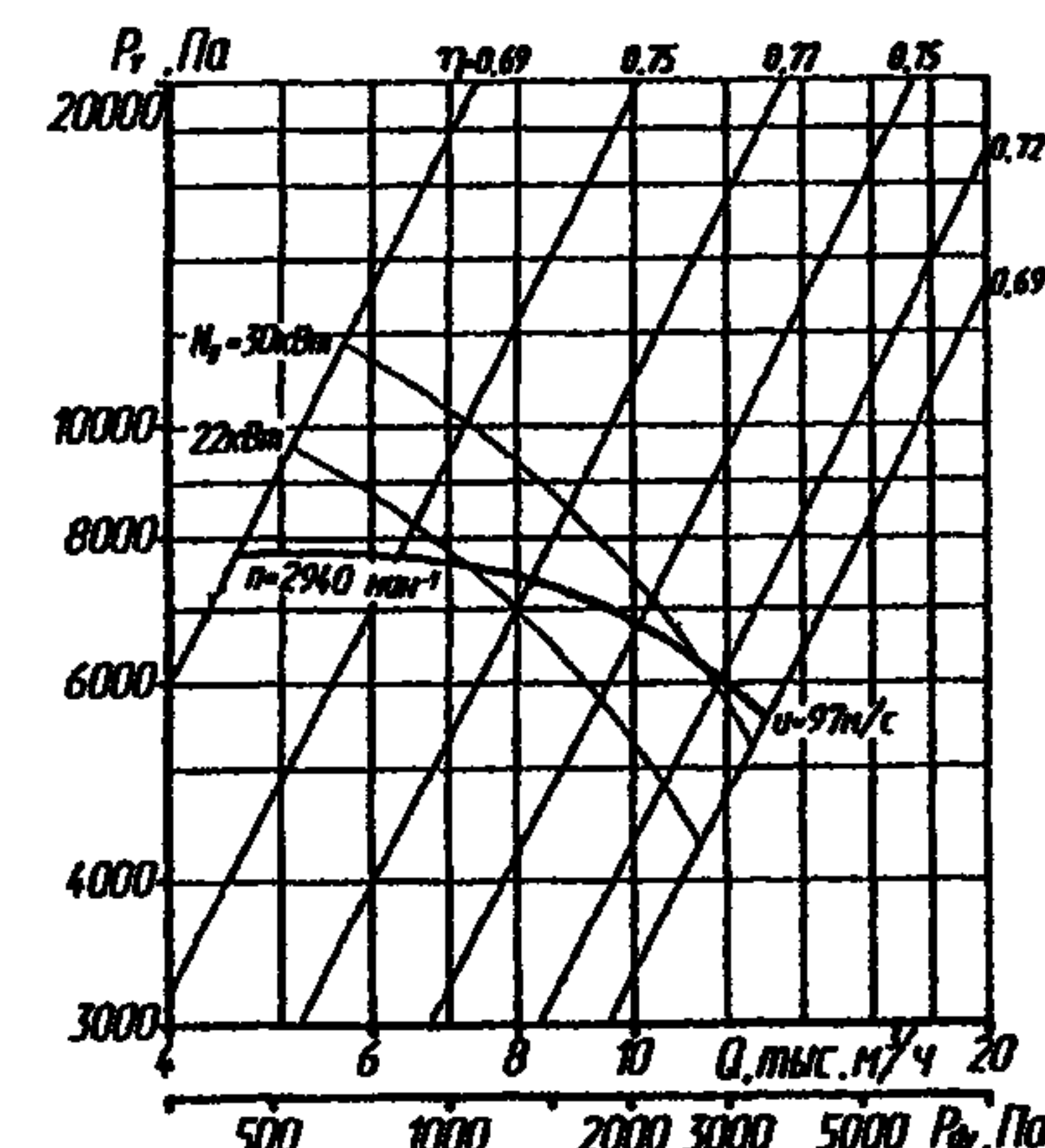
Аэродинамическая характеристика ВР 132-30 №6,3 (1 исполнение).
