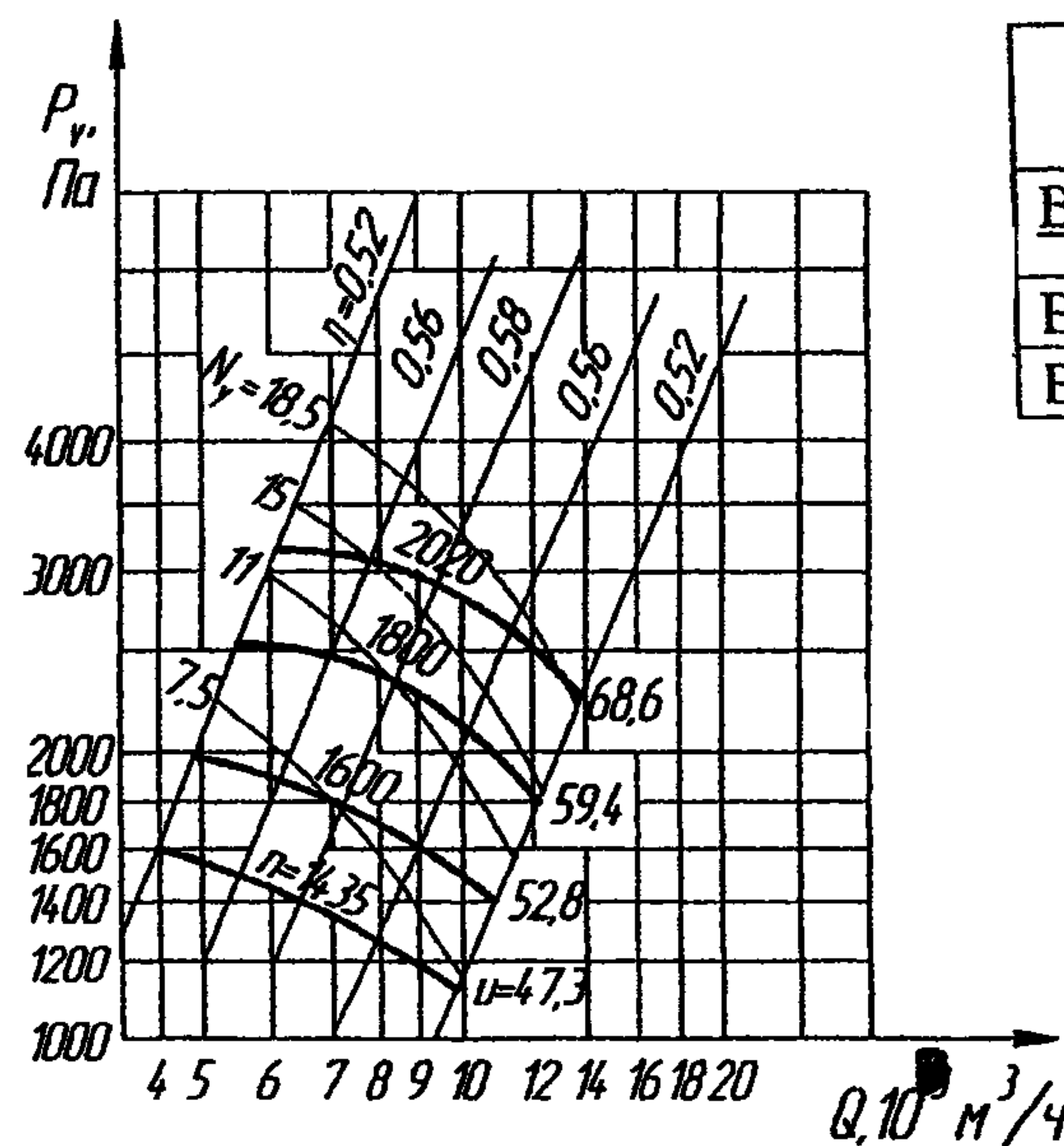
ВРП115-45-6,3
