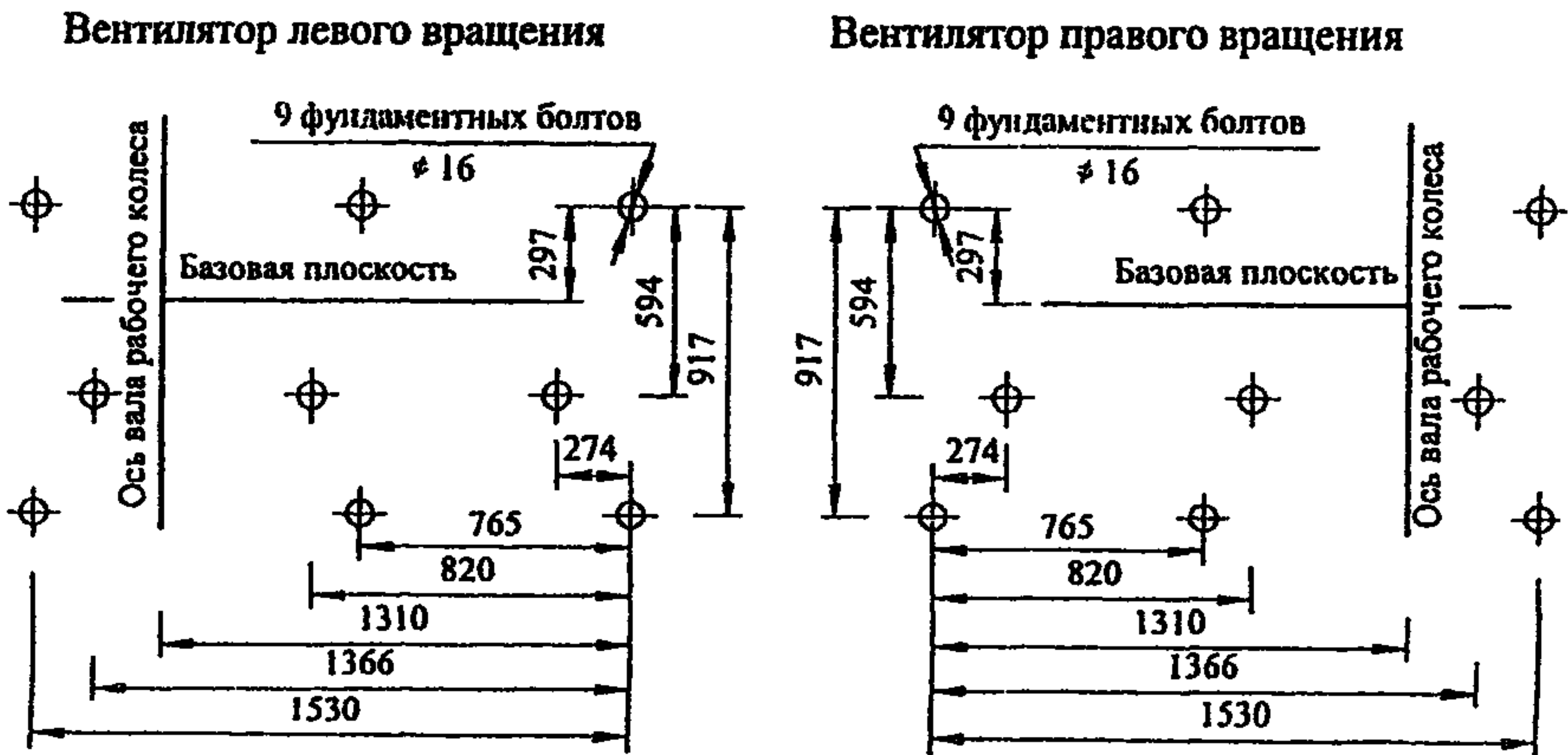
Схема разметки под фундаментные болты вентилятора ВРП-115-49-8.
