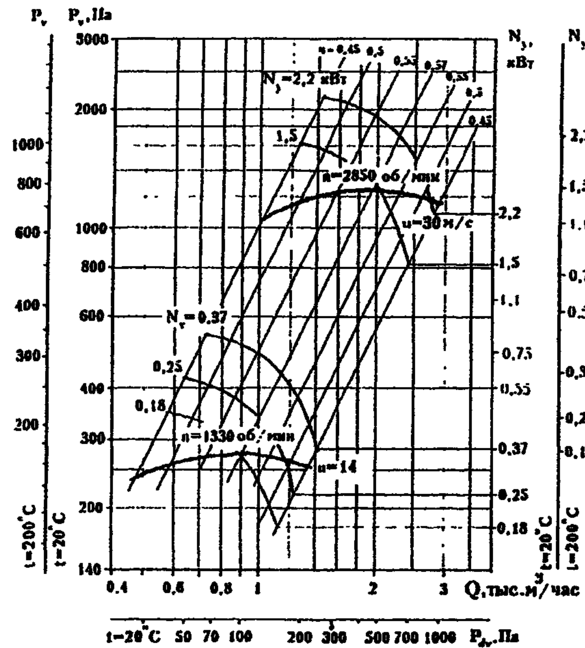
ВР-300-45-3,15
