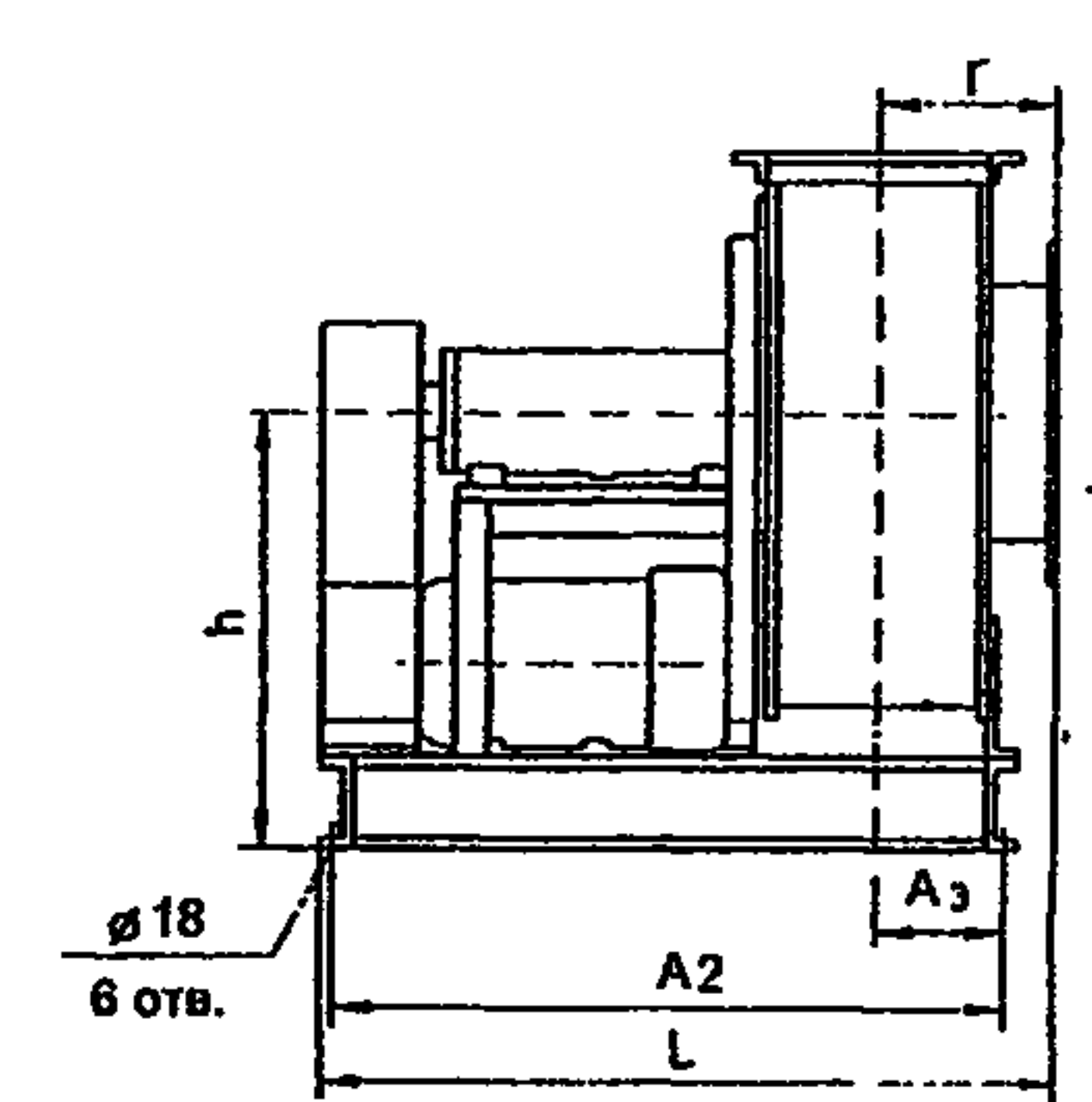
Расположение отверстий для крепления вентилятора
