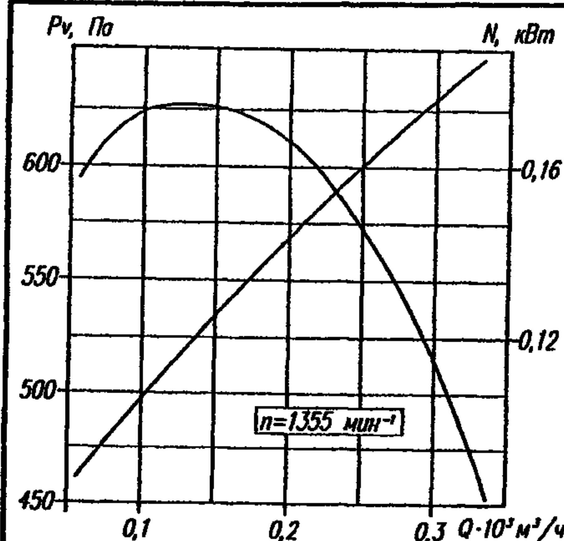
Аэродинамическая характеристика ВР 132-30 №4 (1 исполнение).
