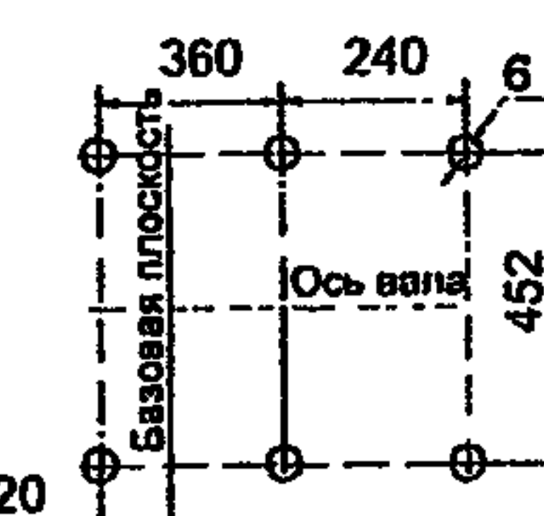
ВР132-30-6,3-02
