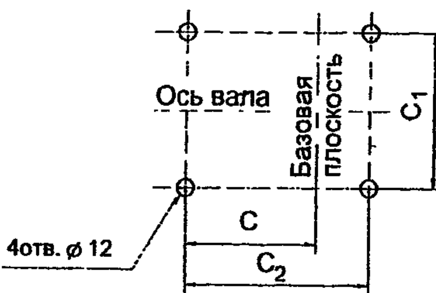
Расположение отверстий для крепления вентилятора ВР-300-45-2,5; -3,15; -4
