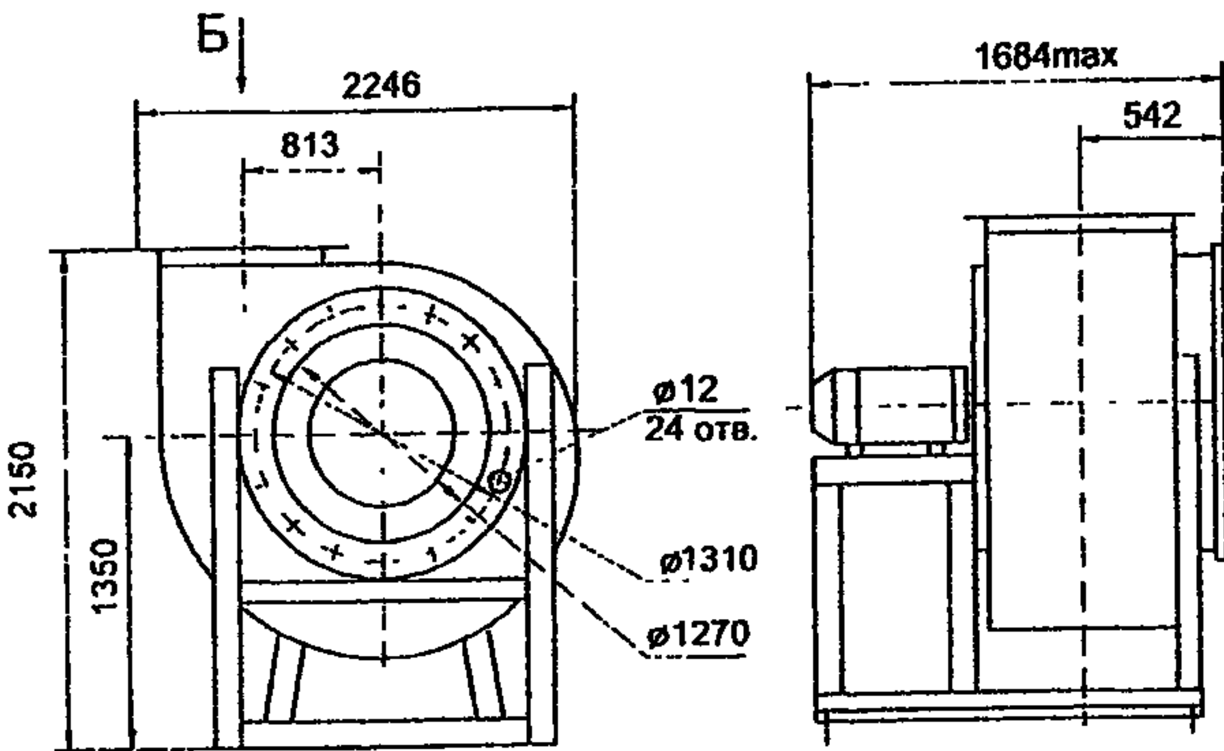
ВР-80-70-12.5-02
