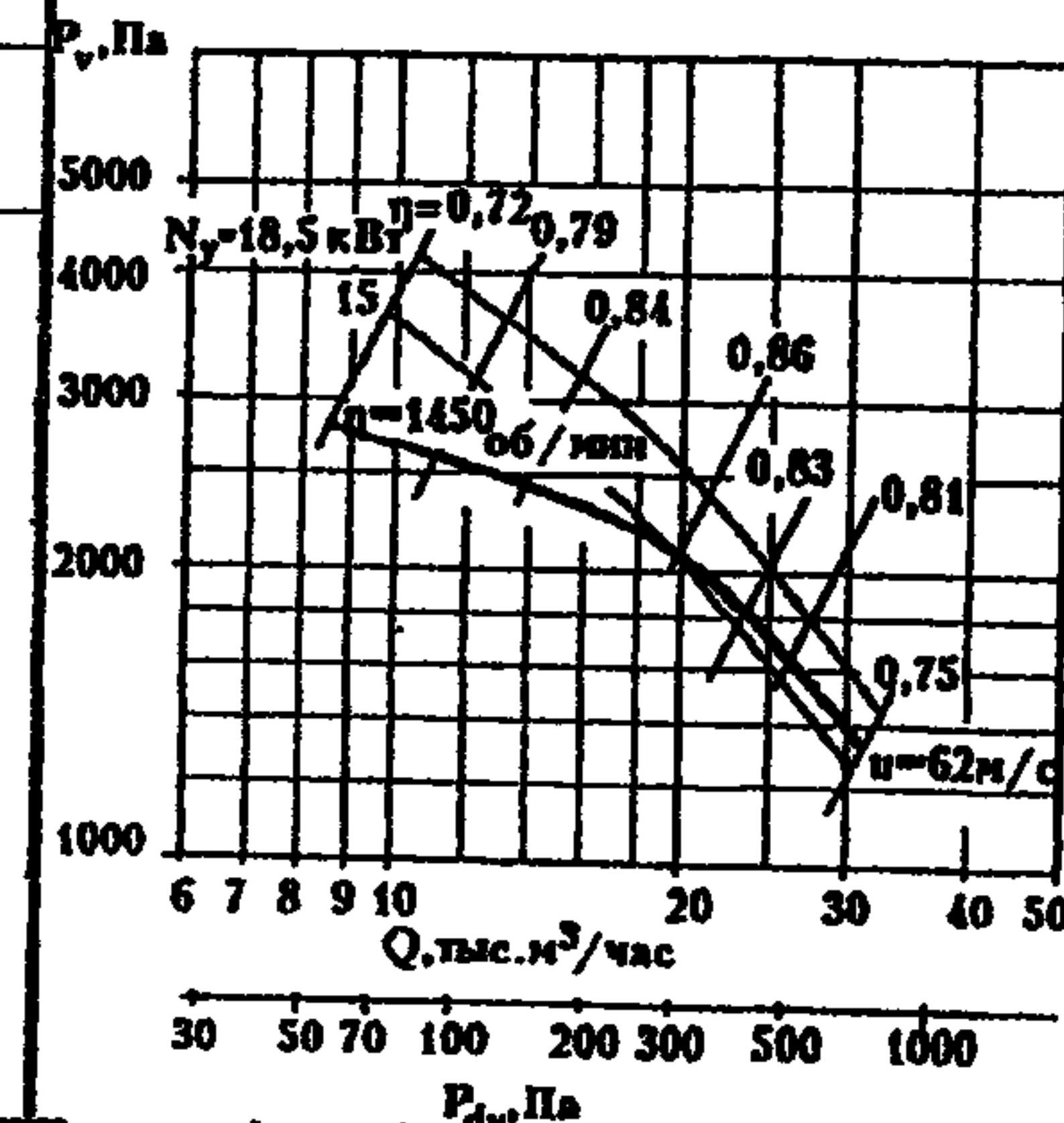
В.Ц5-50-8.02
