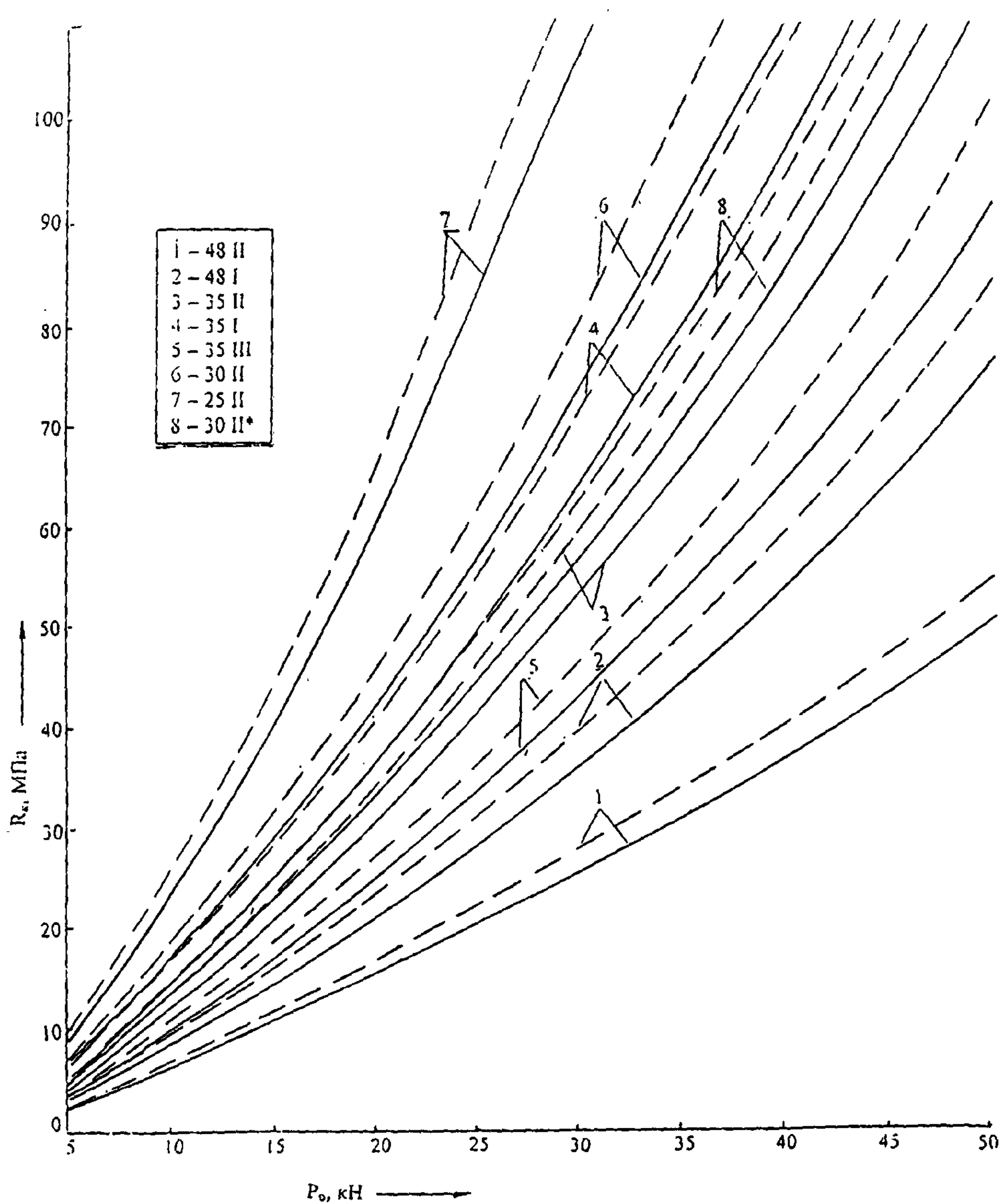
Рис. 3. Расчетные зависимости R_k от P_0 и типа анкера заполнители: • — гранитный • — — — мелкозернистый или гравийный
