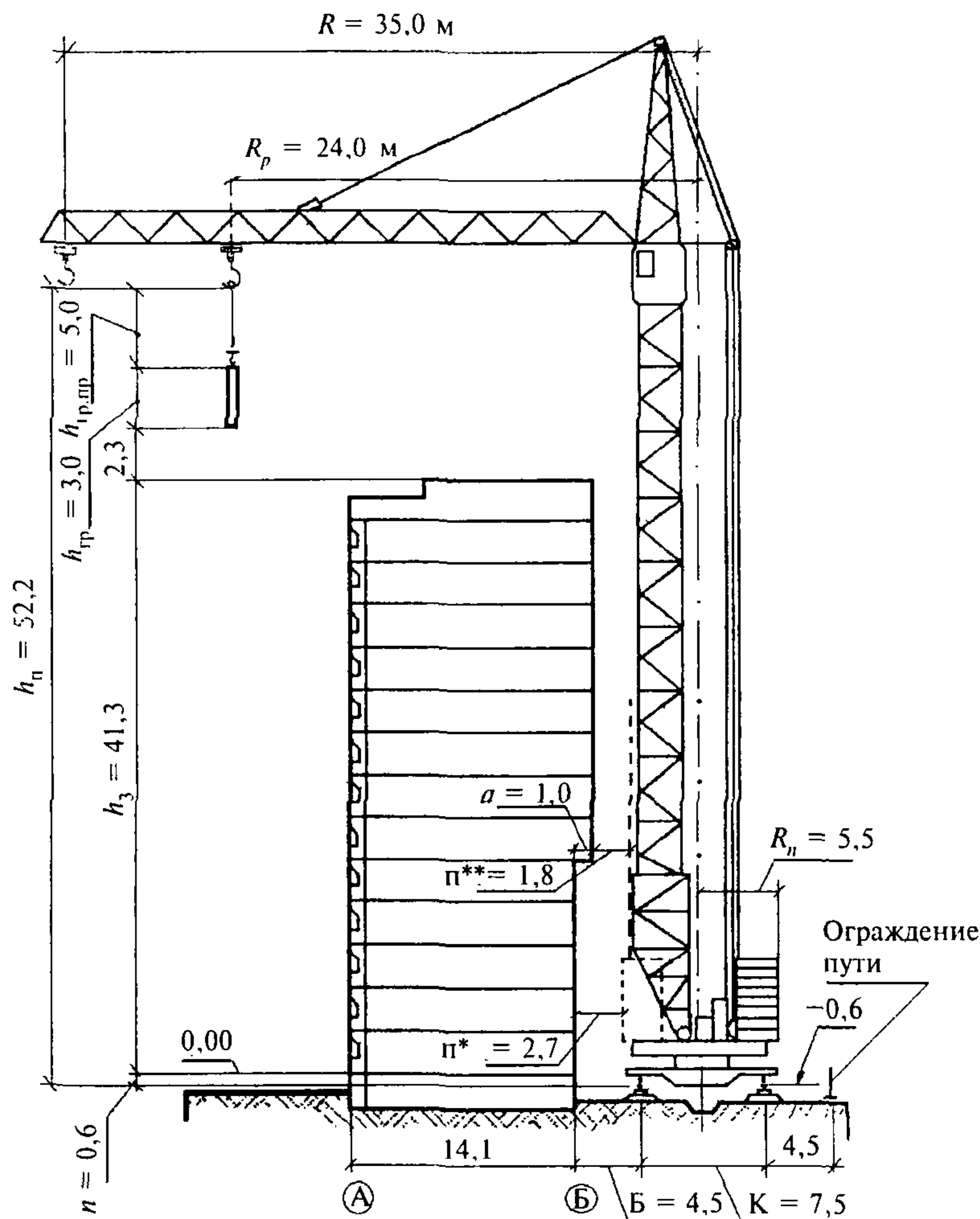
Рисунок 1 — Привязка башенного крана к зданию
