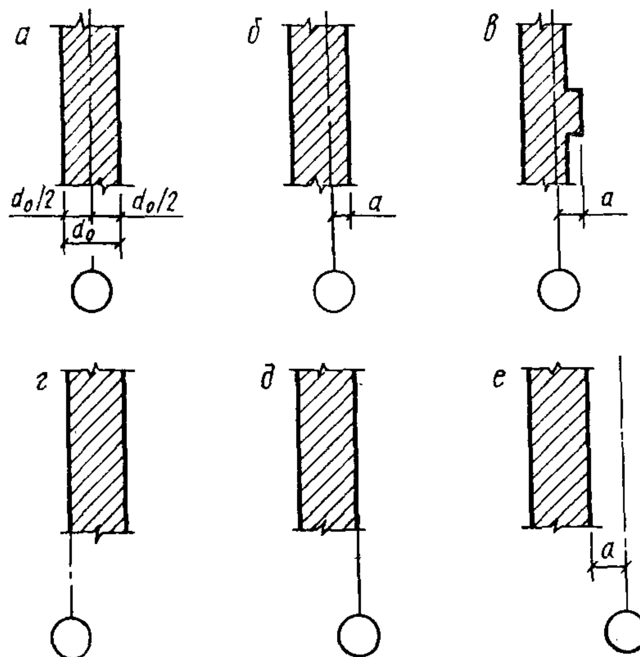
Привязки стен к координационным осям
