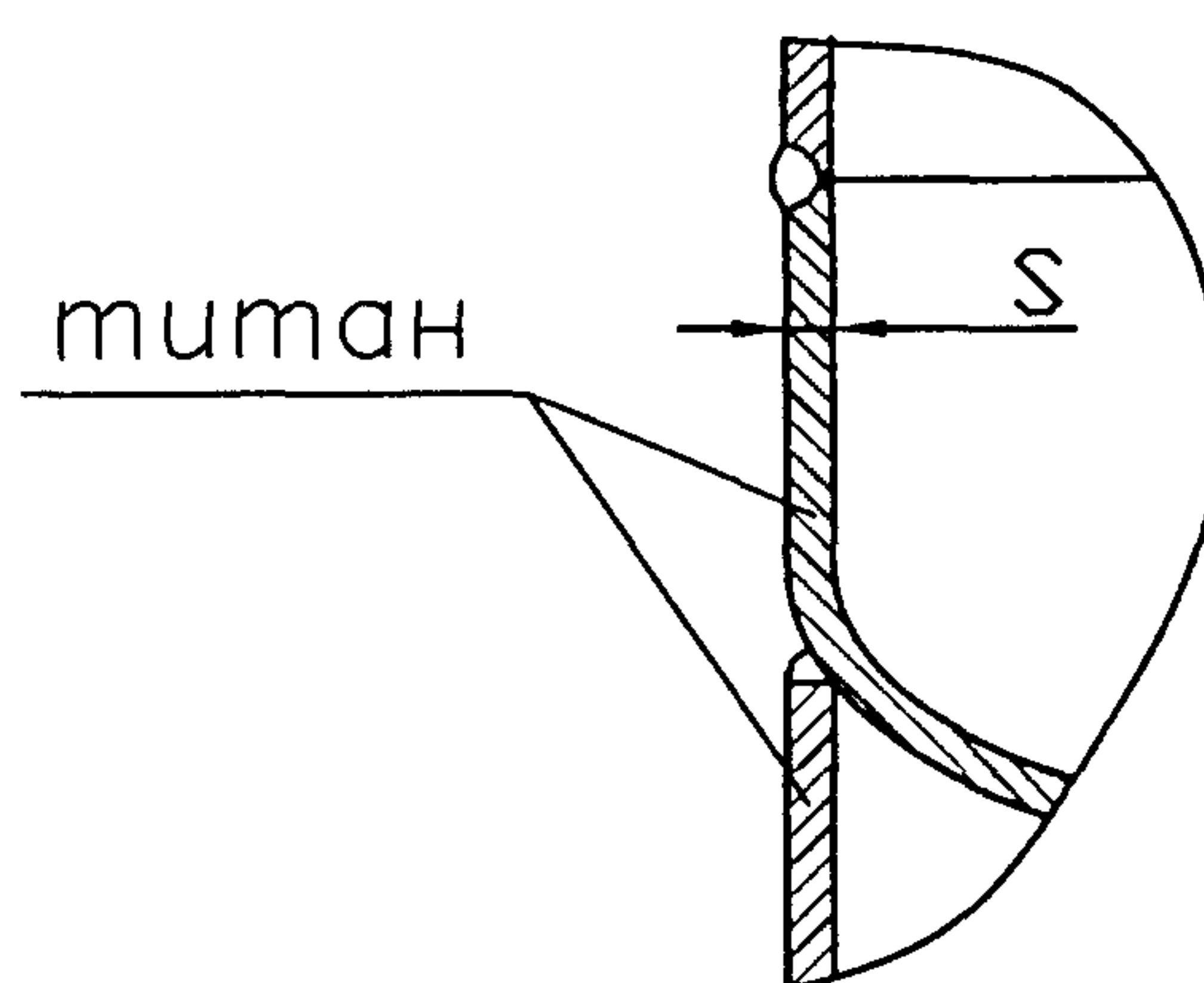
Рисунок 1 – Присоединение переходных элементов
