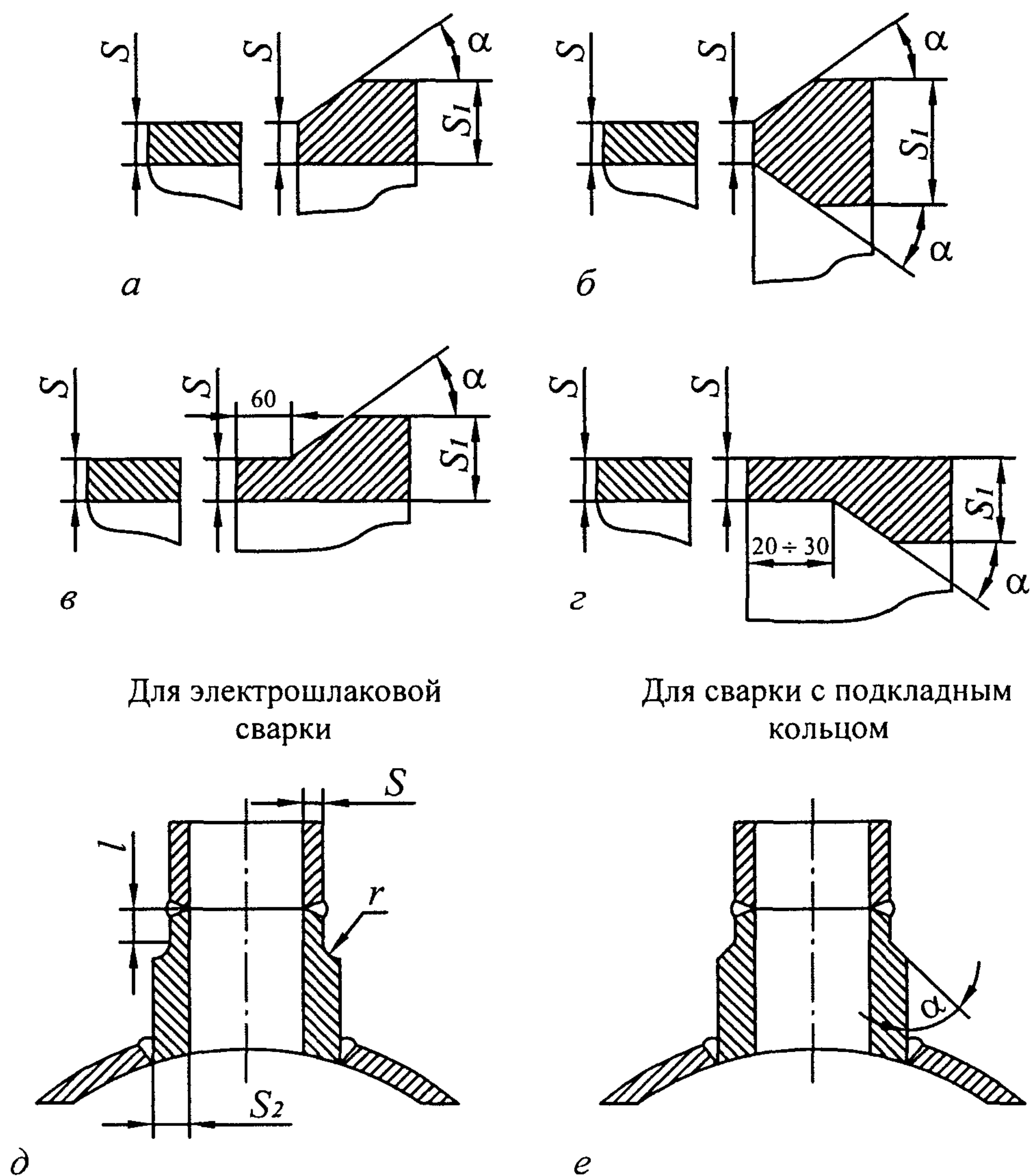
Рисунок 15 – Стыковка элементов разной толщины
