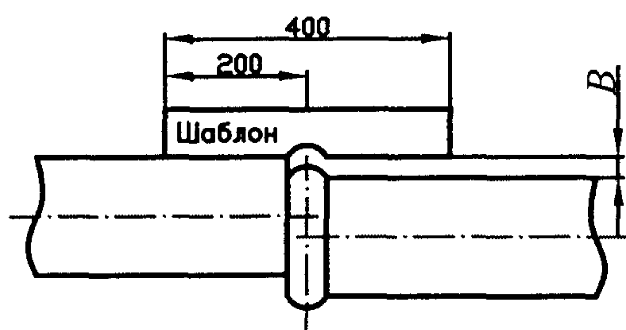
Рисунок 11 – Схема определения смещения кромок стыкуемых труб
