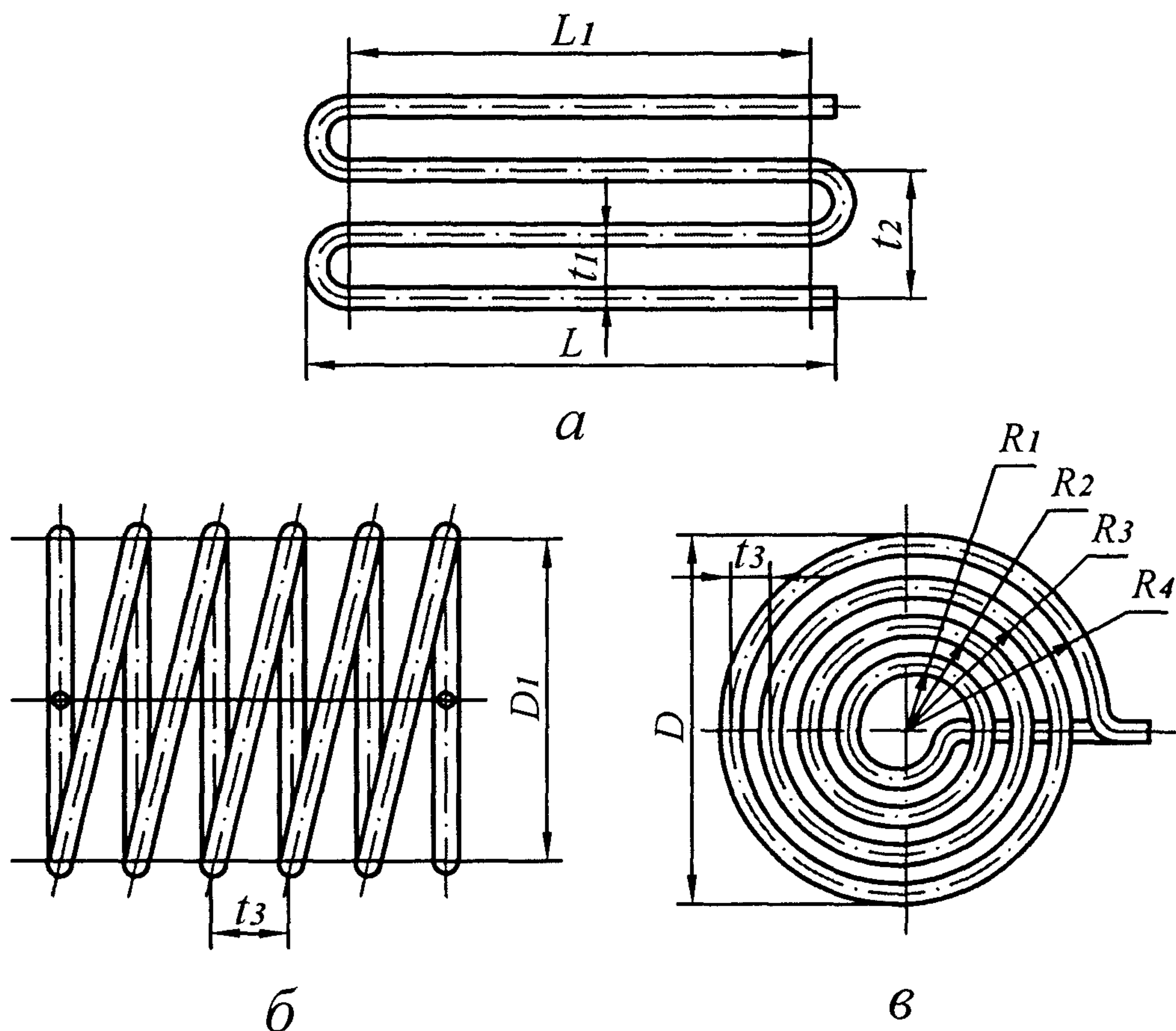
Рисунок 13 – Размеры гнутых змеевиков
