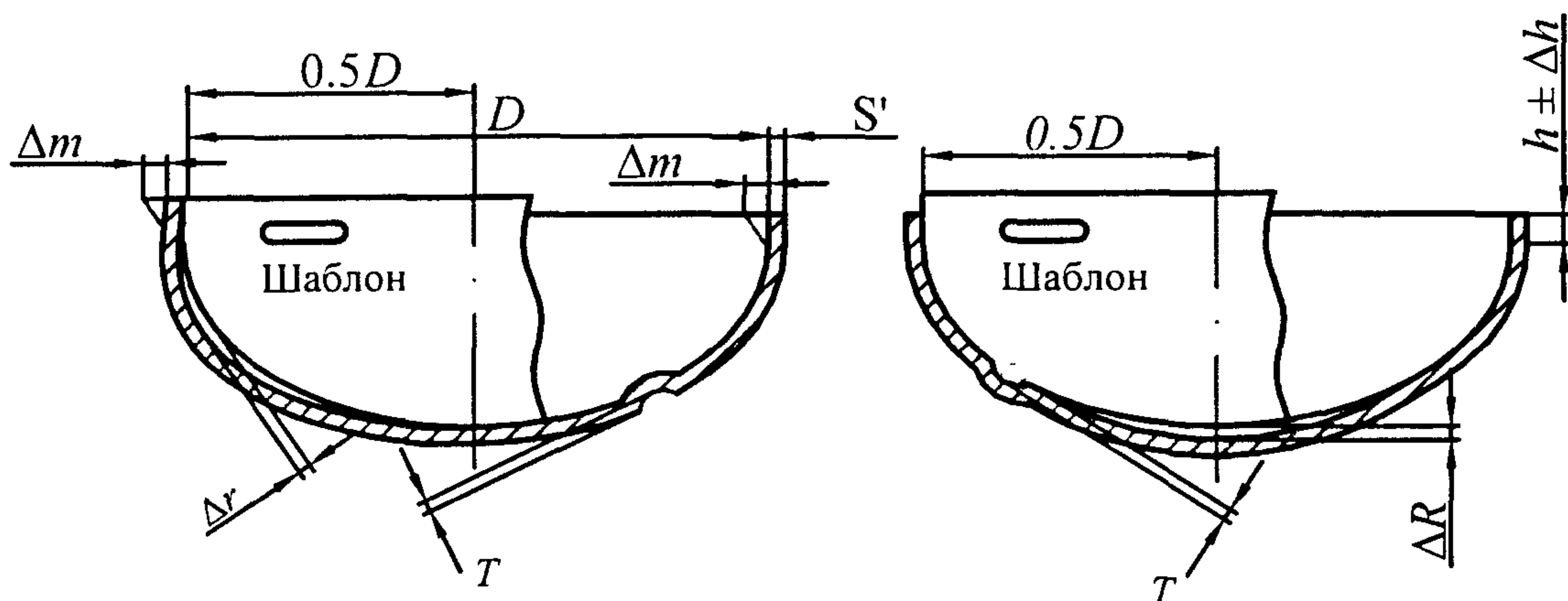
Рисунок 4 – Отклонение размеров и формы эллиптического днища
