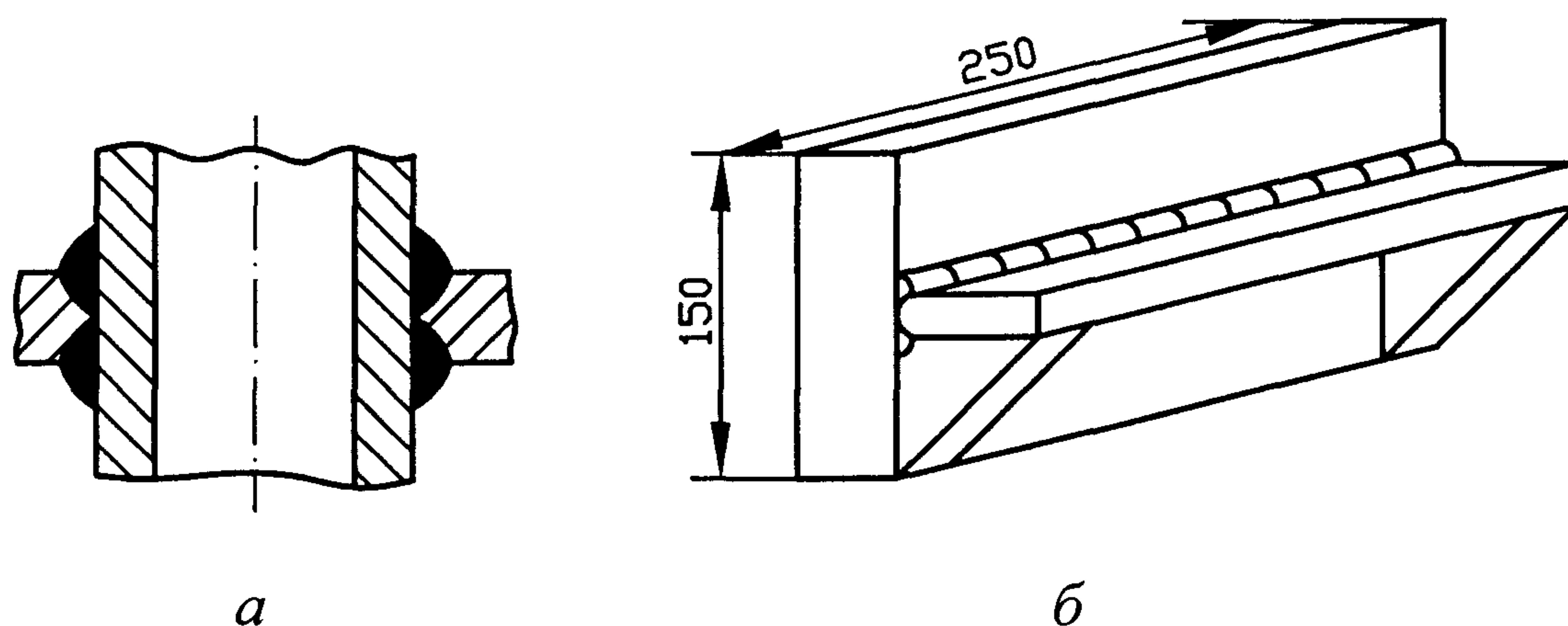
Рисунок 19 – Контрольные сварные соединения для проведения металлографического контроля
