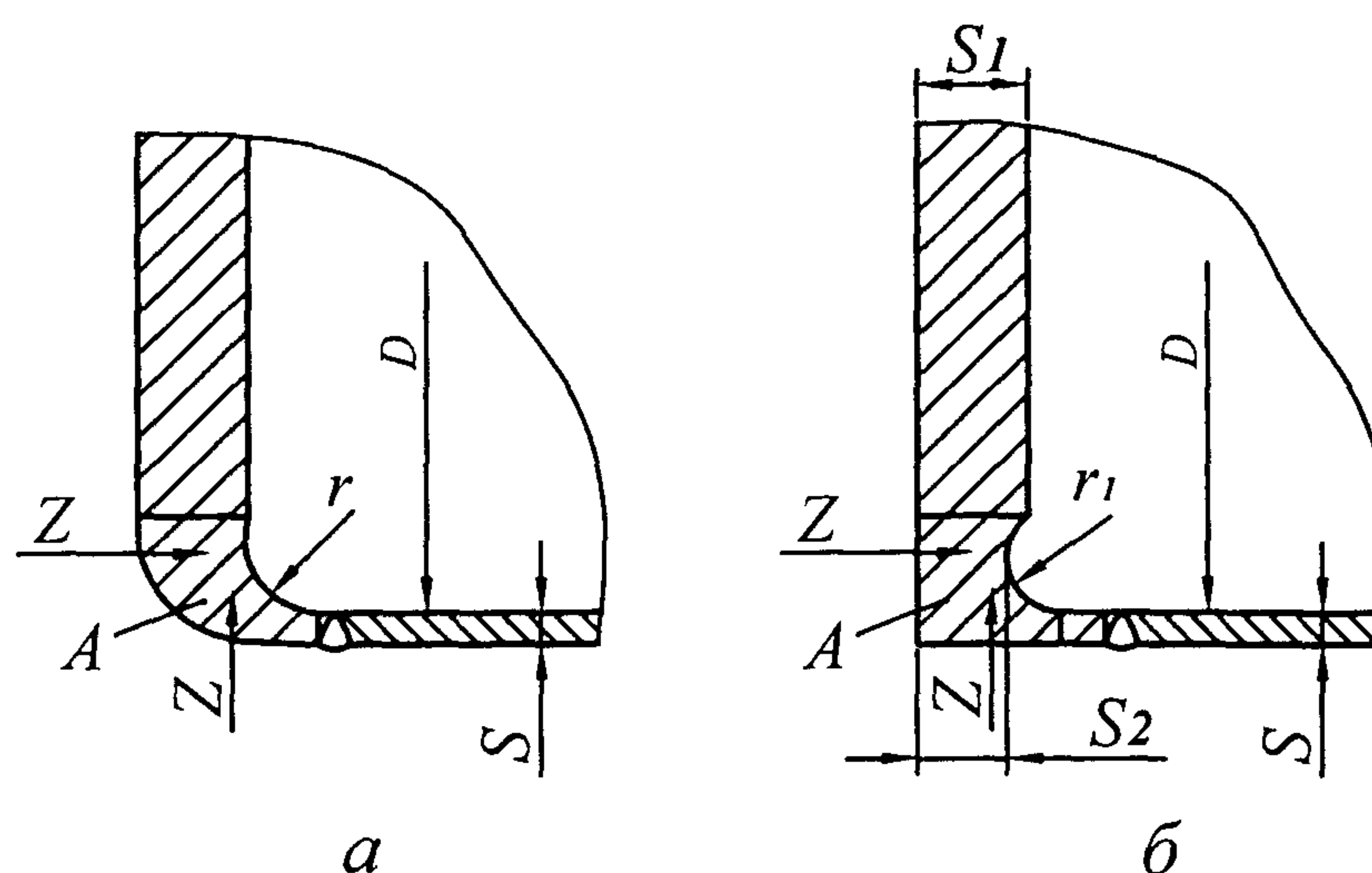
Рисунок 5 – Плоские днища
