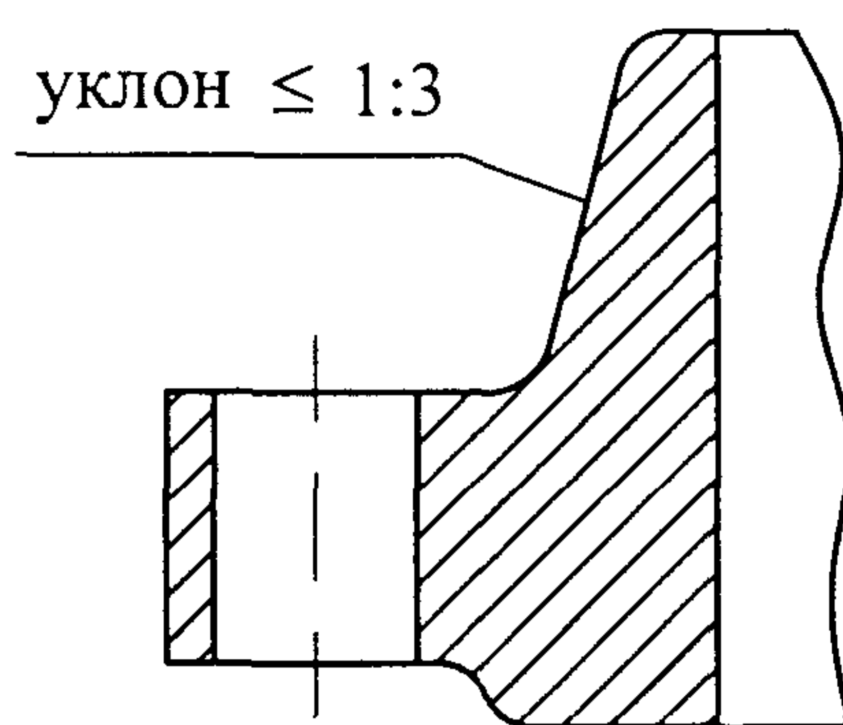
Рисунок 16 – Уклон втулки фланца
