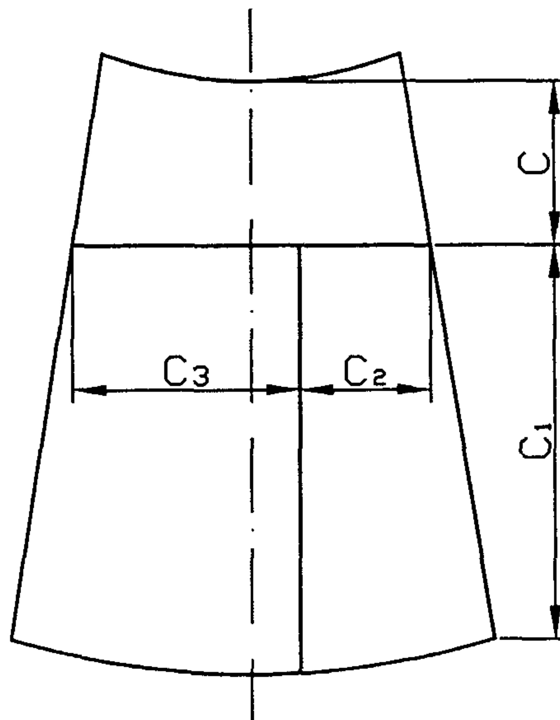
Рисунок 3 – Расположение сварных швов при изготовлении лепестков штамповкой
