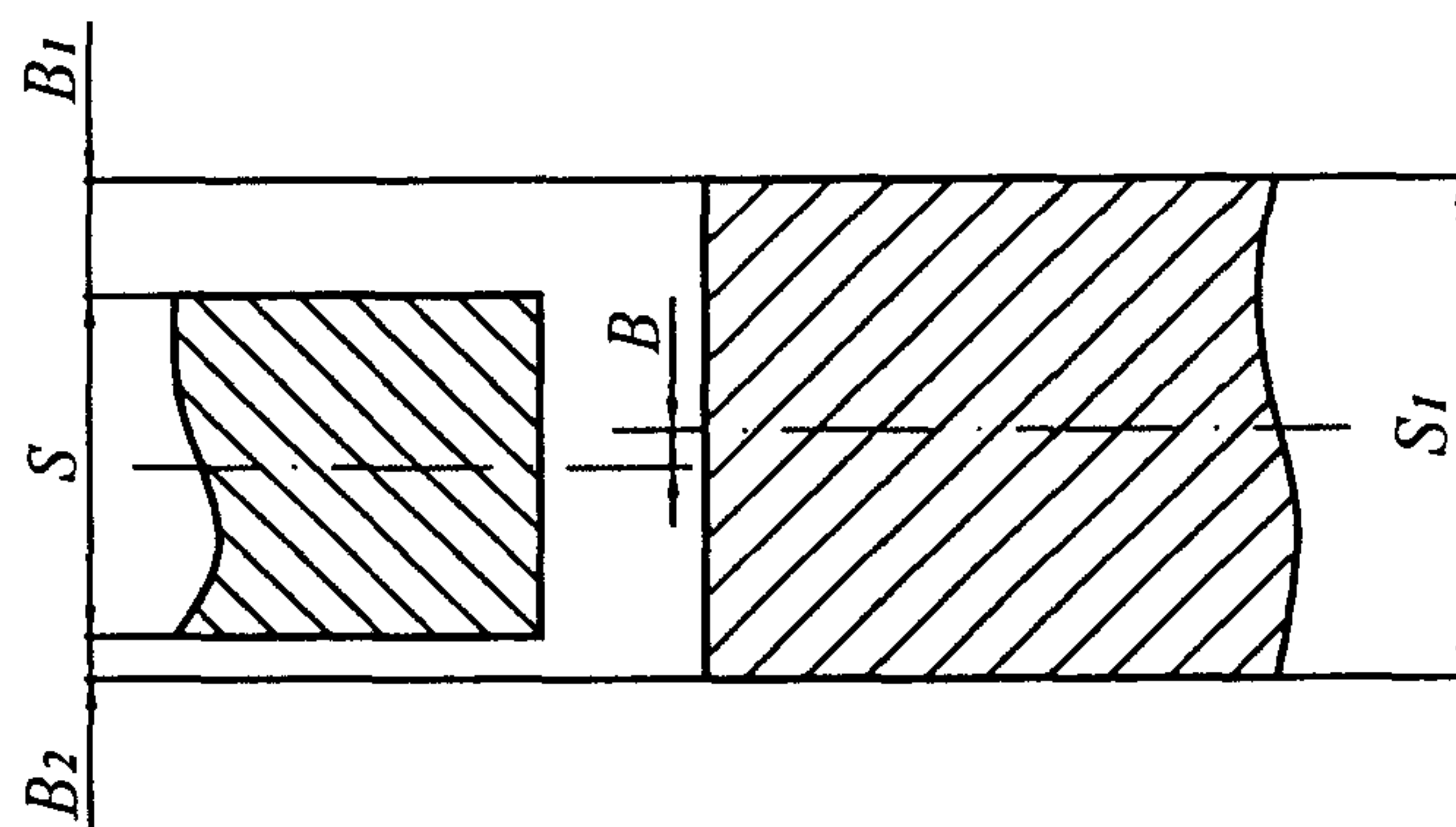
Рисунок 17 – Смещение кромок
