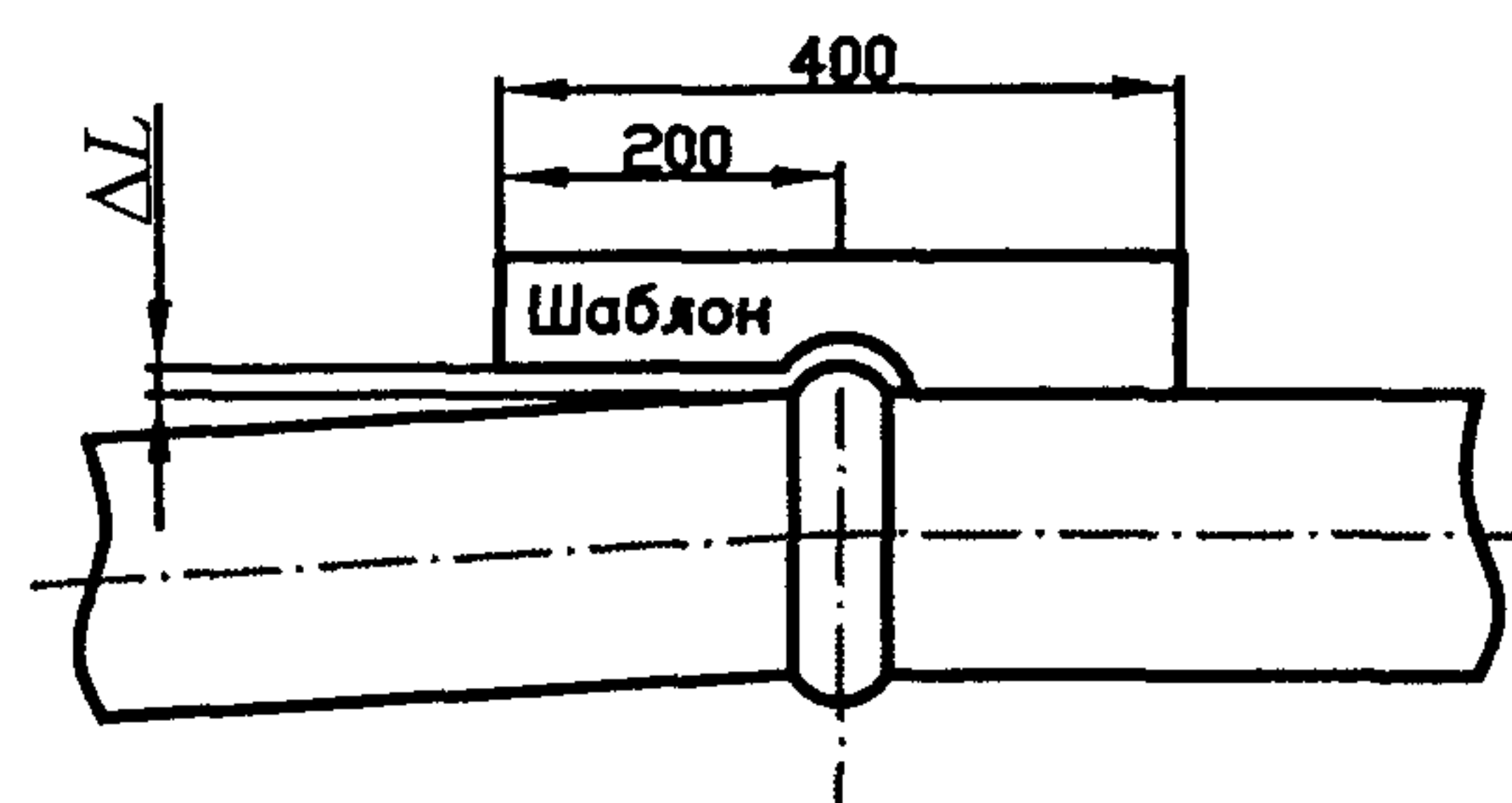
Рисунок 12 – Схема определения отклонения от прямолинейности оси трубы
