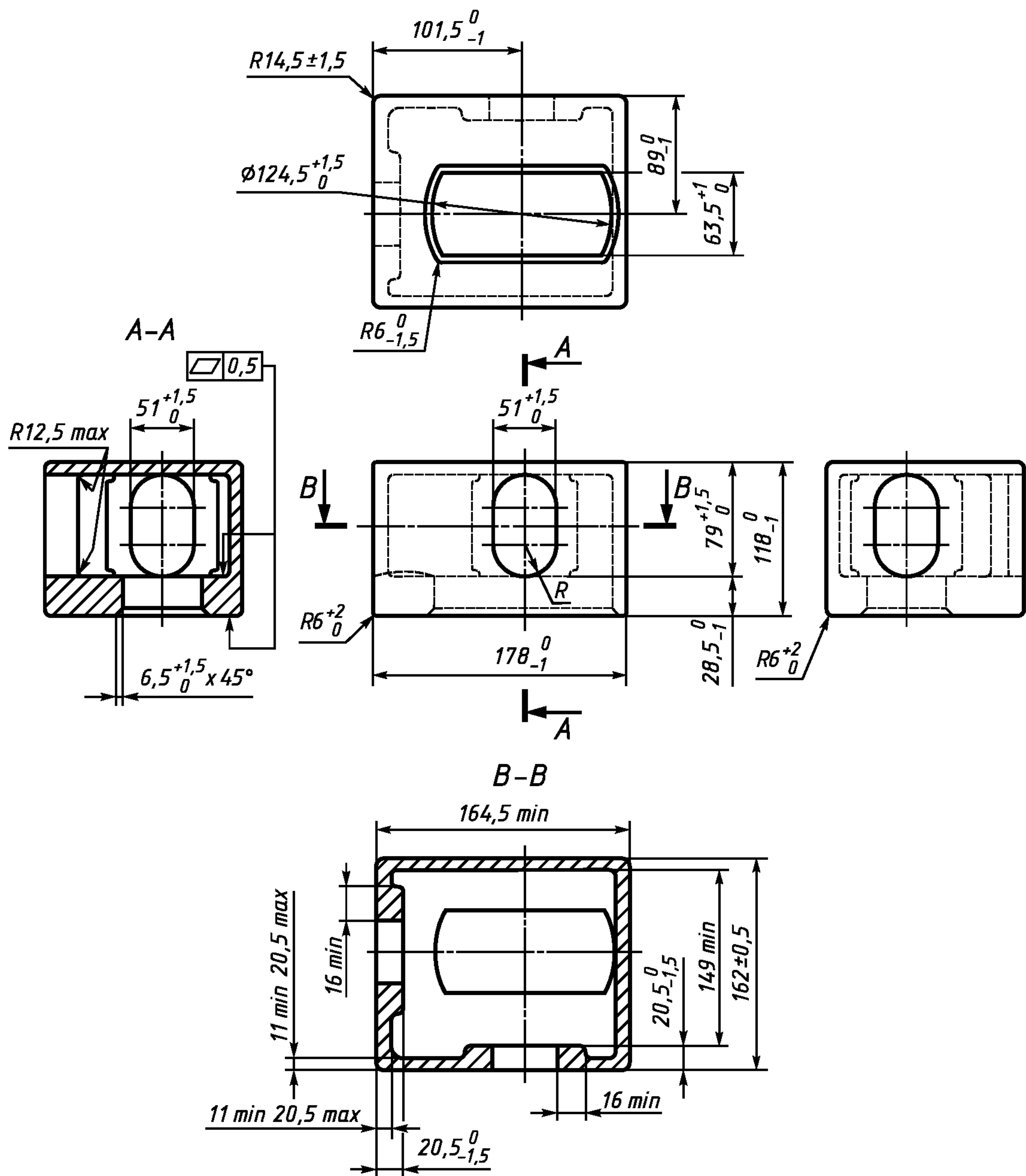
Рисунок 4 — Нижний промежуточный фитинг
