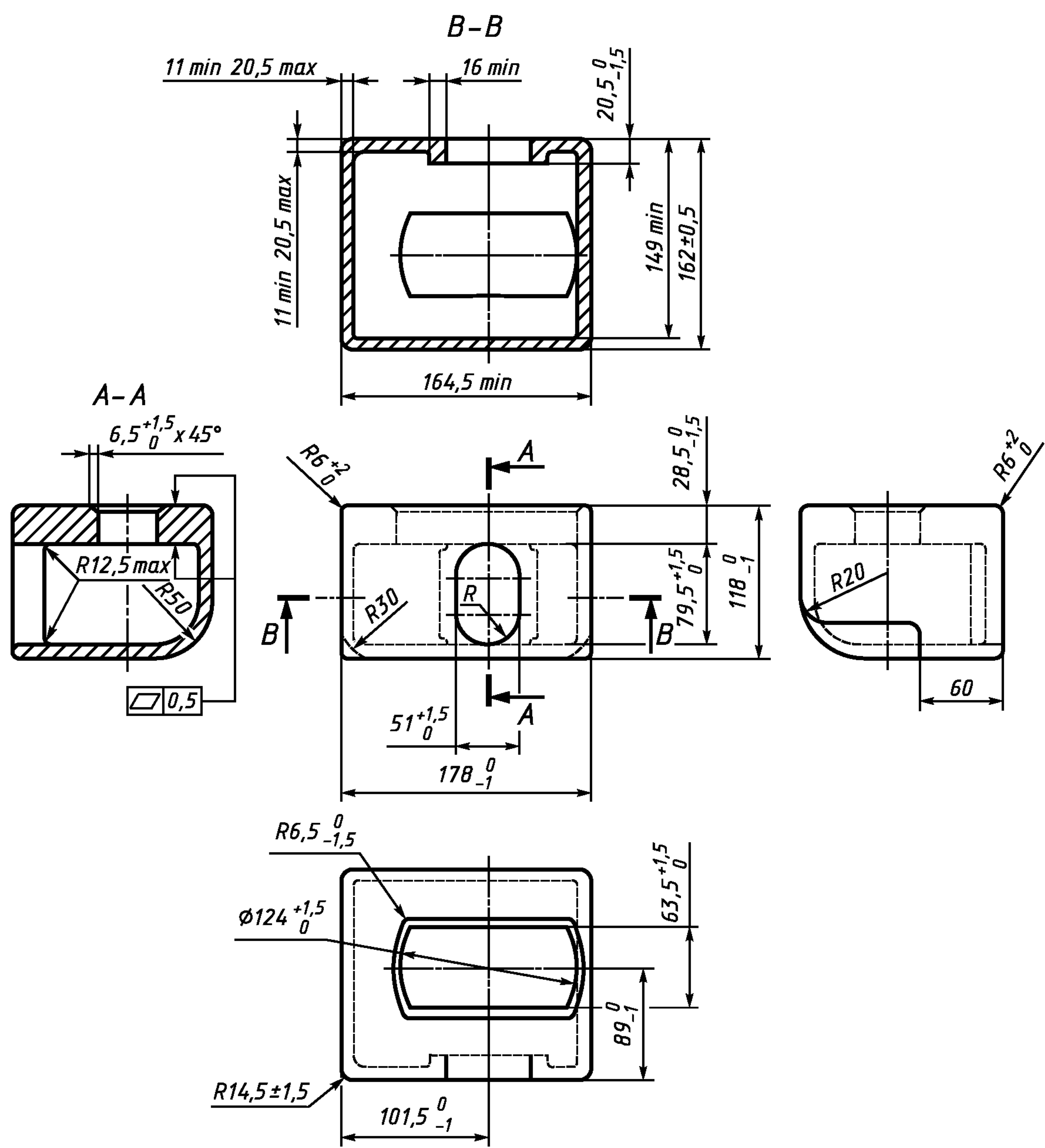
Рисунок 3 — Верхний промежуточный фитинг
