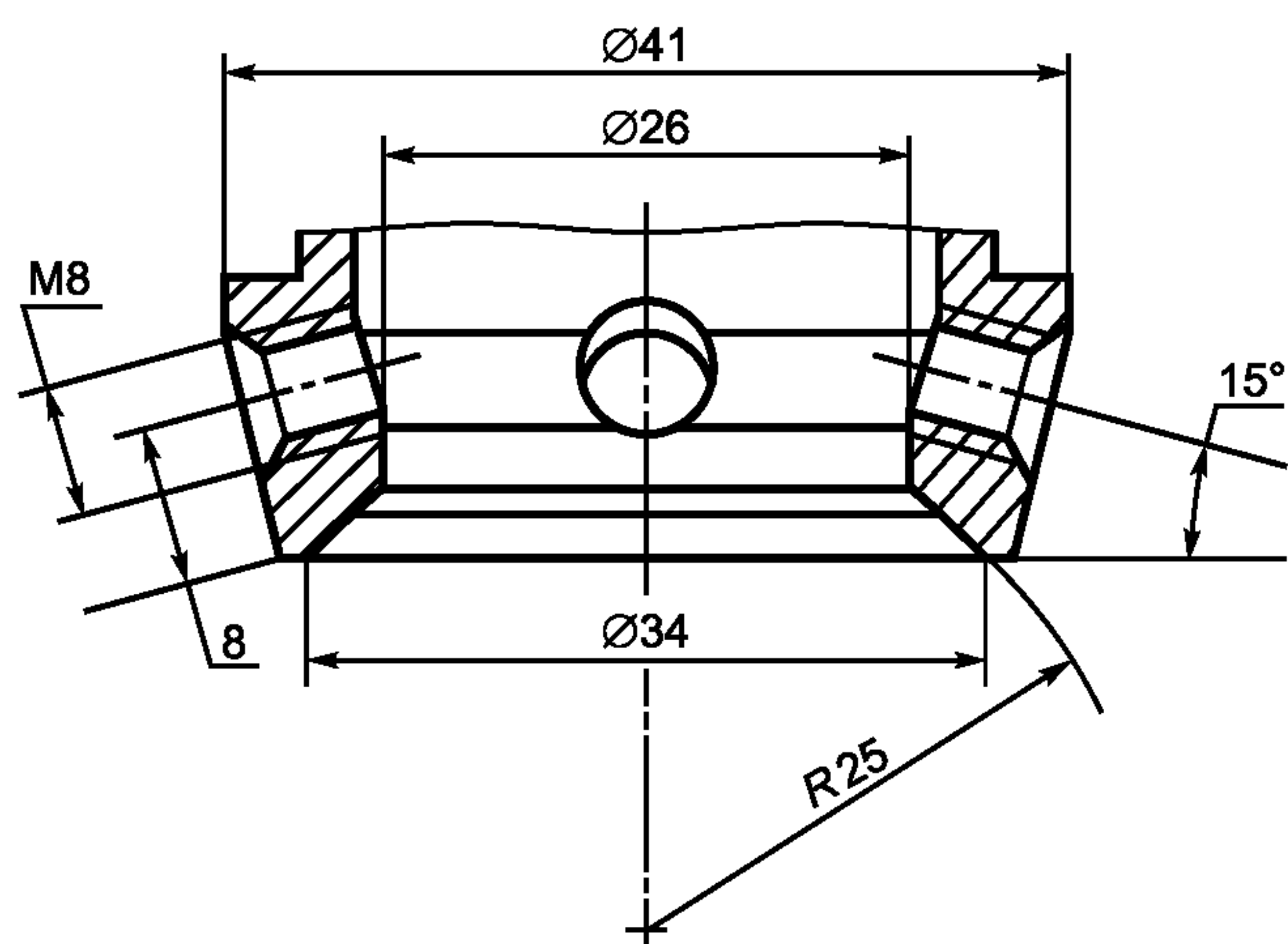
Рисунок А.1 — Гнездо элемента присоединения
