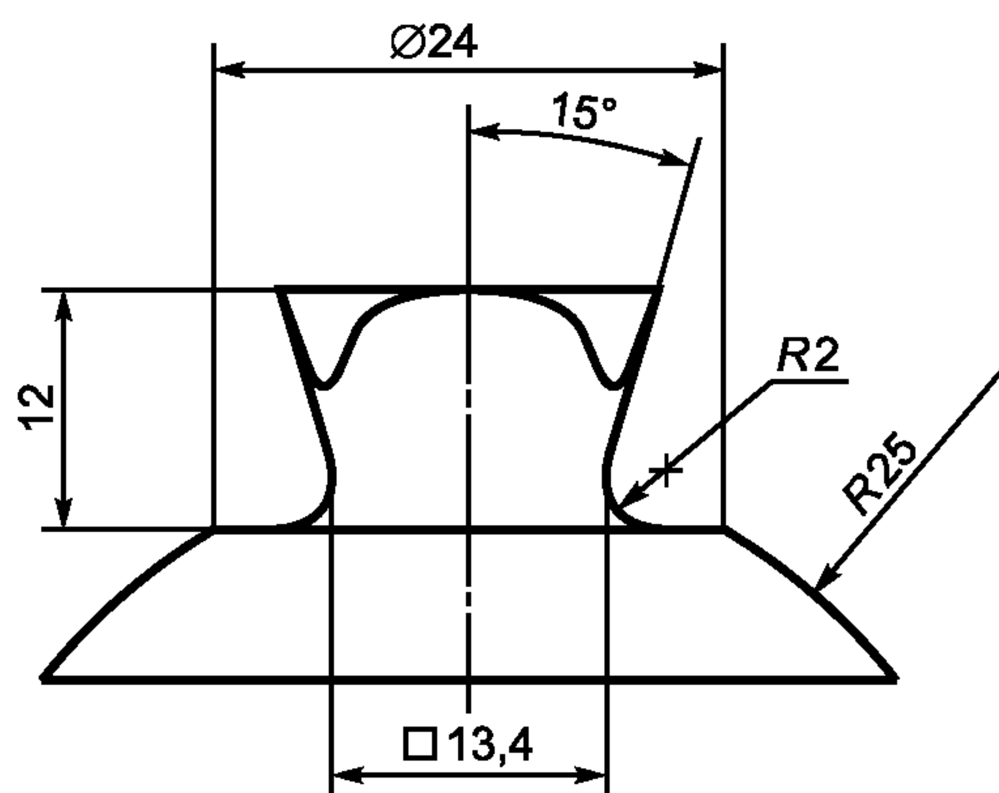
Рисунок А.2 — Пирамидка элемента присоединения
