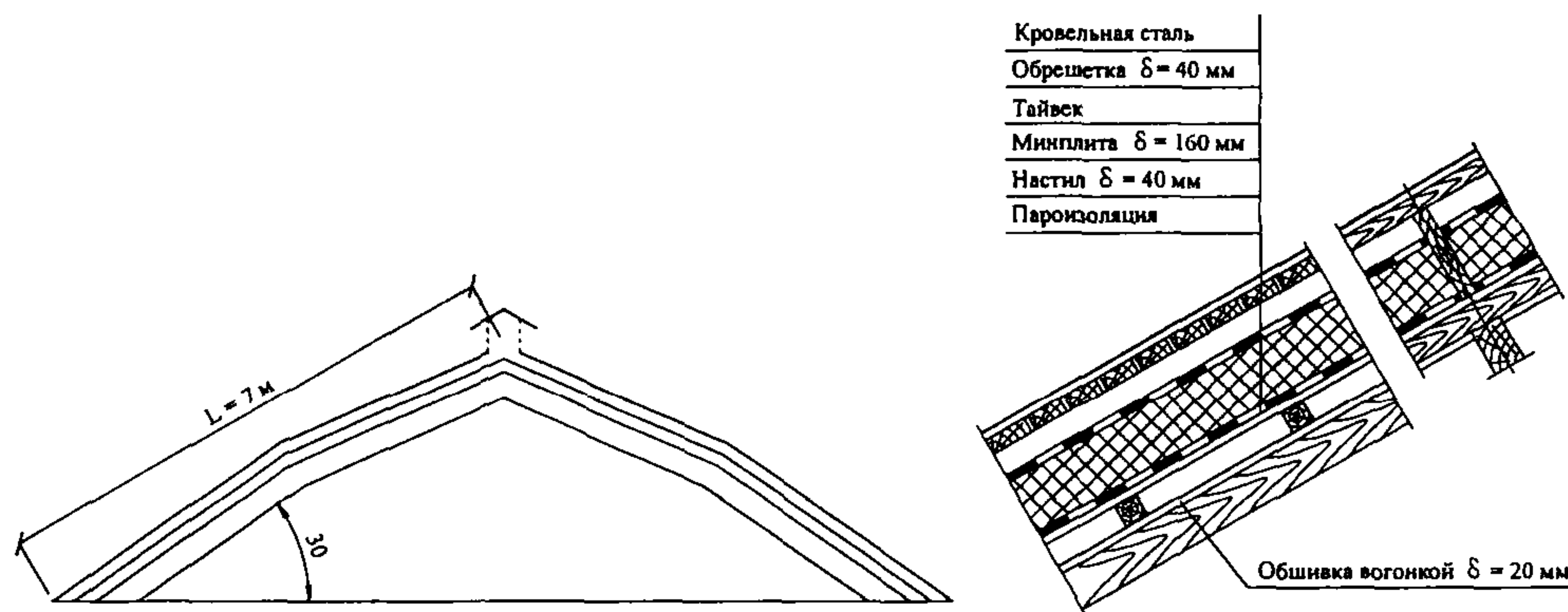
Рис. Конструктивное решение покрытия мансарды
