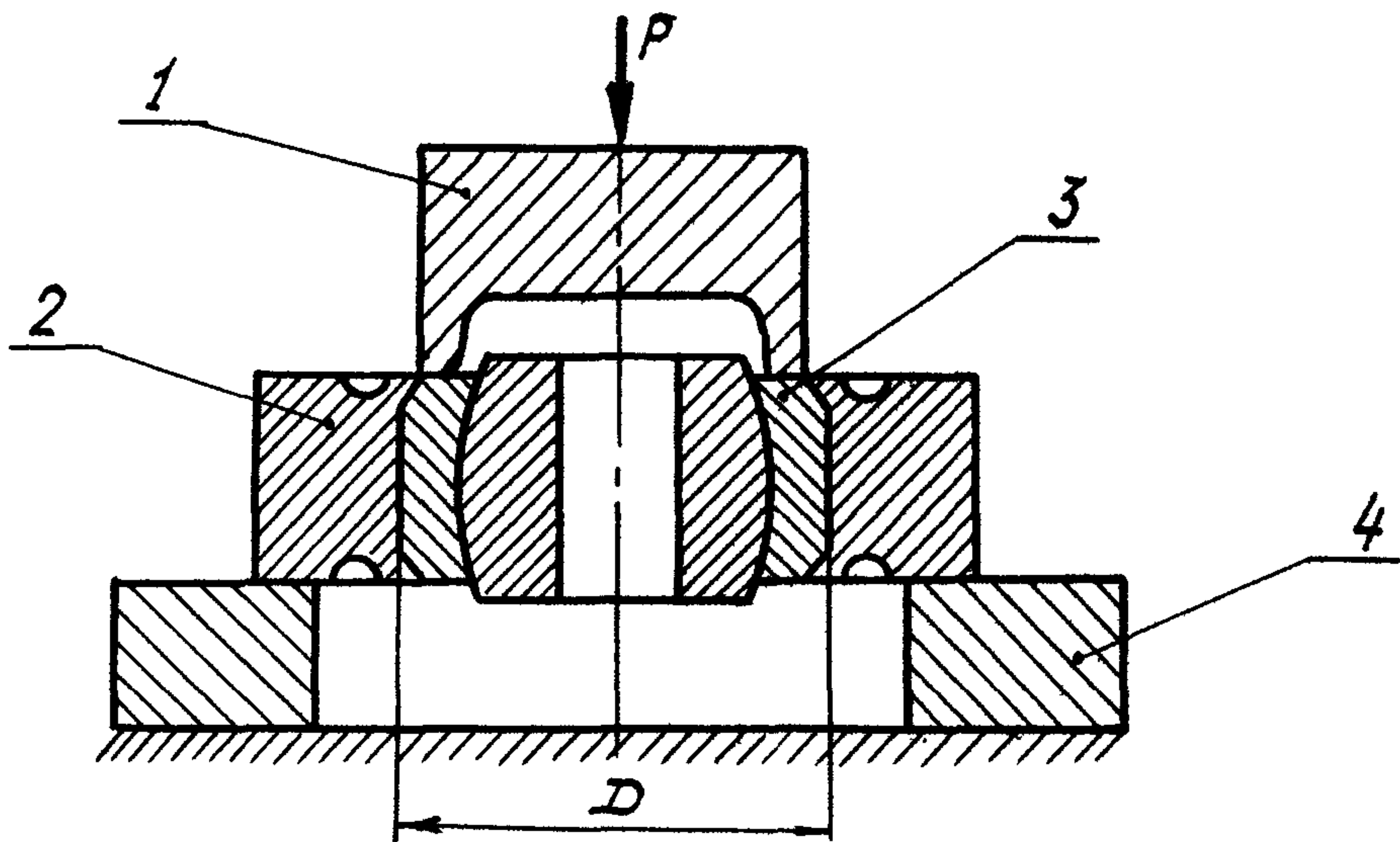
1 - пуансон; 2 - деталь под заделку подшипника; 3 - подшипник; 4 - плита
