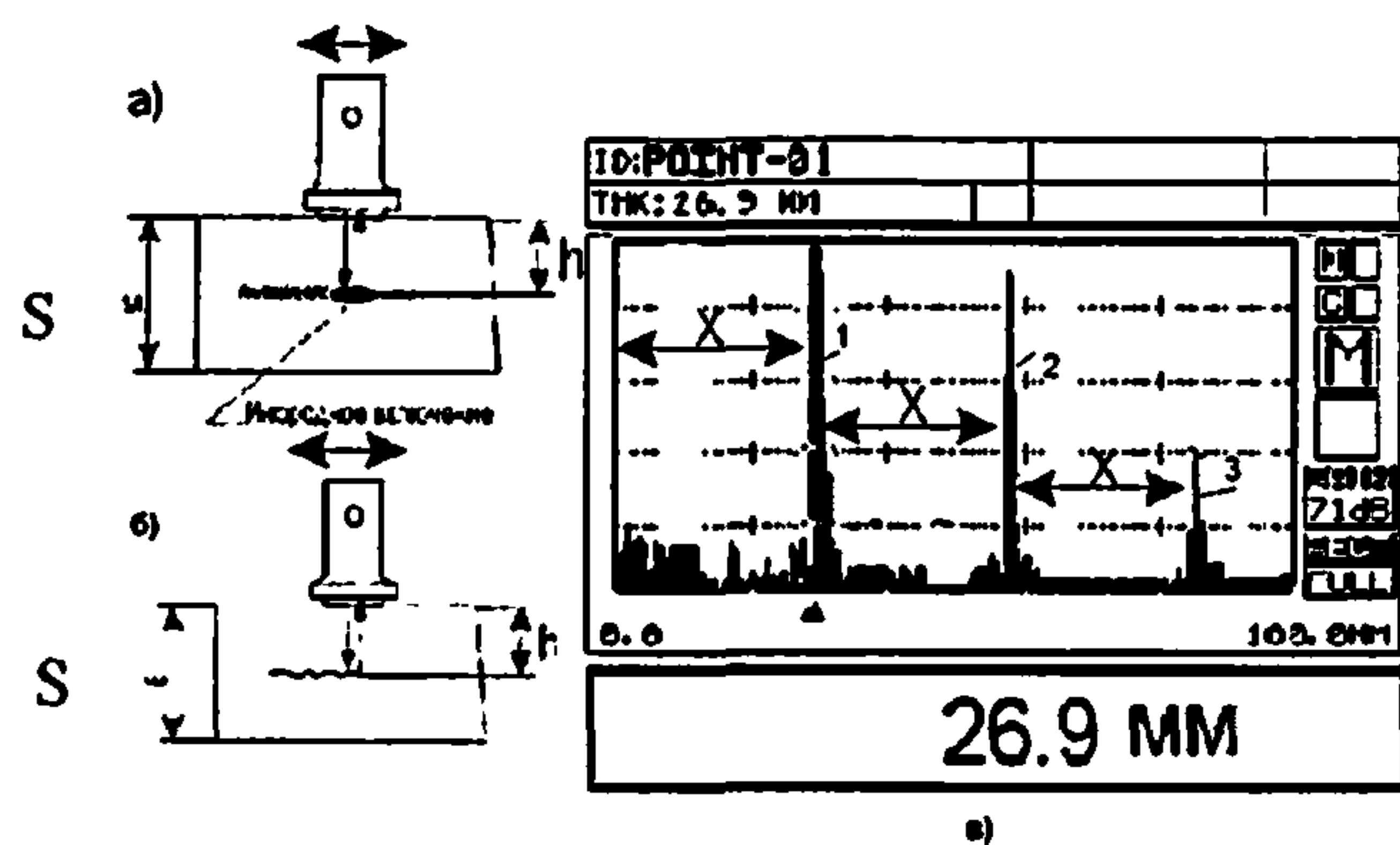
Рисунок Д.1 - Схема прозвучивания (а) и изображение на экране прибора (б) при наличии «полупрозрачных» строчечных дефектов
