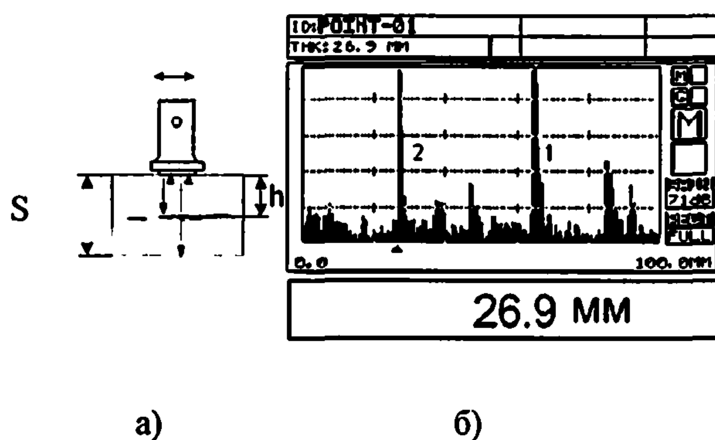
S - толщина элемента; h - расстояние до дефекта; 1 - донный импульс; 2 - эхо-сигнал от «полупрозрачного» дефекта.
