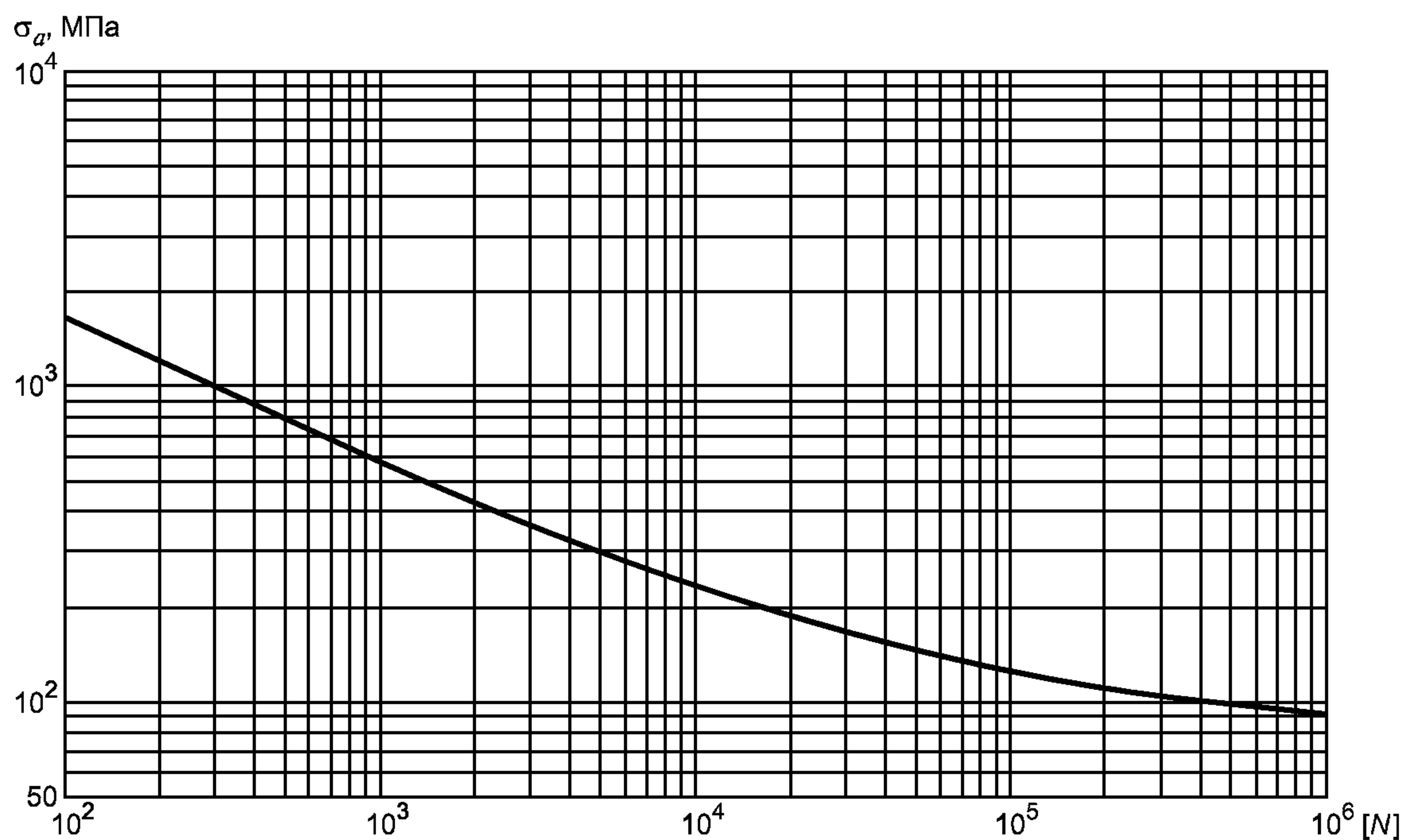
Рисунок 2 — Расчетная кривая усталости для углеродистых сталей (при A = 0,6 \cdot 10^5 МПа, B = 150 МПа, T = 380 °C)
