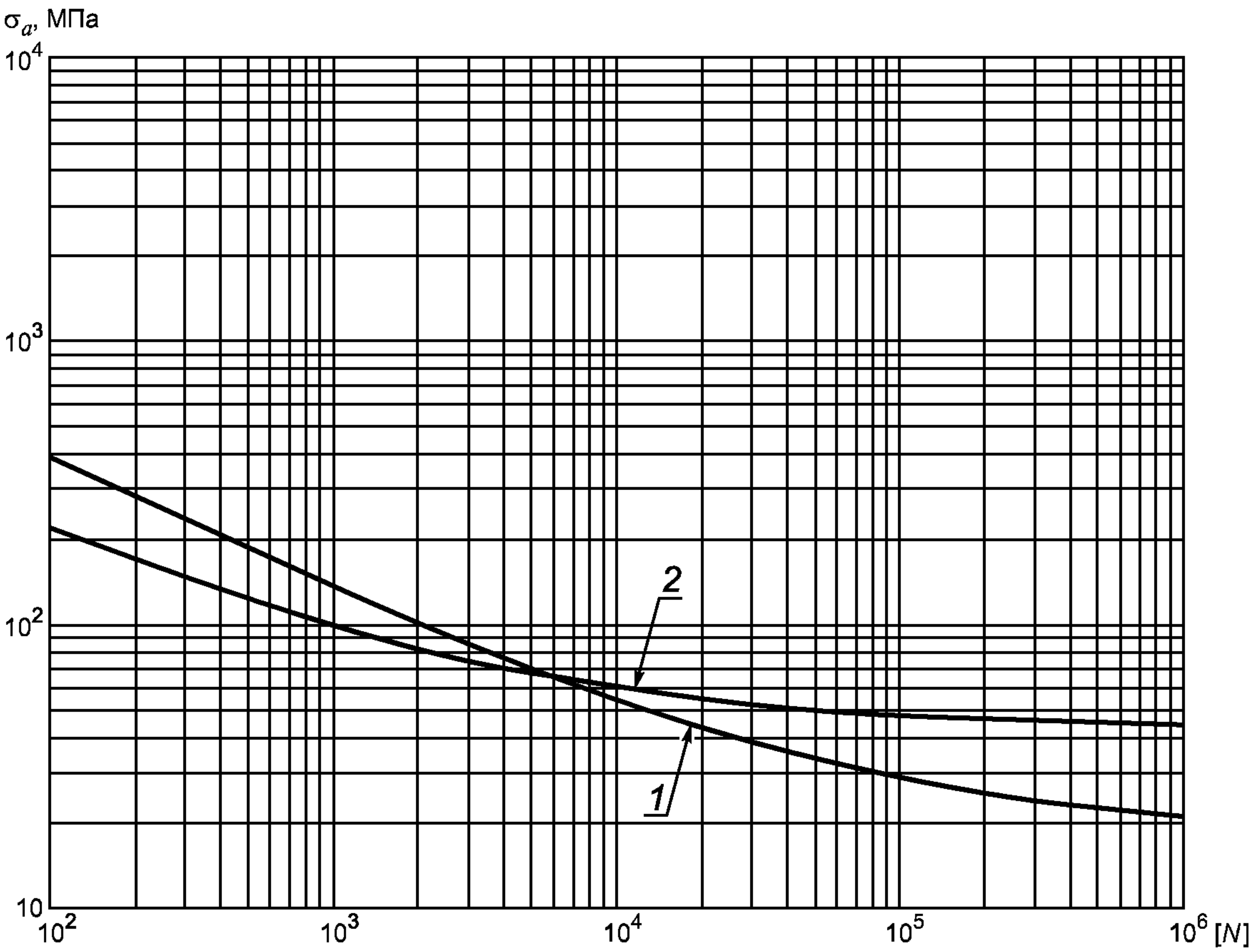
1 — АМцС, АМг2, АМг3 при A = 0,18 \cdot 10^5 МПа, B = 34 МПа, T = 150 °C; 2 — АМг5, АМг6 при A = 0,86 \cdot 10^5 МПа, B = 84 МПа, T = 150 °C
