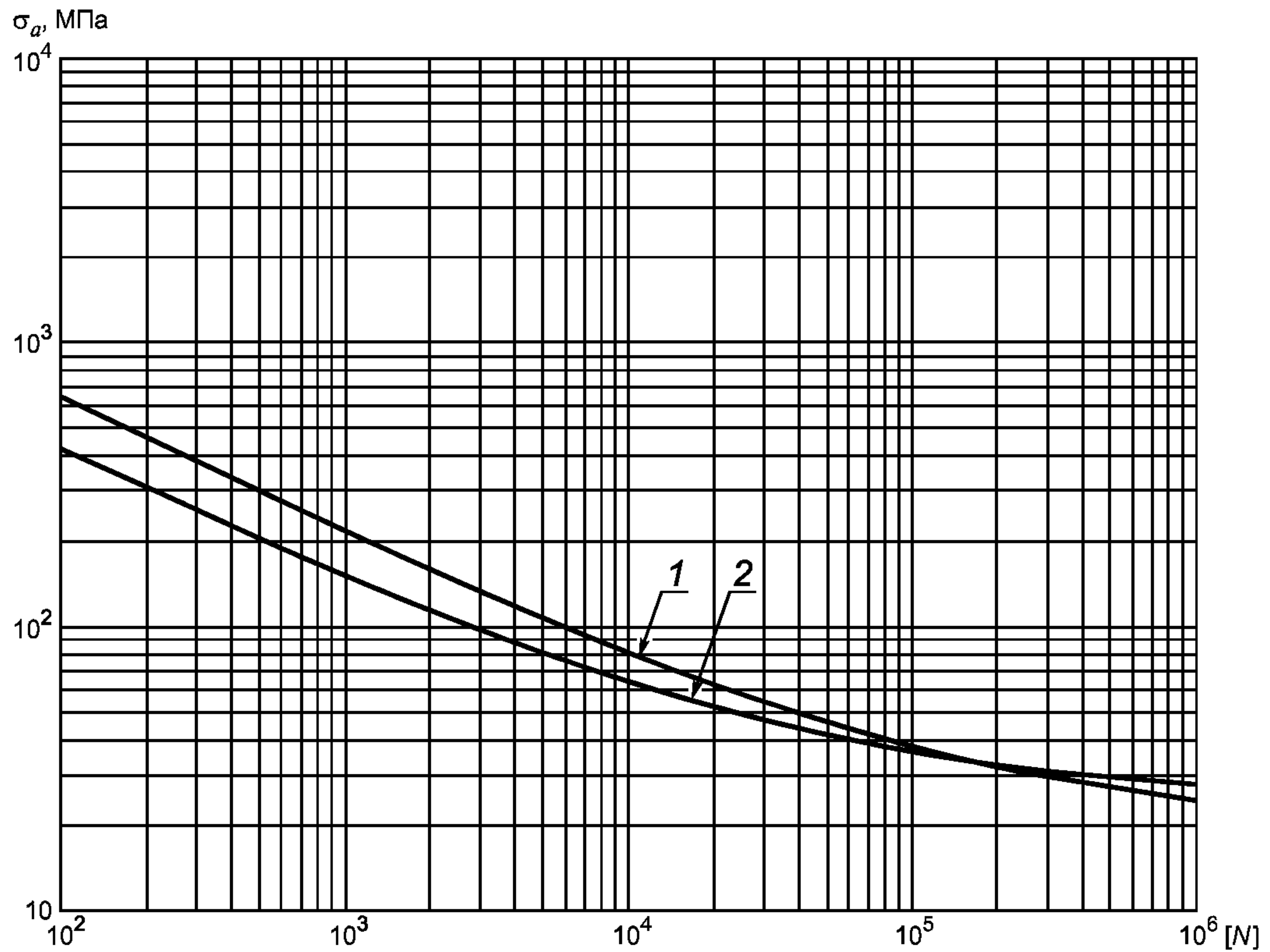
Рисунок 7 — Расчетная кривая усталости для сплавов меди
