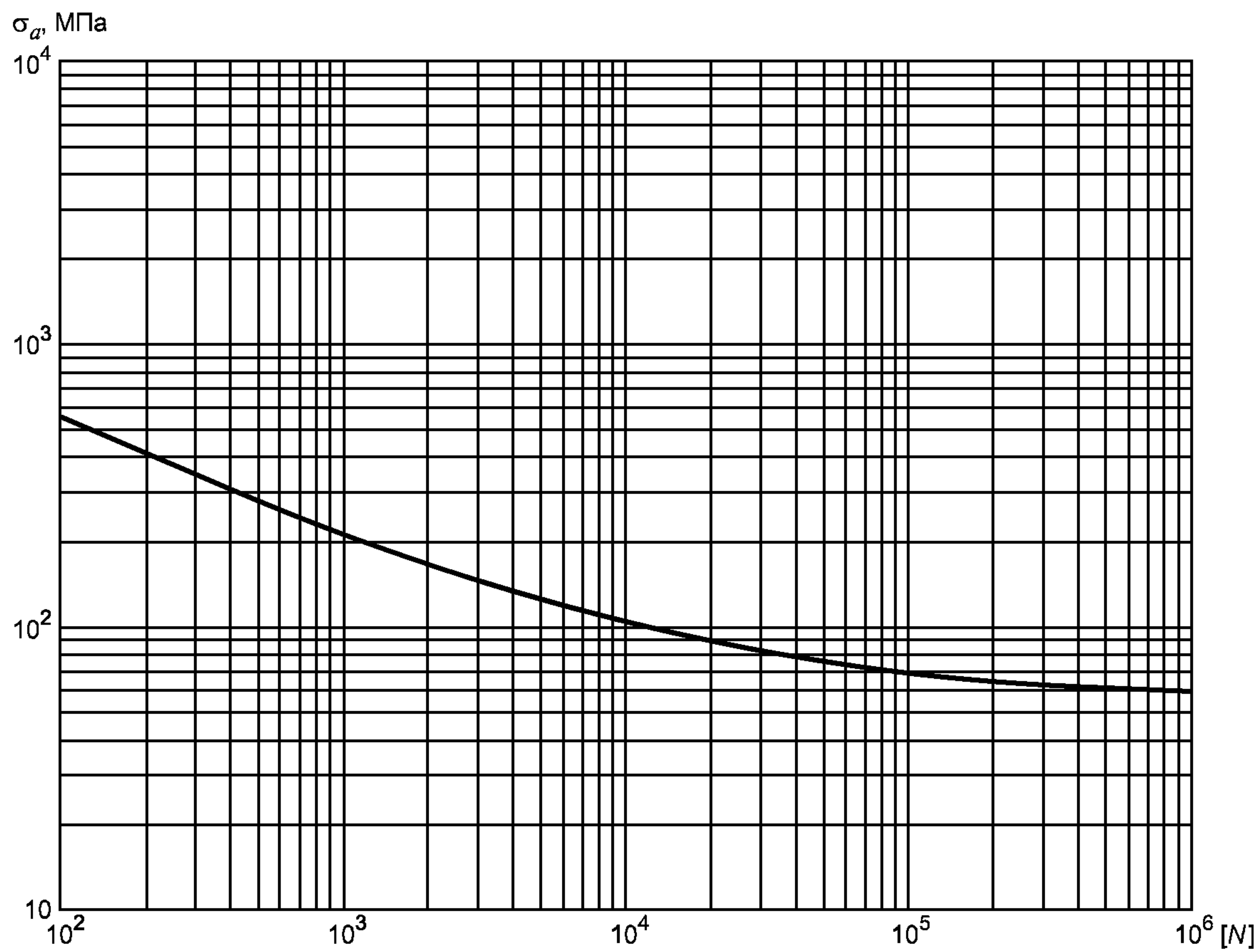
Рисунок 9 — Расчетная кривая усталости для сплава титана АТ3 (при A = 0,31 \cdot 10^5 МПа, B = 133,6 МПа, T = 350 °C)
