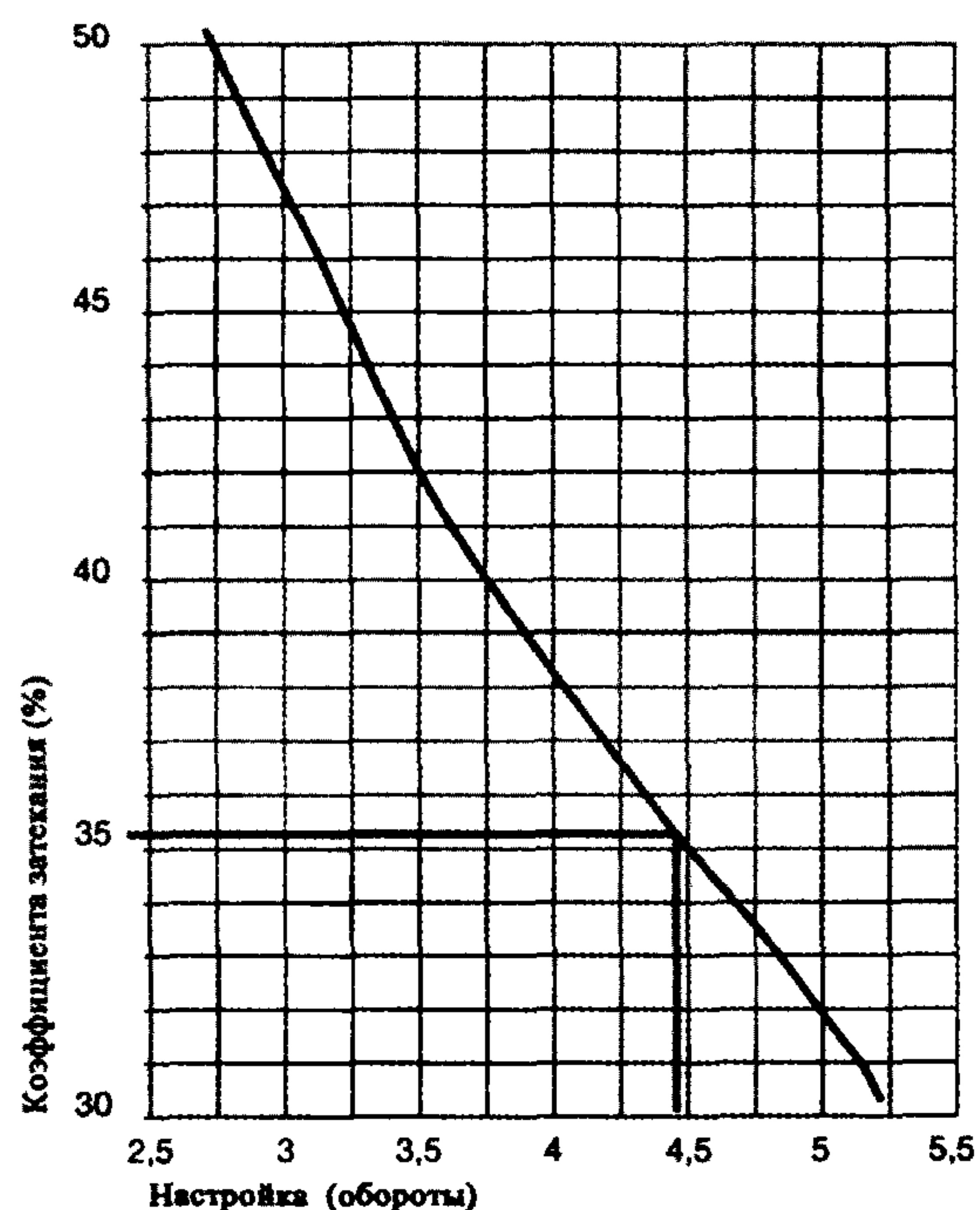
Рис. 2.7. Линия настройки Н-образного клапана «Vekolux»
