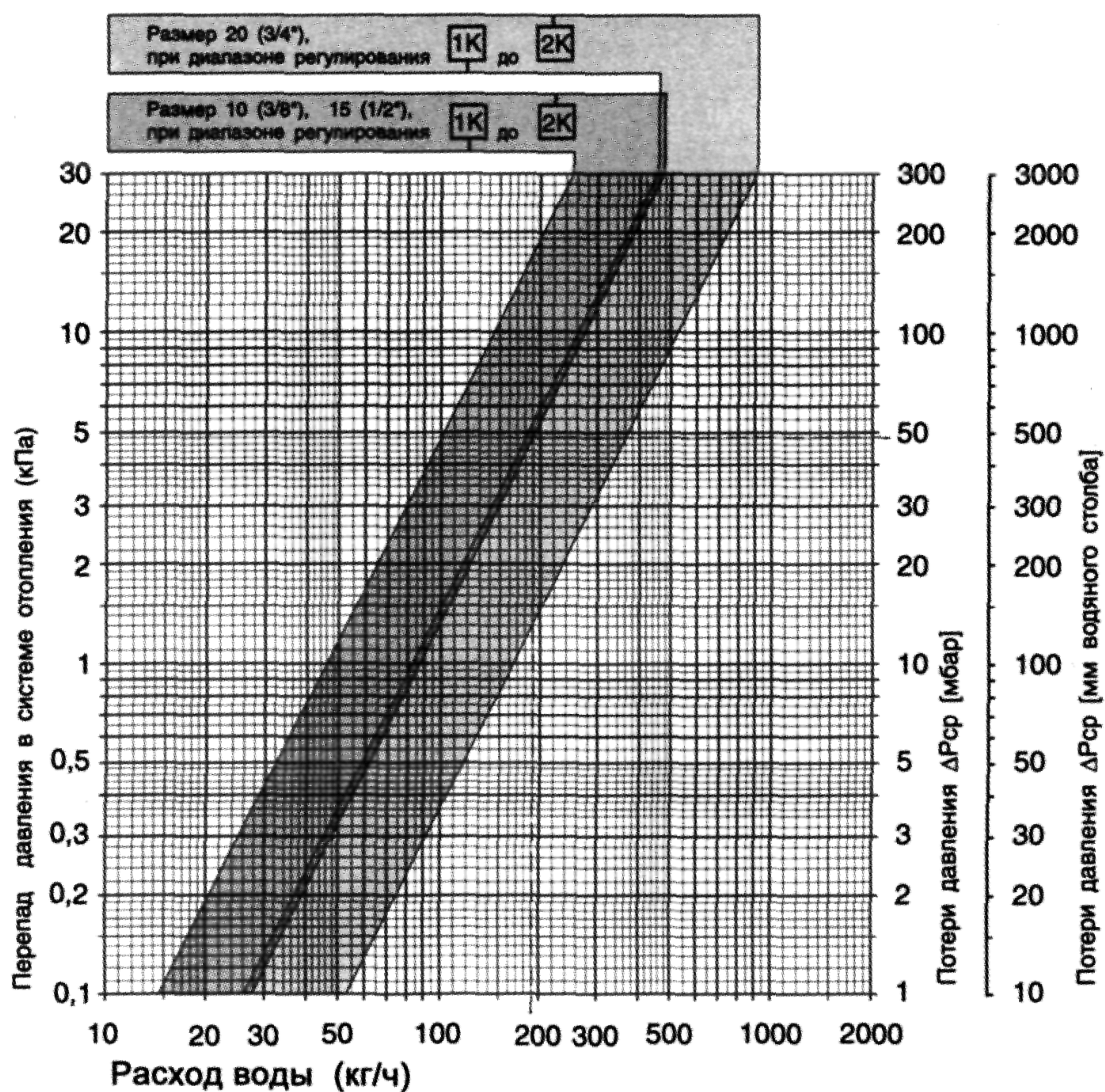
Рис. 2.4. Гидравлические характеристики термостатов «Super» фирмы «Heimeier»
