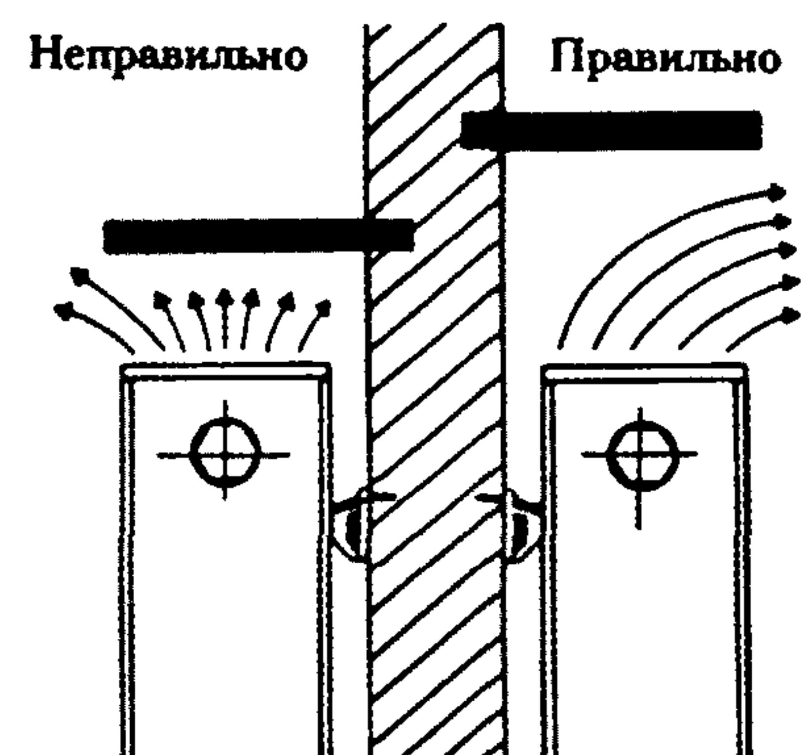
Рис. 5.4. Схемы установки радиатора под подоконником
