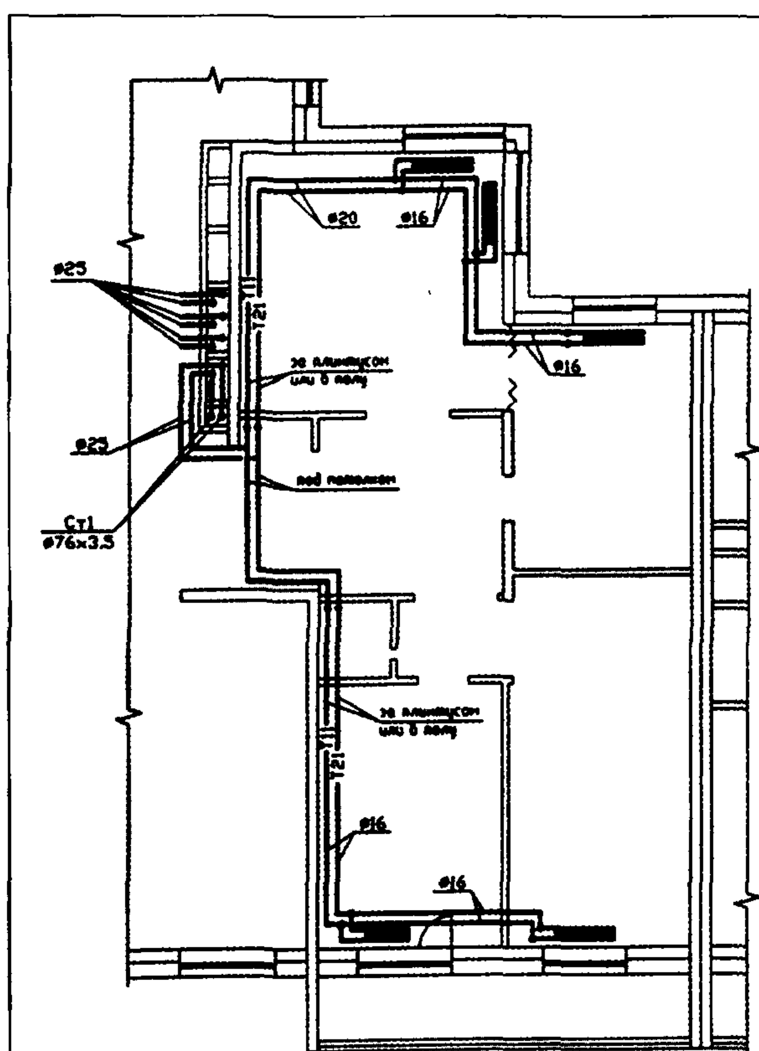
Рис. 1.6. Двухтрубная система отопления с периметральной (плинтусной) разводкой теплопроводов по квартире
