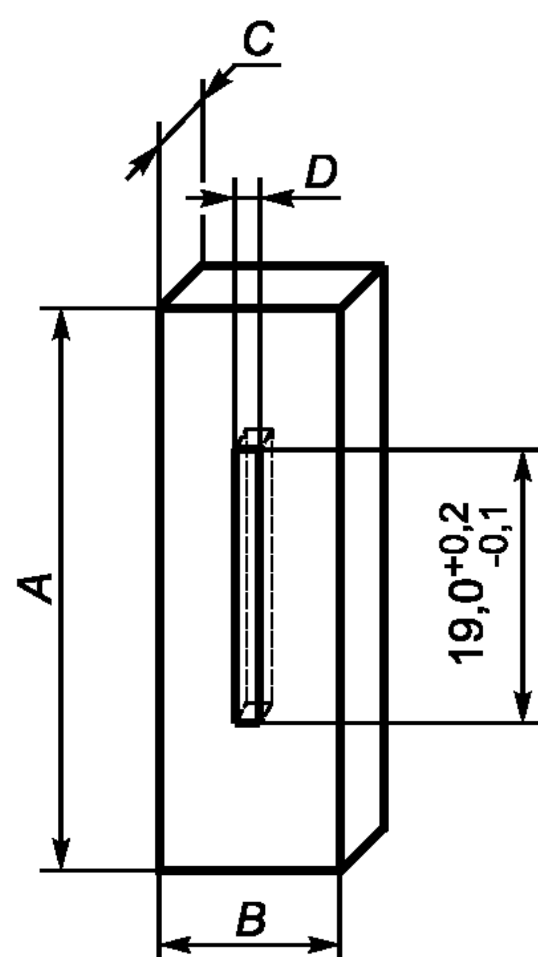
Рисунок 7 — Образец с надрезом
