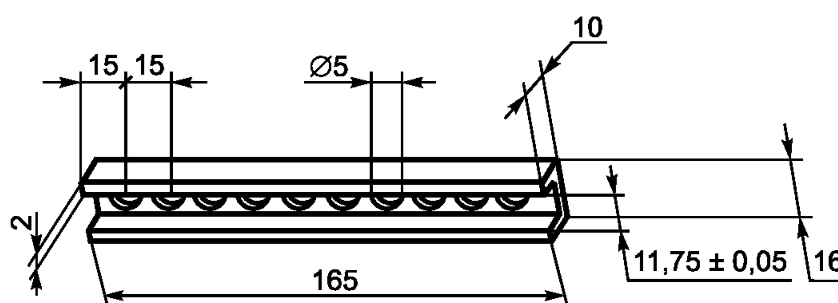
Размер (11,75 \pm 0,05) мм является внутренней шириной держателя
