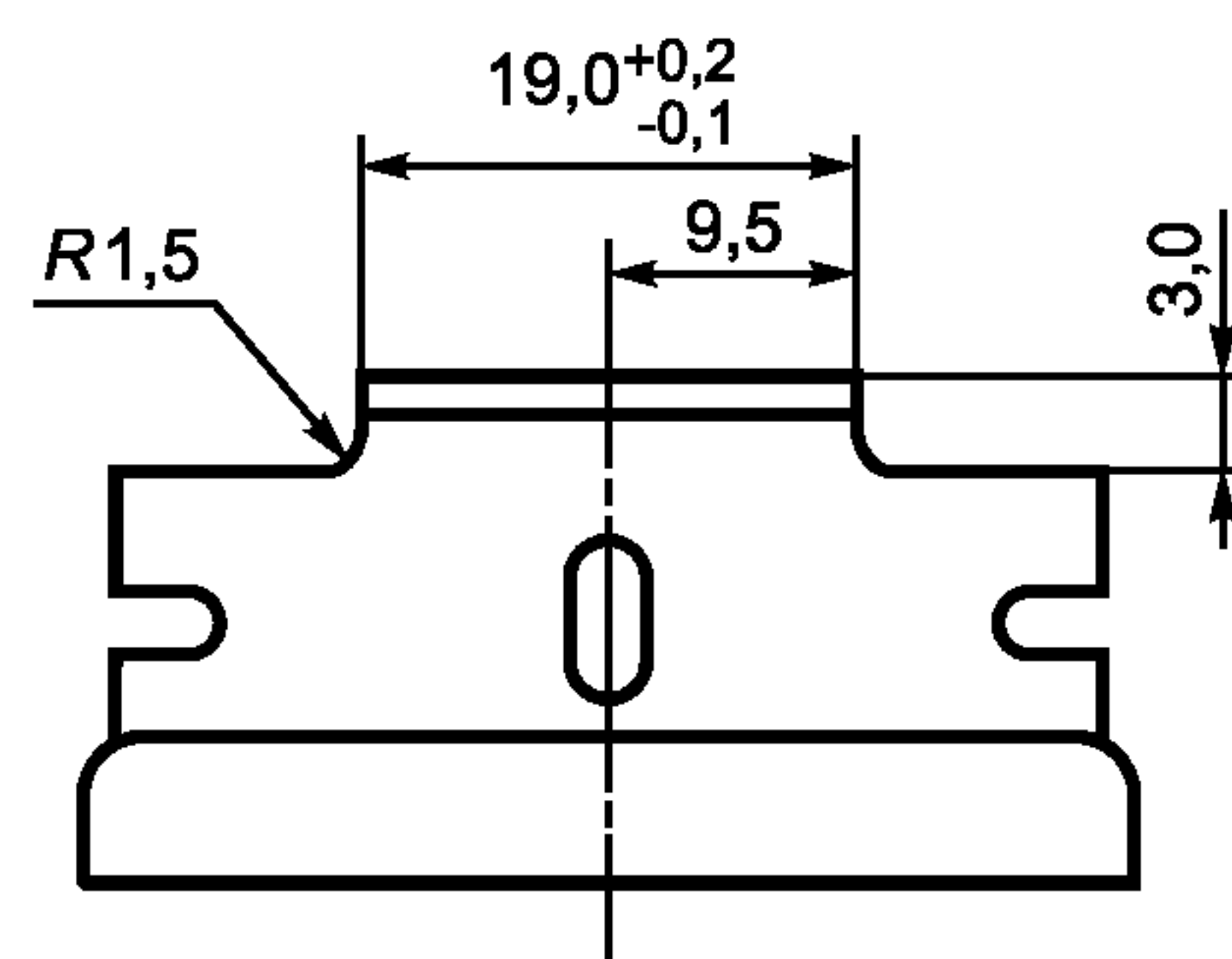
Рисунок 2 — Лезвие
